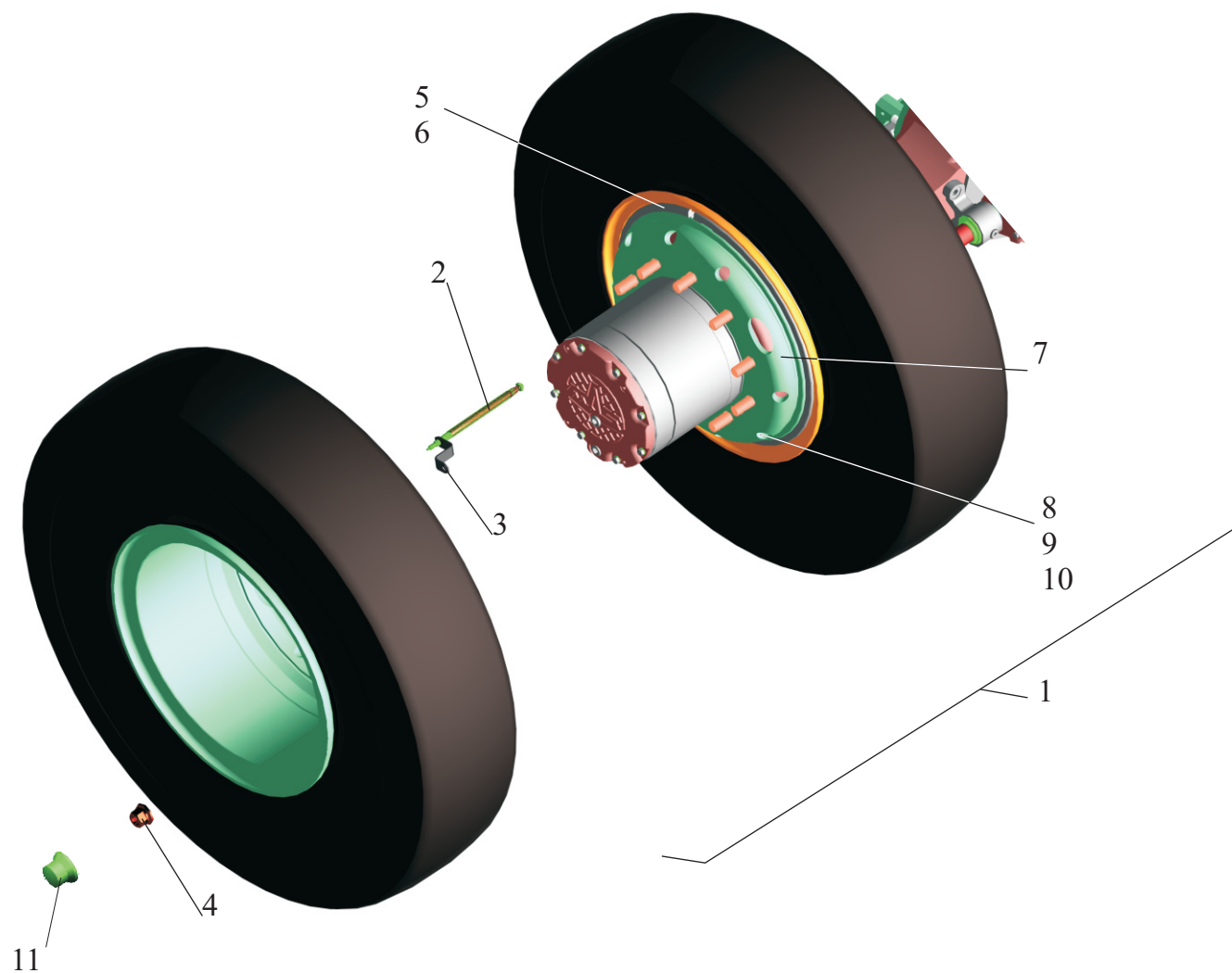
Рис. 24 Установка задних колес 5516-3100002-730, 5516-3100002-030 Fig. 24 Installation rear wheels 5516-3100002-730, 5516-3100002-030
