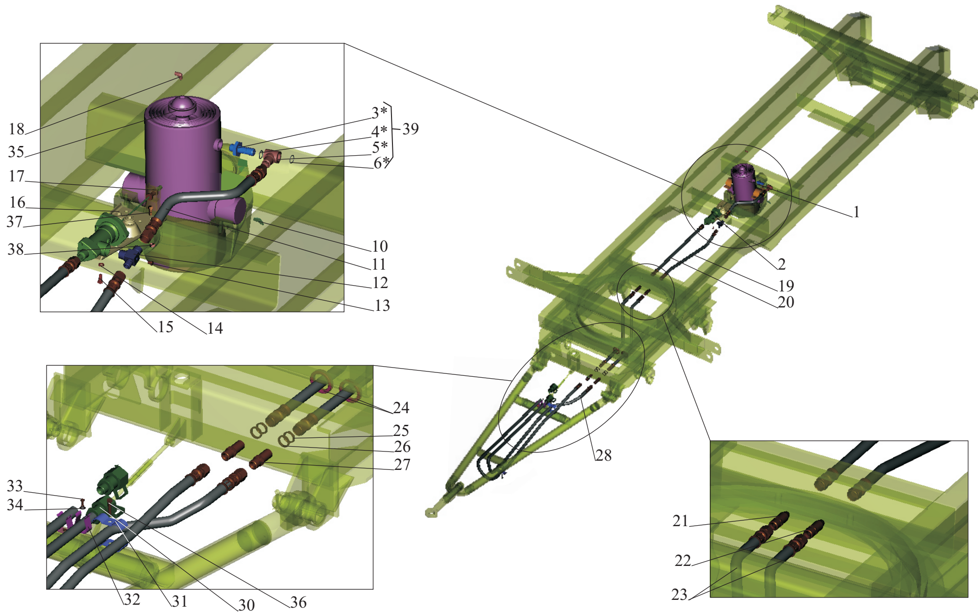
Рис. 56 Установка гидрооборудования 8561-8600005 Fig. 56 Installation of hidroaquipment 8561-8600005
