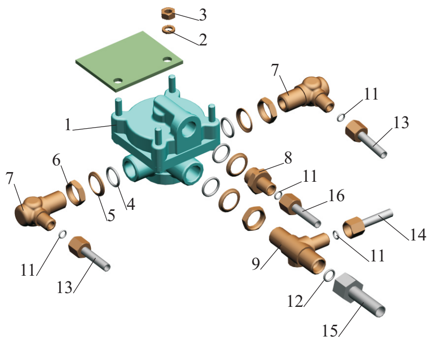
Клапан ускорительный переднего контура Relay valve of front contour
