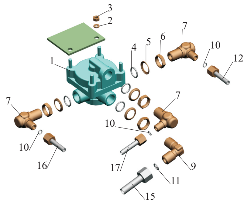
Клапан ускорительный заднего контура Relay valve of rear contour
