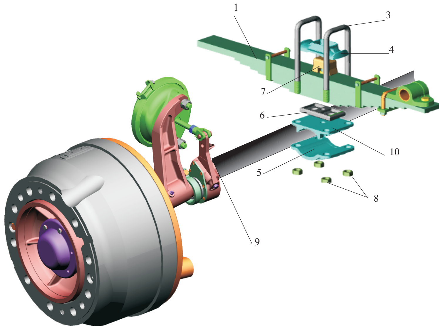
Рис. 15 Ось с рессорами 8571-2410005, 8571-2410005-10 Fig. 15 Axle with springs 8571-2410005, 8571-2410005-10
