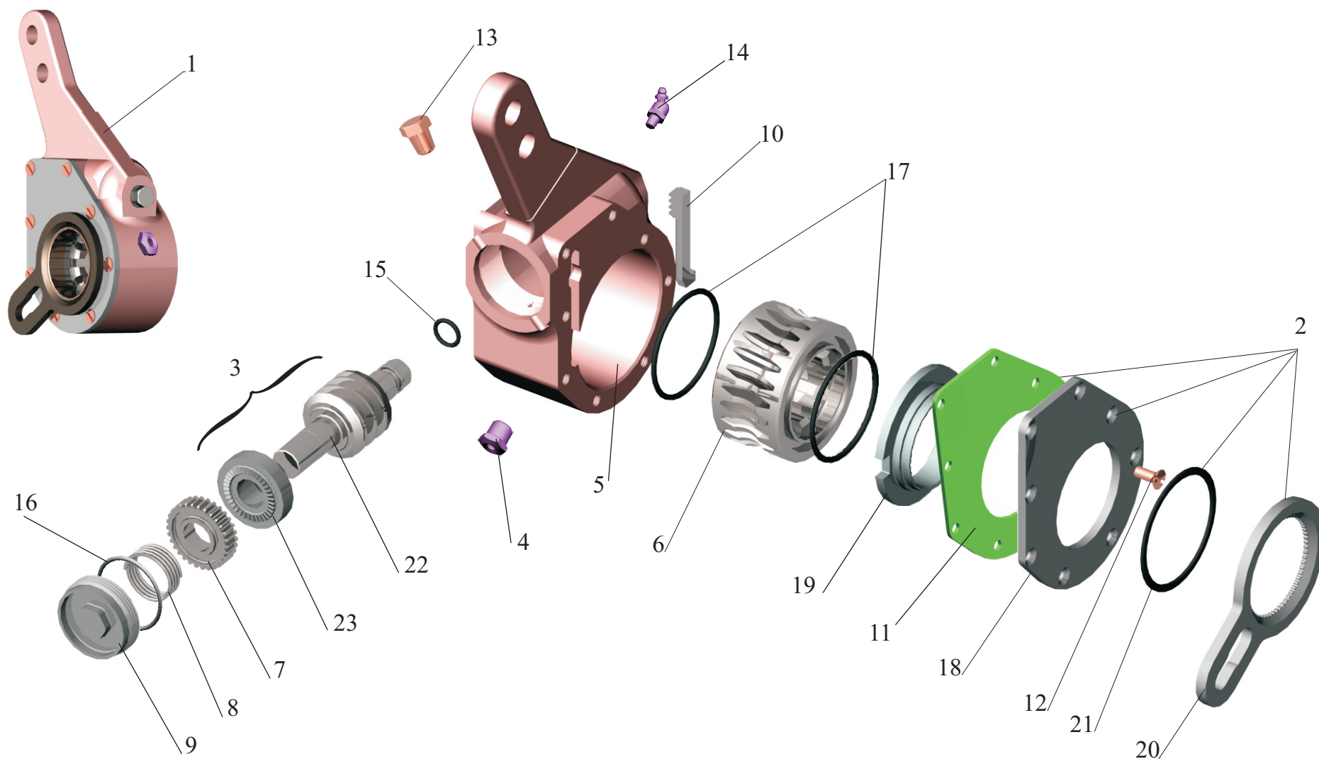
Рис. 12 Рычаг регулировочный 64226-3501136, 64226-3501136-010 Fig. 12 Adjusting lever 64226-3501136, 64226-3501136-010
