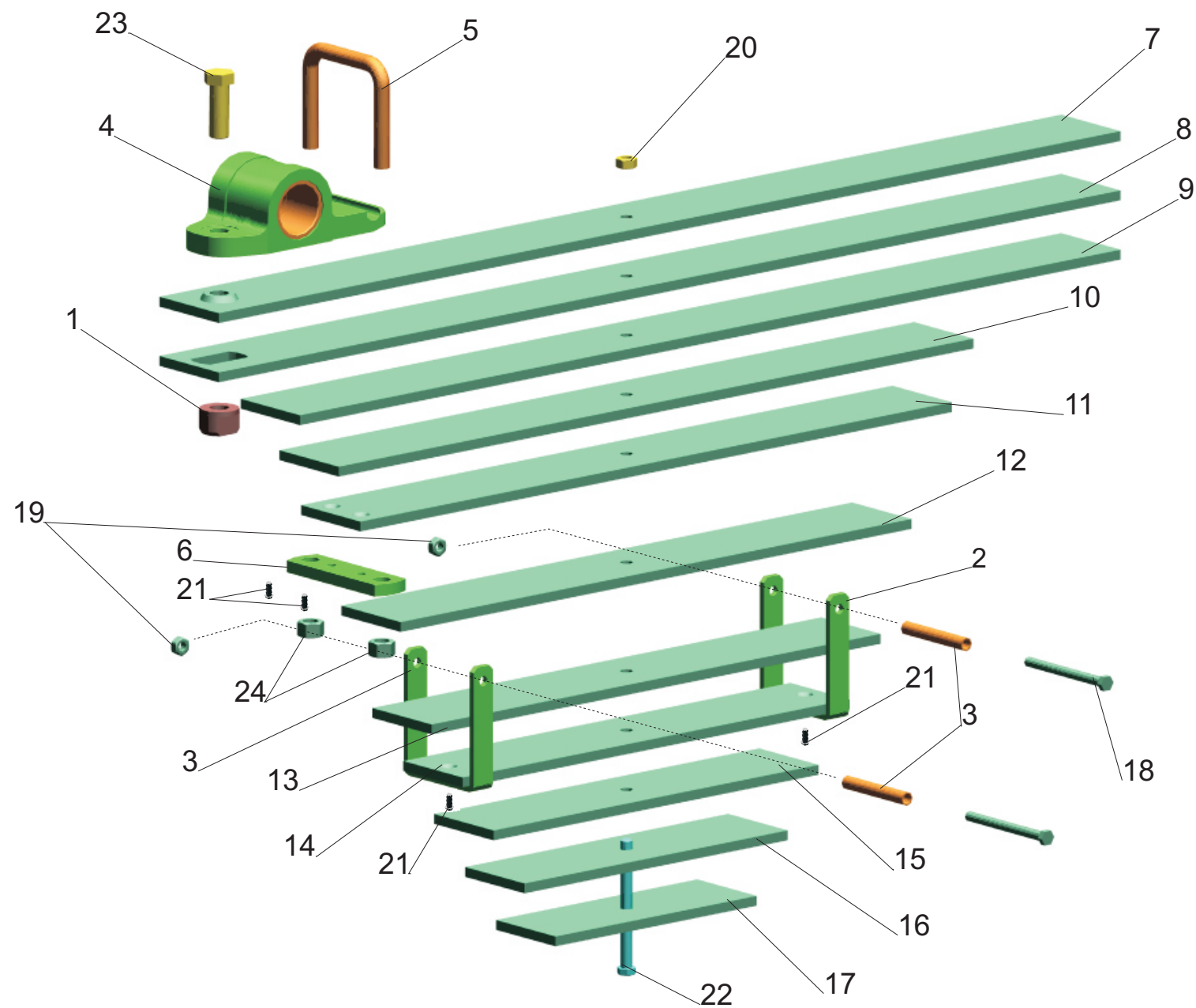
Рис. 18 Рессора 8571-2912012. Fig. 18 Spring 8571-2912012.
