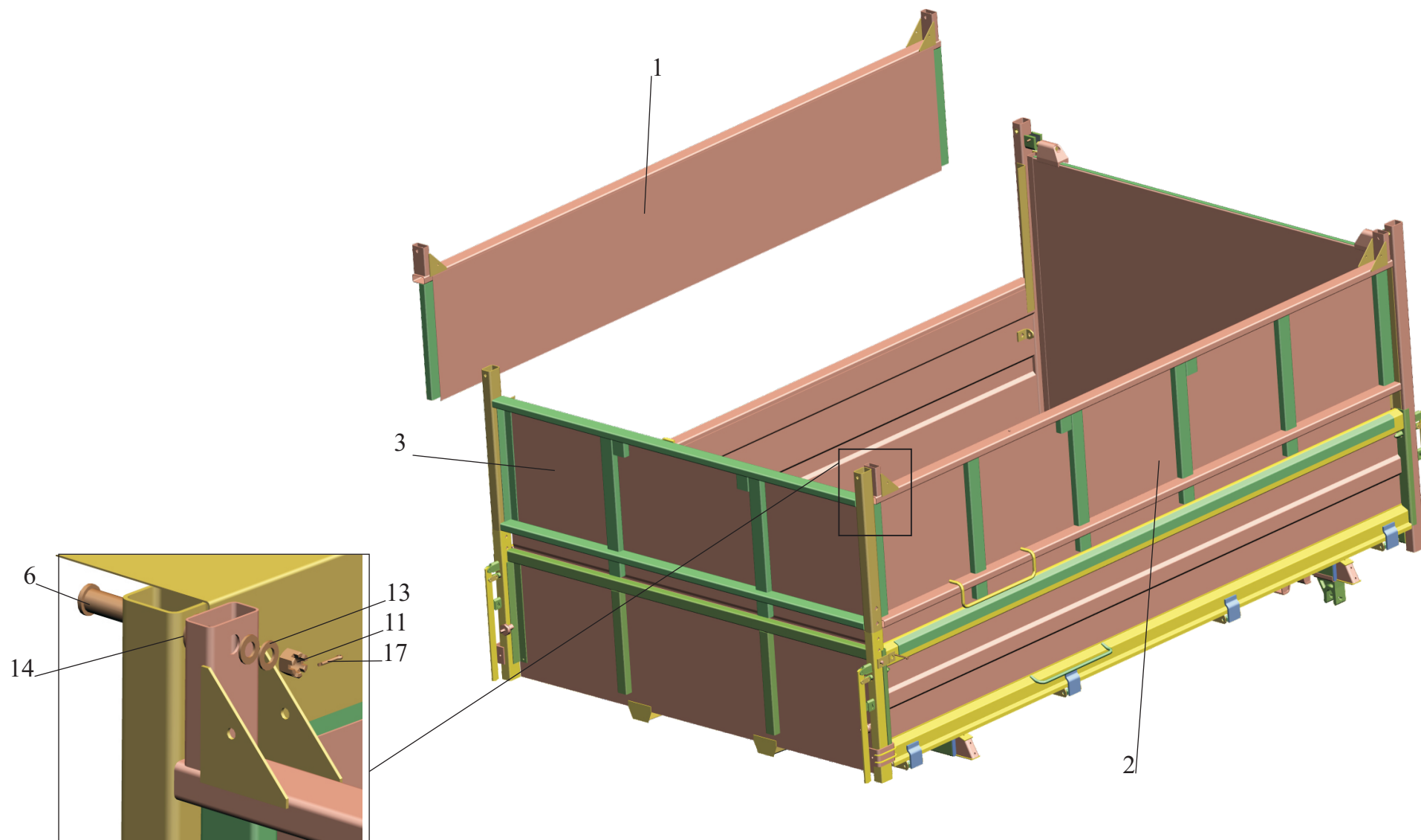
Рис. 51 Установка надставных бортов 8571-8500012-050 Fig. 51 Installation lengthened boards 8571-8500012-050
