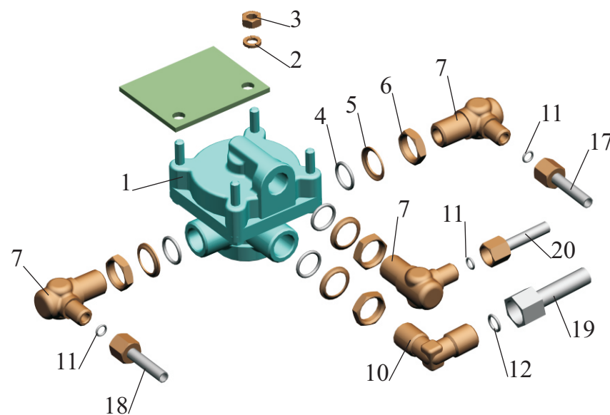
Клапан ускорительный заднего контура Relay valve of rear contour
