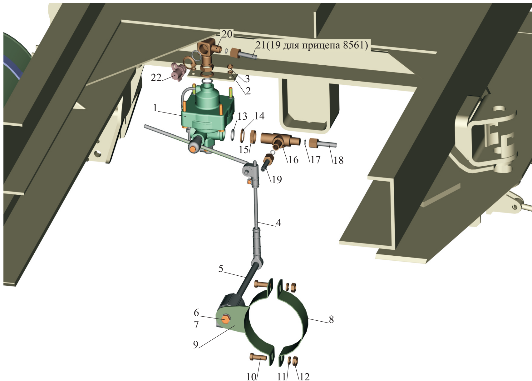
Рис. 31 Установка регулятора тормозных сил и соединительной арматуры Fig. 31 Installation of brake force regulator and attach accessories
