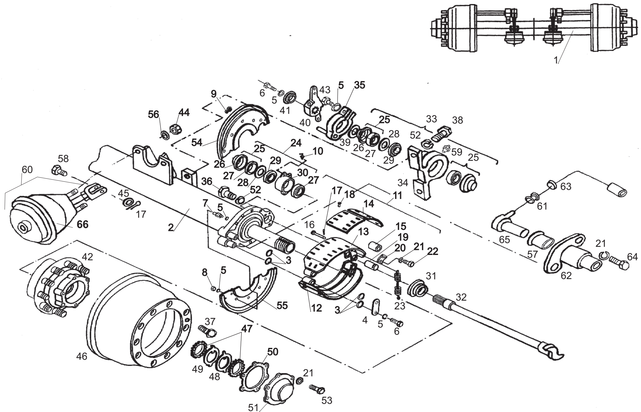
Рис. 10 Оси колес с тормозами 8561-2410008-010, 8561-2410007-010 Fig. 10 Axle of wheels with brake 8561-2410008-010, 8561-2410007-010
