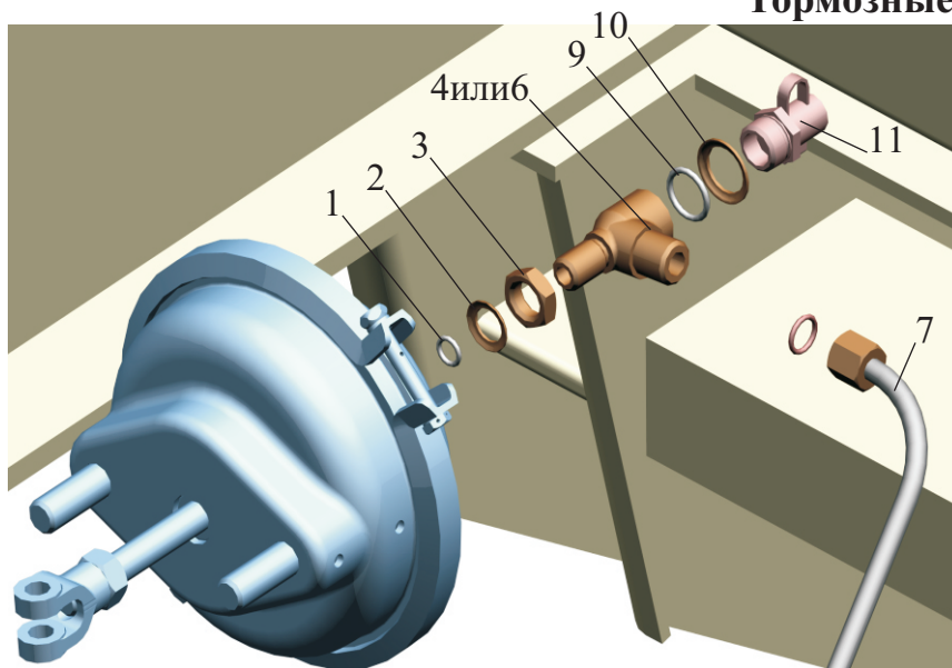
Тормозные камеры задней оси
