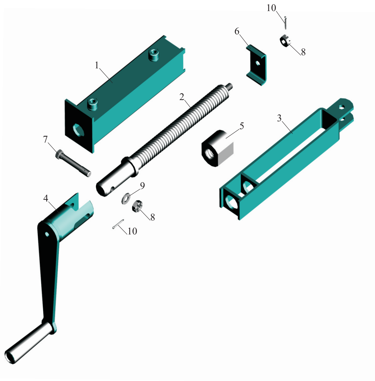
Рис. 40 Привод 9398-3508210-10 Fig. 40 Drive 9398-3508210-10
