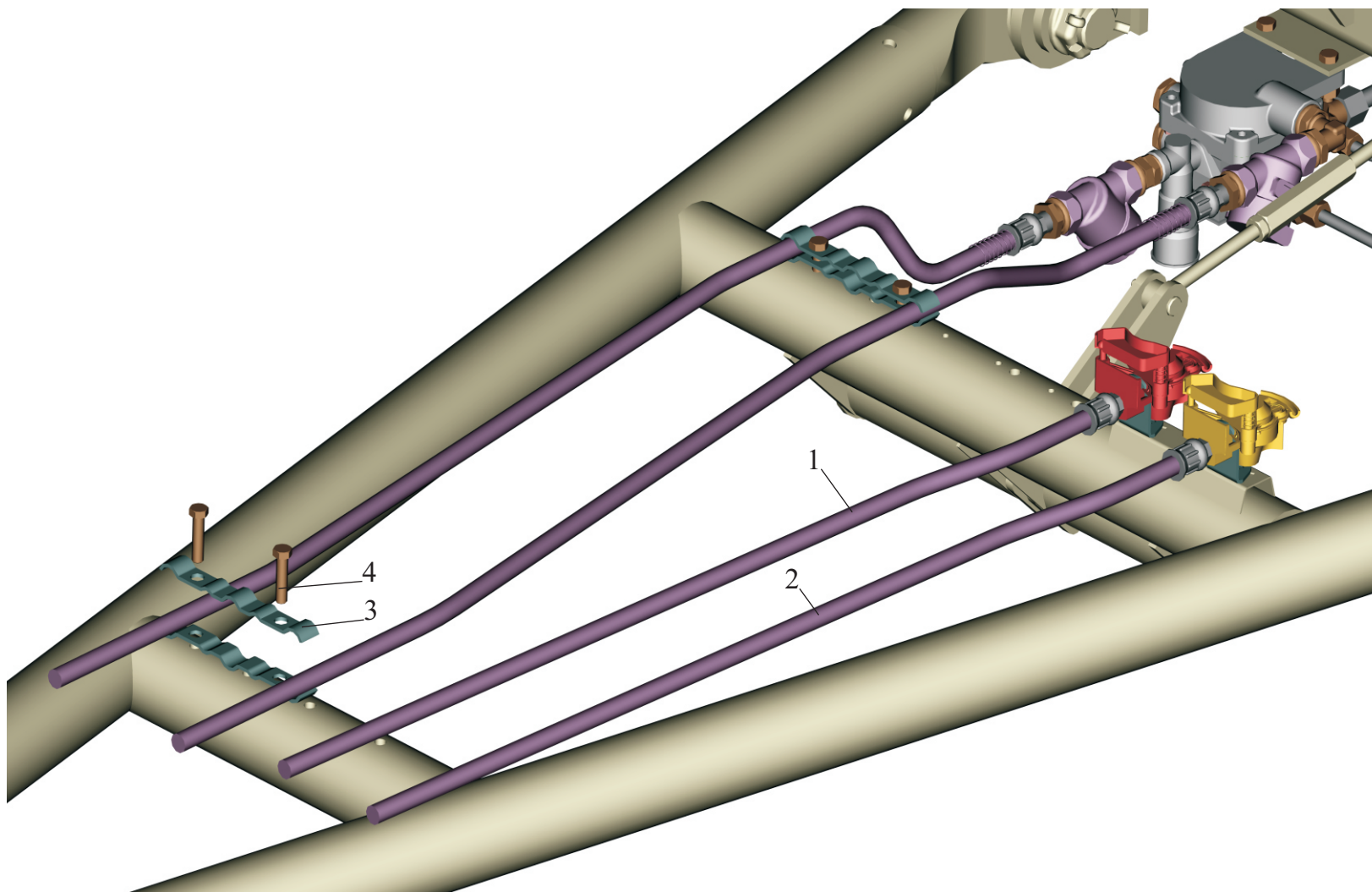
Рис. 32 Установка шлангов питания для соединения с тягачом Fig. 32 Setup of supply hoses for connection with tractor
