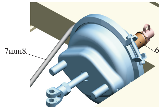
Тормозные камеры передней оси
