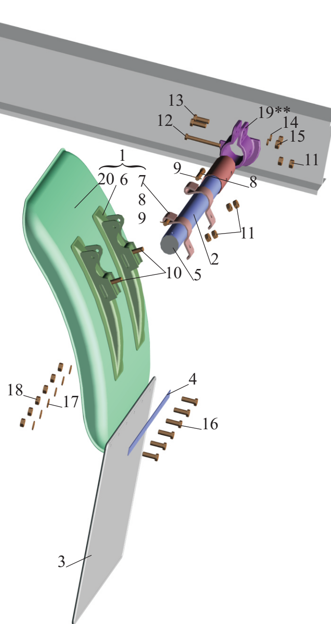
Рис. 54 Установка передних брызговиков 8561-8500042-020 Fig. 54 Installation nut guard front 8561-8500042-020
