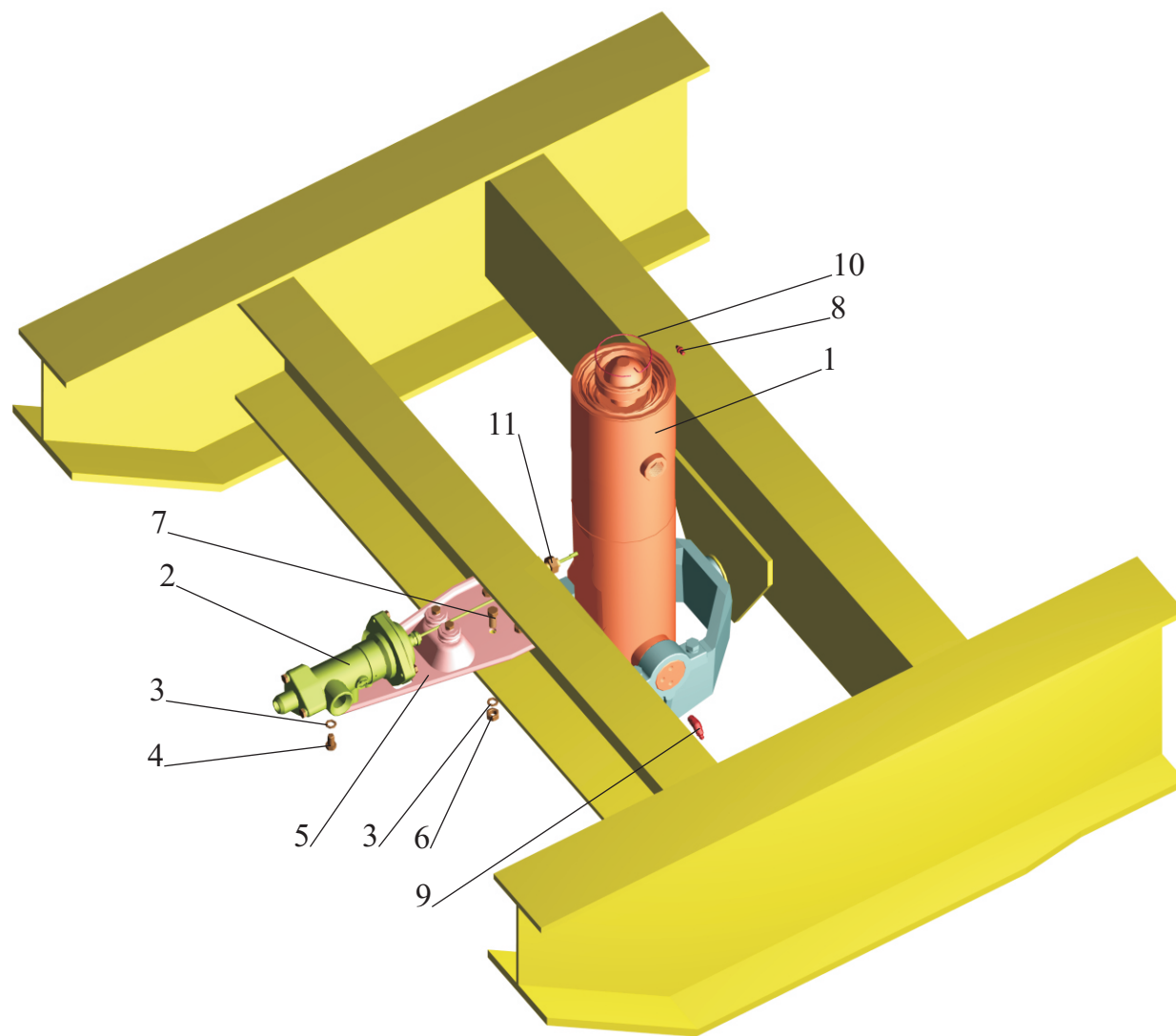
Рис. 58 Установка гидроцилиндра и клапана 8571-8603500 Fig. 58 Installation of cylinder and valve 8571-8603500
