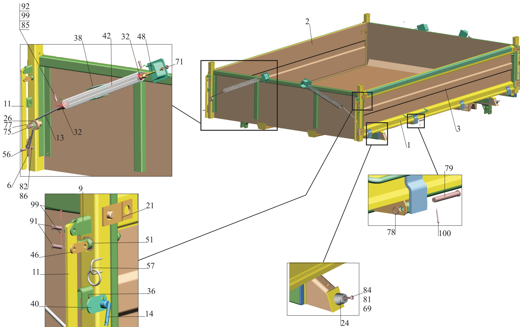
Рис. 47 Платформа 8571-8500020-050 Fig. 47 Platform 8571-8500020-050
