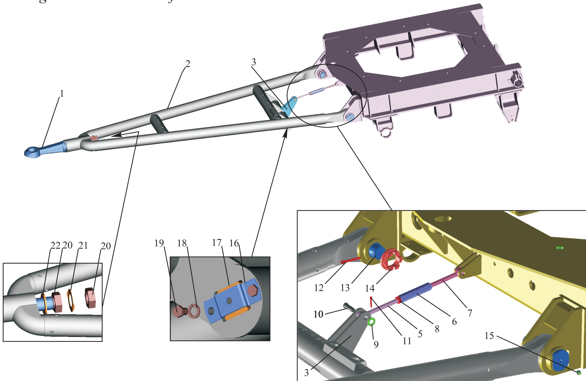
Рис. 5 Установка дышла 8571-2700016 Fig. 5 Installation of trailer hitch
