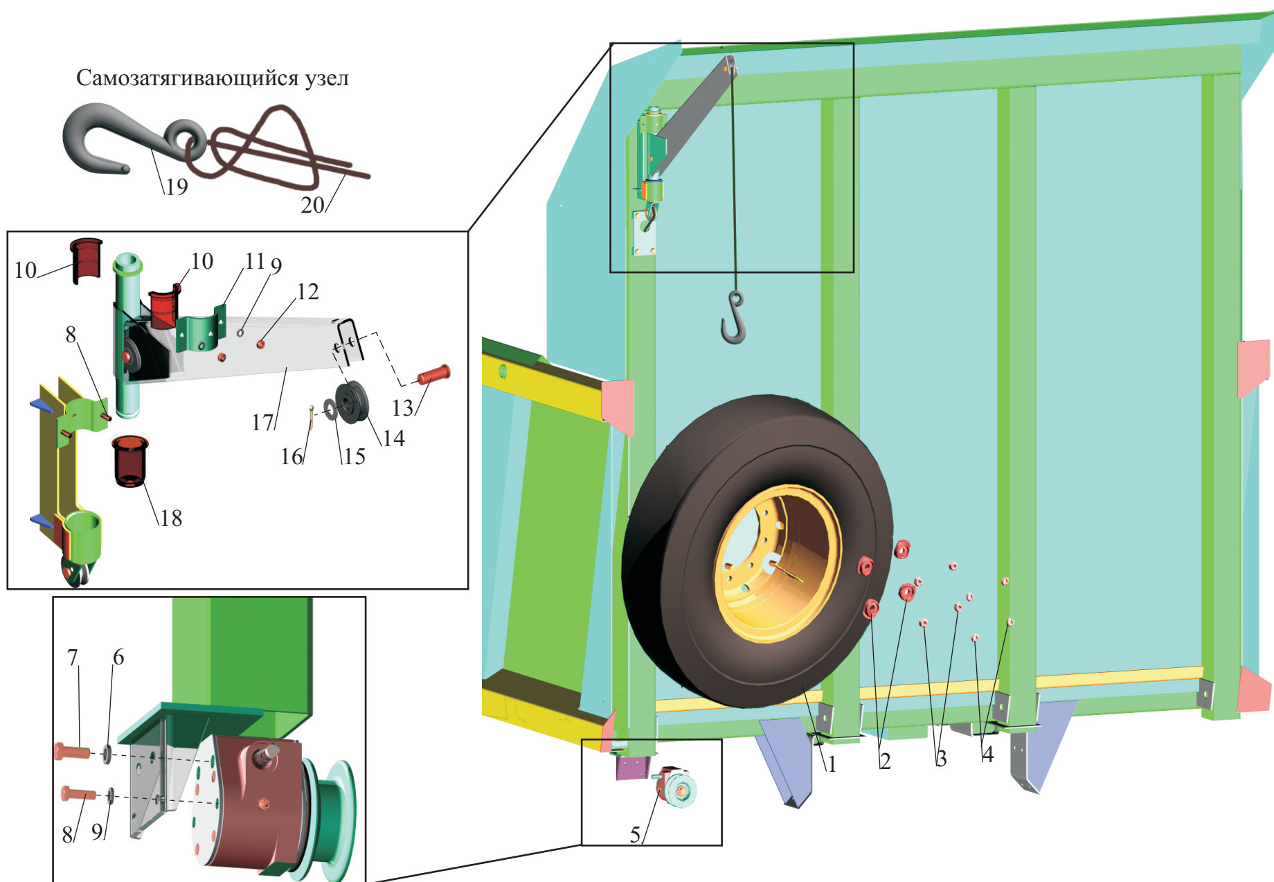
Рис. 22 Установка запасного колеса 551605-3100001-010, 551605-3100001-710 Fig. 22 Truck tractor spare wheel carrier 551605-3100001-010, 551605-3100001-710
