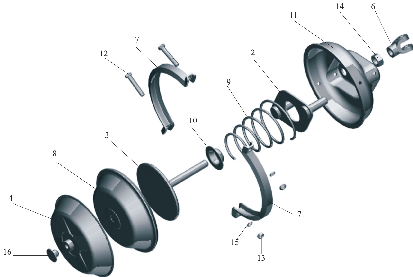
Рис. 17 Камера тормозная 5336-3519210, 5336-3519211 Fig. 17 Brake chamber 5336-3519210, 5336-3519211
