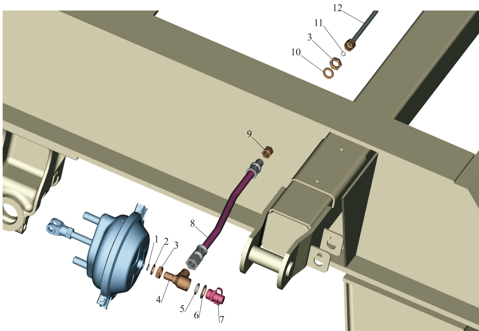
Рис. 25 Присоединительная арматура к тормозным камерам Fig. 25 Connected equipment to brake chambers
