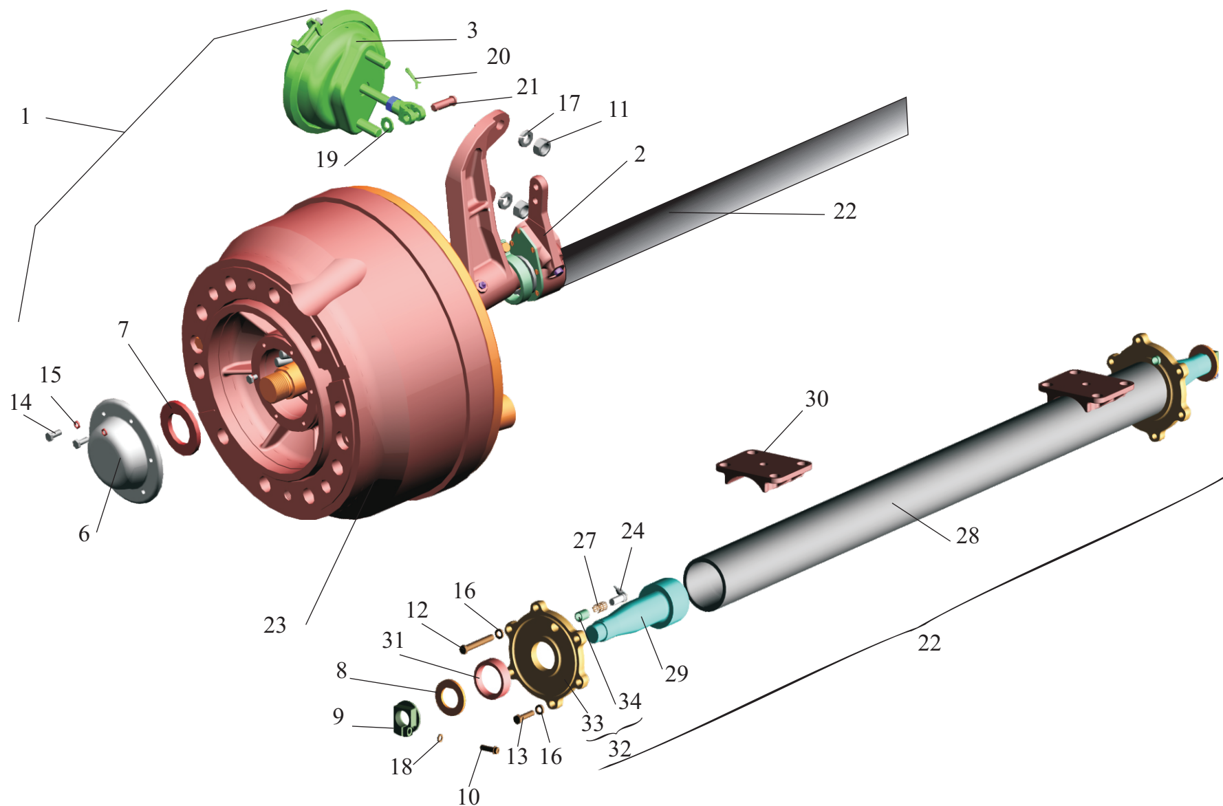
Рис. 16 Ось колес с тормозами 8571-2410007, 8571-2410008 Fig. 16 Axle of wheels 8571-2410007, 8571-2410008
