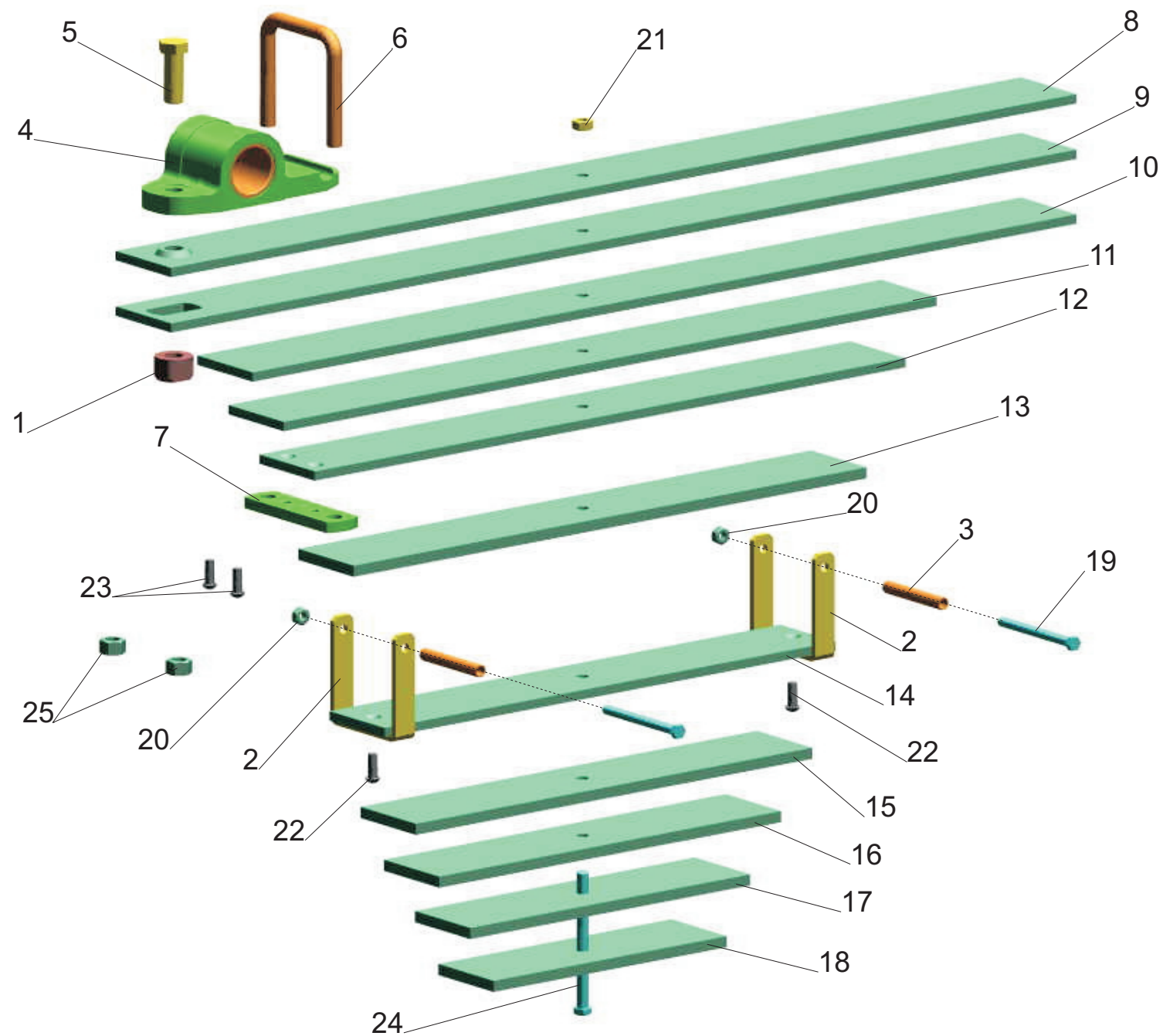
Рис. 9 Рессора 8561-2912012-010. Fig. 9 Spring 8561-2912012-010.
