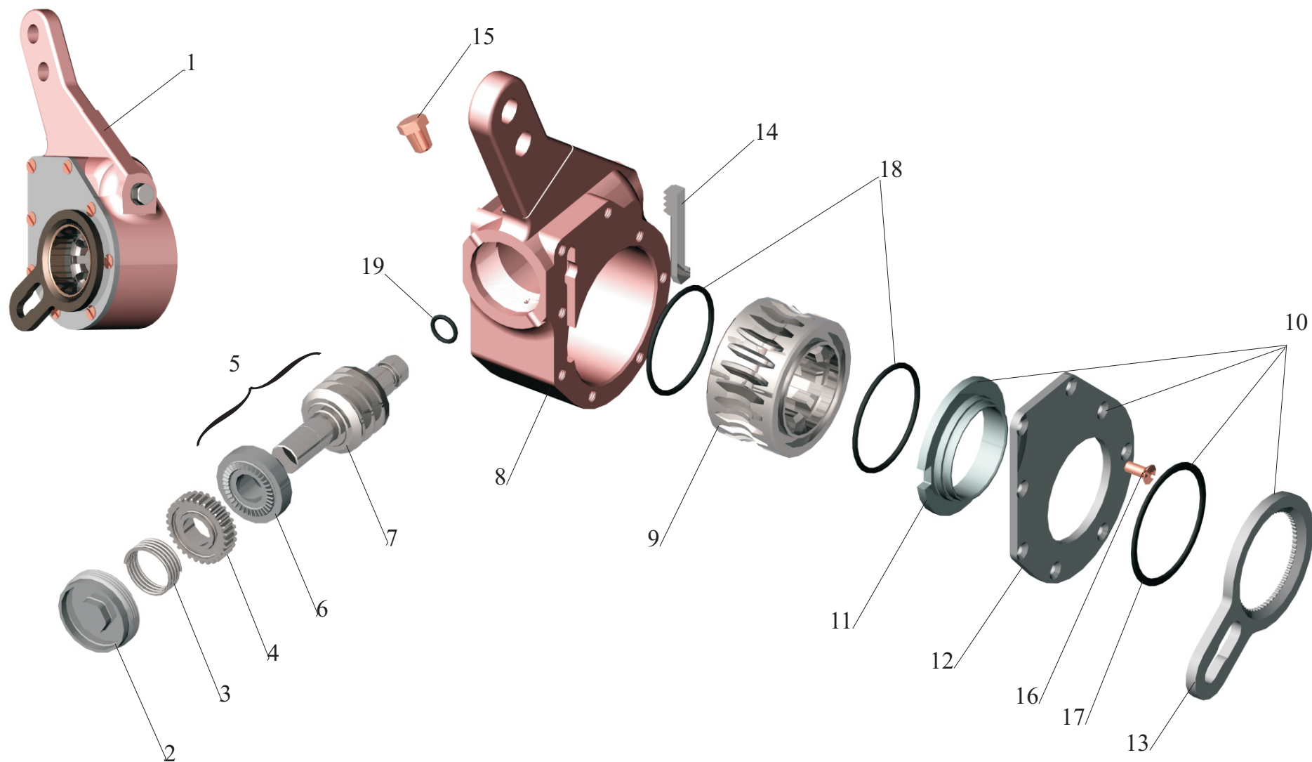
Рис. 19 Рычаг регулировочный. 64226-3501136-010 Fig. 19 Adjusting lever. 64226-3501136-010
