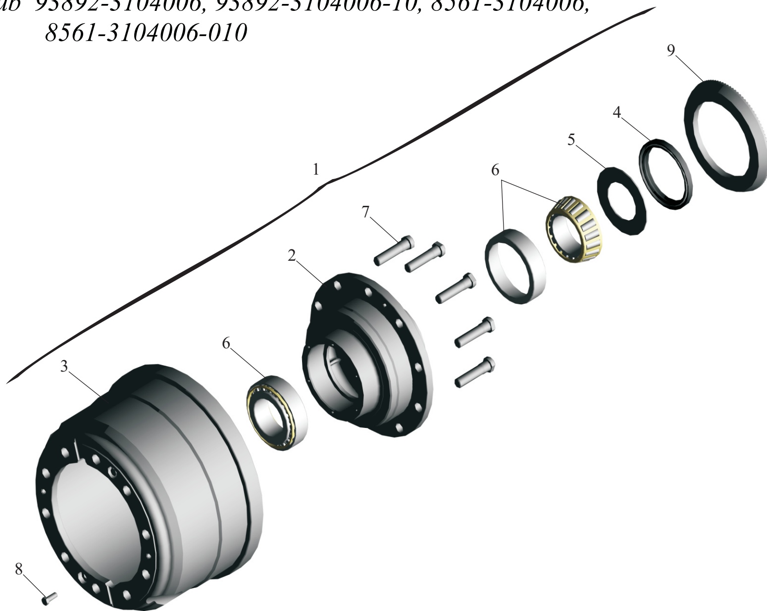
Рис. 13 Ступица 93892-3104006, 93892-3104006-10, 8561-3104006, 8561-3104006-010
