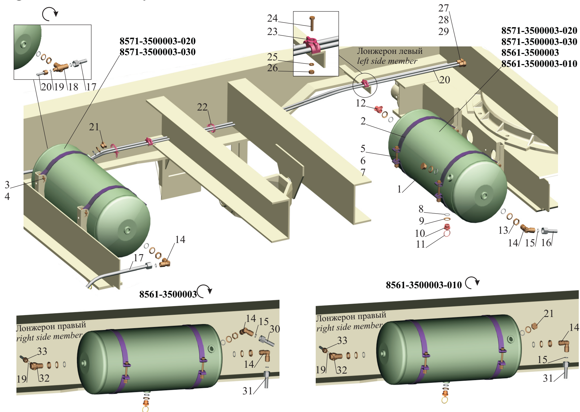
Рис. 35 Установка ресиверов и соединительной арматуры Fig. 35 Installation of receivers and attach accessories
