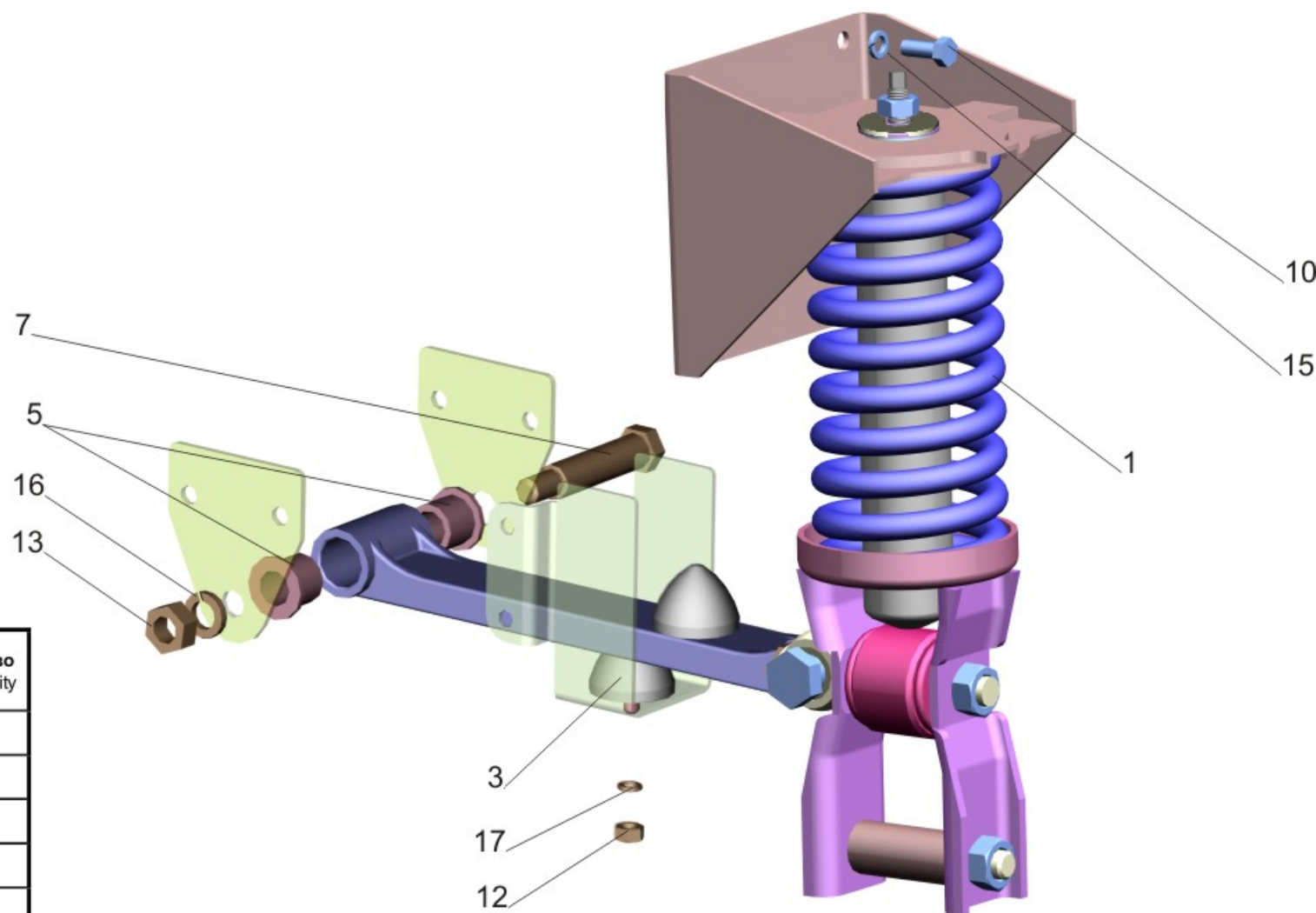
Рис. 216 Заднее подрессоривание 6501-5001800-010 Fig. 216 Rear springing 6501-5001800-010
