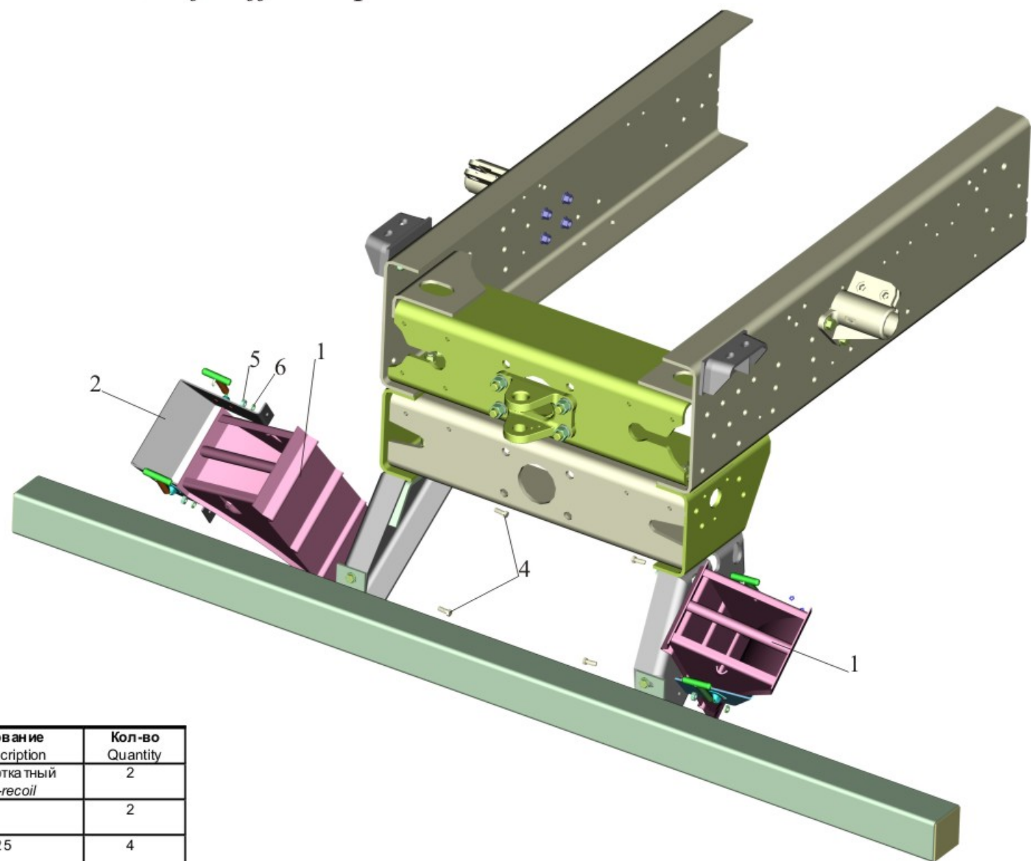
Рис. 210 Установка противооткатных упоров 53373-3900037. Fig. 210 Installation of buffer stop 53373-3900037.
