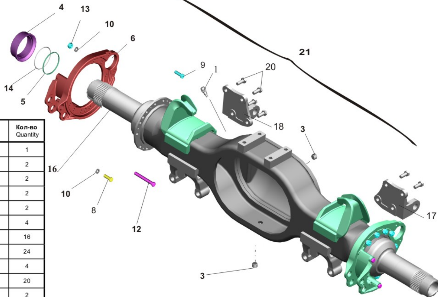
Рис. 64 Мост задний. Картер моста 651608-2401010 Fig. 64 Rear axle. Axle housing 651608-2401010
