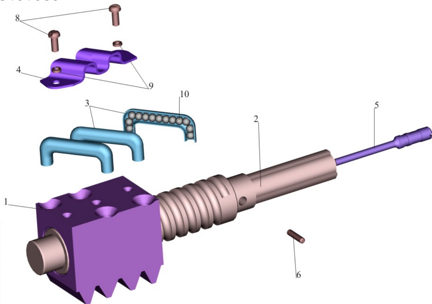
Рис. 138 Винт 64229-3401030
