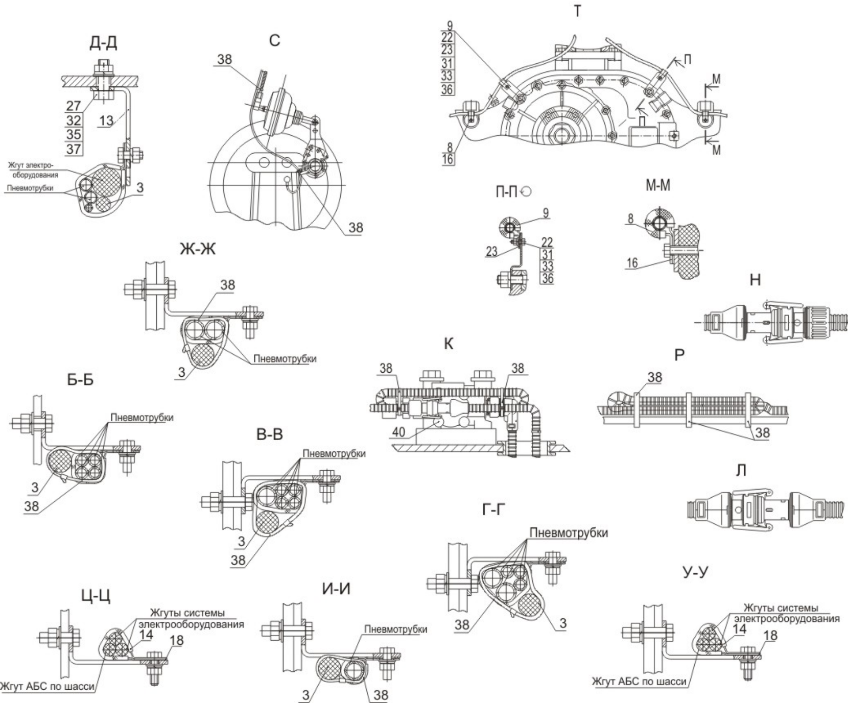
Рис. 205 Установка электрооборудования ABS тормозов (лист 2) Fig. 205 Setting of electrical equipment ABS brakes ( page 2)
