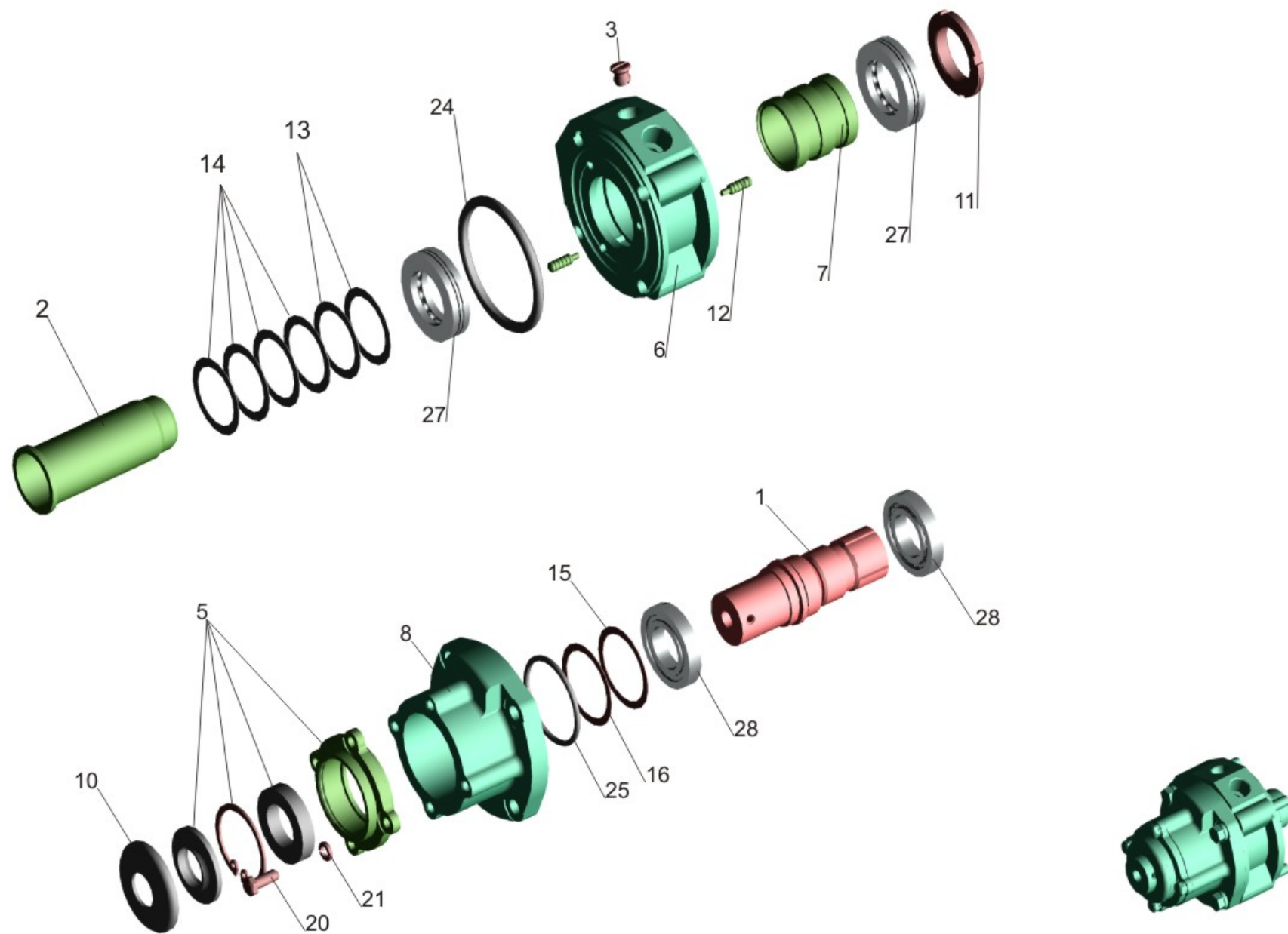
Fig. 142 Divider 5336-3416010-01
