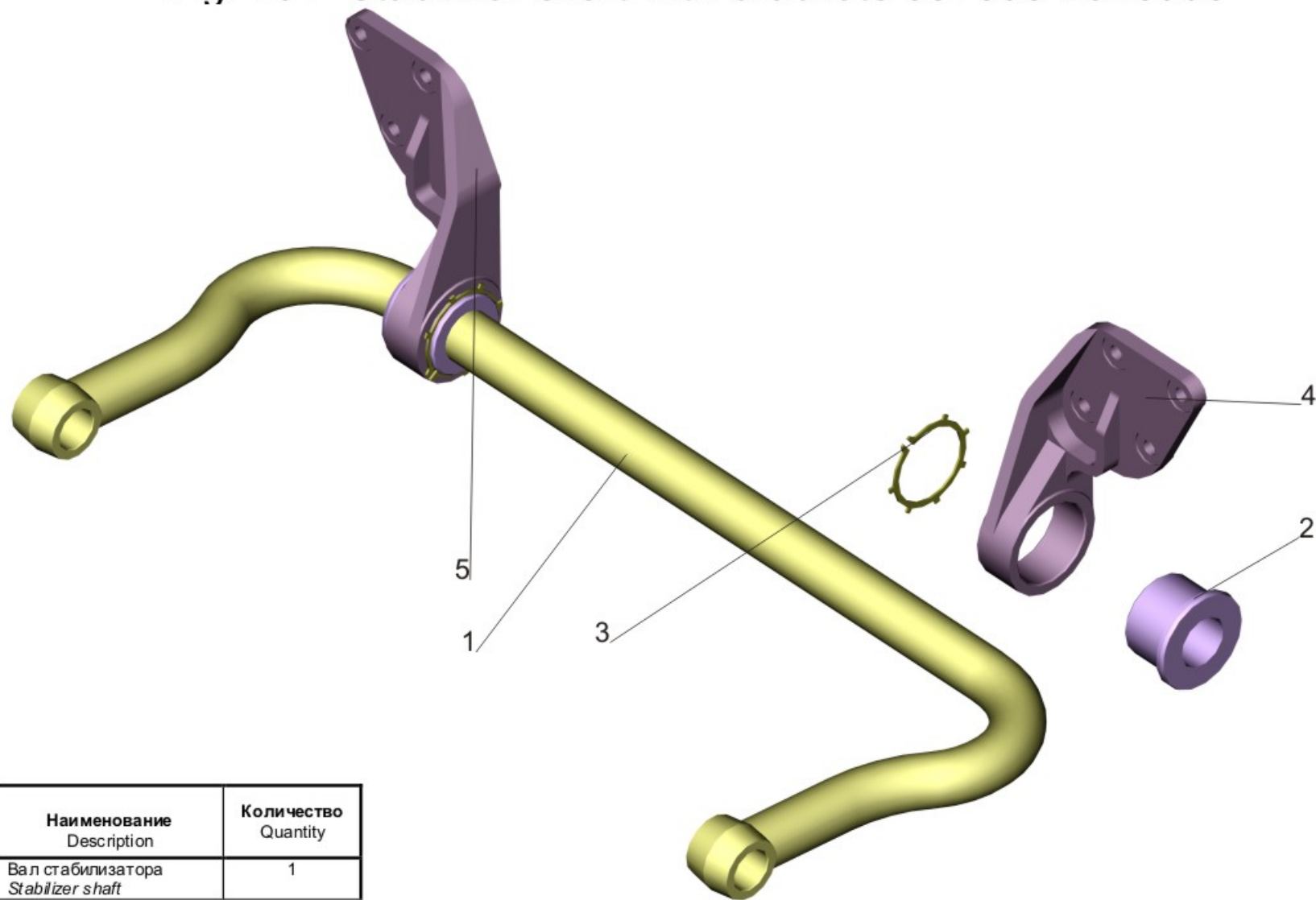
Рис. 101 Вал стабилизатора с кронштейнами 651608-2916006 Fig. 101 Stabilizer shaft with brackets 651608-2916006
