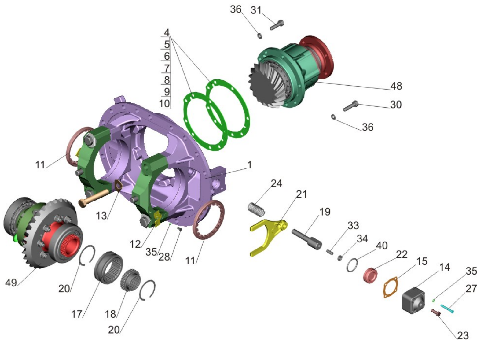
Рис. 65 Редуктор 54323-2402010-040, 54323-2402010-640 Fig. 65 Reducer gear 54323-2402010-040, 54323-2402010-640
