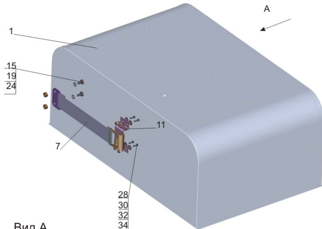
Рис. 252 Ящик инструментальный 6501-5108010 Fig. 252 Box tool 6501-5108010
