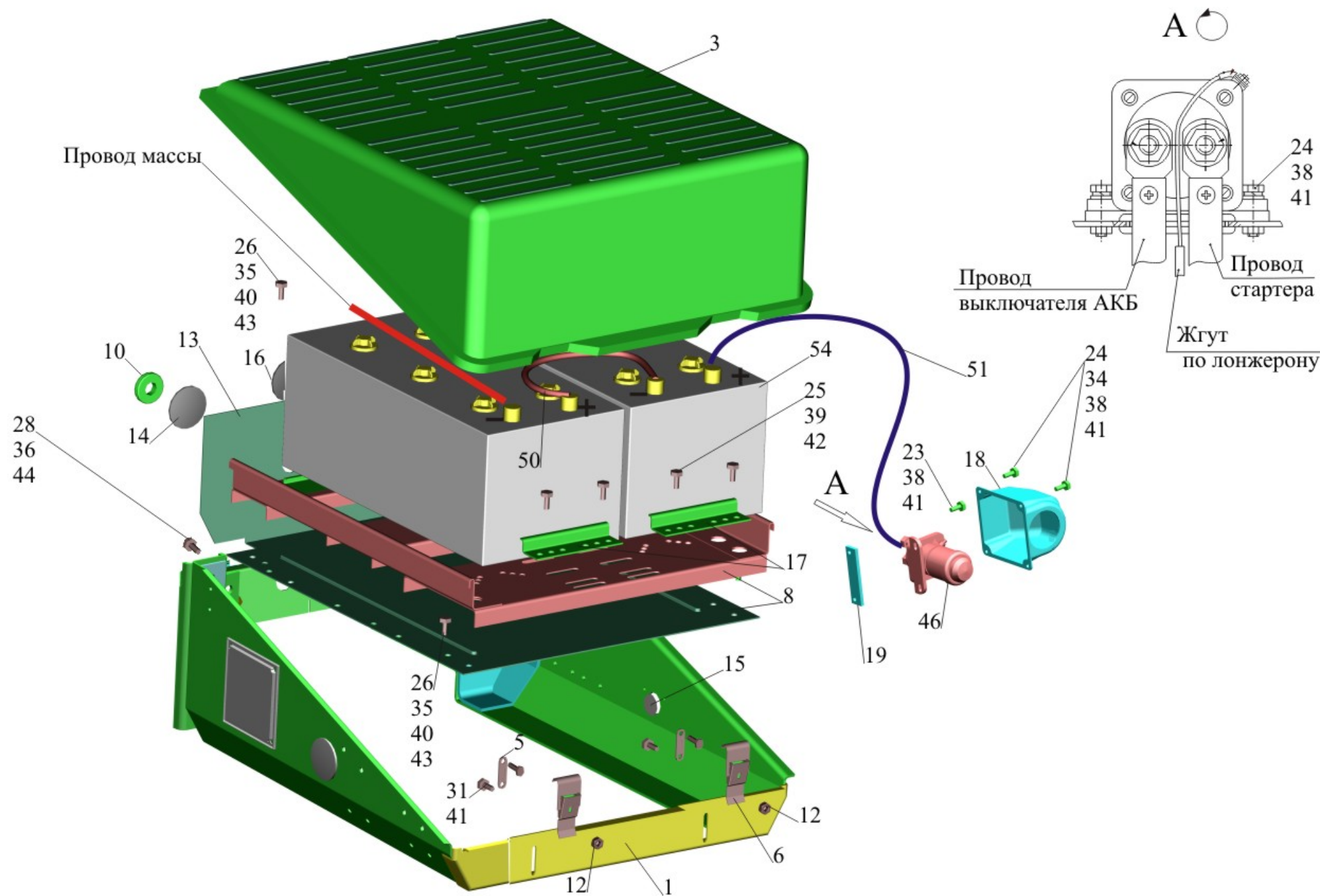
Рис. 175 Установка аккумуляторных батарей 6516А8-3700008, 6516А8-3700008-700 Fig. 175 Installation of storage batteries 6516А8-3700008, 6516А8-3700008-700
