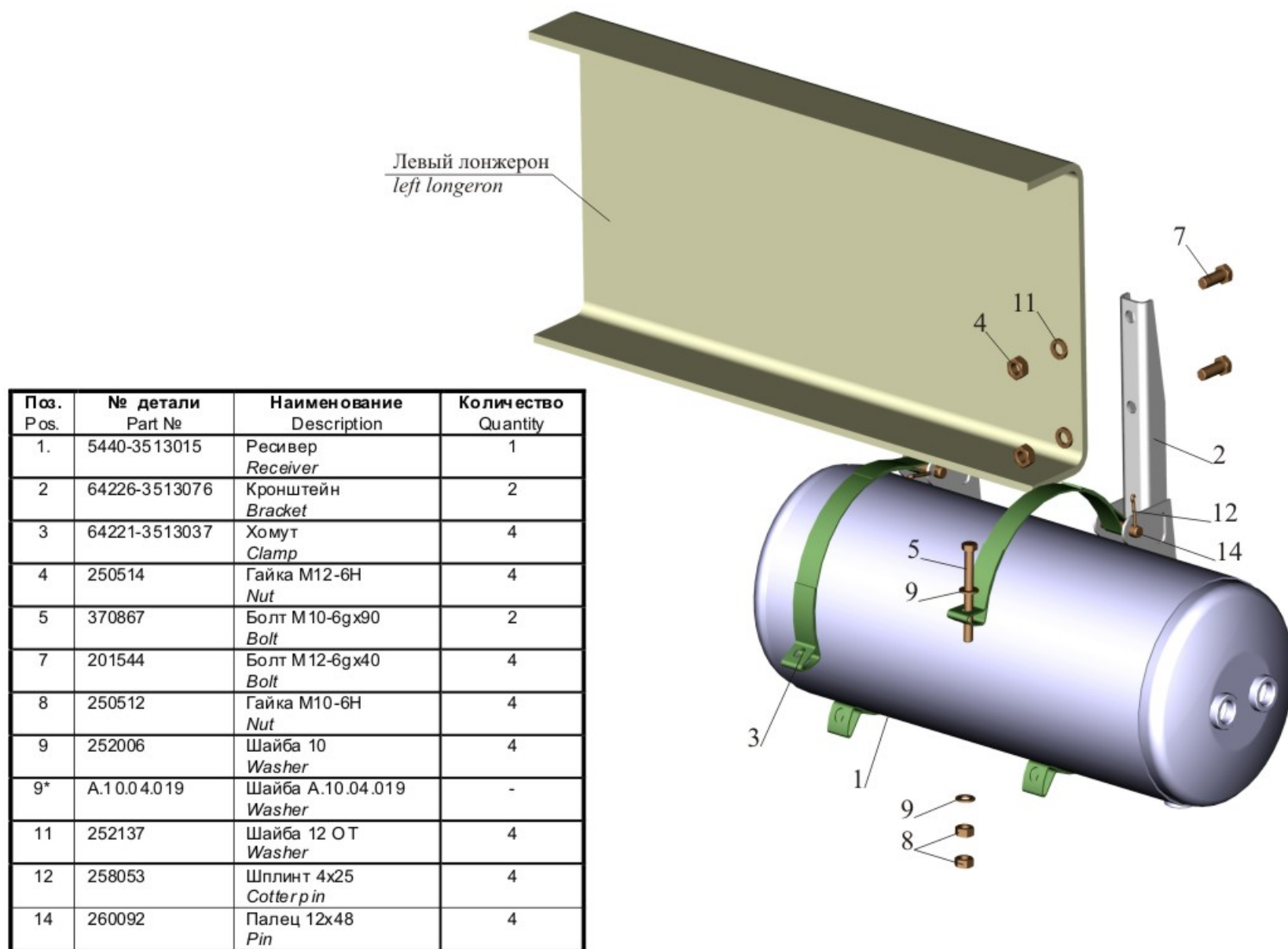
Рис. 158 Крепление ресивера 650108-3513006 Fig. 158 Mounting of receiver 650108-3513006
