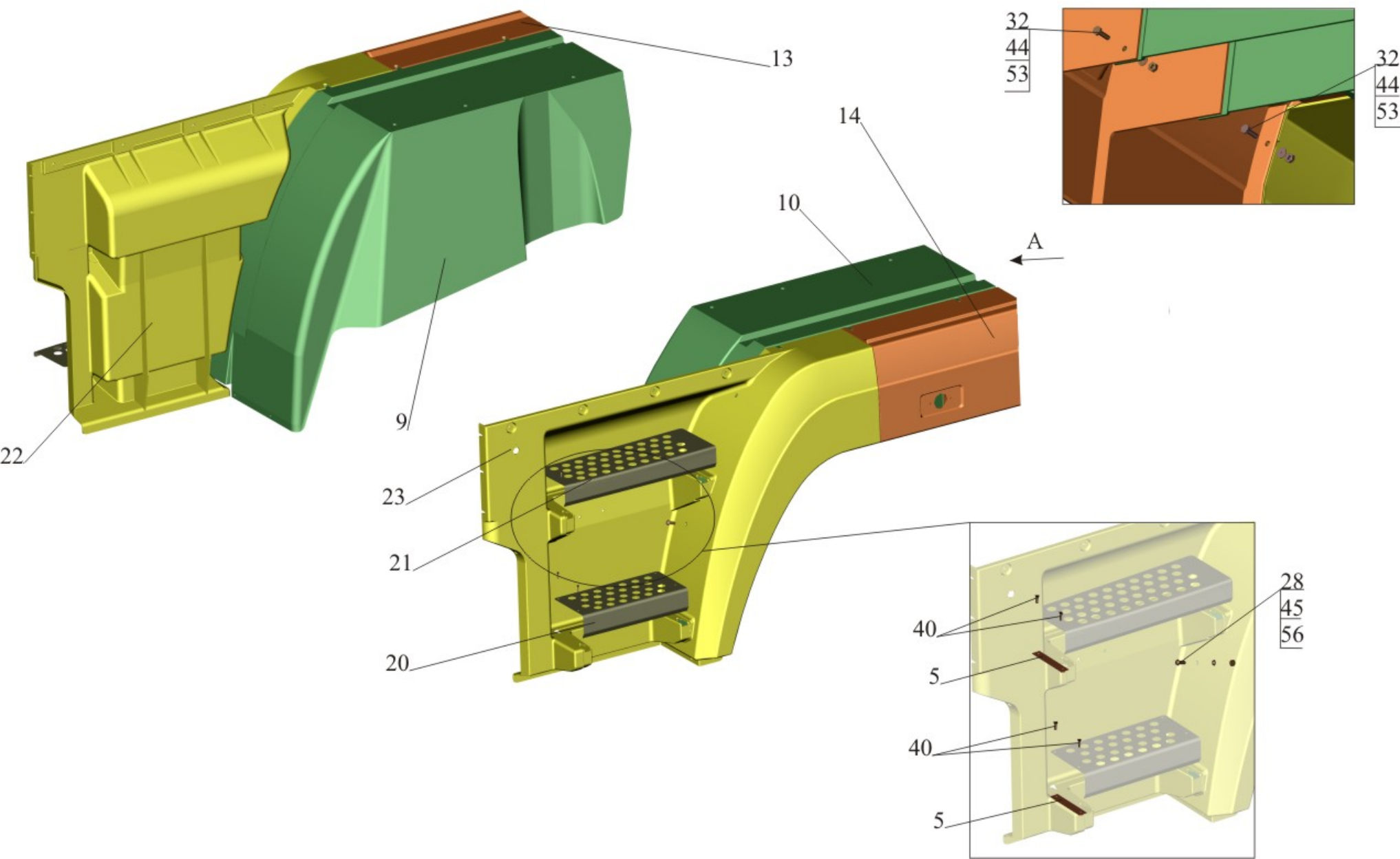
Fig. 272 Plumage 6516A8-8400010-010, 6516A8-8400011-010
