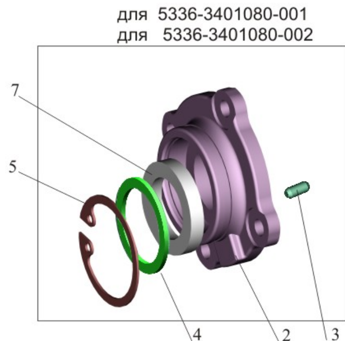
Рис. 139 Крышка 5336-3401080 Fig. 139 Cover 5336-3401080
