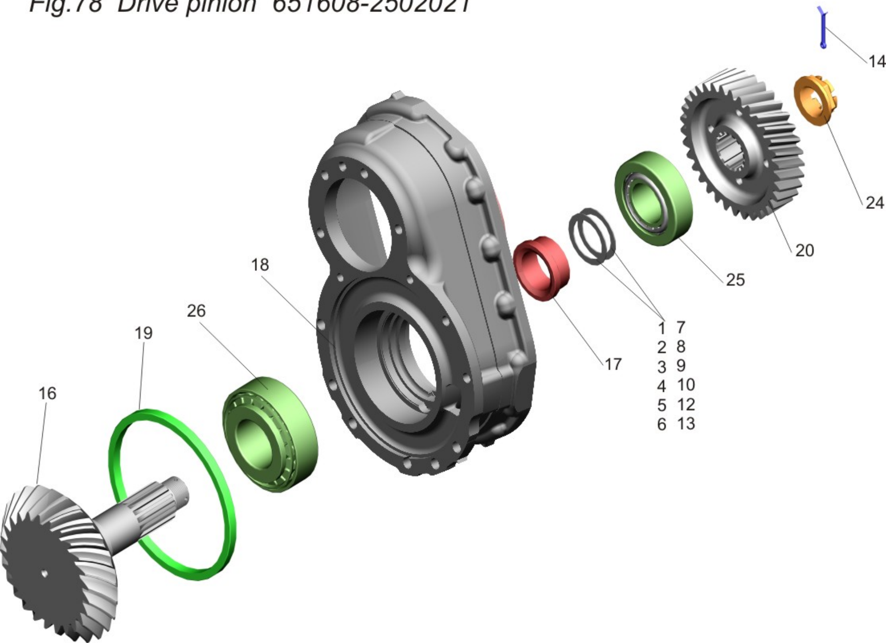
Рис.78 Шестерня ведущая 651608-2502021
