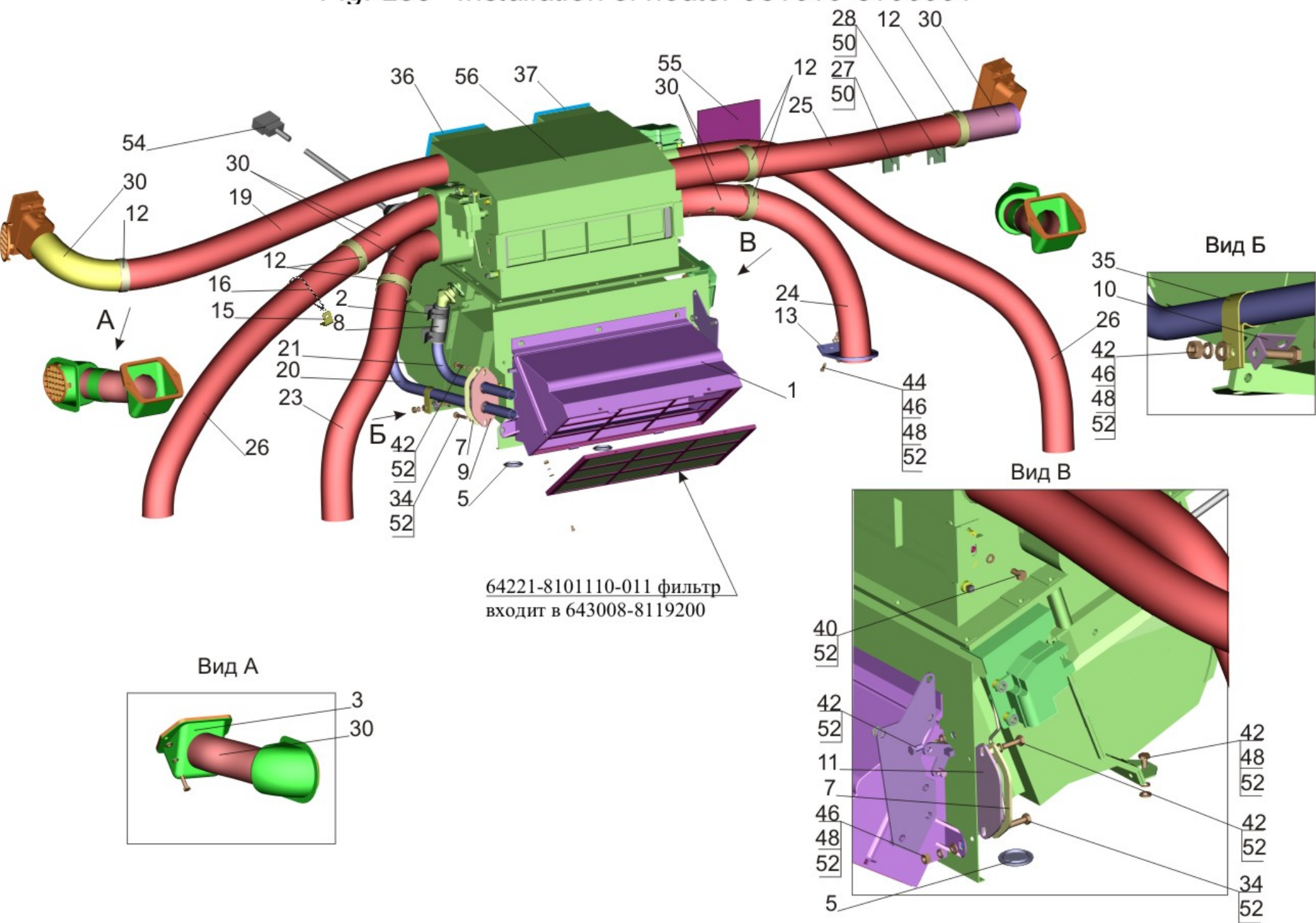
Fig. 255 Installation of heater 631019-8100001
