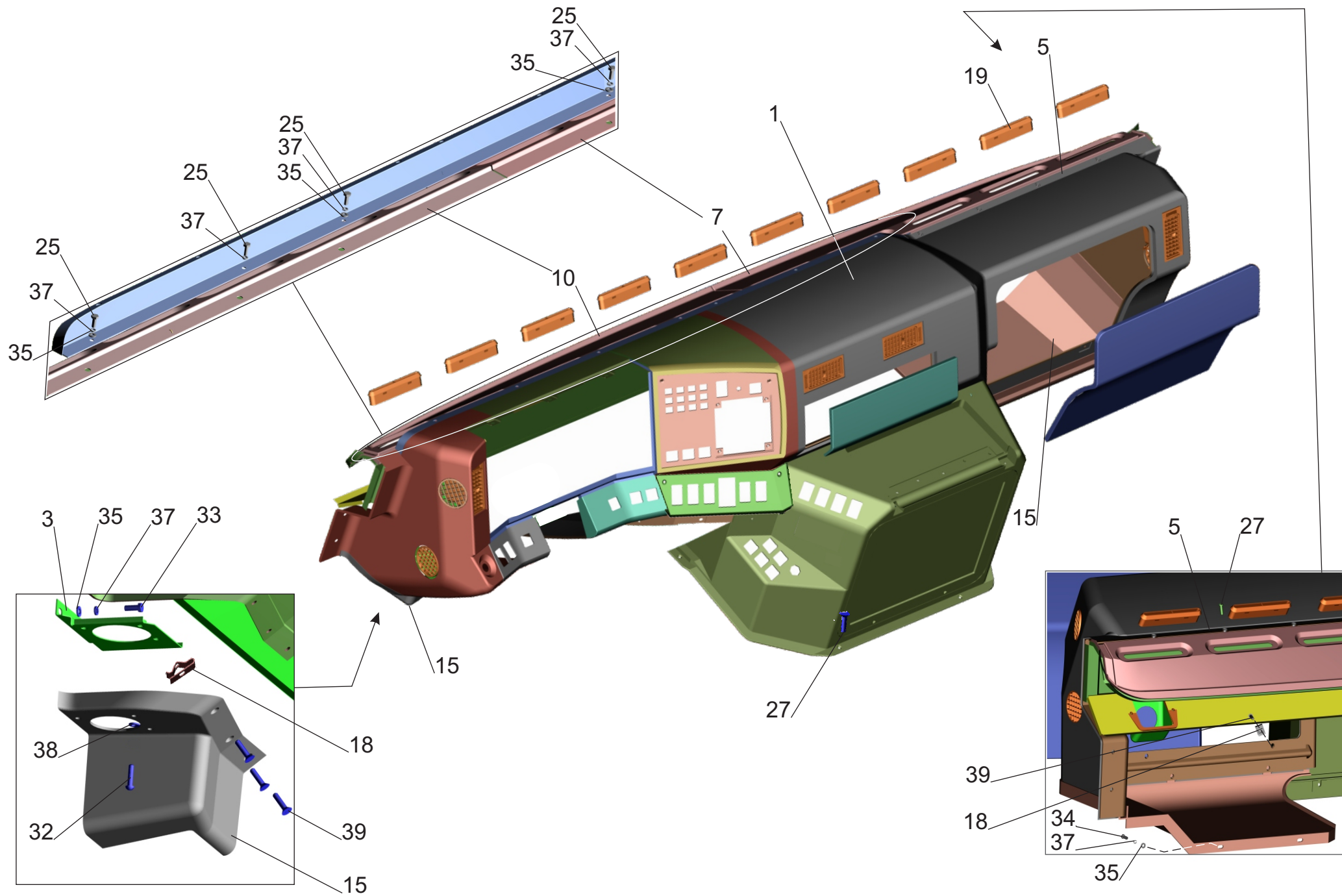
Рис. 224 Установка панели приборов 6430-5300014-020. Fig. 224 Installing of instrument panel 6430-5300014-020.
