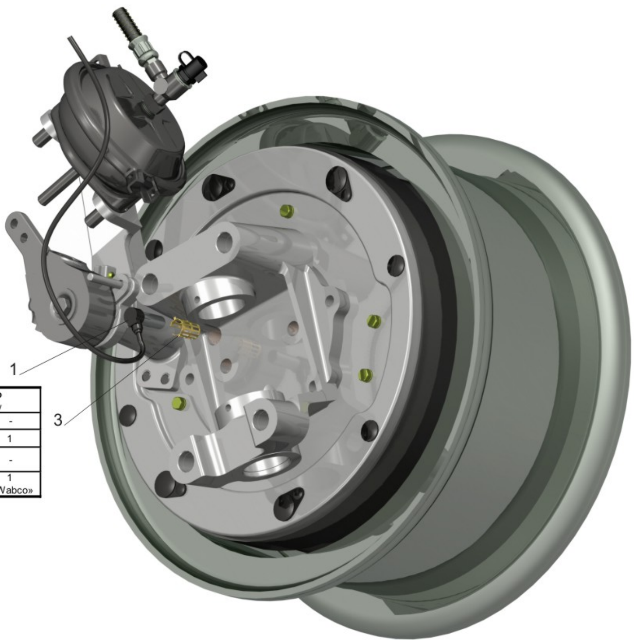
Рис. 206 Установка датчика АБС на передних колесах 54402-3538101, 543240-3538101 Fig. 206 Installation of transmitter ABS on forward sprockets
