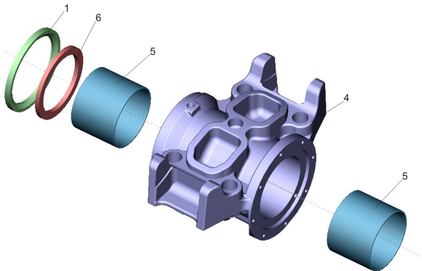
Рис.99 Балансир рессоры 6418-2918018 Fig.99 Walking beam assemblies 6418-2918018
