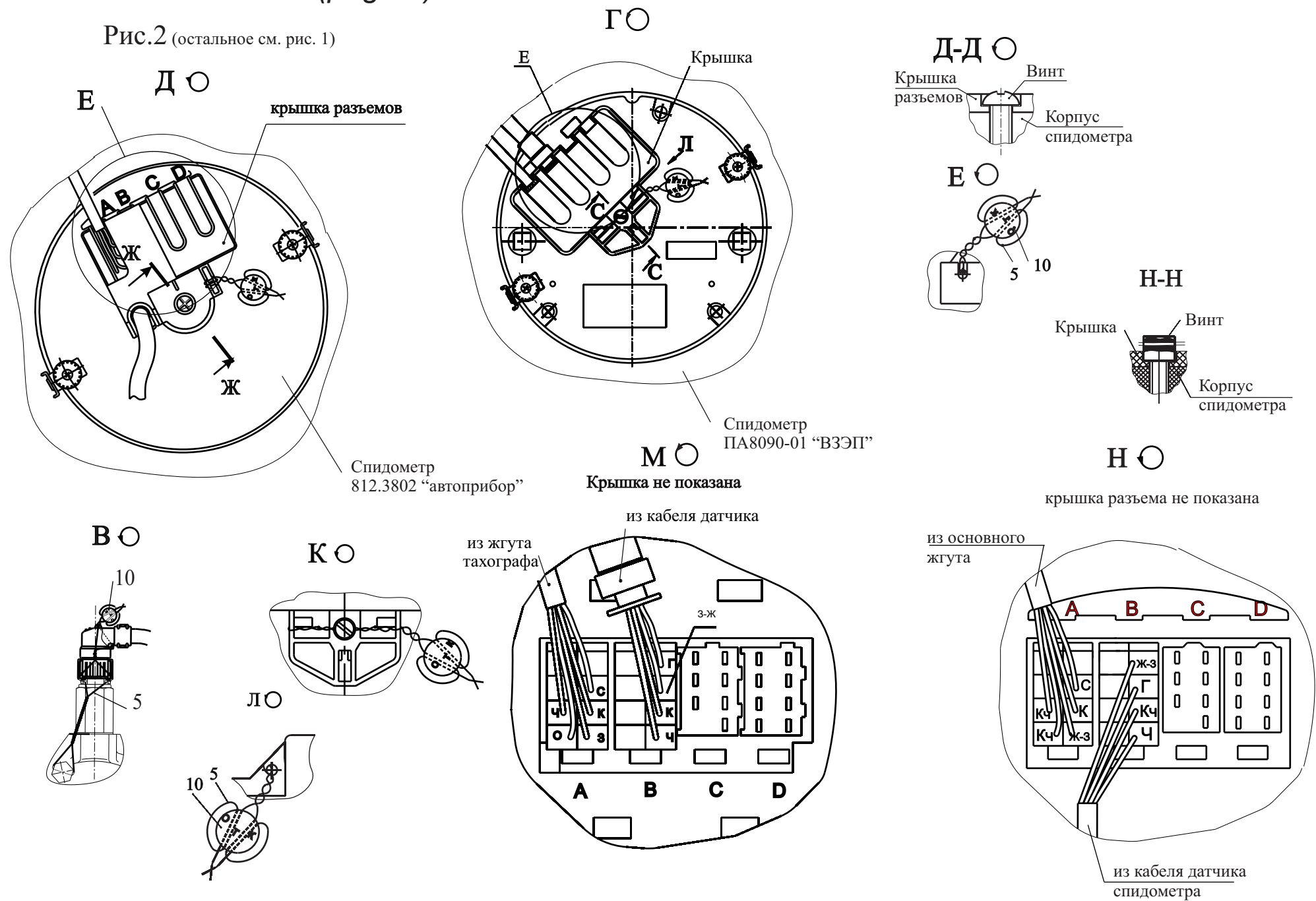
Рис. 200 Установка и пломбировка спидометра 6516А8-3800004-020, 6516А8-3800004-021 (лист 1) Fig. 200 Installation and identification seal of a speedometer 6516А8-3800004-020, 6516А8-3800004-021 (page 1)
