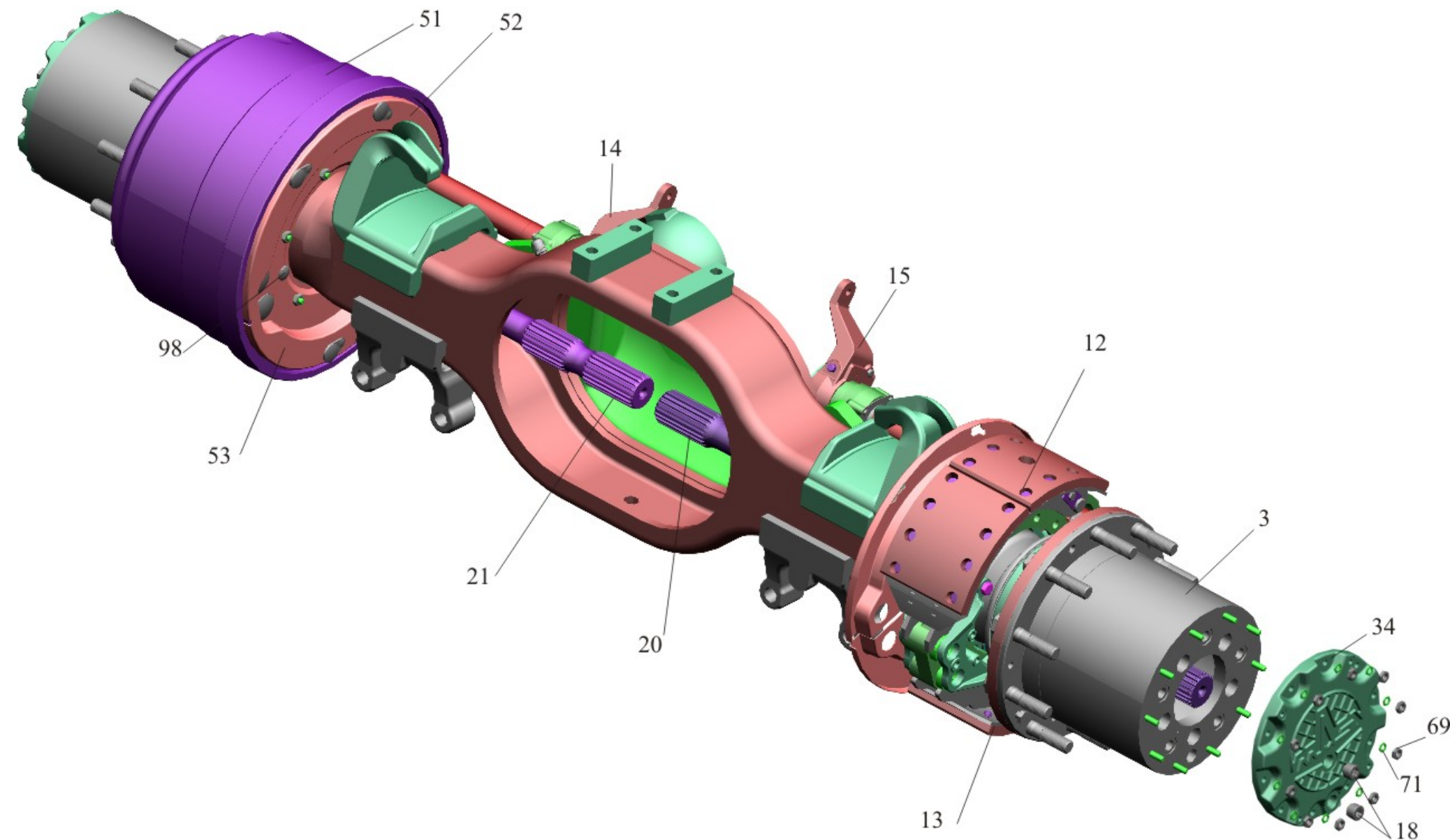
Рис. 72 Мост средний Лист 4 Fig. 72 Intermediate axle Page 4
