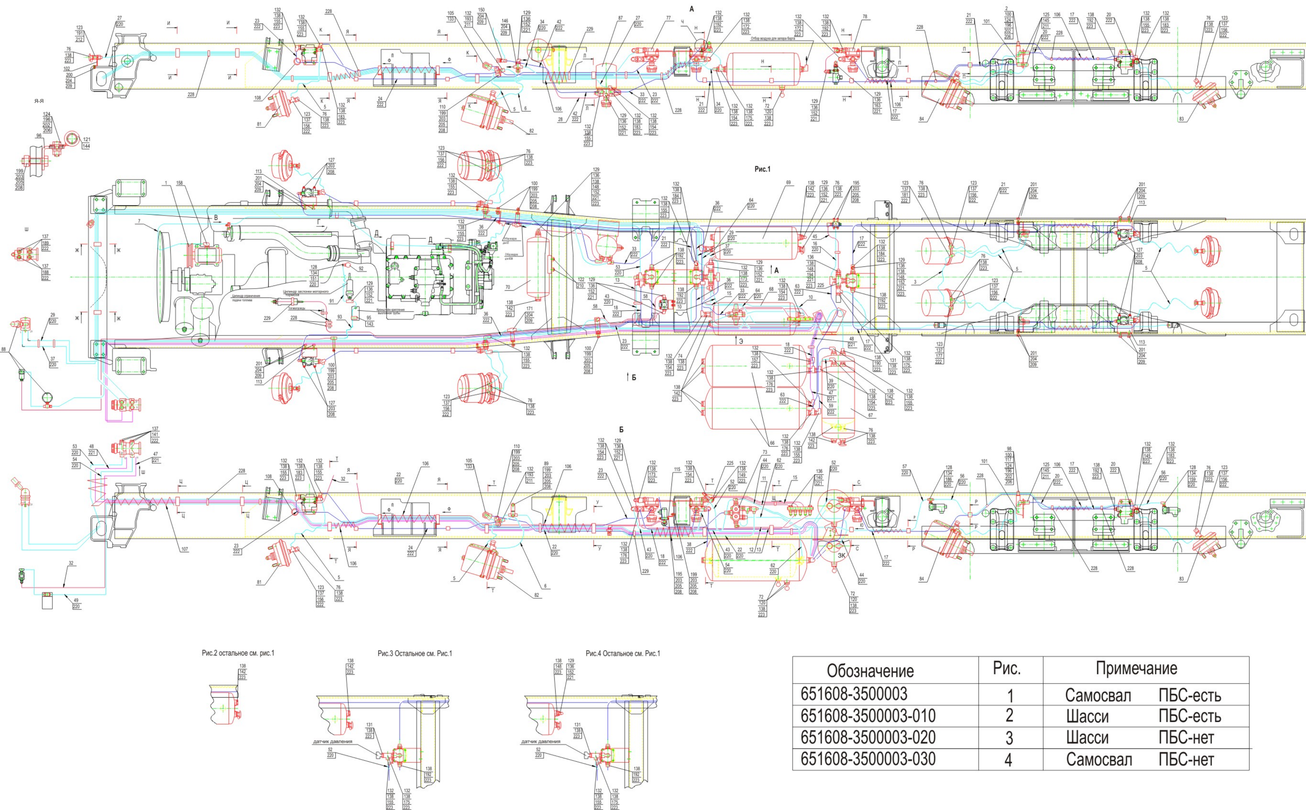
Рис. 154 Установка пневмотормозов 651608-3500003(-010,-020,-020) (лист 1) Fig. 154 Installation pneumobrakes
