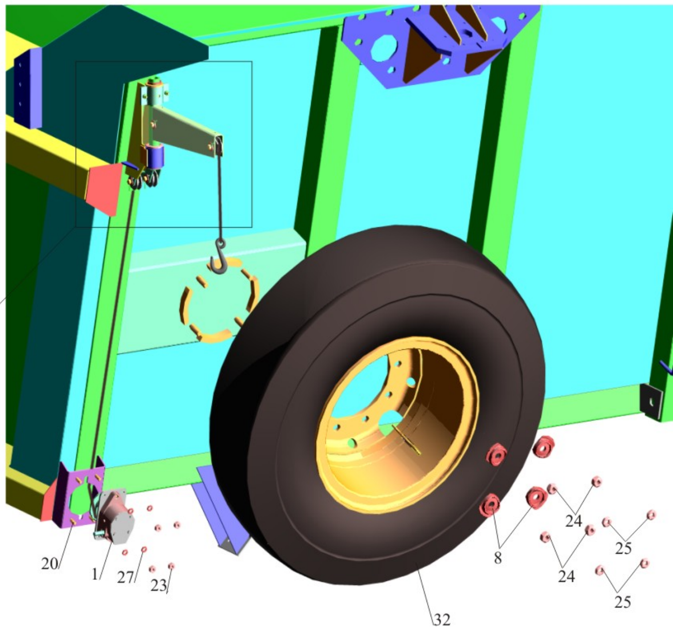
Рис. 125 Установка запасного колеса Fig. 125 Installation spare wheel
