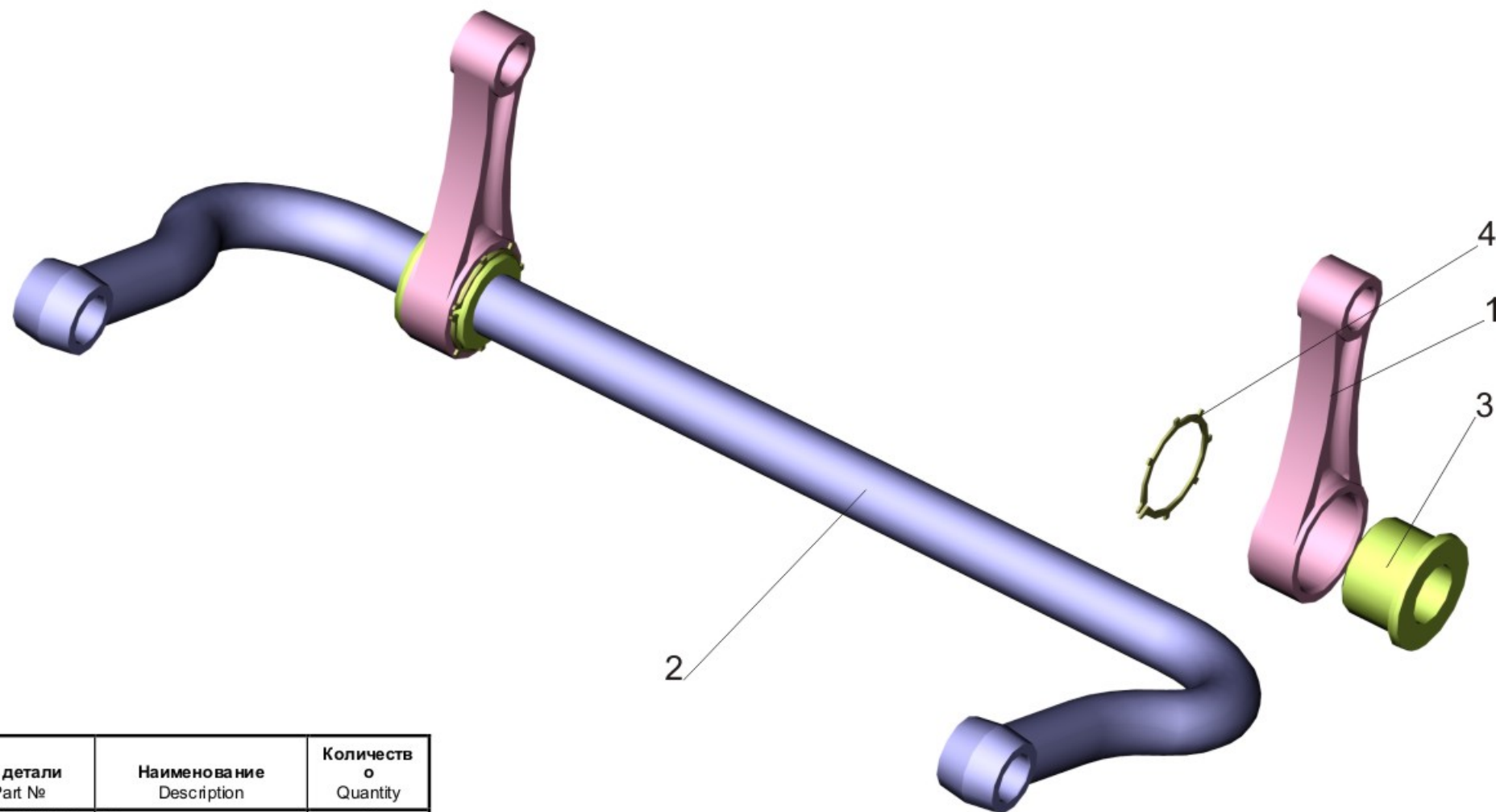
Рис. 100 Вал стабилизатора с рычагами 6501-2916006 Fig. 100 Stabilizer shaft with brackets 6501-2916006
