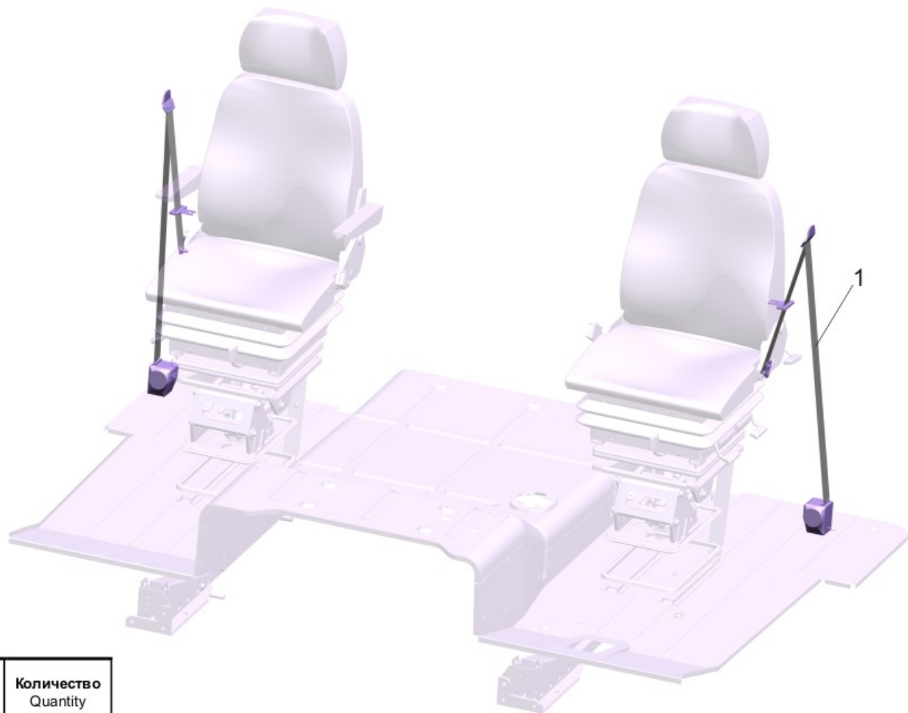
Рис. 251 Установка ремней безопасности 54327-8200024 Fig. 251 Installation safety belt 54327-8200024
