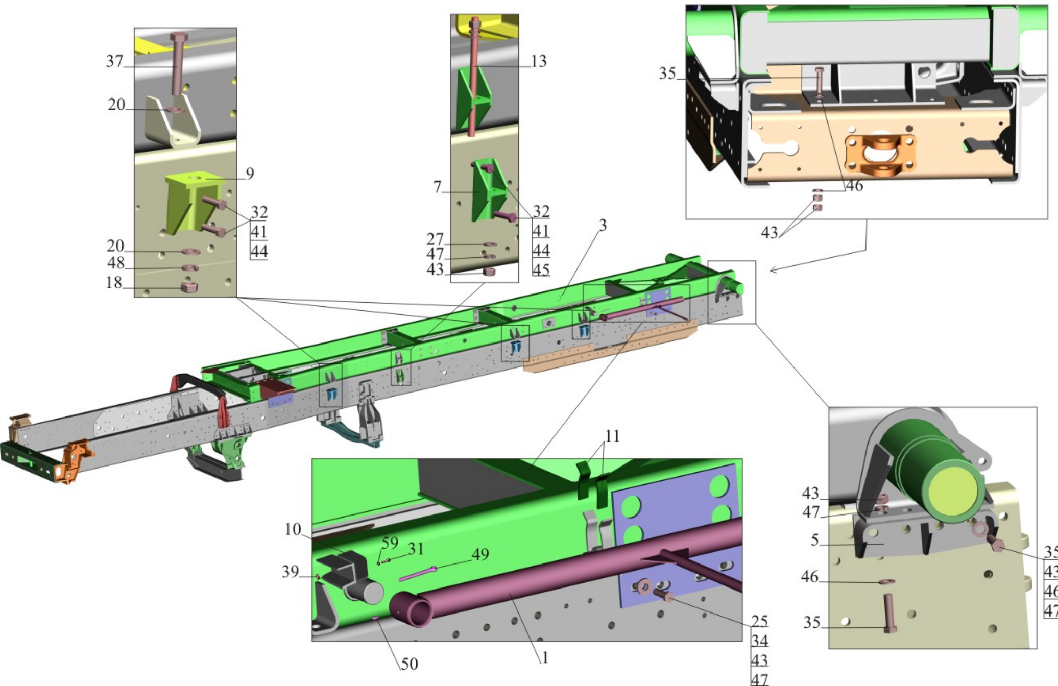
Рис. 284 Установка надрамника 651608-8600002 Fig. 284 Installation above frame 651608-8600002
