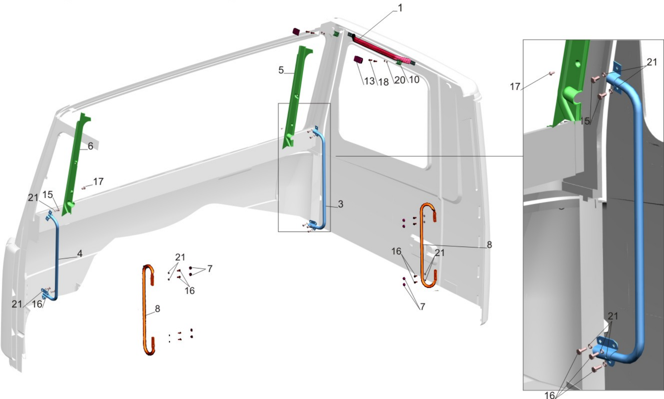
Рис. 230 Установка поручней в кабине 6430-8200030. Fig. 230 Installation of grab handles in cab 6430-8200030.
