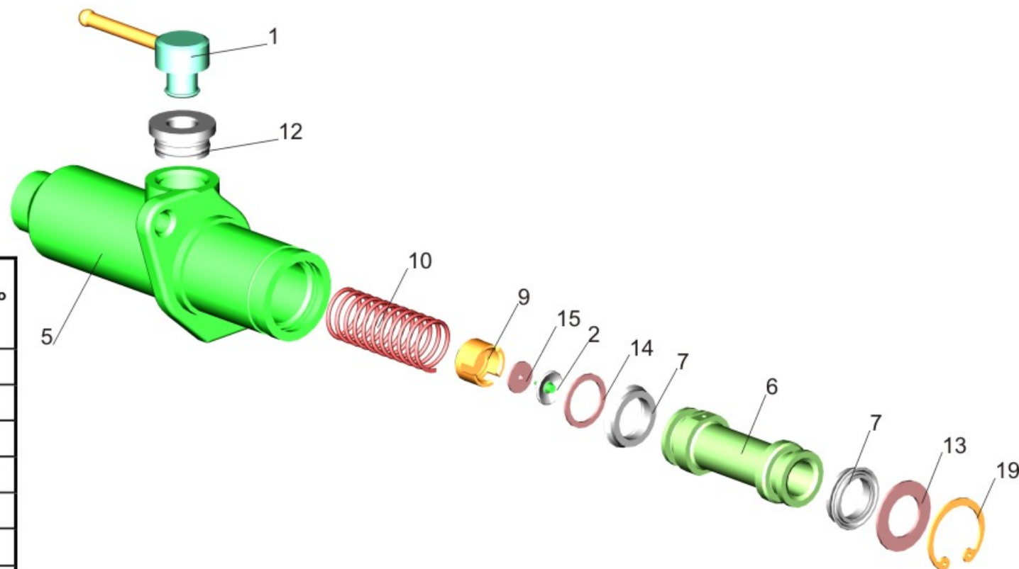
Рис. 35 Цилиндр подпедальный 6430-1602510 Fig. 35 Under pedal cylinder 6430-1602510
