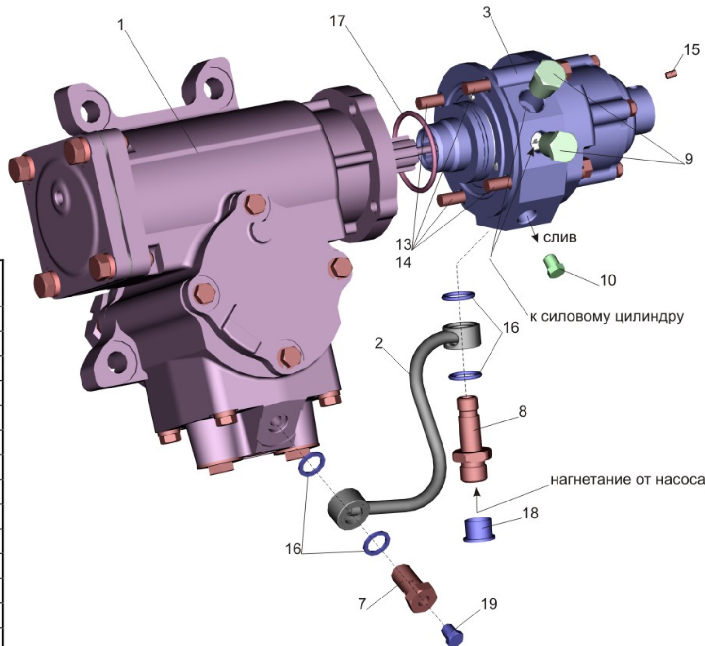
Рис. 136 Рулевой механизм 64221-3400010-10 Fig. 136 Steer 64221-3400010-10
