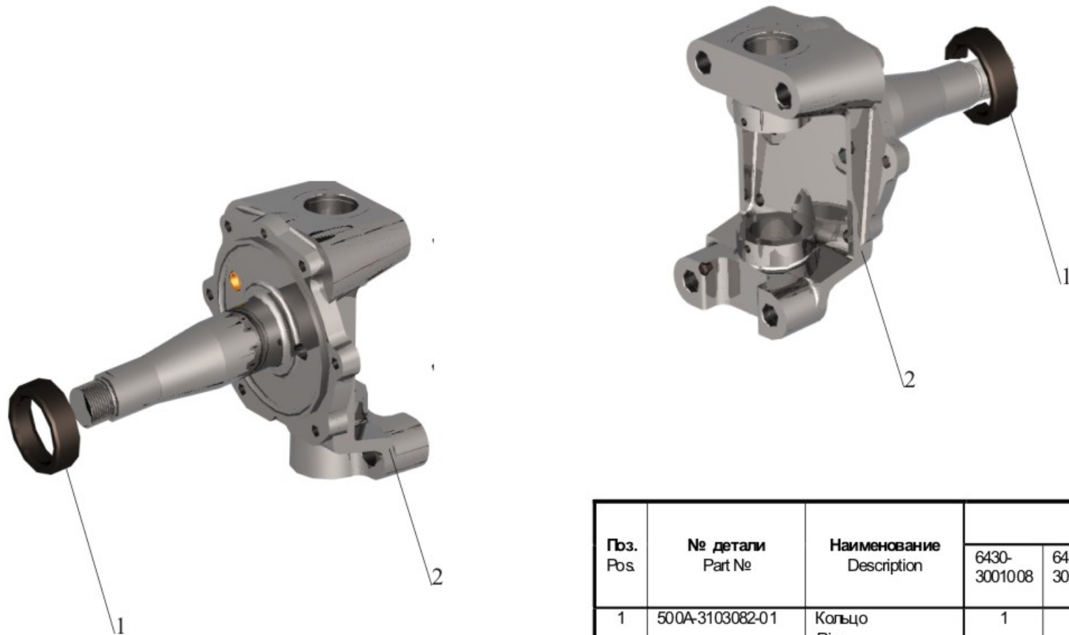
Рис. 112 Кулак поворотный Fig. 112 Steering knuckle
