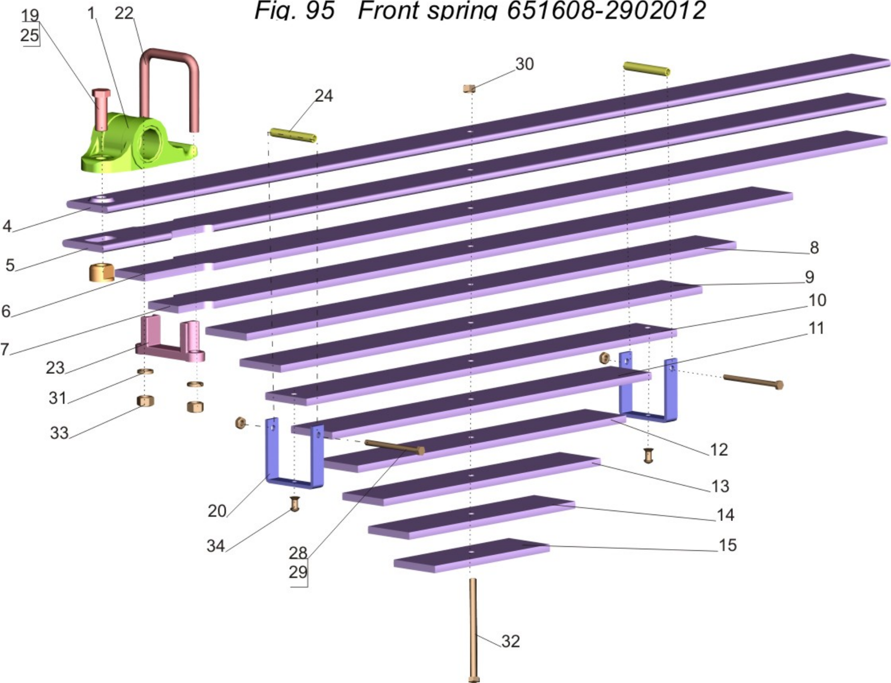
Рис. 95 Рессора передняя 651608-2902012
