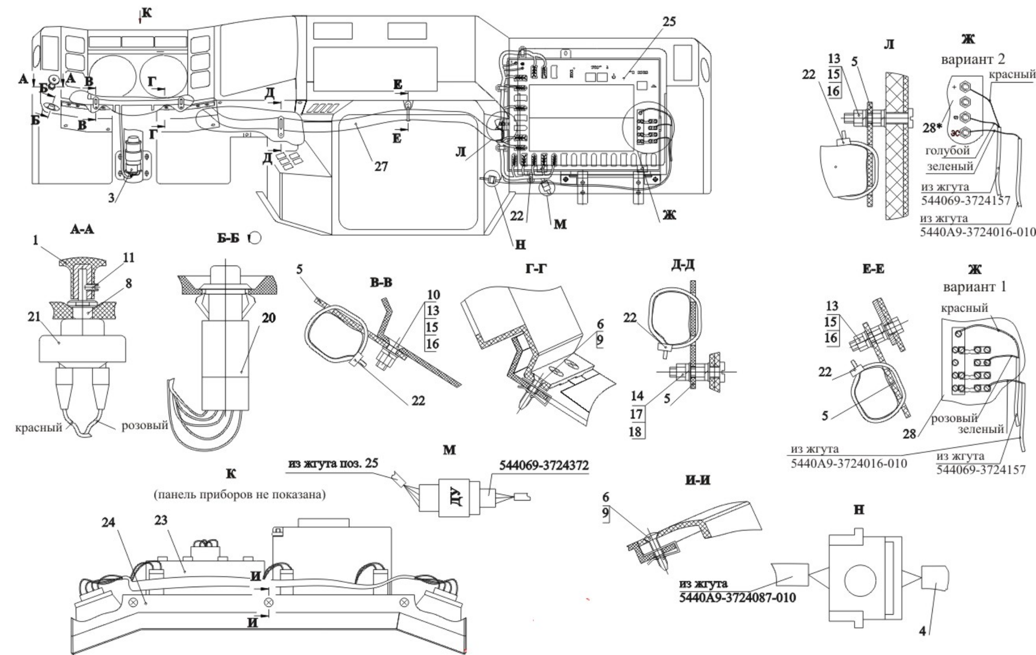
Рис. 198 Установка щитка приборов и коммутационной аппаратуры 6516А8-3800001 (-700) Fig. 198 Installation board devices and switching instrumentation 6516A8-3800001 (-700)
