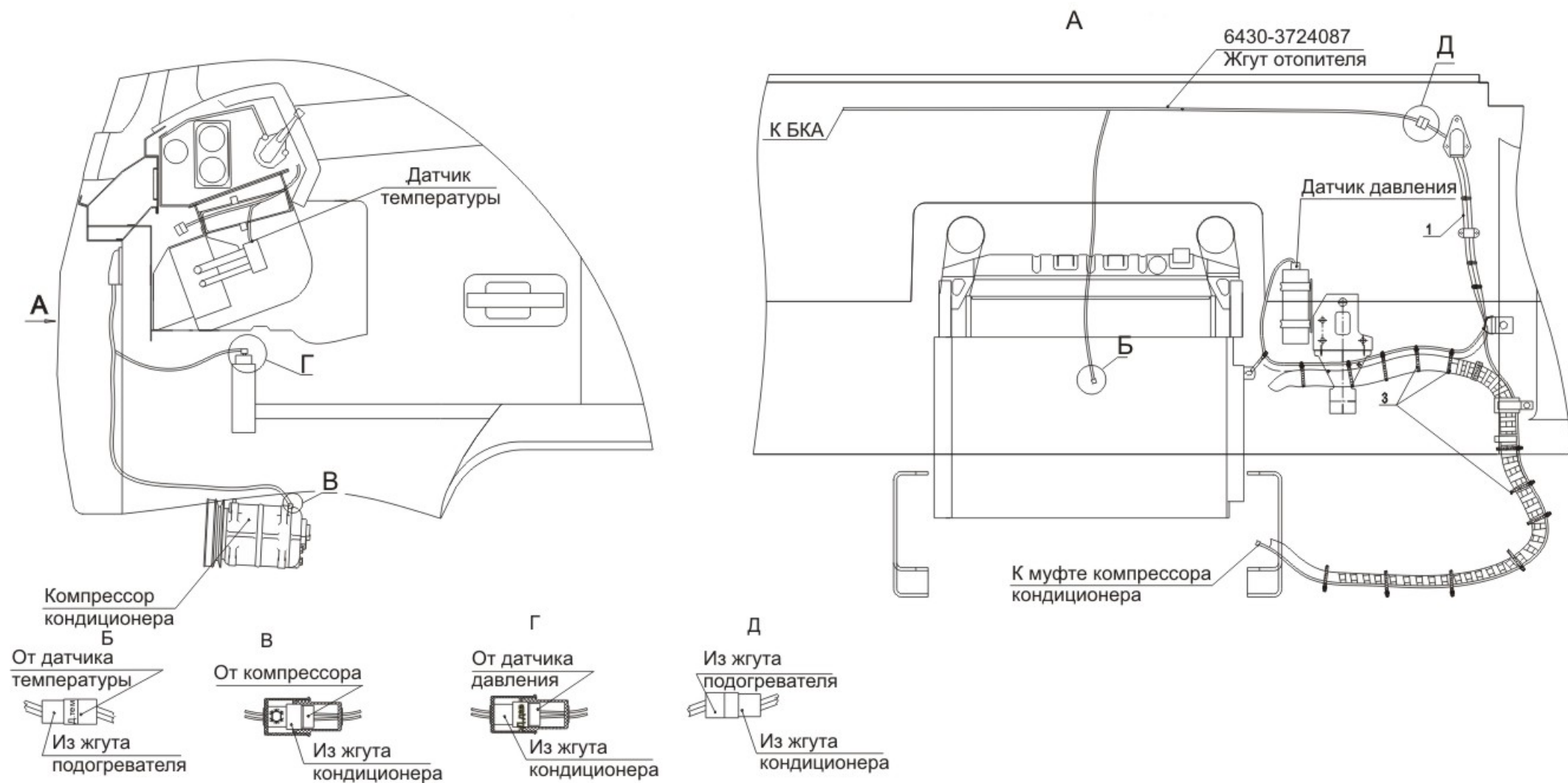
Рис. 187 Установка электрооборудования кондиционера 643008-3700092 Fig. 187 Installation of an electric equipment of the air conditioner 643008-3700092
