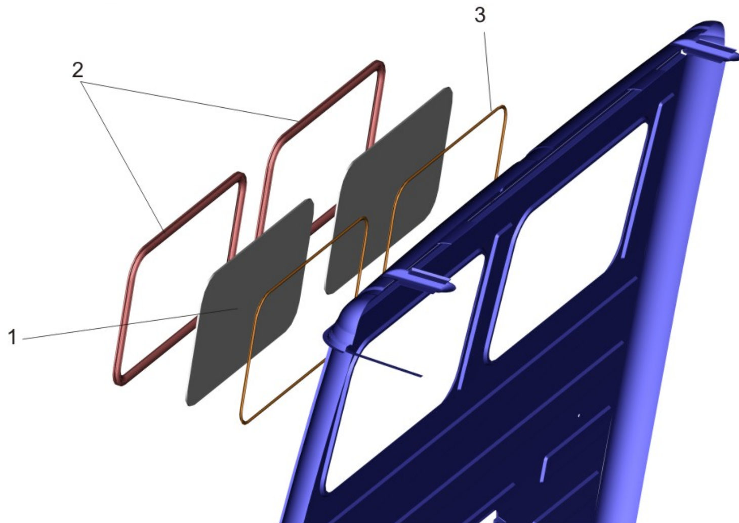
Рис. 223 Установки стекло задка 6501-5600015. Fig. 223 Installation a back glass 6501-5600015.
