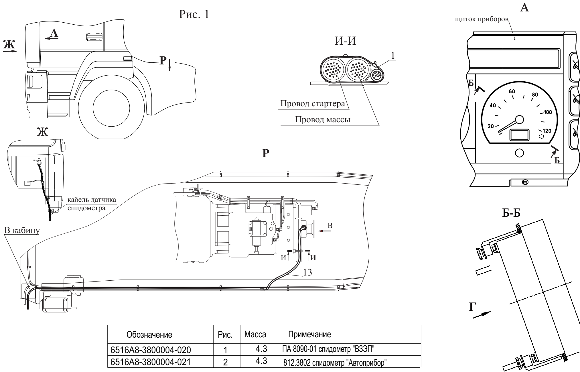
Рис. 200 Установка и пломбировка спидометра 6516А8-3800004-020, 6516А8-3800004-021 (лист 2) Fig. 200 Installation and identification seal of a speedometer 6516А8-3800004-020, 6516А8-3800004-021 (page 2)
