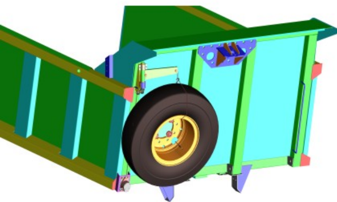
Рис. 125 Установка запасного колеса Fig. 125 Installation spare wheel
