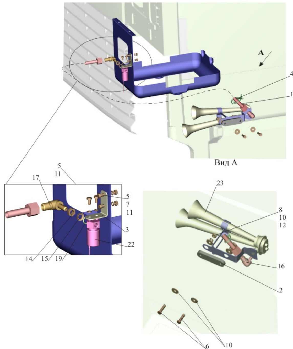
Рис.188 Установка пневмосигнала 6430-3700096, 6430-3700096-700 Fig. 188 Mounting of air horn 6430-3700096, 6430-3700096-700
