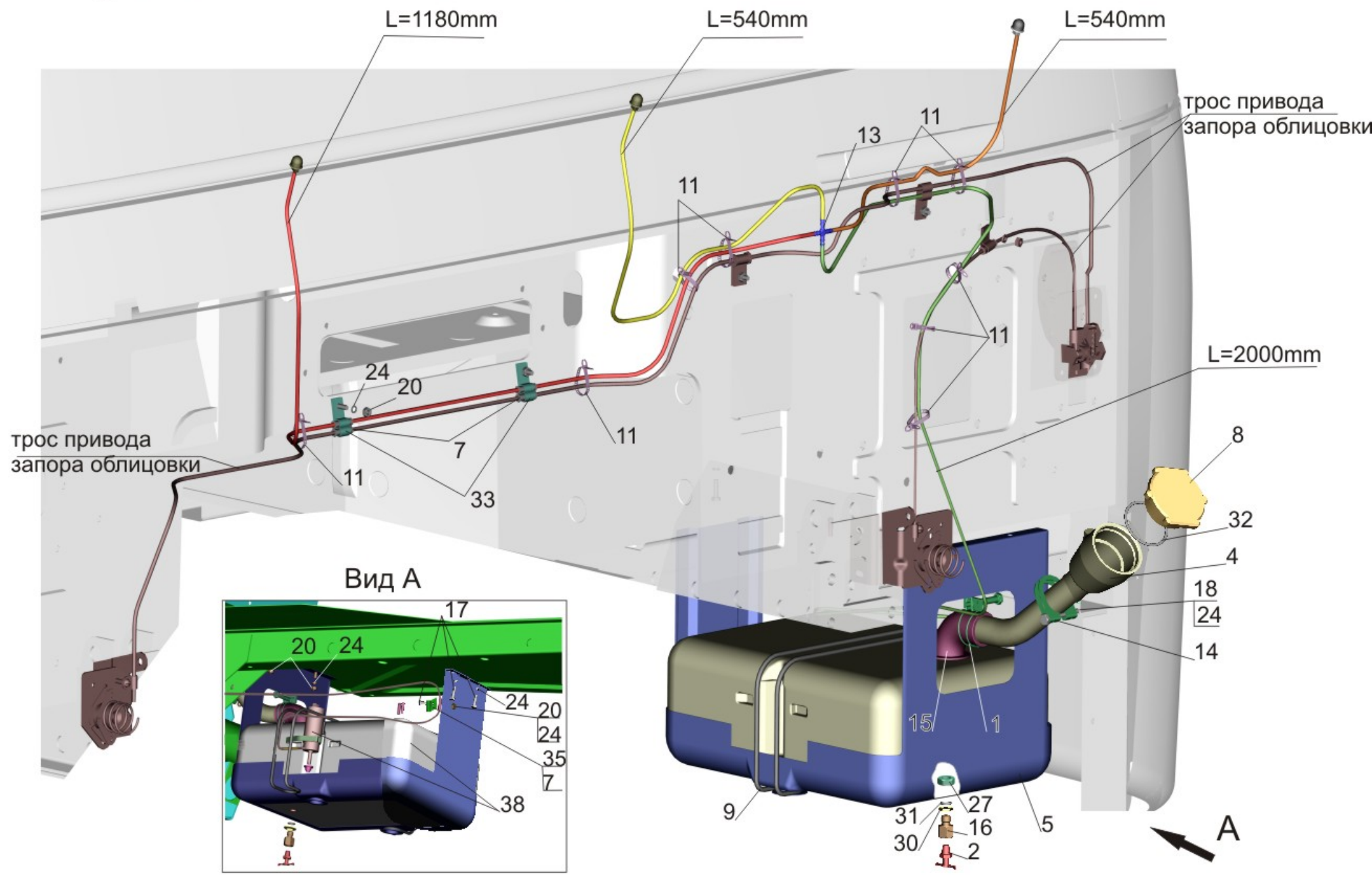
Fig. 221 Installation of washer 6430-5200008
