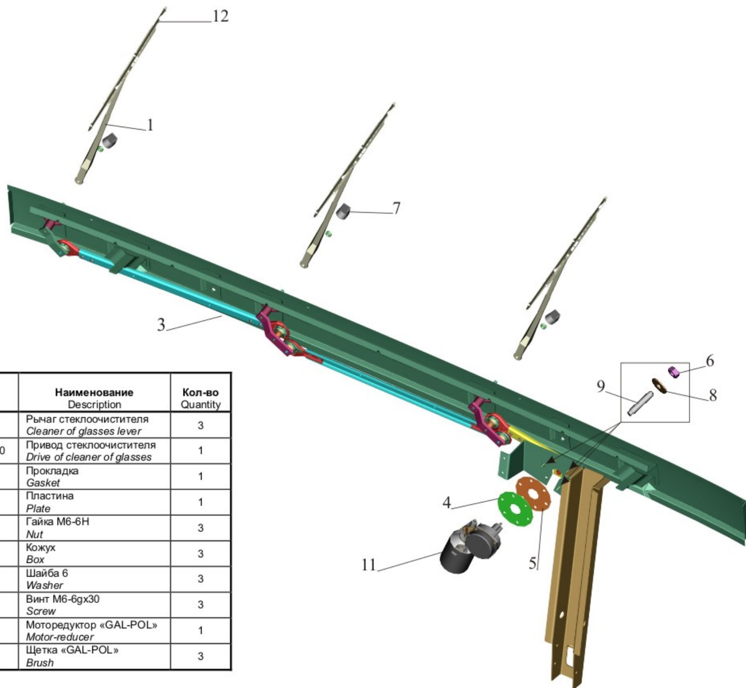
Рис. 234 Установка стеклоочистителя 6430-3700041-001 Fig. 234 Installation of cleaner of glasses 6430-3700041-001
