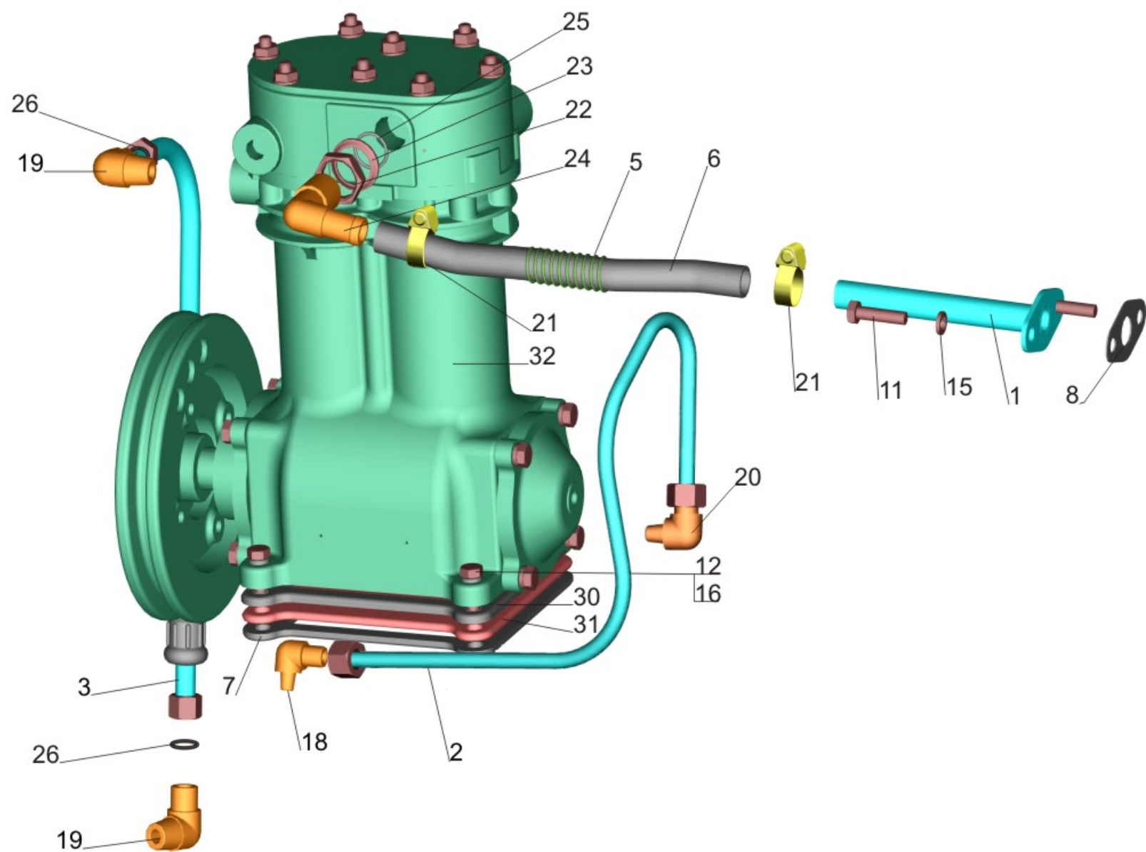
Рис. 155 Установка пневмокомпрессора 642208-3500014 Fig. 155 Installation of pneumatic compressor 642208-3500014
