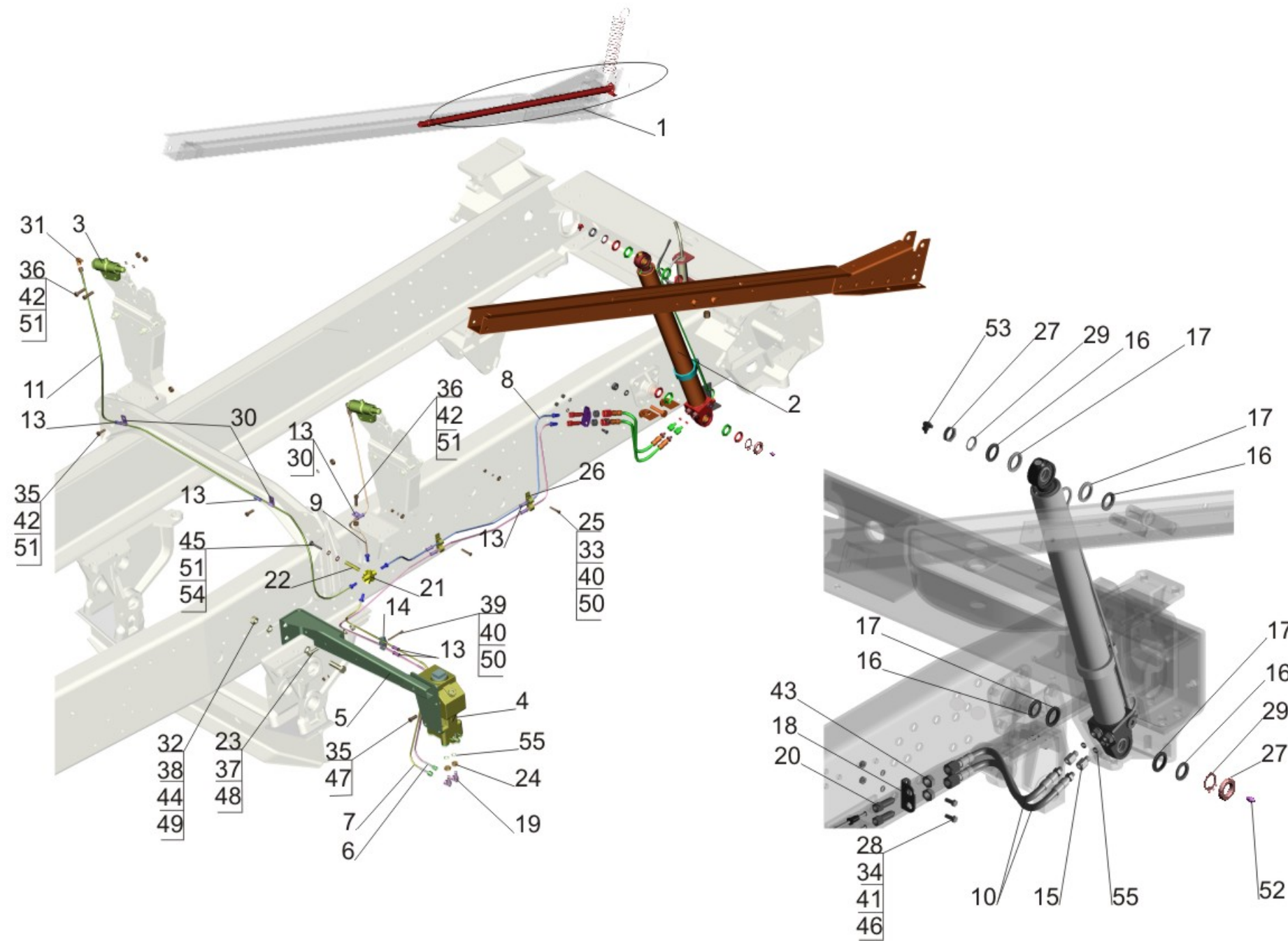
Рис. 236 Механизм подъема кабины 651608-5000040 Fig. 236 Cab tilting mechanism 651608-5000040
