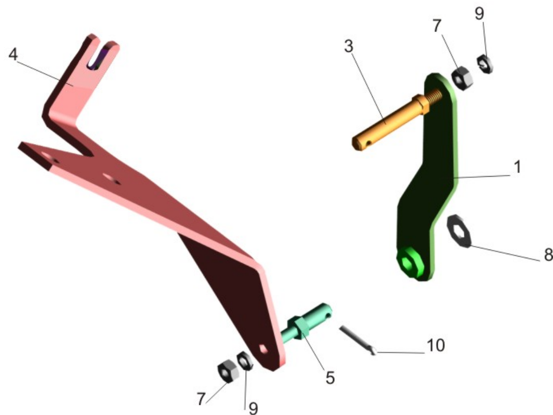
Fig. 20 Bracket 544010-1108135
