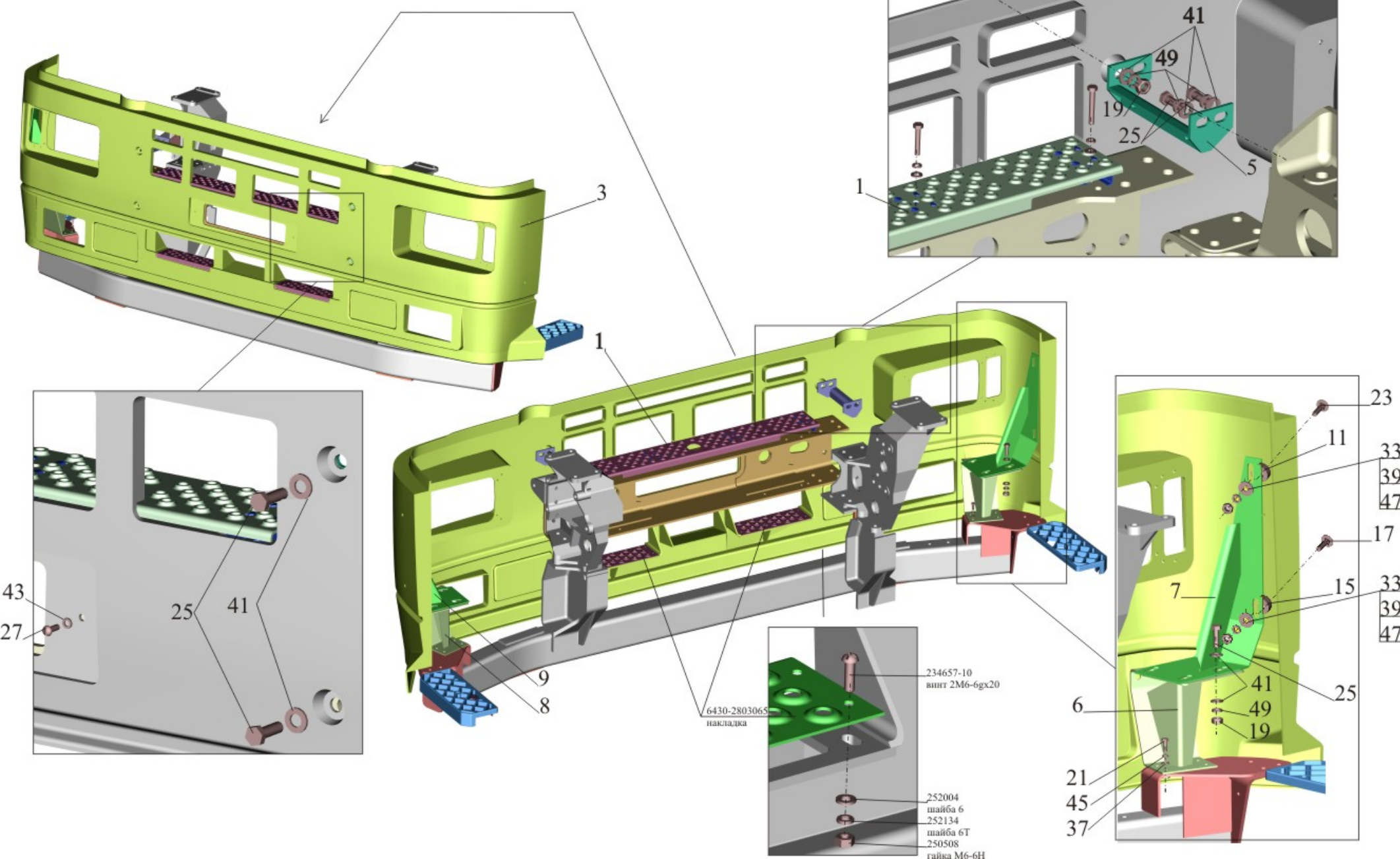
Рис. 85 Установка бампера 651608-2803006-011 Fig. 85 Installation bumper 651608-2803006-011
