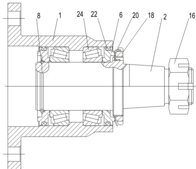
Рис. 124 Кронштейн 6516А8-3403150-000 Fig. 124 Bracket 6516A8-3403150-000
