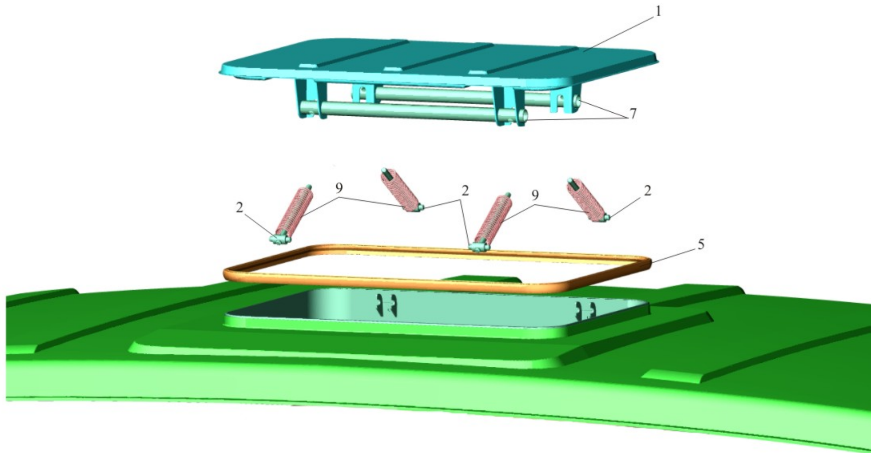
Рис. 225 Установка люка 6501-5700010 Fig. 225 Installation hatch 6501-5700010
