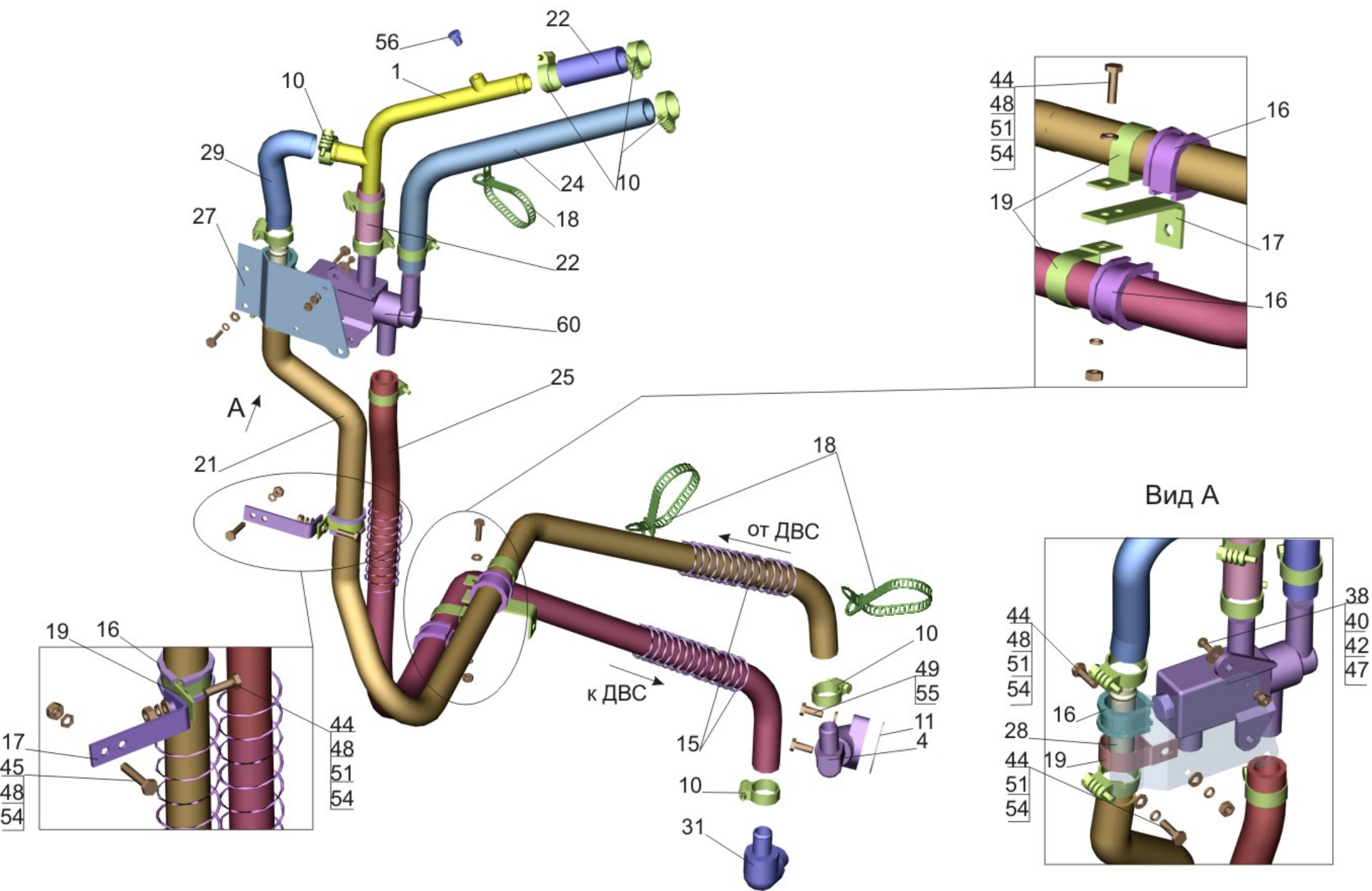
Рис. 262 Установка шлангов отопителя 544004-8100006-020 Fig. 262 Installation of hoses heater 544004-8100006-020
