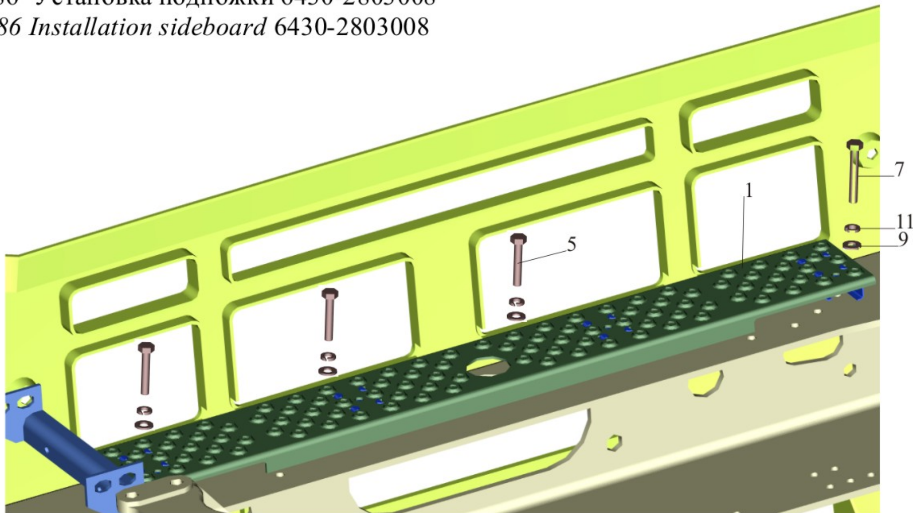
Рис. 86 Установка подножки 6430-2803008
