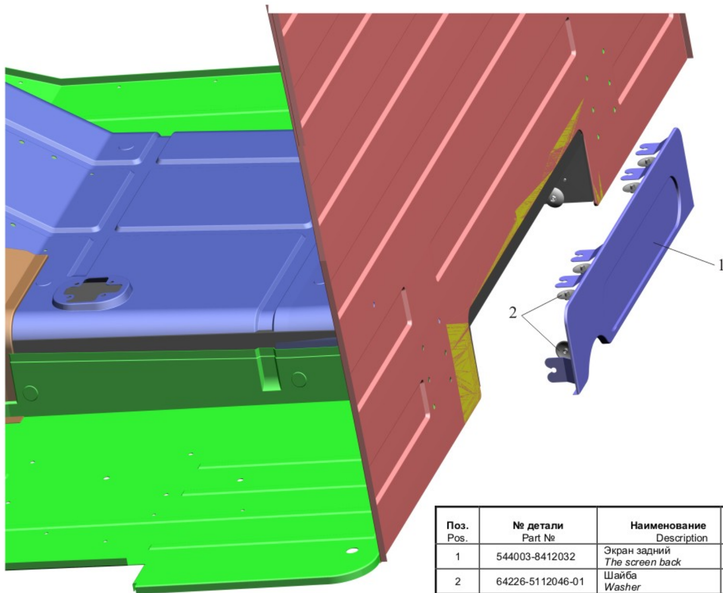
Рис. 274 Установка экранов 544003-8400026 Fig. 274 Installation of screens 544003-8400026
