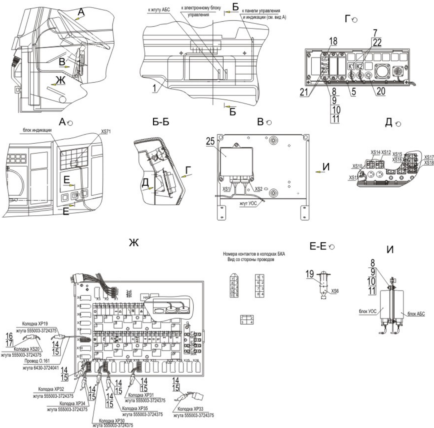
Рис.208 Установка СЭУД по кабине 555003-3800066 Fig.208 Installation system electronic engine control
