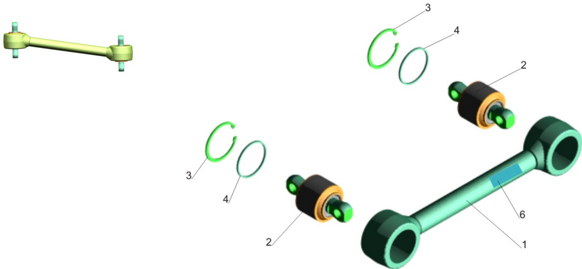
Fig.102 Torque rod 64221-2919014
