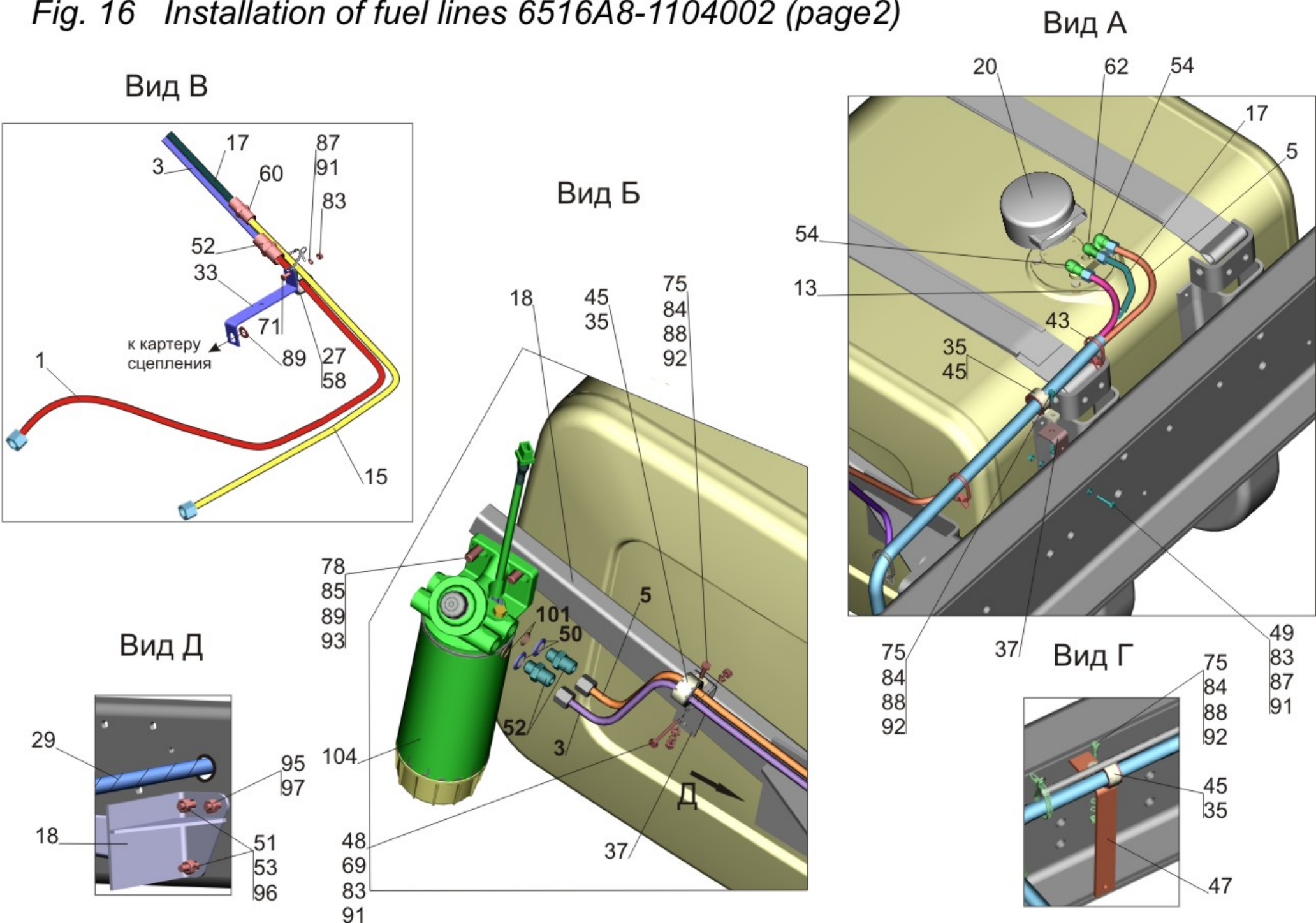
Рис. 16 Крепление топливопроводов 6516А8-1104002 (лист 2)
