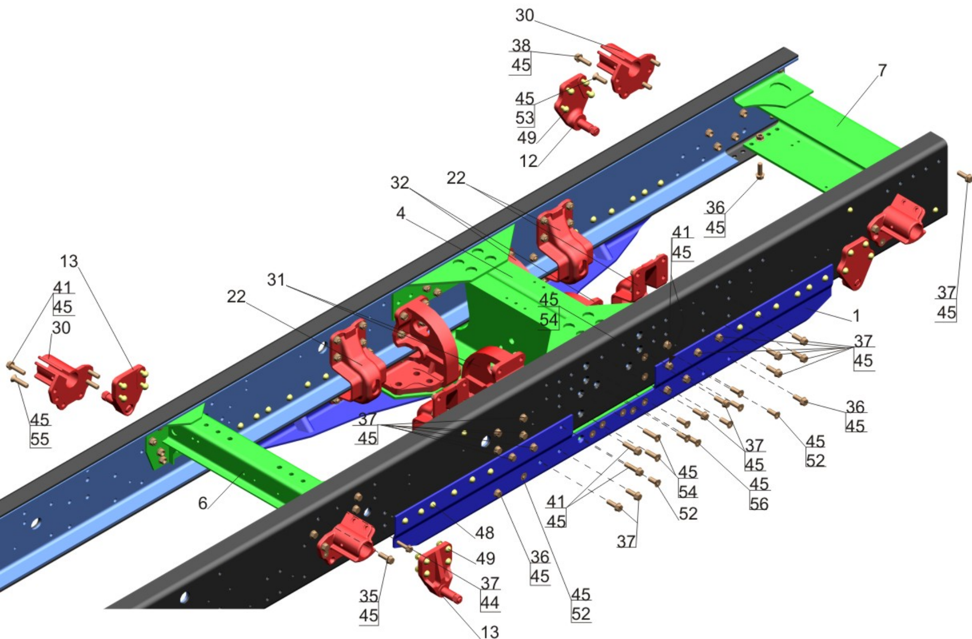
Fig. 88 Frame 6516A8-2801002 (page 2)
