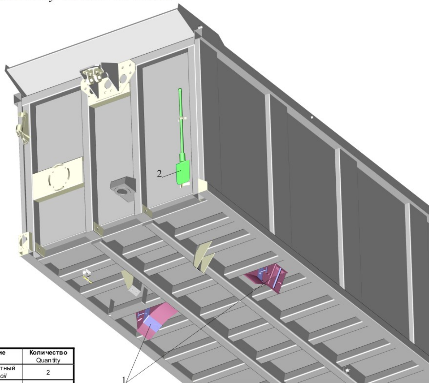
Рис. 209 Установка принадлежностей 651608-3900011 Fig. 209 Installation accessory 651608-3900011
