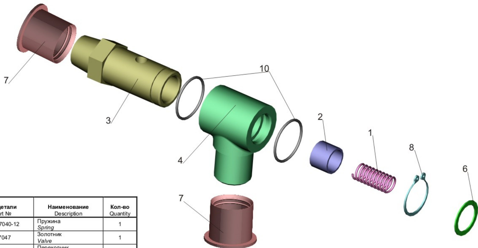
Рис. 290 Клапан 651608-8603508. Fig. 290 Valve 651608-8603508.
