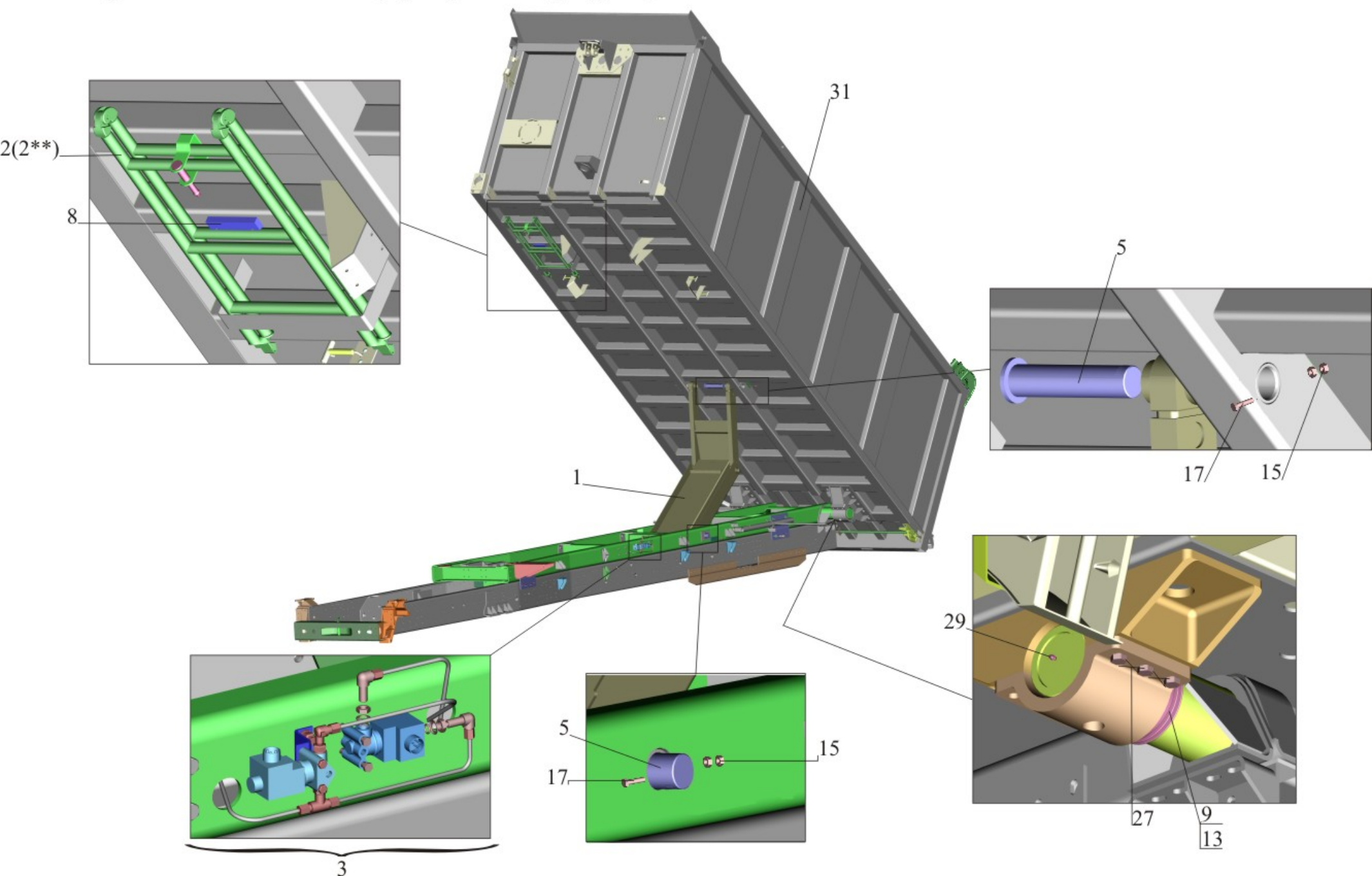
Рис. 276 Установка платформы (лист 2) Fig. 276 Installation of platform (page 2)
