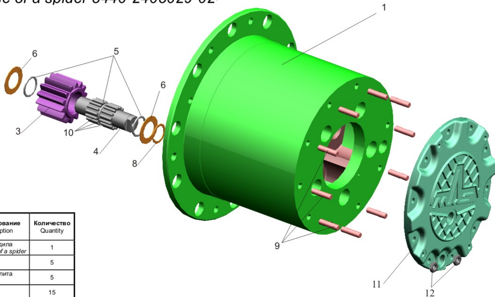
Рис.55 Корпус водила 5440-2405029-020 Fig.55 The case of a spider 5440-2405029-020
