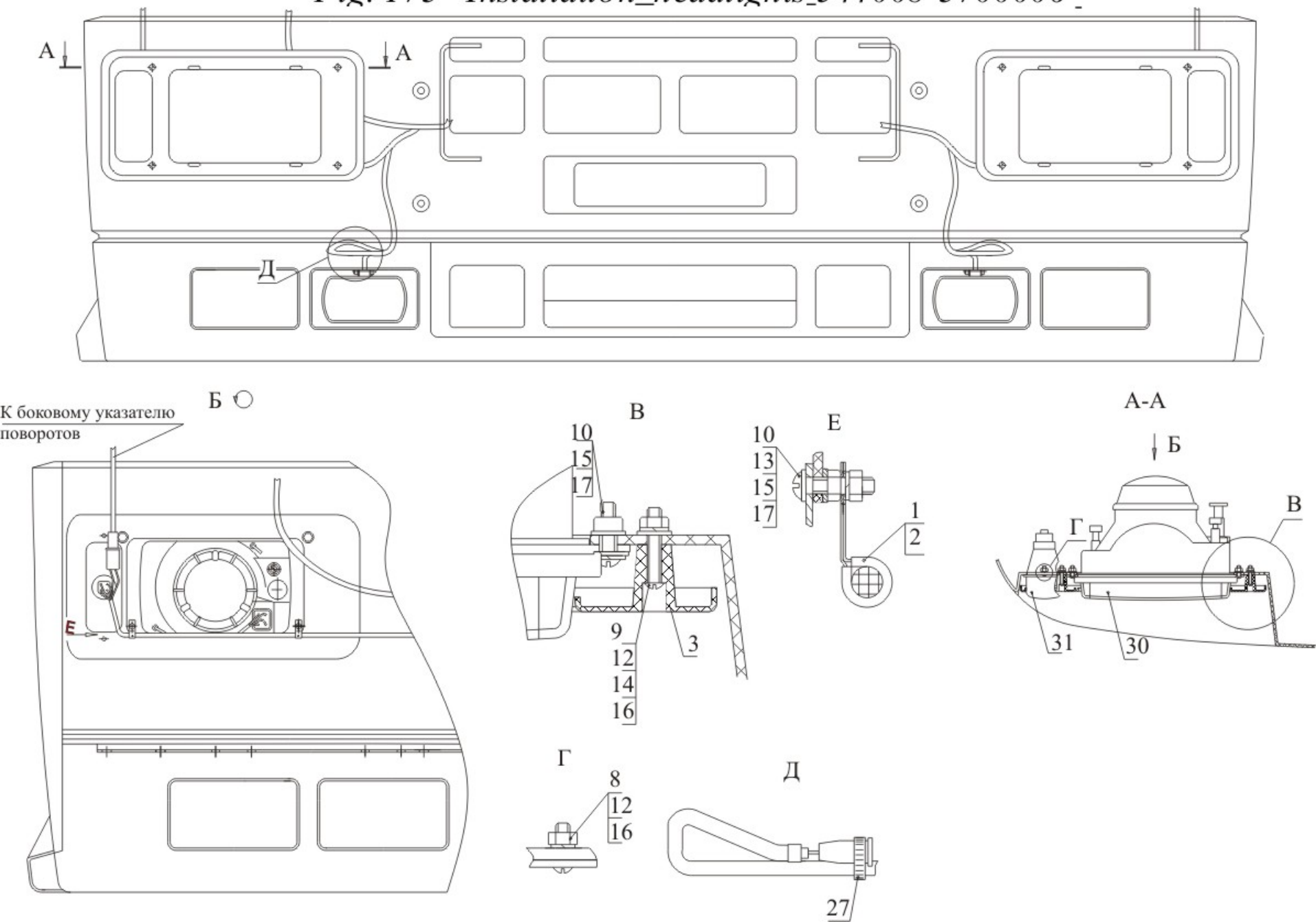
Рис. 173 Установка фар 544008-3700006 Fig. 173 Installation_headlights_544008-3700006
