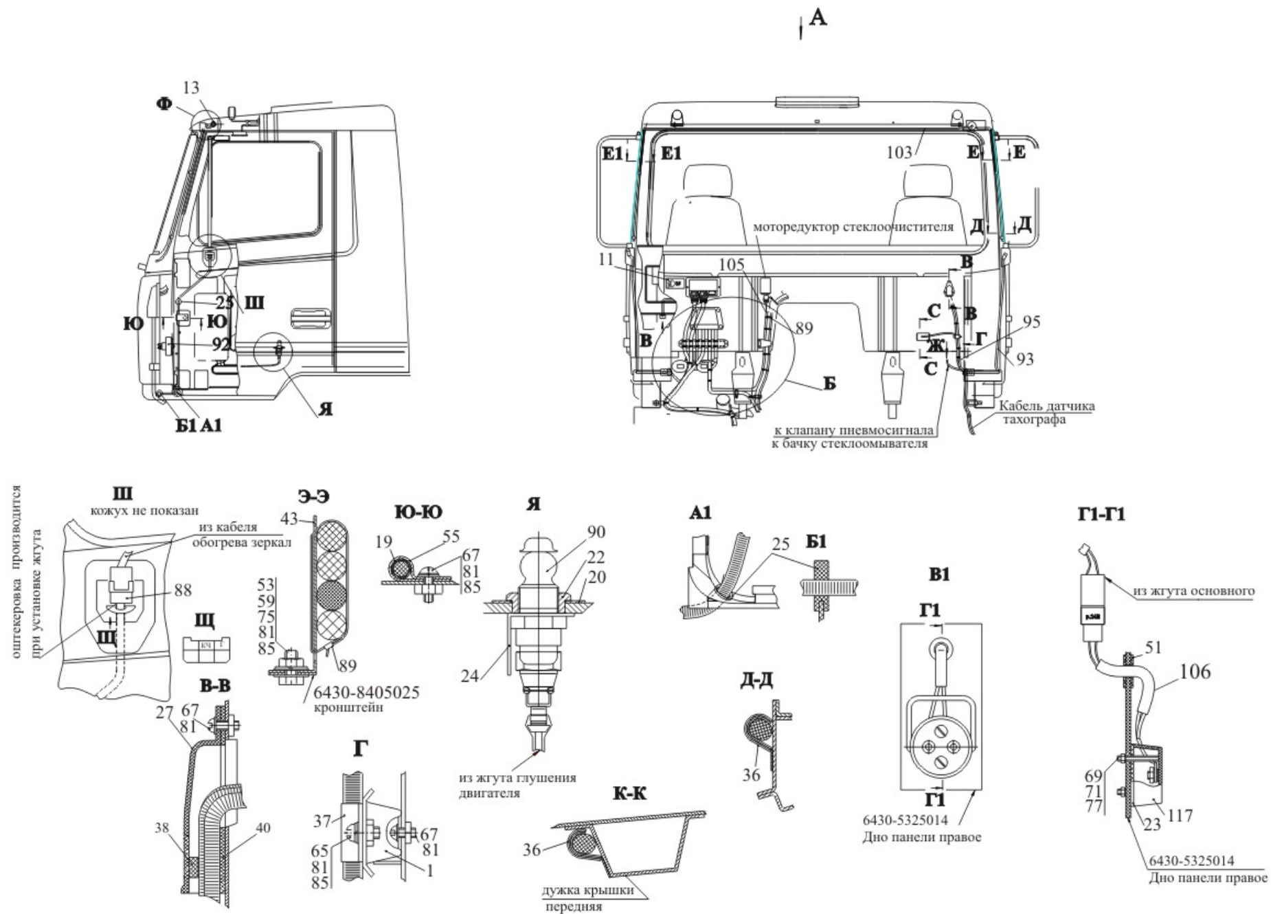
Рис.181 Установка электрооборудования в кабине 555002-3700076(-700) (лист 1) Fig.181 Installation of an electrical equipment in a cabin 555002-3700076(-700) (page 1)
