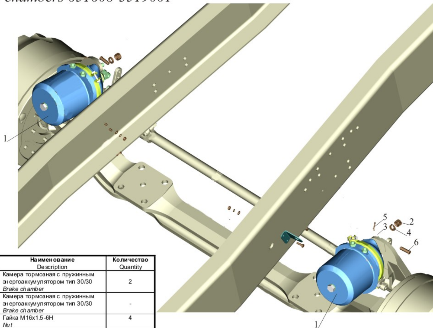
Рис. 164 Крепление тормозных камер 651608-3519001 Fig. 164 Mounting of brake chambers 651608-3519001
