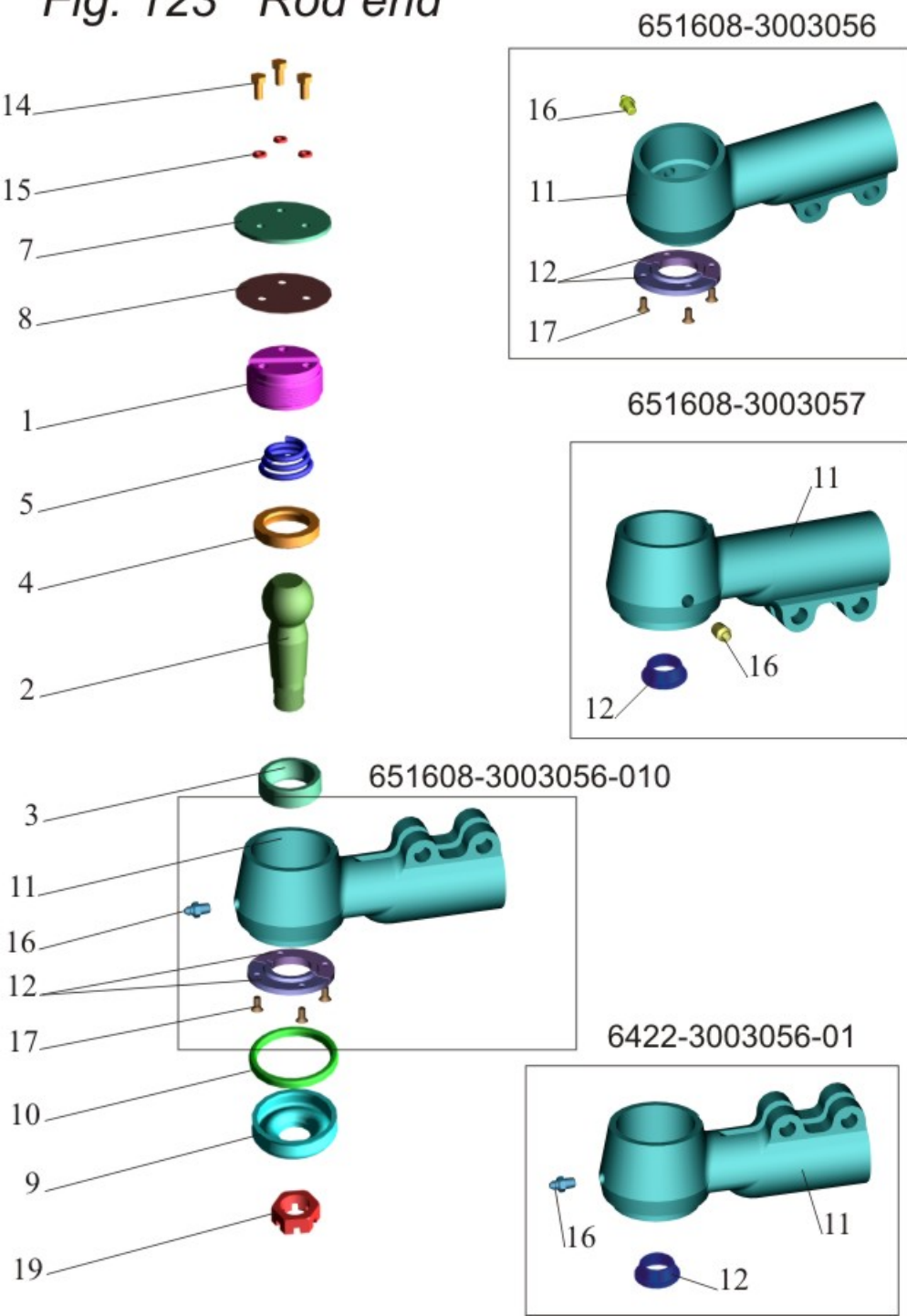
Рис.123 Наконечник Fig. 123 Rod end
