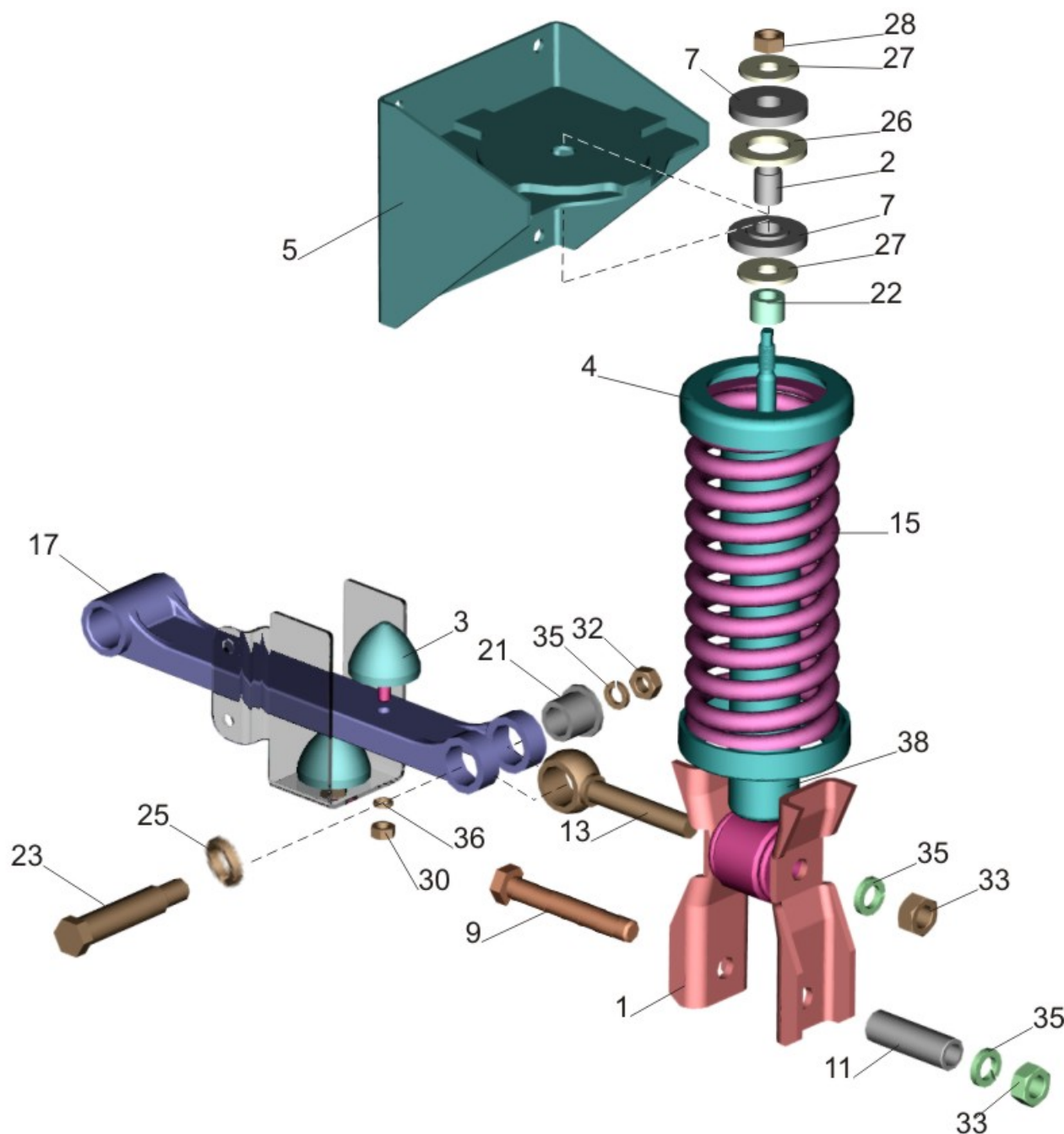
Рис. 217 Заднее подрессоривание кабины 6501-5001802-010 Fig. 217 Cab rear springing 6501-5001802-010
