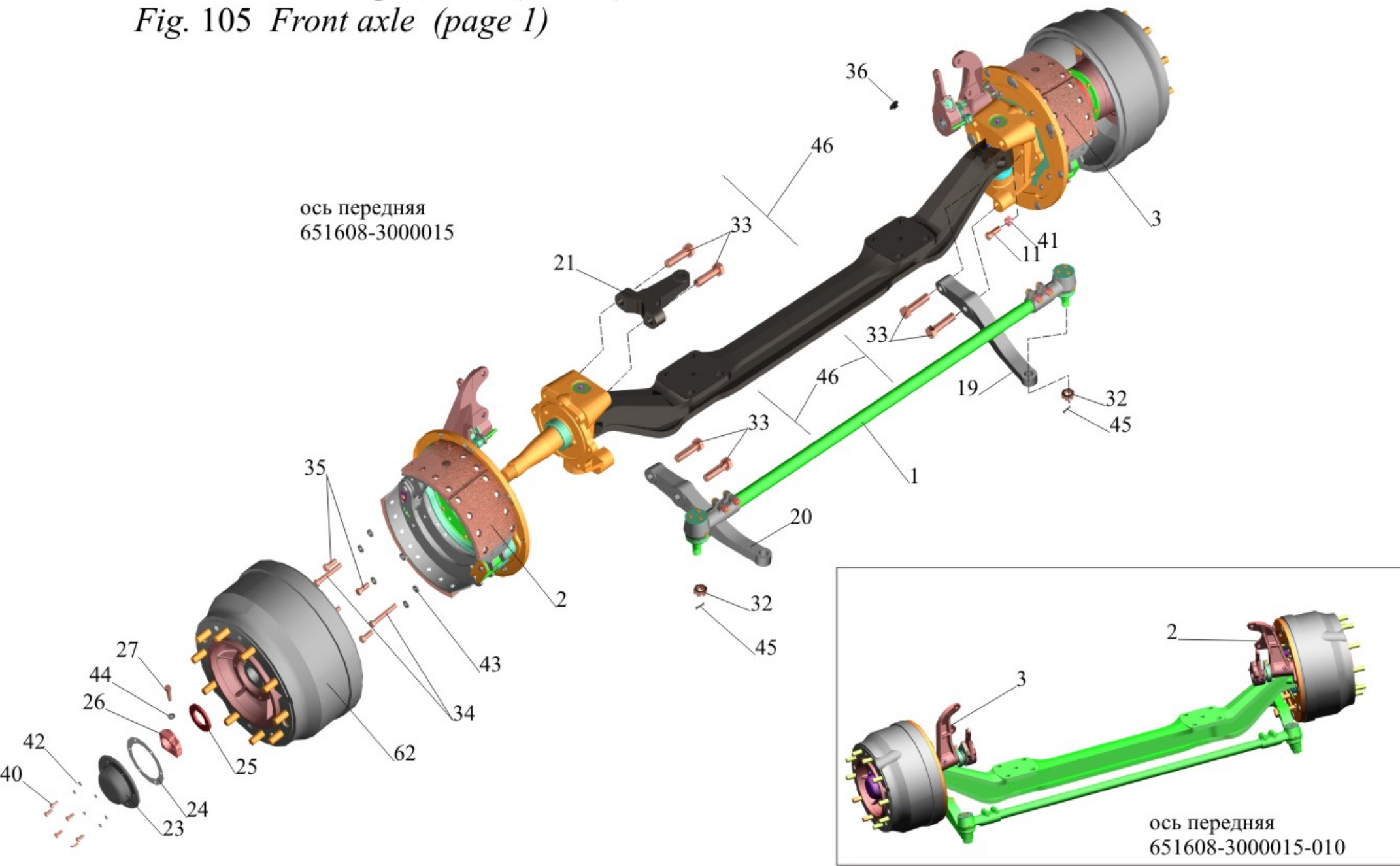
Рис. 105 Ось передняя (лист 1)
