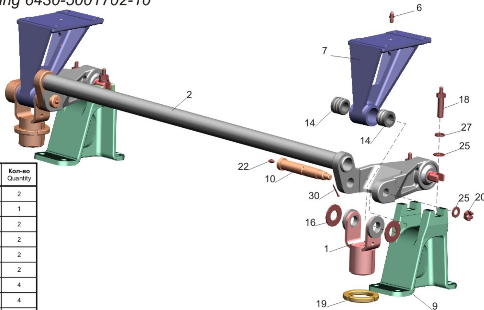
Рис. 215 Переднее подрессоривание 6430-5001702-10 Fig. 215 Front spriging 6430-5001702-10
