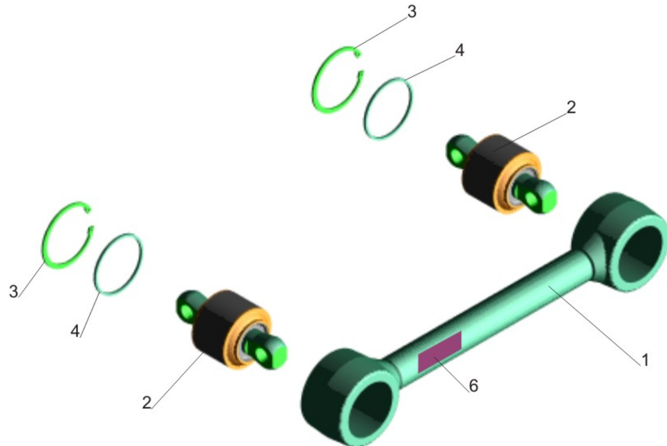
Fig.103 Torque rod 6430-2919014
