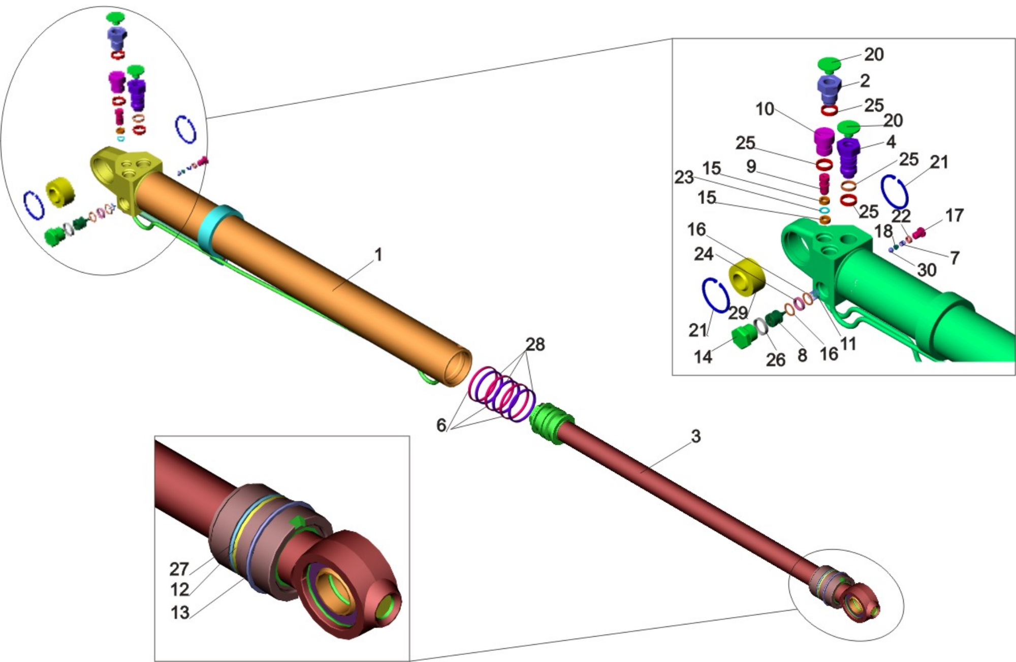
Рис. 241 Гидроцилиндр 6430-5003010 Fig. 241 Hydrocylinder 6430-5003010
