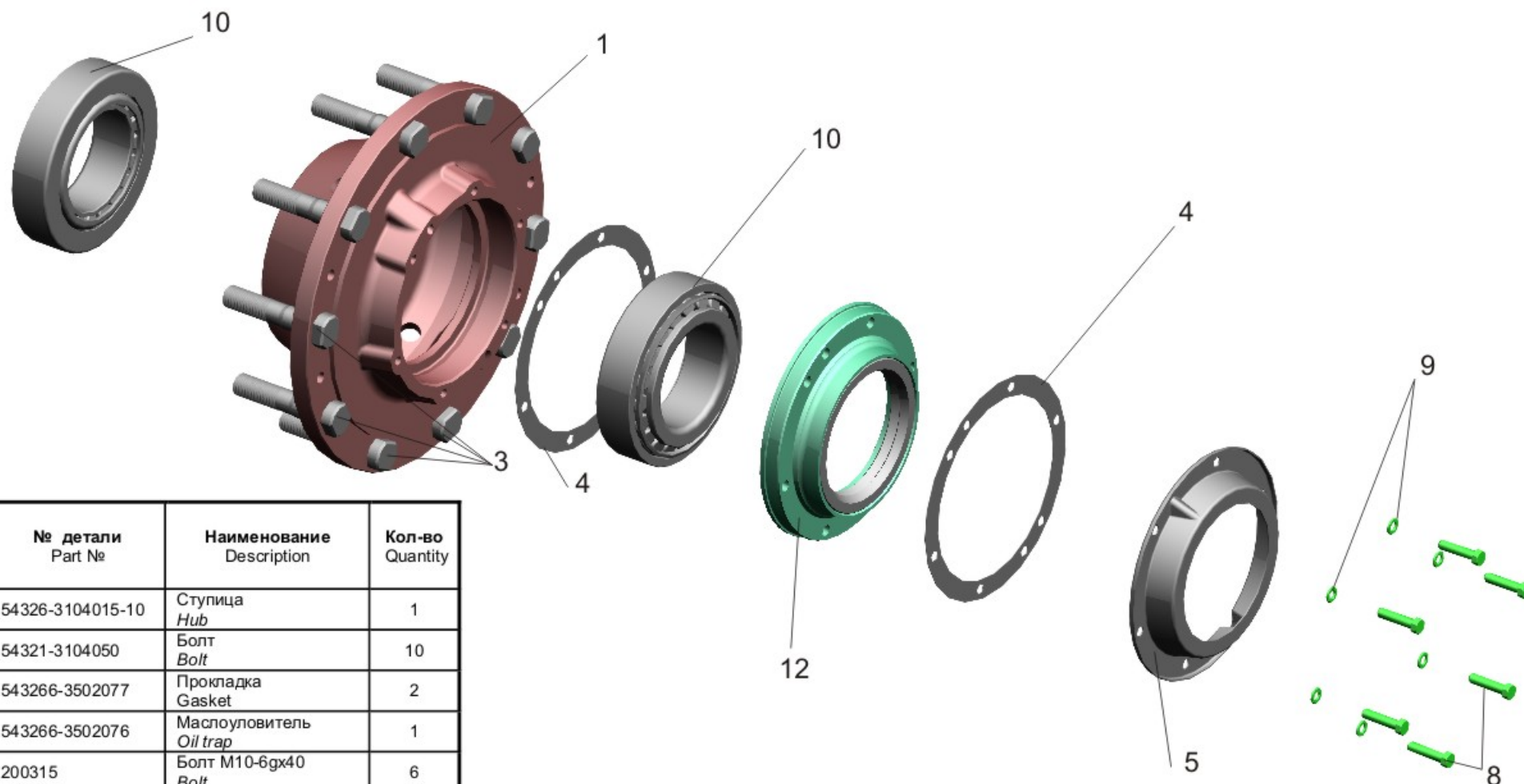
Рис. 82 Ступица с крышкой 54326-3104006-601 Fig. 82 Rear axle hub 54326-3104006-601
