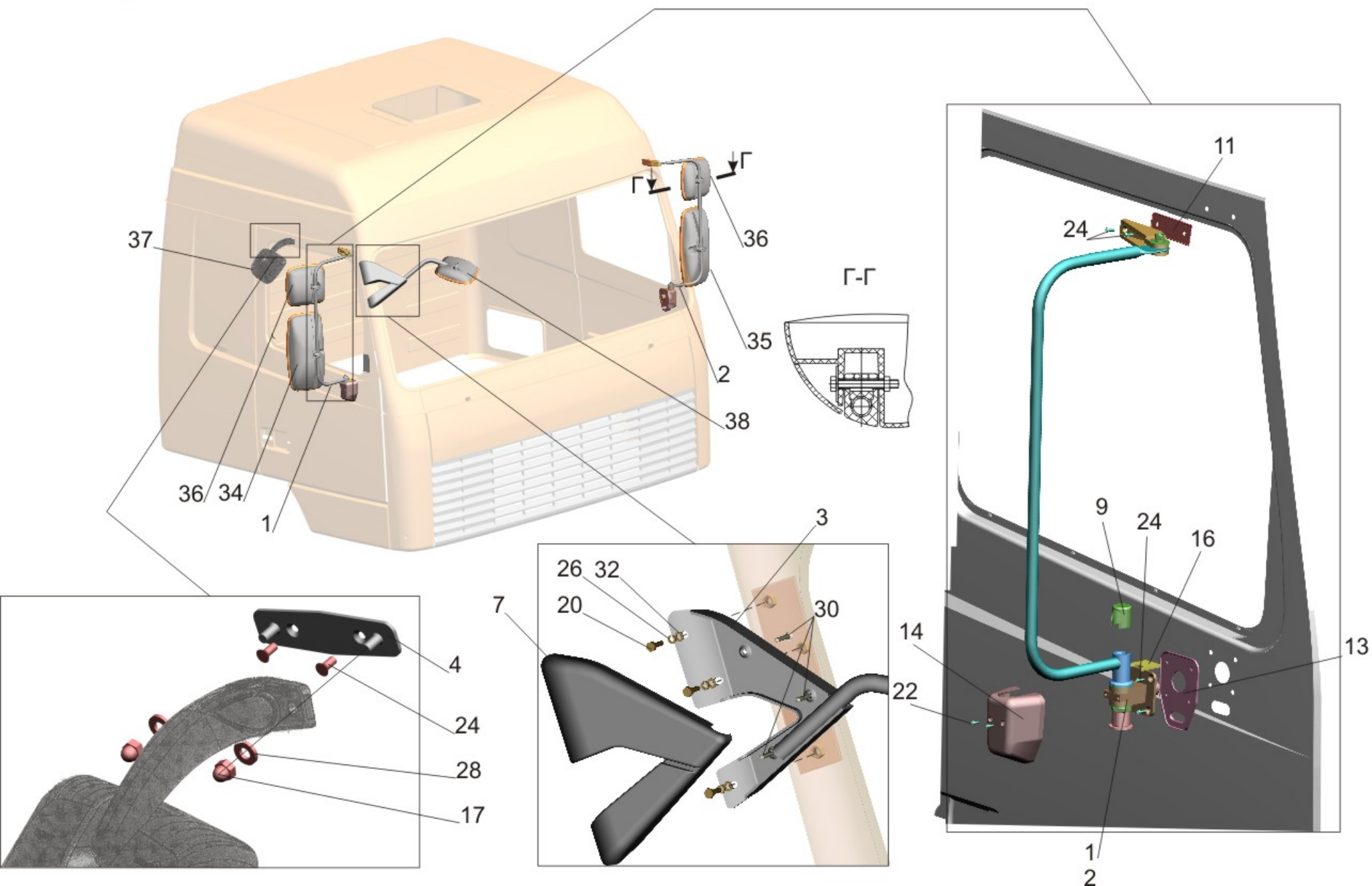
Рис. 229 Установка зеркал 6430-8200005-020 Fig. 229 Installation mirrors 6430-8200005-020
