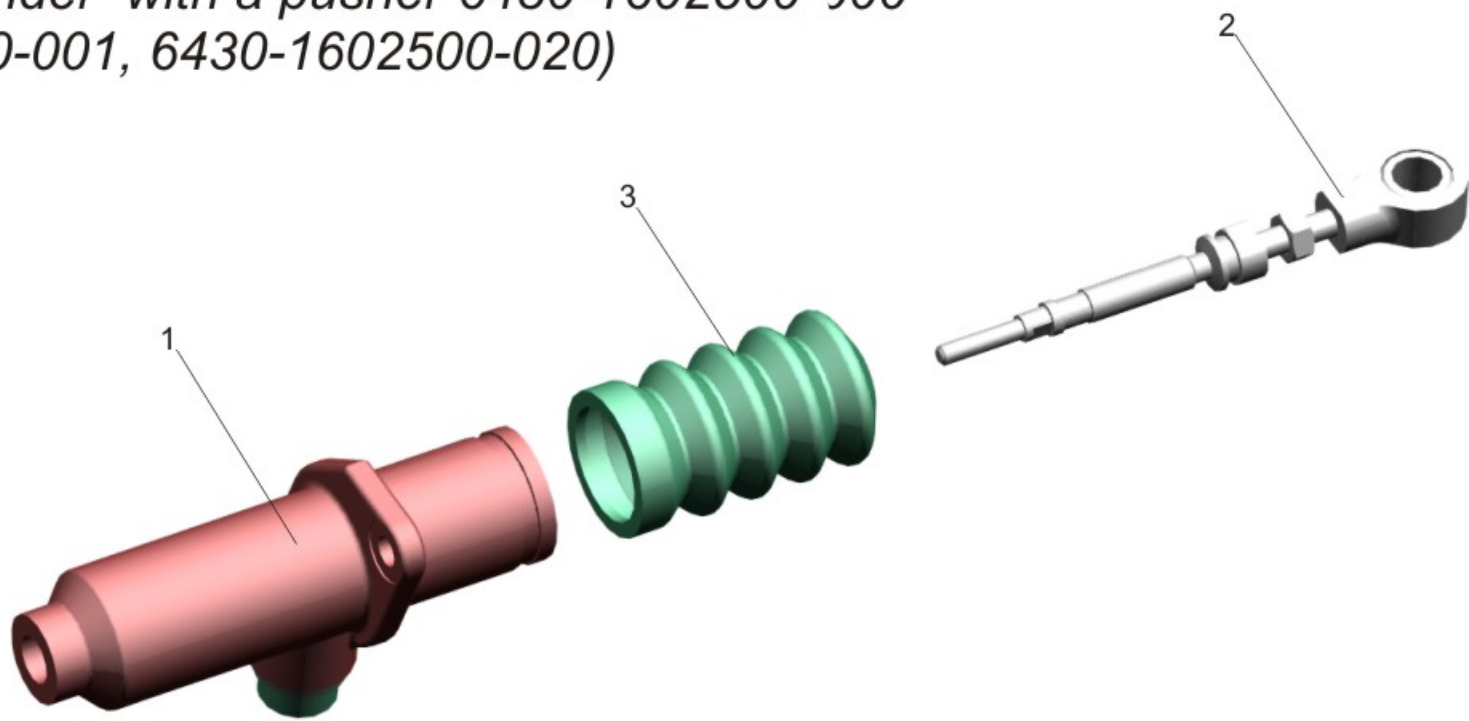
Рис. 34 Цилиндр подпедальный с толкателем 6430-1602500-000 (6430-1602500-001, 6430-1602500-020)
