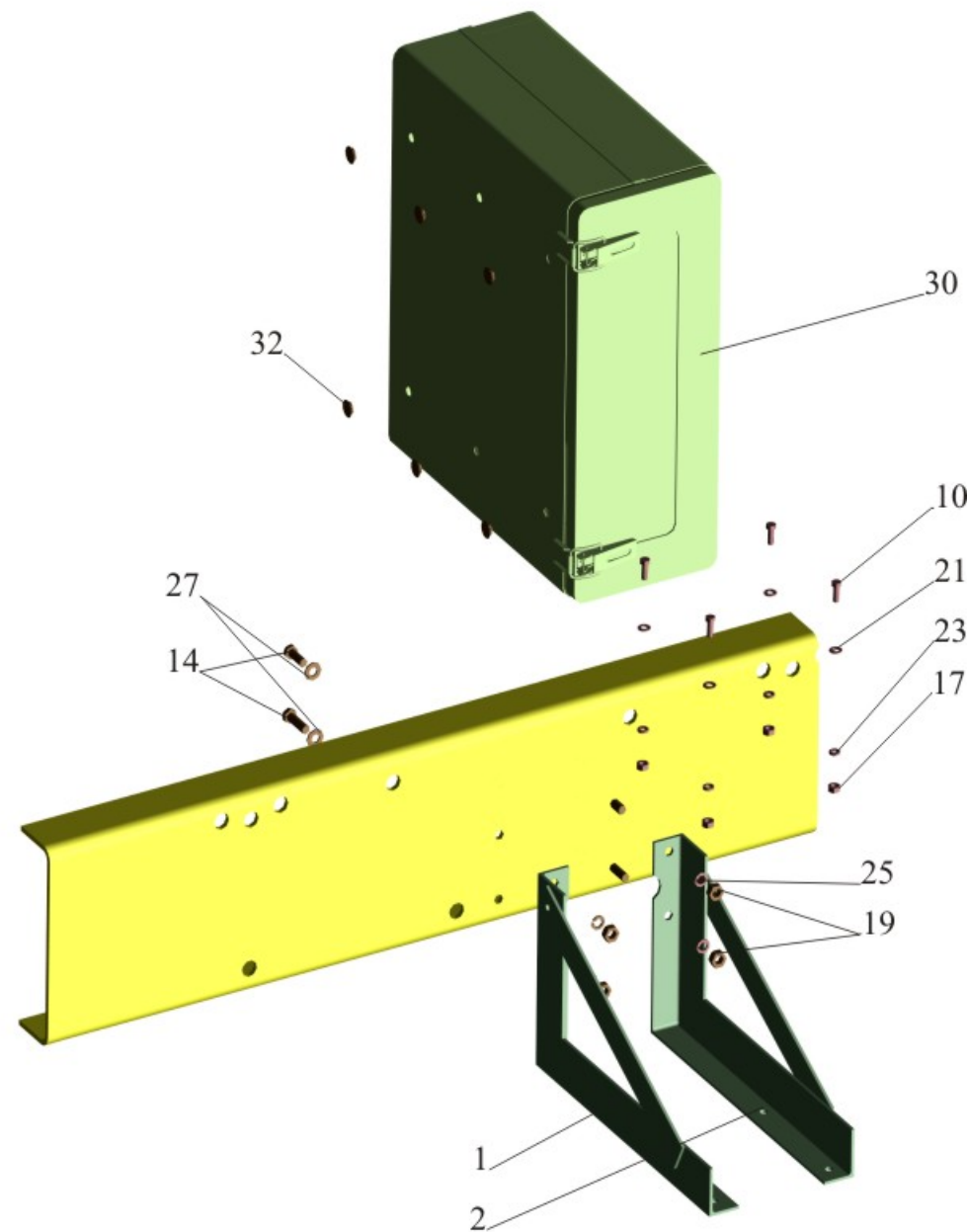
Рис. 281 Установка инструментального ящика 551608-8500009 Fig. 281 The tools box installation 551608-8500009
