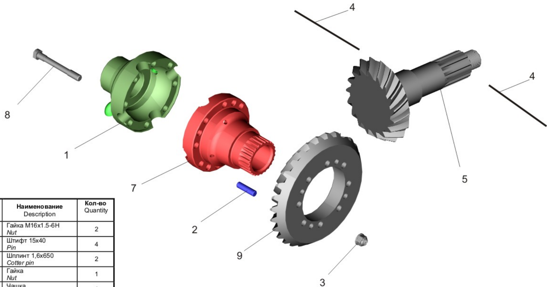
Рис. 71 Шестерни ведущая и ведомая (комплект для запчастей) 54323-2402020-020 Fig. 71 Drive and driven pinions (set for spare parts) 54323-2402020-020
