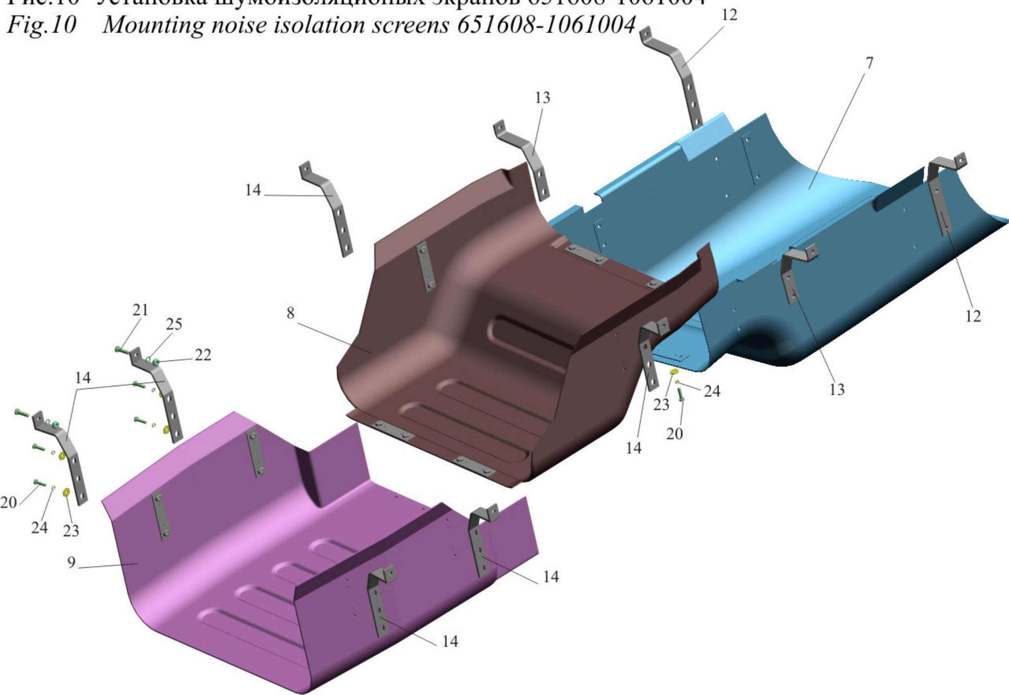
Рис.10 Установка шумоизоляционных экранов 651608-1061004
