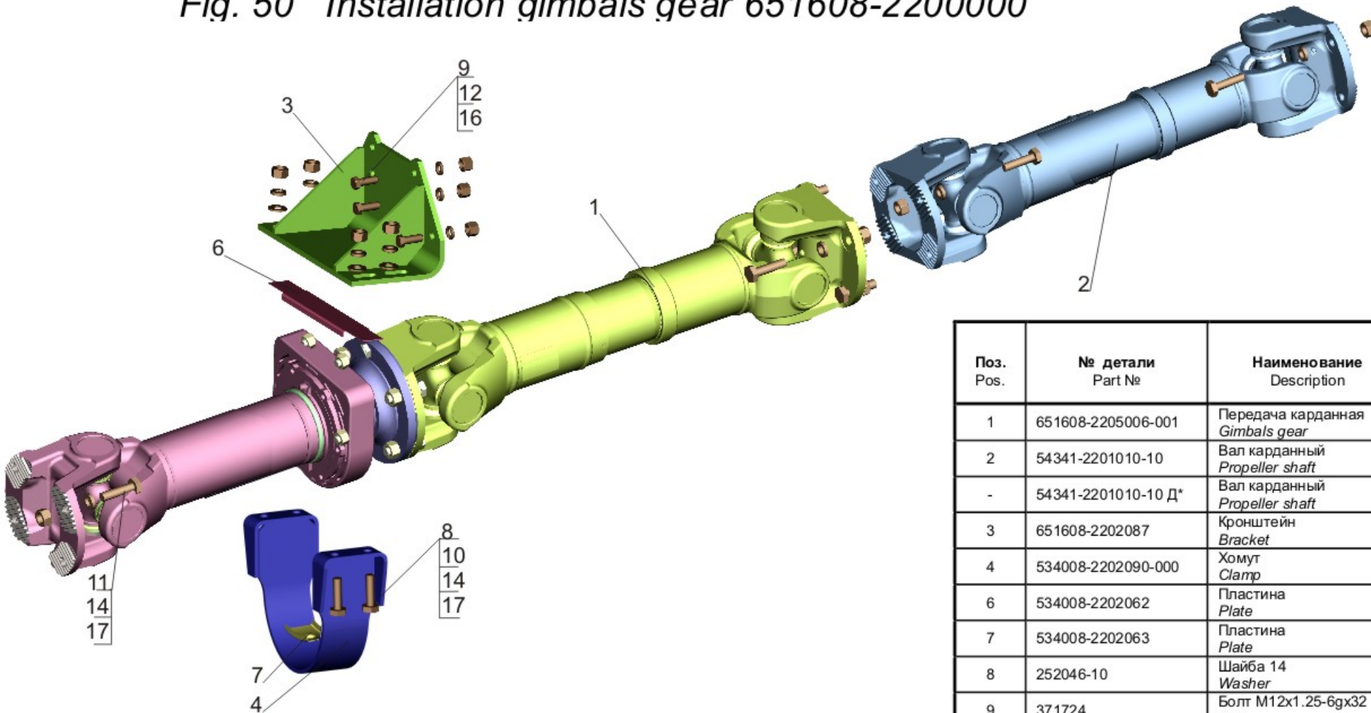
Рис. 50 Установка карданной передачи 651608-2200000
