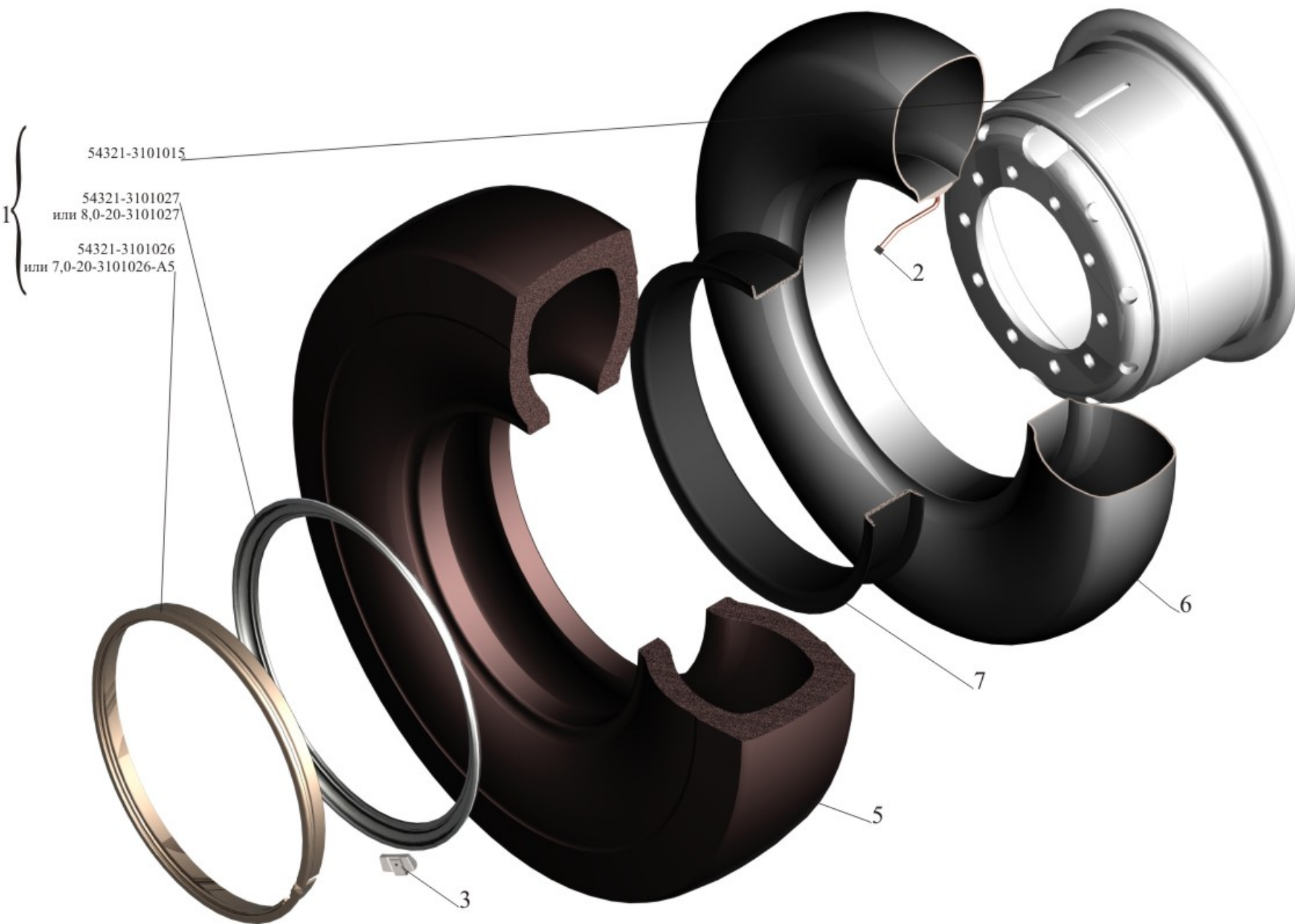
Рис. 131 Колесо и шина Fig. 131 Wheel and trunk
