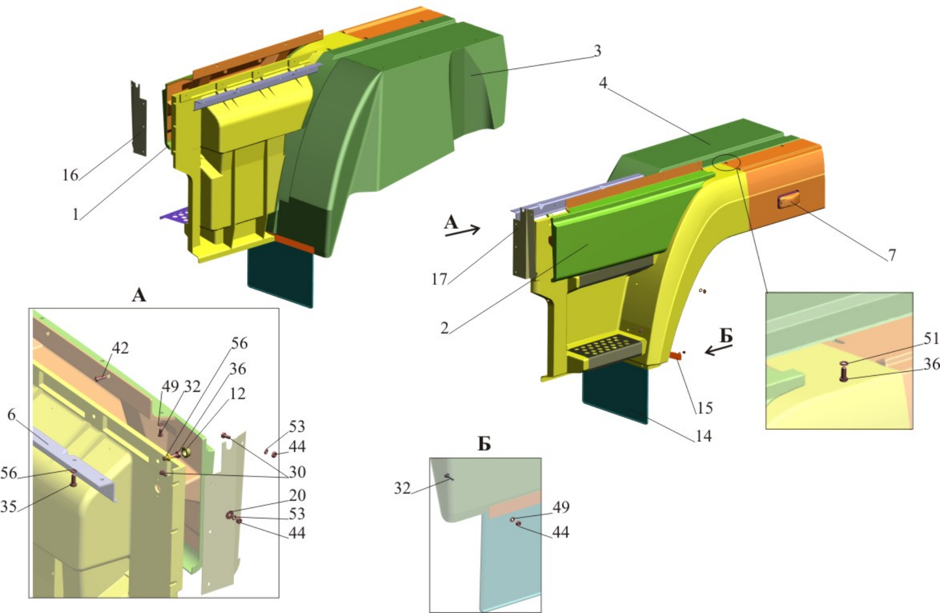
Рис. 271 Установка оперения 6516А8-8400020-010 Fig. 271 Installation of plumage 6516А8-8400020-010
