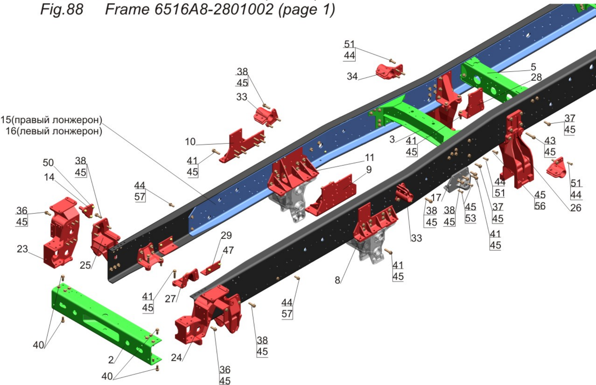
Рис.88 Рама 6516A8-2801002 (лист 1)
