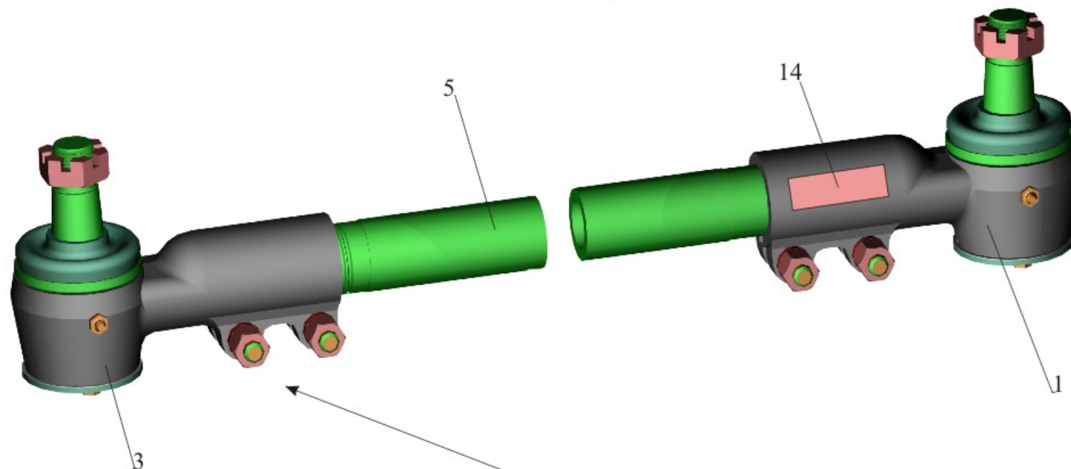
Рис.107 Тяга поперечная 64221-3003052, 64221-3003052-10 Fig. 107 Pull-rod cross 64221-3003052, 64221-3003052-10
