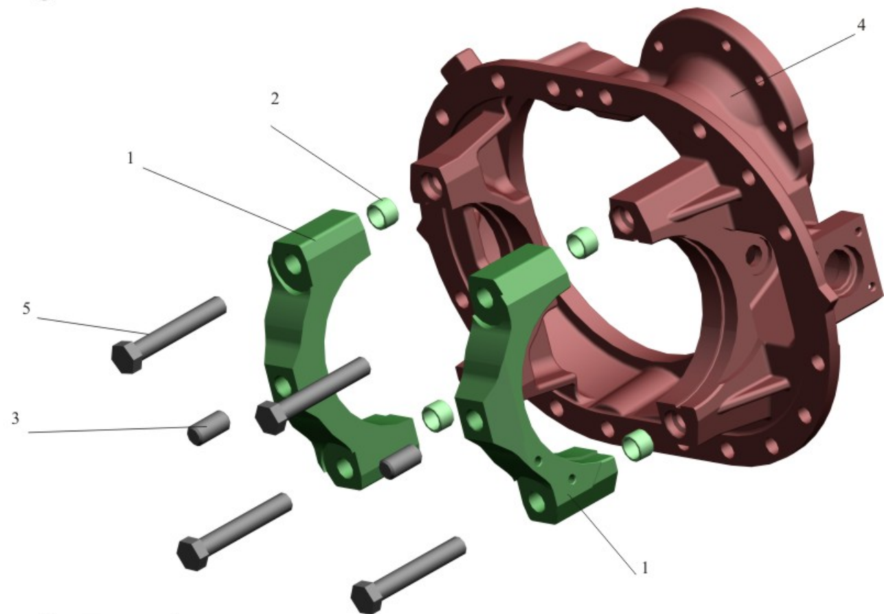
Рис.75 Картер редуктора 64221-2502015-010 Fig.75 Reducer gear housing 64221-2502015-010
