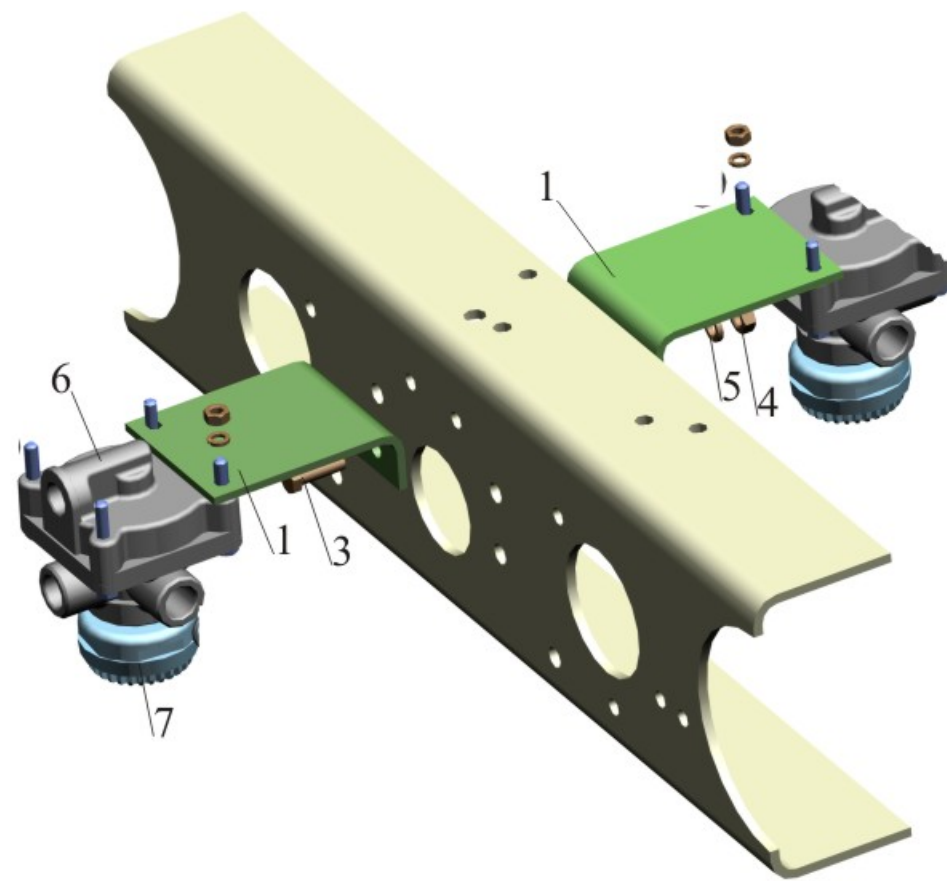
Рис. 161 Крепление клапанов ускорительных 651608-3518004 Fig. 161 Installation of relay valves 651608-3518004
