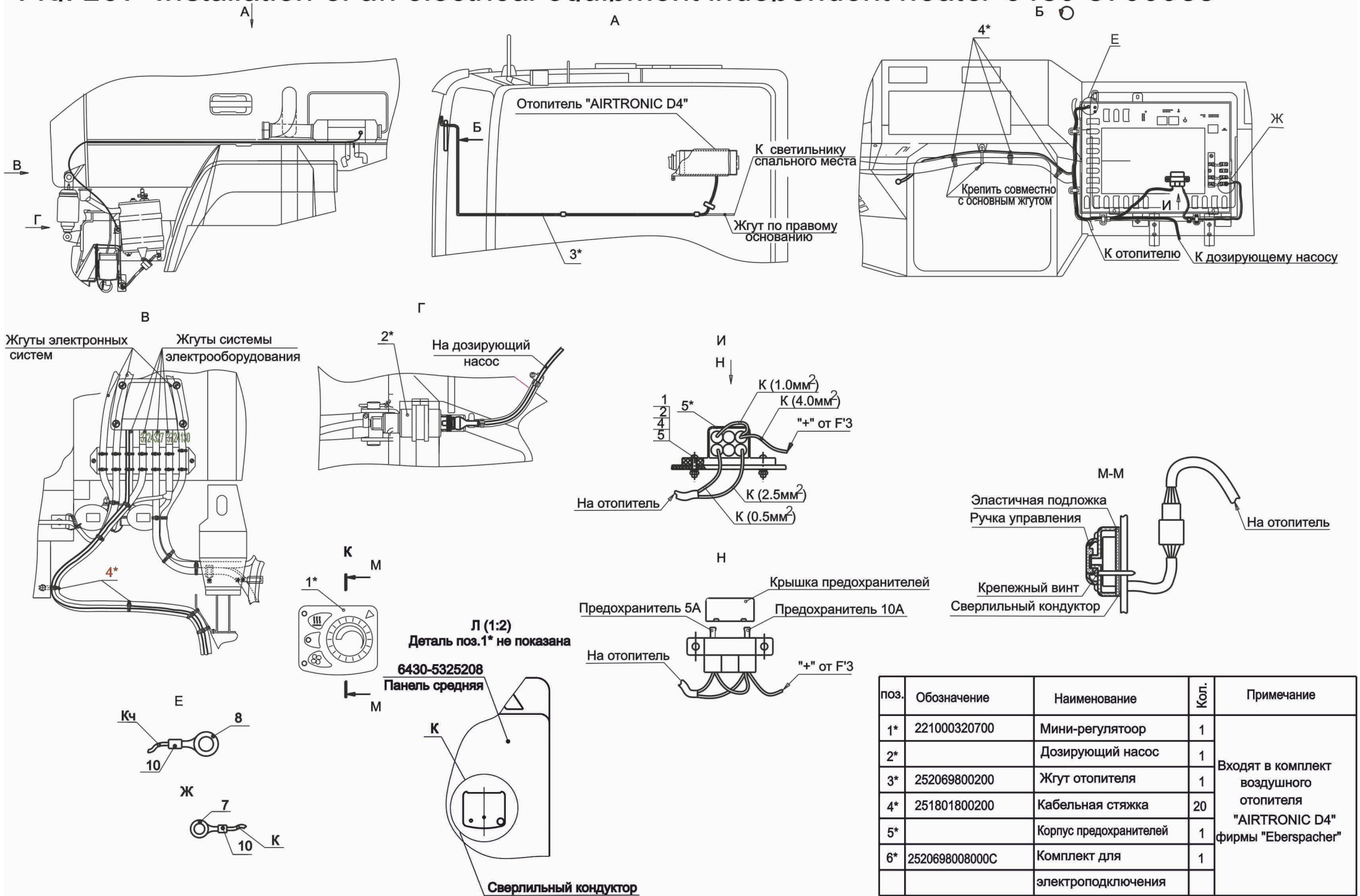
Рис. 297 Установка электрооборудования независимого отопителя 6430-3700088 Fig. 297 Installation of an electrical equipment independent heater 6430-3700088
