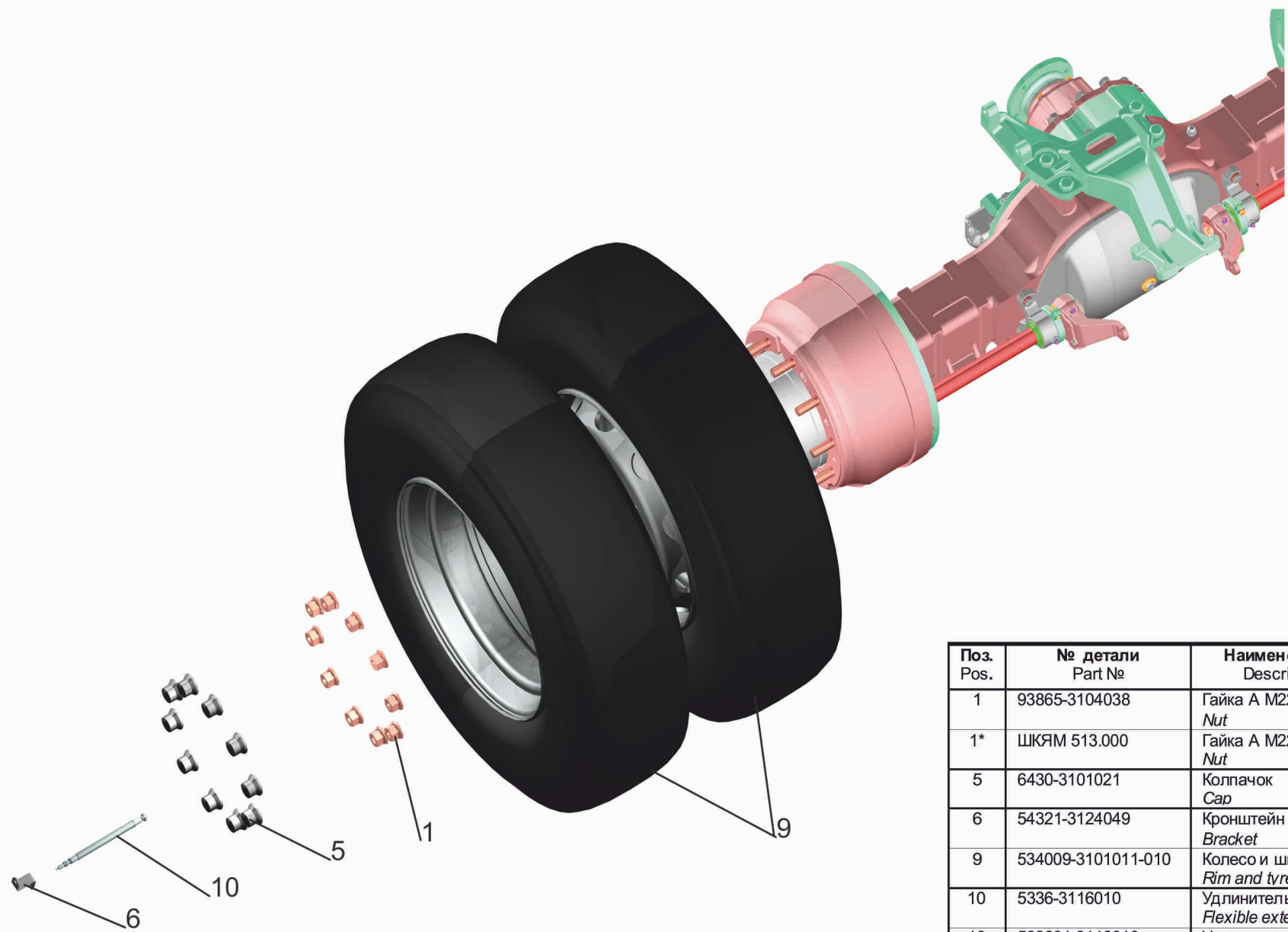
Рис. 134 Установка задних колес 534009-3100002 Fig. 134 Installation rear wheels
