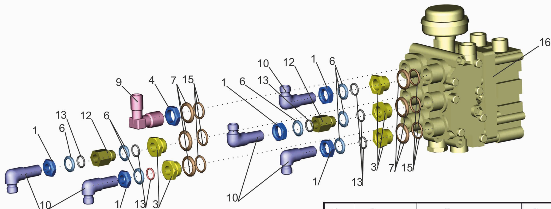
Рис. 111 Блок электропневмоклапанов ECAS с угольниками 631019-2926006 Fig. 111 Block ECAS with elbows 631019-2926006
