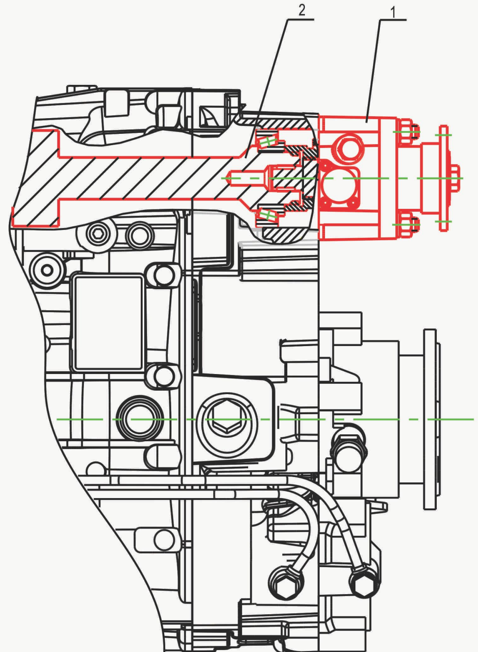
Рис. 327 Установка коробки отбора мощности 6310E9-8600007-069 Fig. 327 Installation power take-off gear box 6310E9-8600007-069
