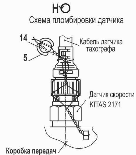
Рис. 189 Установка и пломбировка тахографа 5440-3800005 (лист 2 ) Fig. 189 Installation and identification seal of tachograph 5440-3800005 (page 2)
