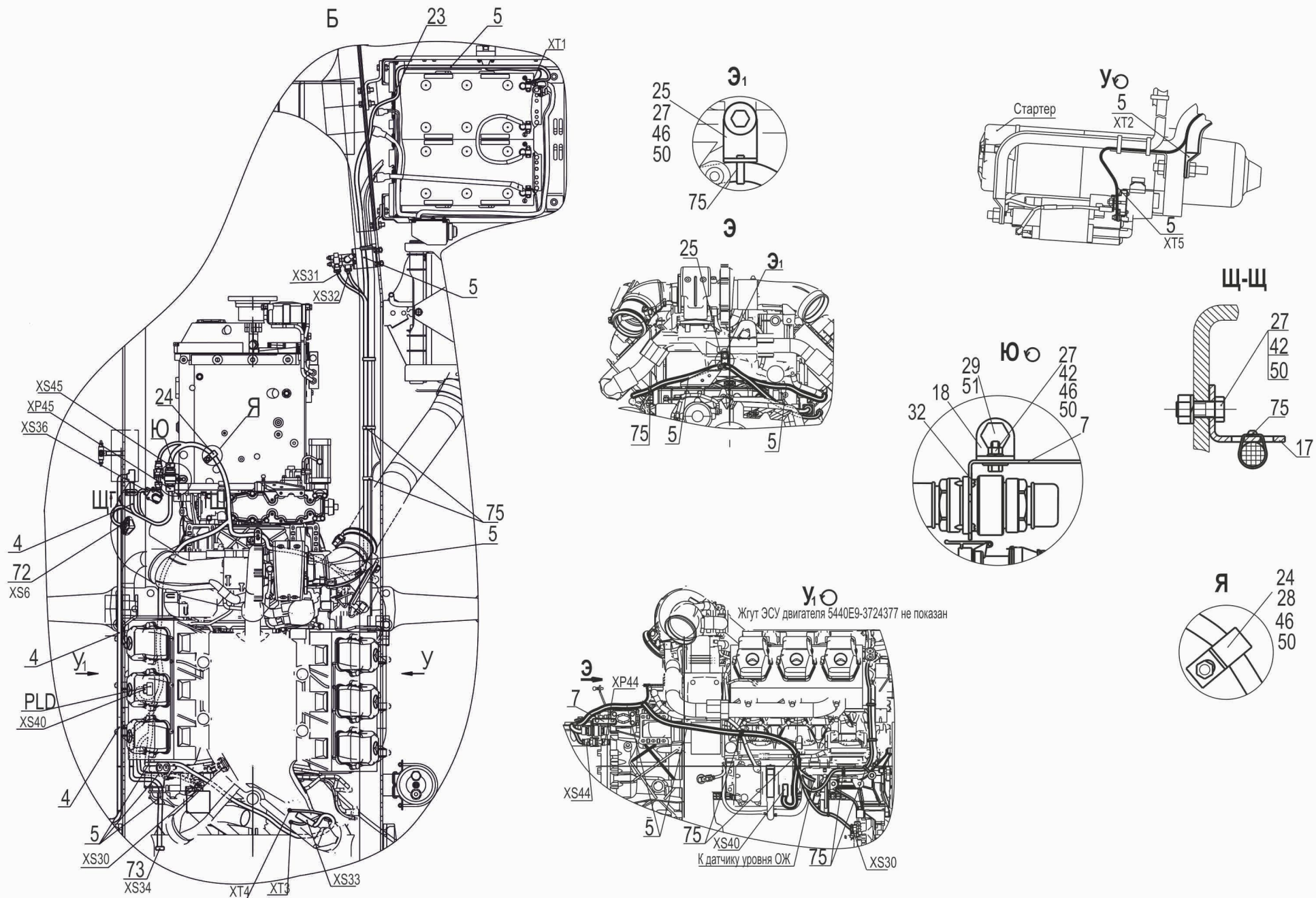
Рис. 221 Установка электрооборудования ЭСУ двигателя 643018-3800060-000, (-010) (лист 3) Fig. 221 Installation of electronic control system of the engine 643018-3800060-000, (-010) (page 3)
