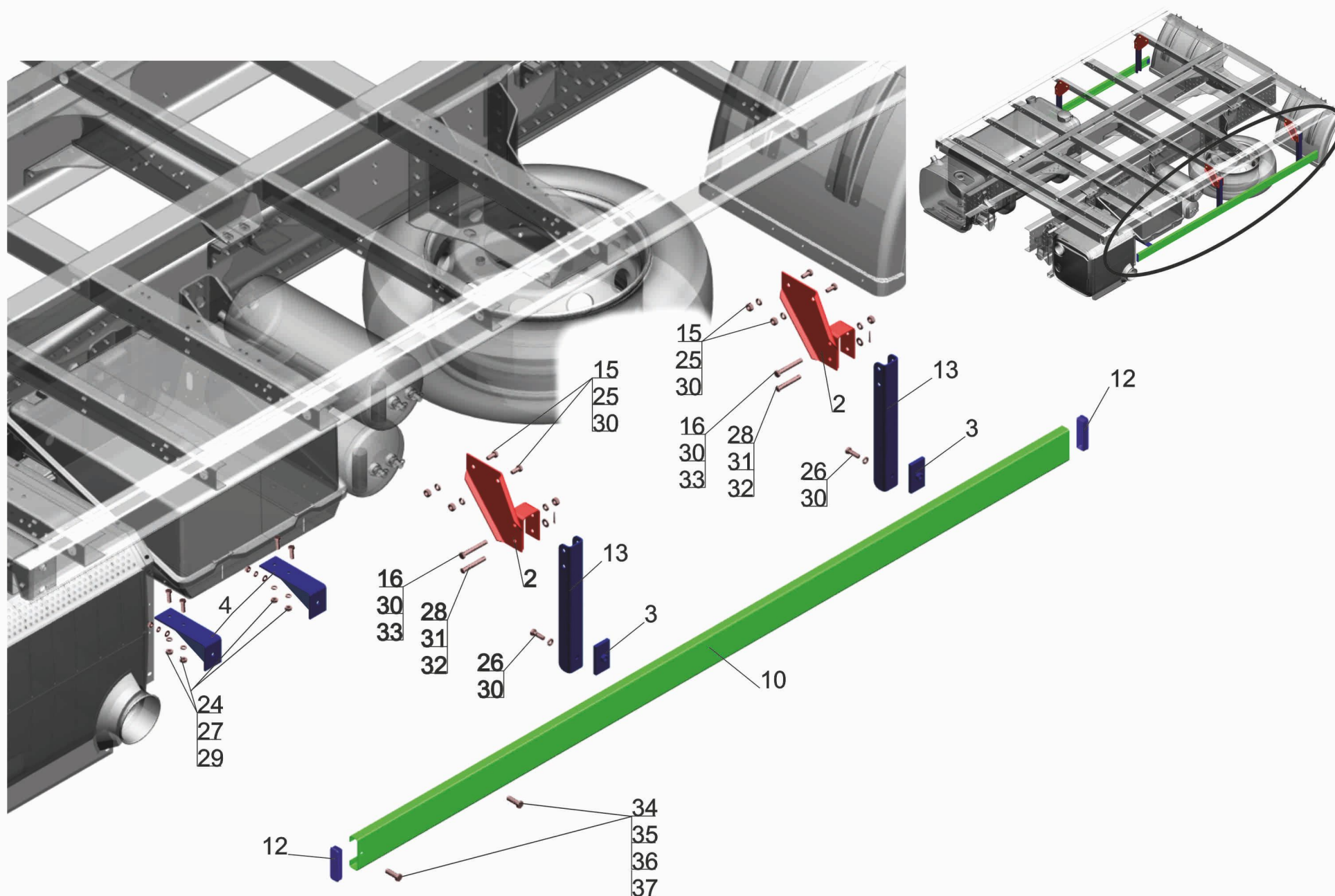
Рис. 95 Установка бокового ограждения 631019-2800040 (лист 2) Fig. 95 Installation of a lateral protection 631019-2800040 (page 2)
