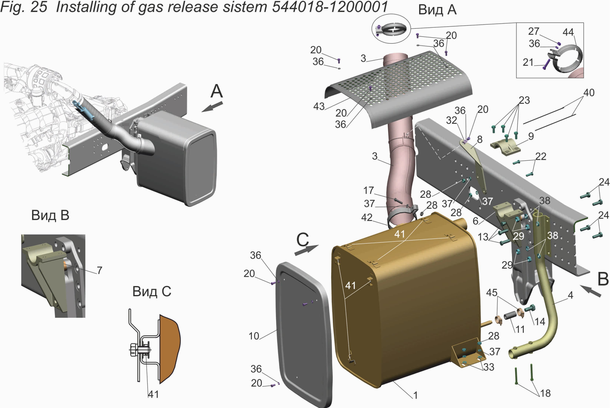
Рис. 25 Установка системы выпуска газов 544018-1200001
