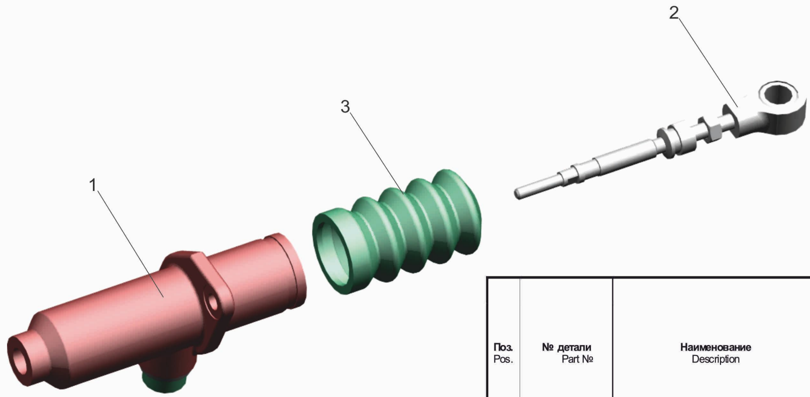
Рис. 41 Цилиндр подпедальный с толкателем 6430-1602500-000 (6430-1602500-001, 6430-1602500-020, 6430-1602500-002) Fig. 41 Under pedal cylinder with a pusher 6430-1602500-000 (6430-1602500-001, 6430-1602500-020, 6430-1602500-002)
