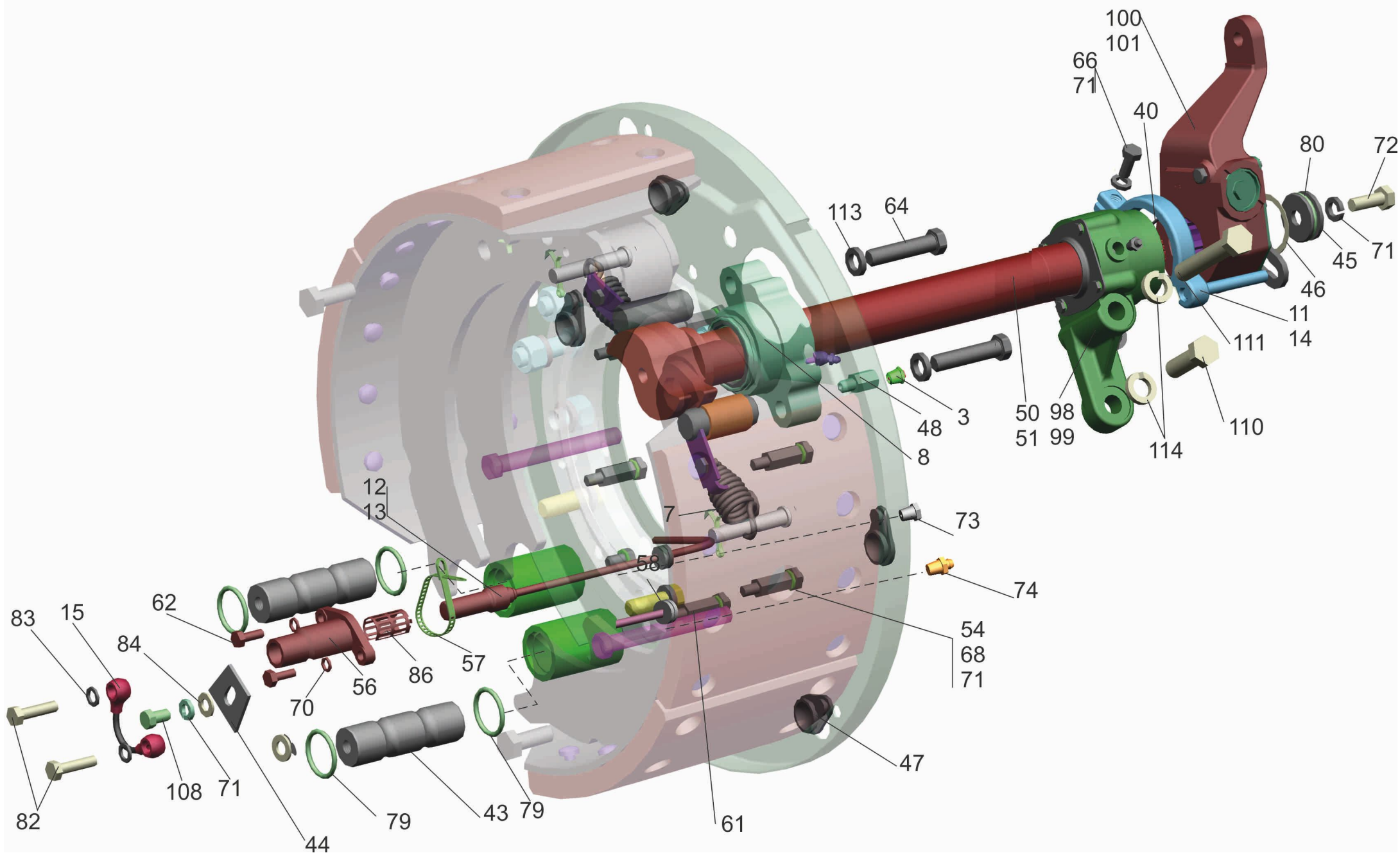
Рис. 63 Мост задний Лист 2 Fig. 63 Rear axle Page 2
