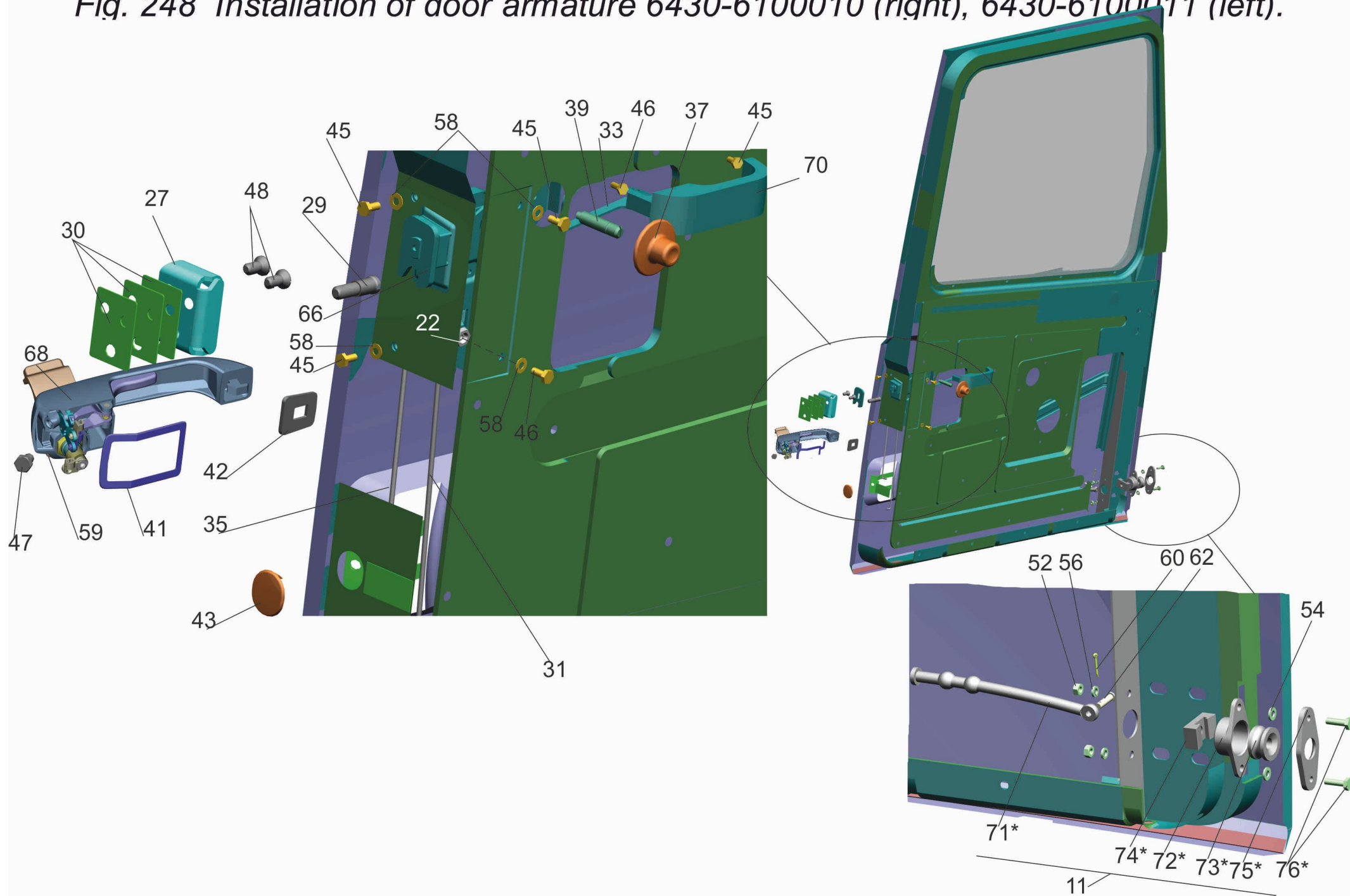
Рис. 248 Установка дверной арматуры 6430-6100010 (правая), 6430-6100011 (левая).(лист1)
