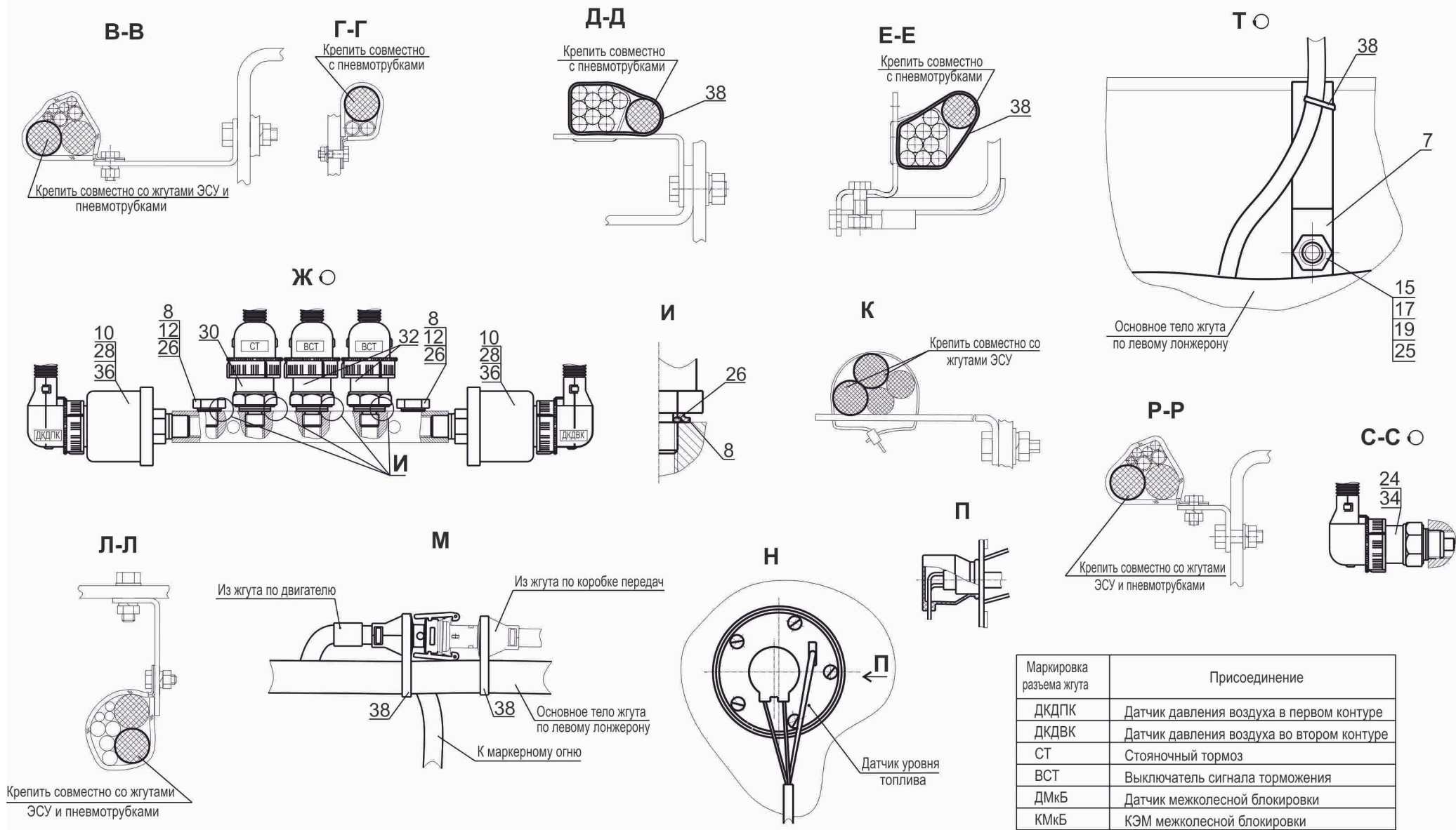
Рис. 195 Установка электрооборудования на шасси 5340Е9-3700010, (-700) (лист 2) Fig. 195 Installation of electrical equipment on the chassis 5340Е9-3700010, (-700) (page 2)
