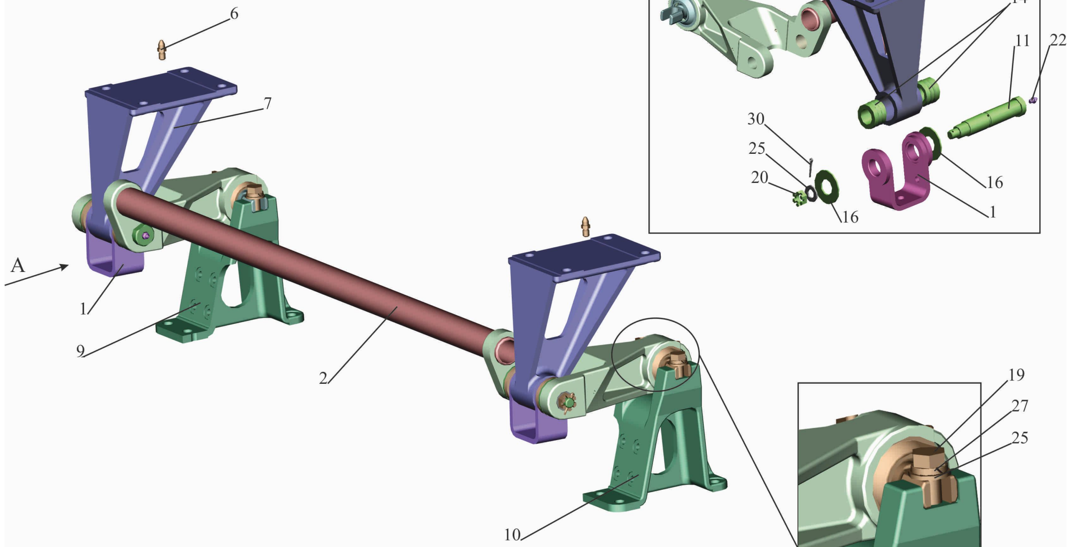
Рис. 229 Переднее подрессоривание Fig. 229 Front spriging
