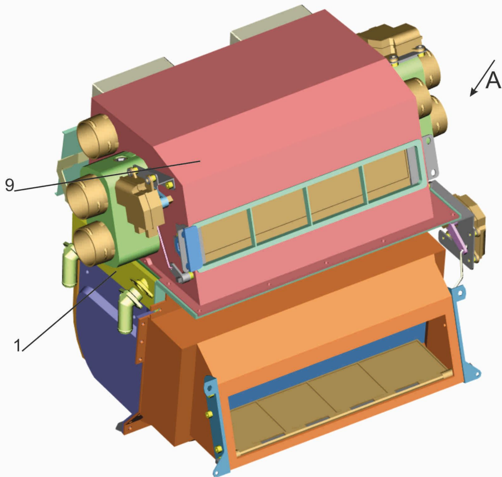
Рис. 284 Отопитель 631019-8101010 Fig. 284 Heater 631019-8101010
