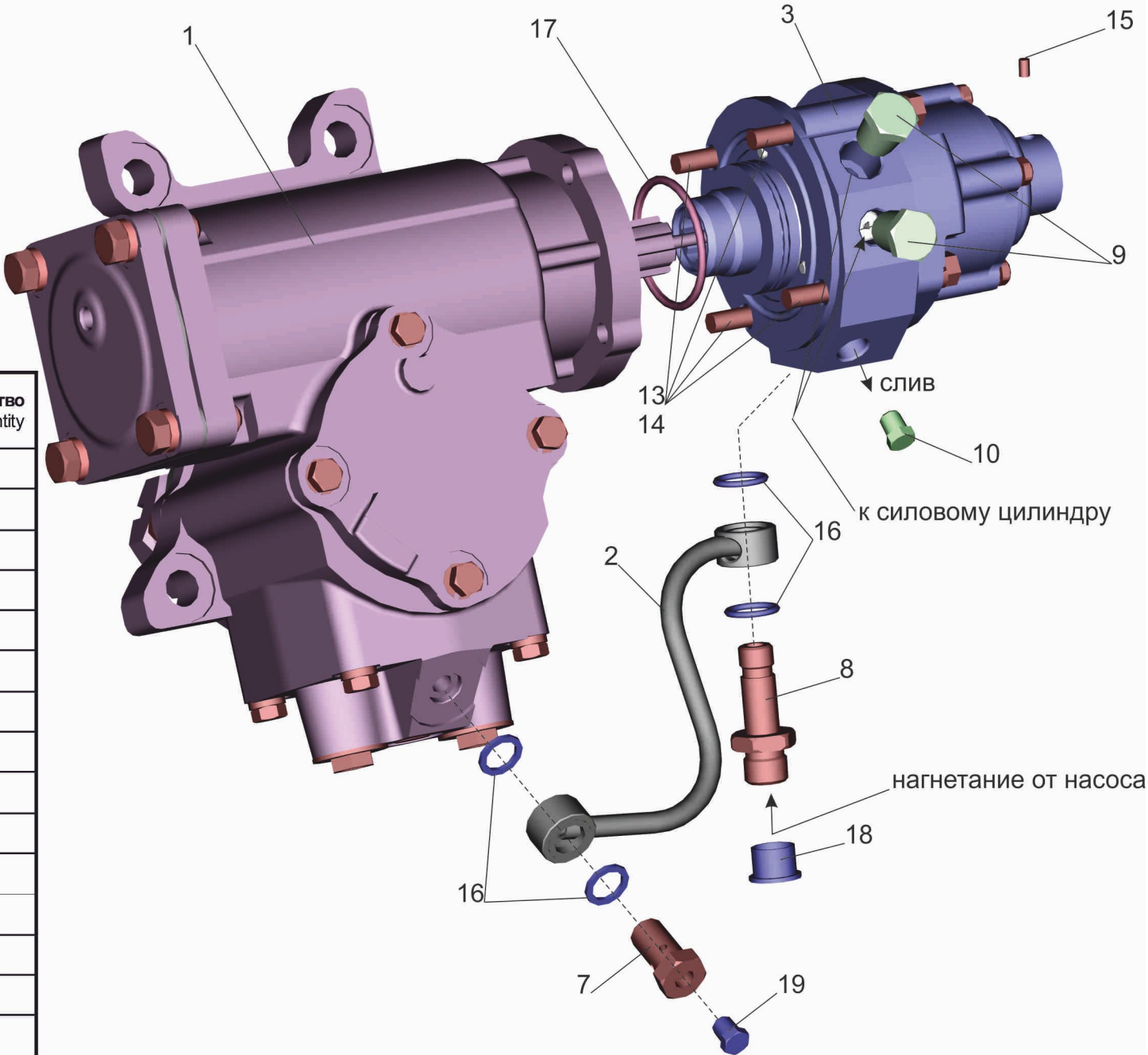
Рис. 140 Рулевой механизм с распределителем 64221-3400010-10 Fig. 140 Steer with the allocator 64221-3400010-10
