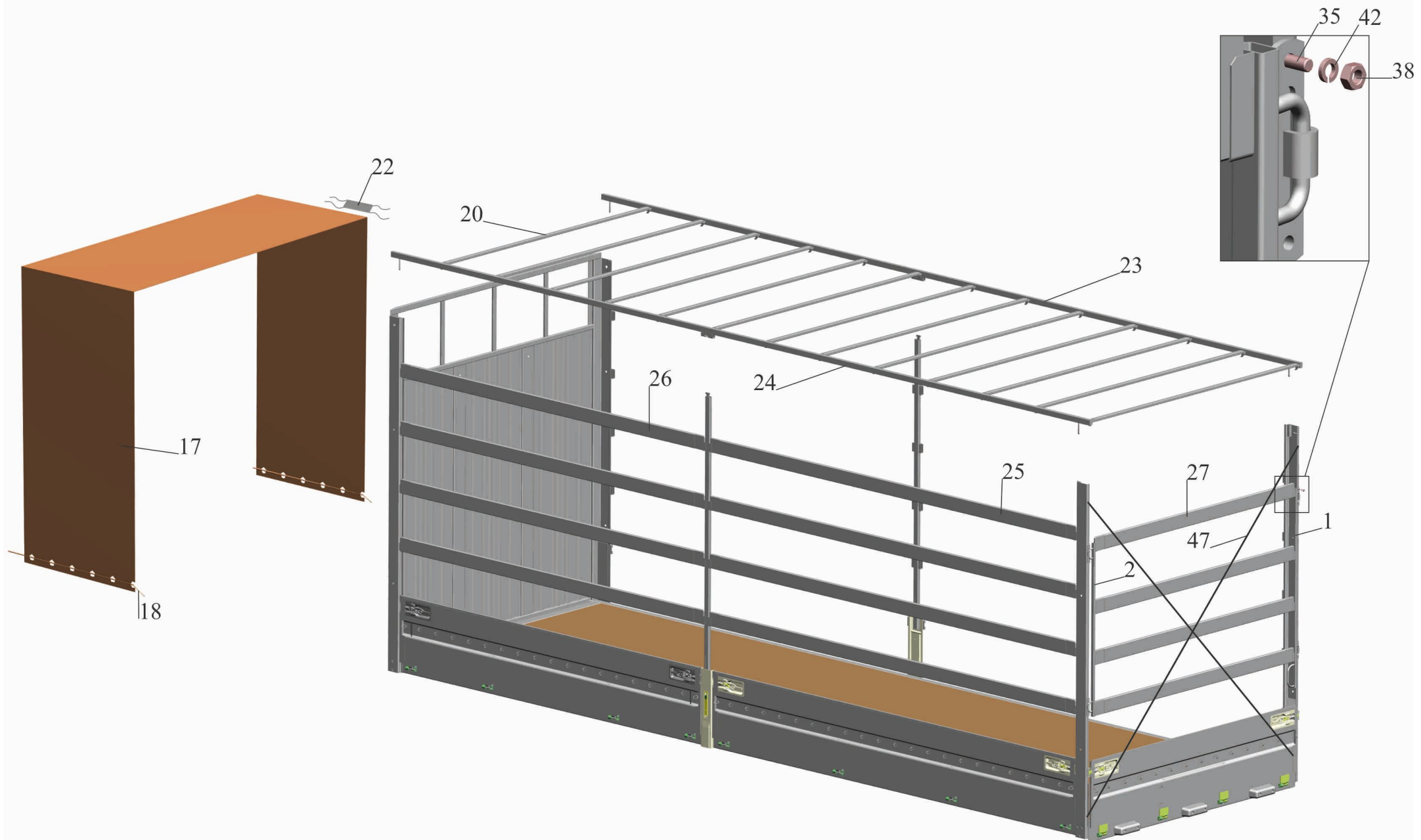
Рис. 313 Платформа (тентовая надстройка и тент) ( лист 1) Fig. 313 Platform (canopy superstructure and canopy) ( page 1)
