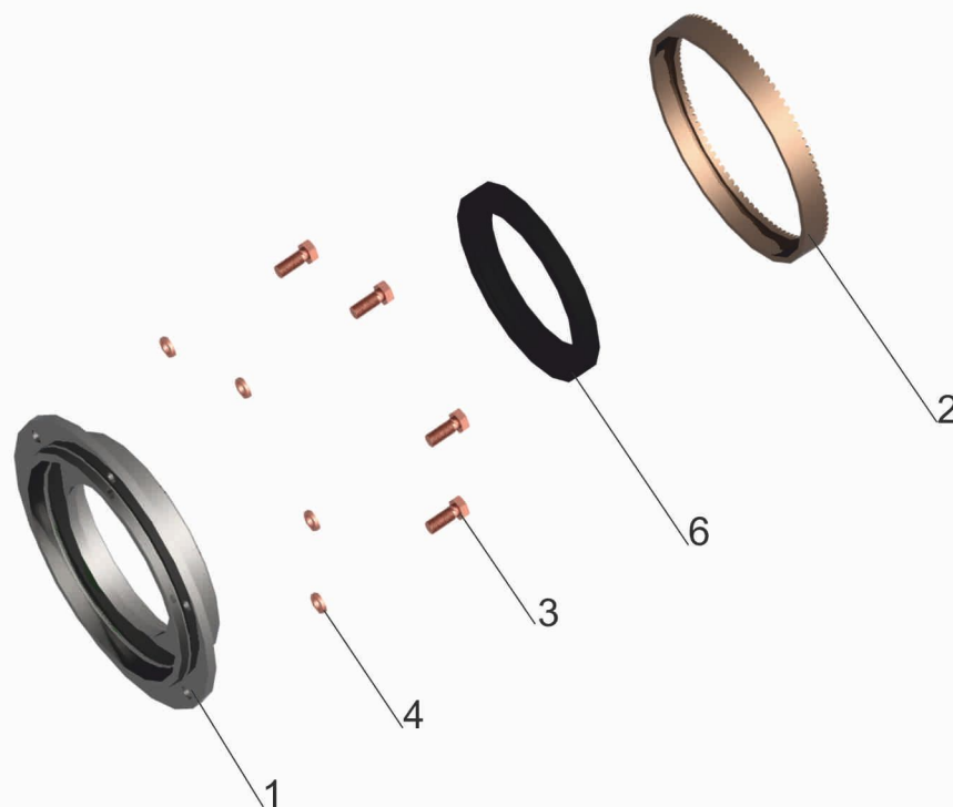
Рис. 117 Крышка 8701-3103034 Fig. 117 Cover 8701-3103034
