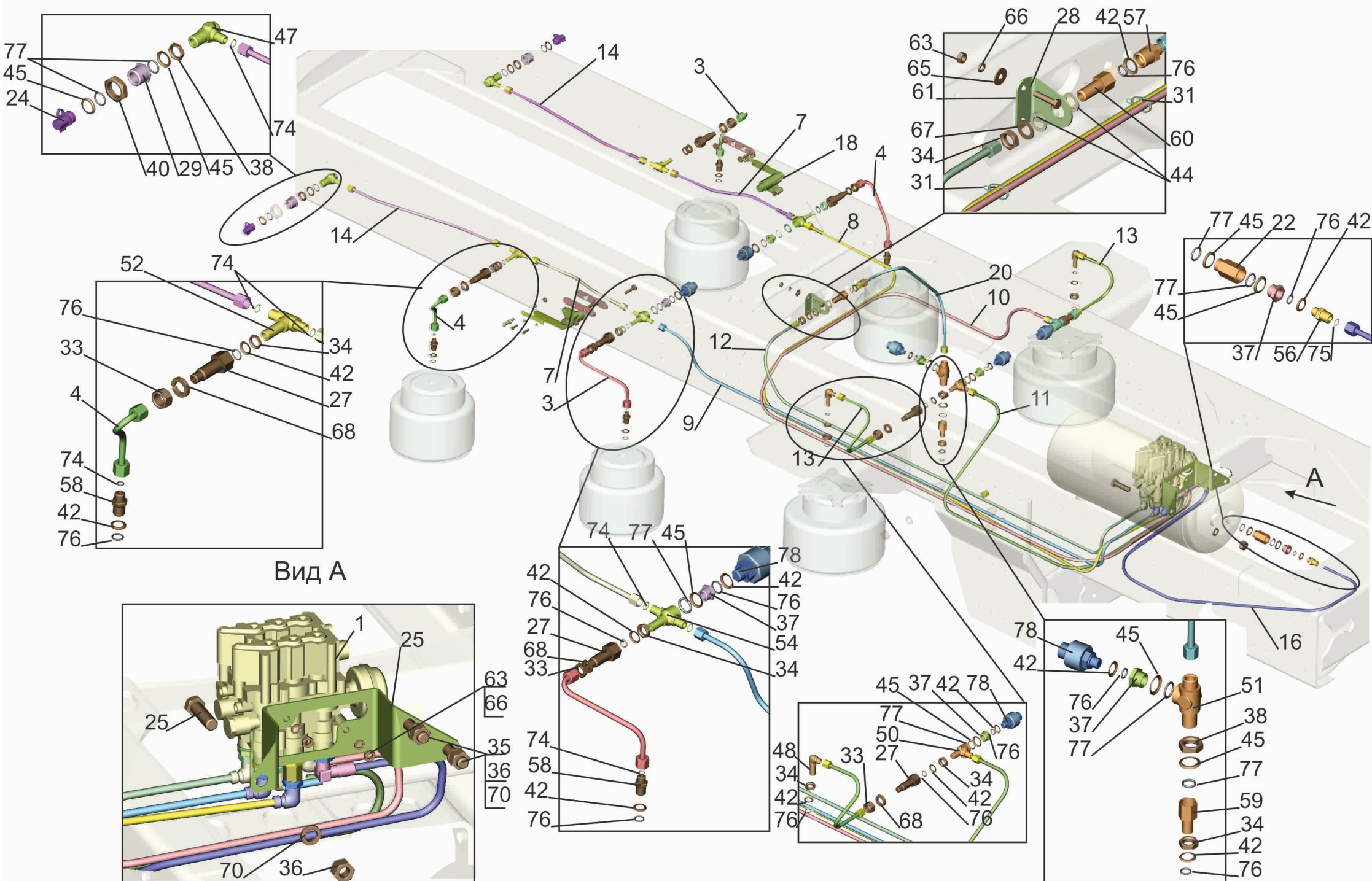
Fig. 110 Installation of pipelines ECAS 6310E9-2900018-000
