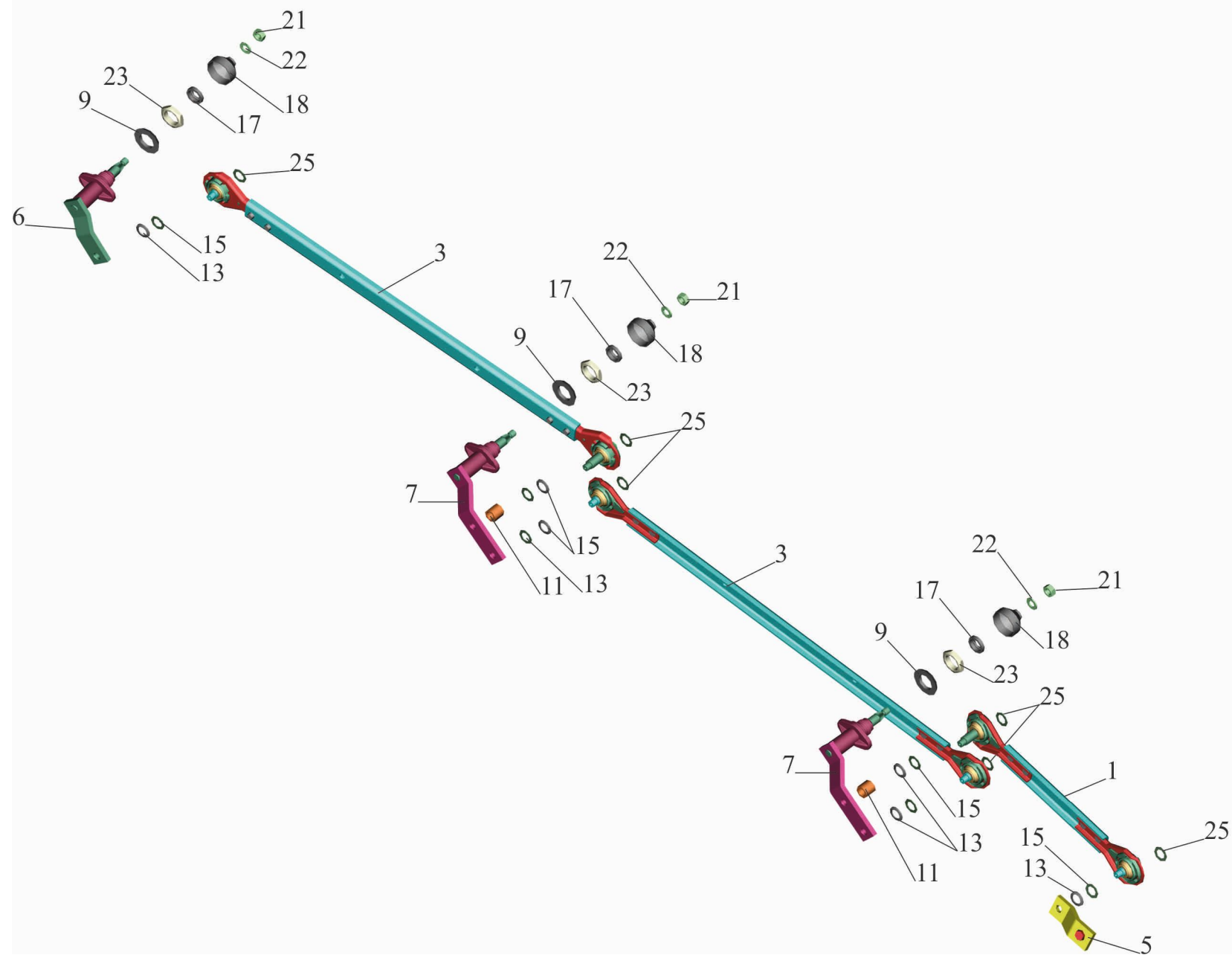
Рис. 239 Привод стеклоочистителя 6430-5205500-010 Fig. 239 Drive of cleaner of glasses 6430-5205500-010
