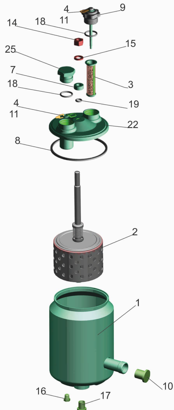
Рис. 153 Бак масляный 5336-3410010-10 Fig. 153 Oil tank 5336-3410010-10
