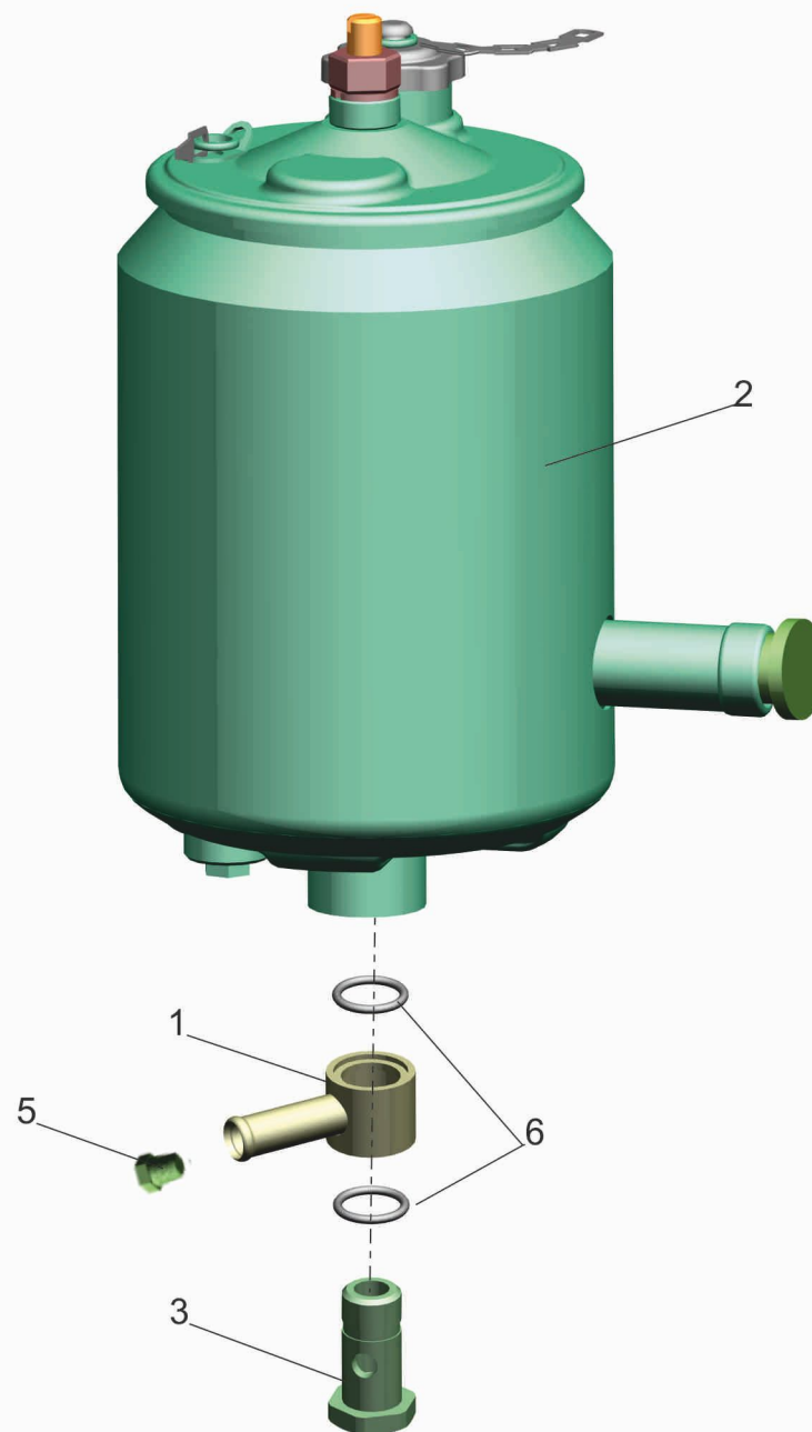
Рис. 152 Бак масляный 64221-3410008 Fig. 152 Oil tank 64221-3410008
