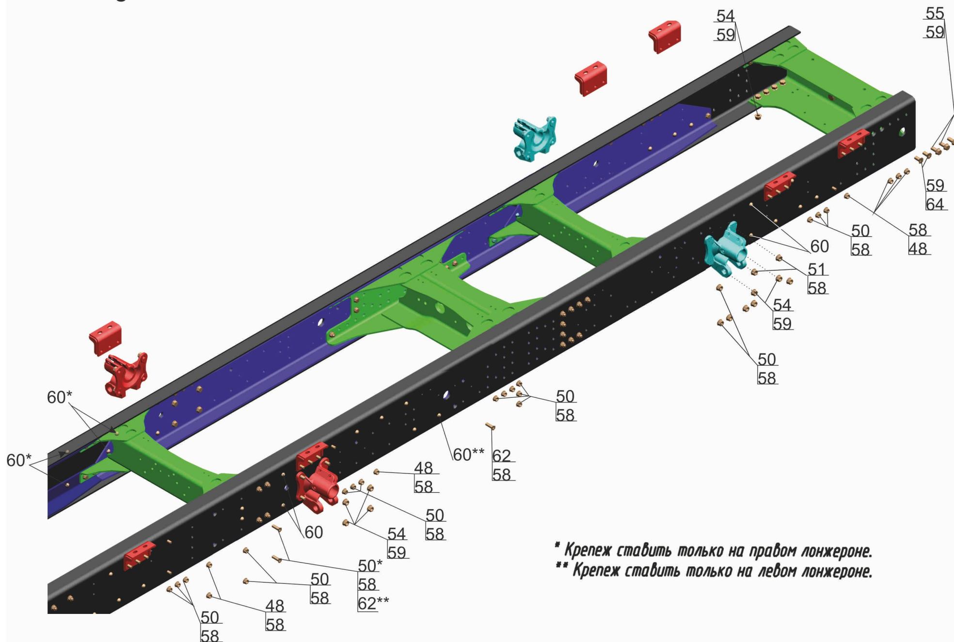
Рис. 90 Рама 6310E9-2801002-031 (лист 3) Fig. 90 Frame 6310E9-2801002-031
