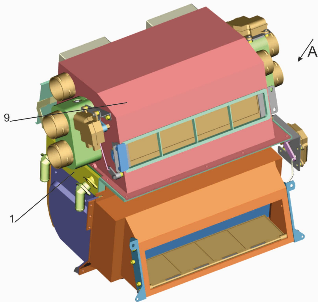
Рис. 286 Отопитель 643008-8101010 Fig. 286 Heater 643008-8101010
