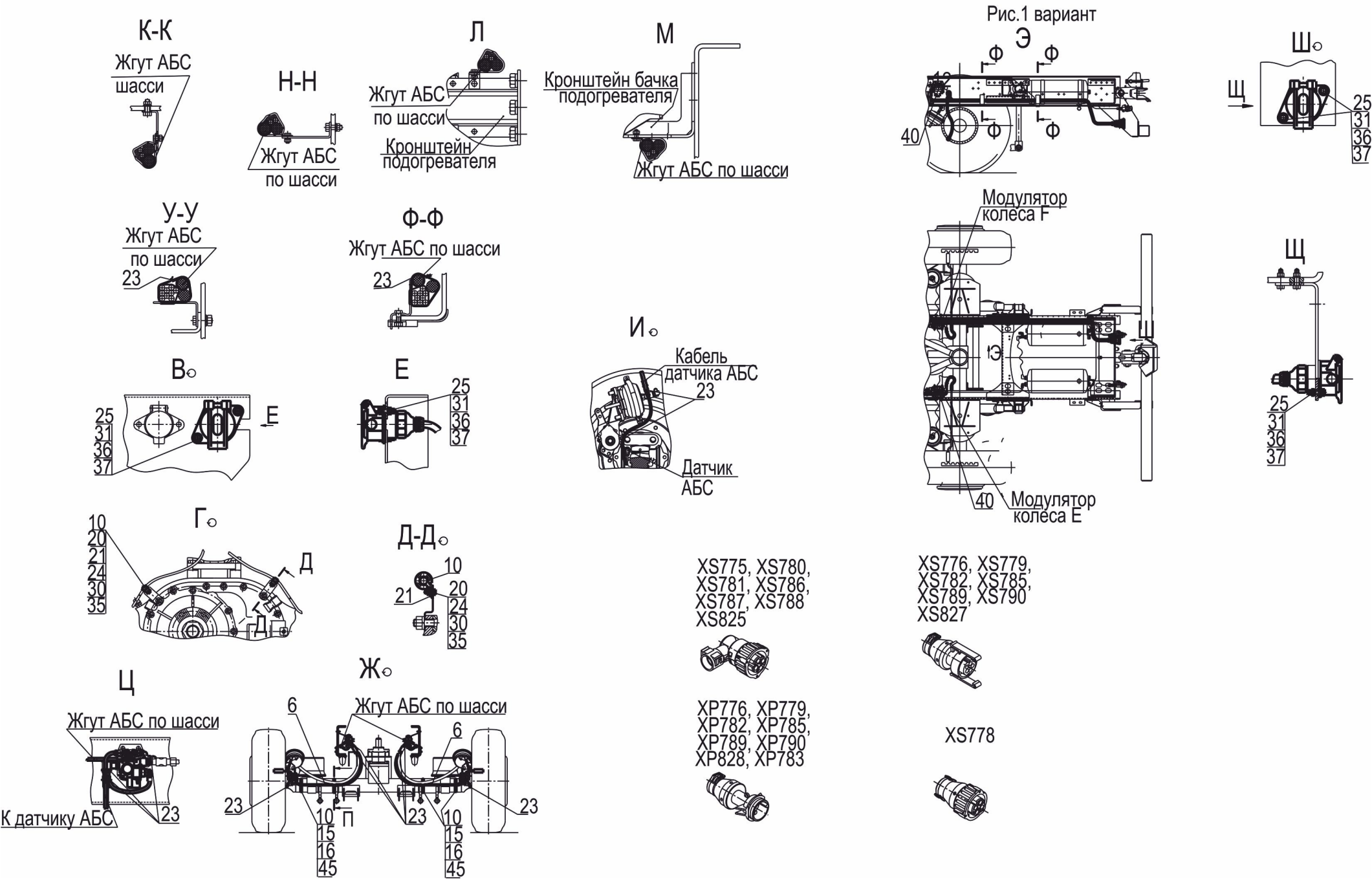
Рис. 214 Установка электрооборудования АБС тормозов 6310Е9-3800040 (лист 2) Fig. 214 Setting of electrical equipment ABS brakes 6310Е9-3800040 (page 2)
