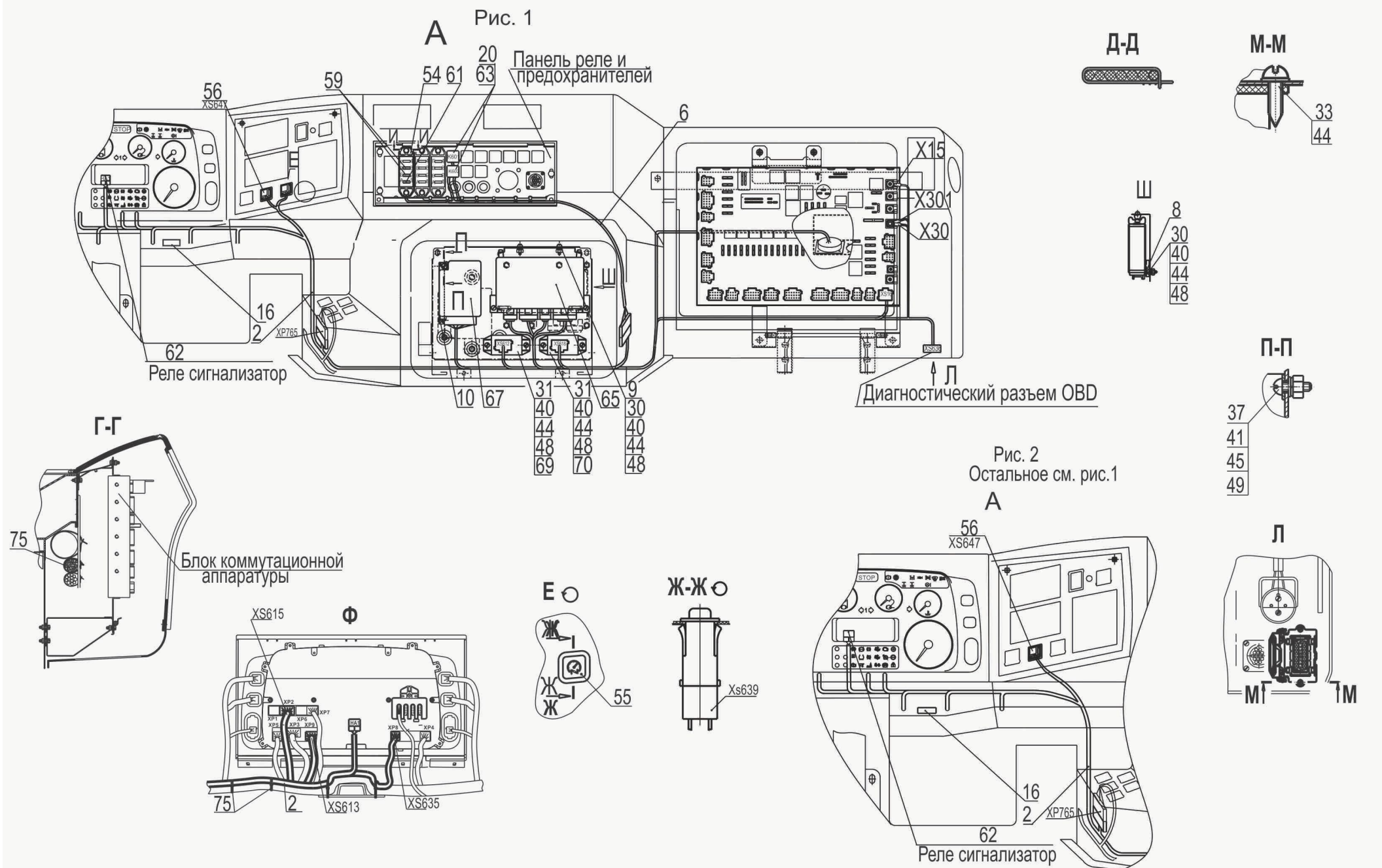
Рис. 221 Установка электрооборудования ЭСУ двигателя 643018-3800060-000, (-010) (лист 2) Fig. 221 Installation of electronic control system of the engine 643018-3800060-000, (-010) (page 2)
