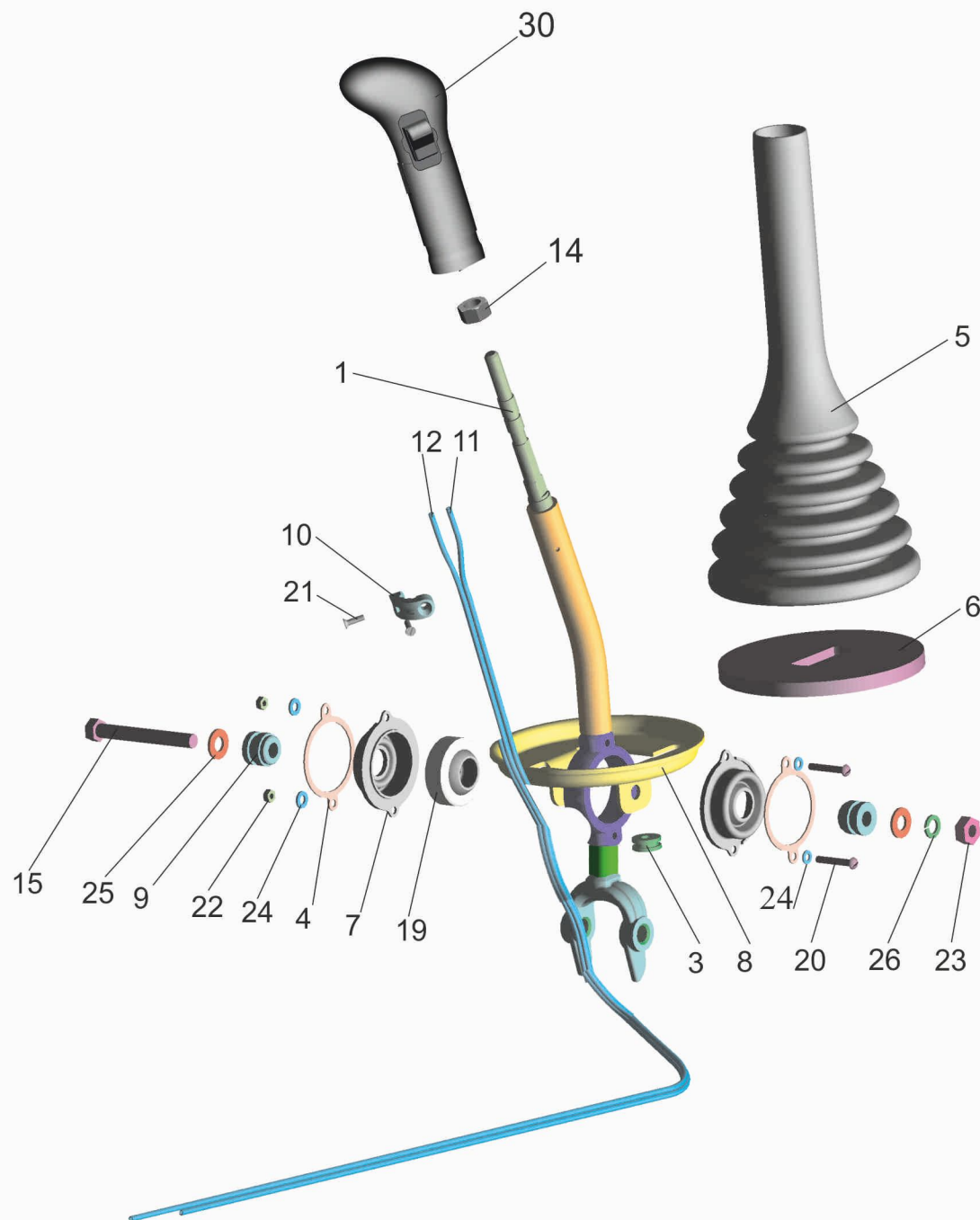
Fig. 50 Lever 64301-1703410-050
