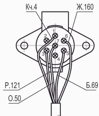
В Подсоединение проводов к розетке 24S (Чехол поз.4 не показан)
