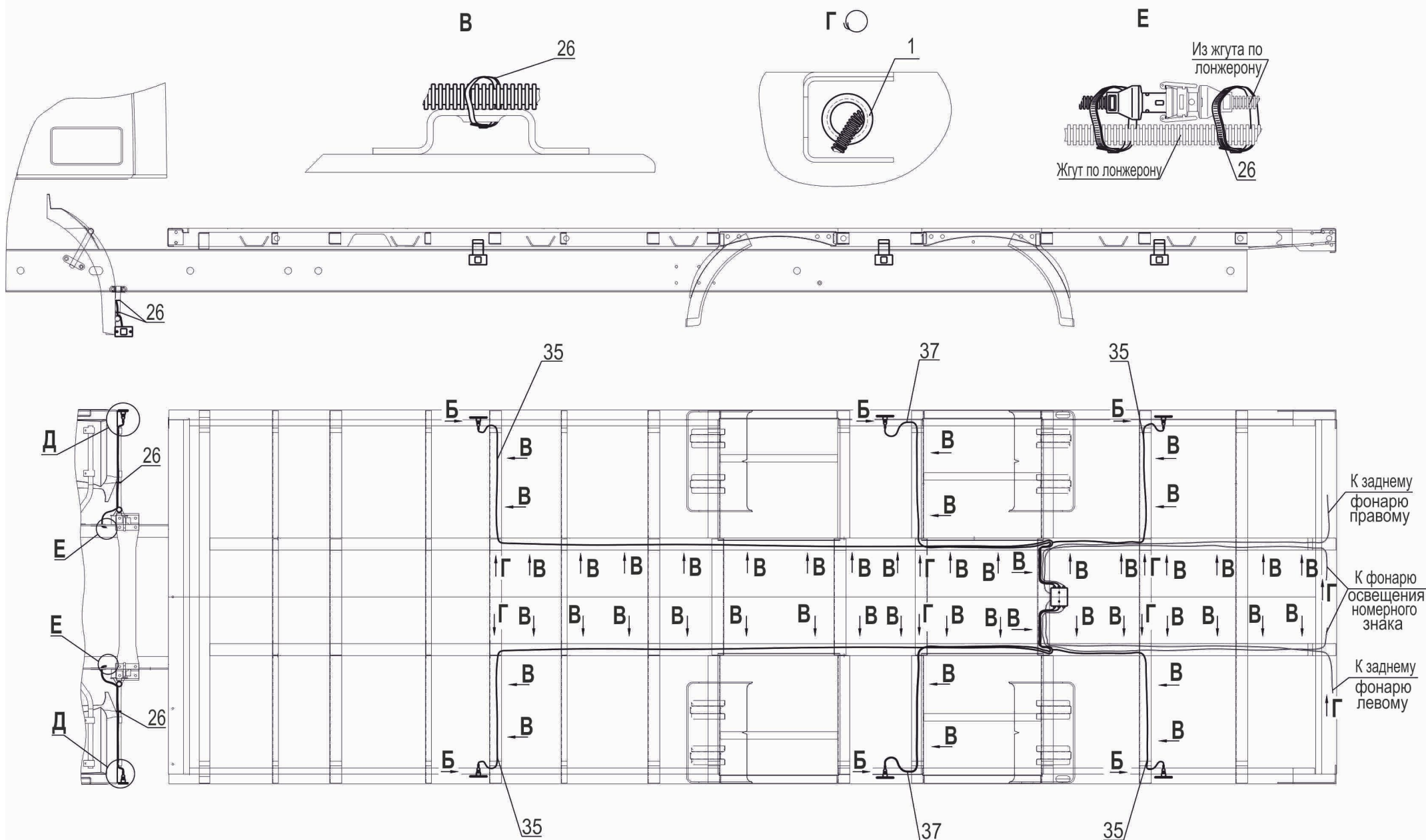
Рис. 205 Установка боковых габаритных фонарей 631019-3700080, (-700) (лист 1) Fig. 205 Setting of a lateral marker light 631019-3700080, (-700) (page 1)
