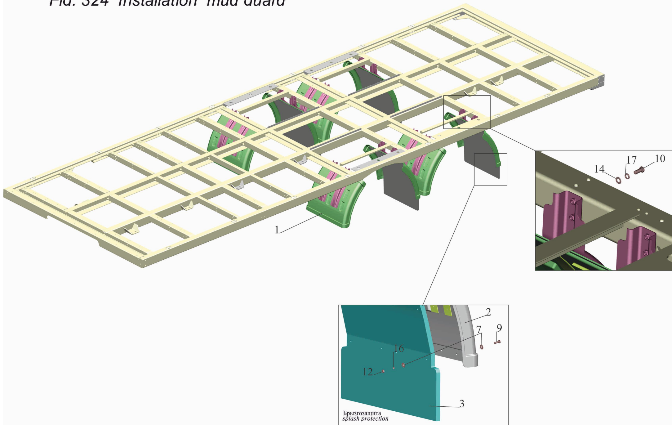
Рис. 324 Установка брызговиков 6310E9-8500048-010 Fig. 324 Installation mud guard
