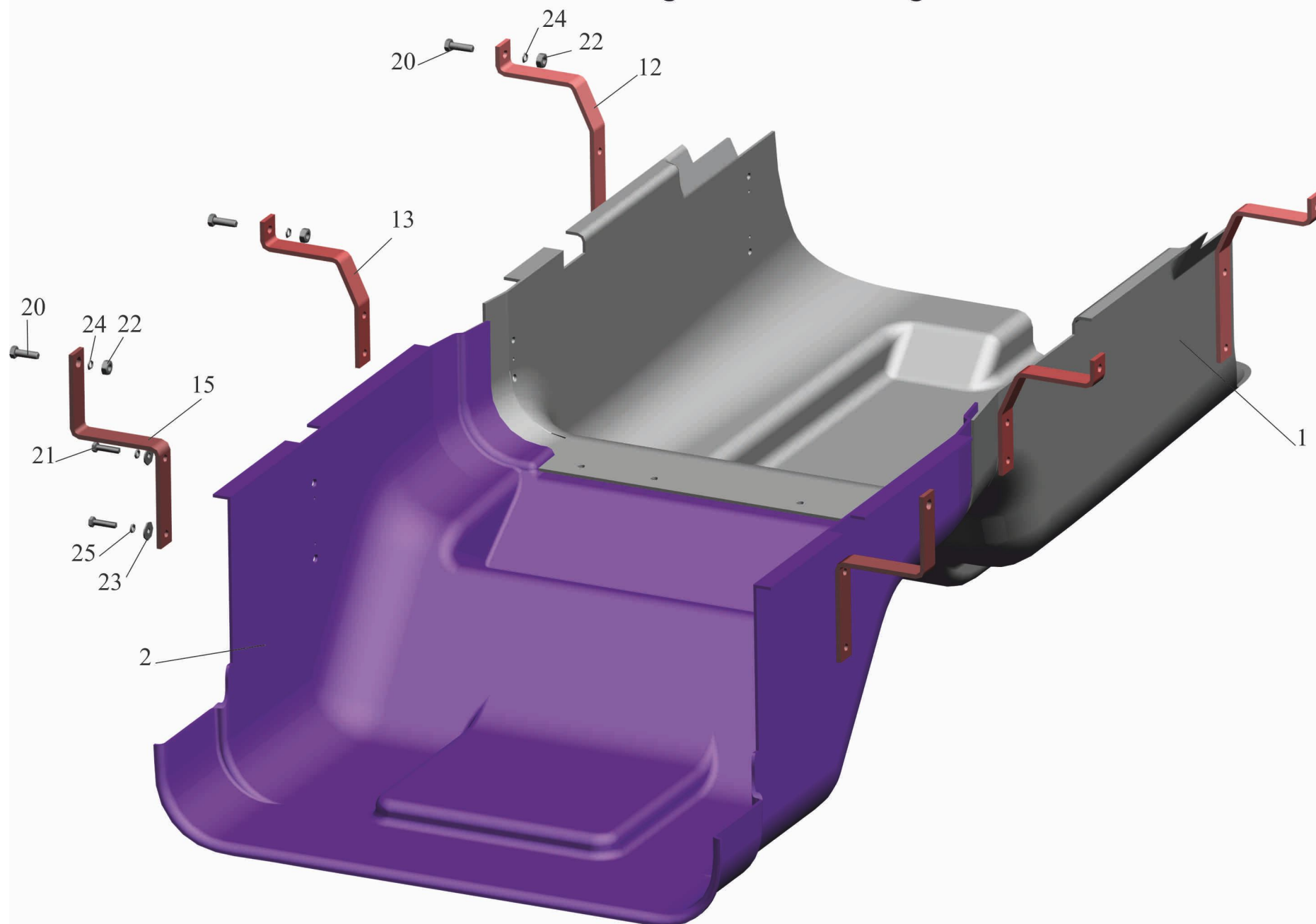
Рис.11 Установка шумоизоляционных экранов Fig. 11 Mounting noise isolation screens
