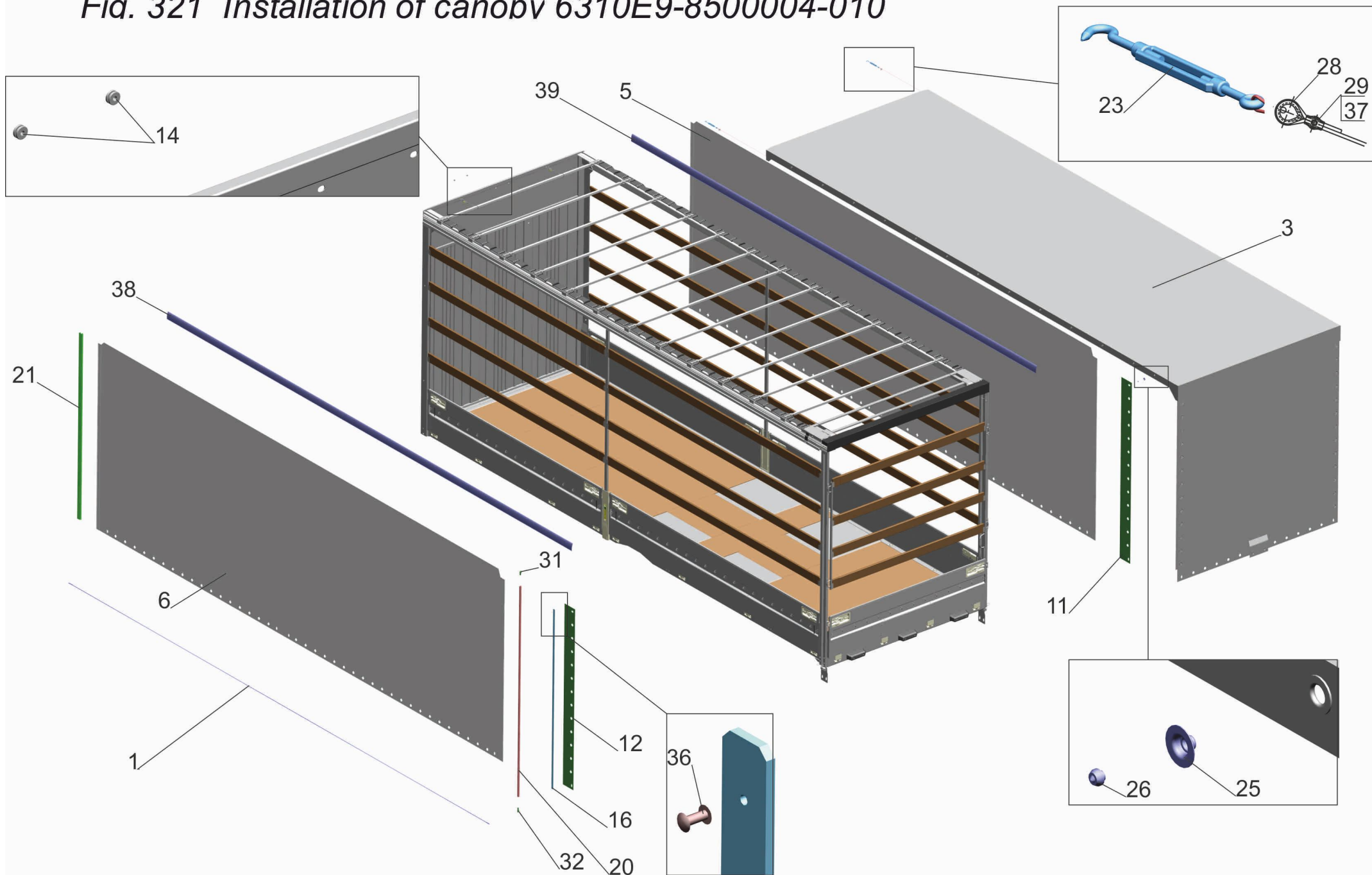
Рис. 321 Установка тента 6310E9-8500004-010
