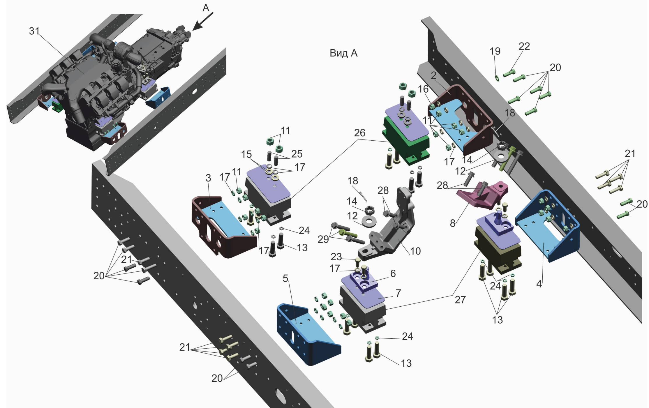
Рис. 2 Крепление двигателя 534019-1001002, (-010), 544018-1001002, (-010) Fig. 2 Mounting diesel 534019-1001002, (-010), 544018-1001002, (-010)
