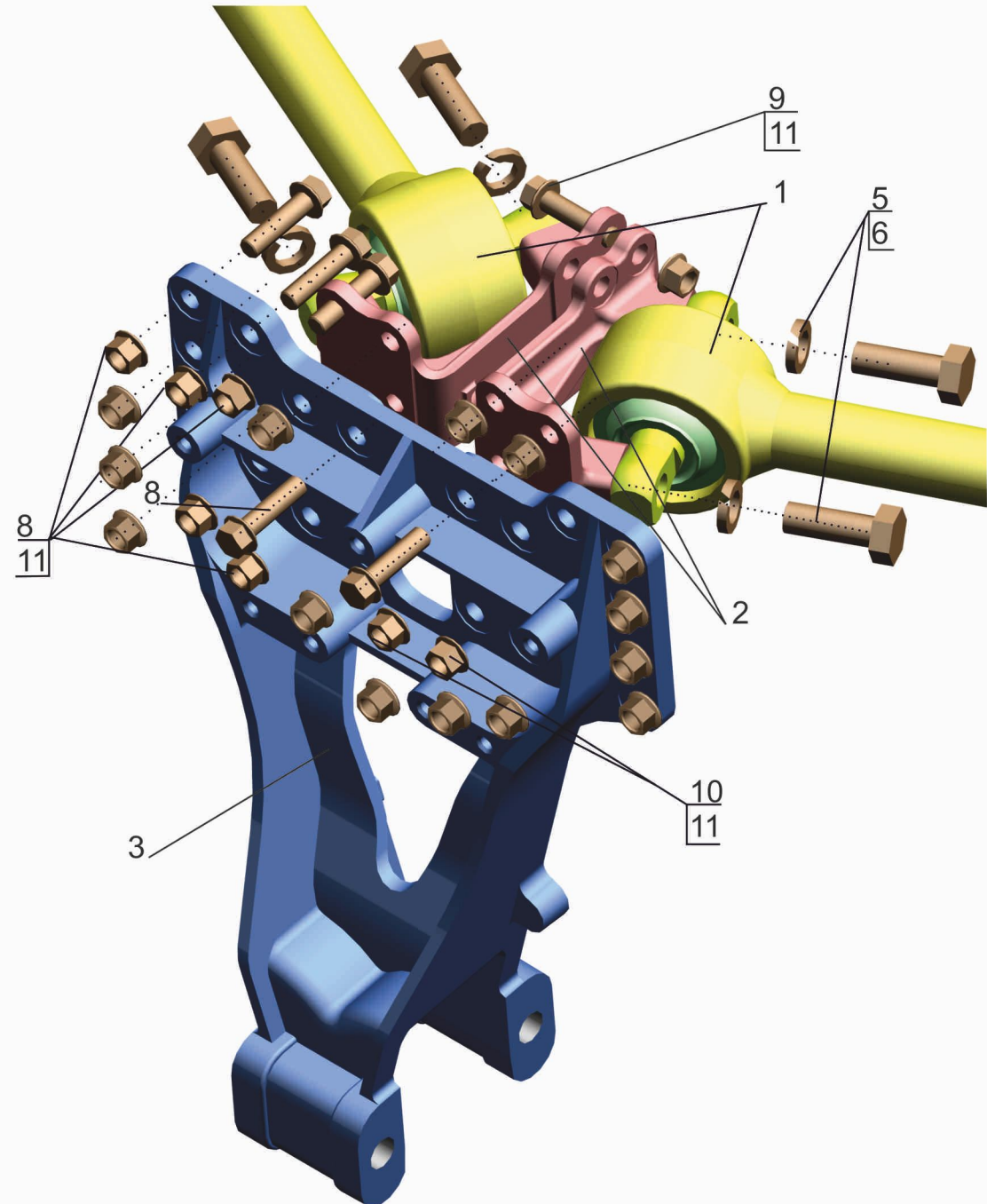
Рис. 105 Кронштейны с креплением 631019-2933110-000 Fig. 105 Bracket 631019-2933110-000
