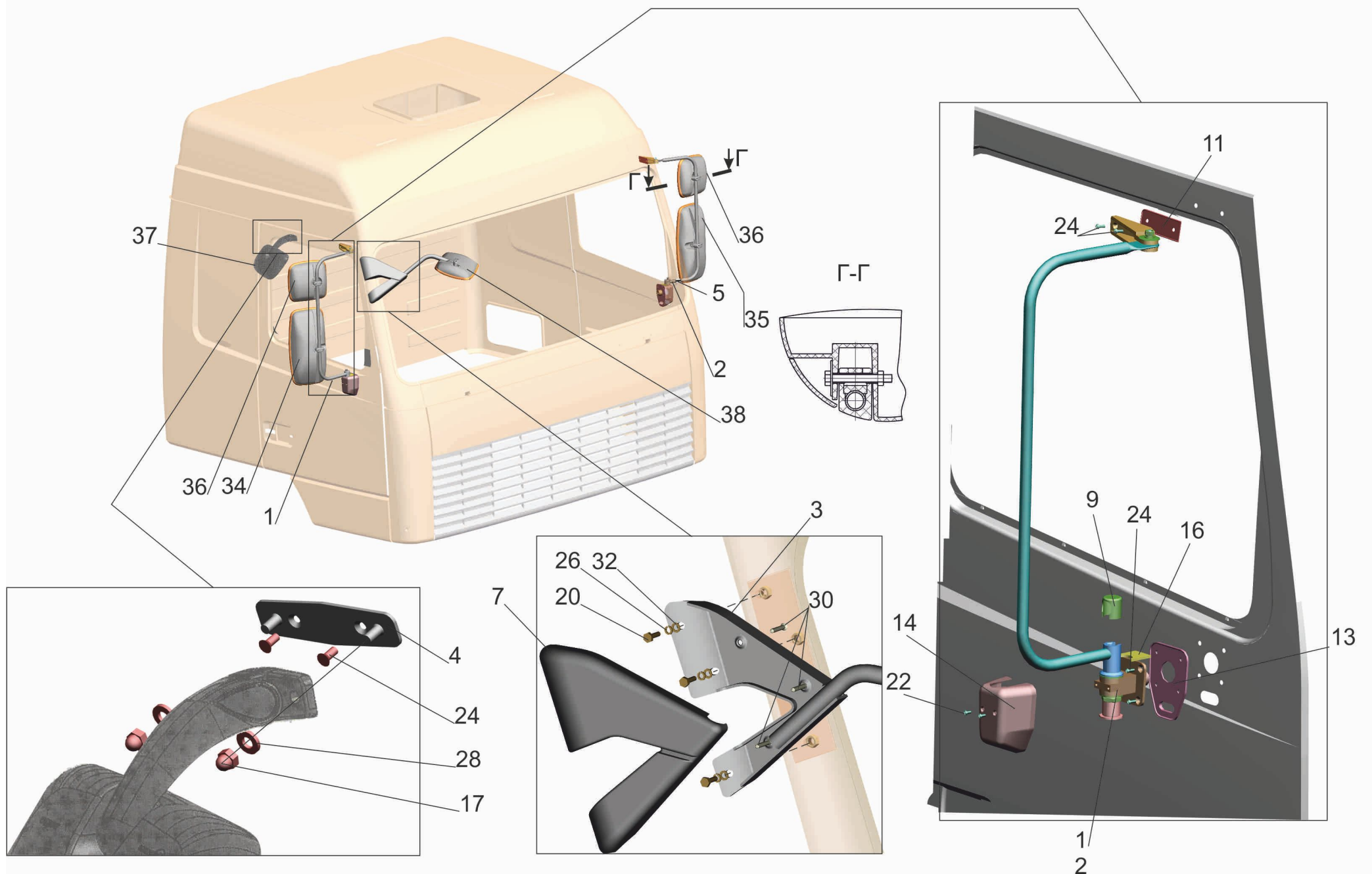
Рис. 265 Установка зеркал 6430-8200005-020 Fig. 265 Installation mirrors 6430-8200005-020
