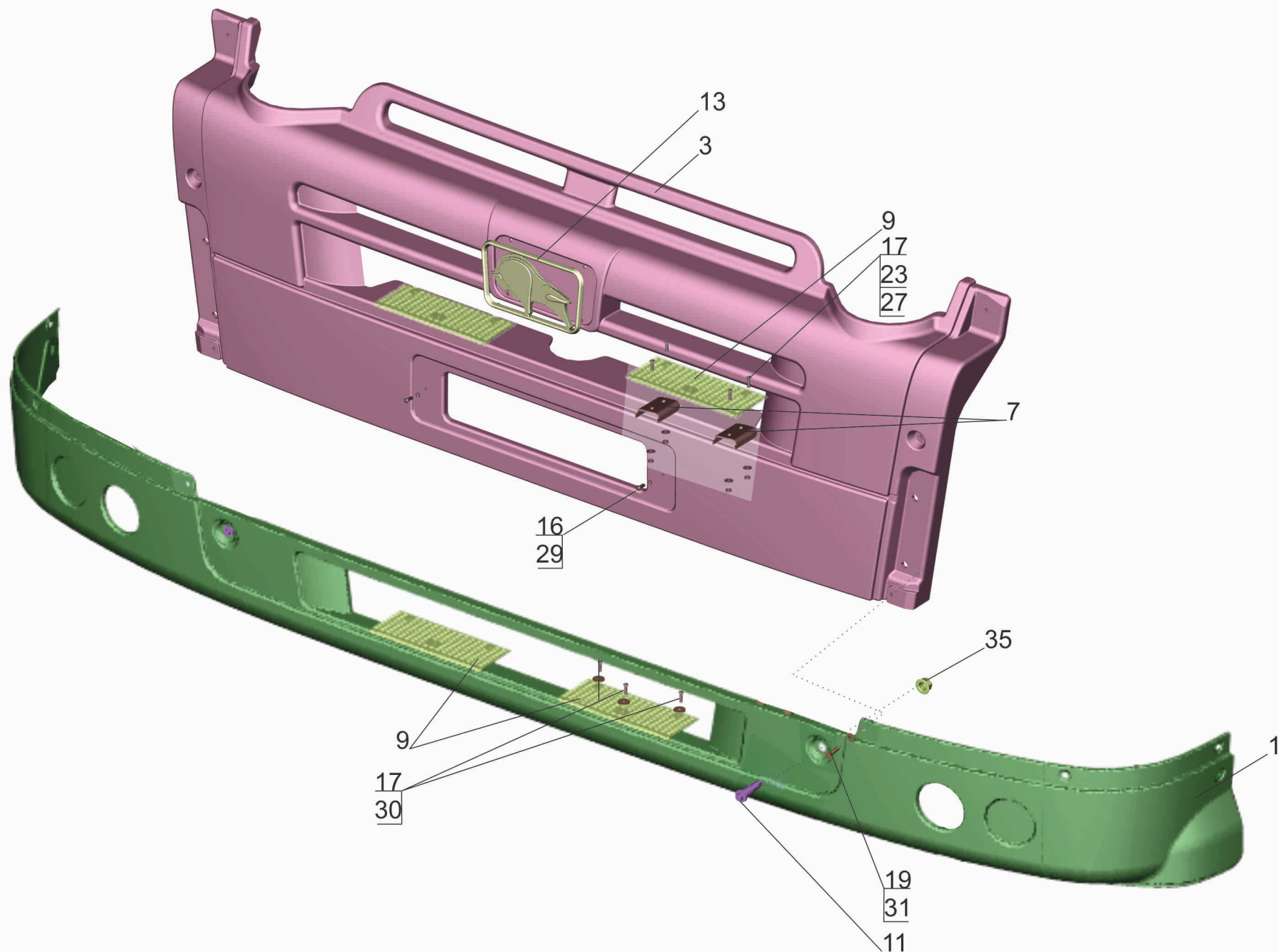
Рис. 84 Бампер передний 643019-2803010 Fig. 84 Bumper 643019-2803010
