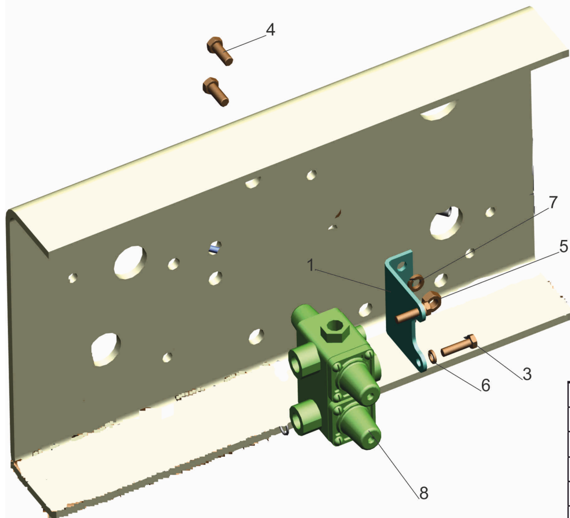
Рис. 168 Крепление четырехконтурного клапана 544019-3515002 Fig. 168 Four-circuit safety valve mounting 544019-3515002
