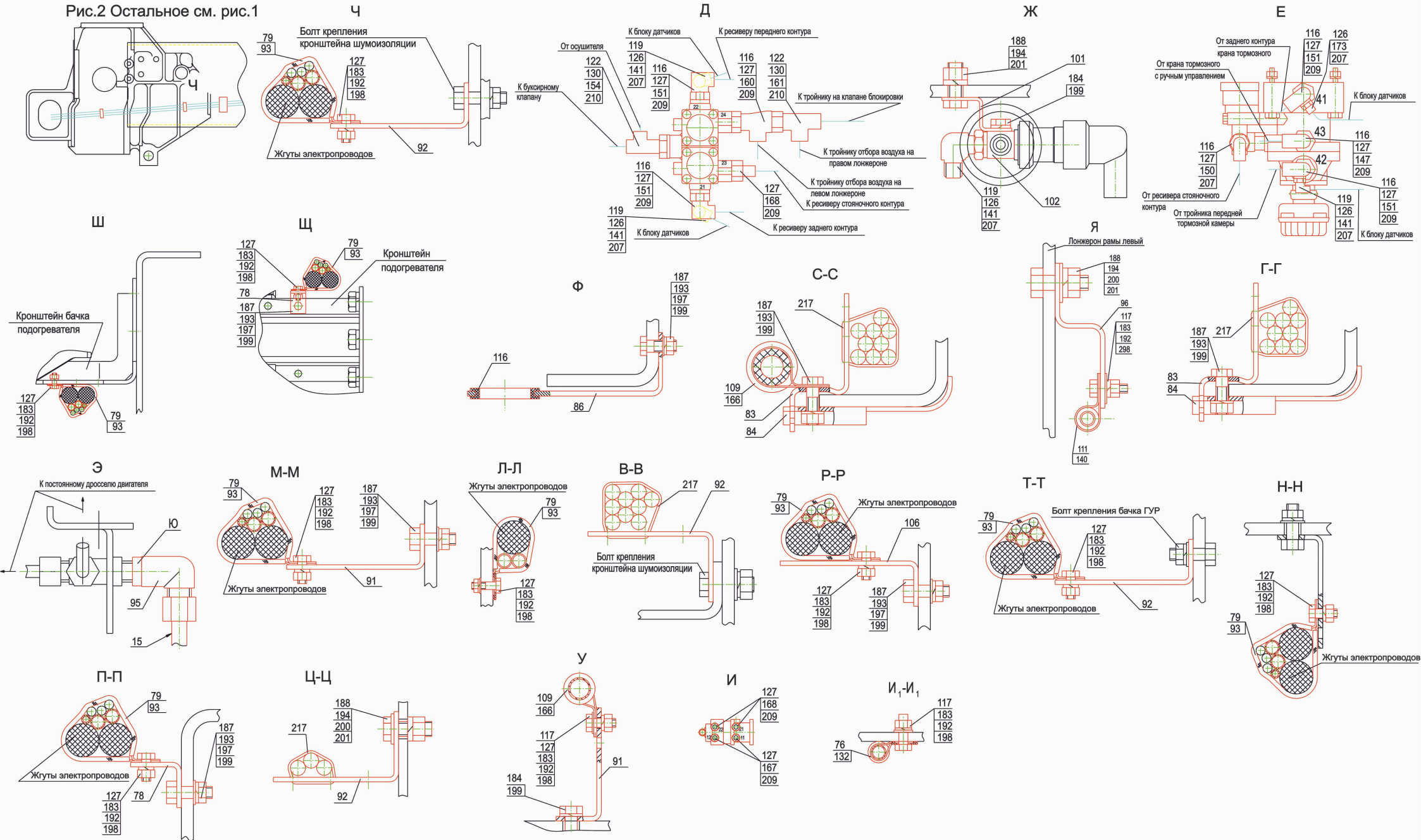
Рис. 163 Установка пневмотормозов 6310Е9-3500003 (-001) (лист 2) Fig. 163 Installation pneumobrakes
