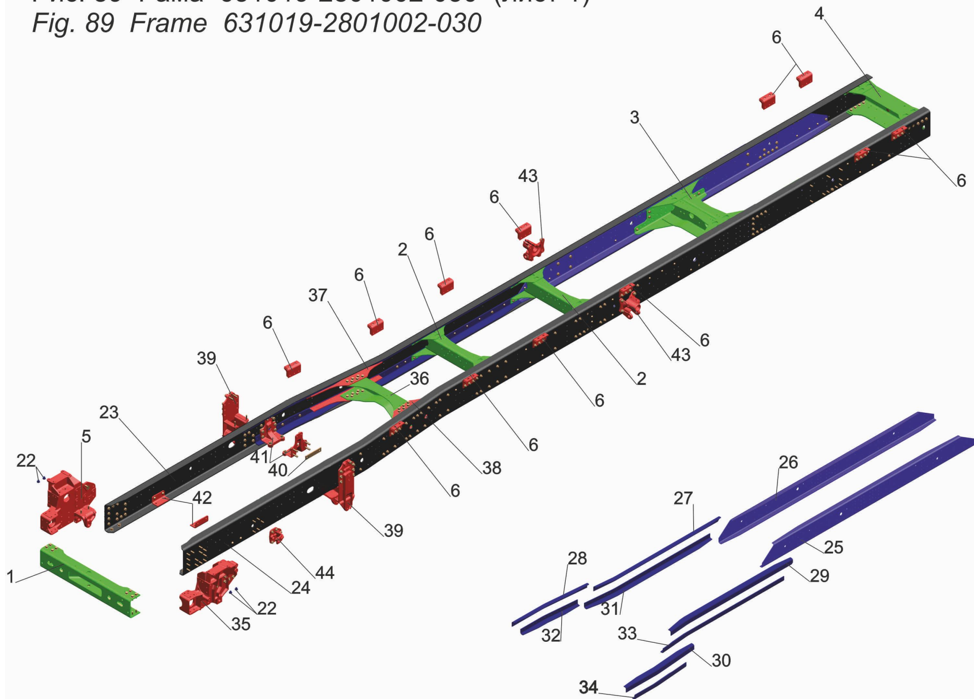
Рис. 89 Рама 631019-2801002-030 (лист 1)
