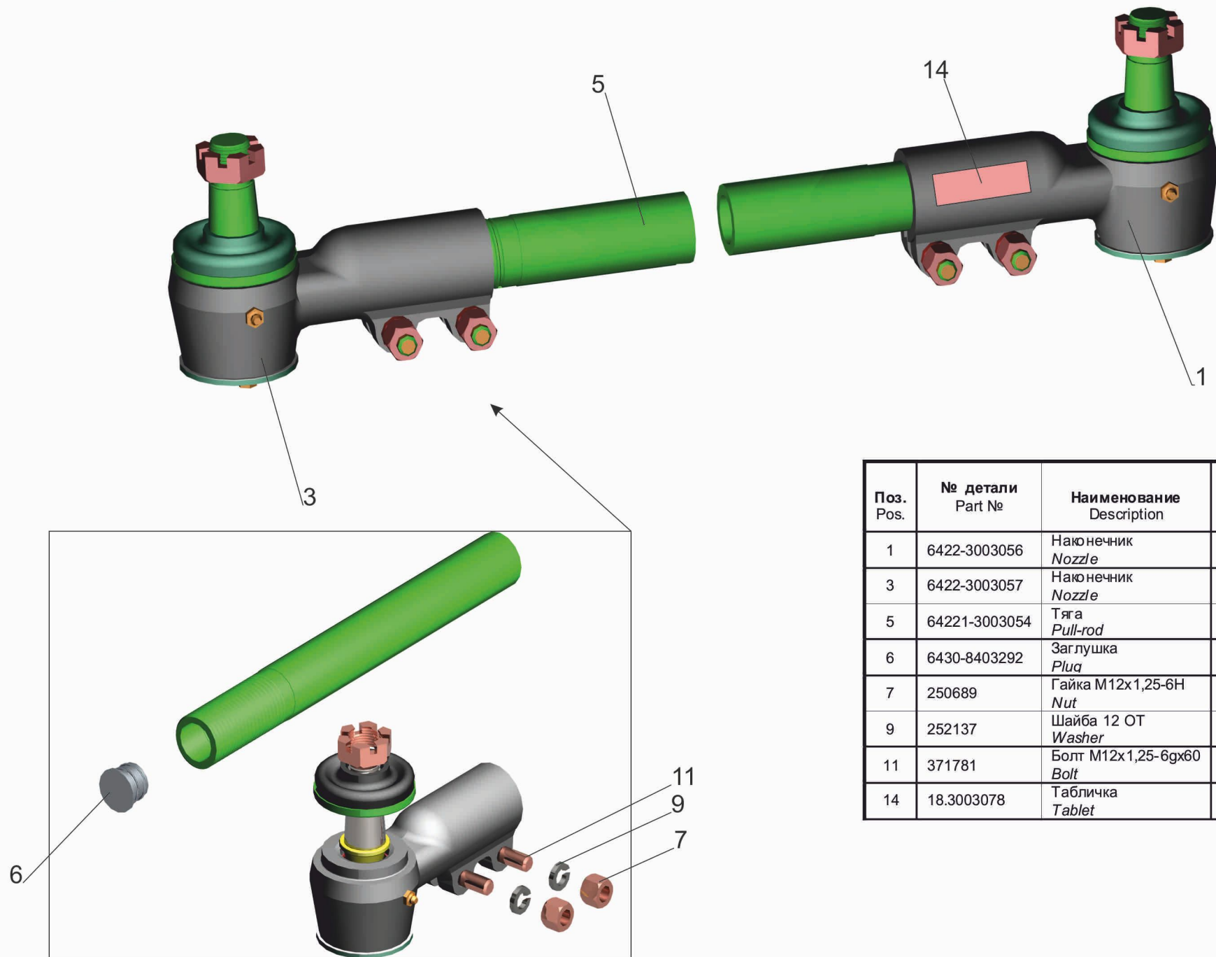
Рис. 123 Тяга поперечная 64221-3003052 Fig. 123 Pull-rod cross 64221-3003052
