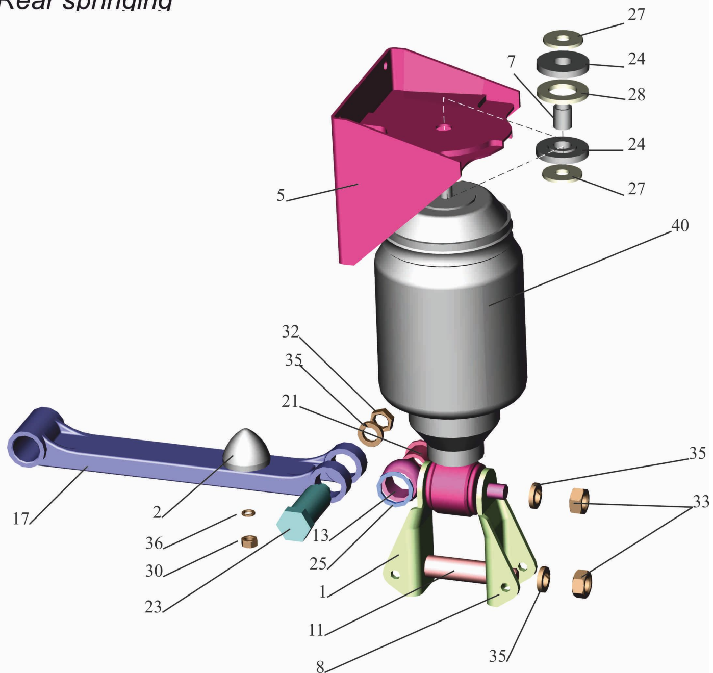
Рис. 231 Заднее подрессоривание Fig. 231 Rear springing
