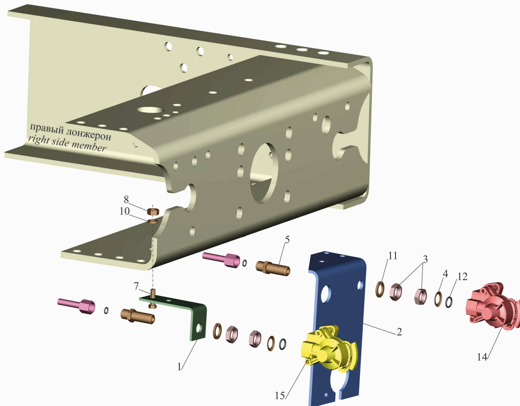
Рис. 174 Пневмовывод к прицепу 6310E9-3521004-010 Fig. 174 Pneumatic lead to trailer 6310E9-3521004-010
