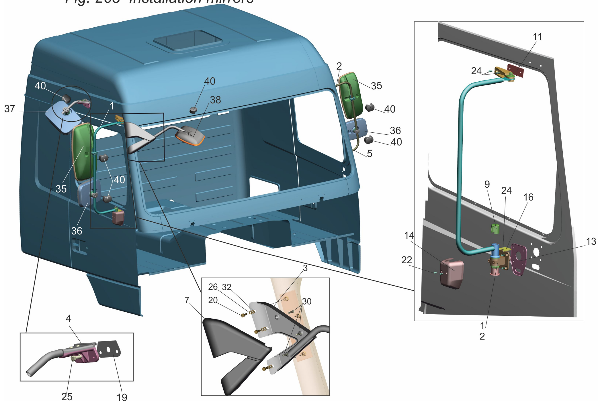
Рис. 263 Установка зеркал Fig. 263 Installation mirrors
