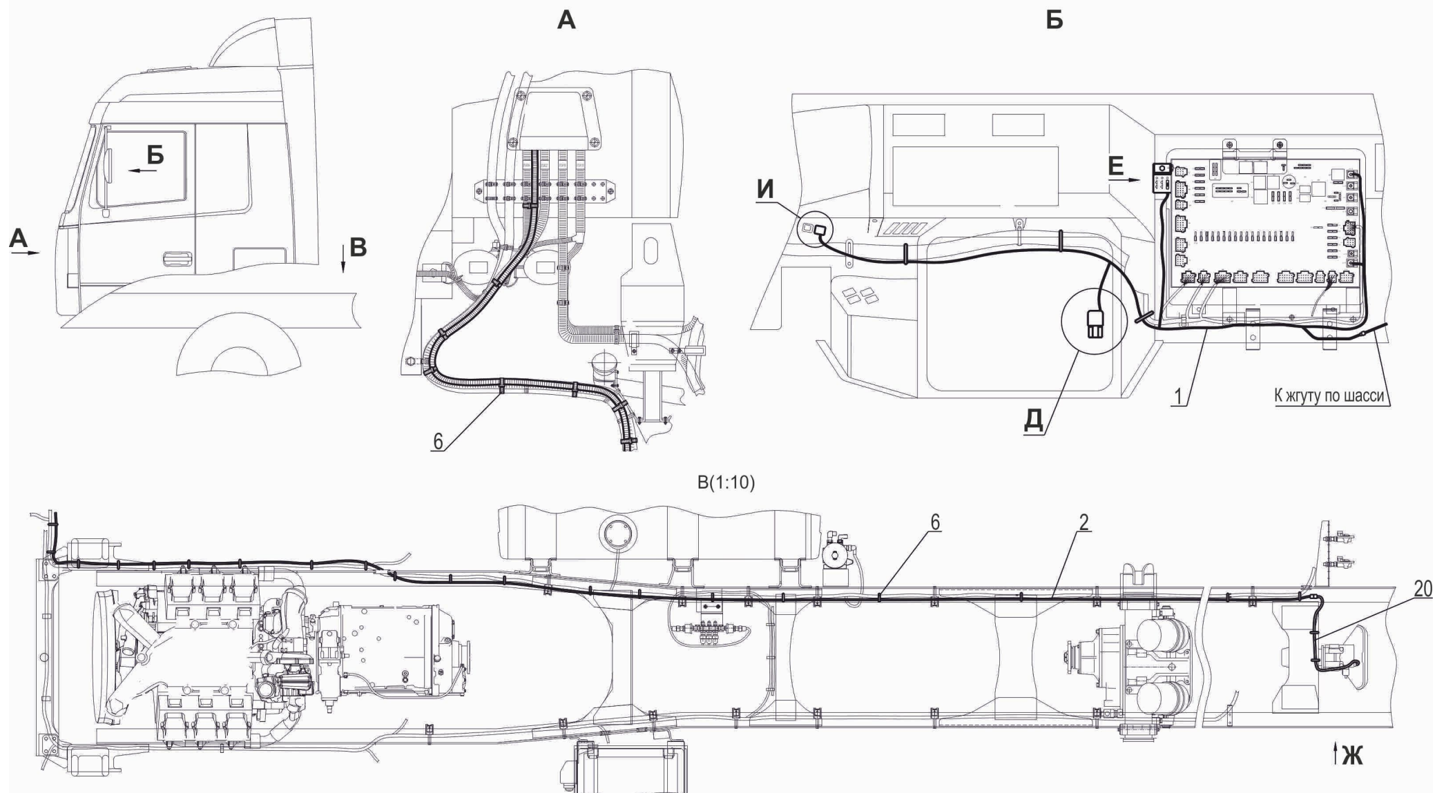
Рис. 186 Установка датчика сцепки 534019-3700164-000 (лист 1) Fig. 186 Installation of coupling sensor 534019-3700164-000 (page 1)
