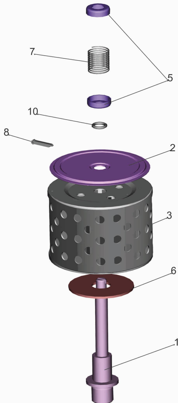
Рис. 154 Фильтр с клапаном 5336-3410051 Fig. 154 Filter with the valve 5336-3410051
