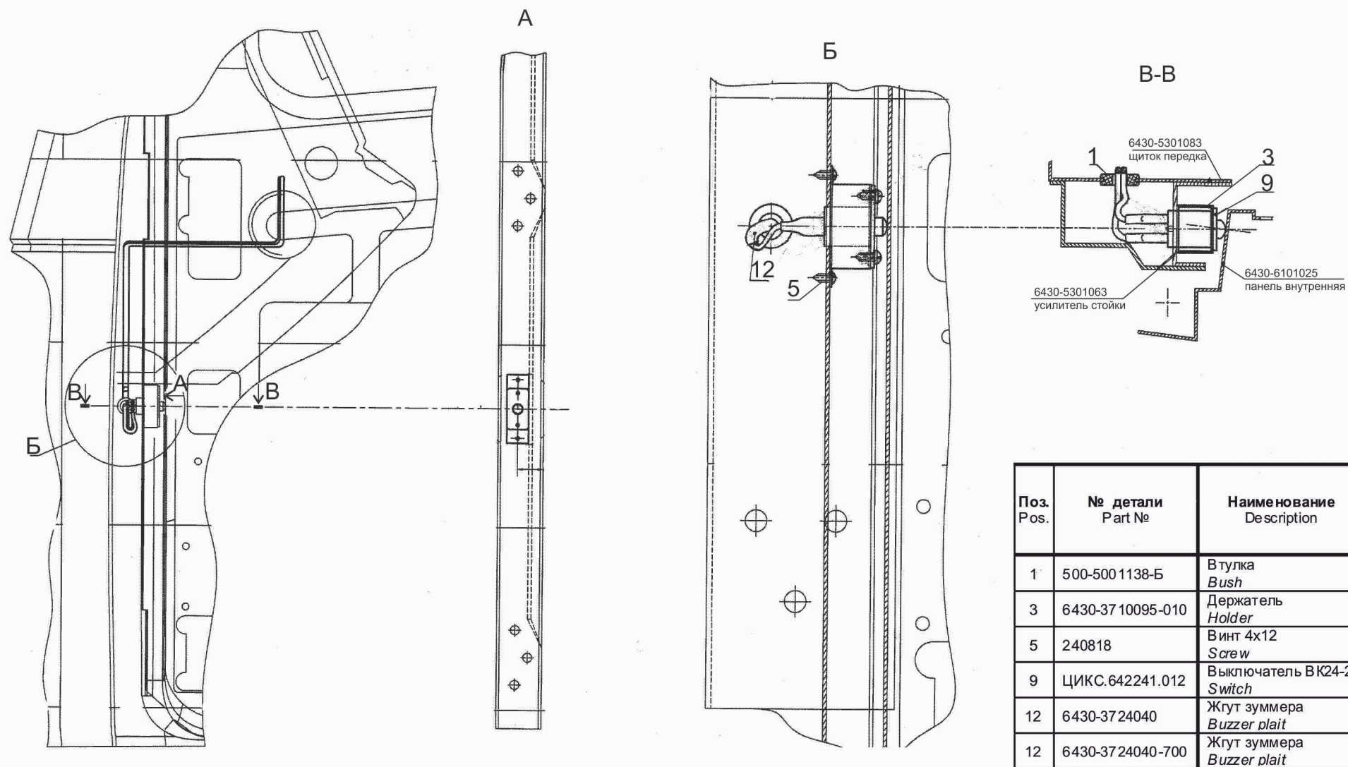
Рис. 204 Установка датчика открытой двери 6430-3700218-010 Fig. 204 Installation of the gauge of an open door 6430-3700218-010
