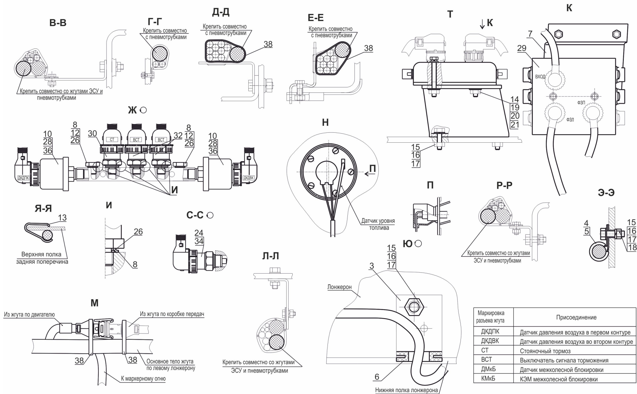
Рис. 196 Установка электрооборудования на шасси 6310E9-3700010-000, (-700) (лист 2) Fig. 196 Installation of electrical equipment on the chassis 6310E9-3700010-000, (-700) (page 2)
