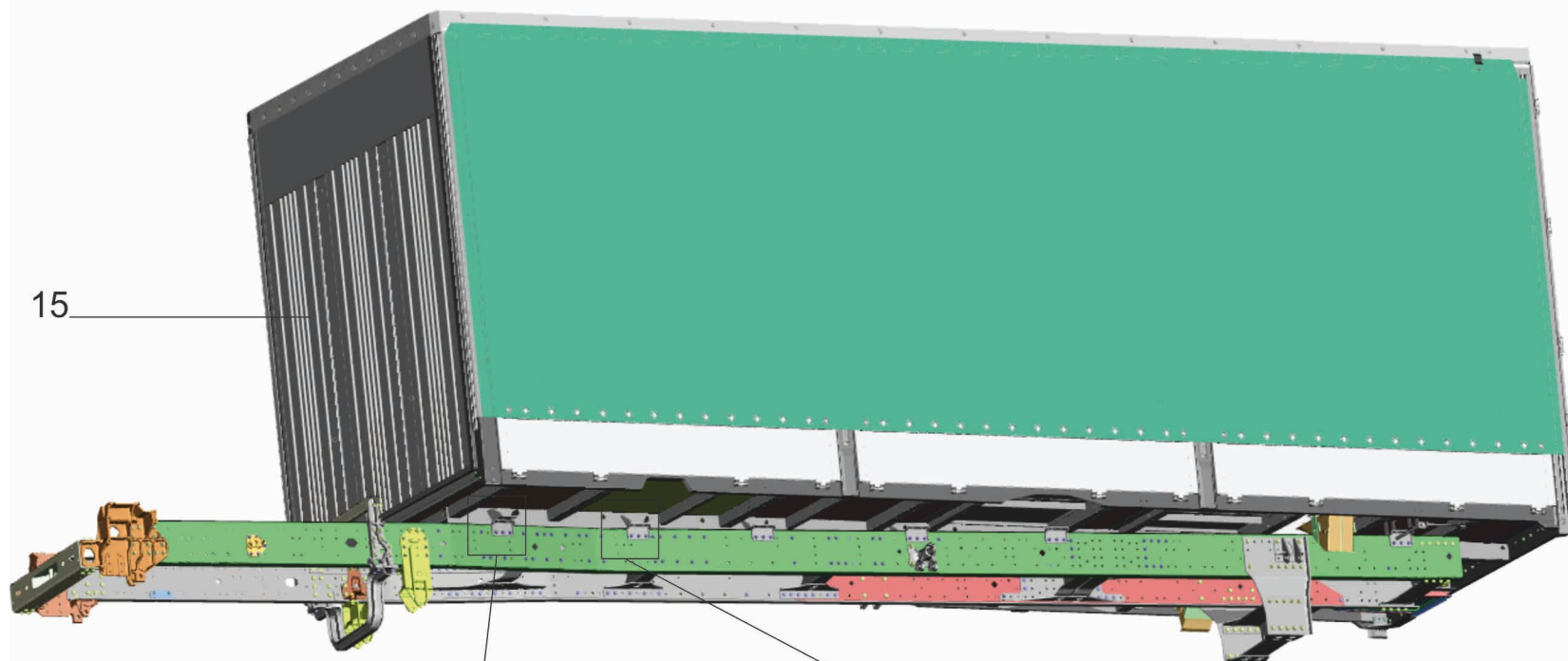
Рис. 312 Установка платформы 631014-8500002-020 Fig. 312 Installation of platform
