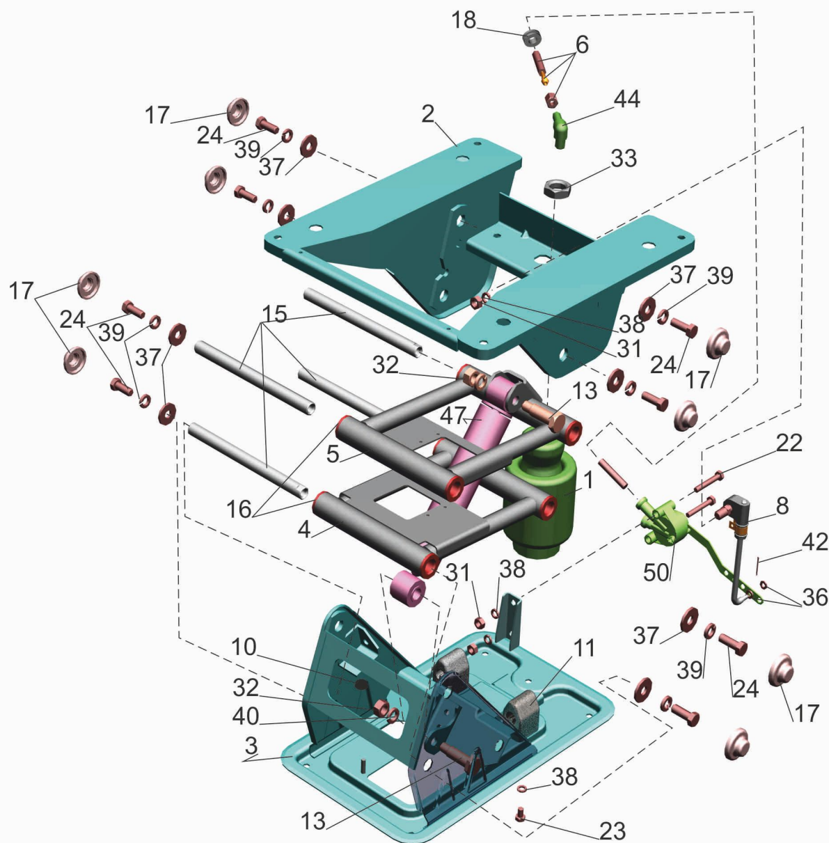
Рис. 253 Подставка сиденья с пневмооборудованием 6430-6807006-010 Fig. 253 Seat support with pneumatic equipment 6430-6807006-010
