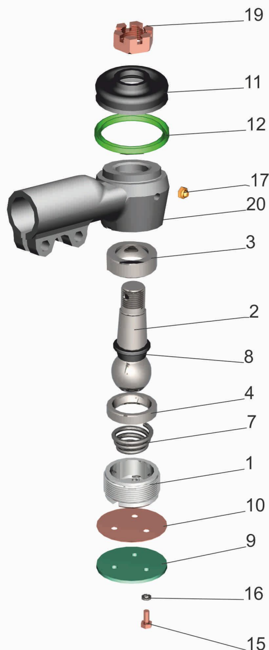
Рис. 126 Наконечник 6422-3003057 Fig. 126 Nozzle 6422-3003057
