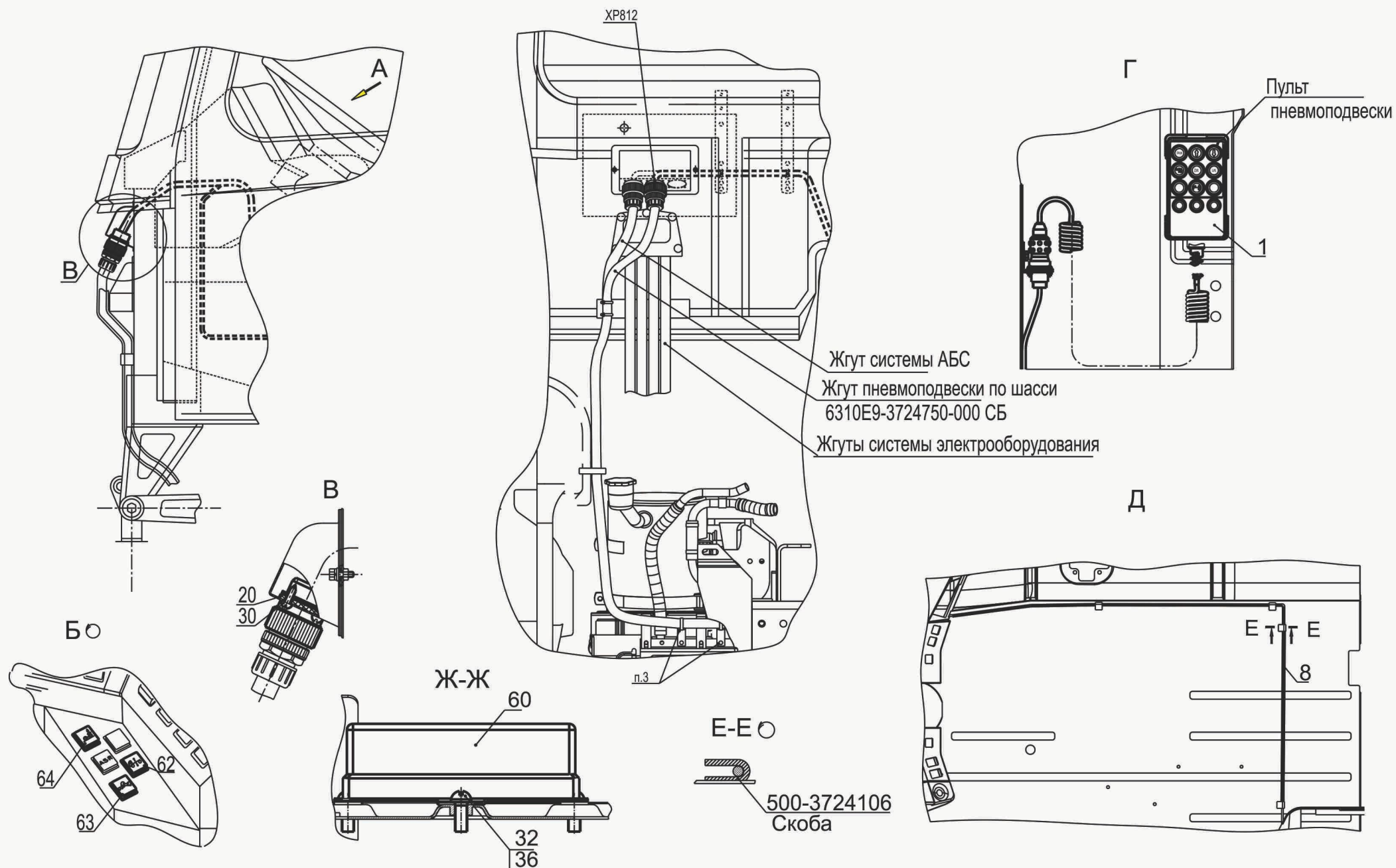
Рис. 218 Установка электрооборудования пневмоподвески по кабине 631019-3700128 (лист 1) Fig. 218 Setting of electrical equipment pneumosuspender on cabin 63101919-3700128 (page 1)
