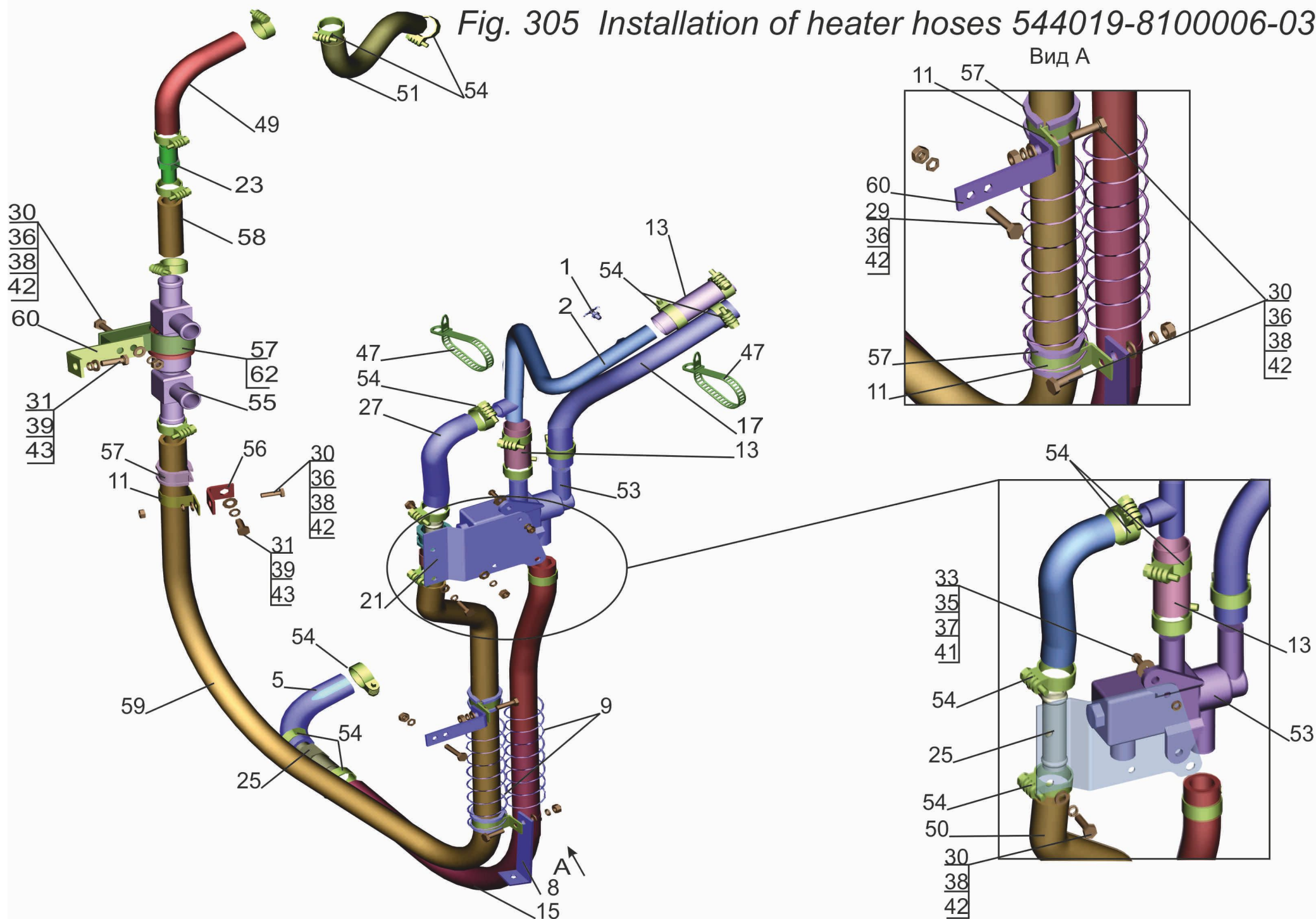
Рис. 305 Установка шлангов отопителя 544019-8100006-030
