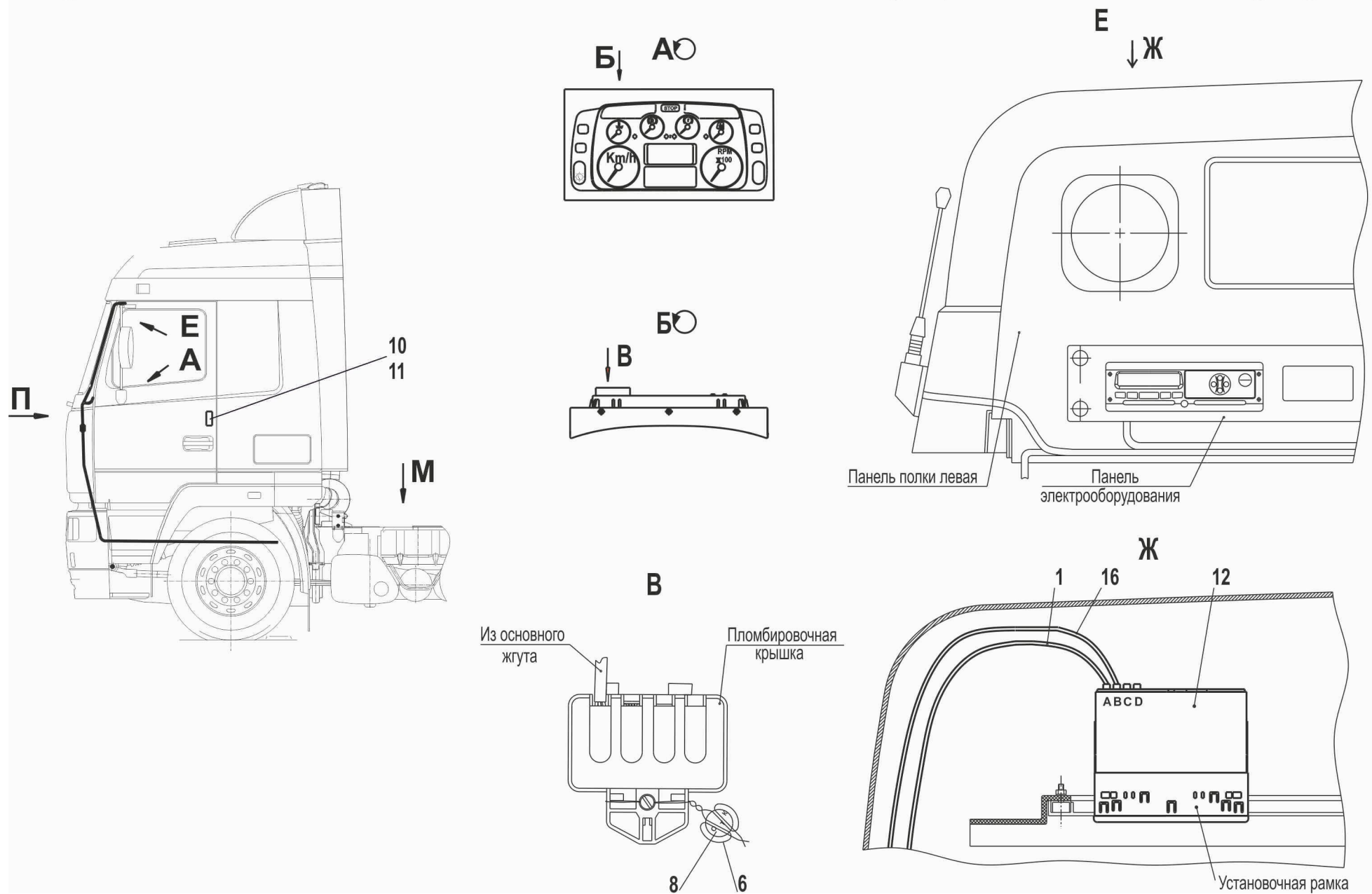
Рис. 189 Установка и пломбировка тахографа 5440-3800005 (лист 1) Fig. 189 Installation and identification seal of tachograph 5440-3800005 (page 1)
