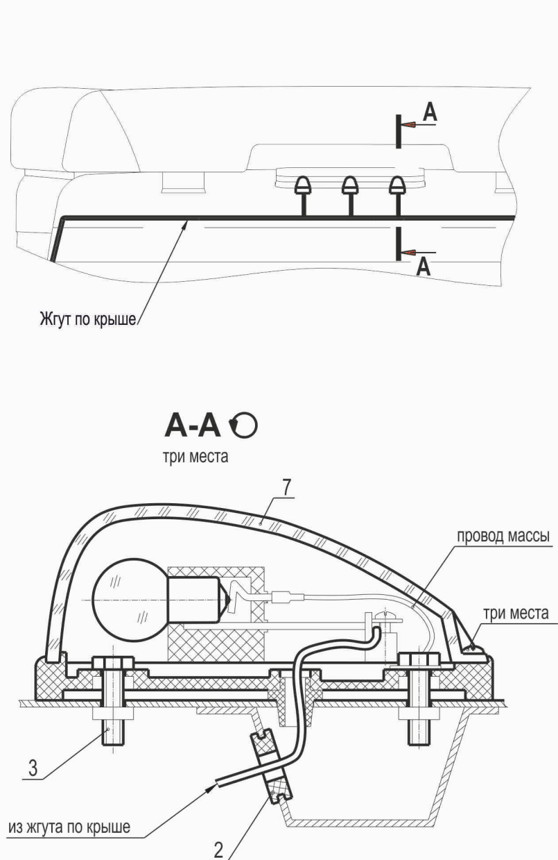
Рис. 208 Установка фонарей знаков автопоезда 6430-3700099, 6430-3700099-700 Fig. 208 Installation of long vehicle signal 6430-3700099, 6430-3700099-700
