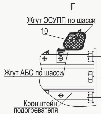
Рис. 217 Установка электрооборудования пневмоподвески 631019-3800050 (лист 2) Fig. 217 Setting of electrical equipment pneumosuspender 631019-3800050 (page 2)
