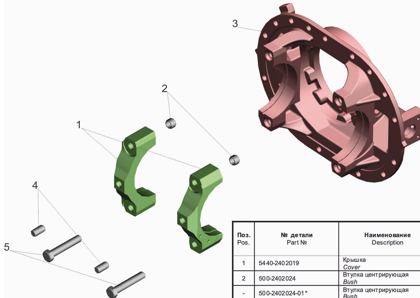
Рис. 76 Картер редуктора 5440-2402015-010 Fig. 76 Reducer gear housing 5440-2402015-010
