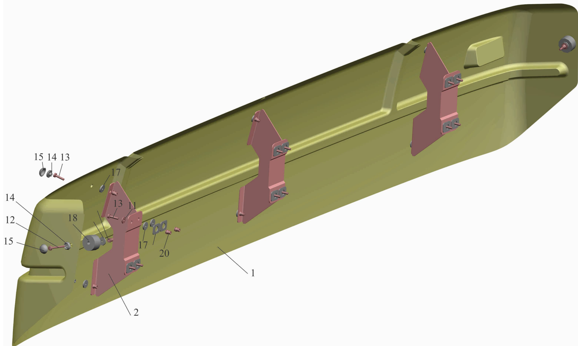
Рис. 279 Установка козырька 6430-8000012 Fig. 279 Installation deflector 6430-8000012
