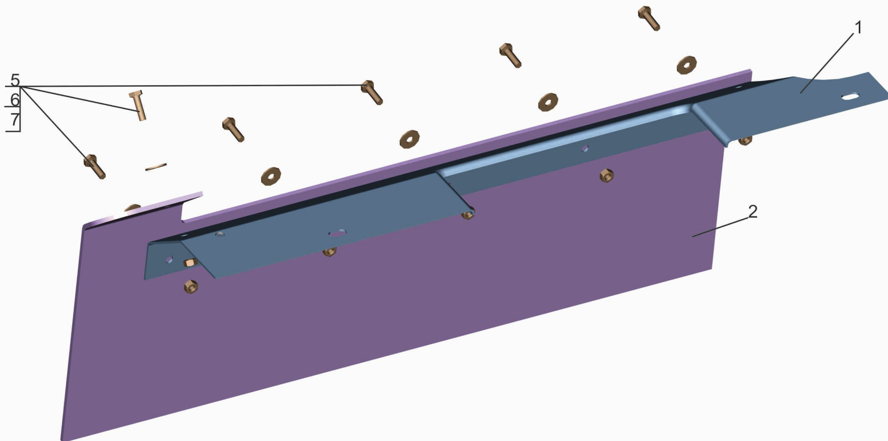
Рис. 29 Уплотнитель с пластиной 544019-1310068-010 Fig. 29 Seal with plate 544019-1310068-010
