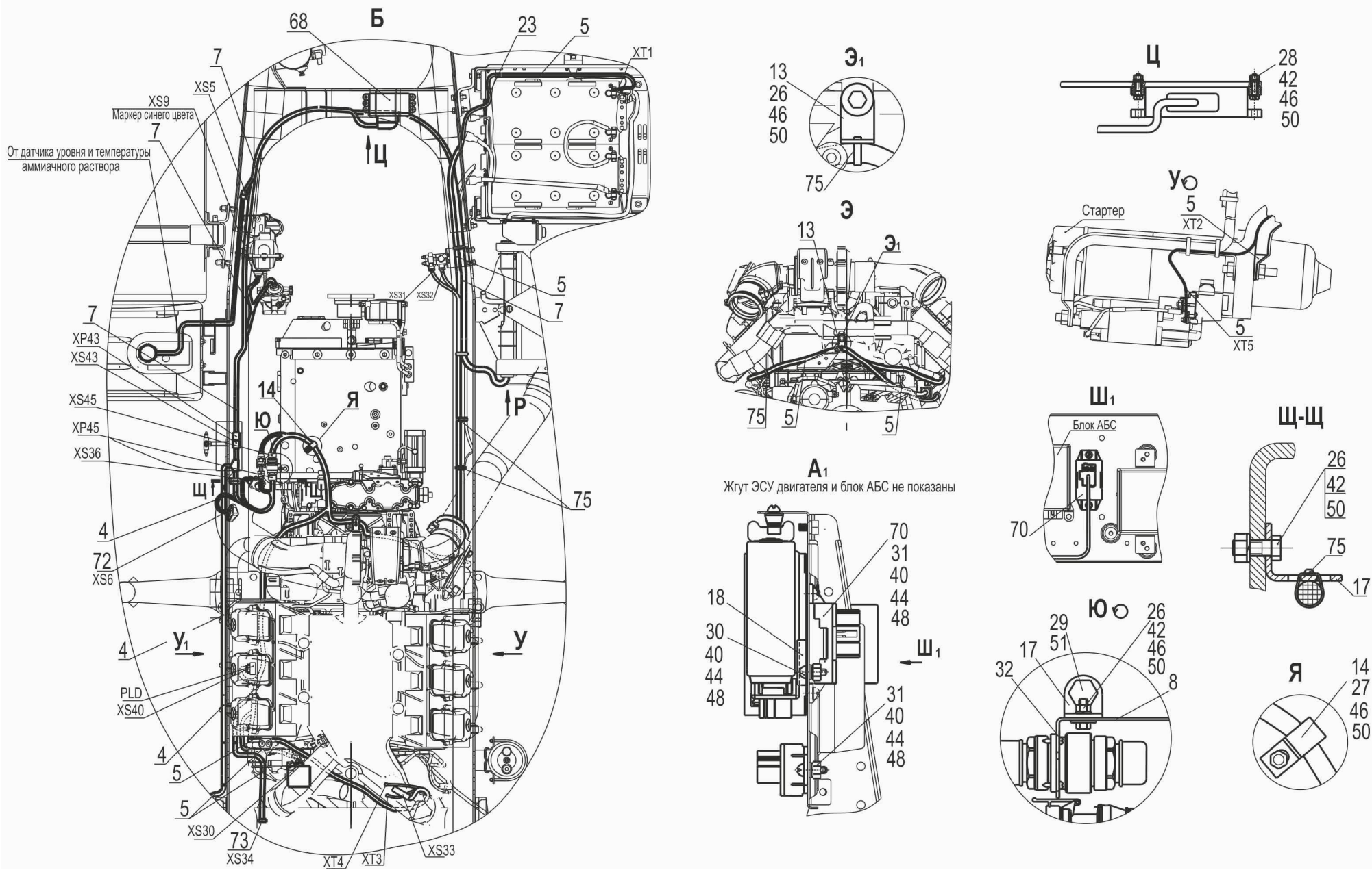
Рис. 220 Установка электрооборудования ЭСУ двигателя 5440Е9-3800060-000 (лист 3) Fig. 220 Installation of electronic control system of the engine 5440Е9-3800060-000 (page 3)
