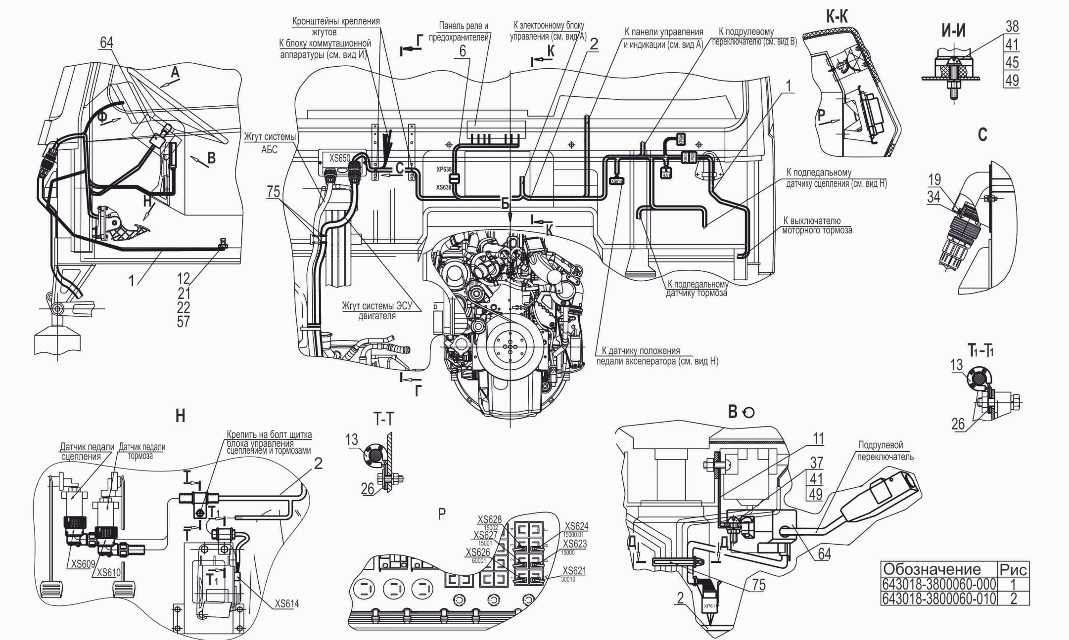
Рис. 221 Установка электрооборудования ЭСУ двигателя 643018-3800060-000,(-010) (лист 1) Fig. 221 Installation of electronic control system of the engine 643018-3800060-000,(-010) (page 1)
