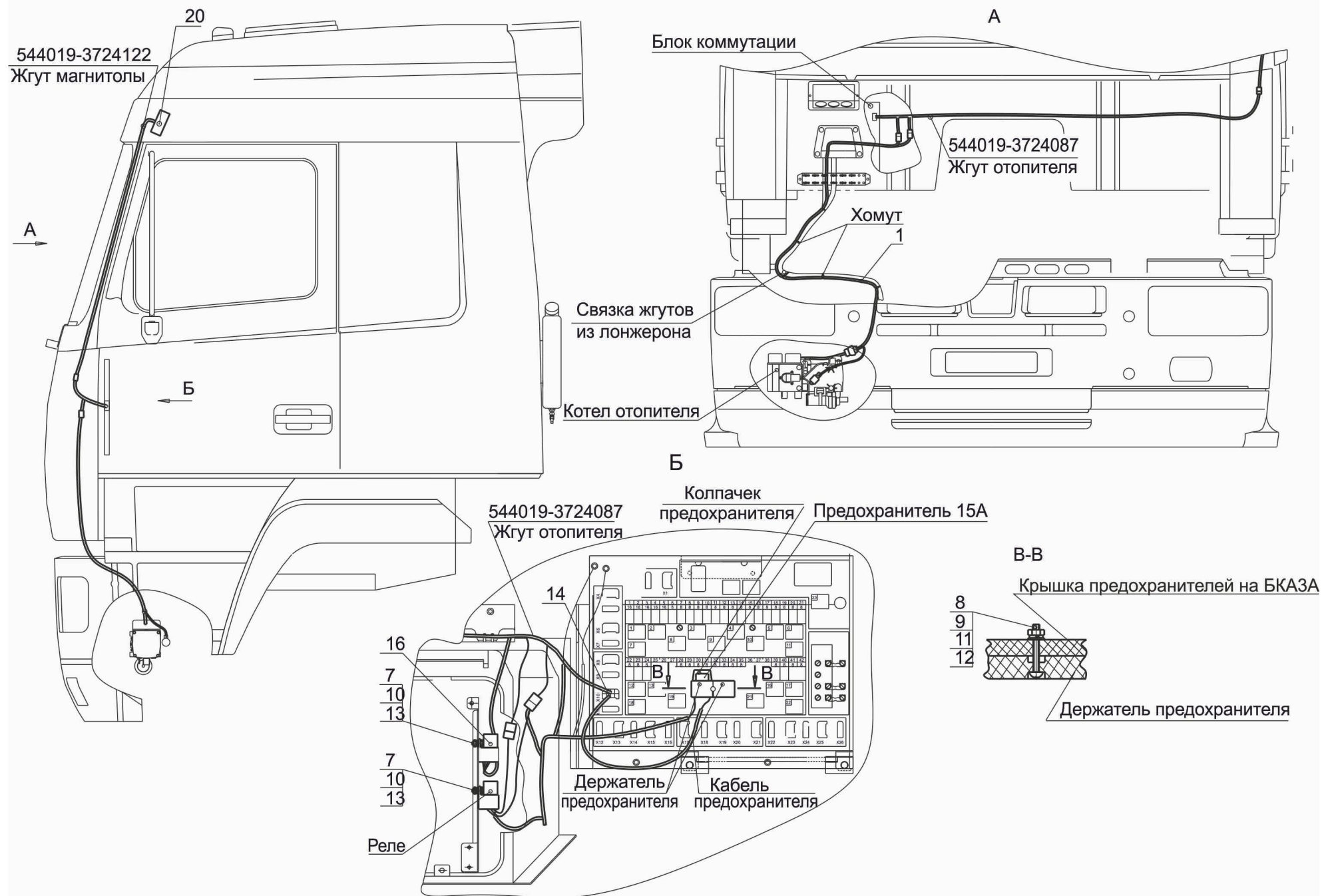
Рис. 8 Установка электрооборудования подогревателя 544019-3700085 Fig. 8 Mounting of electrical equipment heater 544019-3700085
