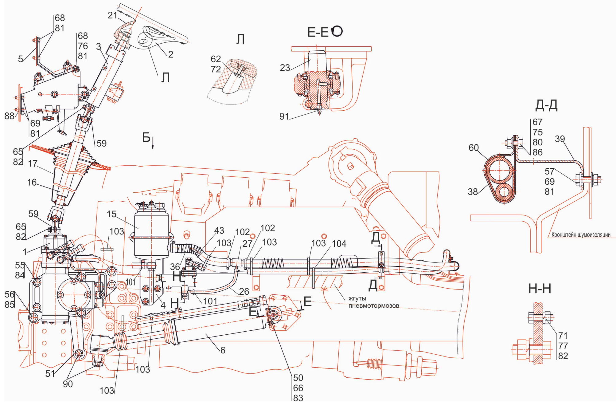
Рис. 138 Установка рулевого управления 631019-3400001 (лист 1) Fig. 138 Steering installation 631019-3400001 (page 1)
