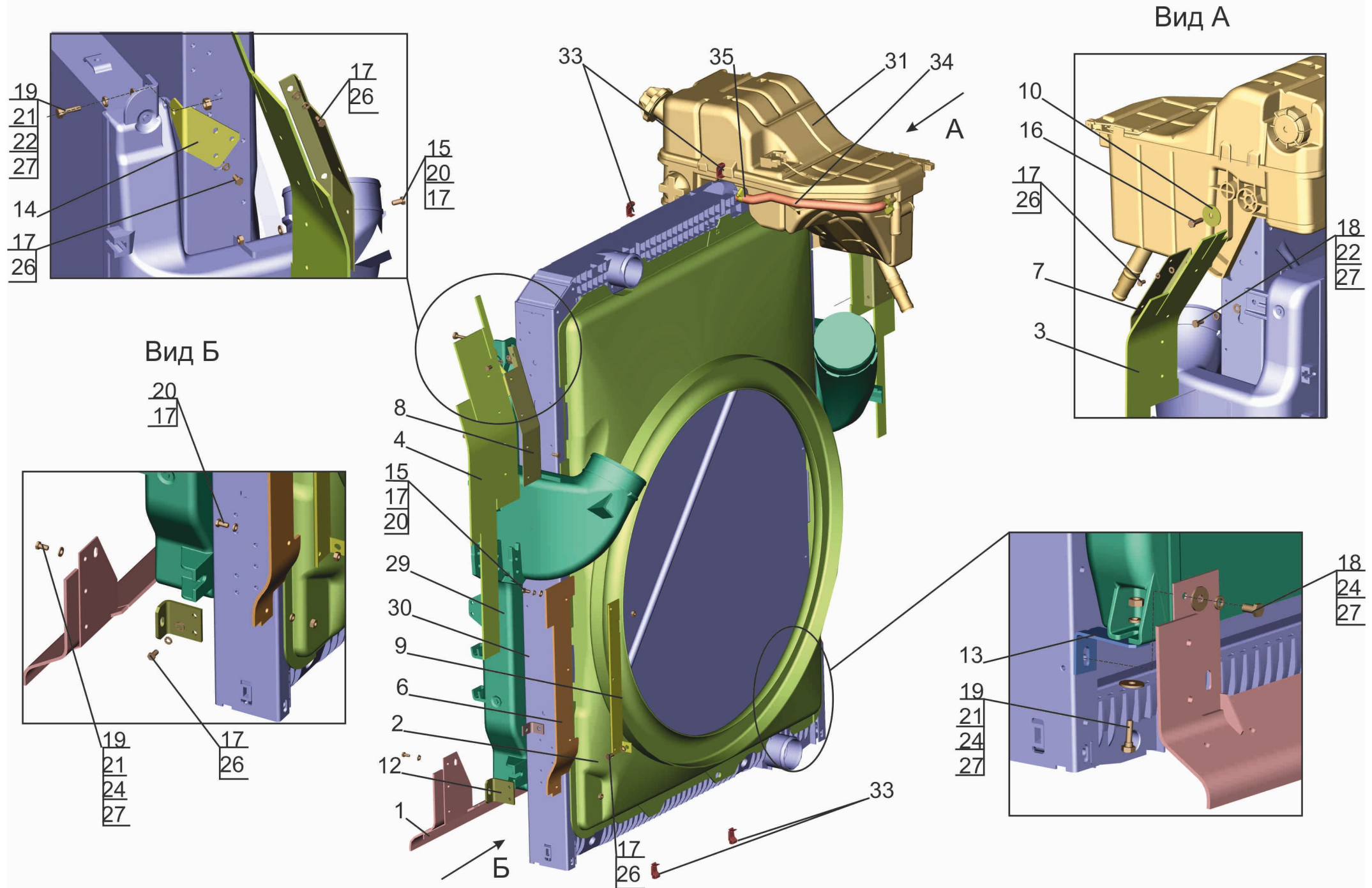
Рис. 31 Радиатор с кожухом 544019-1301009 Fig. 31 Cooler with housing 544019-1301009
