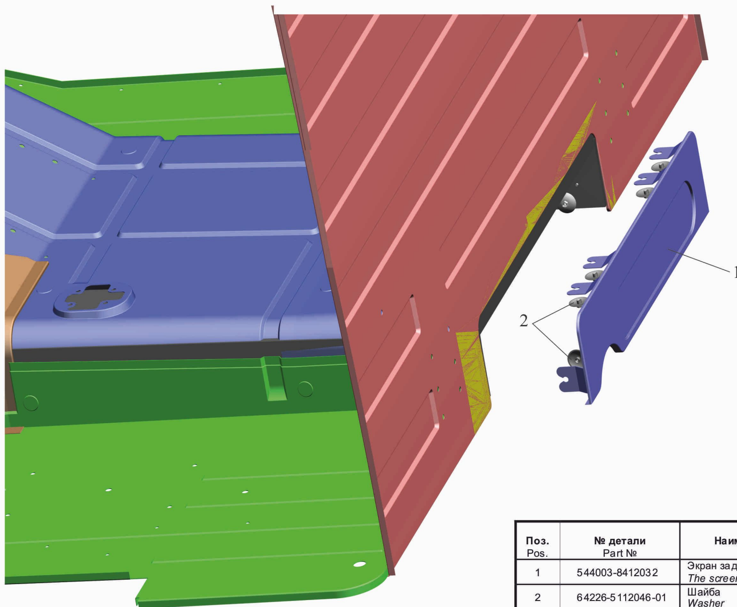
Рис. 308 Установка экранов 544003-8400026 Fig. 308 Installation of screens 544003-8400026
