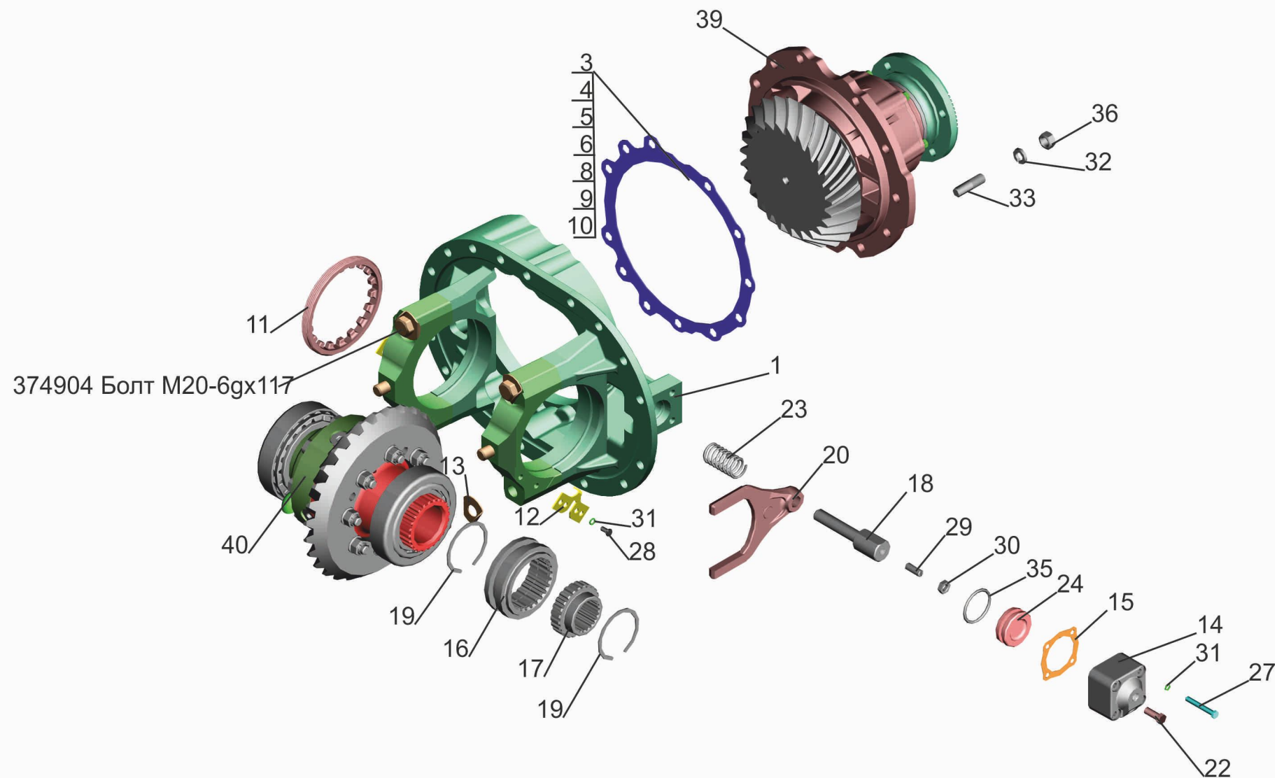
Рис. 75 Редуктор заднего моста Fig. 75 Reducer gear
