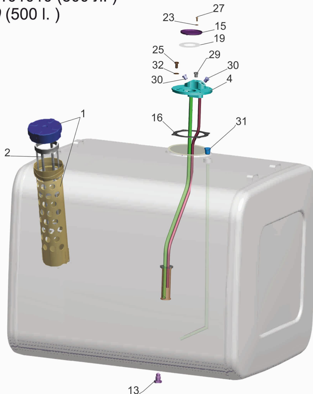
Рис. 14 Бак топливный 5440B9-1101010 (500 л. )
