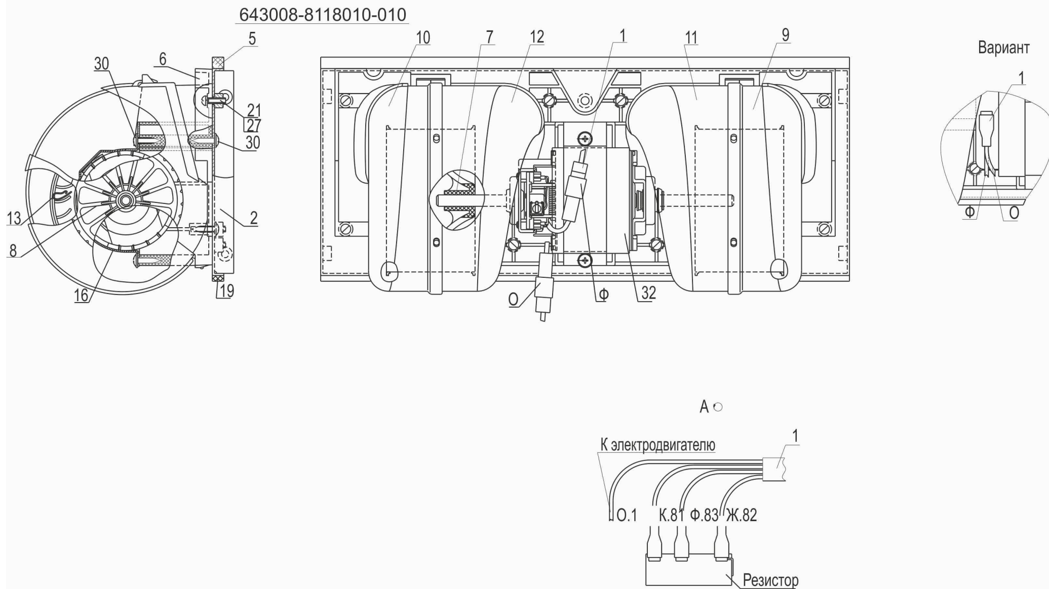
Рис. 289 Блок вентиляторный 643008-8118010-010, (-030) Fig. 289 Fan unit 643008-8118010-010, (-030)
