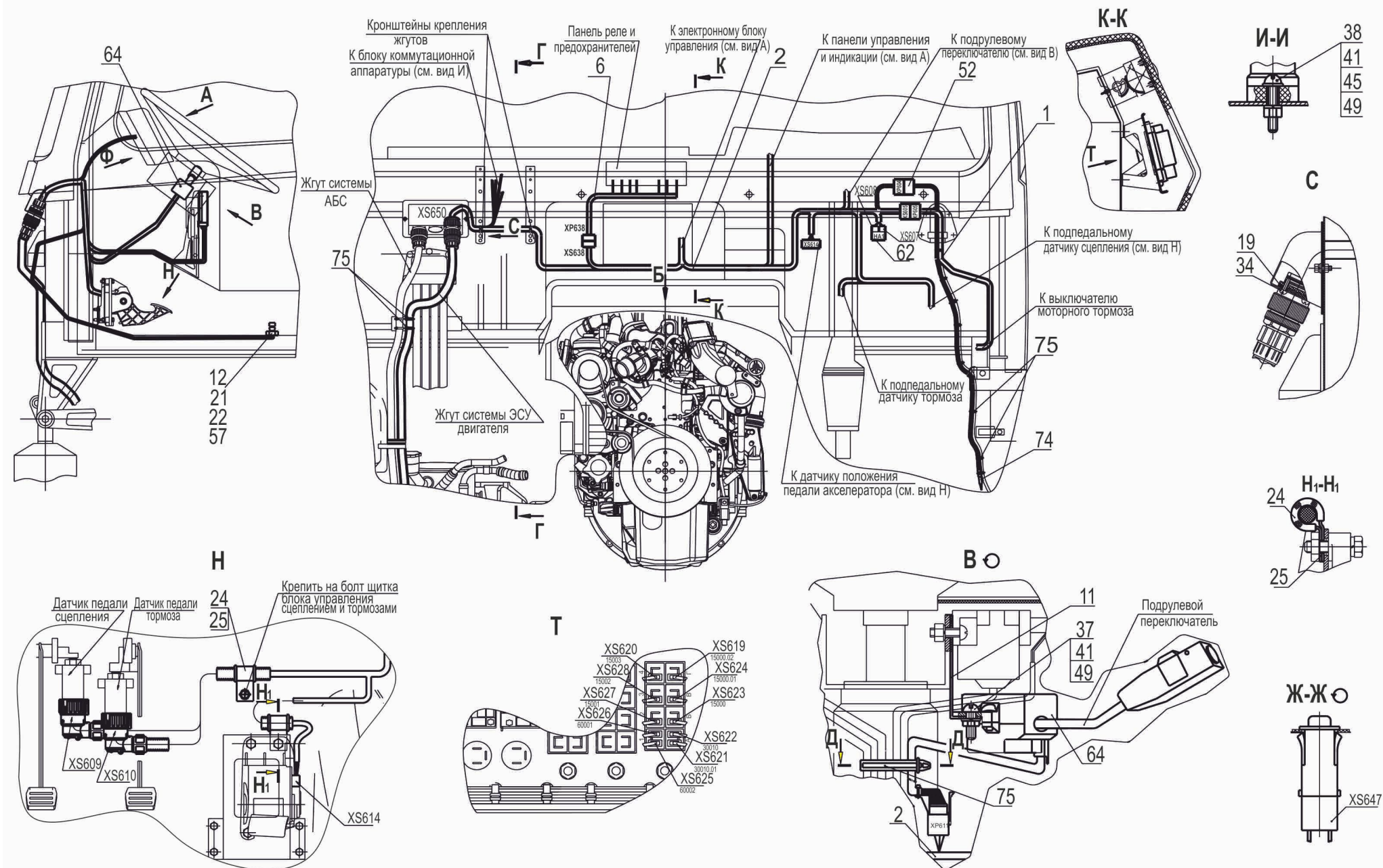
Рис. 220 Установка электрооборудования ЭСУ двигателя 5440E9-3800060-000 (лист 1) Fig. 220 Installation of electronic control system of the engine 5440E9-3800060-000 (page 1)
