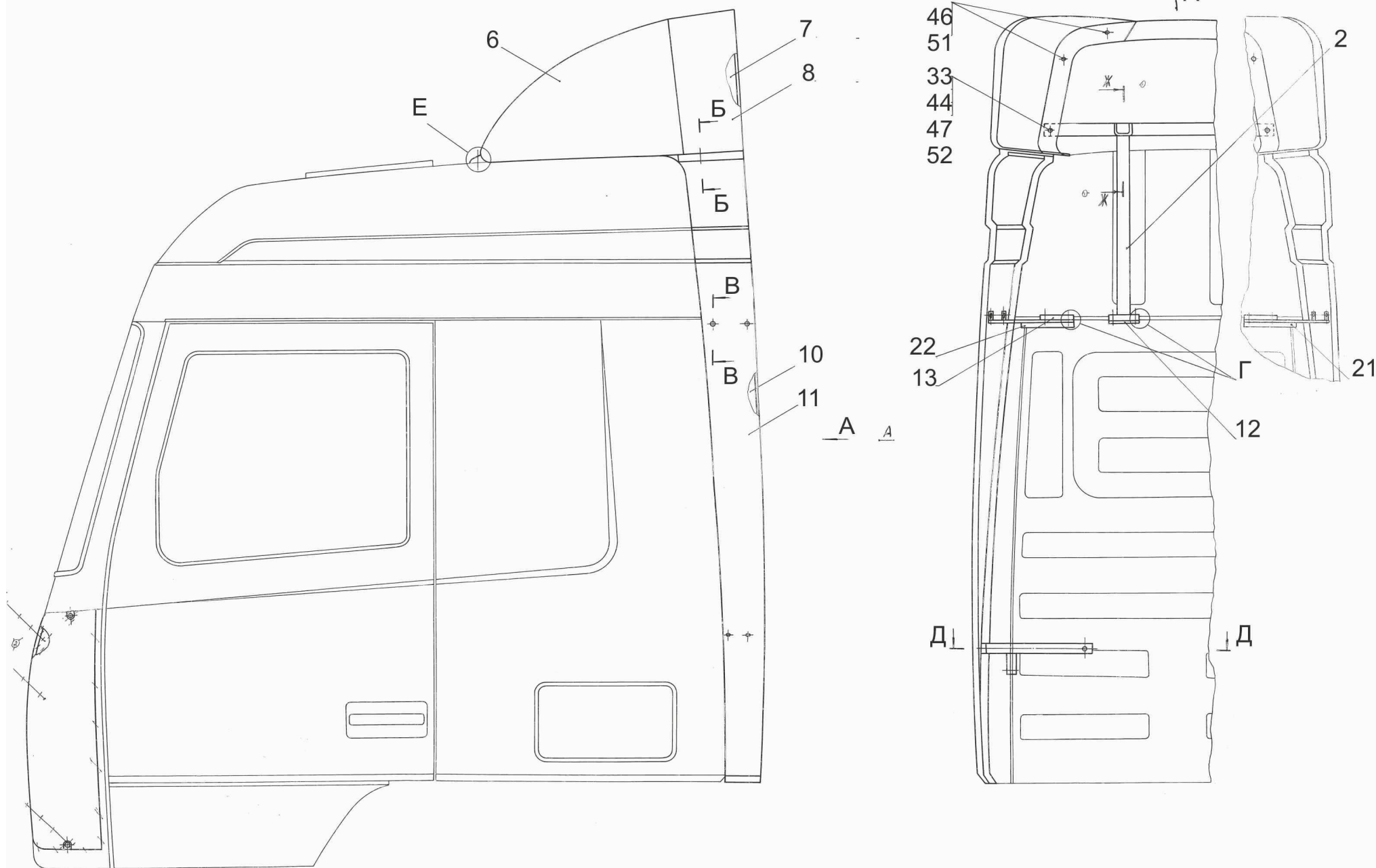
Рис. 280 Установка обтекателей 6312-8000014 Лист 1 Fig. 280 Installation of faing 6312-8000014 Page 1
