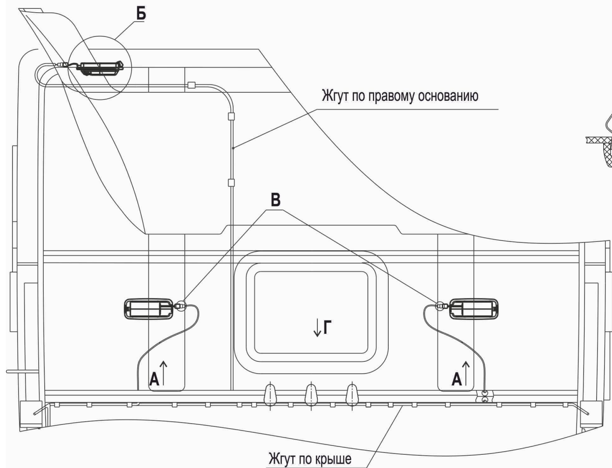
Рис. 200 Установка светильников в кабине 544008-3700136 Fig. 200 Installation of fixtures in a cabin 544008-3700136
