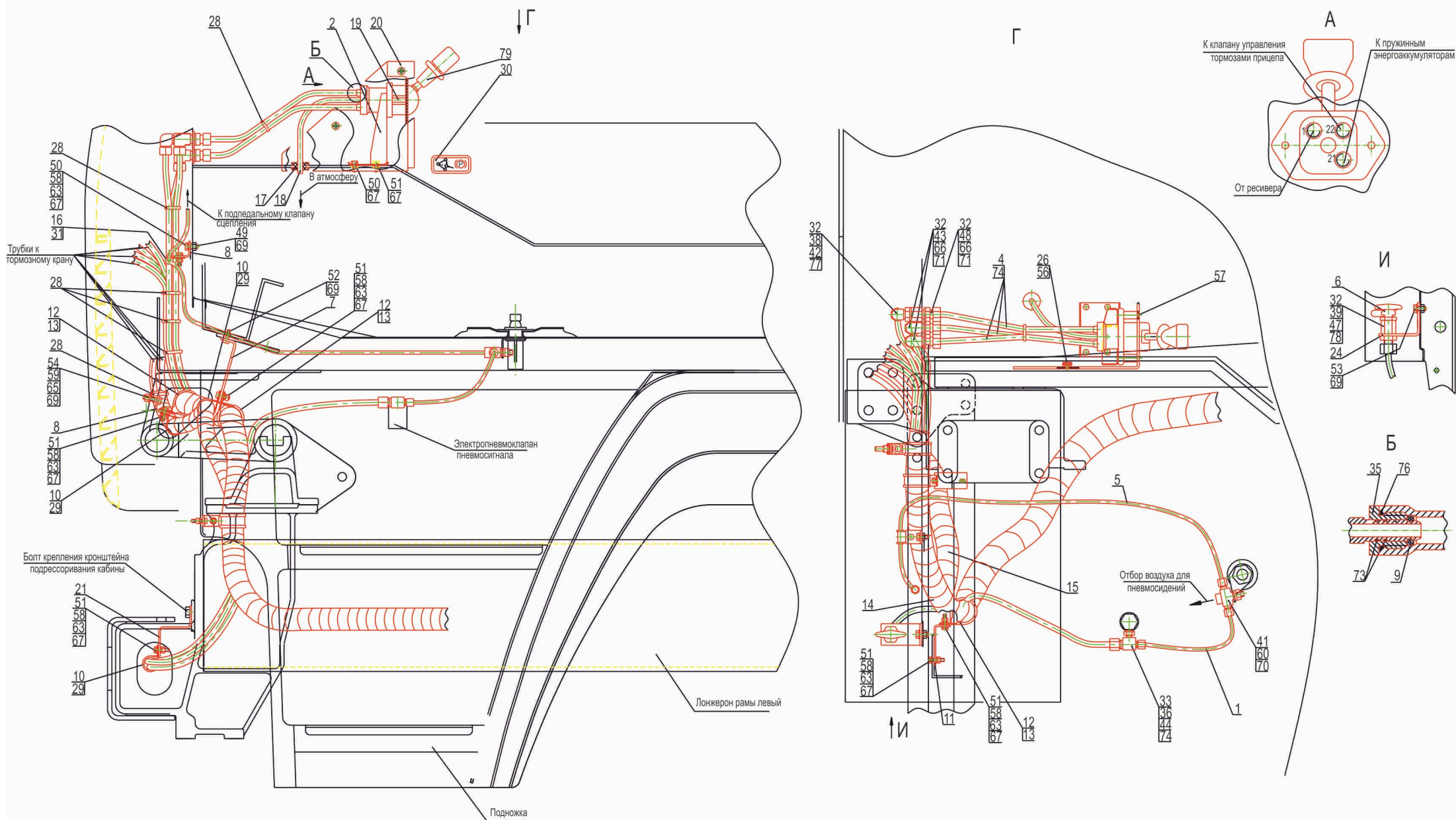
Рис. 178 Привод стояночного тормоза 544019-3537006 Fig. 178 Drive of a parking brake 544019-3537006
