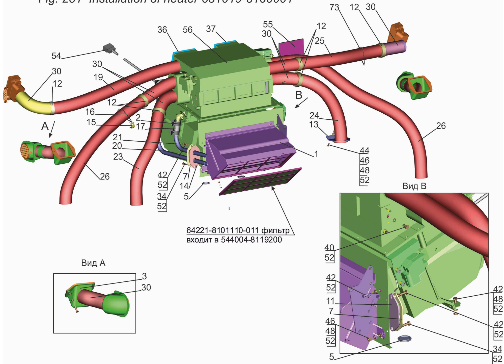
Fig. 281 Installation of heater 631019-8100001
