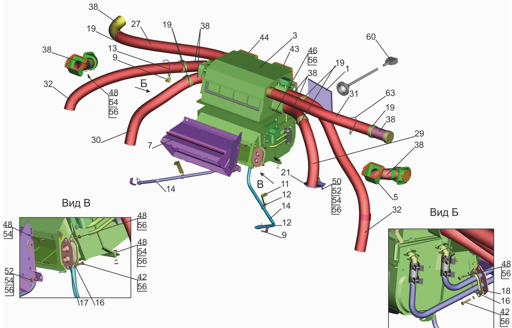
Рис. 282 Установка отопителя 631019-8100001-010 Fig. 282 Installation of heater 631019-8100001-010
