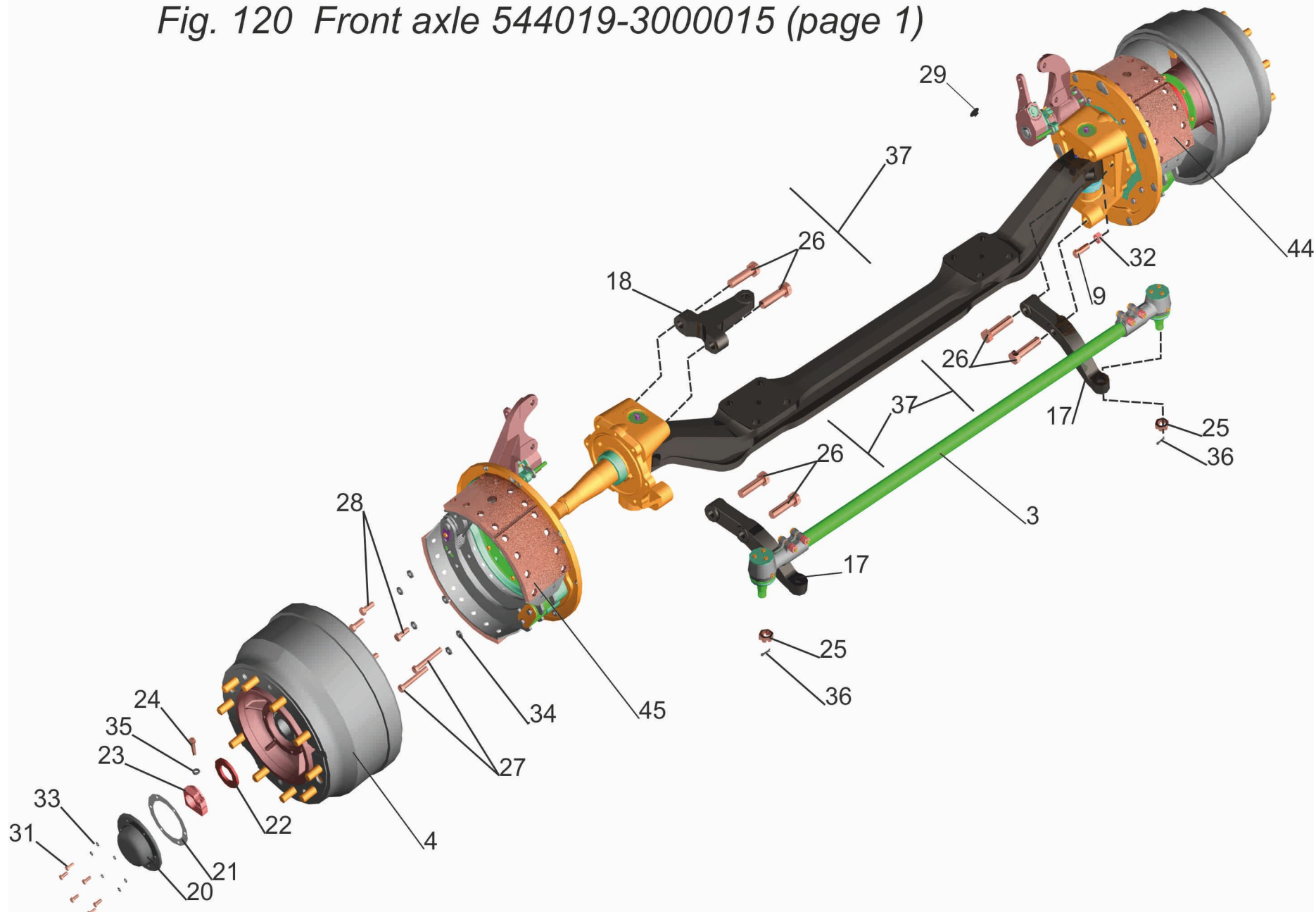
Рис. 120 Передняя ось 544019-3000015 (лист 1)
