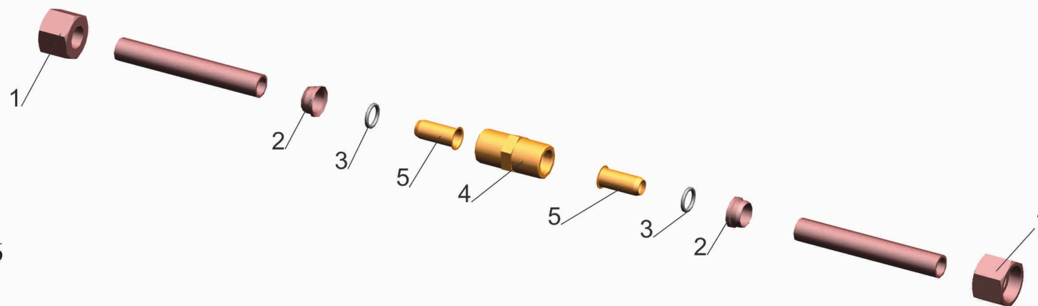
Рис.180 Соединение для ремонта поврежденных трубопроводов Fig.180 Connection for repair of the damaged pipelines
