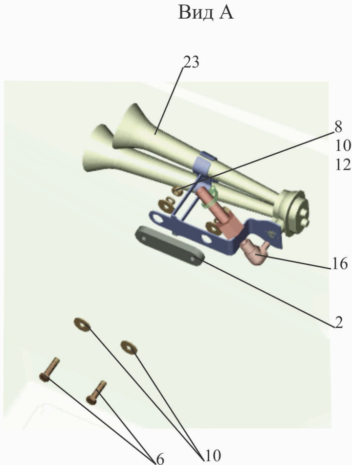
Рис. 206 Установка пневмосигнала 6430-3700096, 6430-3700096-700 Fig. 206 Mounting of air horn 6430-3700096, 6430-3700096-700
