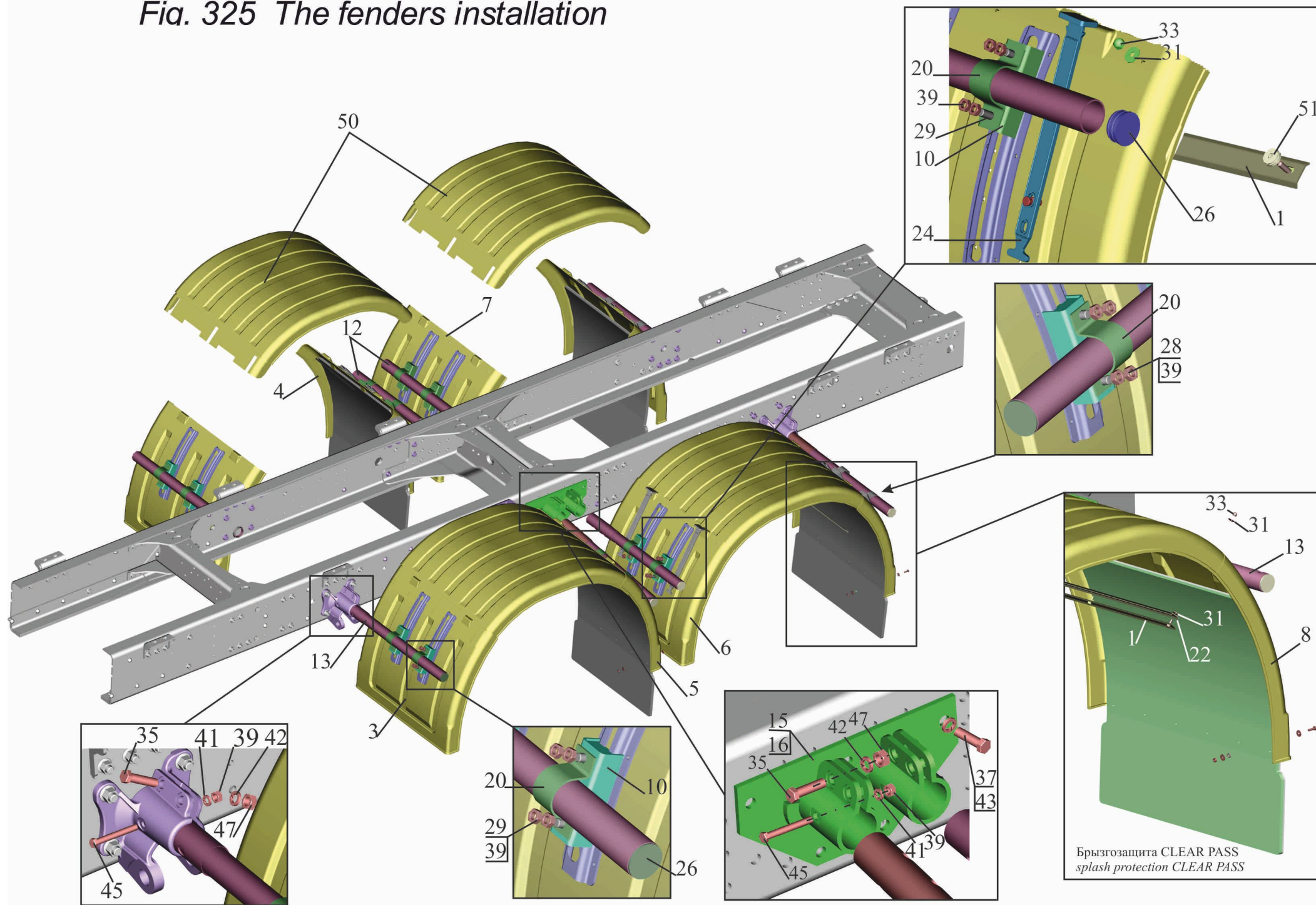
Рис. 325 Установка крыльев 6310E9-8500048-050
