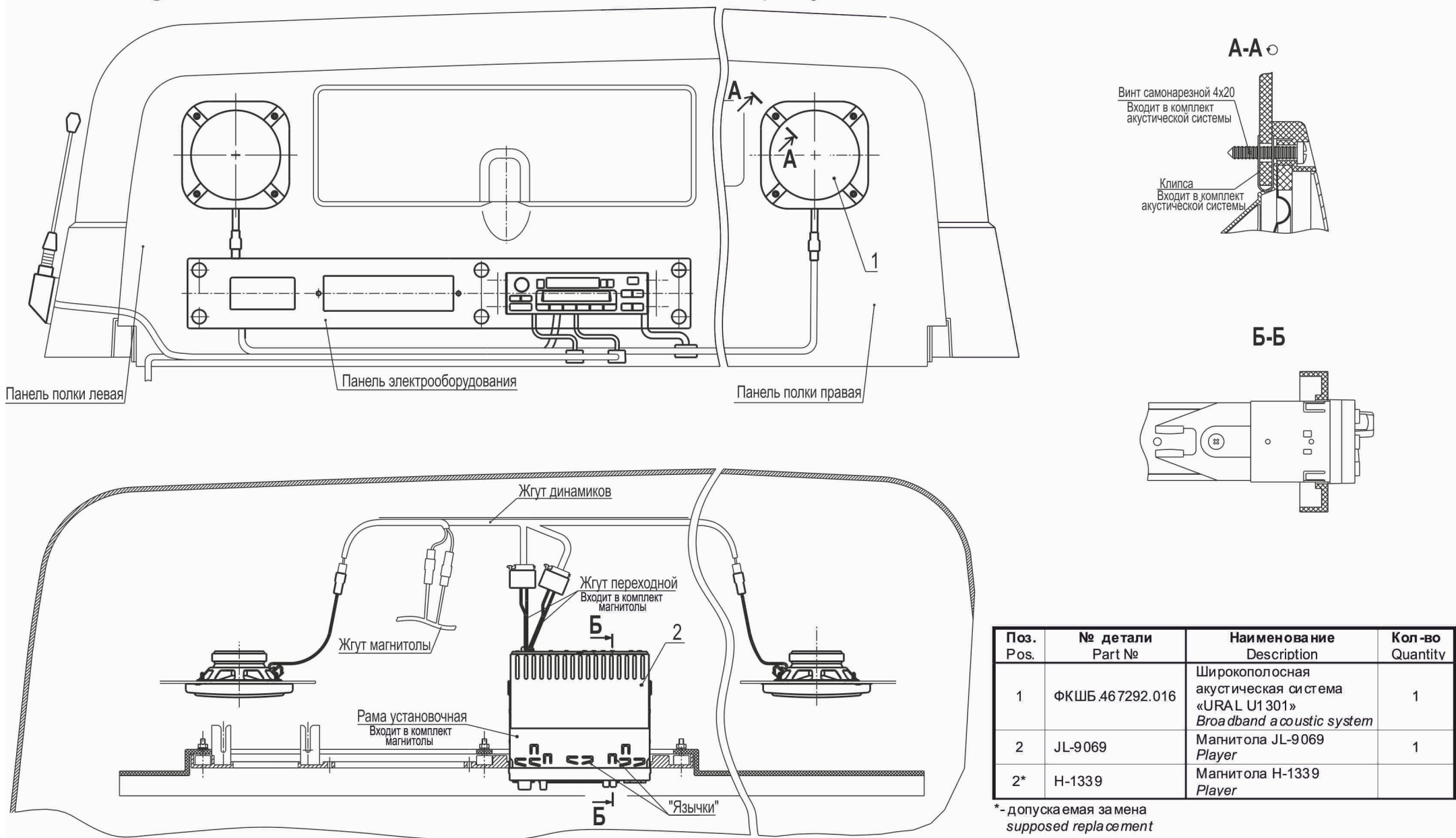
Рис. 190 Установка радиоприемника с CD проигрывателем 6430-7900030 Fig. 190 Installation of receiver with CD player 6430-7900030
