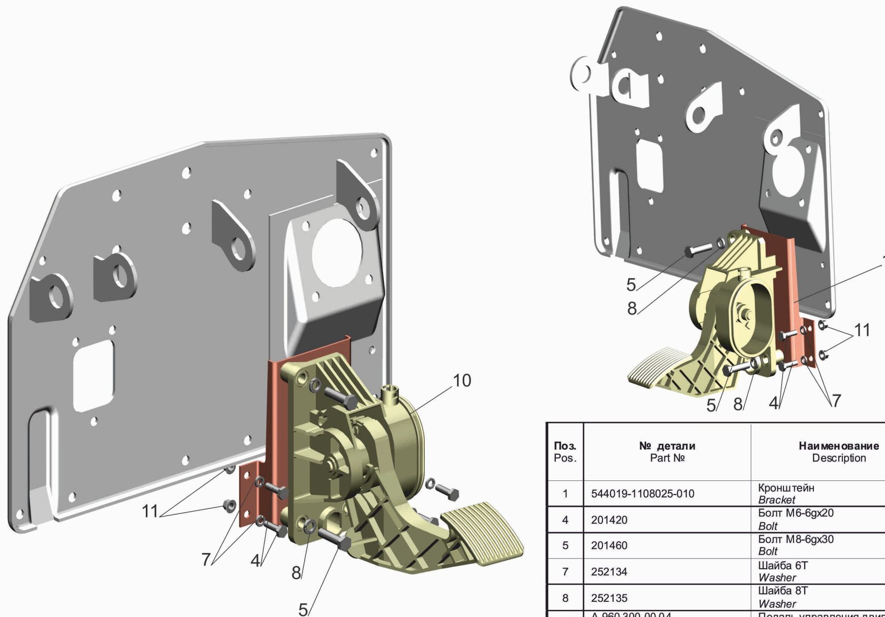
Рис. 21 Установка педали управления двигателем 544019-1108002-010 Fig. 21 Installation of the shift pedal by the engine 544019-1108002-010
