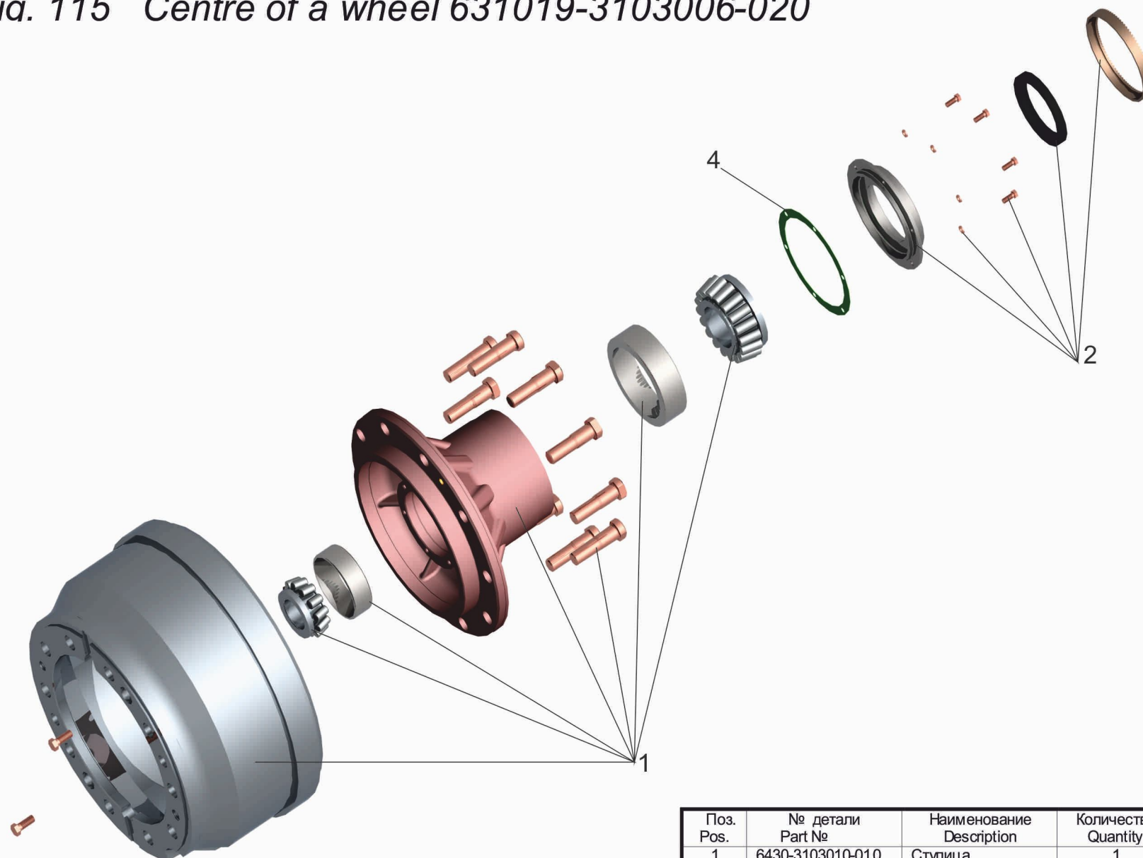
Рис. 115 Ступица 631019-3103006-020
