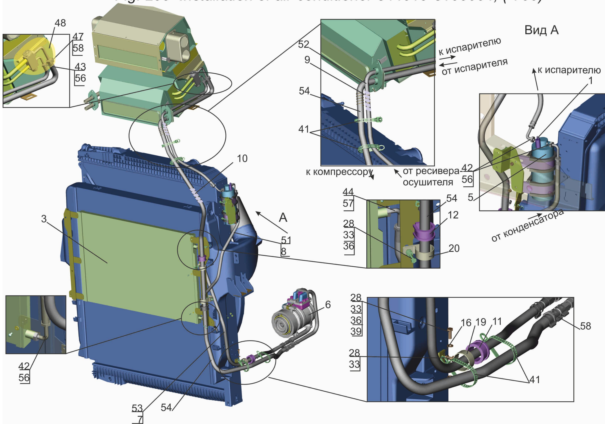
Рис. 299 Установка кондиционера 544019-8100004, (-700) Fig. 299 Installation of air-conditioner 544019-8100004, (-700)
