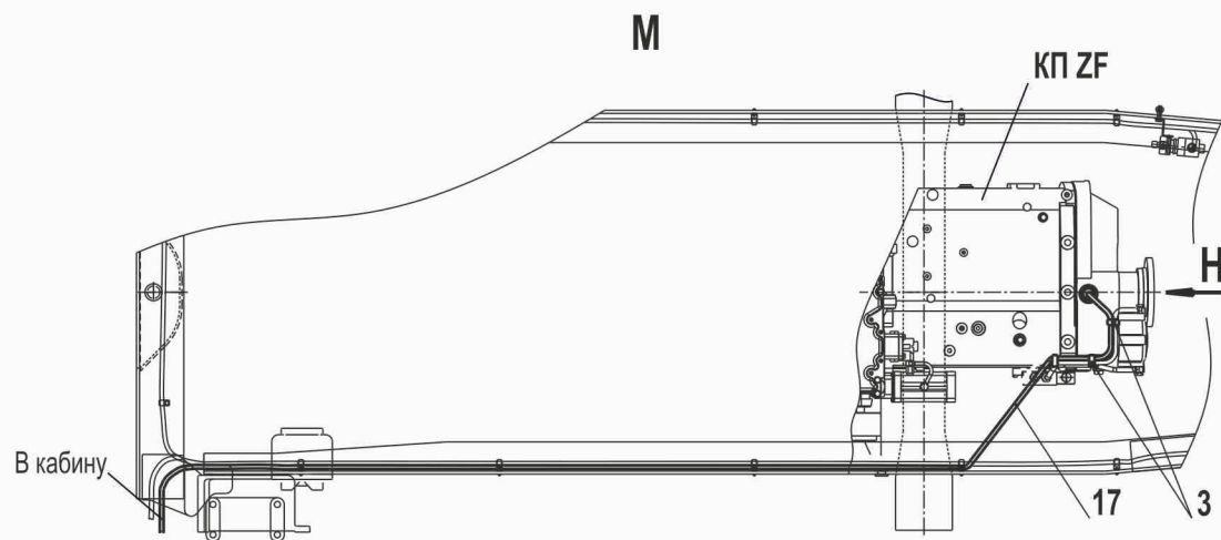
Рис. 189 Установка и пломбировка тахографа 5440-3800005 (лист 2 ) Fig. 189 Installation and identification seal of tachograph 5440-3800005 (page 2)
