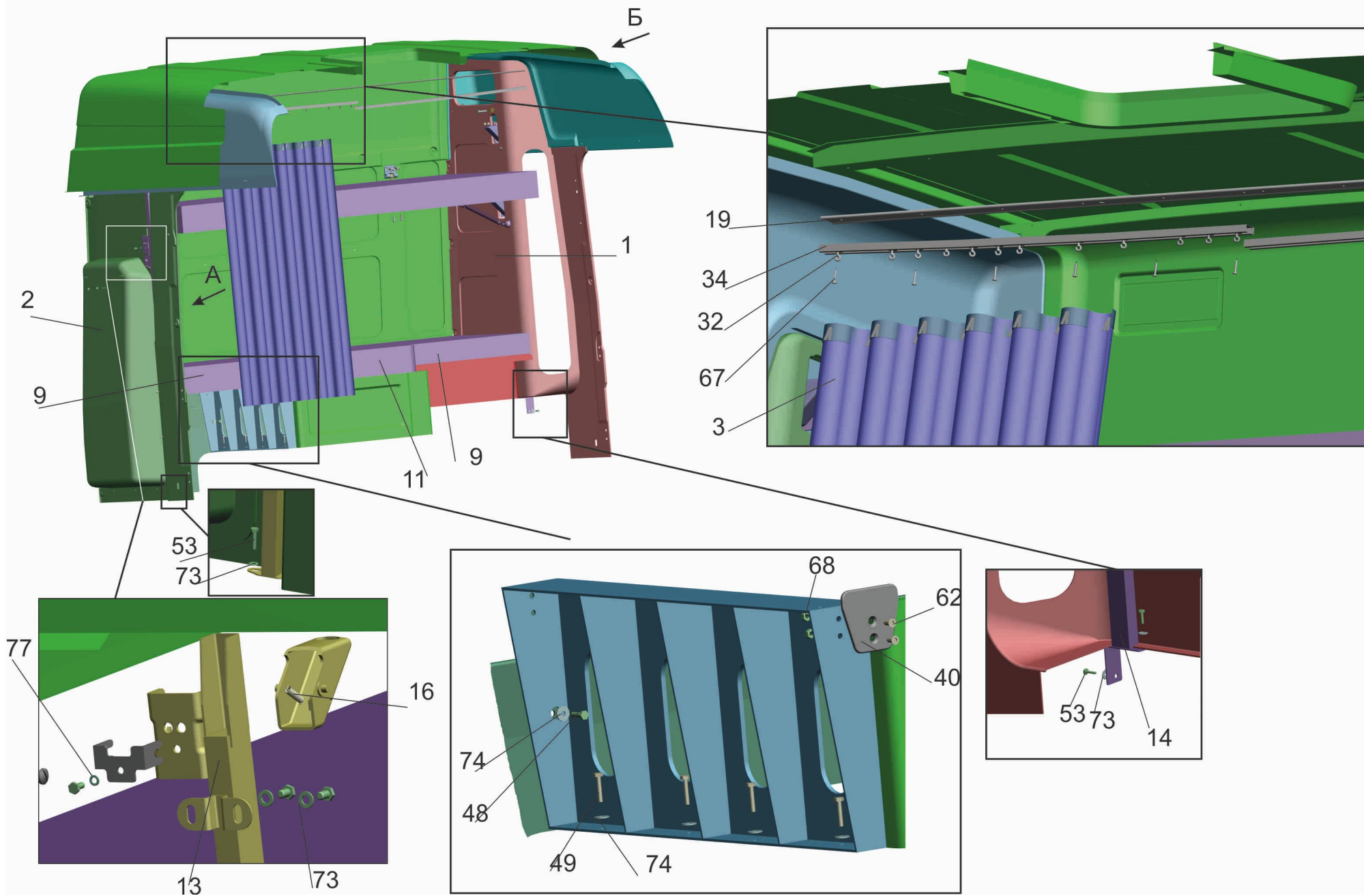
Рис. 266 Установка спальных мест 6430-8200010-020(лист 1) Fig. 266 Mounting of sleeping berths 6430-8200010-020 (page 1)
