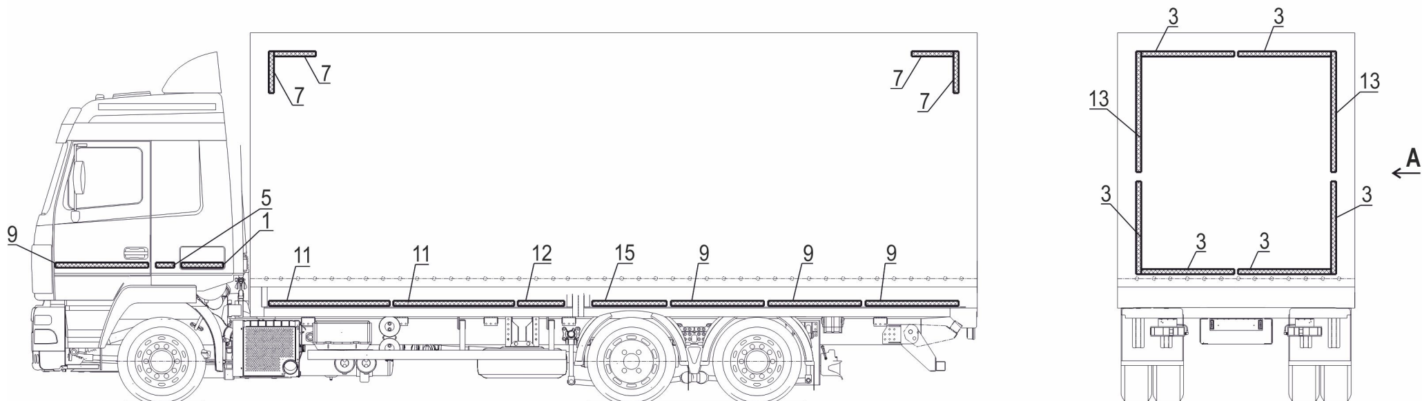
Рис. 192 Установка светоотражающей маркировки 631019-8200002 Fig. 192 Installation of switches 631019-8200002
