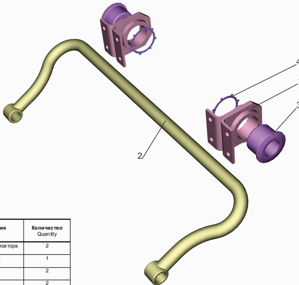
Рис. 104 Вал стабилизатора с кронштейнами 631019-2916006 Fig. 104 Stabilizer shaft with brackets 631019-2916006
