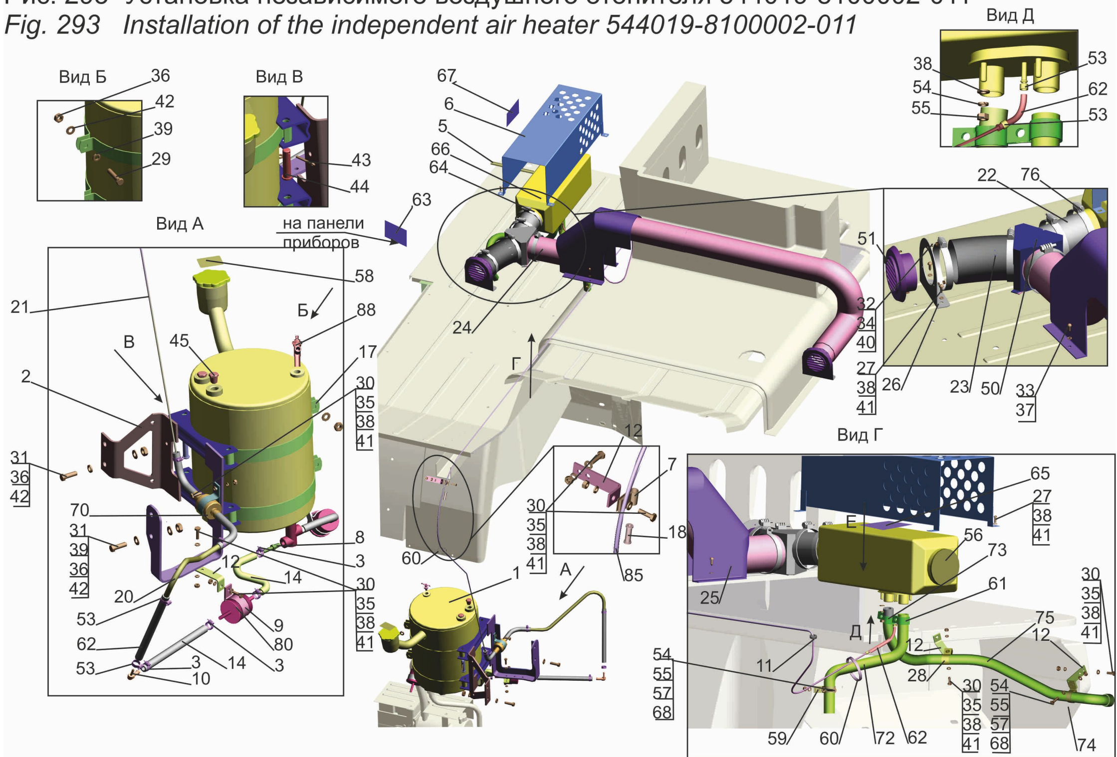
Рис. 293 Установка независимого воздушного отопителя 544019-8100002-011
