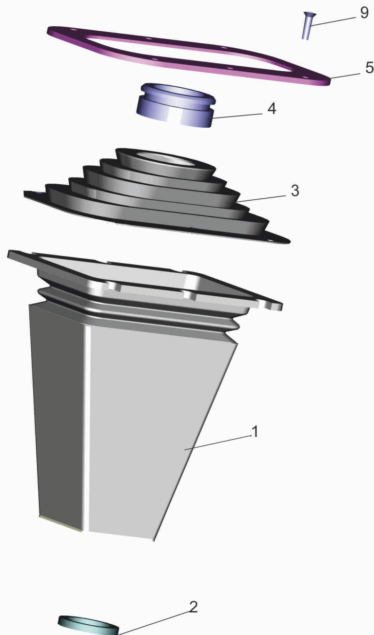
Рис. 161 Уплотнение люка кабины 5440-3444256-010 Fig. 161 Sealing hatch of cabin 5440-3444256-010
