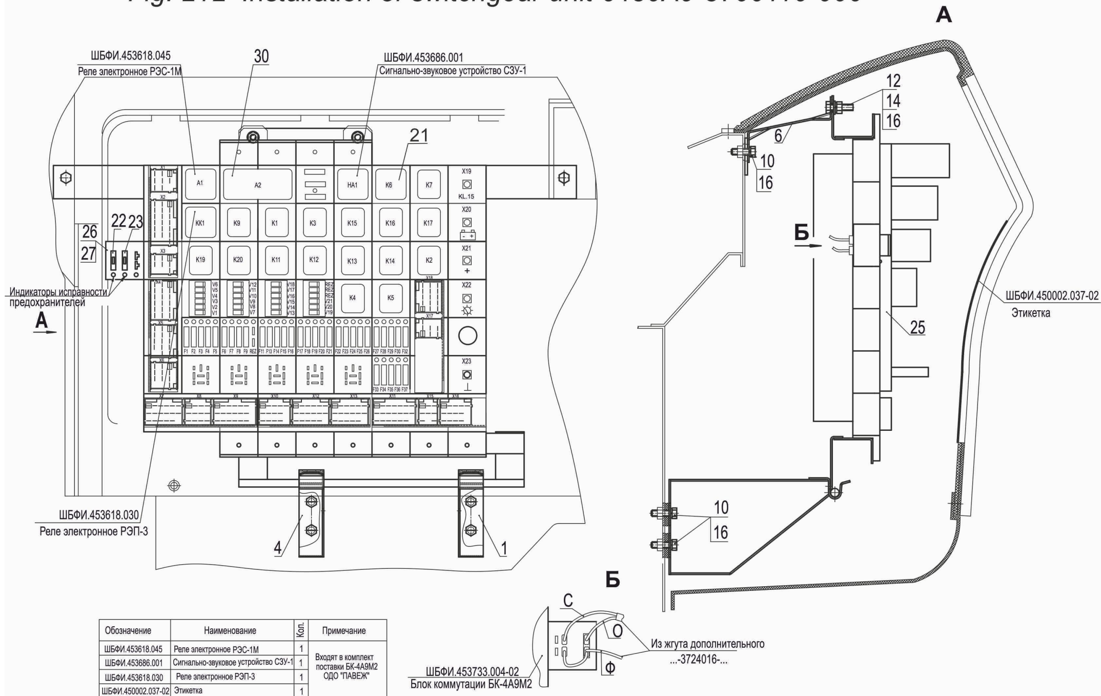
Рис. 212 Установка БКА-N4 6430A9-3700110-000 Fig. 212 Installation of switchgear unit 6430A9-3700110-000
