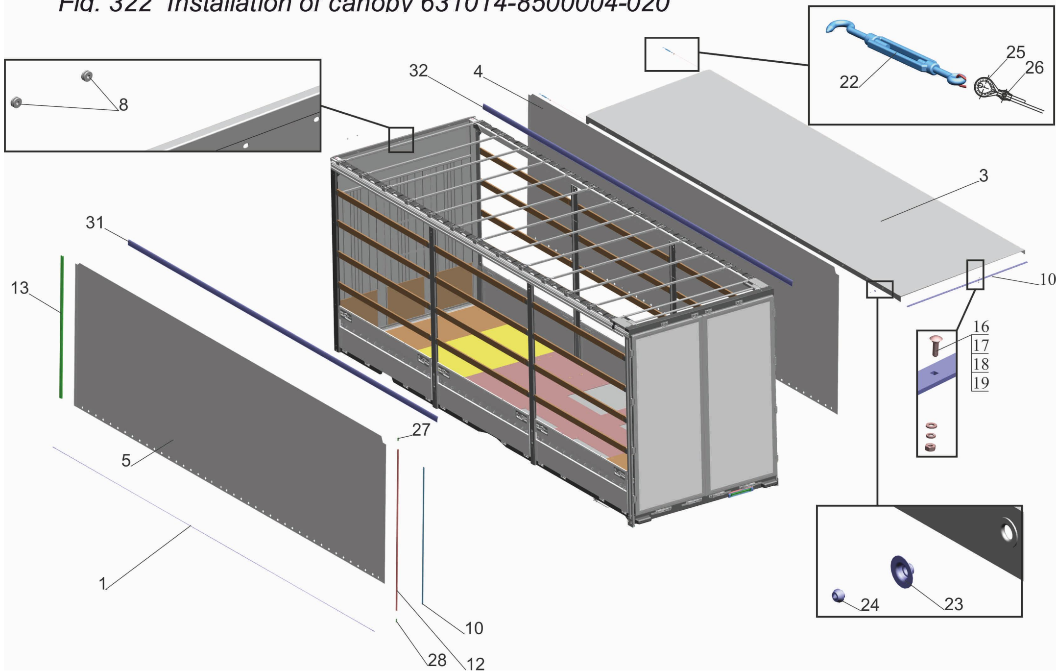
Рис. 322 Установка тента 631014-8500004-020 Fig. 322 Installation of canopy 631014-8500004-020
