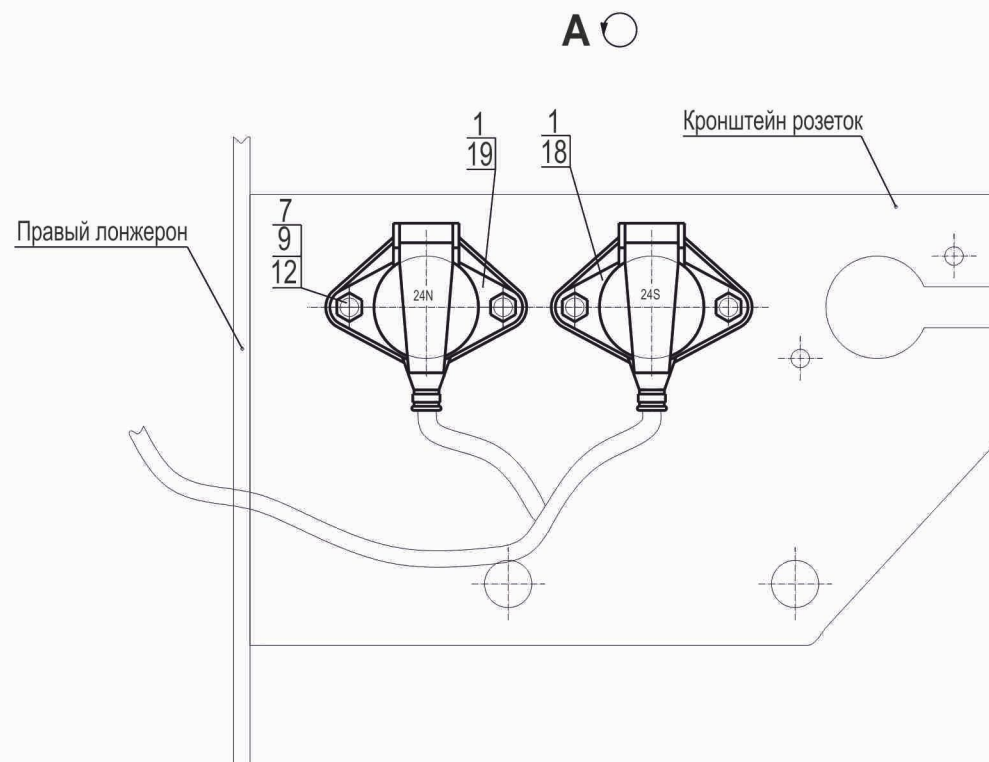
Рис. 197 Установка штепсельных розеток 631019-3700015, (-700) Fig. 197 Installation of outlet sockets 631019-3700015, (-700)
