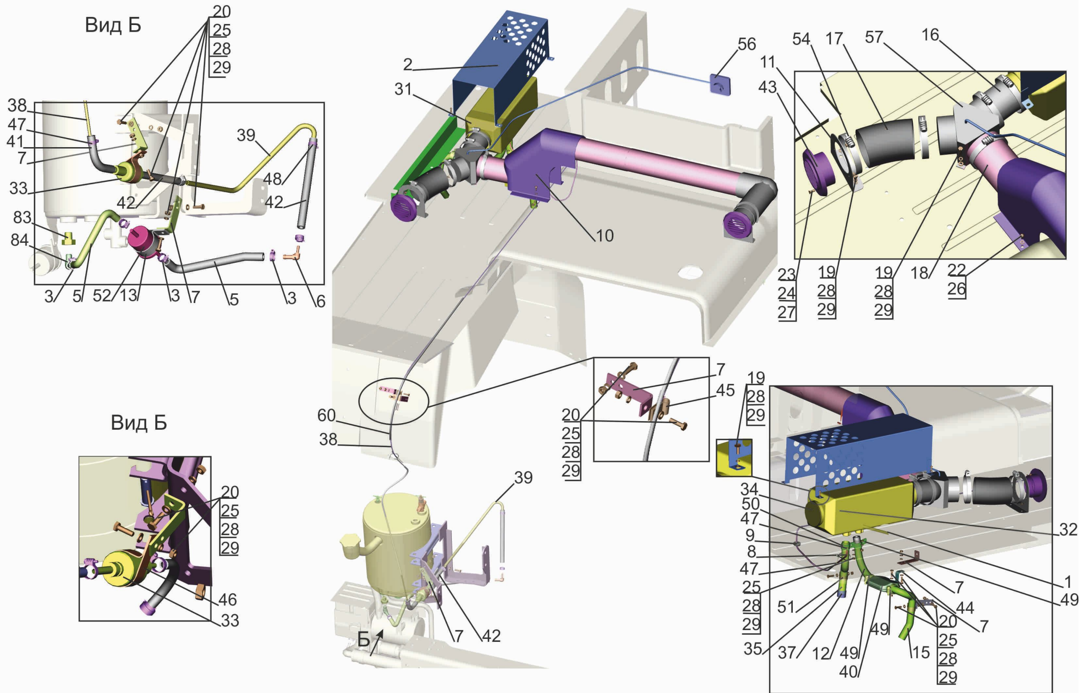
Рис. 294 Установка независимого воздушного отопителя 6430-8100002 Fig. 294 Installation of the independent air heater 6430-8100002
