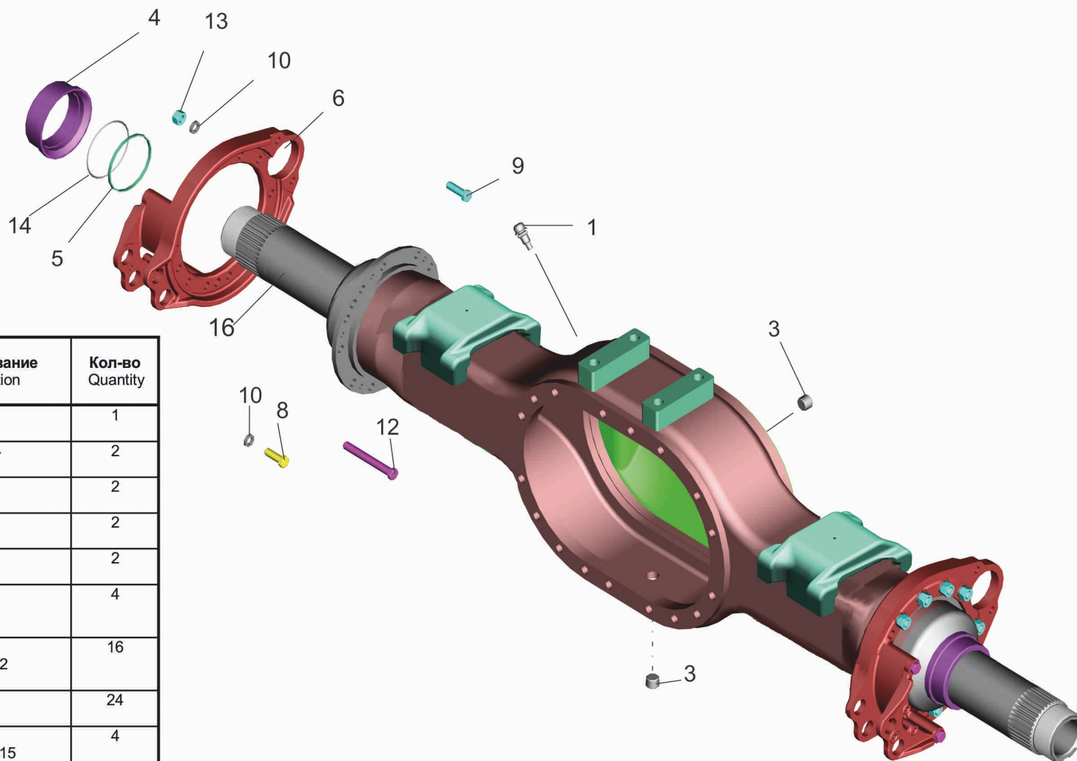
Рис. 74 Мост задний. Картер моста 64301-2401010-030 Fig. 74 Rear axle. Axle housing 64301-2401010-030
