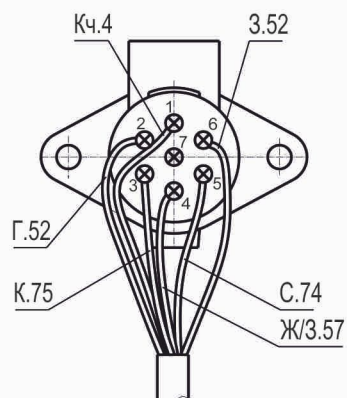
Б Подсоединение проводов к розетке 24N (Чехол поз.4 не показан)
