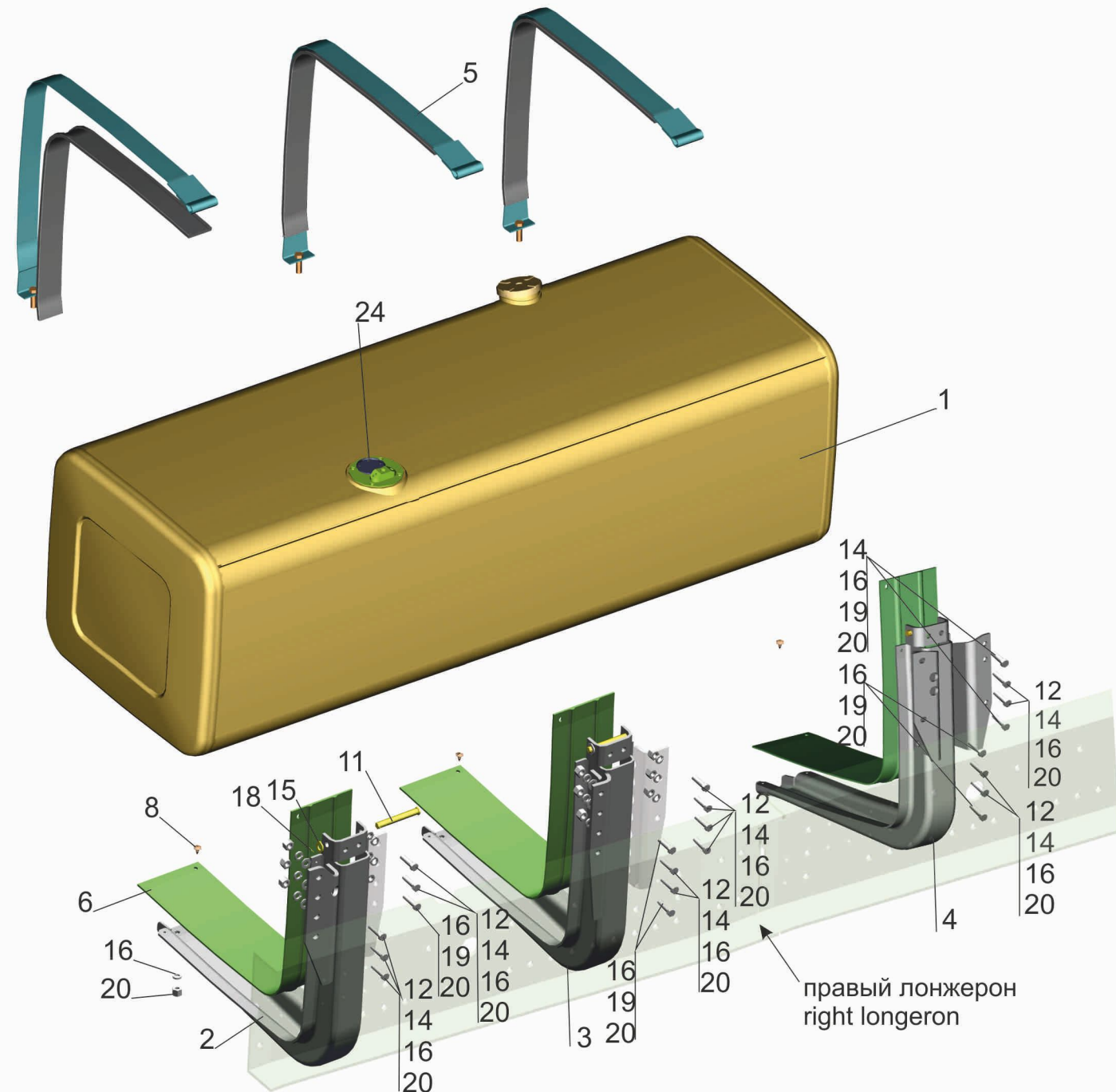
Рис. 13 Крепление топливного бака 631219-1101002-030 (700 литров) Fig. 13 Mounting of fuel tank 631219-1101002-030 (700 liters)
