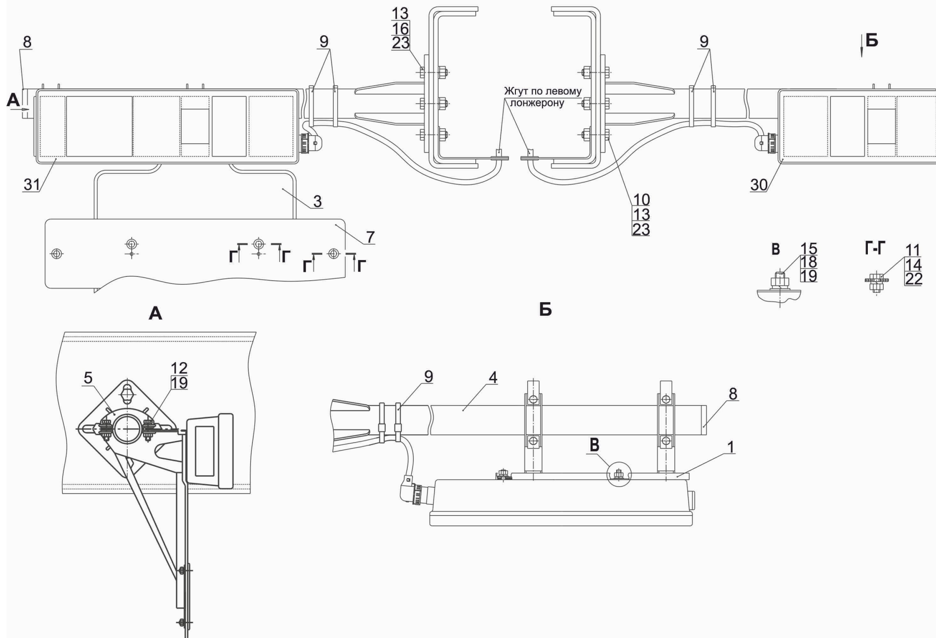
Рис. 183 Установка задних фонарей 6501А5-3700009 Fig. 183 Installation of tail lights 6501А5-3700009
