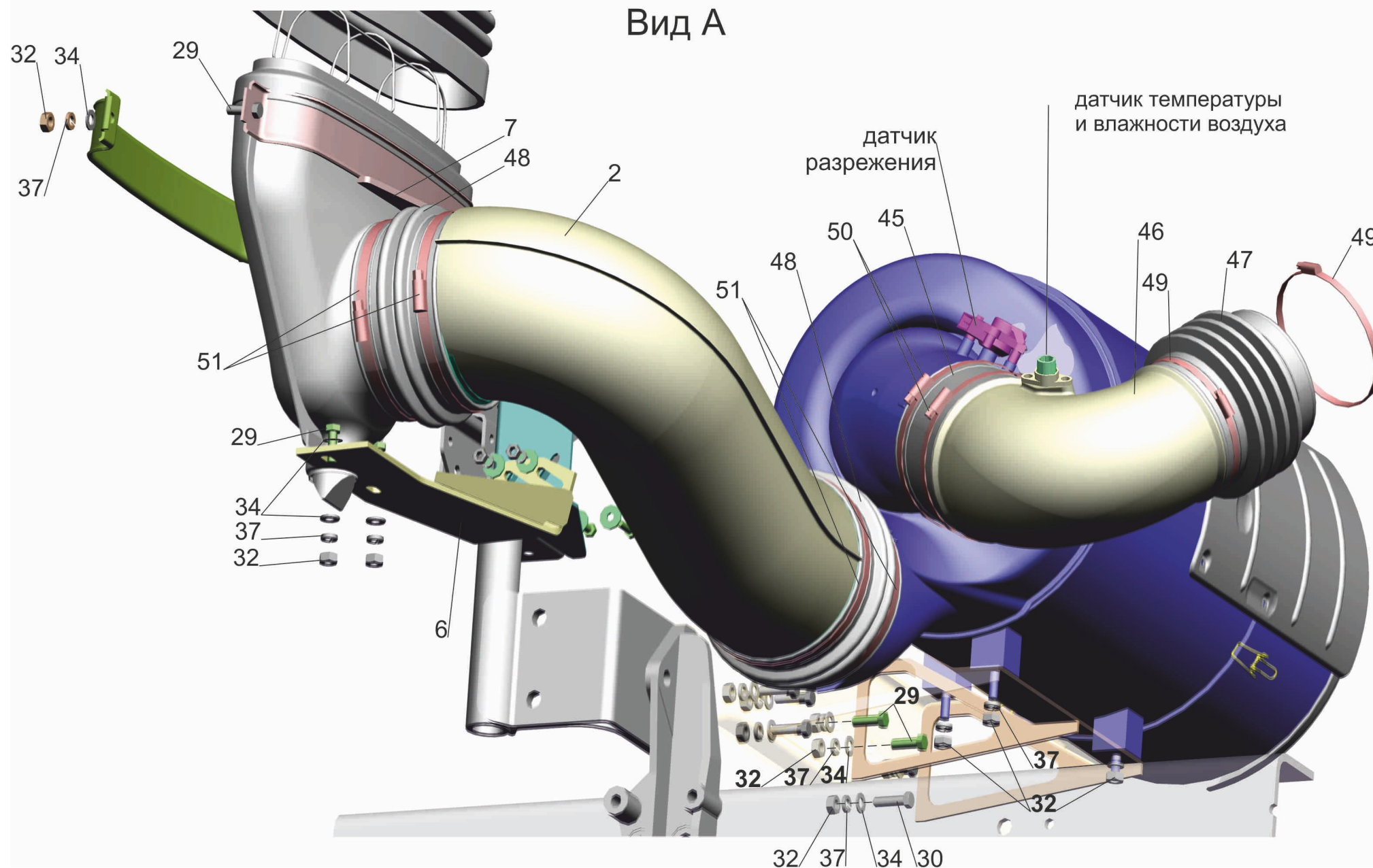
Рис. 22 Крепление воздушного фильтра 544019-1109002-001 (лист 2) Fig. 22 Air filter mounting 544019-1109002-001 (page 2)
