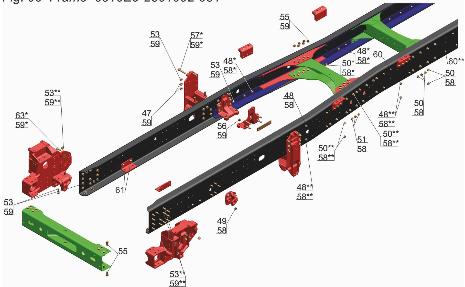
Fig. 90 Frame 6310E9-2801002-031
