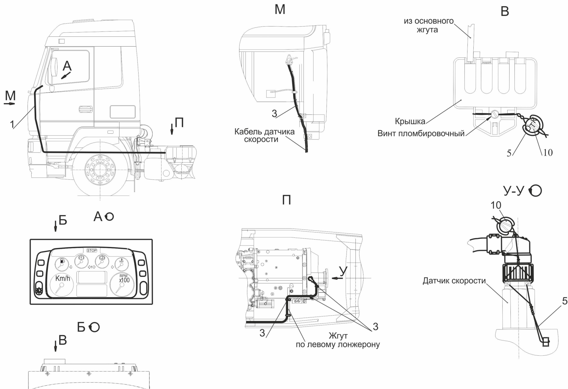
Рис. 188 Установка и пломбировка спидометра 6516V8-3800004-030 Fig. 188 Installation and identification seal of a speedometer 6516V8-3800004-030
