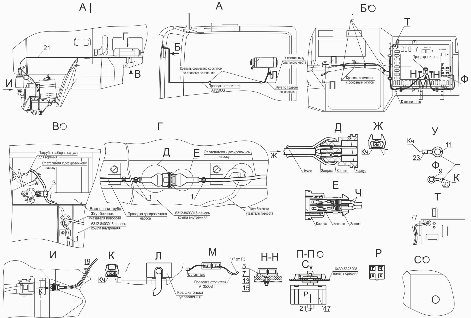
Рис. 298 Установка электрооборудования независимого отопителя 6430-3700088-010 Fig. 298 Setting of an electrical equipment of an independent heater 6430-3700088-010
