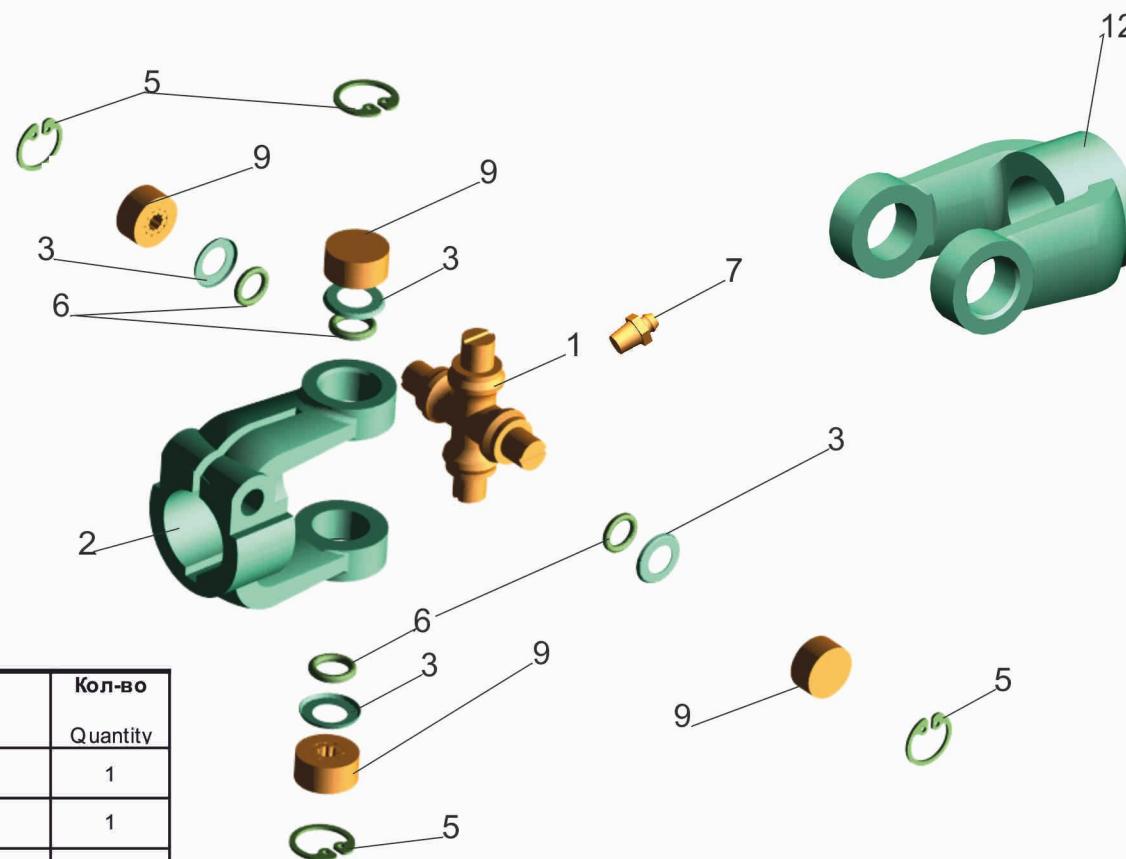
Рис. 156 Шарнир карданный 6430-3444052-001 Fig. 156 Hinge cardan 6430-3444052-001
