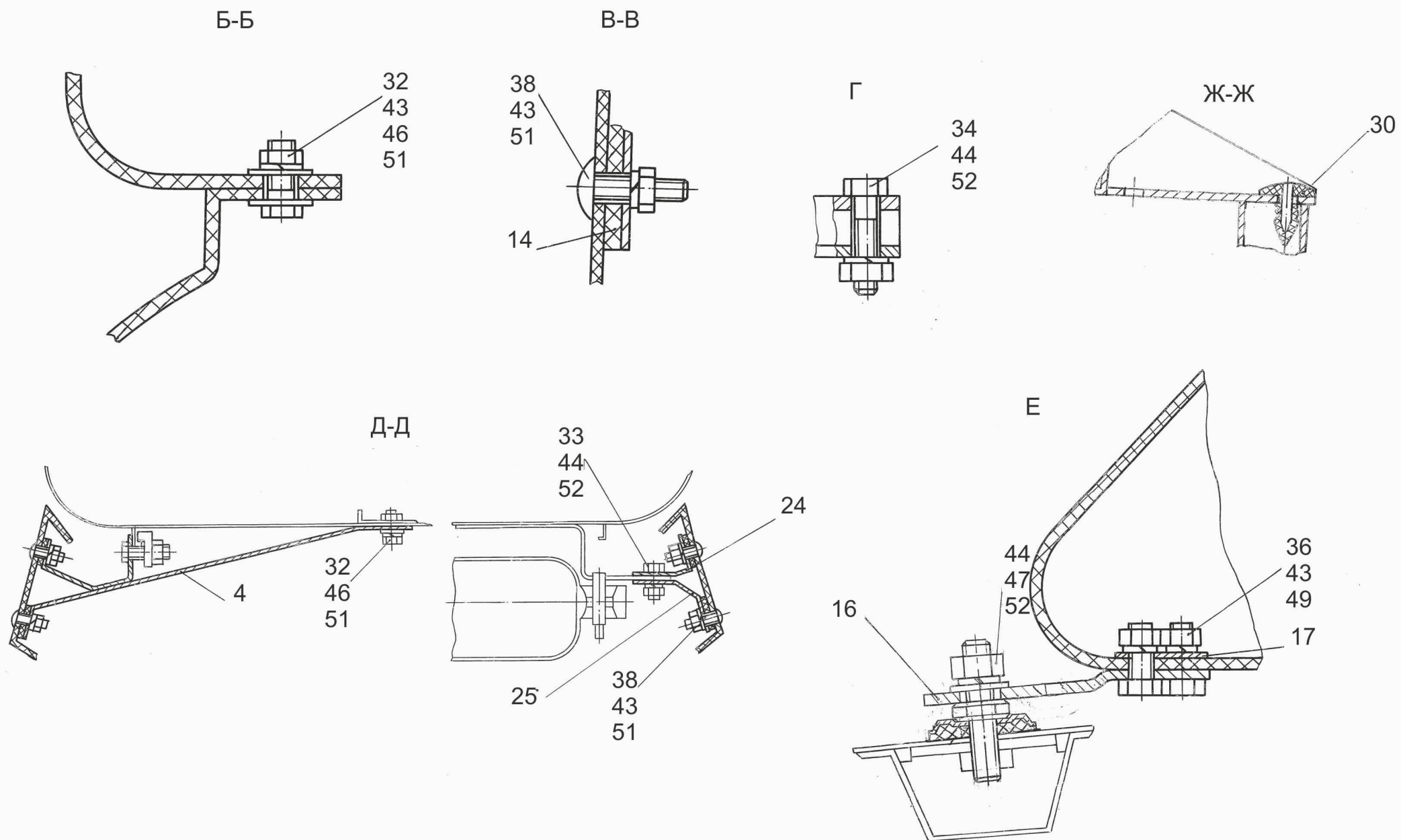
Рис. 280 Установка обтекателей 6312-8000014 Лист 2 Fig. 280 Installation of faing 6312-8000014 Page 2
