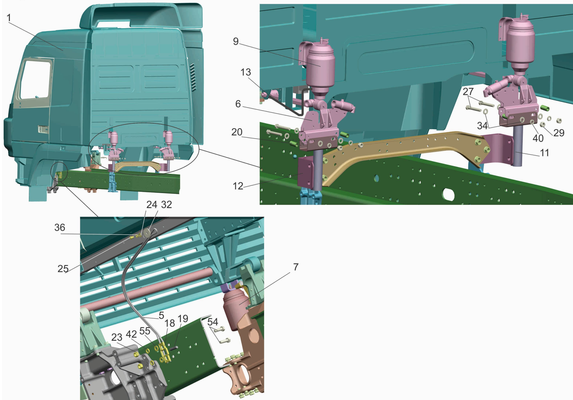
Рис. 226 Установка кабины 643119-5000002-000 Fig. 226 Installation of a cabin 643119-5000002-000
