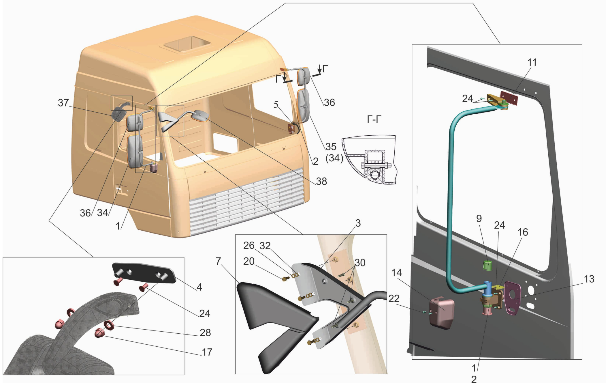
Рис. 264 Установка зеркал 6430-8200005-010,(-012) Fig. 264 Installation mirrors 6430-8200005-010,(-012)
