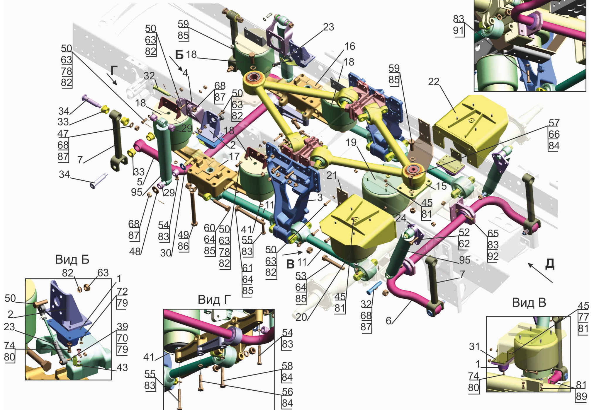
Рис. 99 Установка подвески задней 631019-2900002 Fig. 99 Back suspension mounting 631019-2900002
