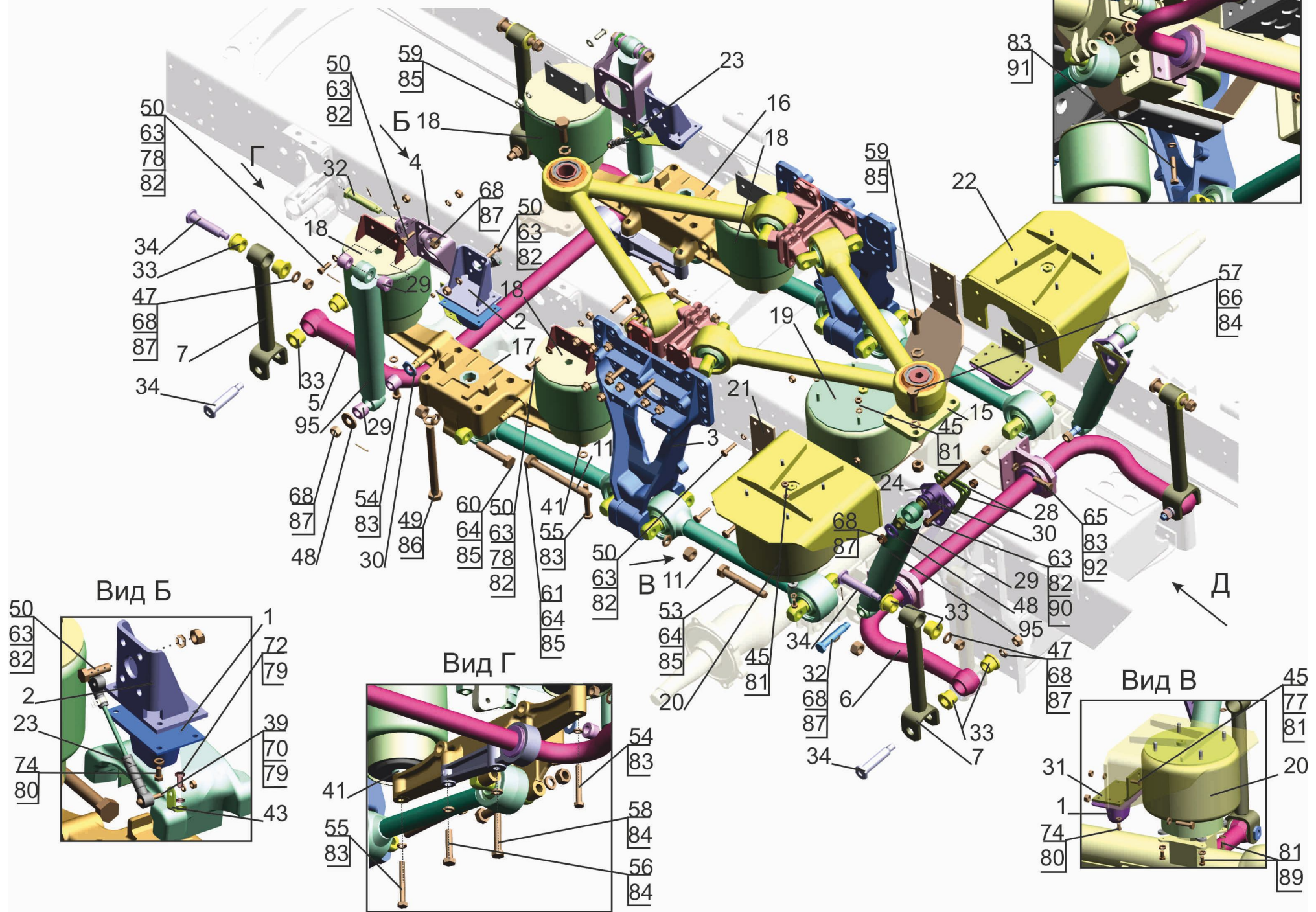
Рис. 100 Установка подвески задней 6310E9-2900002-000 Fig. 100 Back suspension mounting 6310E9-2900002-000
