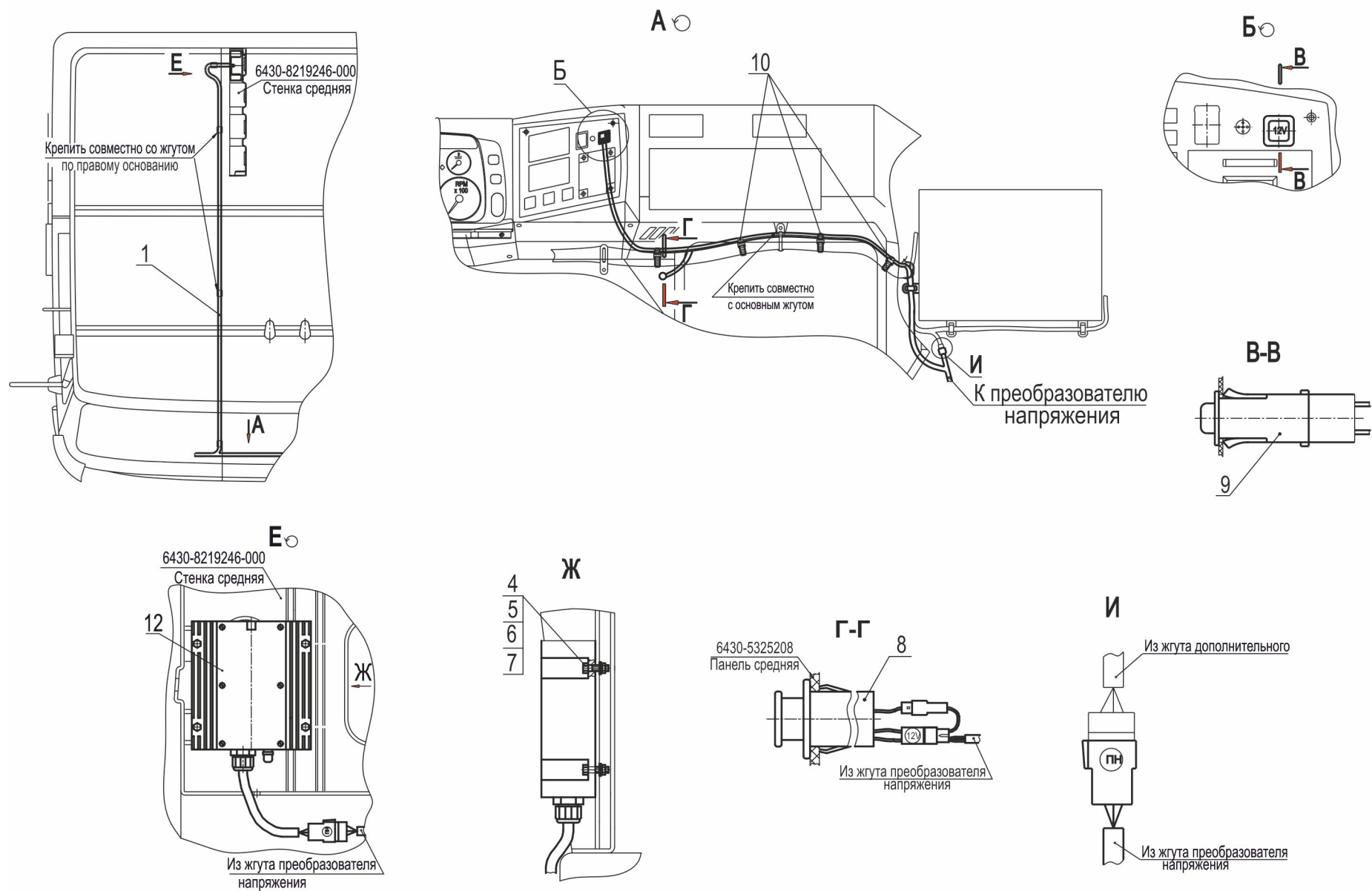
Рис. 185 Установка преобразователя напряжения 6430-3700109 Fig. 185 Installation of a voltage changer 6430-3700109
