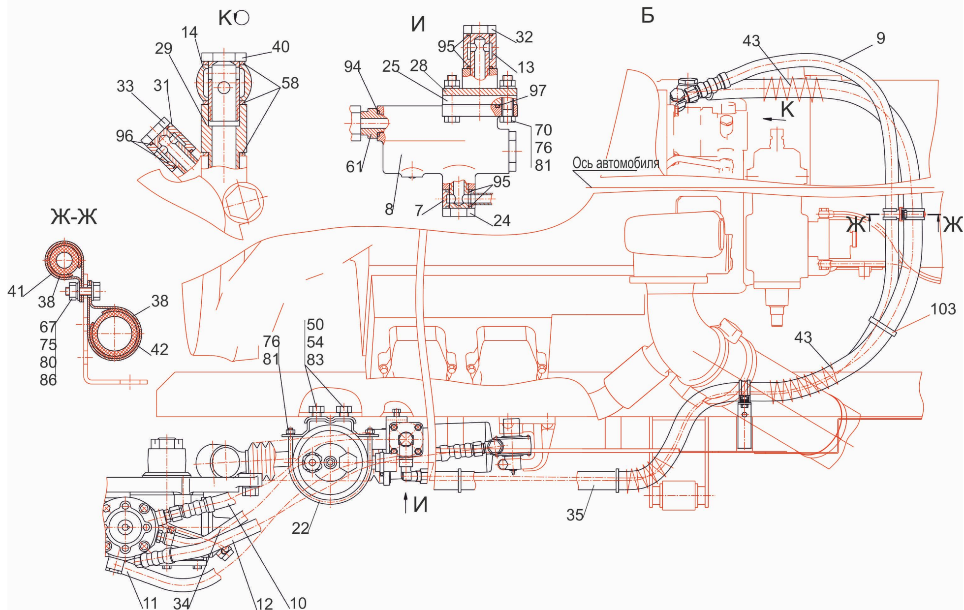
Рис. 138 Установка рулевого управления 631019-3400001 (лист 2) Fig. 138 Steering installation 631019-3400001 (page 2)
