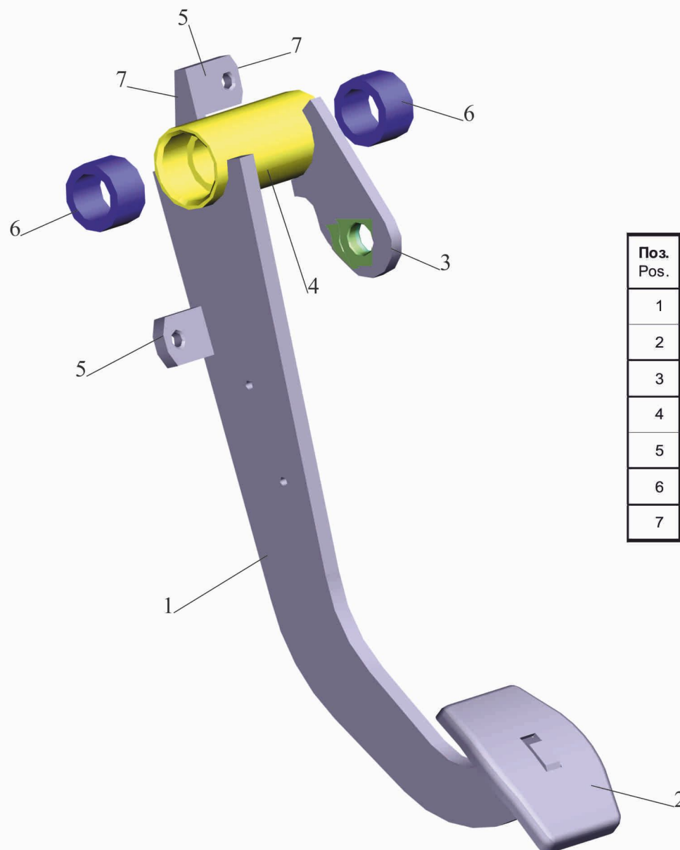
Рис. 43 Педаль 6430-1602112 Fig. 43 Pedal 6430-1602112
