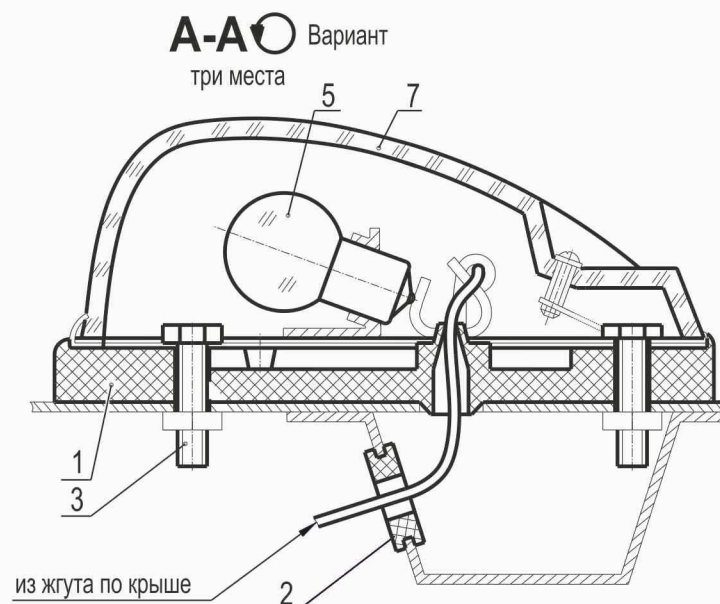
Рис. 208 Установка фонарей знаков автопоезда 6430-3700099, 6430-3700099-700 Fig. 208 Installation of long vehicle signal 6430-3700099, 6430-3700099-700
