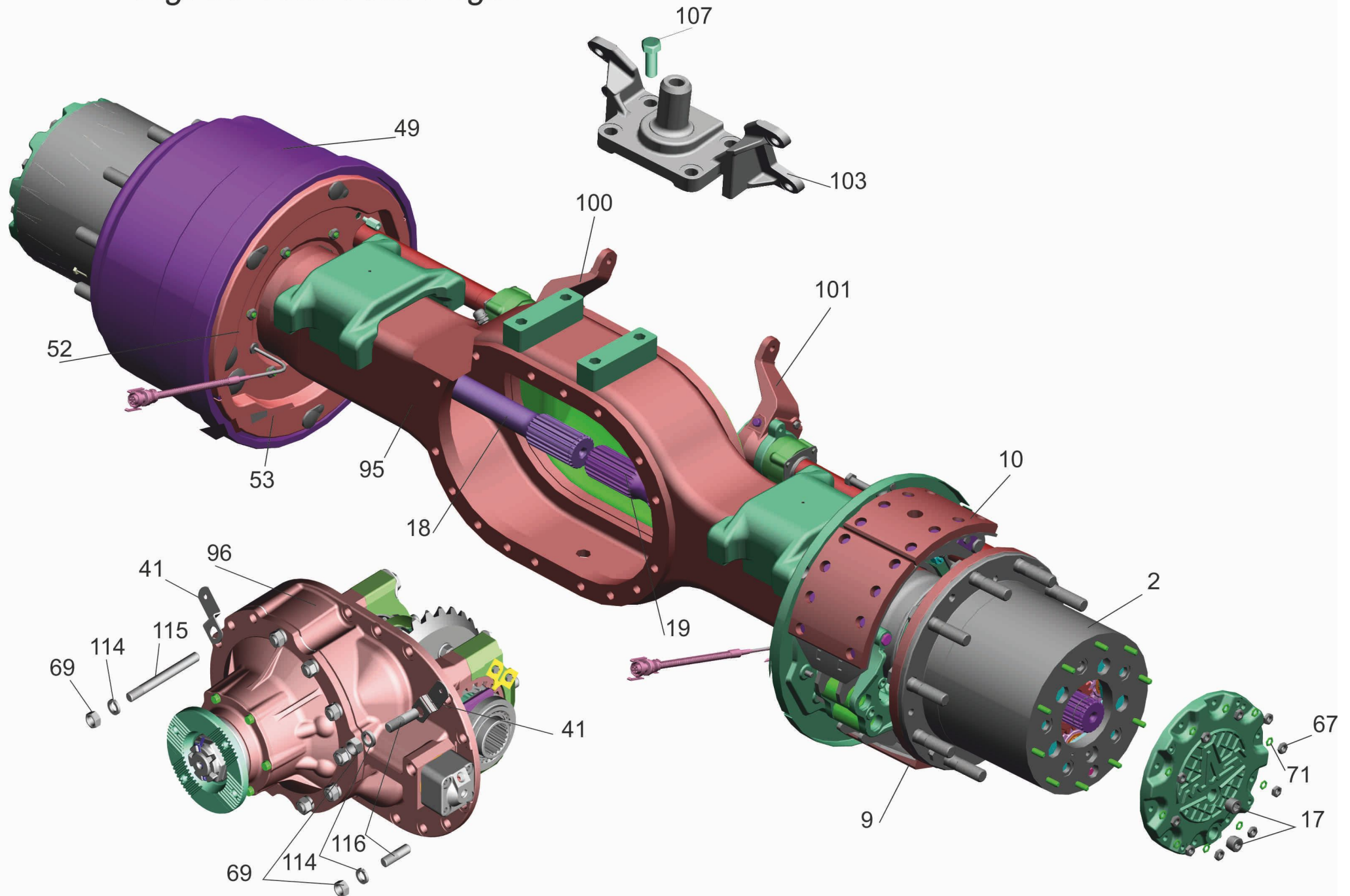
Рис. 63 Мост задний Лист 1
