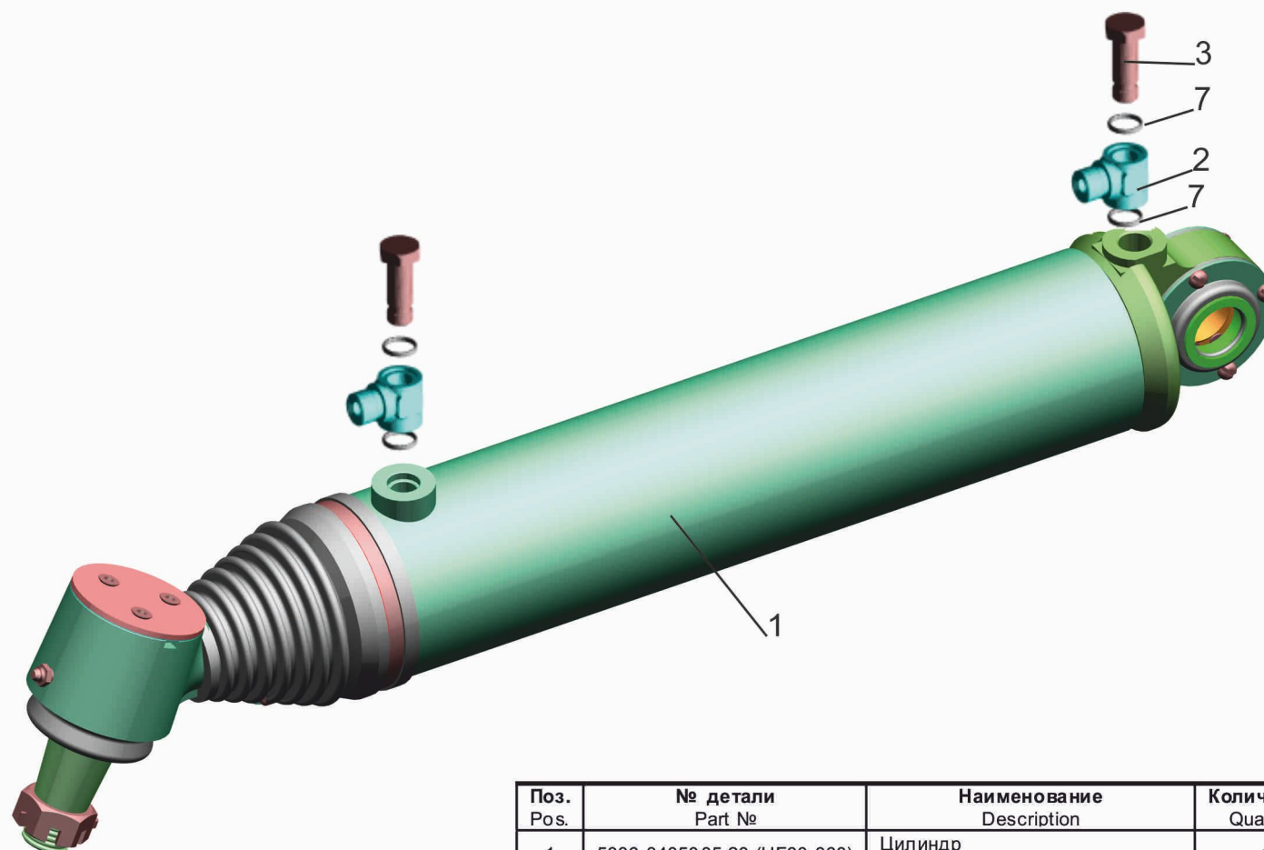
Рис. 158 Цилиндр гидравлический 64221-3405004 Fig. 158 Cylinder hydraulic 64221-3405004
