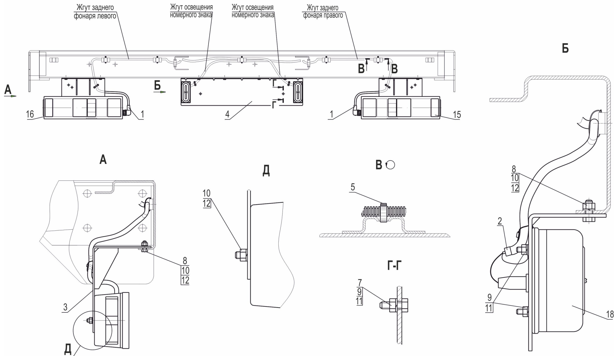
Рис. 182 Установка задних фонарей 631019-3700009 Fig. 182 Installation of tail lights 631019-3700009
