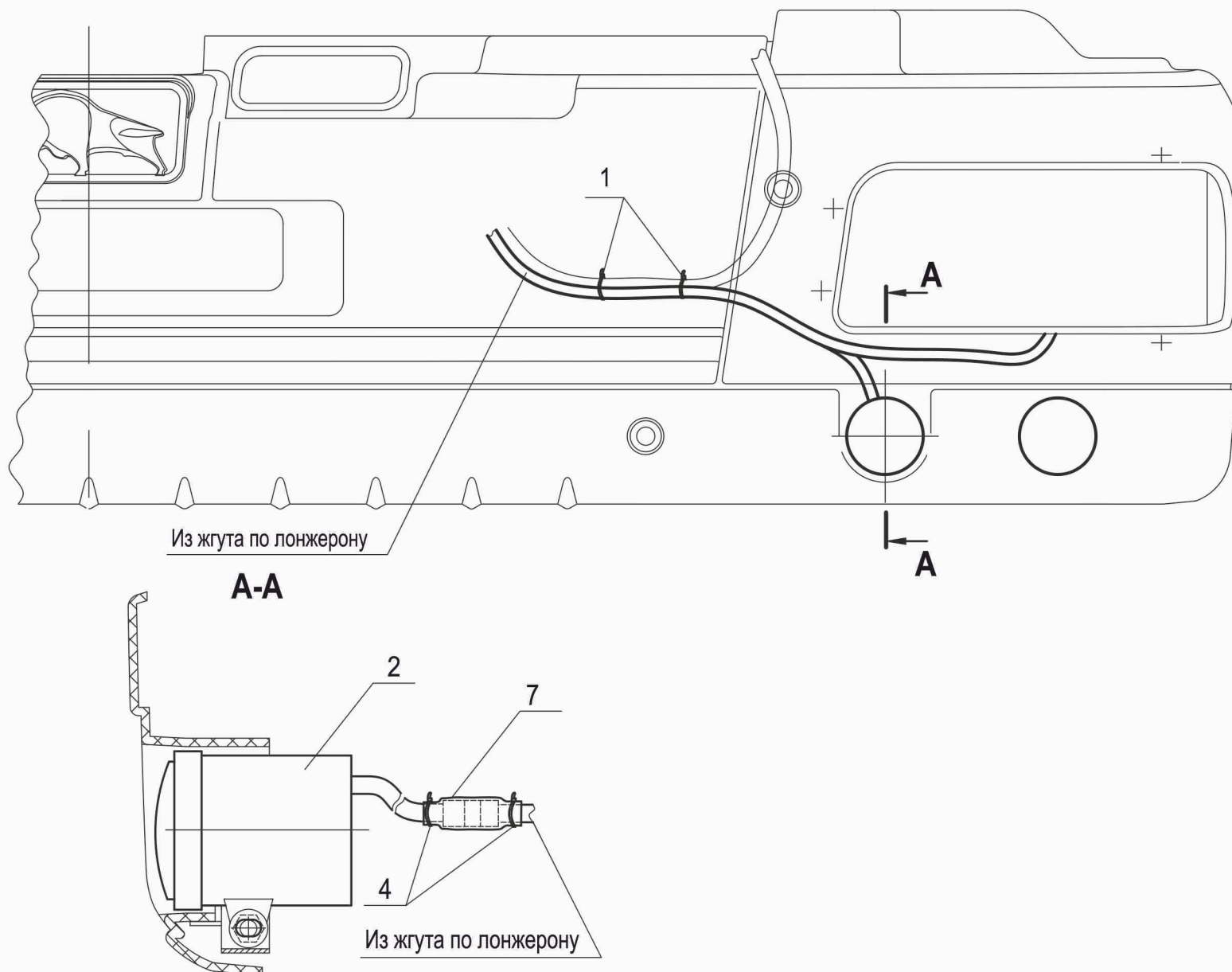
Рис. 181 Установка противотуманных фар 643019-3700007 Fig. 181 Installation of fog lights 643019-3700007
