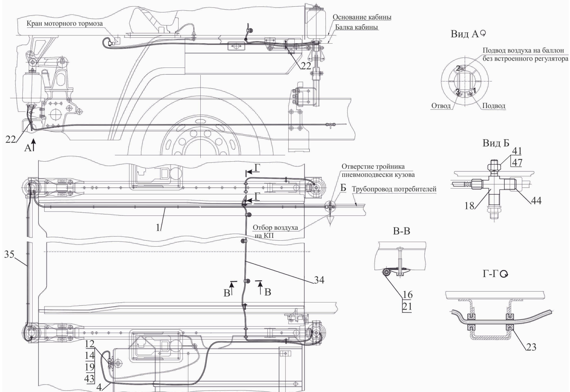
Рис. 232 Пневмопитание подвески кабины 643019-5001930 Fig. 232 Cab suspension air supply 643019-5001930
