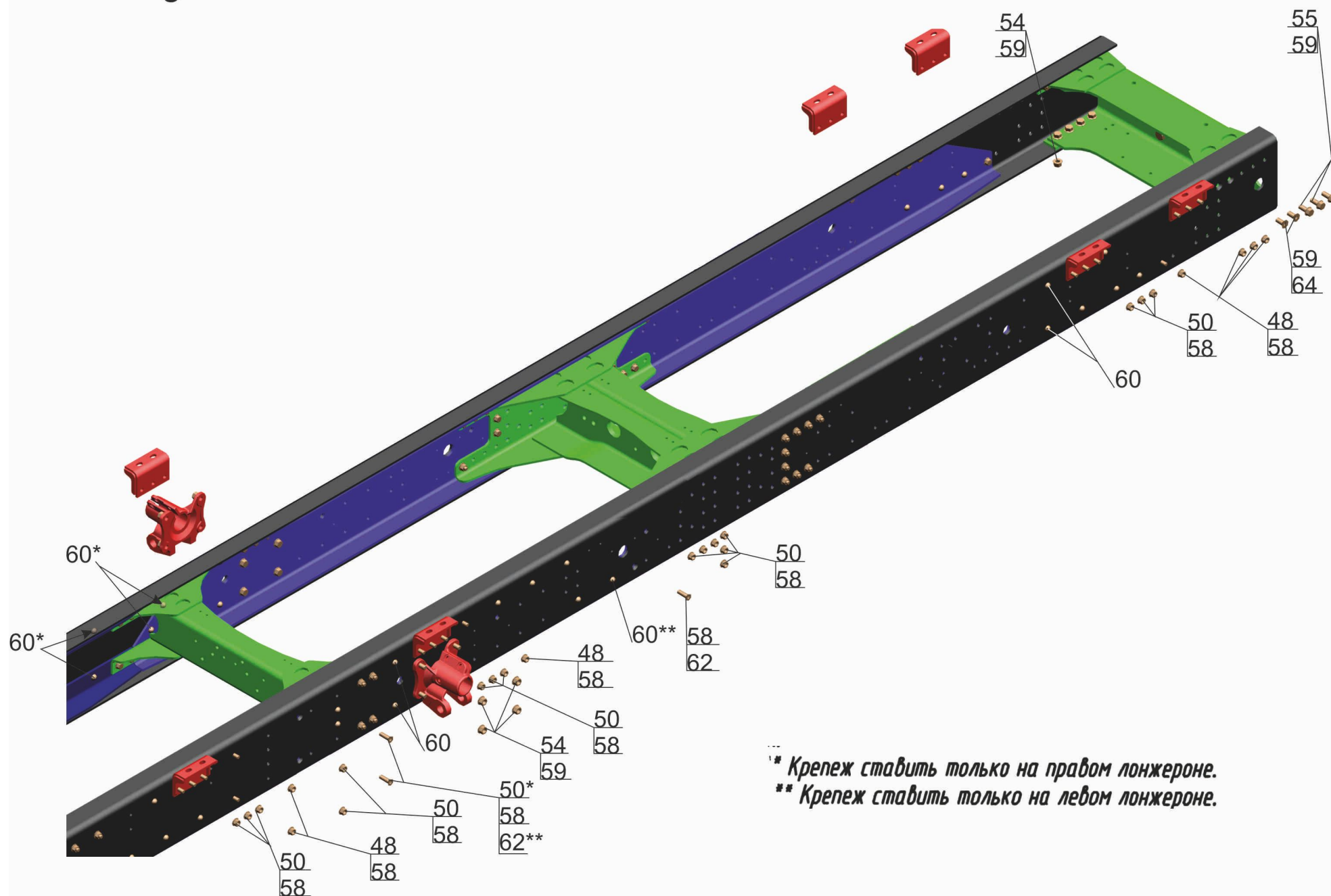
Fig. 89 Frame 631019-2801002-030
