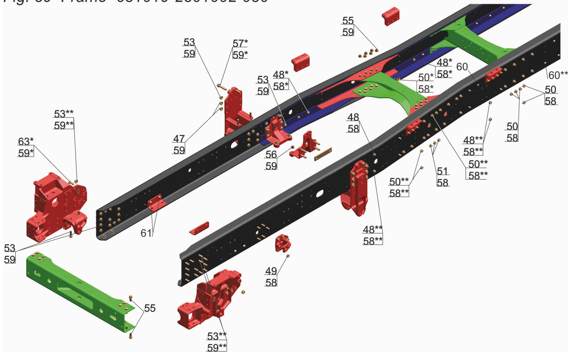
Fig. 89 Frame 631019-2801002-030
