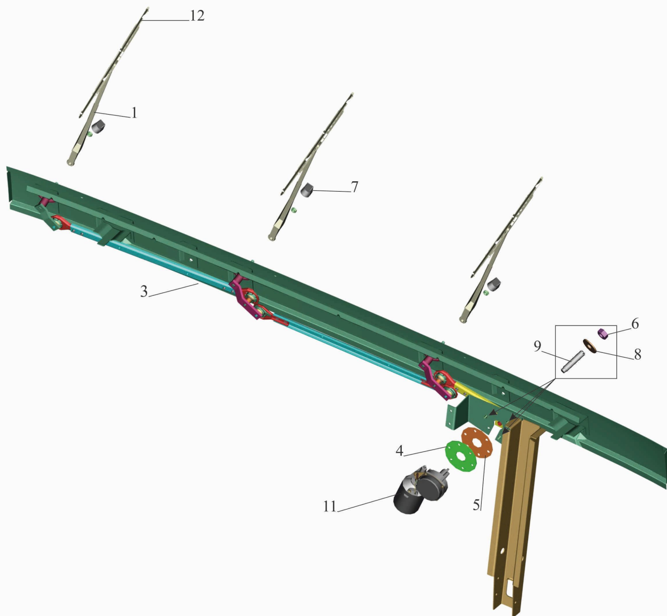
Рис. 238 Установка стеклоочистителя 6430-3700041-001 Fig. 238 Installation of cleaner of glasses 6430-3700041-001
