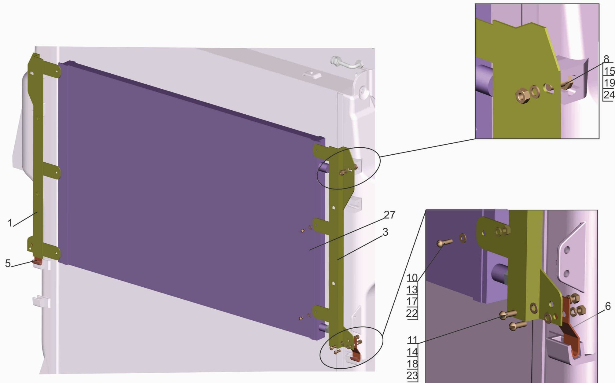
Рис. 300 Установка конденсатора 544019-8100034 Fig. 300 Installation of capacitor 544019-8100034
