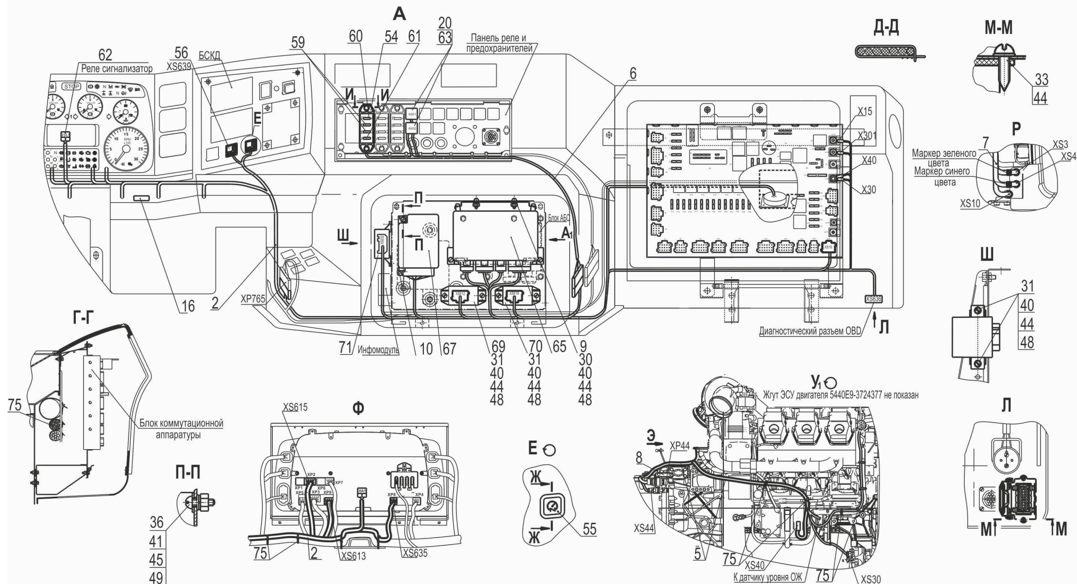
Рис. 220 Установка электрооборудования ЭСУ двигателя 5440E9-3800060-000 (лист 2) Fig. 220 Installation of electronic control system of the engine 5440E9-3800060-000 (page 2)
