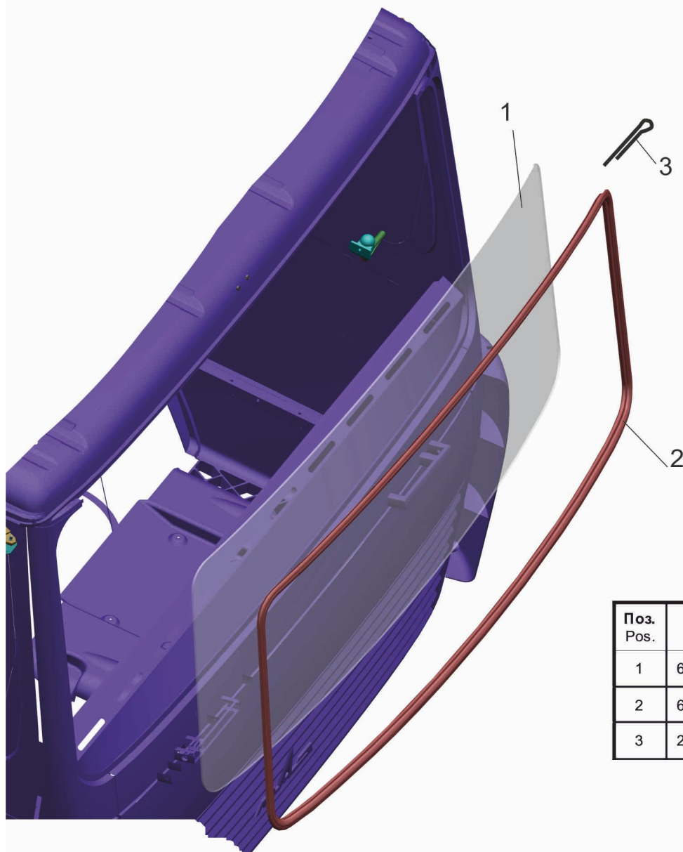
Рис. 243 Установки стекла 6430-5200010 Fig. 243 Installation of a glass 6430-5200010
