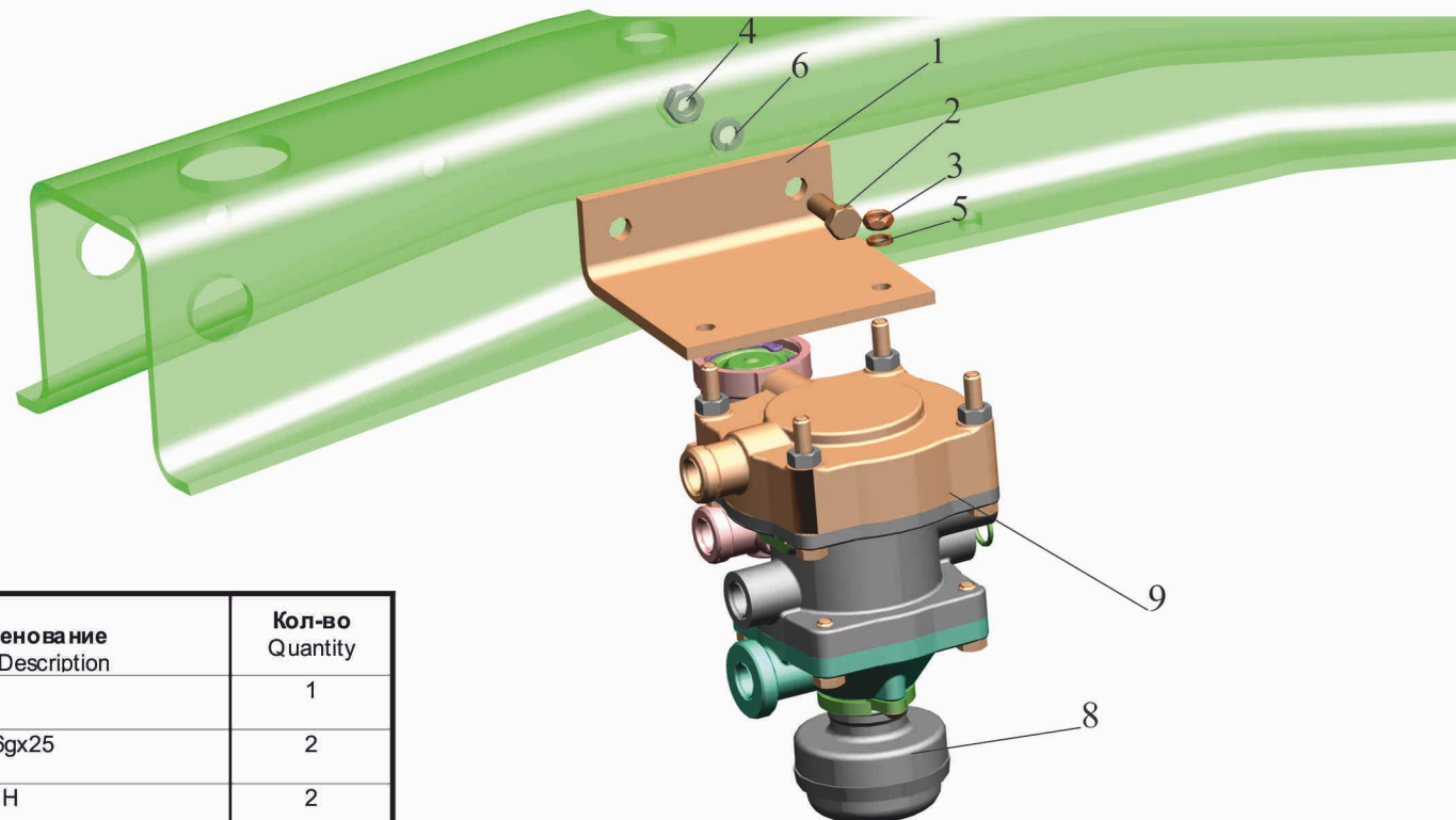
Рис. 175 Установка клапана управления тормозами прицепа 54401-3522005 Fig. 175 Installation of trailer brake control valve 54401-3522005
