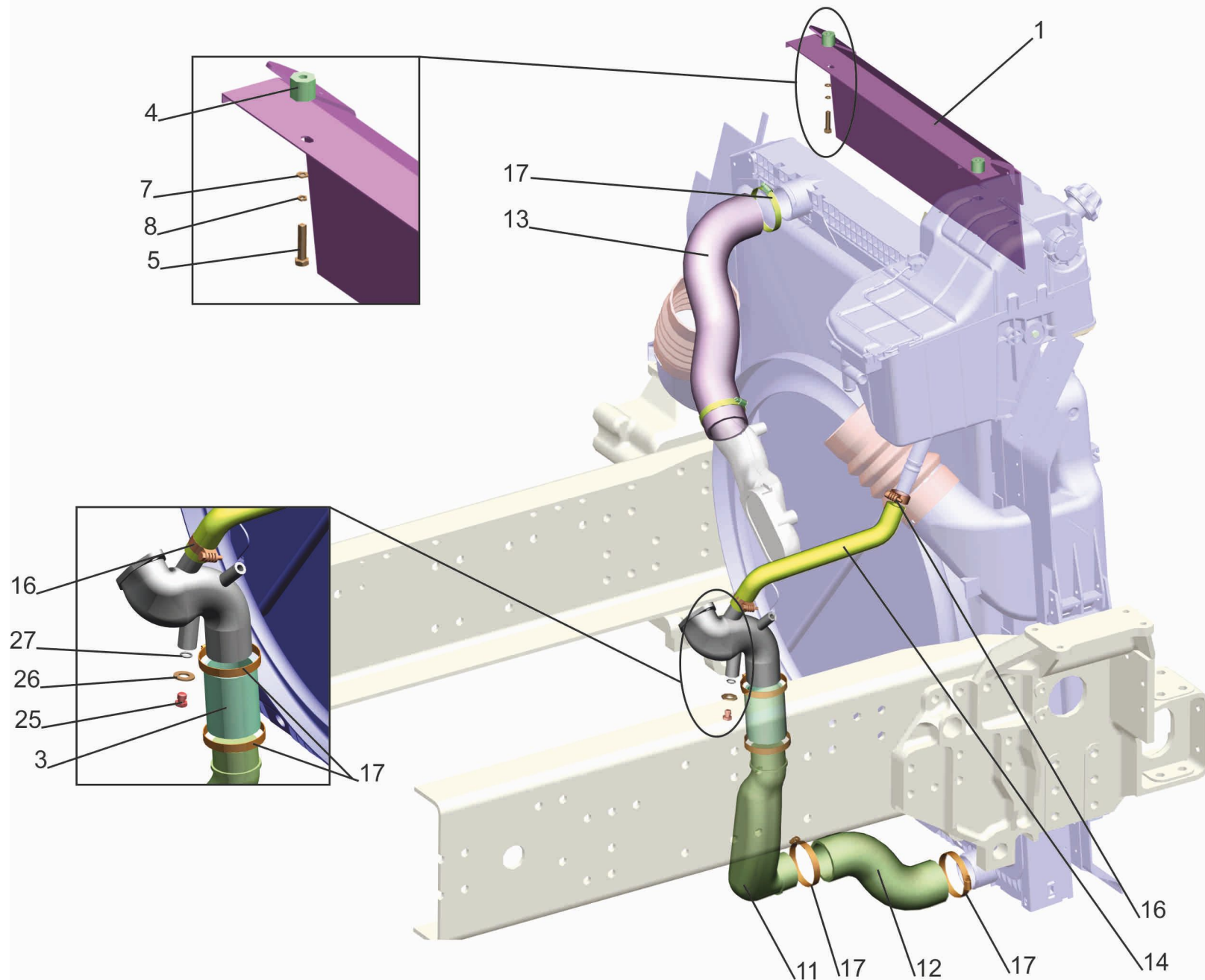
Рис. 27 Установка системы охлаждения 544019-1300005-010 Fig. 27 Installation of cooling system set 544019-1300005-010
