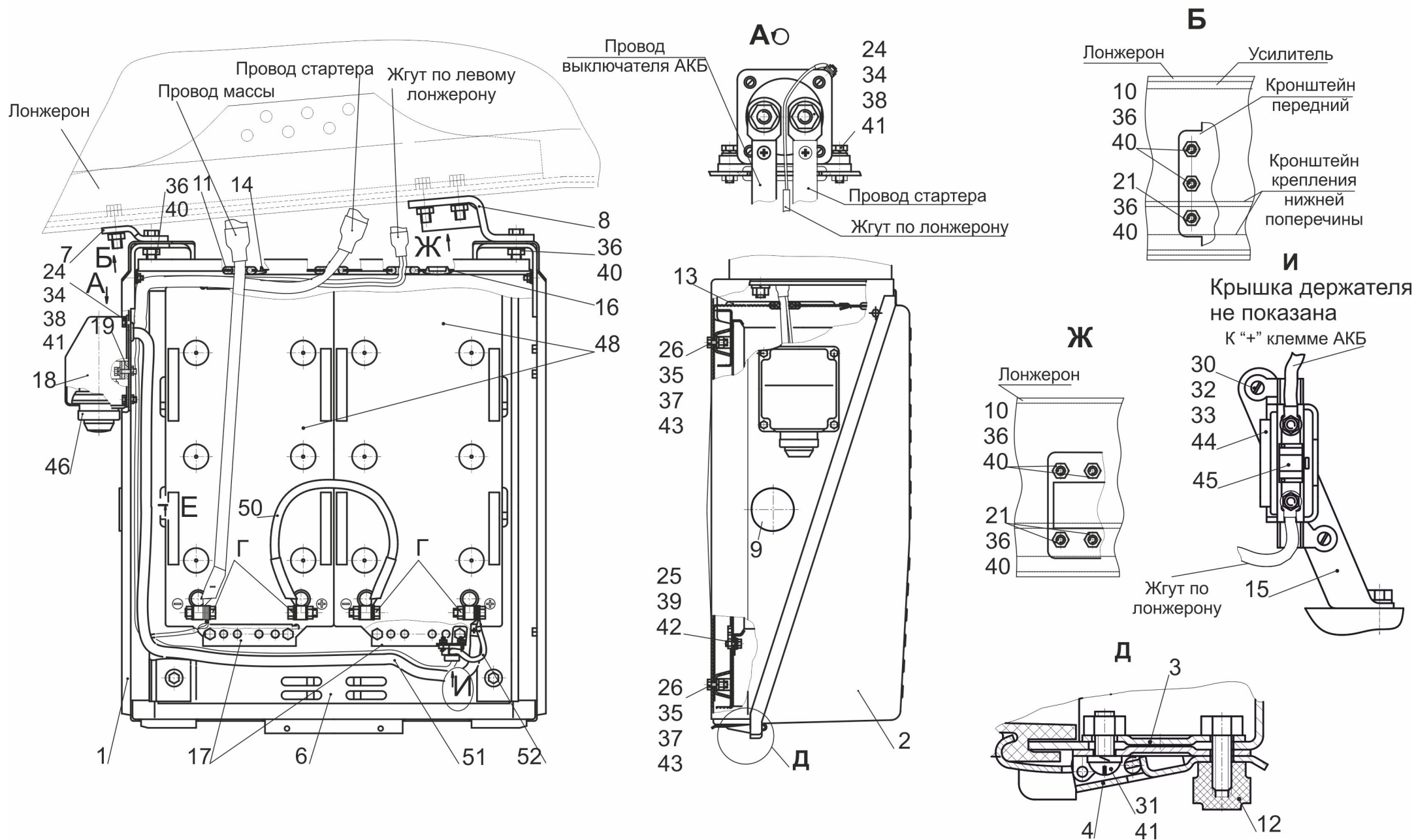
Рис. 194 Установка аккумуляторных батарей 650119-3700008, (-700) Fig. 194 Installation of storage batteries 650119-3700008, (-700)
