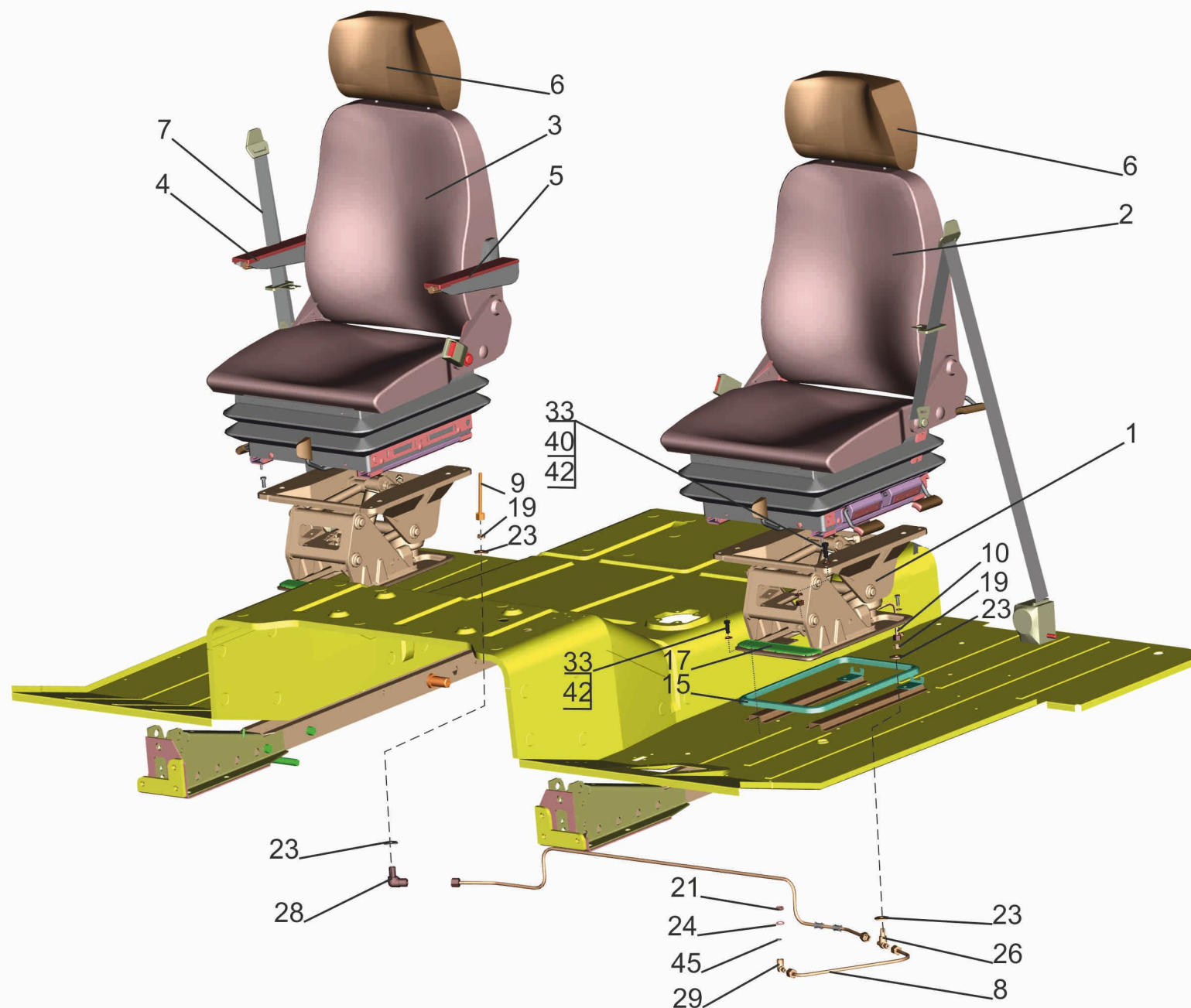
Рис. 250 Установка и пневмопитание сидений 6430-6800006-001 Fig. 250 Installation and pneumatic supply of seat 6430-6800006-001
