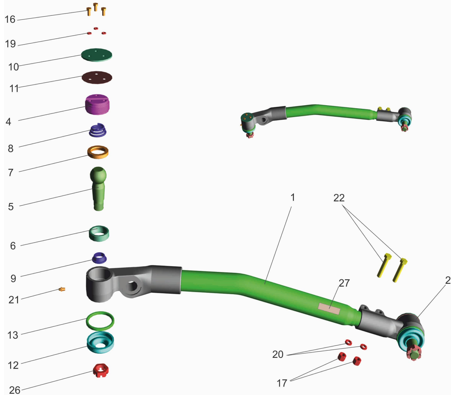
Рис. 130 Тяга продольная 5440-3003010 Fig. 130 Drag Rod 5440-3003010
