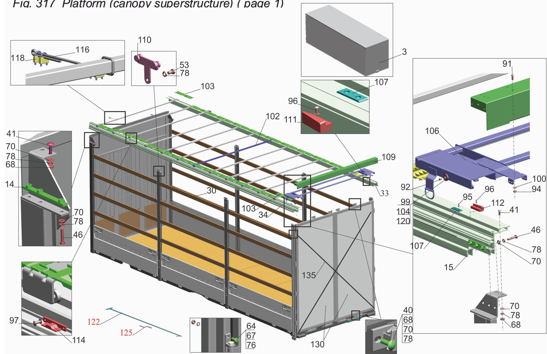
Рис. 317 Платформа 631014-8500008-020 (тентовая надстройка) ( лист 1)
