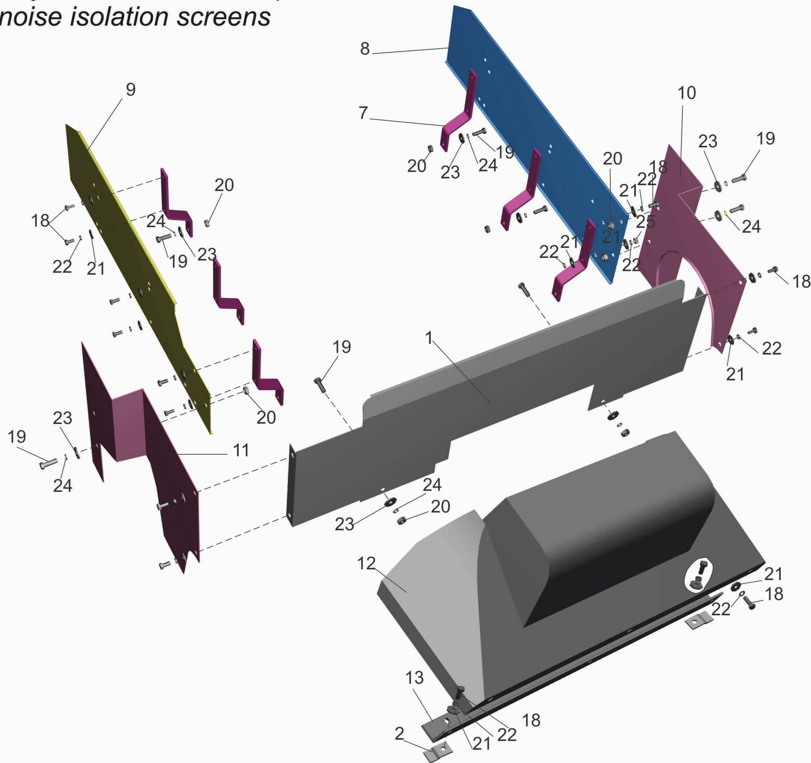
Рис. 10 Установка шумоизоляционных экранов 631019-1061003-006
