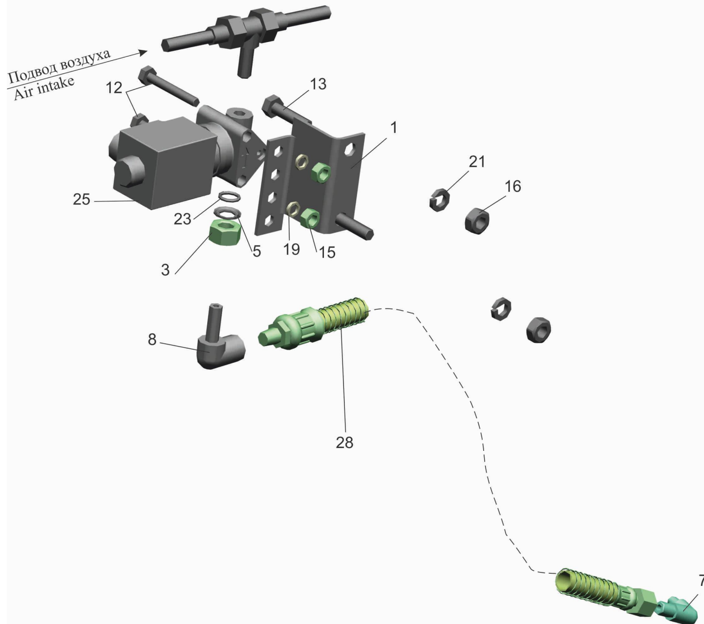
Рис. 82 Установка привода управления блокировки 631019-2400024 Fig. 82 Installation of a drive of management by blocking 631019-2400024
