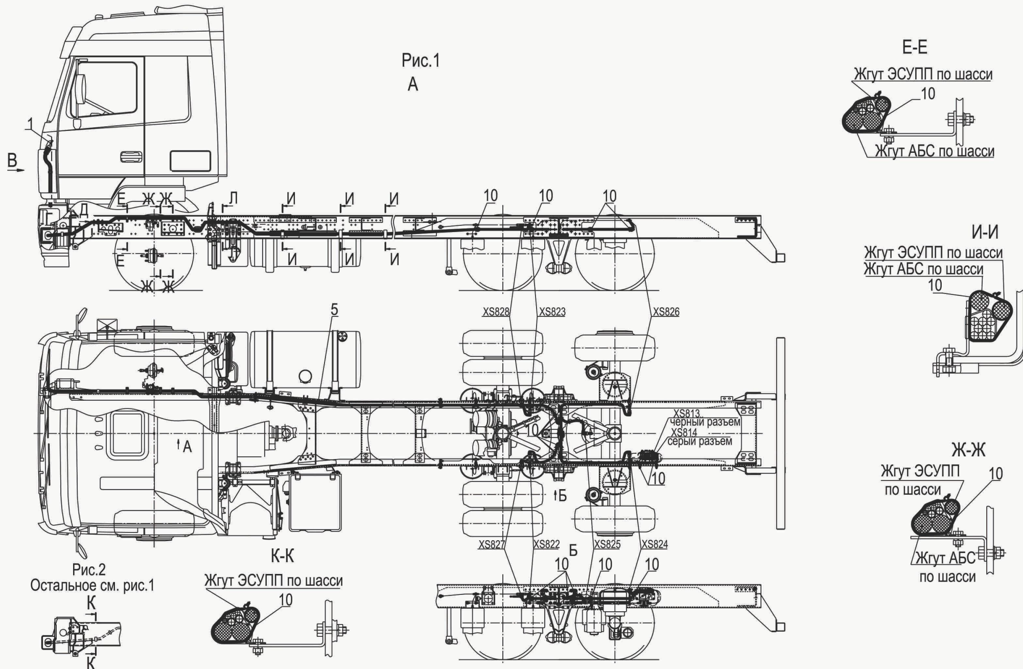
Рис. 217 Установка электрооборудования пневмоподвески 631019-3800050 (лист 1) Fig. 217 Setting of electrical equipment pneumosuspender 631019-3800050 (page 1)
