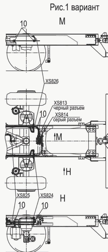
Рис. 217 Установка электрооборудования пневмоподвески 631019-3800050 (лист 2) Fig. 217 Setting of electrical equipment pneumosuspender 631019-3800050 (page 2)
