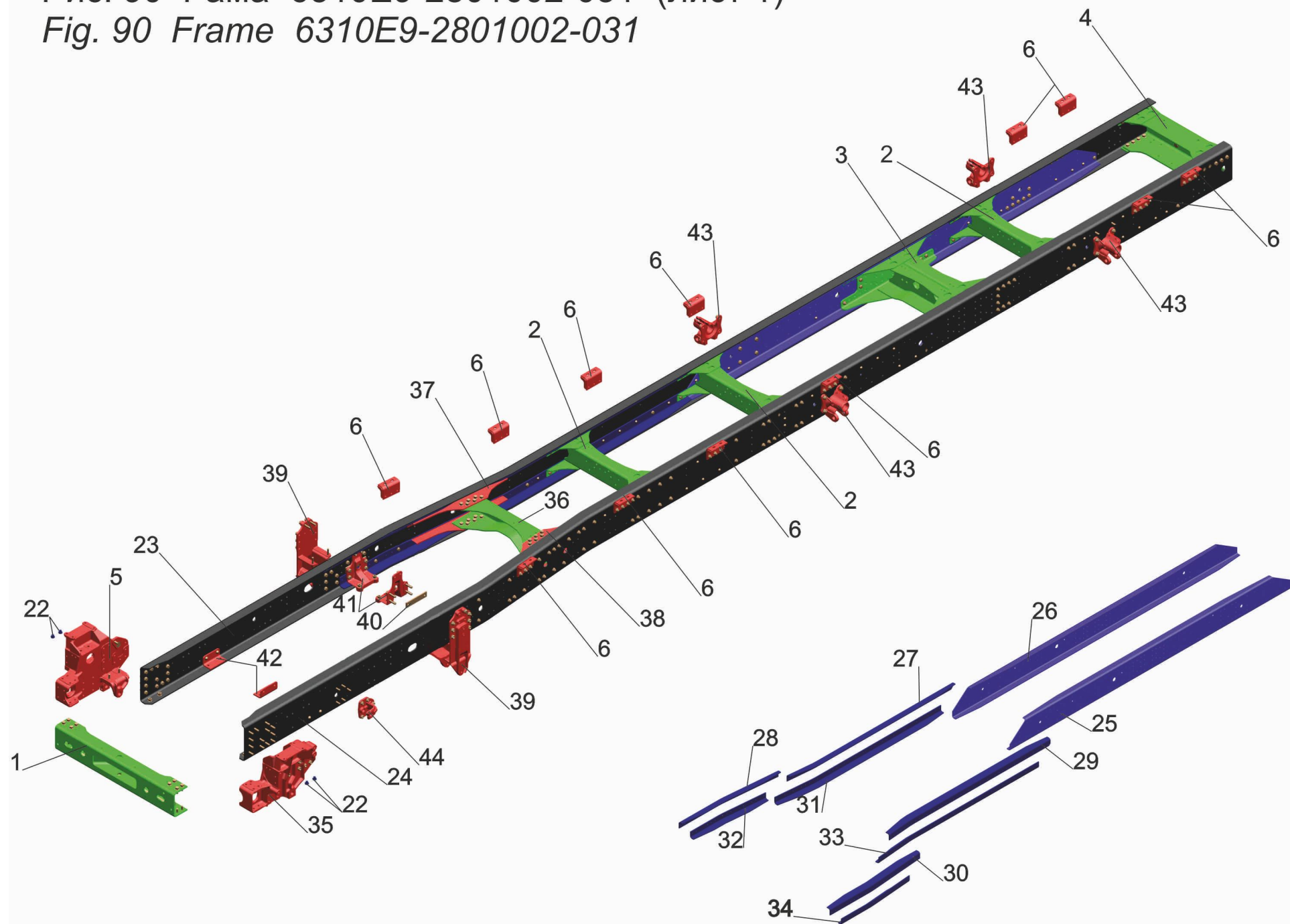
Рис. 90 Рама 6310Е9-2801002-031 (лист 1)
