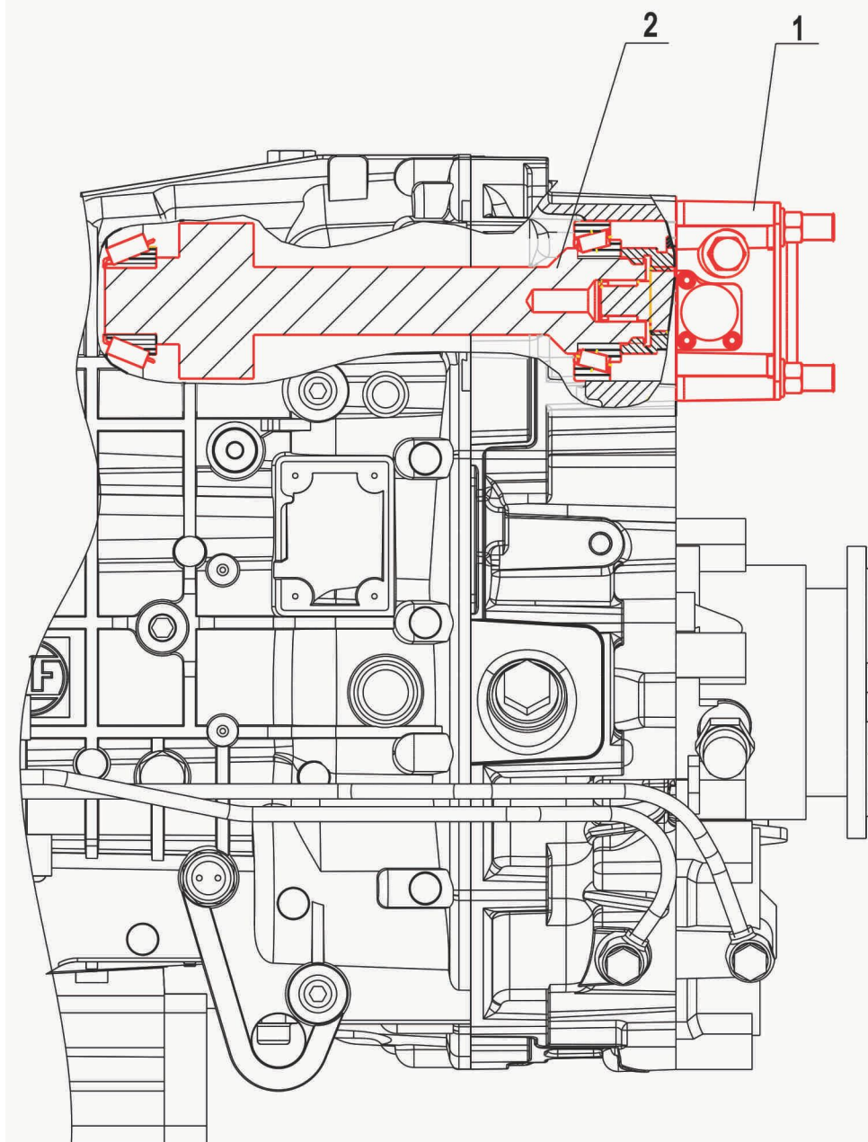
Рис. 326 Установка коробки отбора мощности 5550V5-8600007-069 Fig. 326 Installation power take-off gear box 5550V5-8600007-069
