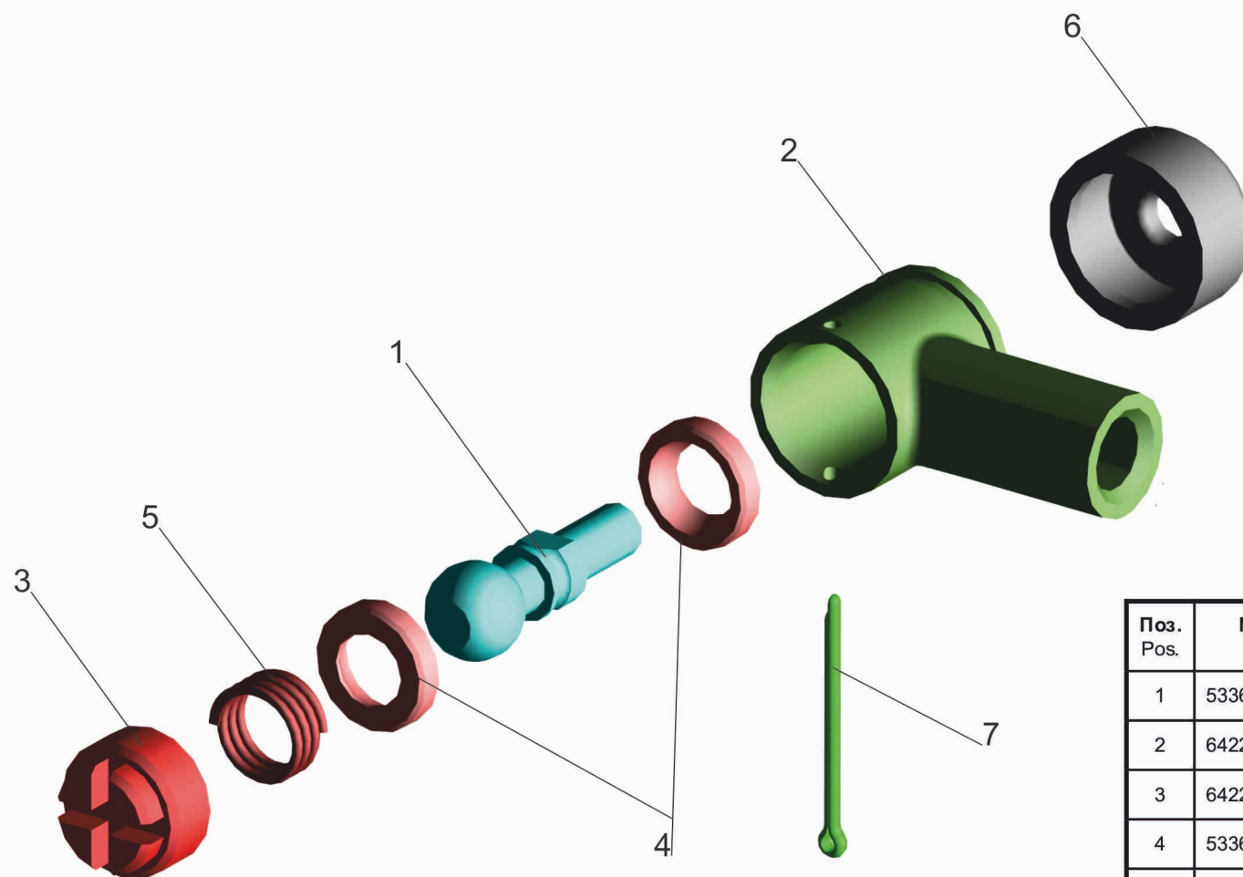
Рис. 58 Наконечник 6422-1703250 Fig. 58 Nozzle 6422-1703250
