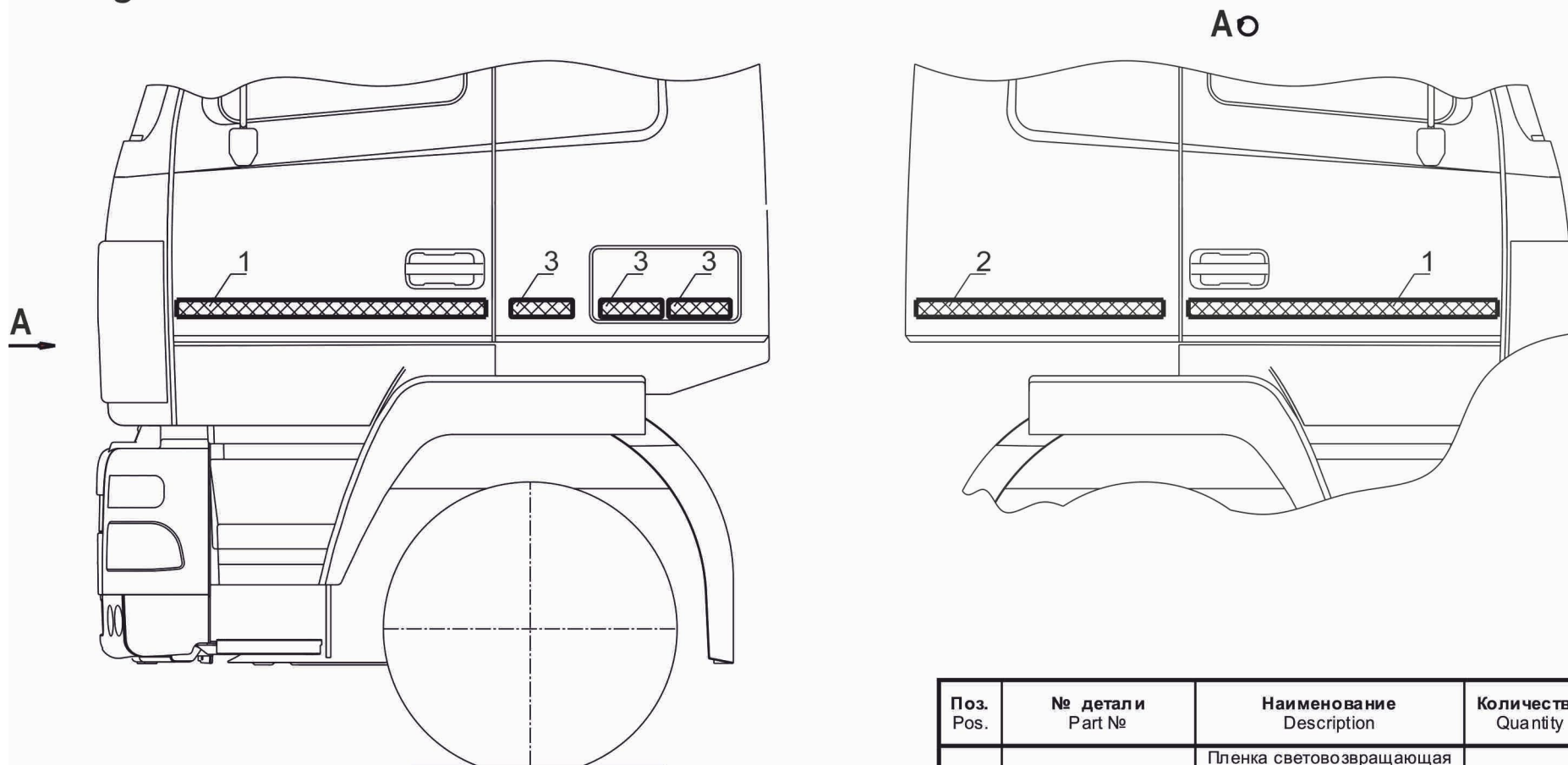
Рис. 193 Установка светоотражающей маркировки 6430-8200002 Fig. 193 Installation of switches 6430-8200002
