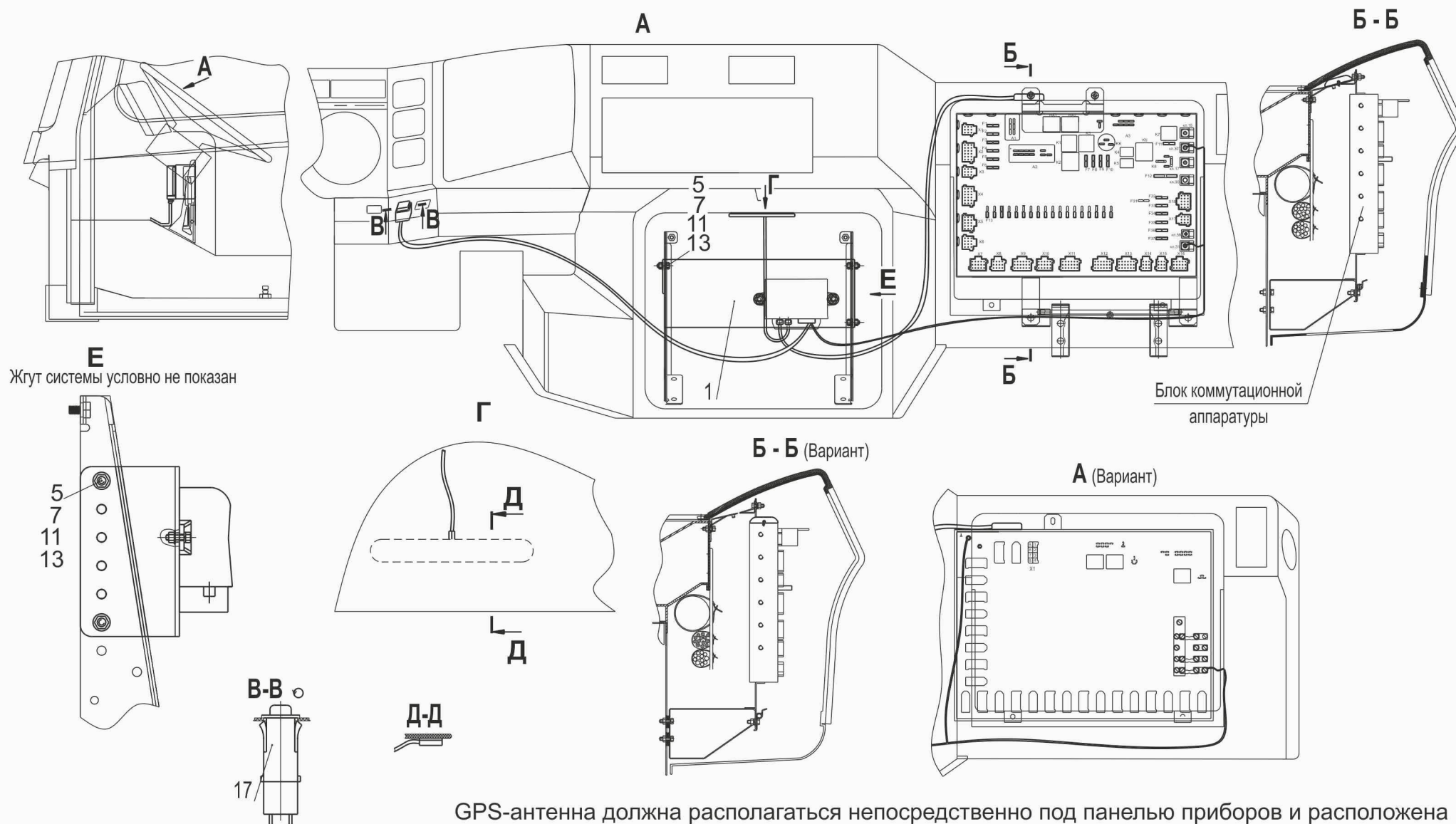
Рис. 191 Установка навигационного оборудования 643008-7937001-000 Fig. 191 Installation of navigation equipment 643008-7937001-000
