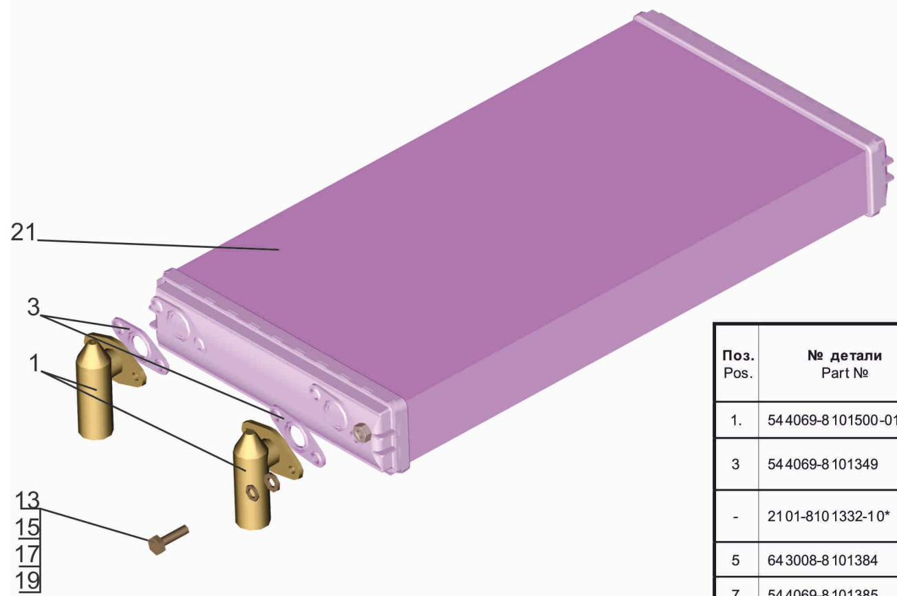
Рис. 288 Радиатор отопителя 643008-8101060-010 Fig. 288 Radiator of heating 643008-8101060-010
