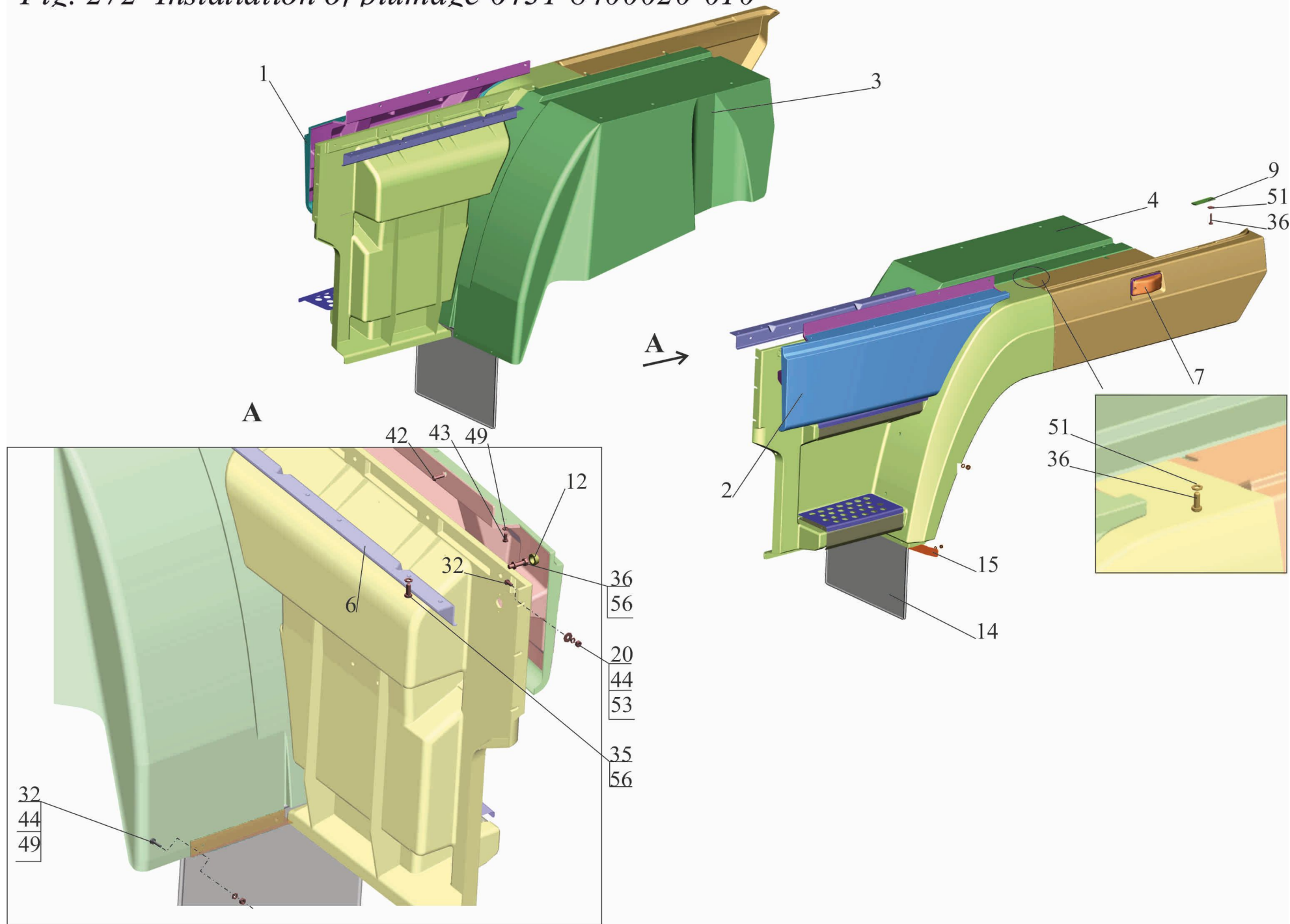
Fig. 272 Installation of plumage 6431-8400020-010
