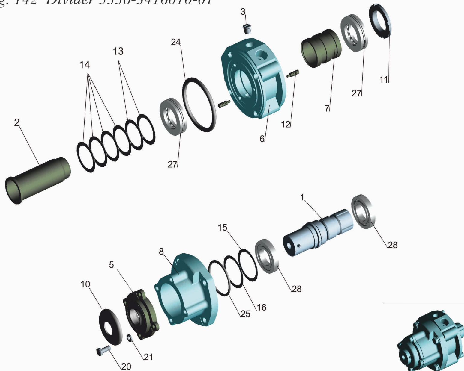
Рис. 142 Распределитель 5336-3416010-01 Fig. 142 Divider 5336-3416010-01
