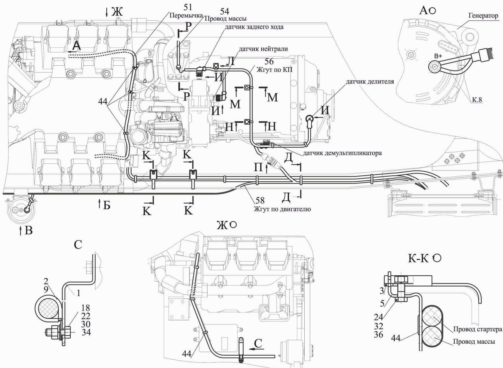
Рис. 207 Установка электрооборудования на двигателе 5340Е9-3700098 (лист 1) Fig. 207 Electric equipment installation on the engine 5340Е9-3700098 (page 1)
