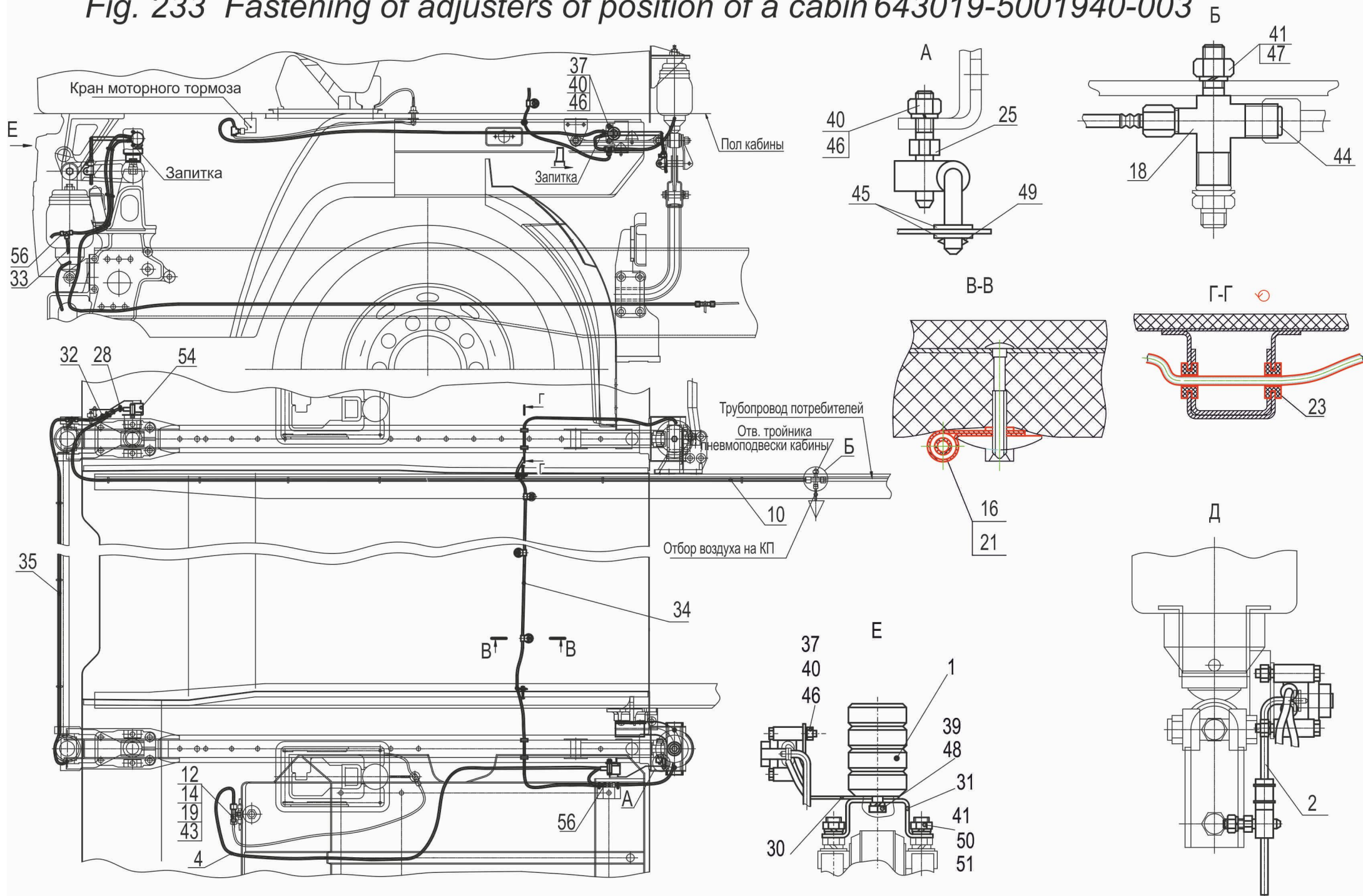
Рис. 233 Крепление регуляторов положения кабины 643019-5001940-003
