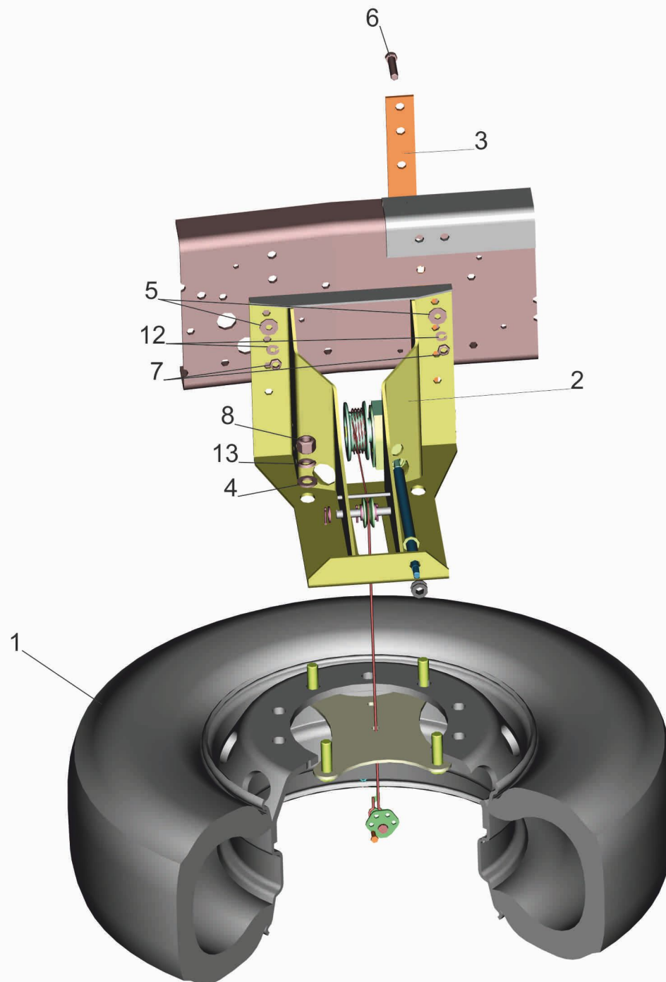
Рис. 132 Установка запасного колеса 6310E9-3100001
