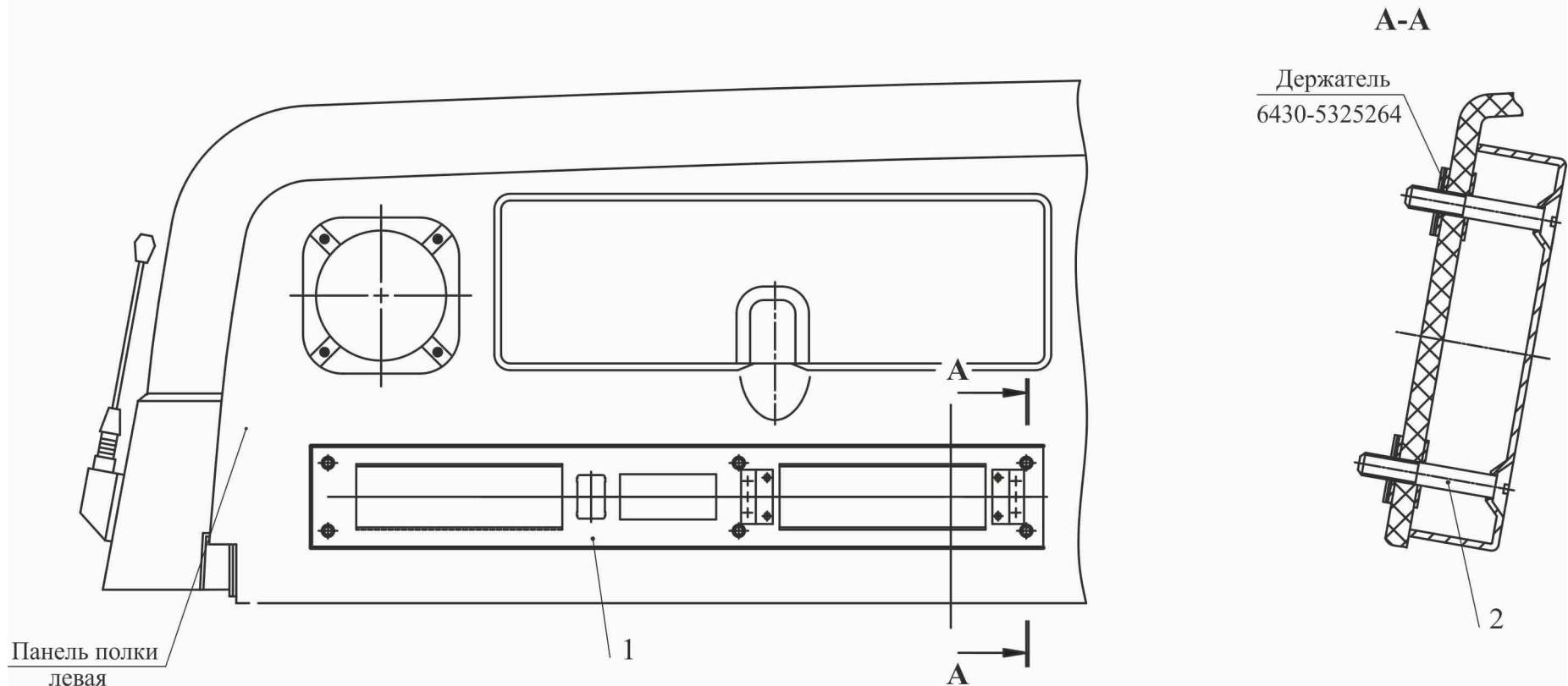
Рис. 187 Установка панели на полке 544019-7901080 Fig. 187 Panel installation on shelf 544019-7901080
