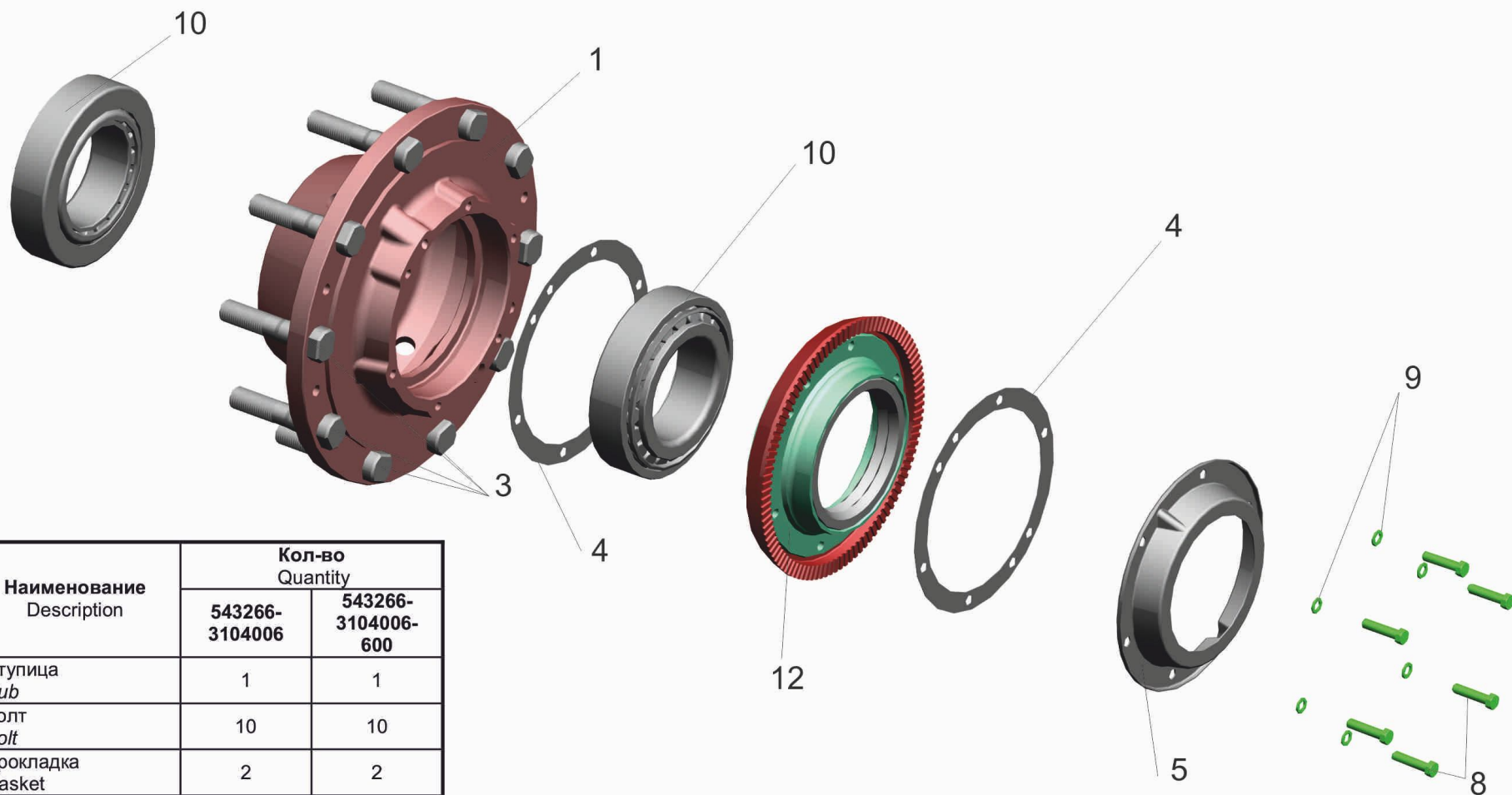
Рис. 70 Ступица с крышкой Fig. 70 Rear axle hub
