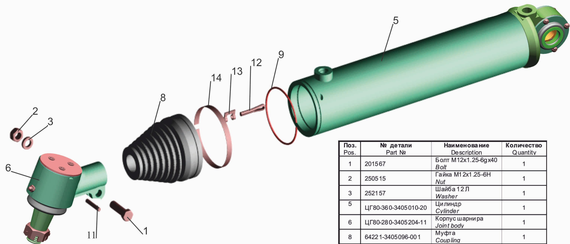
Рис. 159 Цилиндр 5336-3405005-20 (ЦГ80-360) Fig. 159 Cylinder 5336-3405005-20 (ЦГ80-360)
