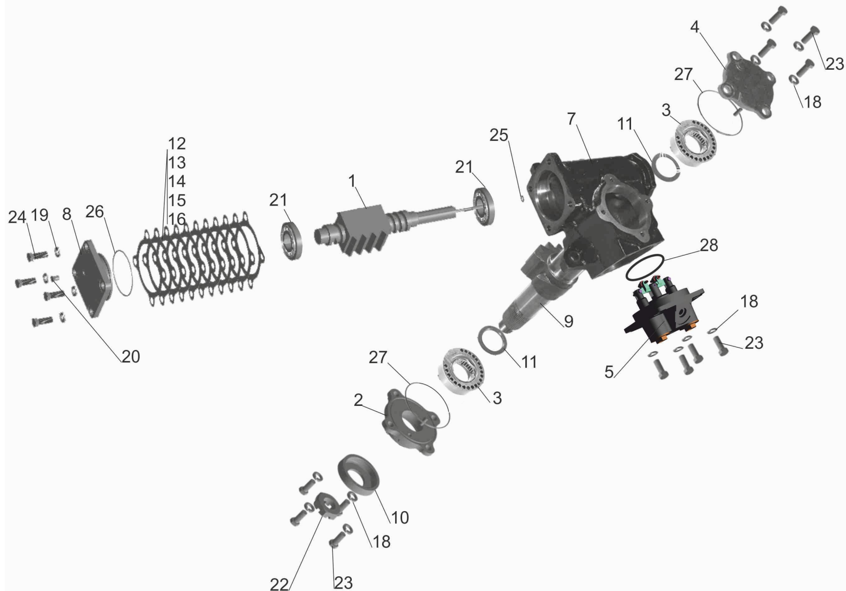
Рис. 141 Механизм рулевой 64221-3401005-10 Fig. 141 Steering mechanism 64221-3401005-10
