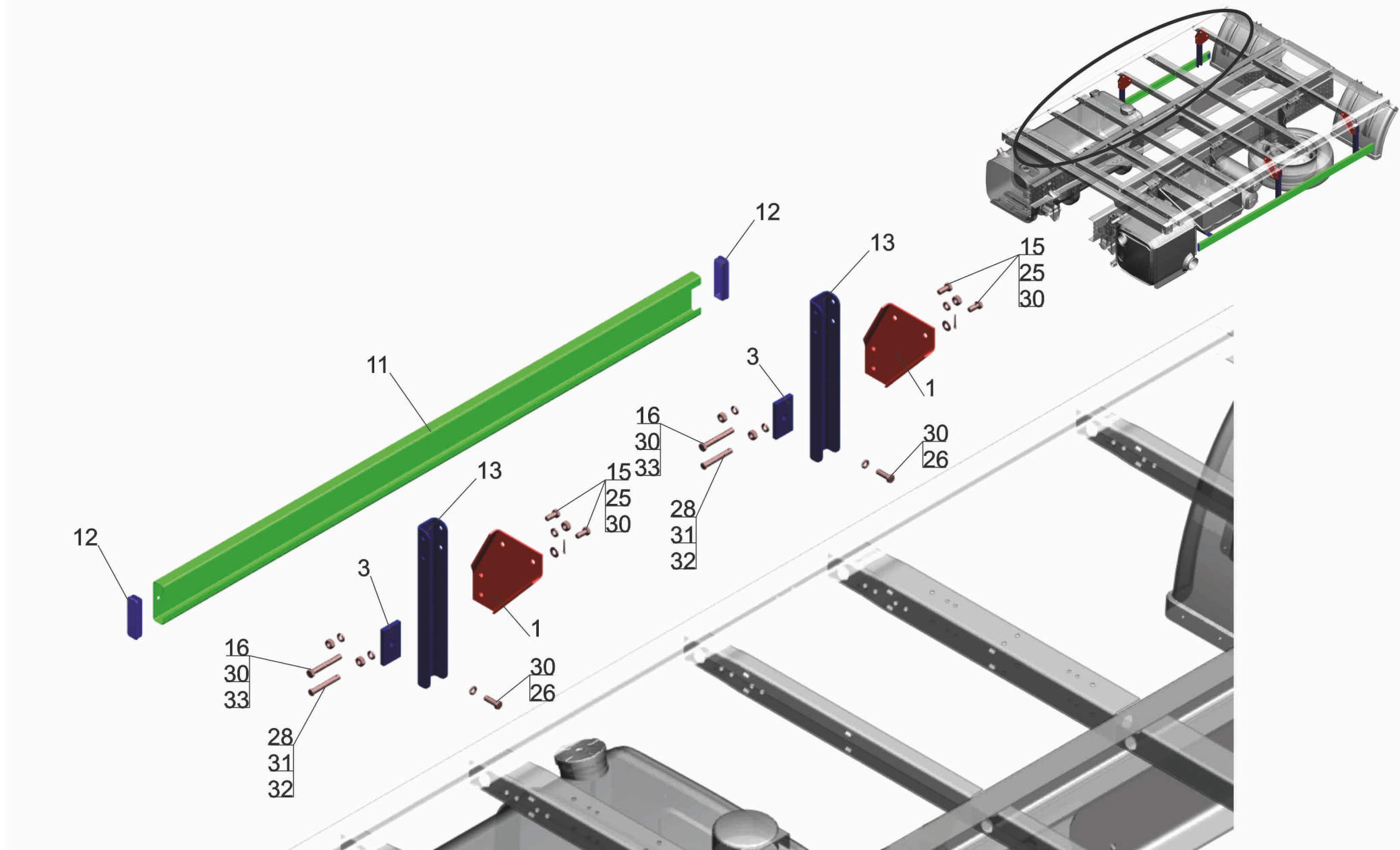
Рис. 95 Установка бокового ограждения 631019-2800040 (лист 1) Fig. 95 Installation of a lateral protection 631019-2800040 (page 1)
