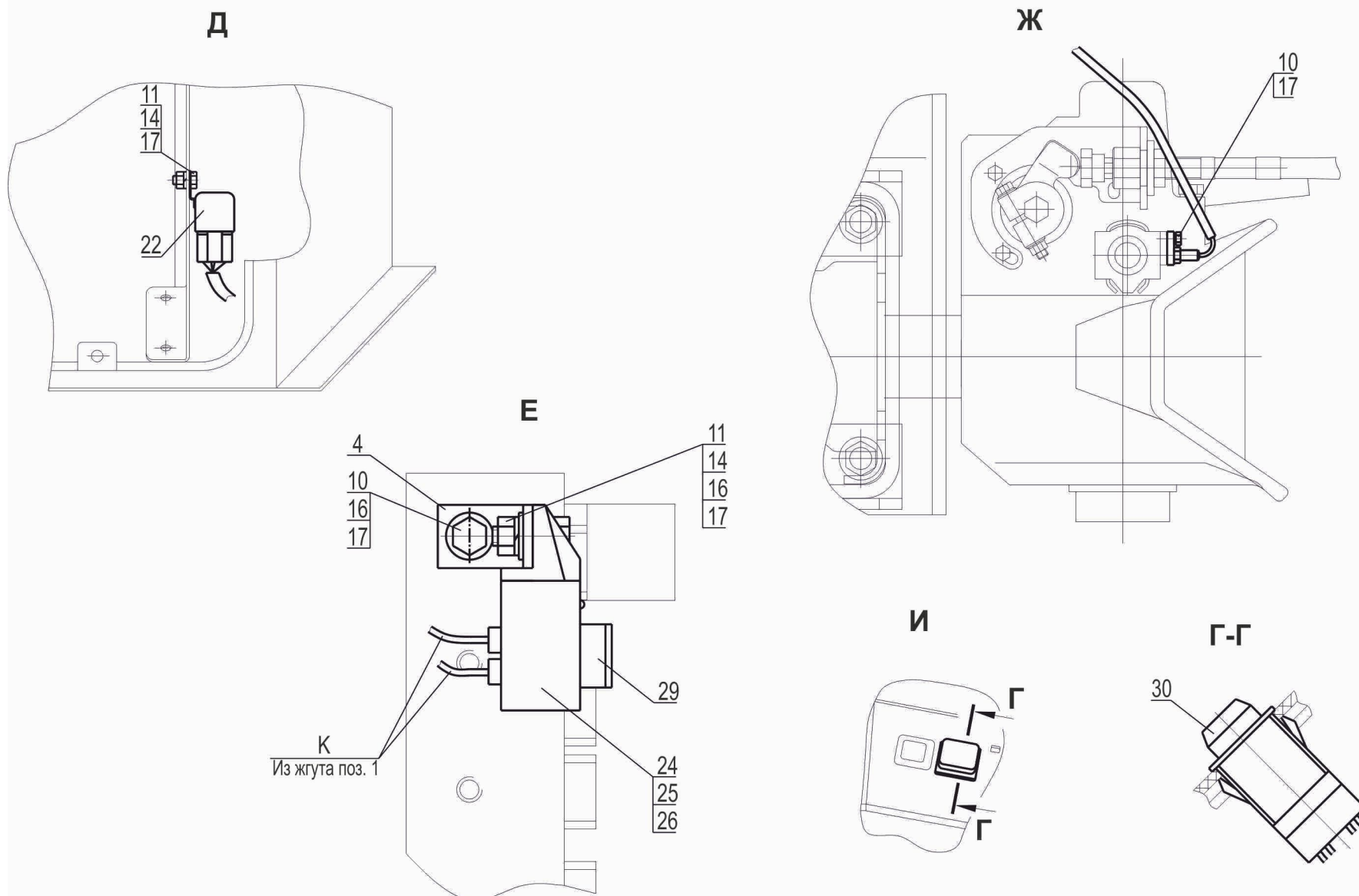
Рис. 186 Установка датчика сцепки 534019-3700164-000 (лист 2) Fig. 186 Installation of coupling sensor 534019-3700164-000 (page 2)
