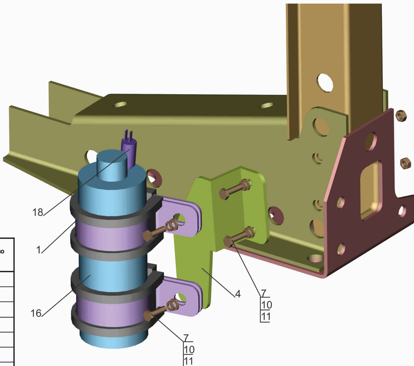
Рис. 301 Установка ресивера-осушителя 544020-8100036 Fig. 301 Installation of receiver-drier 544020-8100036
