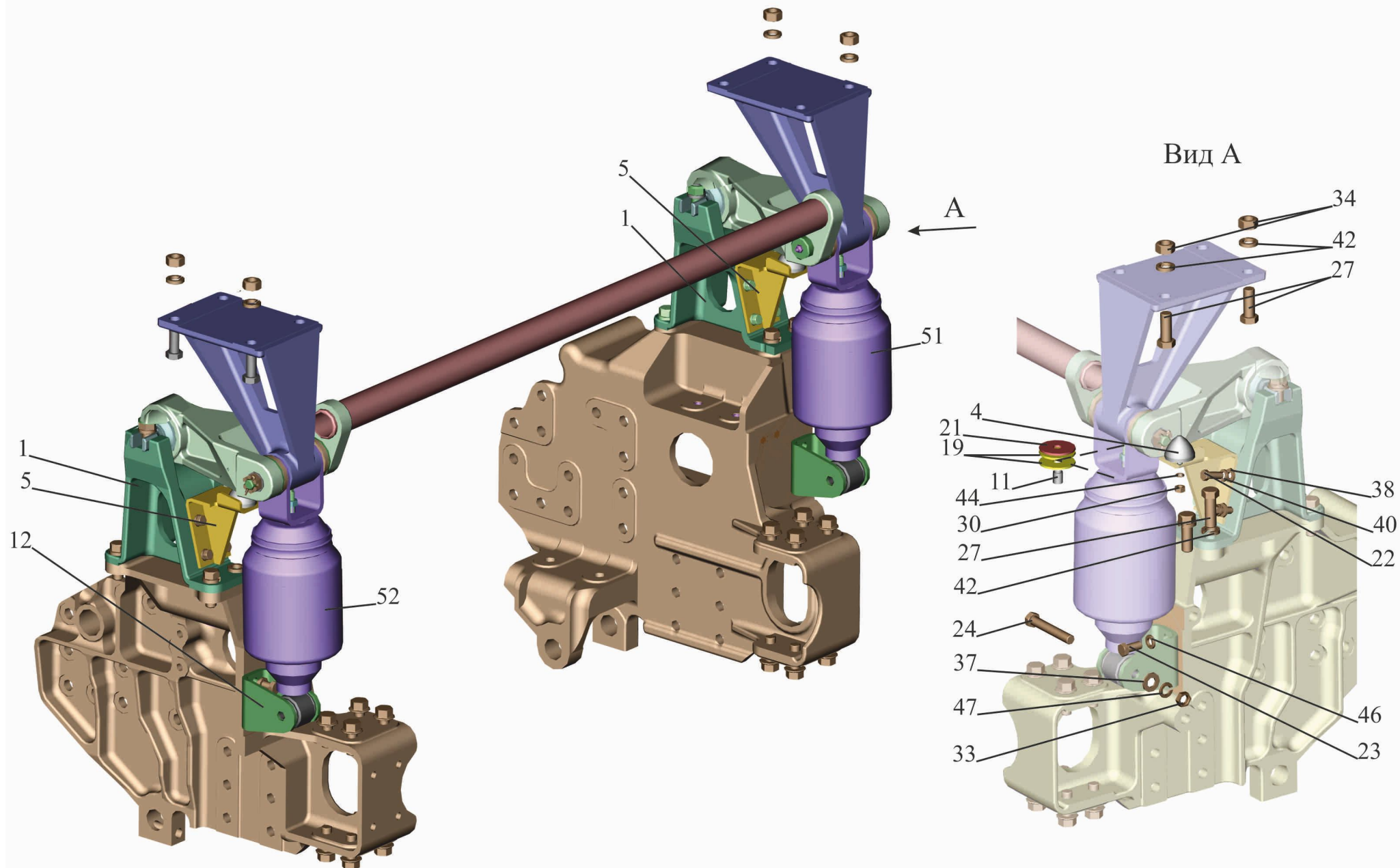
Рис. 228 Переднее подрессоривание кабины Fig. 228 Front springing the cab
