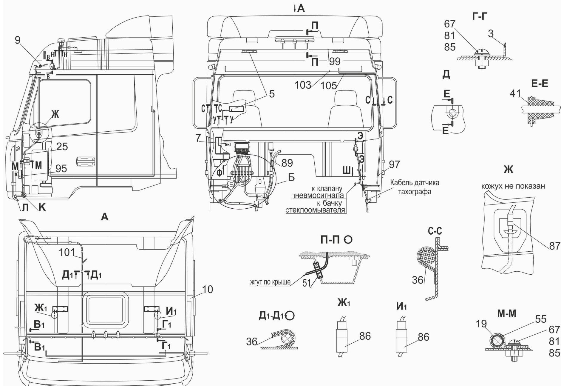
Рис. 199 Установка электрооборудования по кабине 5440А9-3700076 (лист 1) Fig. 199 Electric equipment installation on a cabin 5440A9-3700076 (page 1)
