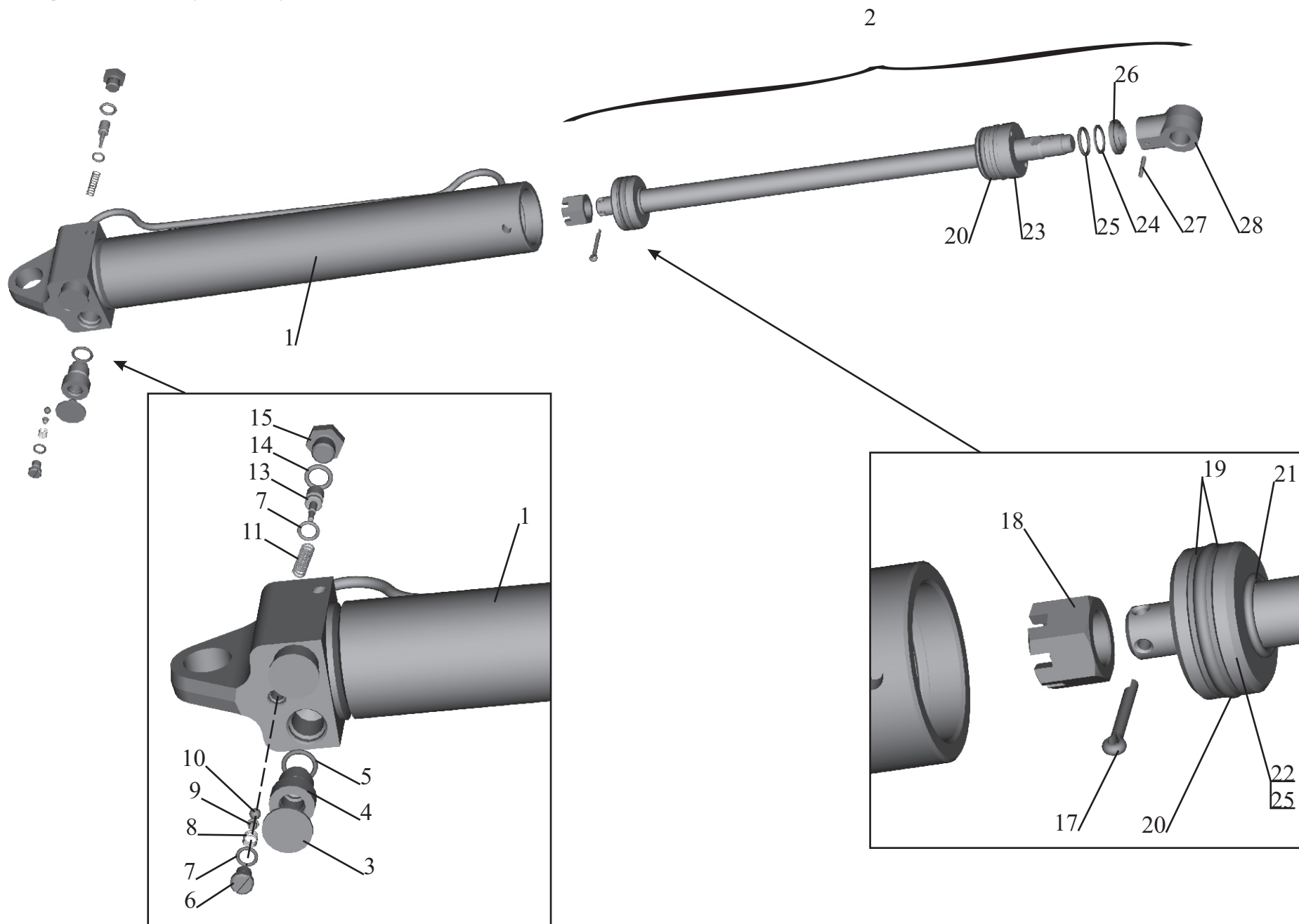
Рис. 208 Гидроцилиндр 64221-5003010 Fig. 208 Hydrocylinder 64221-5003010
