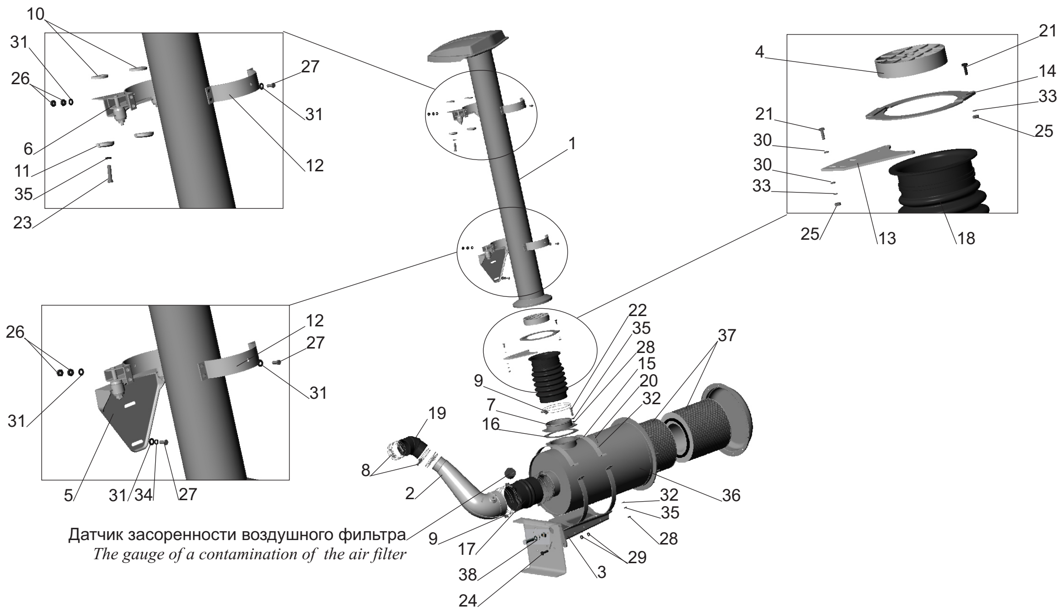
Рис. 19 Крепление воздушного фильтра 551605-1109002-020 Fig. 19 Mounting air cleaner 551605-1109002-020
