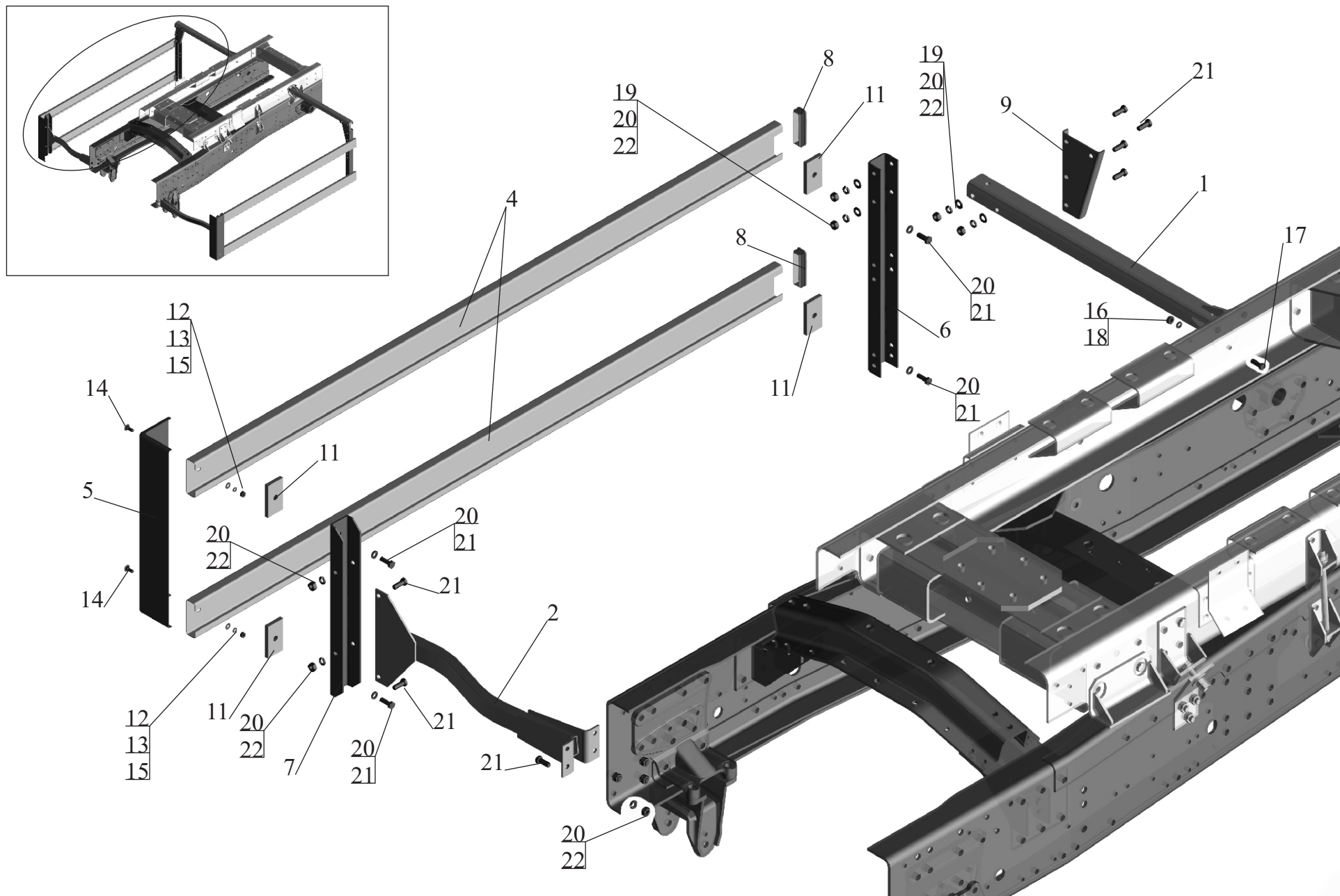
Рис. 72 Установка бокового ограждения 551605-2800040-010 (лист 1) Fig. 72 Installation of a lateral protection 551605-2800040-010 (page1)
