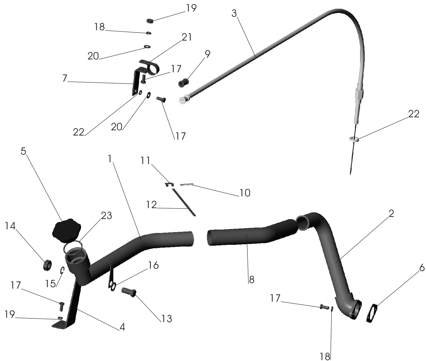
Рис. 2 Установка системы заливки и контроля уровня масла 630300-1018002 Fig. 2 Installation of system of oil priming and its level checking 630300-1018002
