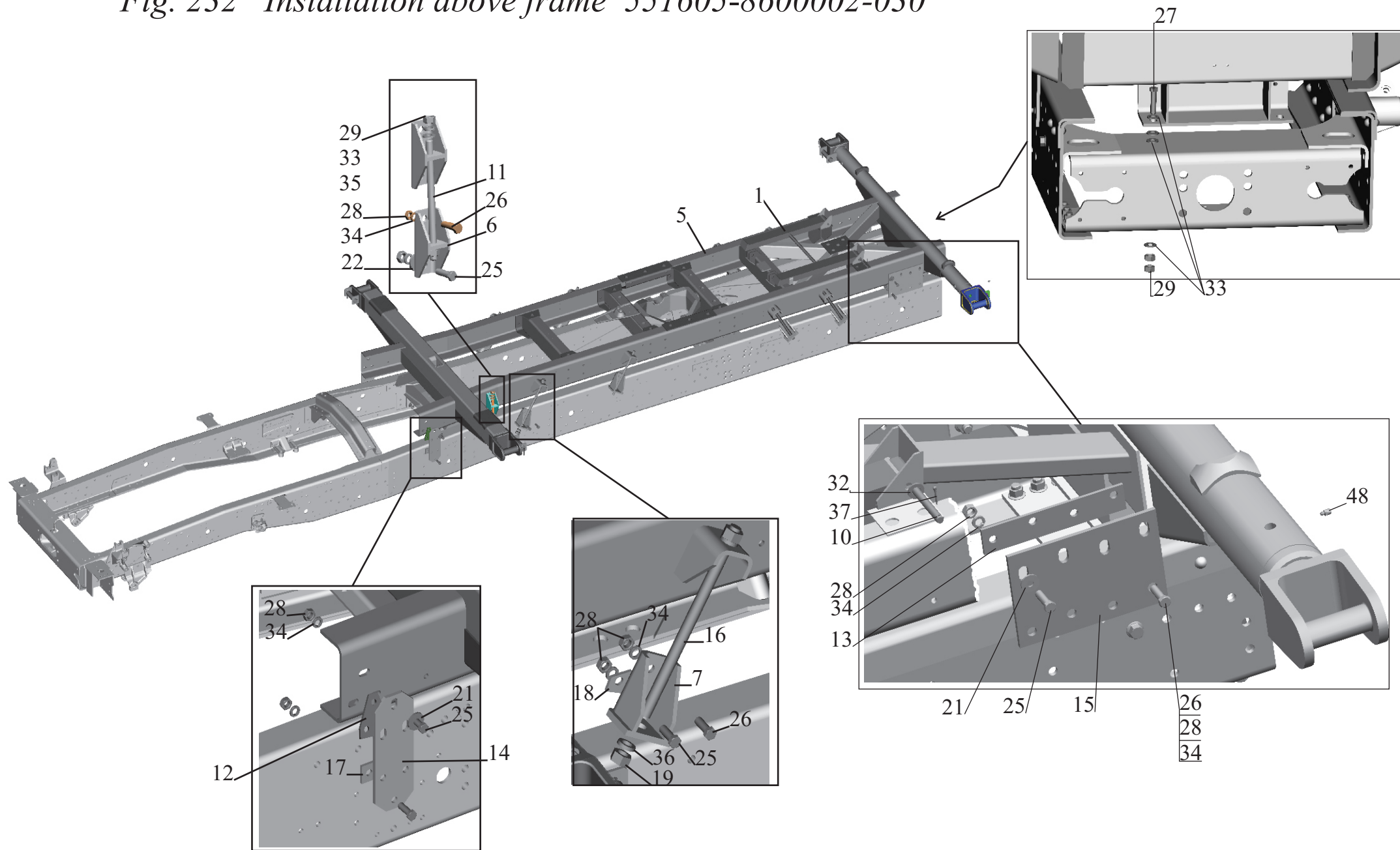
Рис. 232 Установка надрамника 551605-8600002-030 Fig. 232 Installation above frame 551605-8600002-030
