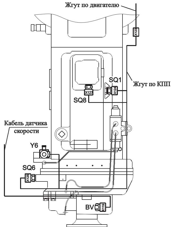
КПП ЯМЗ-239 gearbox ЯМЗ-239
