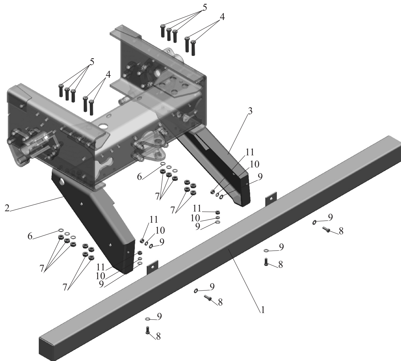
Рис. 69 Установка заднего бампера на МАЗ-551605 с трехсторонней разгрузкой Fig. 69 Installation of a back bumper on MAZ-551605 with tripartite unloading
