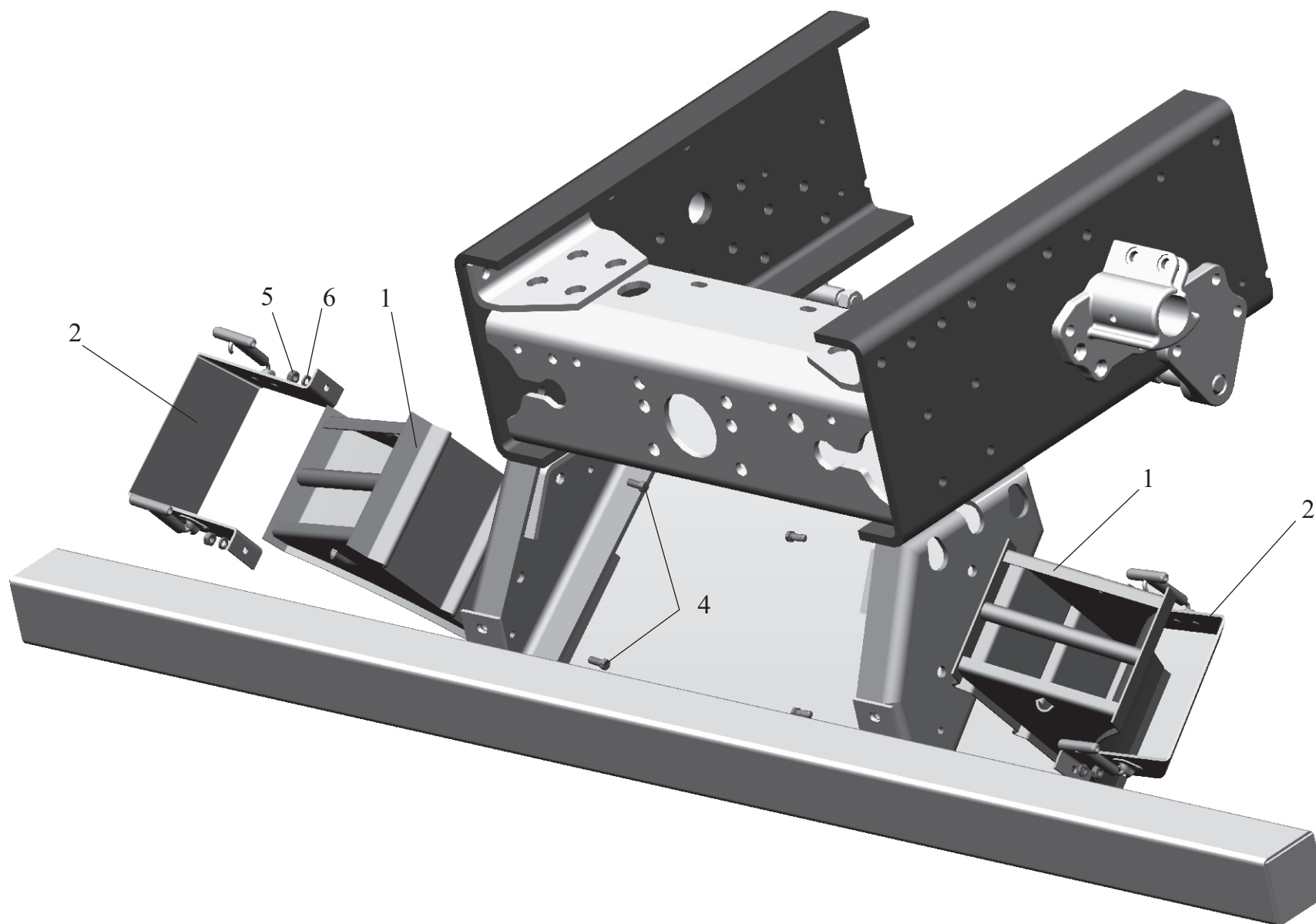
Рис. 169 Установка противооткатных упоров 53373-3900037 Fig. 169 Installation of buffer stop 53373-3900037
