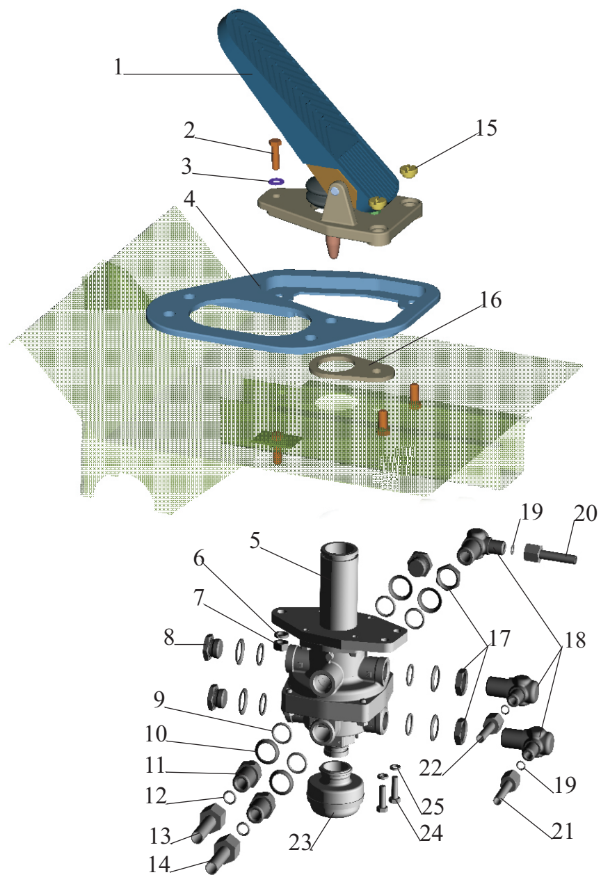
Рис. 109 Крепление тормозного крана 64221-3514004-20 Fig. 109 Mounting brake valve 64221-3514004-20
