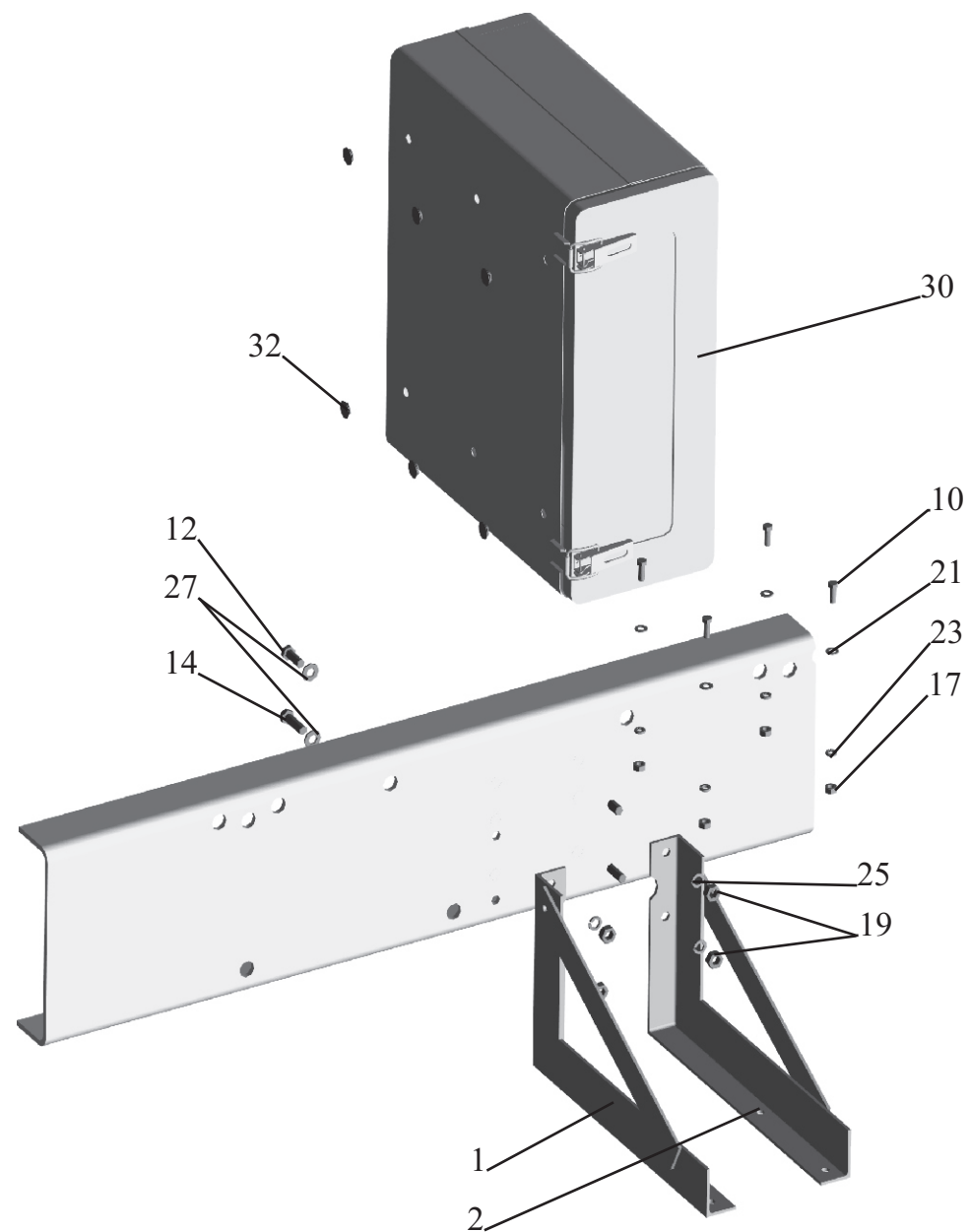
Рис. 227 Установка инструментального ящика 551639-8500009-010 Fig. 227 The tools box installation 551639-8500009-010
