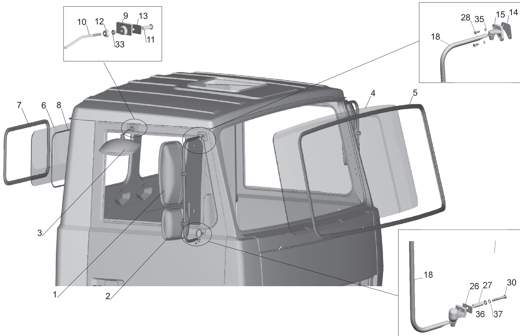
Рис. 188 Установка стекол и зеркал на малую кабину 555102-5000012 Fig. 188 Installation glasses and mirrors on small cab 555102-5000012
