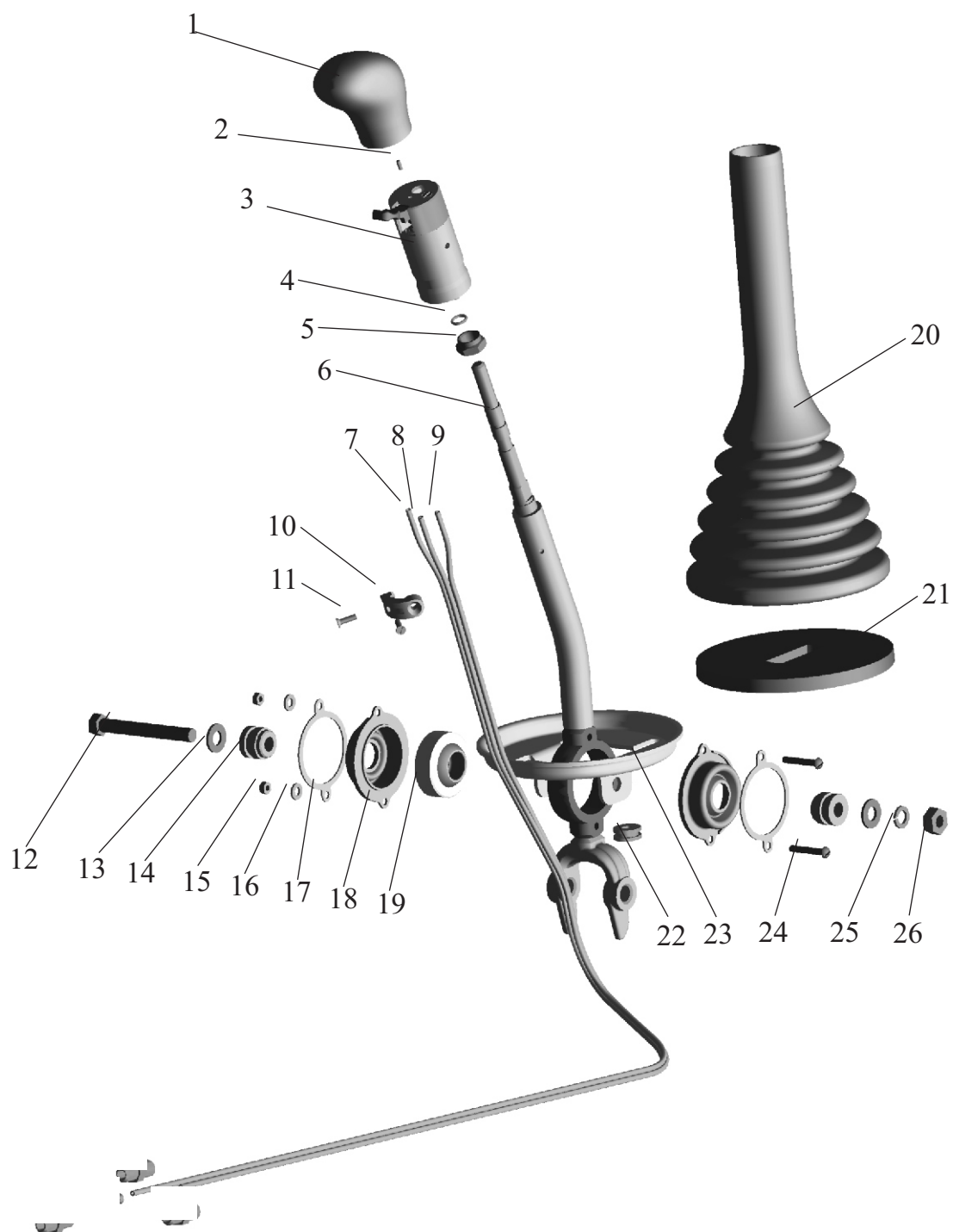
Рис. 36 Рычаг 64221-1703410-01 Fig. 36 Lever 64221-1703410-01
