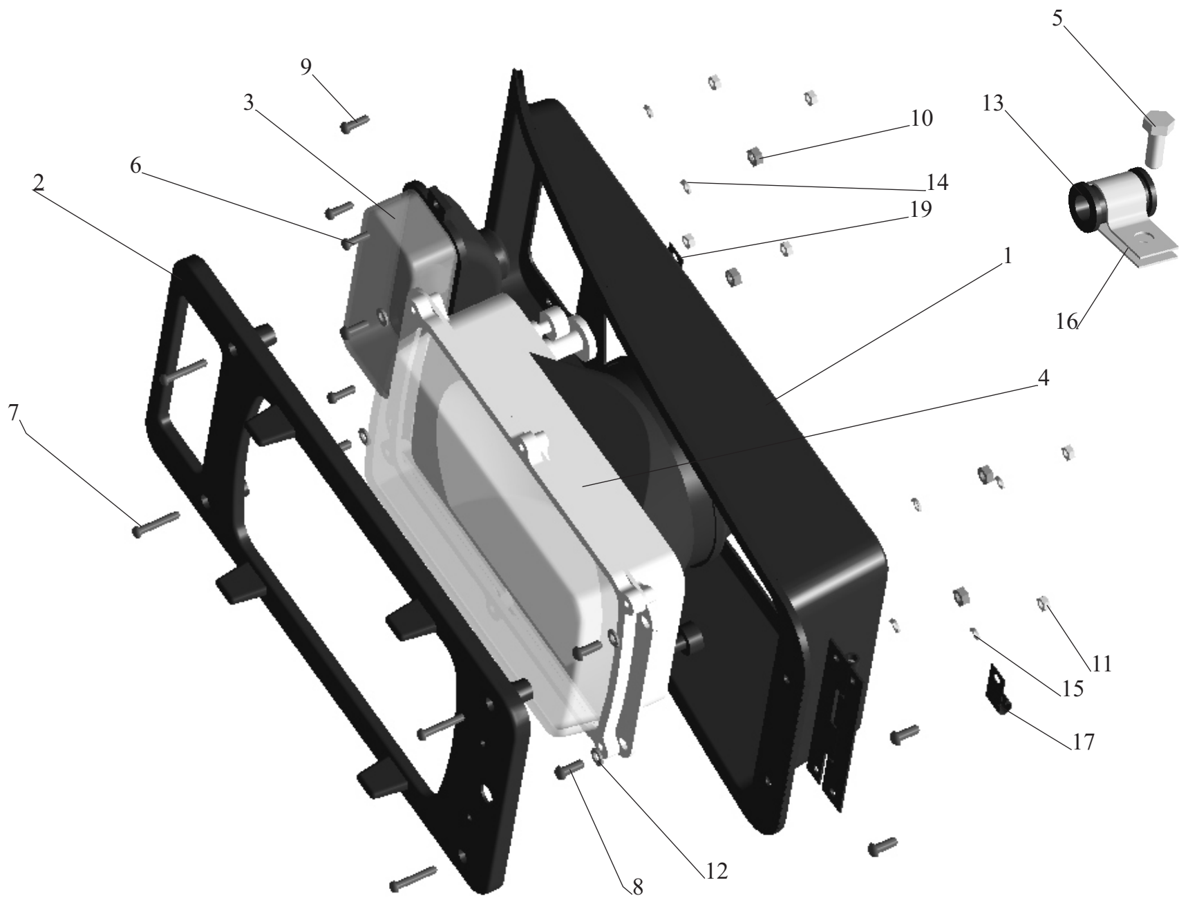
Рис. 130 Установка головных фар 64221-3711029-010, 64221-3711030-010 Fig. 130 Installing of head lights 64221-3711029-010, 64221-3711030-010
