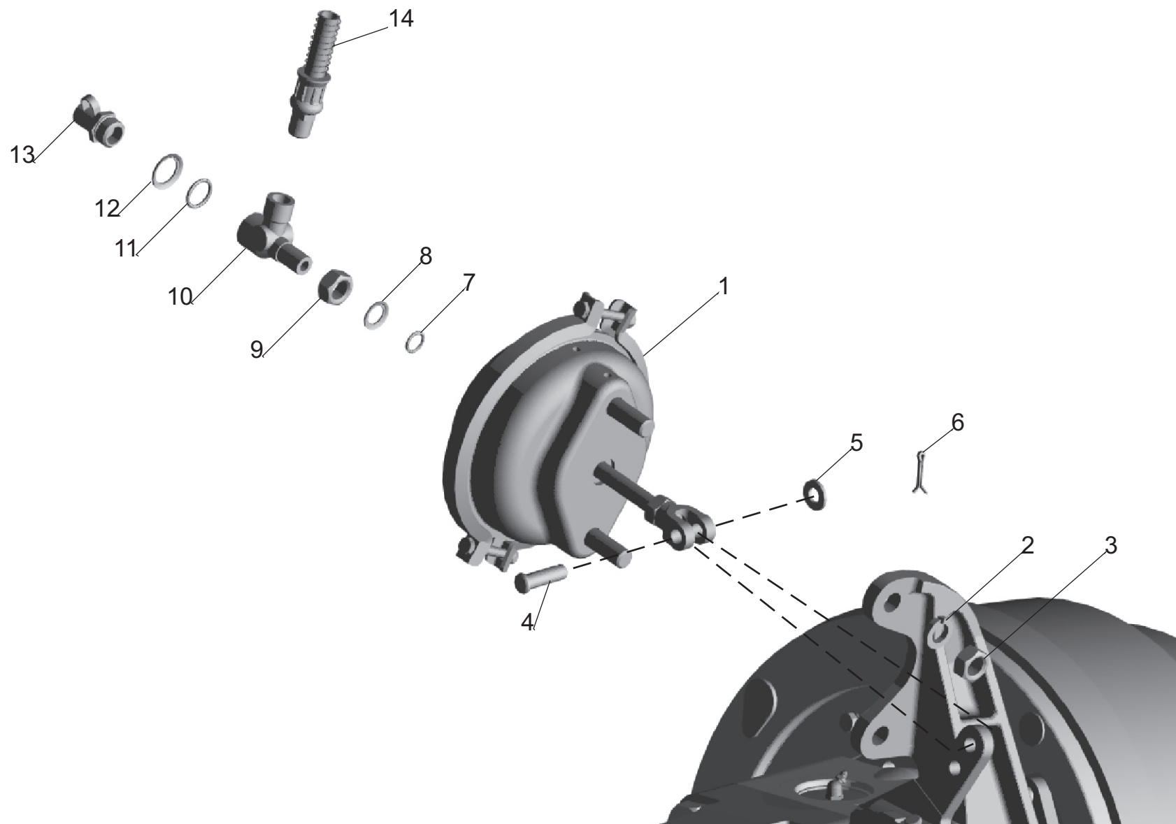
Рис. 113 Крепление тормозных камер 643008-3519001 Fig. 113 Mounting of brake chambers 643008-3519001
