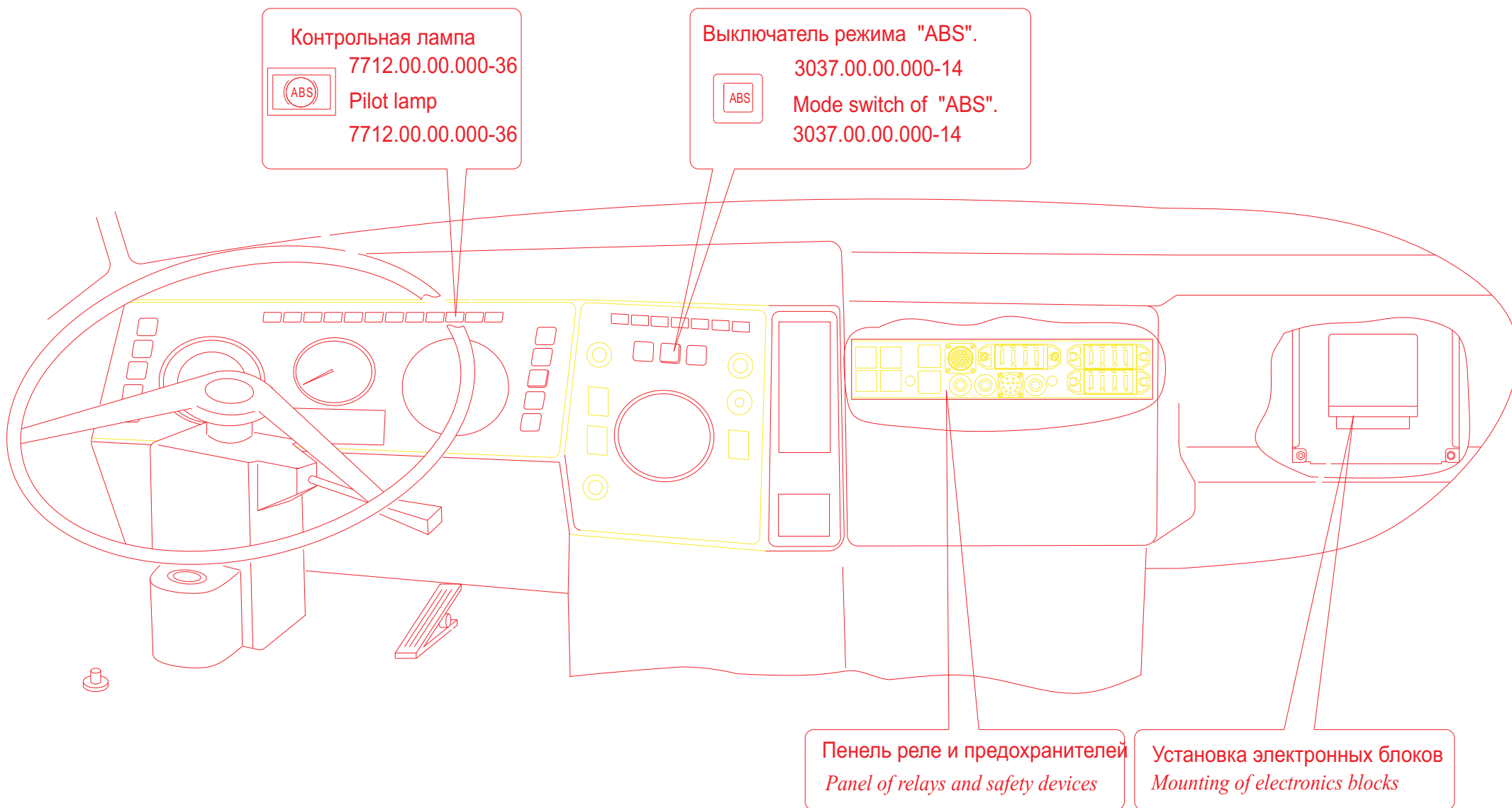
Рис. 162 Расположение элементов электронных систем в кабине автомобиля МАЗ - 551605 без прицепа Fig. 162 Elements arrangement of electronical systems in vehicle cabin of MAZ - 551605 without the trailer
