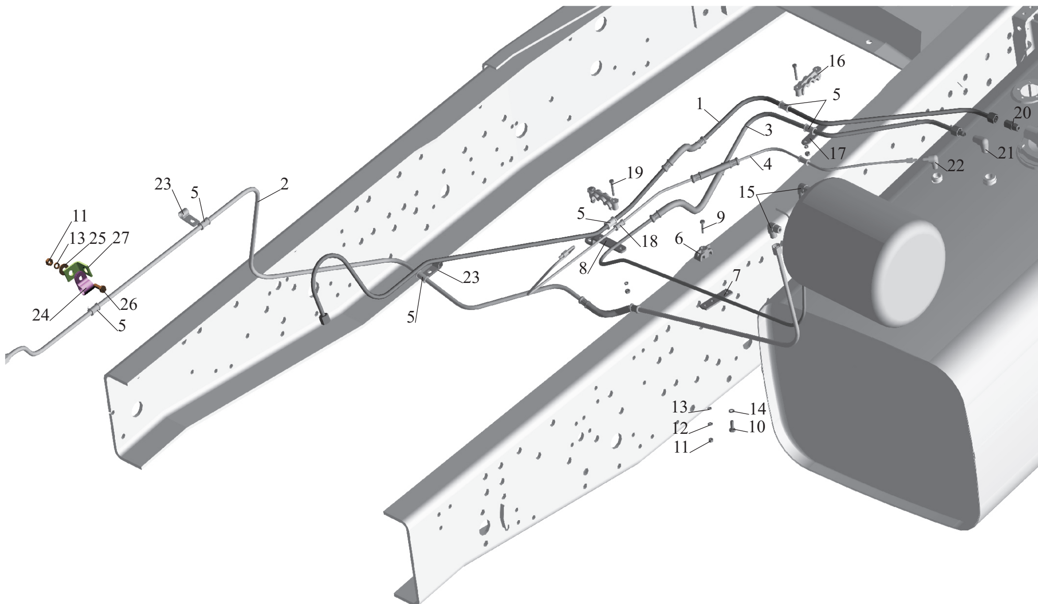
Рис. 13 Установка топливopоводов 551605-1104002 (с подогревателем) Fig. 13 Installation of fuel lines 551605-1104002 (with heater)
