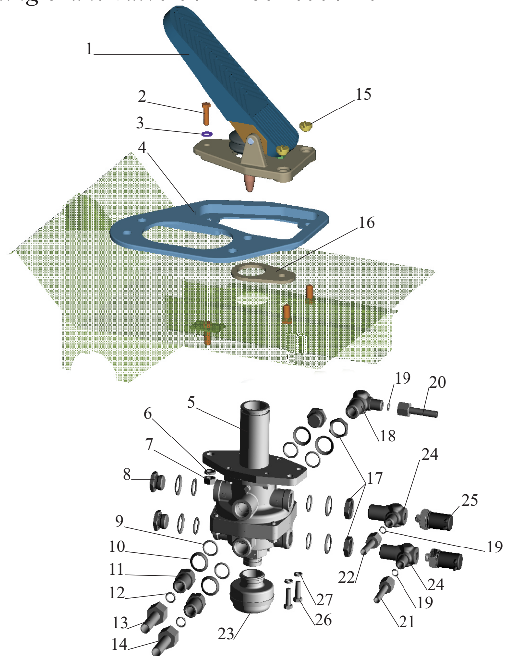
Рис. 108 Крепление тормозного крана 64221-3514004-20 Fig. 108 Mounting brake valve 64221-3514004-20
