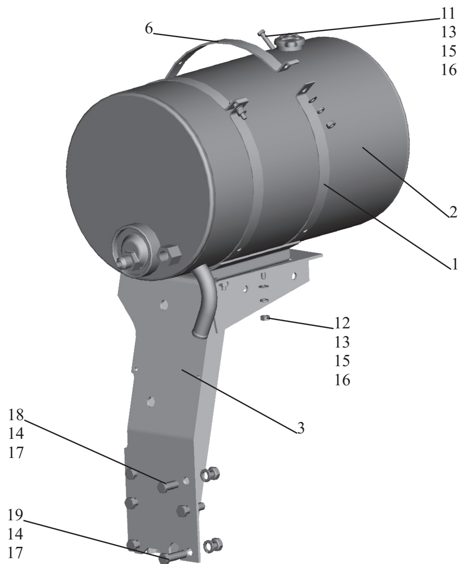
Рис. 246 Установка масляного бака 551605-8600034-025 Fig. 246 Installation oil tank 551605-8600034-025
