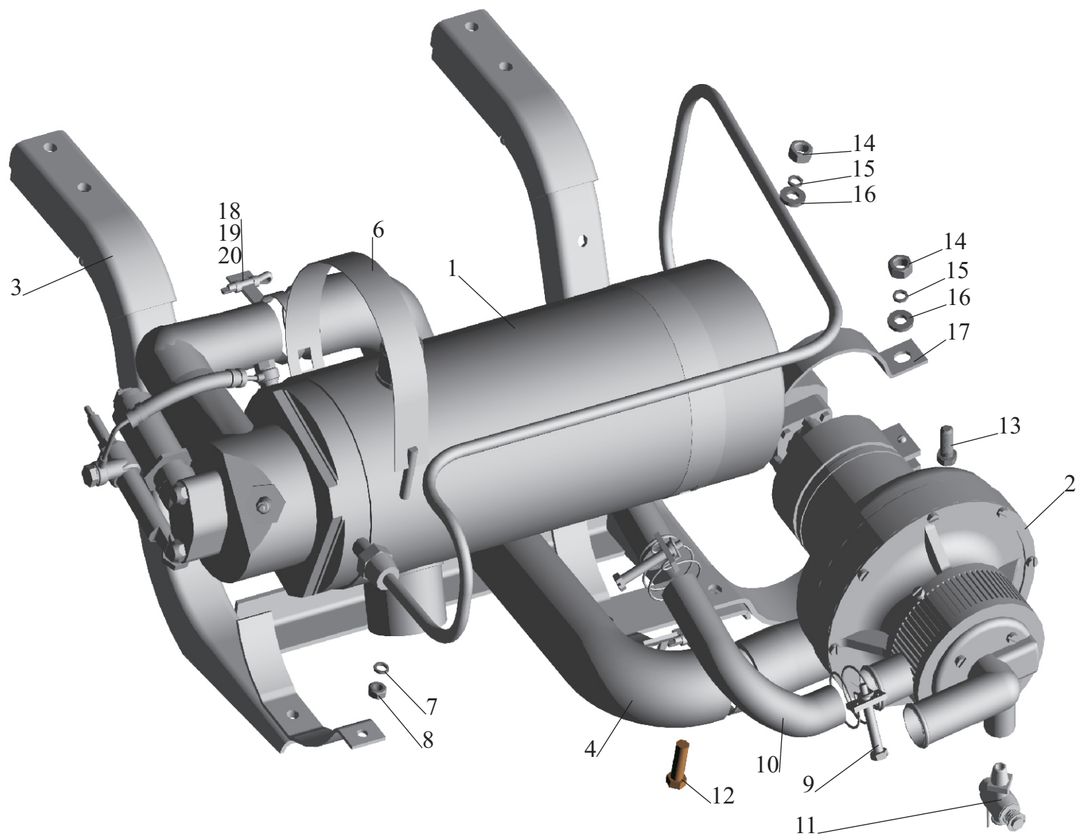
Рис. 6 Подогреватель 6422-1015006 Fig. 6 Heater 6422-1015006
