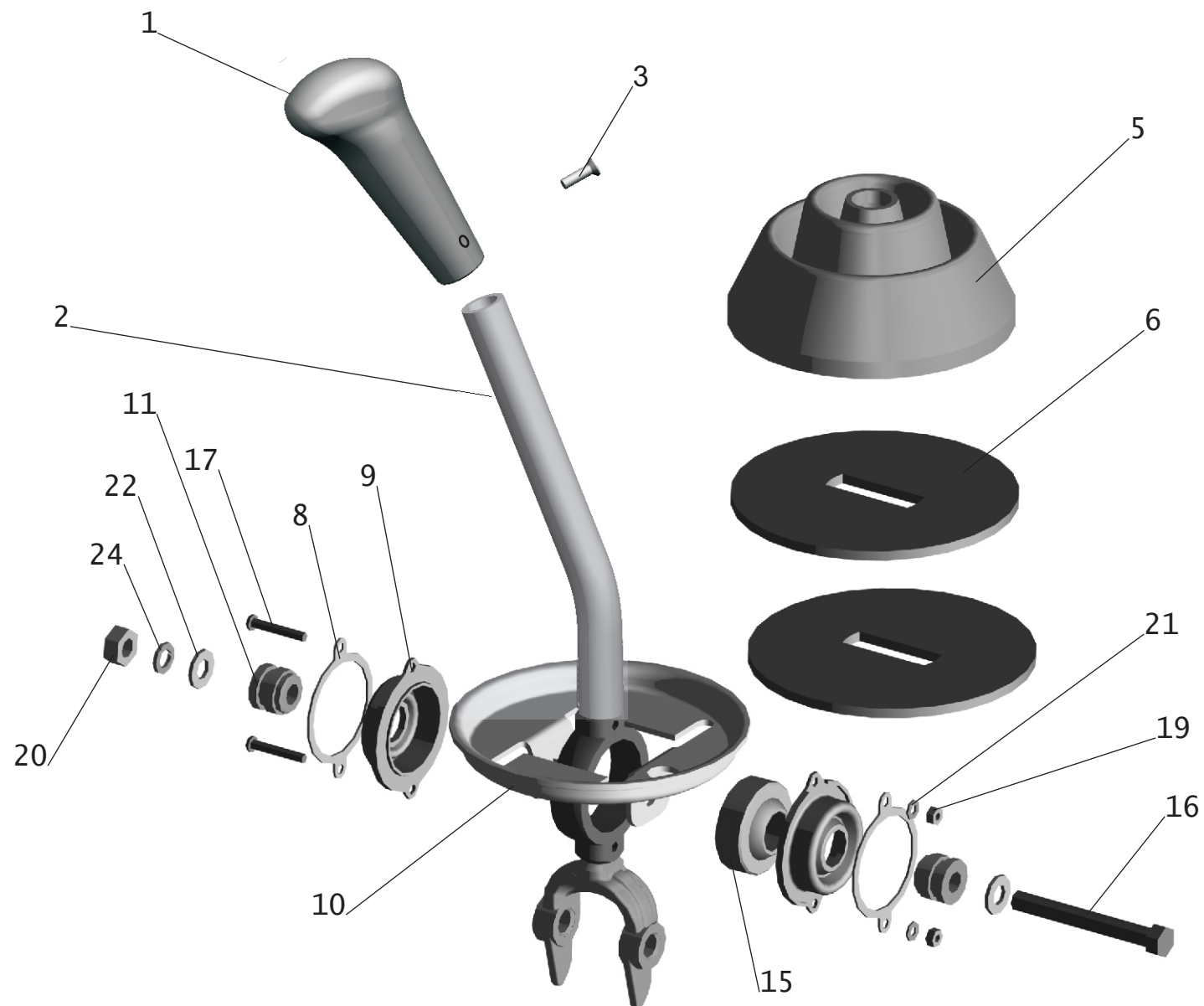
Рис. 37 Рычаг 4370-1703410 Fig. 37 Lever 4370-1703410
