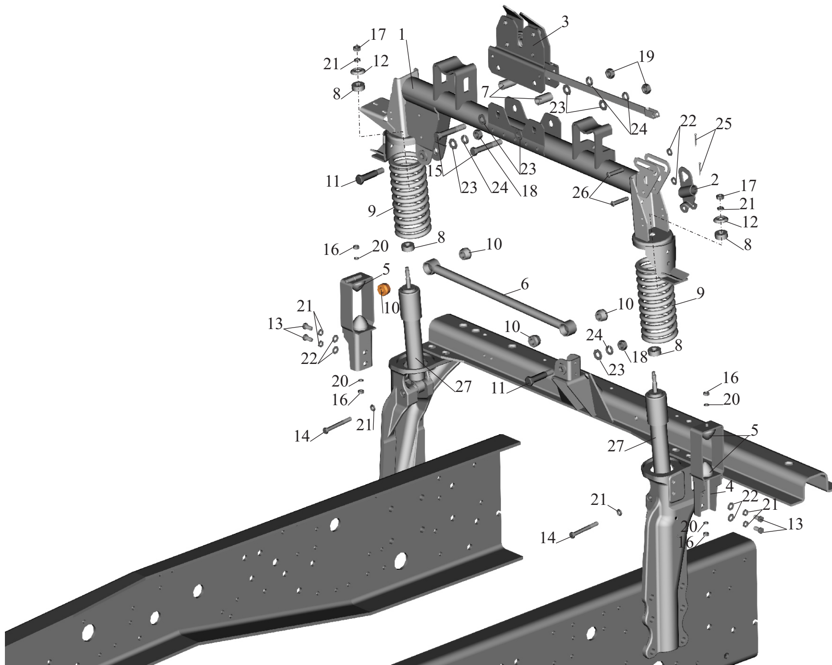
Рис. 180 Заднее подрессоривание большой кабины 64221-5001800 Fig. 180 Rear springing the large cab 64221-5001800
