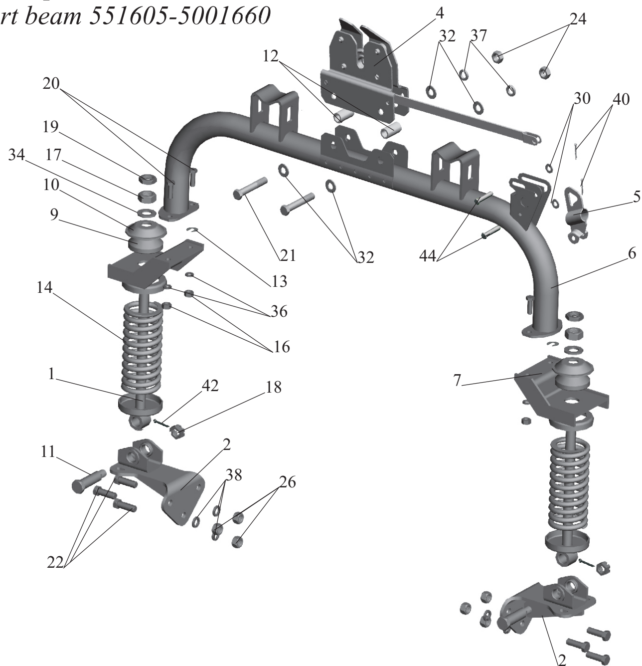
Рис. 177 Балка опоры 551605-5001660
