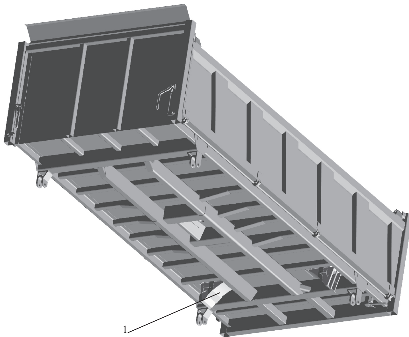
Рис. 170 Установка противооткатных упоров 551605-3900037 Fig. 170 Installation of buffer stop 551605-3900037
