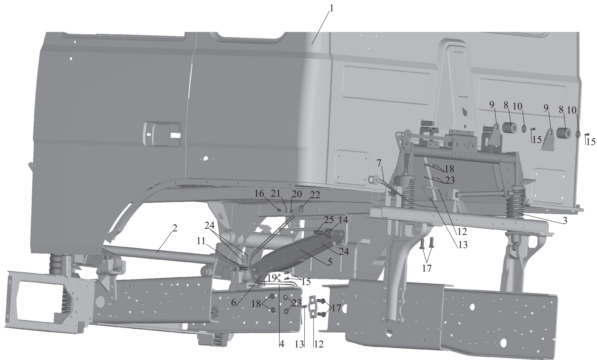
Рис. 178 Установка большой кабины Fig. 178 Installation of large cab
