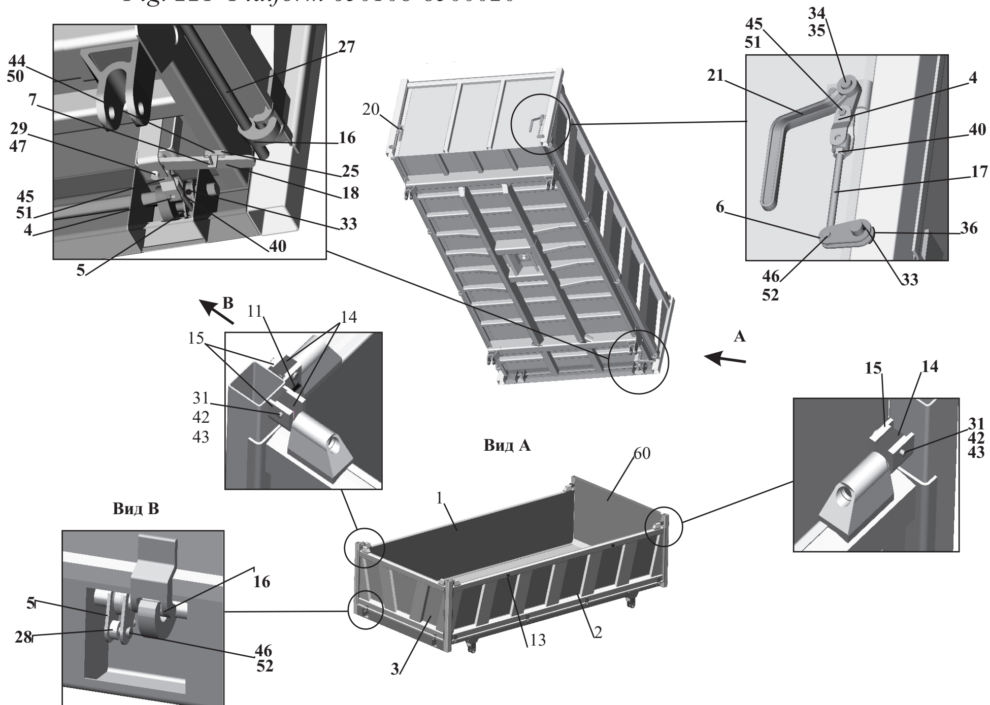
Fig. 221 Platform 650108-8500020
