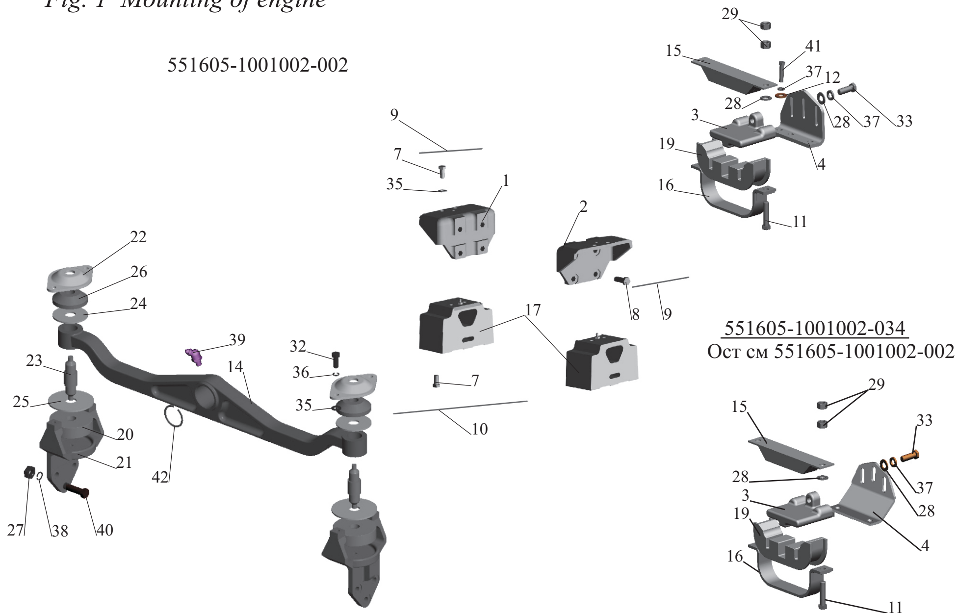
Рис. 1 Крепление двигателя Fig. 1 Mounting of engine
