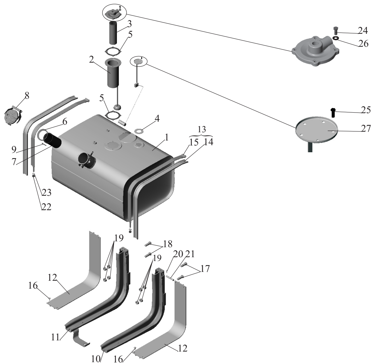
Рис. 11 Крепление топливного бака 551605-1101002 Fig. 11 Mounting of fuel tank 551605-1101002
