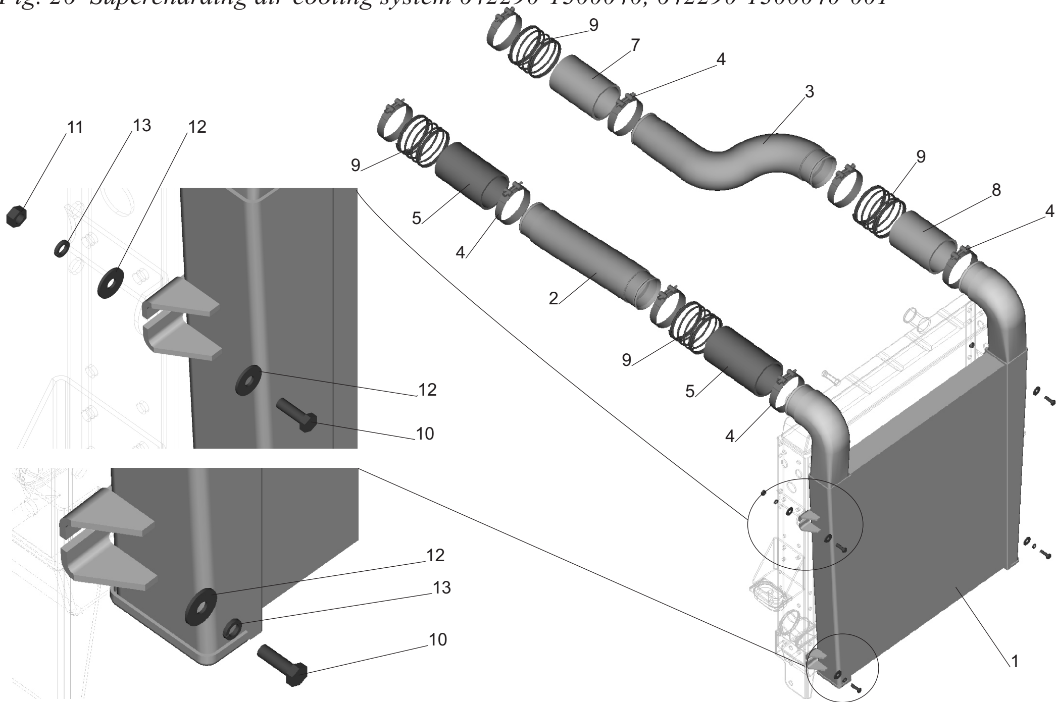
Рис. 26 Система охлаждения наддувочного воздуха 642290-1300040, 642290-1300040-001 Fig. 26 Supercharging air cooling system 642290-1300040, 642290-1300040-001
