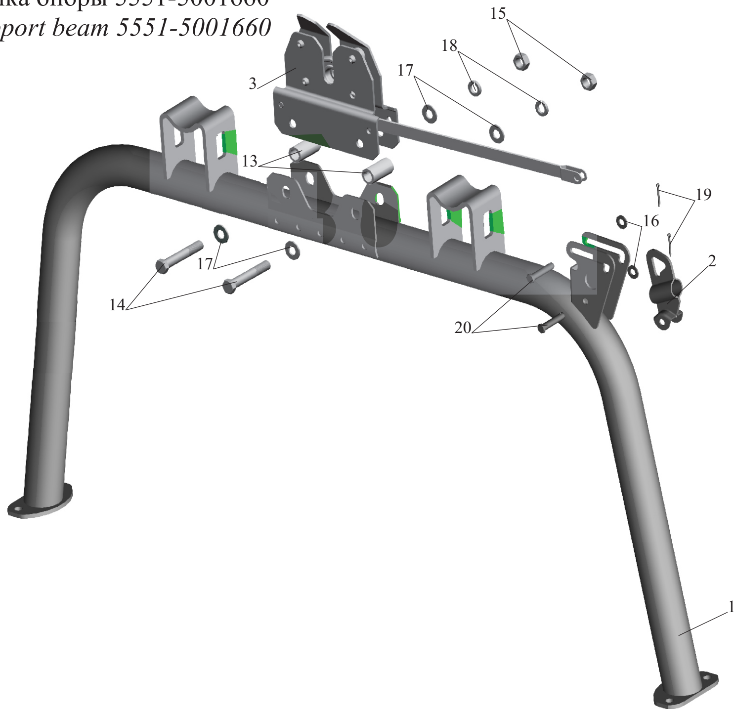
Рис. 174 Балка опоры 5551-5001660
