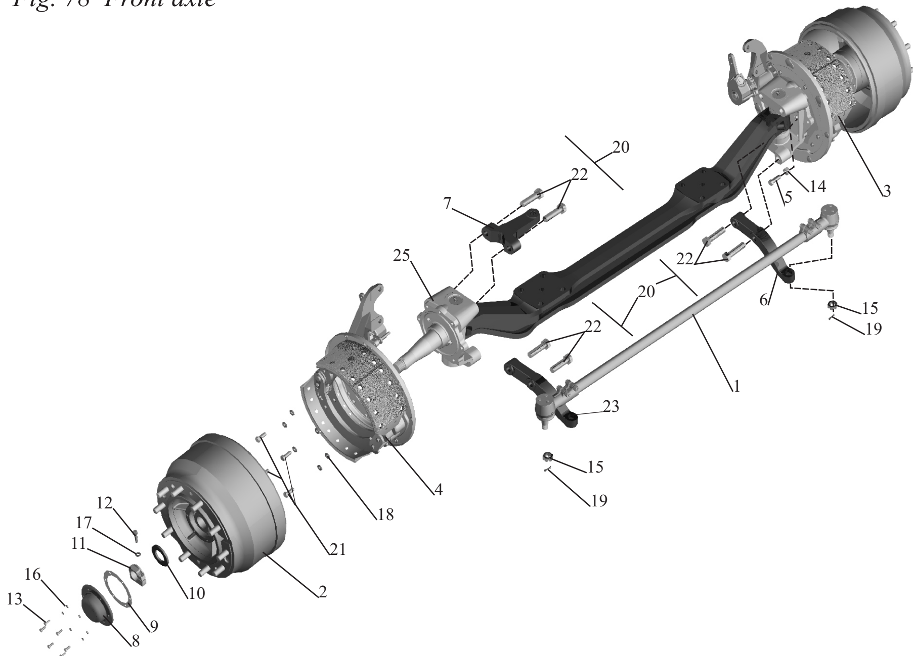
Рис. 78 Передняя ось Fig. 78 Front axle
