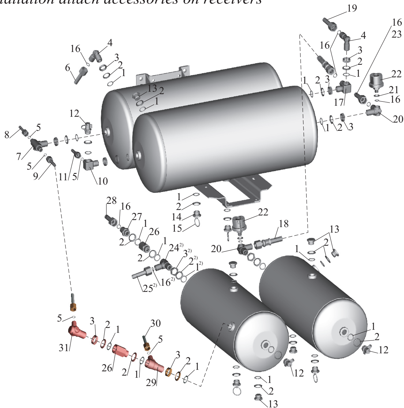
Рис. 105 Установка присоединительной арматуры на ресиверах Fig. 105 Installation attach accessories on receivers
