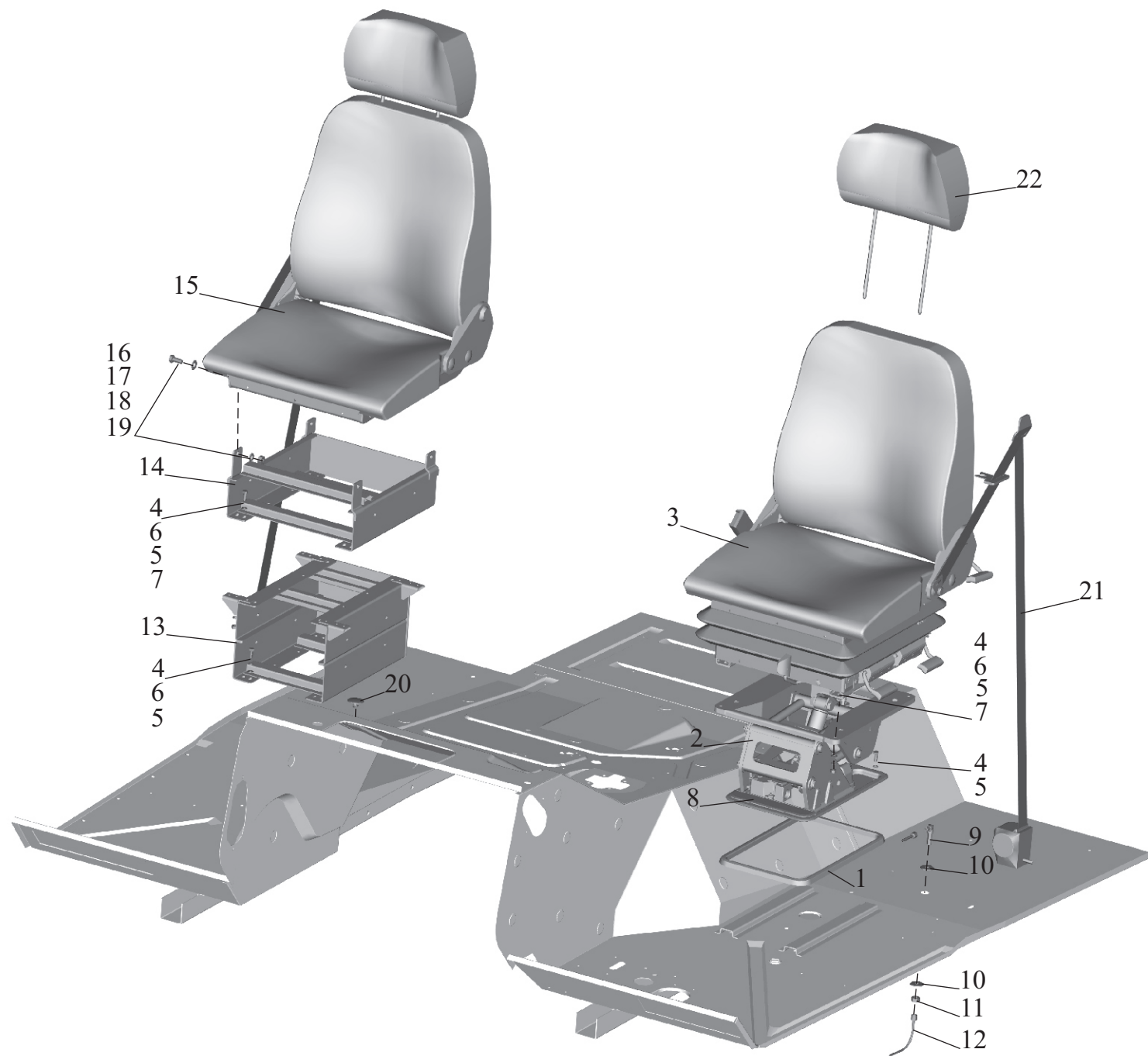
Рис. 191 Установка и пневмопитание сидений 5551-6800006-040 Fig. 191 Installation and pneumatic supply of seat 5551-6800006-040
