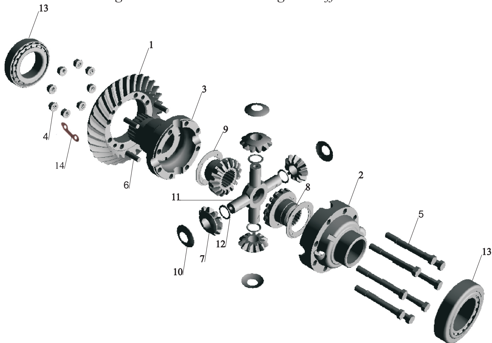
Рис. 46 Редуктор заднего моста. Дифференциал. Fig. 46 Rear axle reduction gear. Differential.
