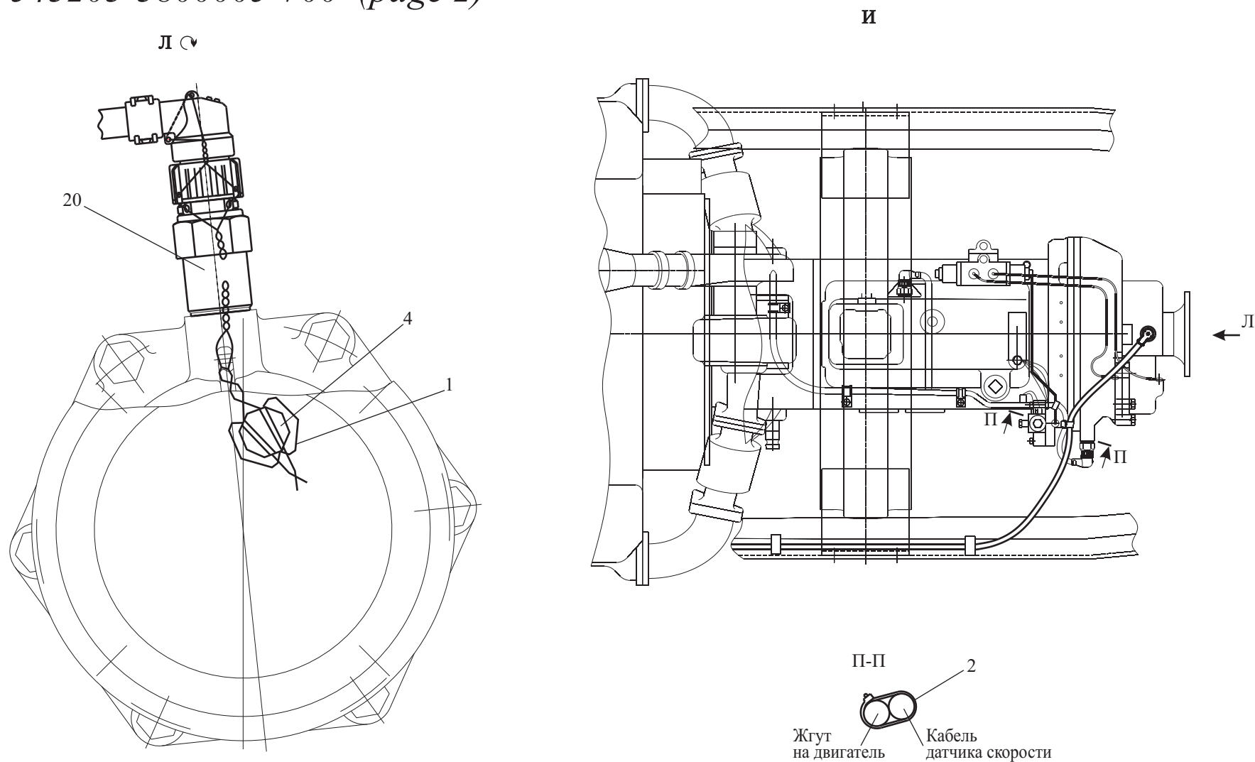
Рис. 143 Установка и пломбировка тахографа 543203-3800005, 543203-3800005-700 (лист 2) Fig. 143 Installation and identification seal of a tachograph 543203-3800005, 543203-3800005-700 (page 2)
