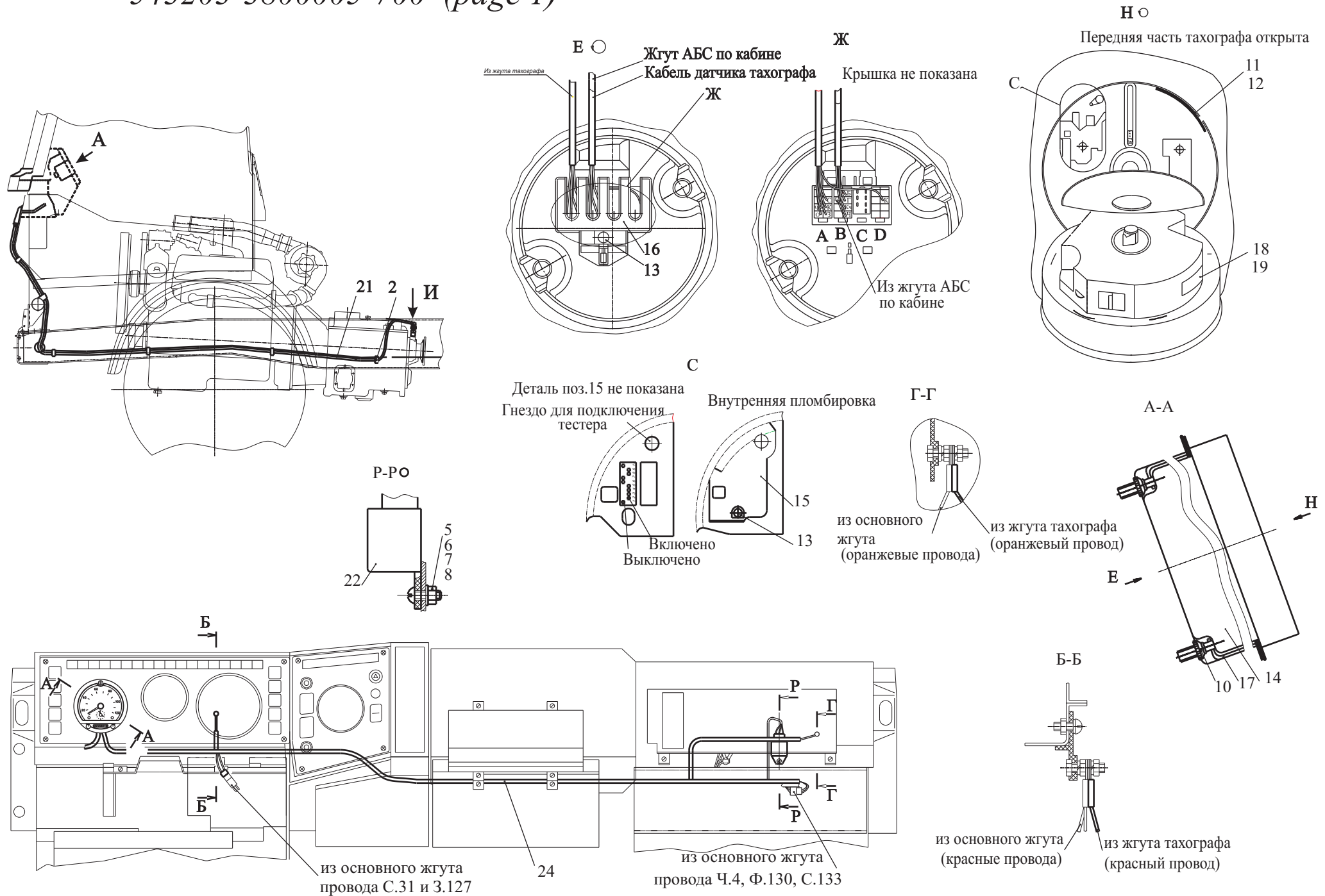
Рис. 143 Установка и пломбировка тахографа 543203-3800005, 543203-3800005-700 (лист 1) Fig. 143 Installation and identification seal of a tachograph 543203-3800005, 543203-3800005-700 (page 1)
