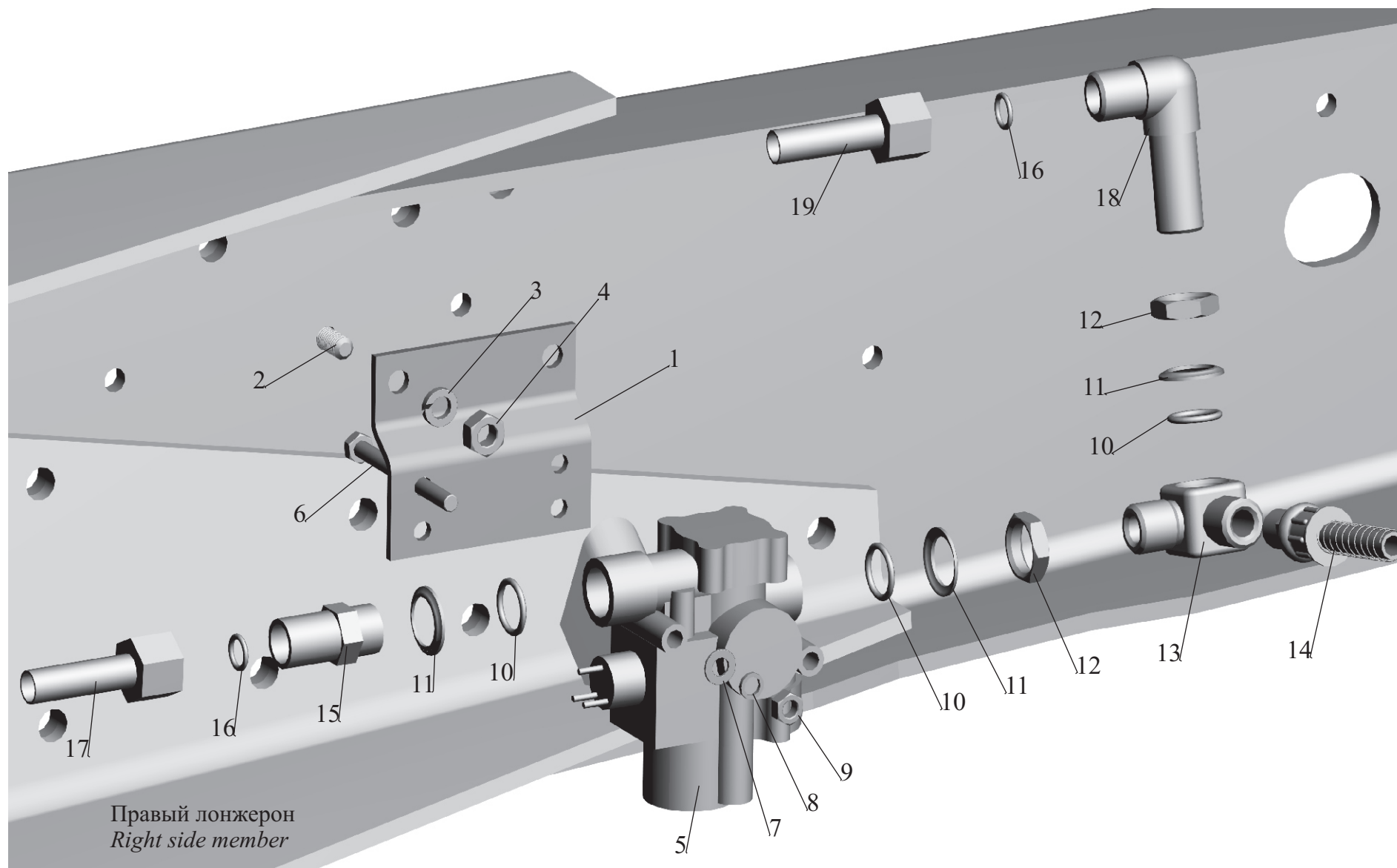
Рис. 126 Установка задних модуляторов и соединительной арматуры Fig. 126 Installation of rear modulators and attach accessories
