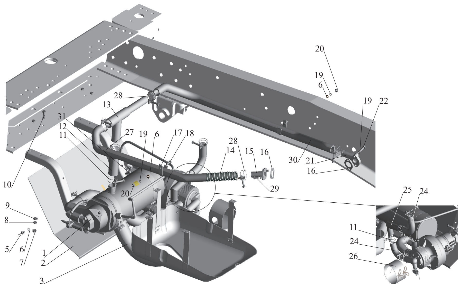
Рис. 5 Крепление предпускового подогревателя 642290-1015001 Fig. 5 Mounting of a prestarting heater 642290-1015001
