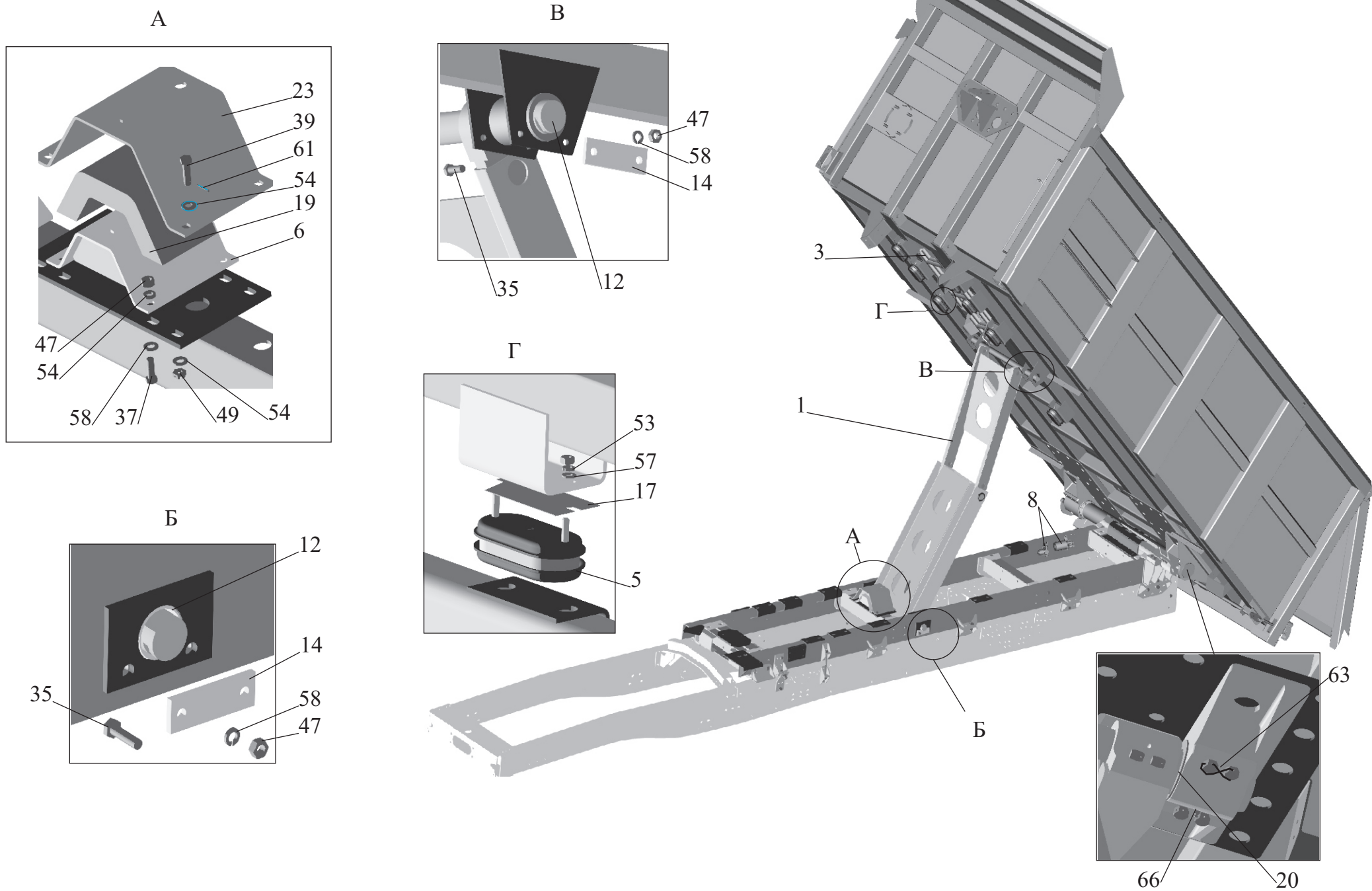
Рис. 216 Установка платформы V=12.5m^3 (лист 2) Fig. 216 Installation of platform V=12.5m^3 (page2)
