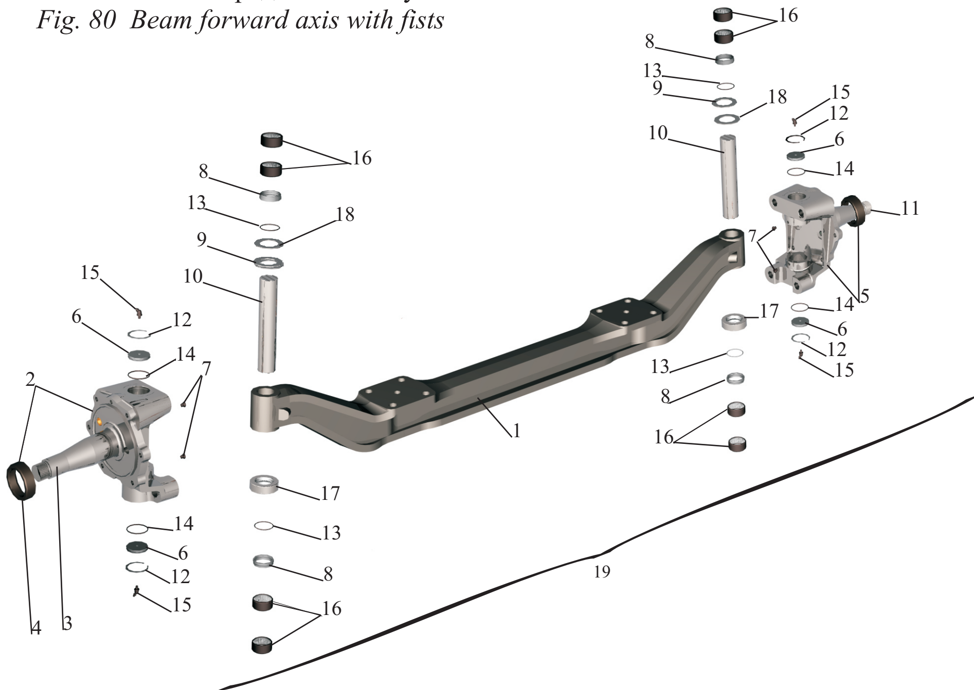
Рис. 80 Балка передней оси с кулаками
