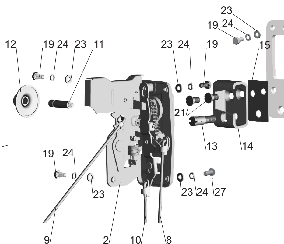
Рис. 185 Установка наружной ручки и замка двери (входит в 64221-6100010-10)
