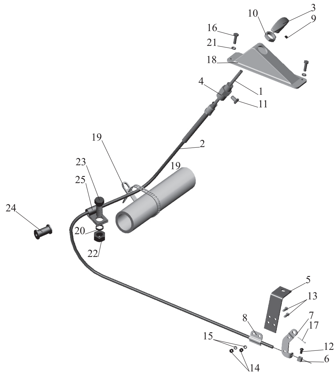
Рис. 12 Привод останова двигателя 543208-1115002-010 Fig. 12 Engine shut-off device 543208-1115002-010
