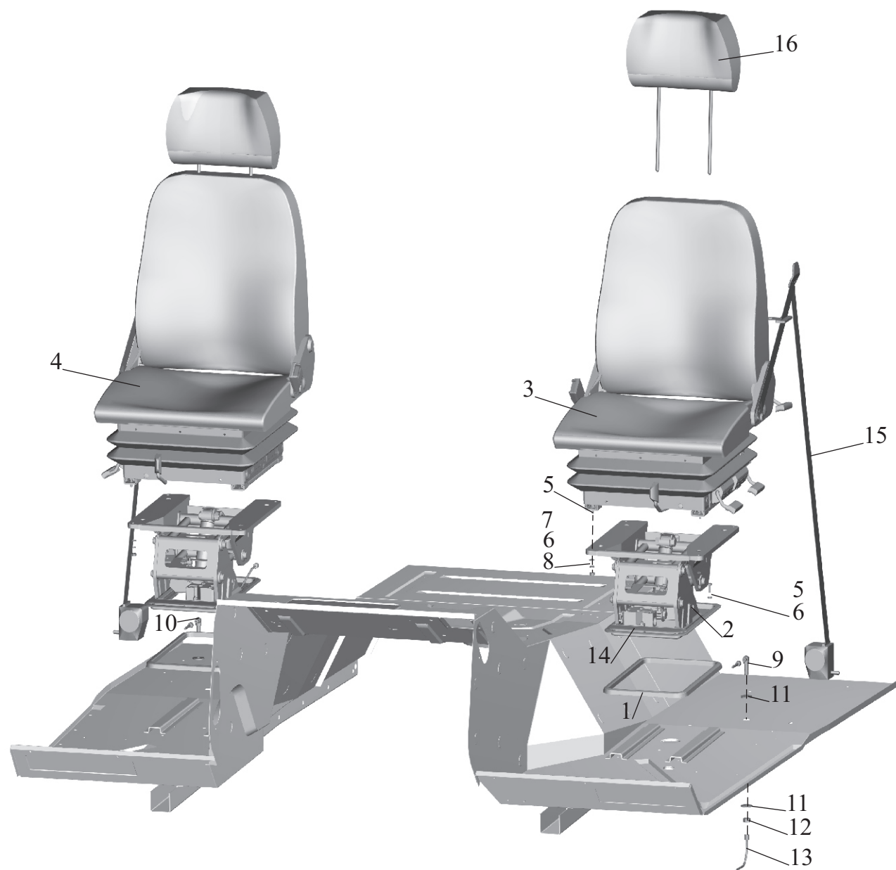
Рис. 189 Установка и пневмопитание сидений 64221-6800006-10 Fig. 189 Installation and pneumatic supply of seat 64221-6800006-10
