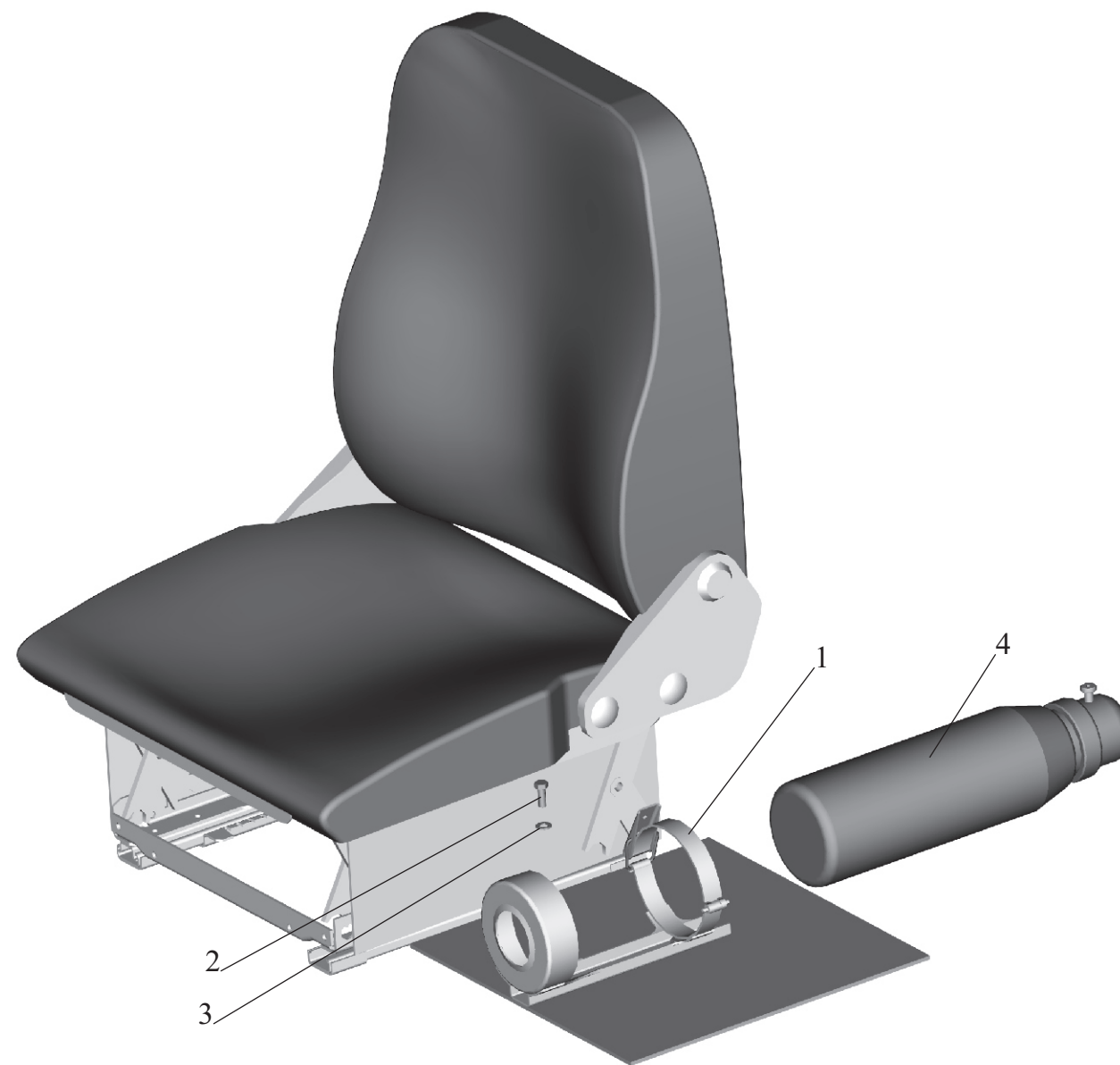
Рис. 171 Установка огнетушителя 5516-3910040 Fig. 171 Installation fire extinguisher 5516-3910040
