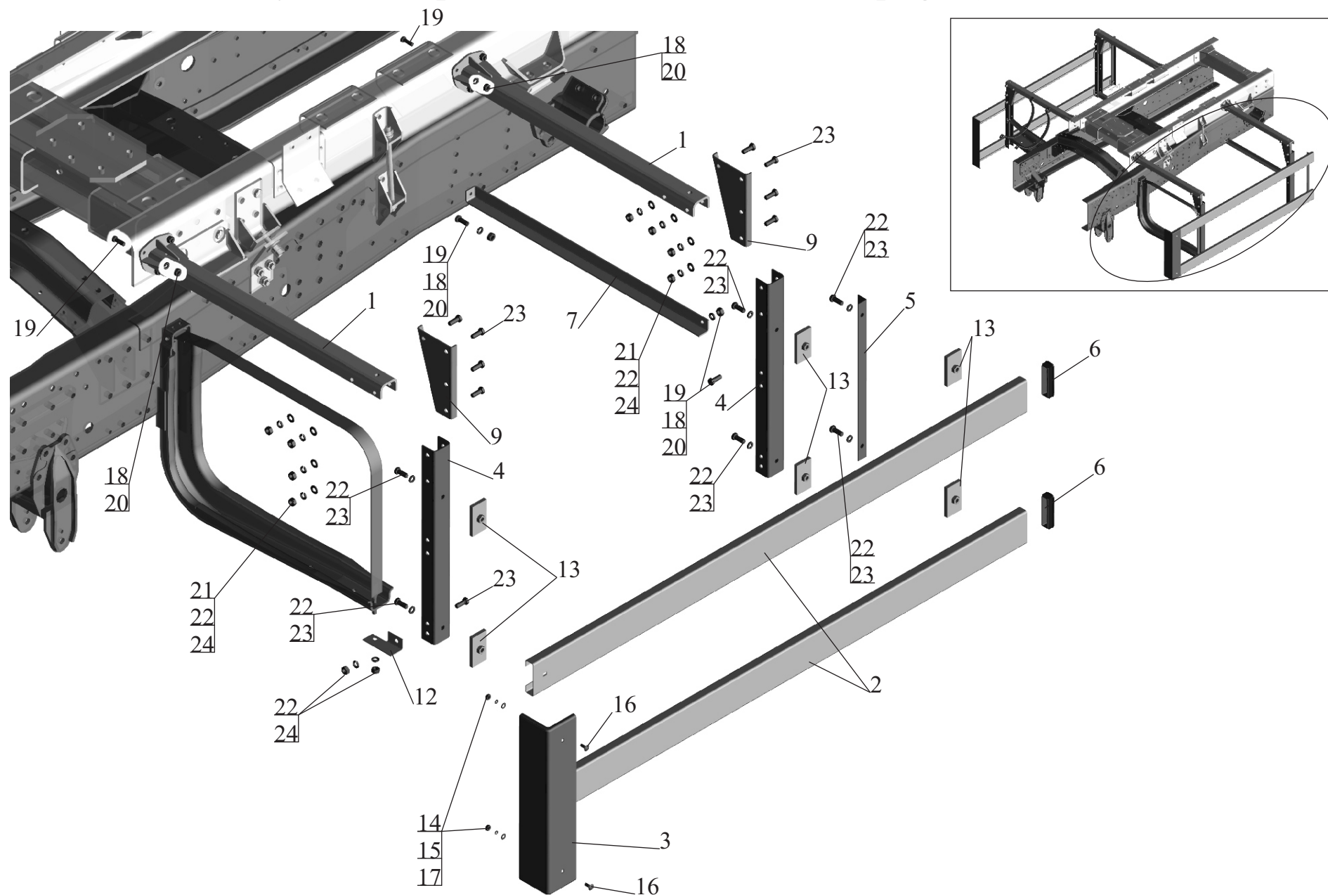
Рис. 71 Установка бокового ограждения 551605-2800040 (лист 2) Fig. 71 Installation of a lateral protection 551605-2800040 (page 2)
