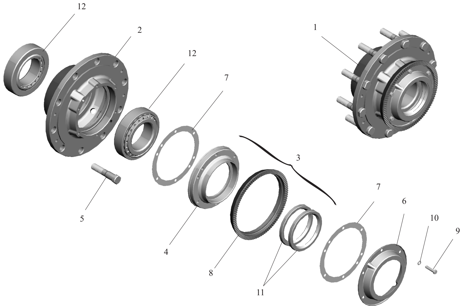
Рис. 49 Ступица заднего моста. Fig. 49 Rear axle hub.
