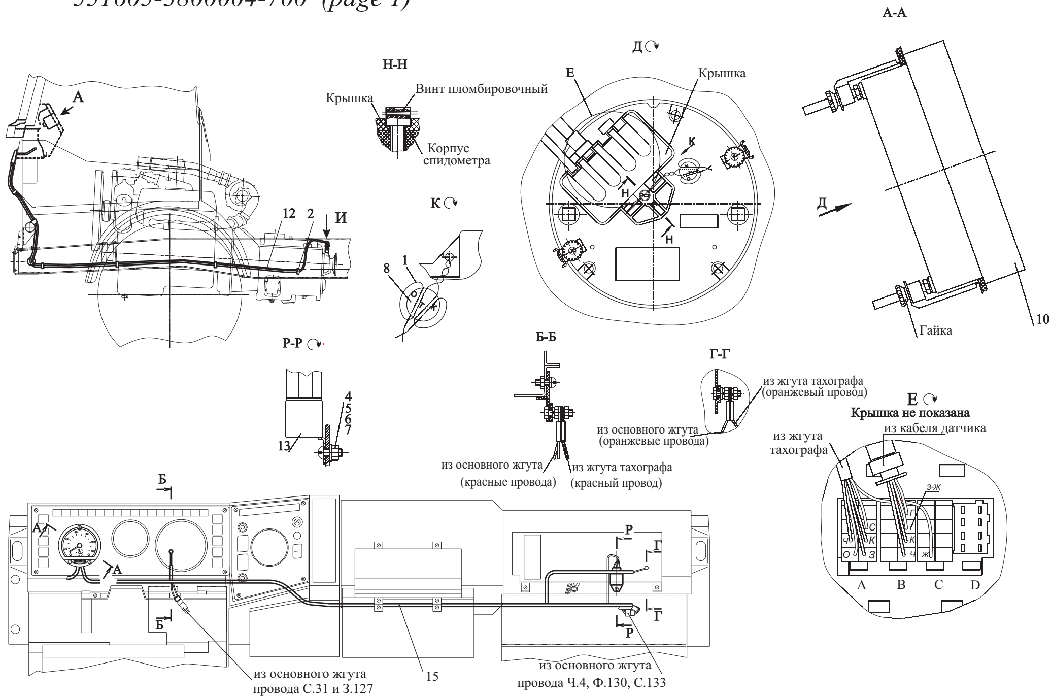
Рис. 142 Установка и пломбировка спидометра 551605-3800004, 551605-3800004-700 (лист 1) Fig. 142 Installation and identification seal of a speedometer 551605-3800004 551605-3800004-700 (page 1)
