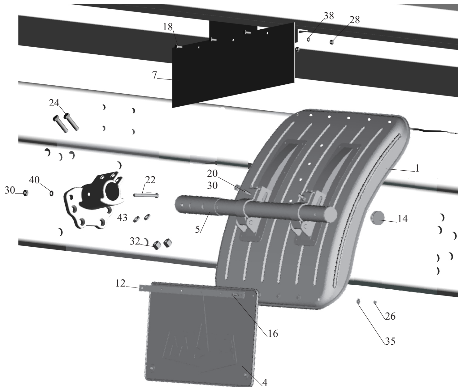
Рис. 228 Установка крыльев 5516-8500048-10 Fig. 228 The fenders installation 5516-8500048-10
