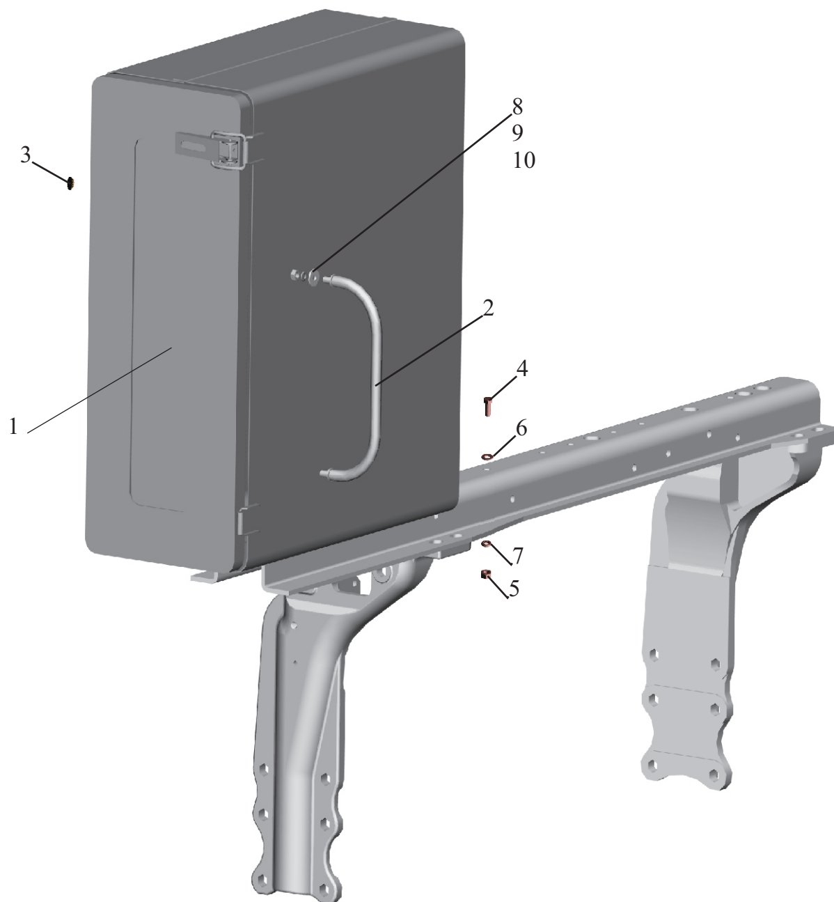
Рис. 226 Установка инструментального ящика 64229-8500009-10 Fig. 226 The tools box installation 64229-8500009-10
