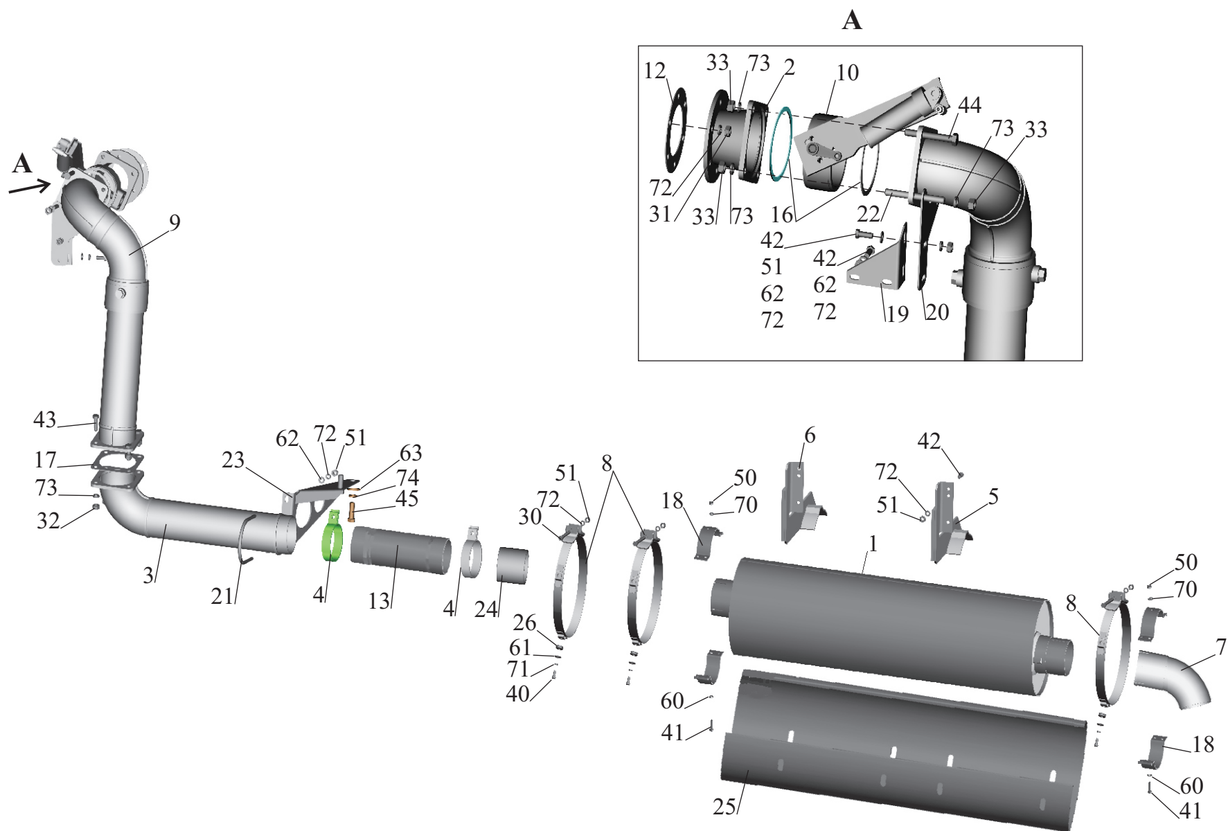
Рис. 22 Установка системы выпуска газов 551605-1200001-070 (-170) Fig. 22 Installation of exhaust system of gases 551605-1200001-070 (-170)
