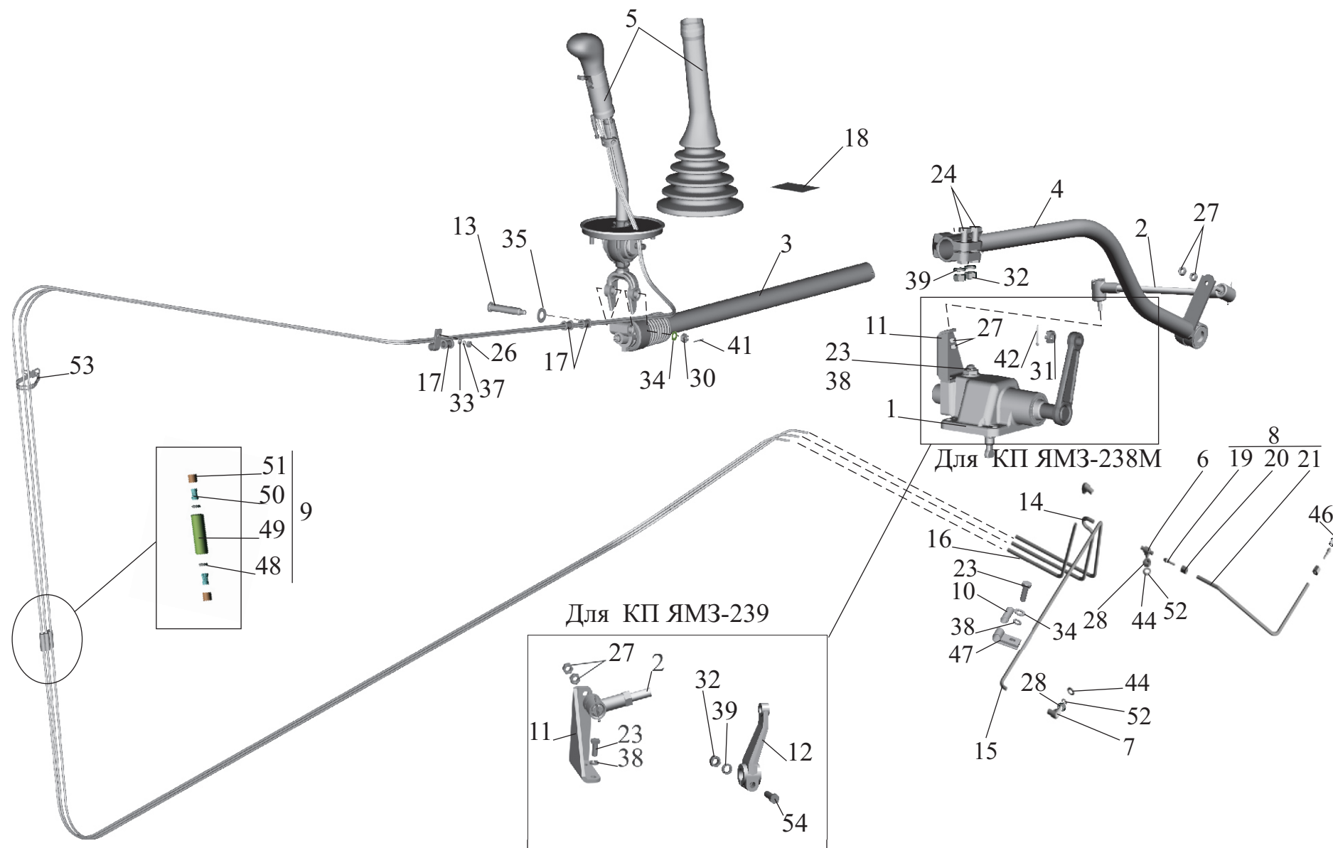
Рис. 31 Установка привода управления коробкой передач 642205-1700002, 642208-1700002 Fig. 31 Installation of drive of control of gear box 642205-1700002, 642208-1700002
