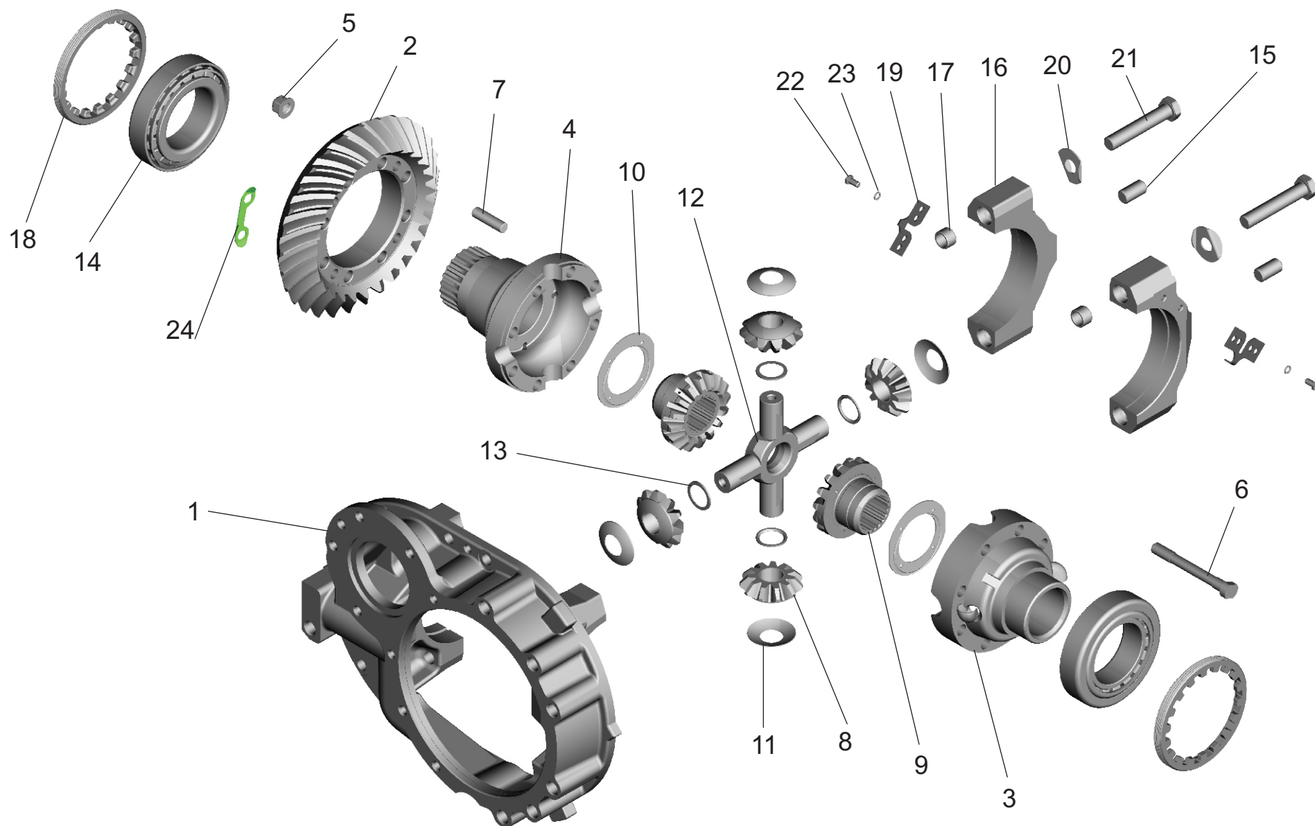
Рис. 57 Редуктор среднего моста. Дифференциал с картером редуктора Fig. 57 Intermediate axle reduction gear. Differential with gear housing
