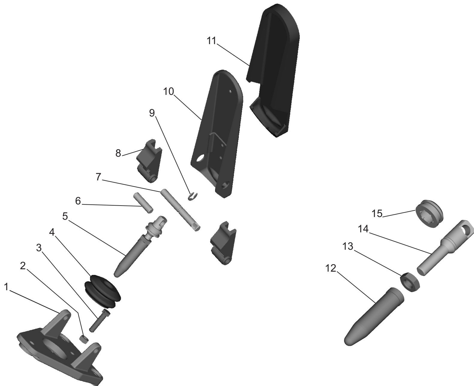
Рис. 107 Педаль привода тормозного крана Fig. 107 Pedal Brake Valve
