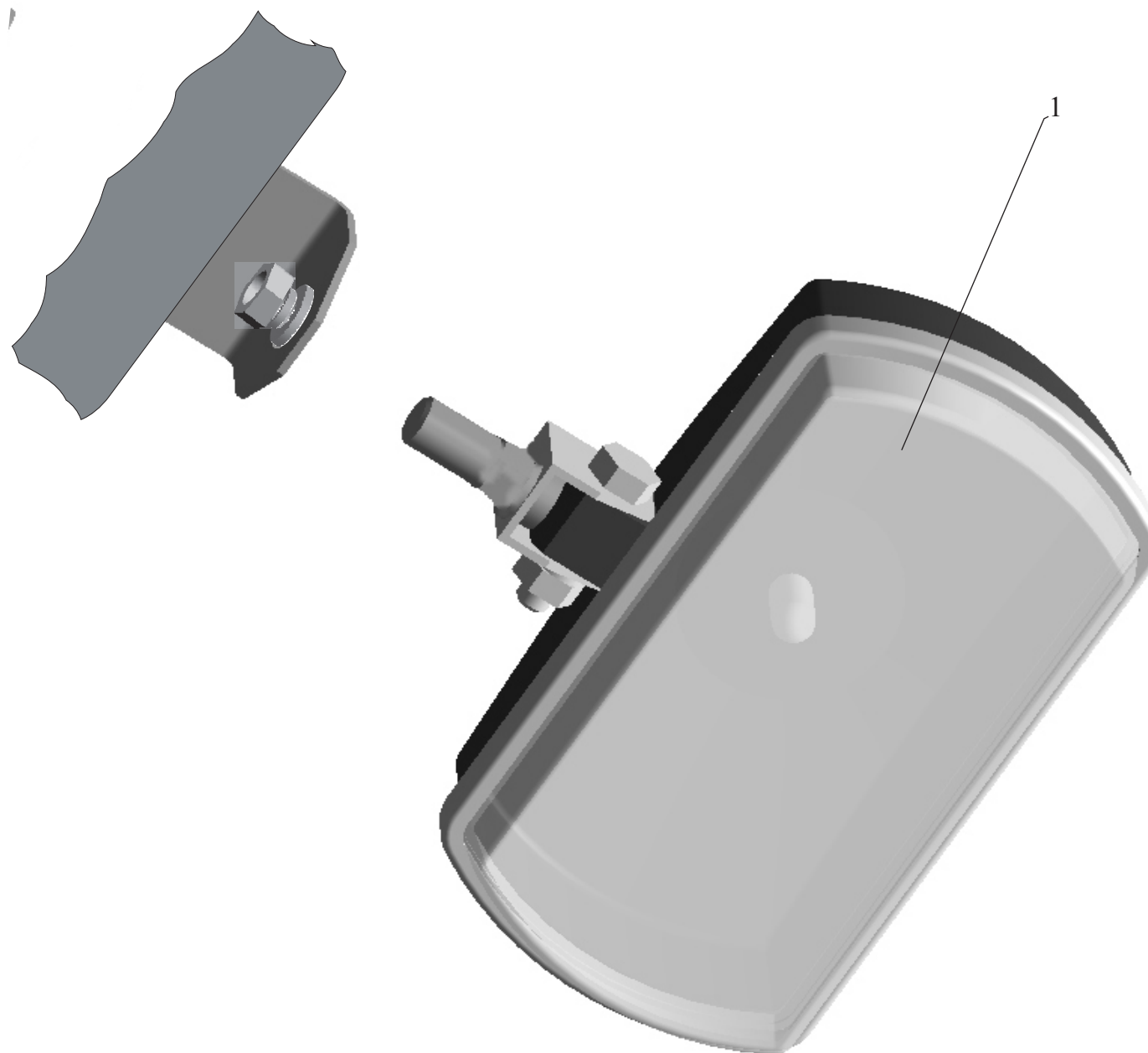
Рис. 147 Установка противотуманной фары Fig. 147 Installing of fog Light
