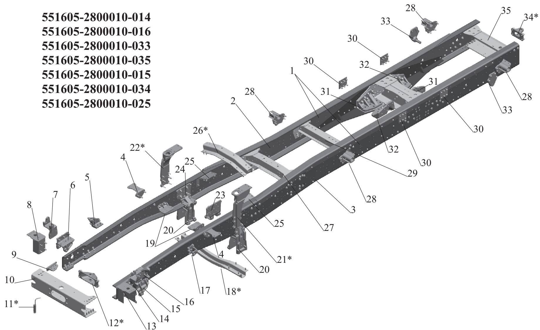
Рис. 66 Рама (лист 1) Fig. 66 Frame (page 1)
