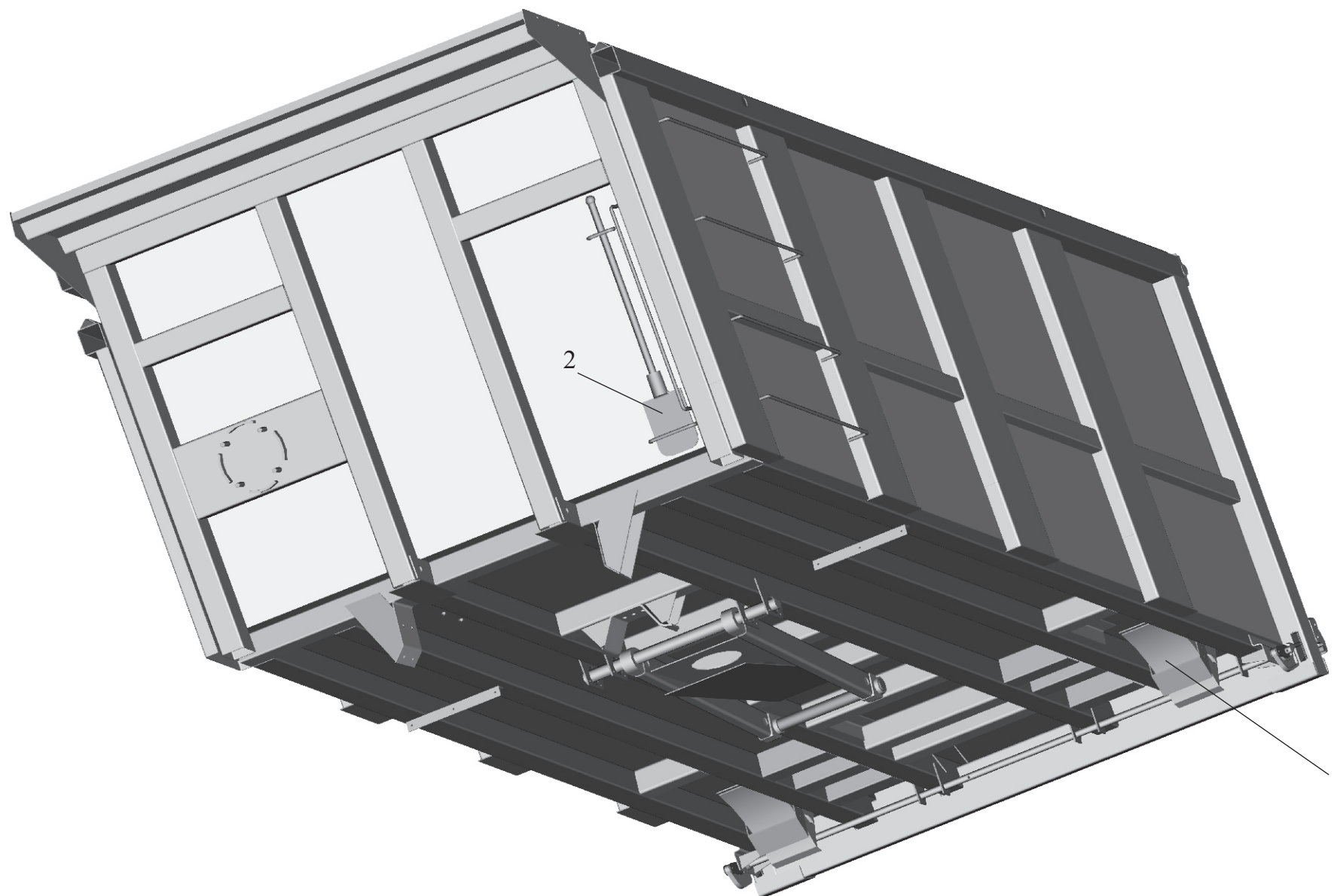
Рис. 168 Установка дополнительных принадлежностей 5516-3900011 Fig. 168 Installation of additional accessories 5516-3900011
