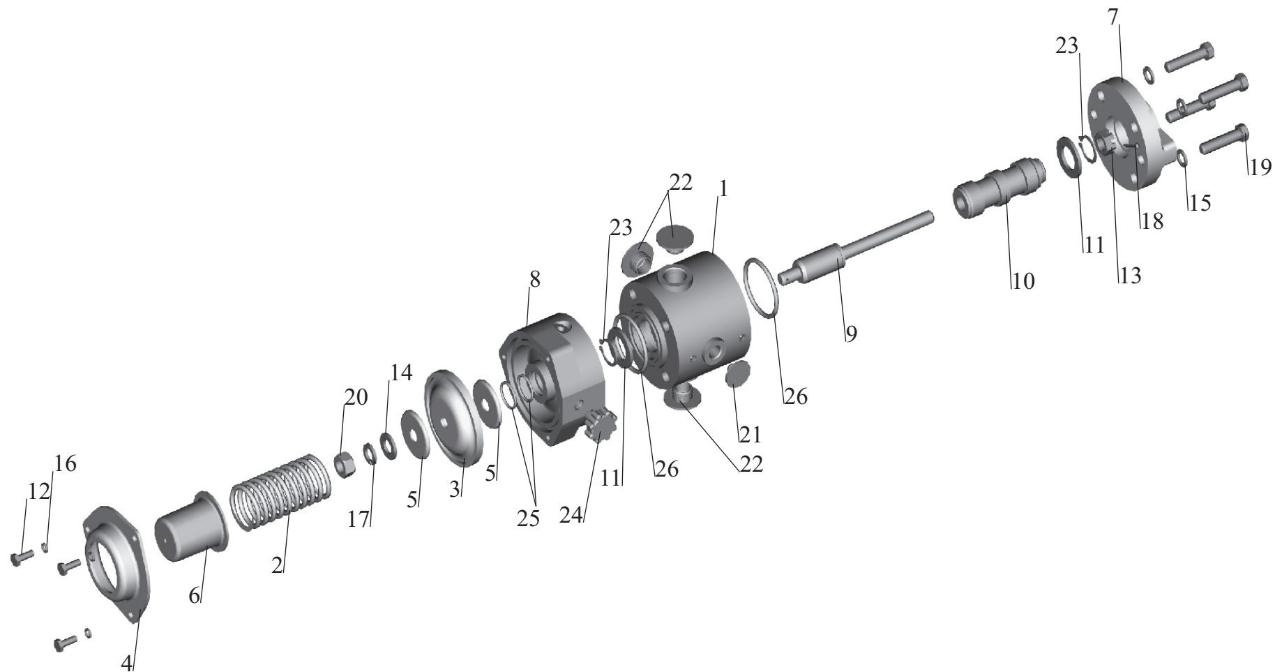
Fig. 242 Valve 555102-8607300
