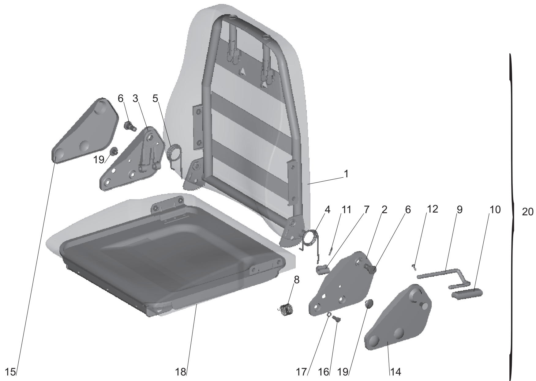
Рис. 193 Подушка и спинка сиденья 6430-6800012, 6430-6810012* Fig. 193 Pad and seat back 6430-6800012, 6430-6810012*
