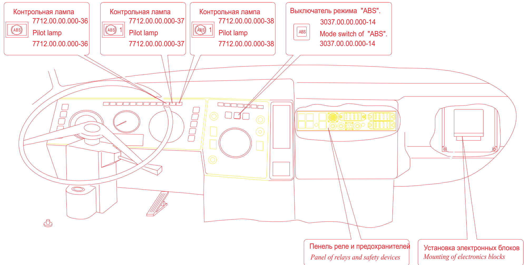
Рис. 163 Расположение элементов электронных систем в кабине автомобиля МАЗ-551605 с прицепом Fig. 163 Elements arrangement of electronical systems in vehicle cabin of MAZ - 551605 with the trailer
