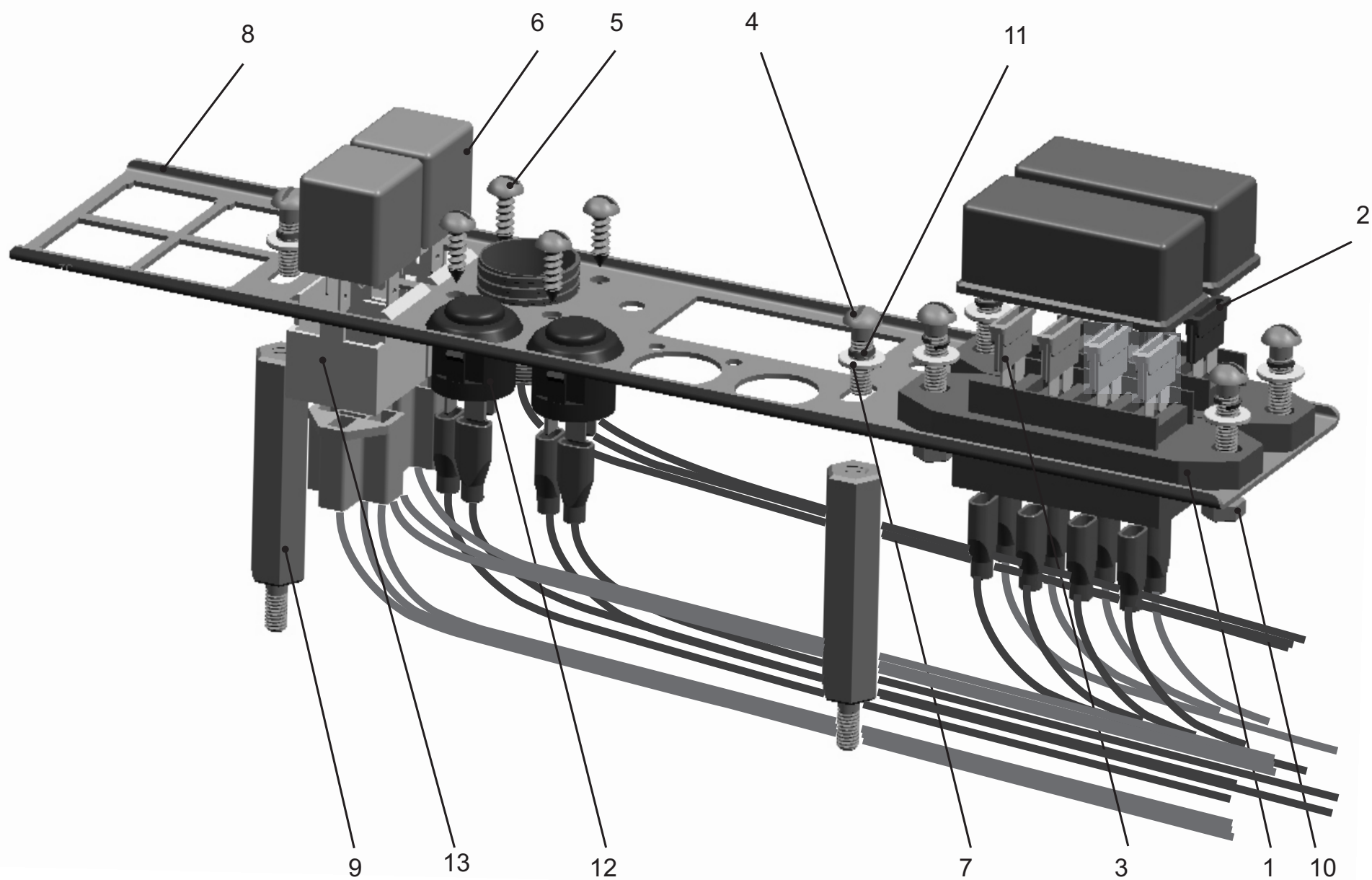
Рис. 167 Панель реле и предохранителей автомобиля Fig. 167 Panel of relays and safety devices vehicles
