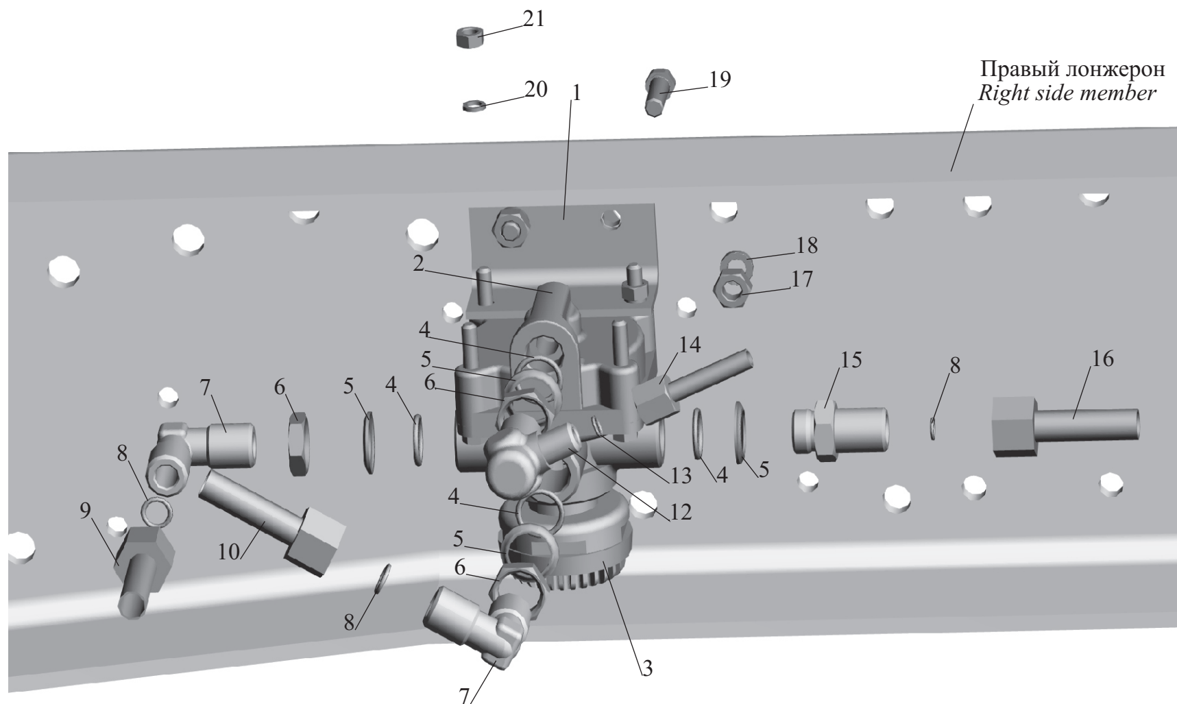
Рис. 111 Установка ускорительного клапана 543403-3518004-010 Fig. 111 Installation of relay valve 543403-3518004-010
