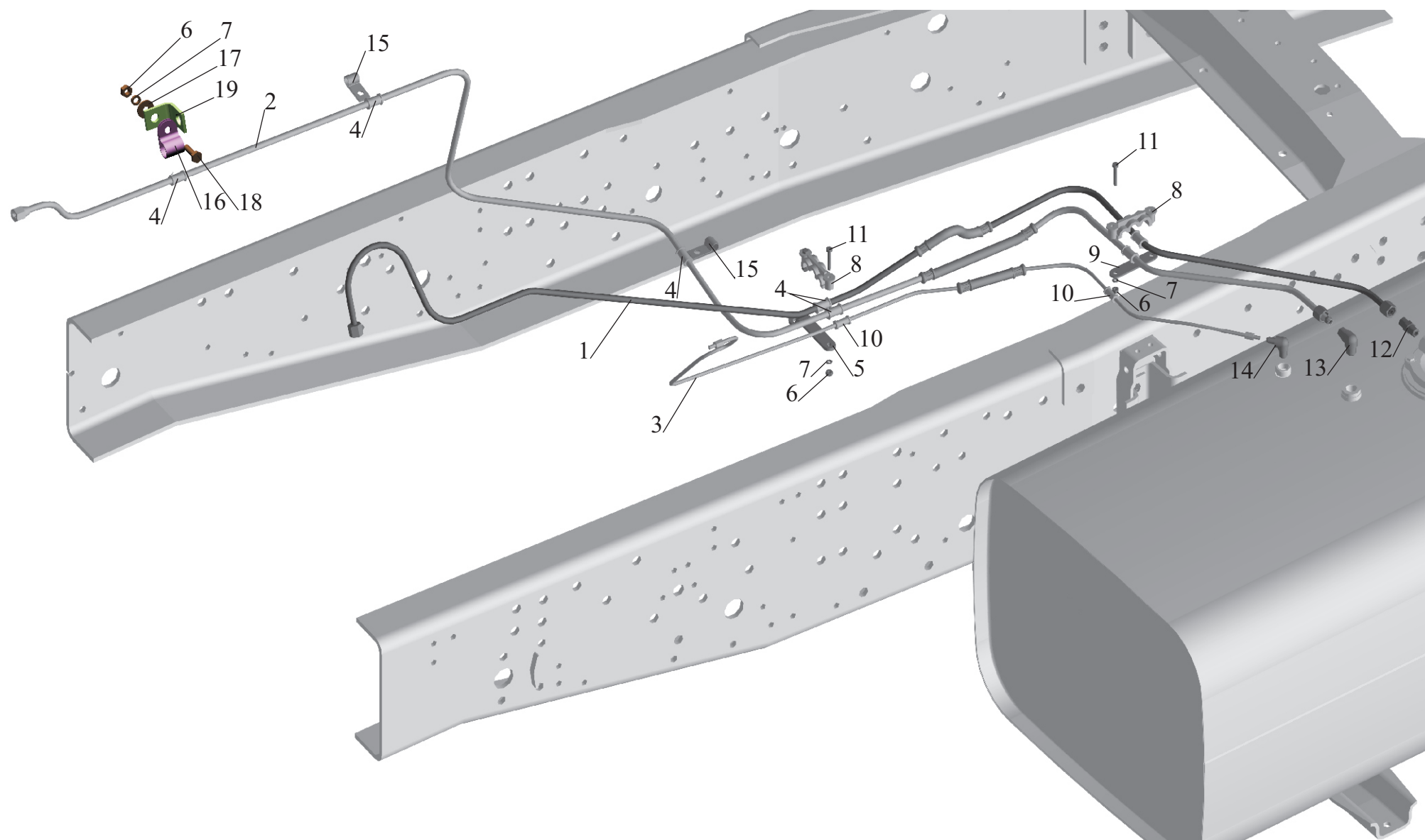
Рис. 14 Установка топливopроводов (без подогревателя) Fig. 14 Installation of fuel lines (without heater)
