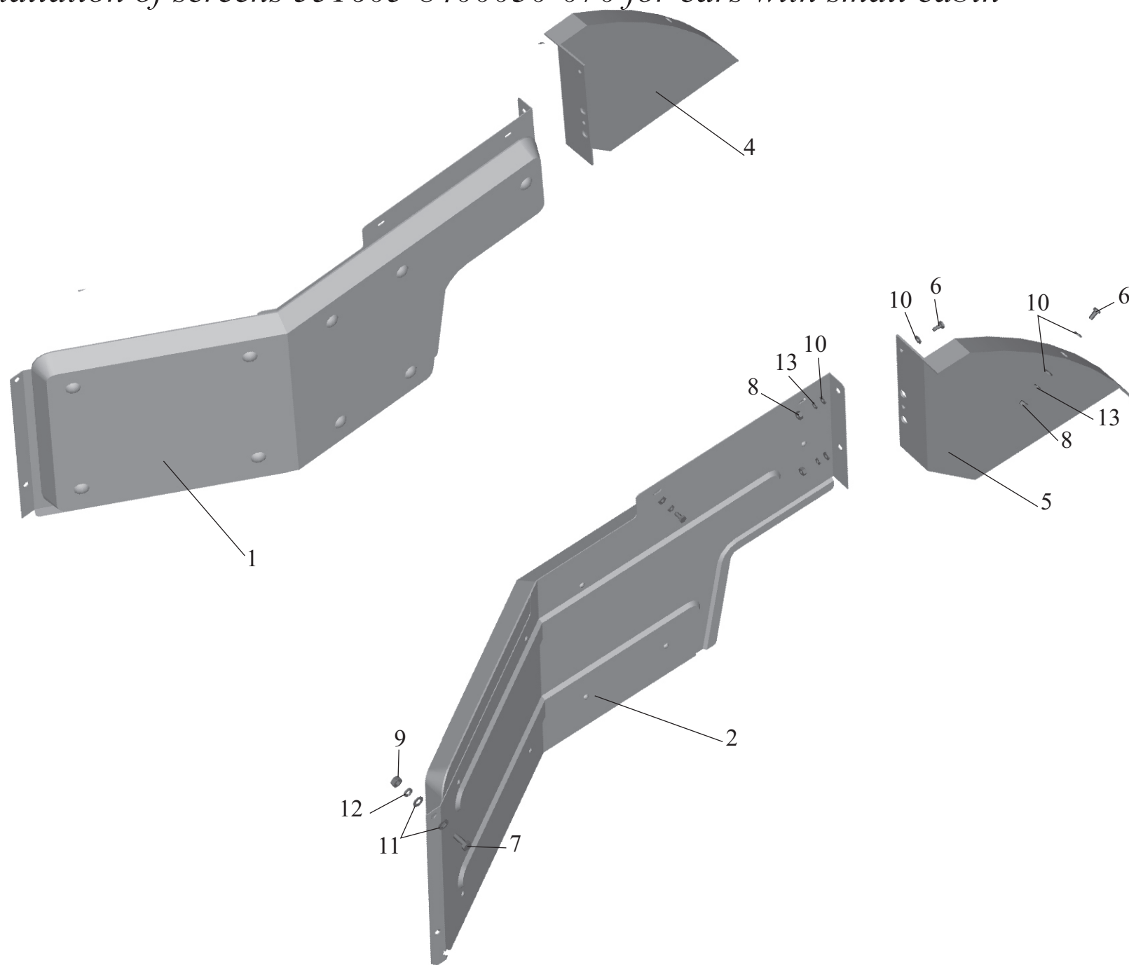
Рис. 209 Установка экранов 551605-8400030-070 для автомобилей с малой кабиной Fig. 209 Installation of screens 551605-8400030-070 for cars with small cabin
