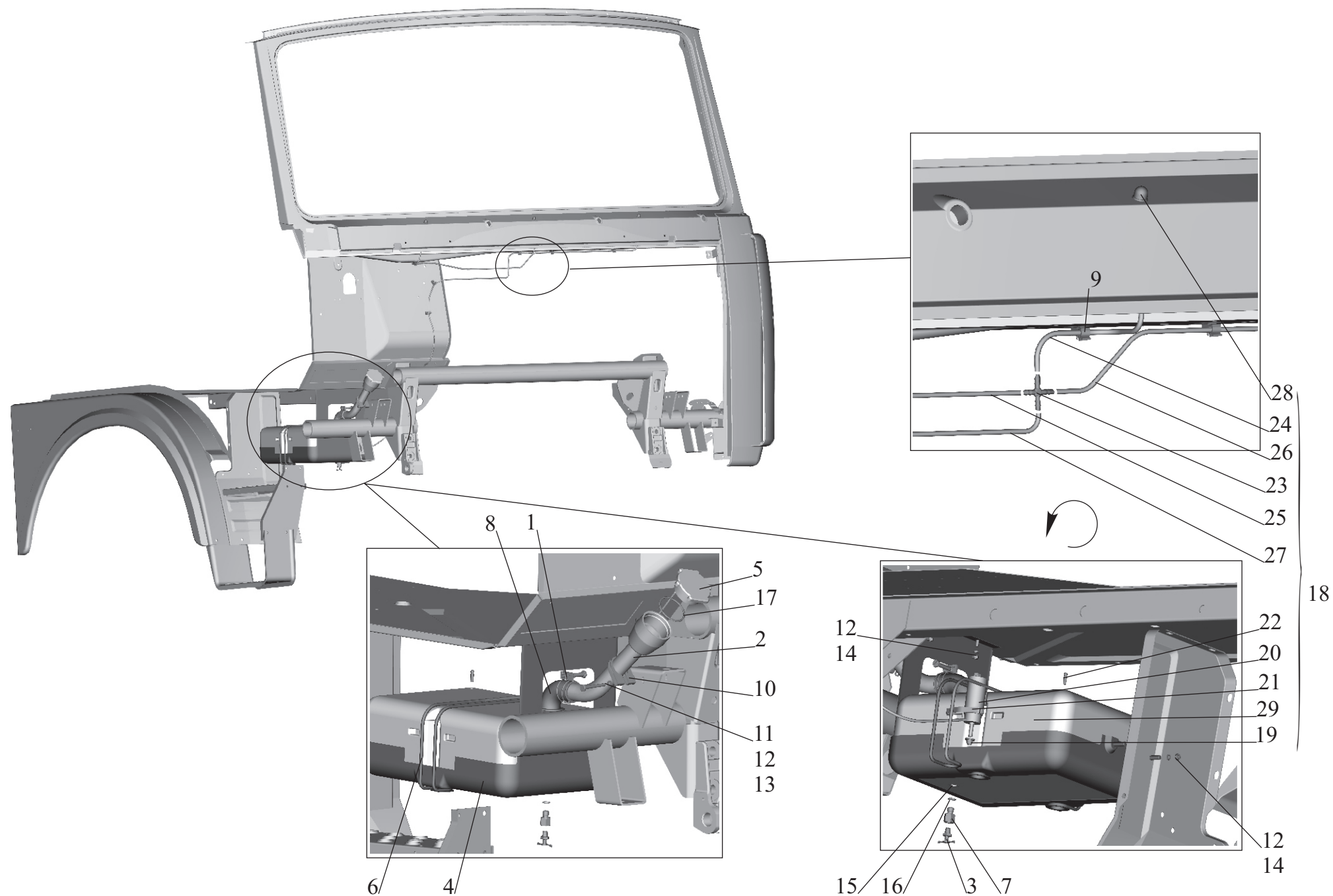
Рис. 181 Установка омывателя 64221-5200008-01 Fig. 181 Installation of washer 64221-5200008-01
