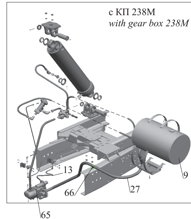
Рис. 233 Установка гидрооборудования Fig. 233 Installation of hydroequipment
