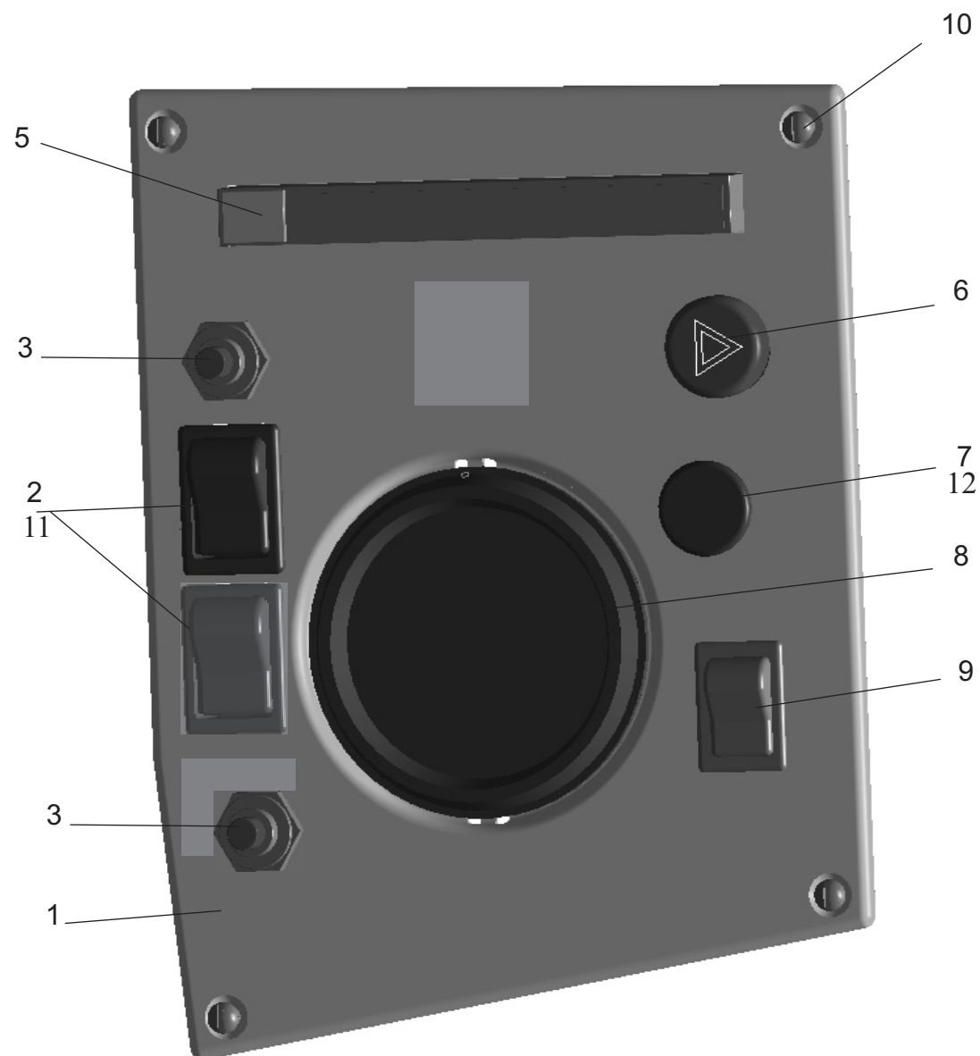
Рис. 139 Установка дополнительного щитка приборов 64229-3805012 Fig. 139 Installation of additional control panel 64229-3805012
