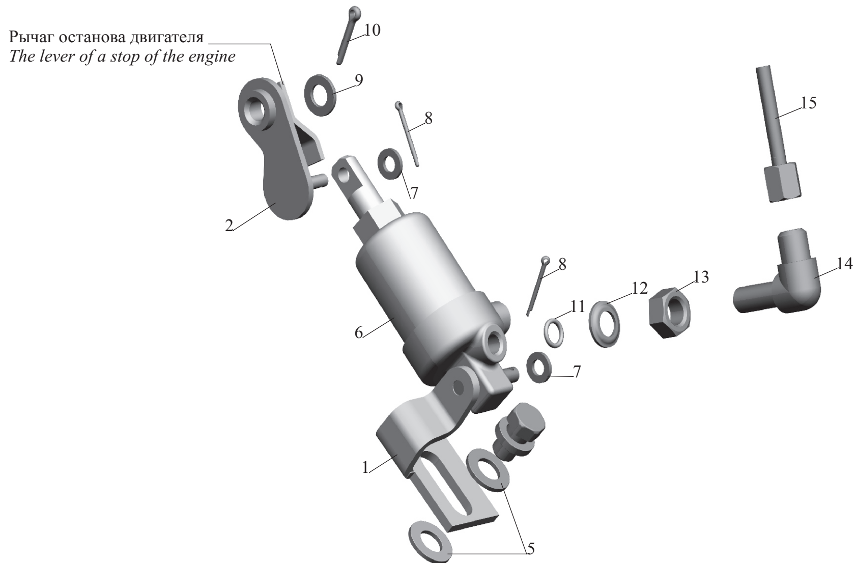
Рис. 123 Цилиндр останова двигателя 642208-3570004 Fig. 123 The cylinder of a stop of the engine 642208-3570004
