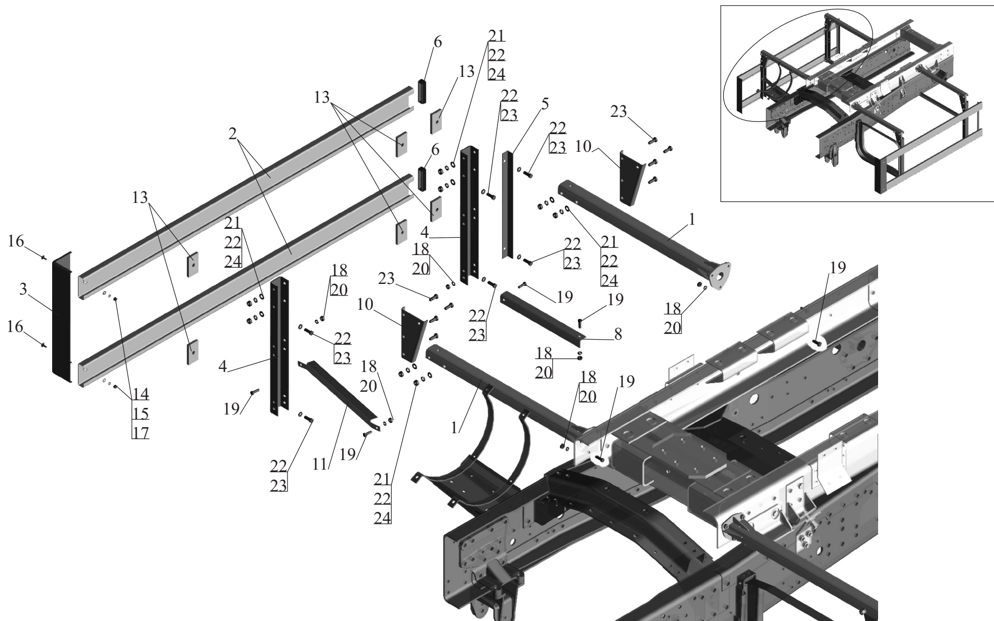
Рис. 71 Установка бокового ограждения 551605-2800040 (лист 1) Fig. 71 Installation of a lateral protection 551605-2800040 (page 1)
