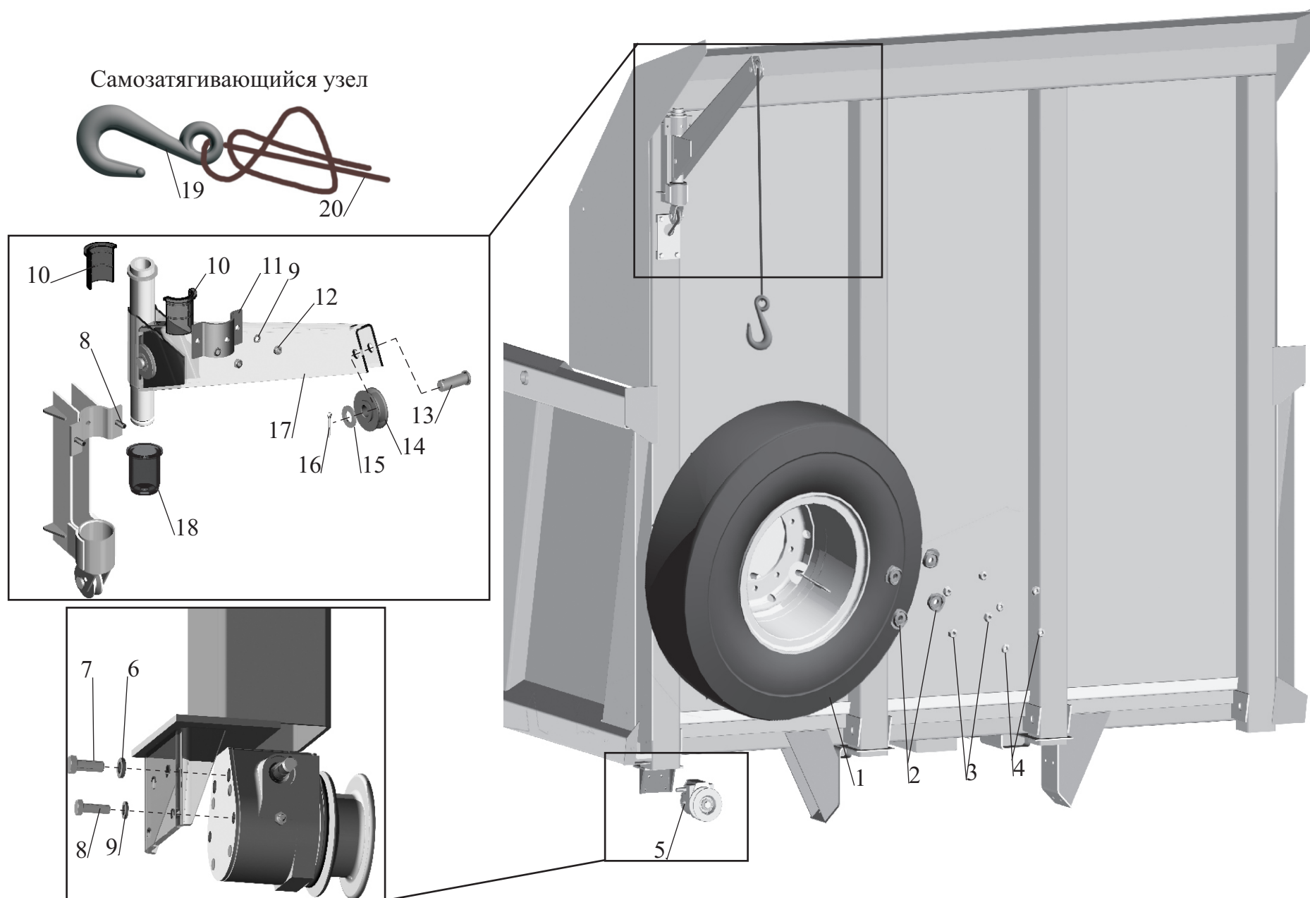
Рис. 85 Установка запасного колеса 551605-3100001-010, 551605-3100001-710 Fig. 85 Truck tractor spare wheel carrier 551605-3100001-010, 551605-3100001-710
