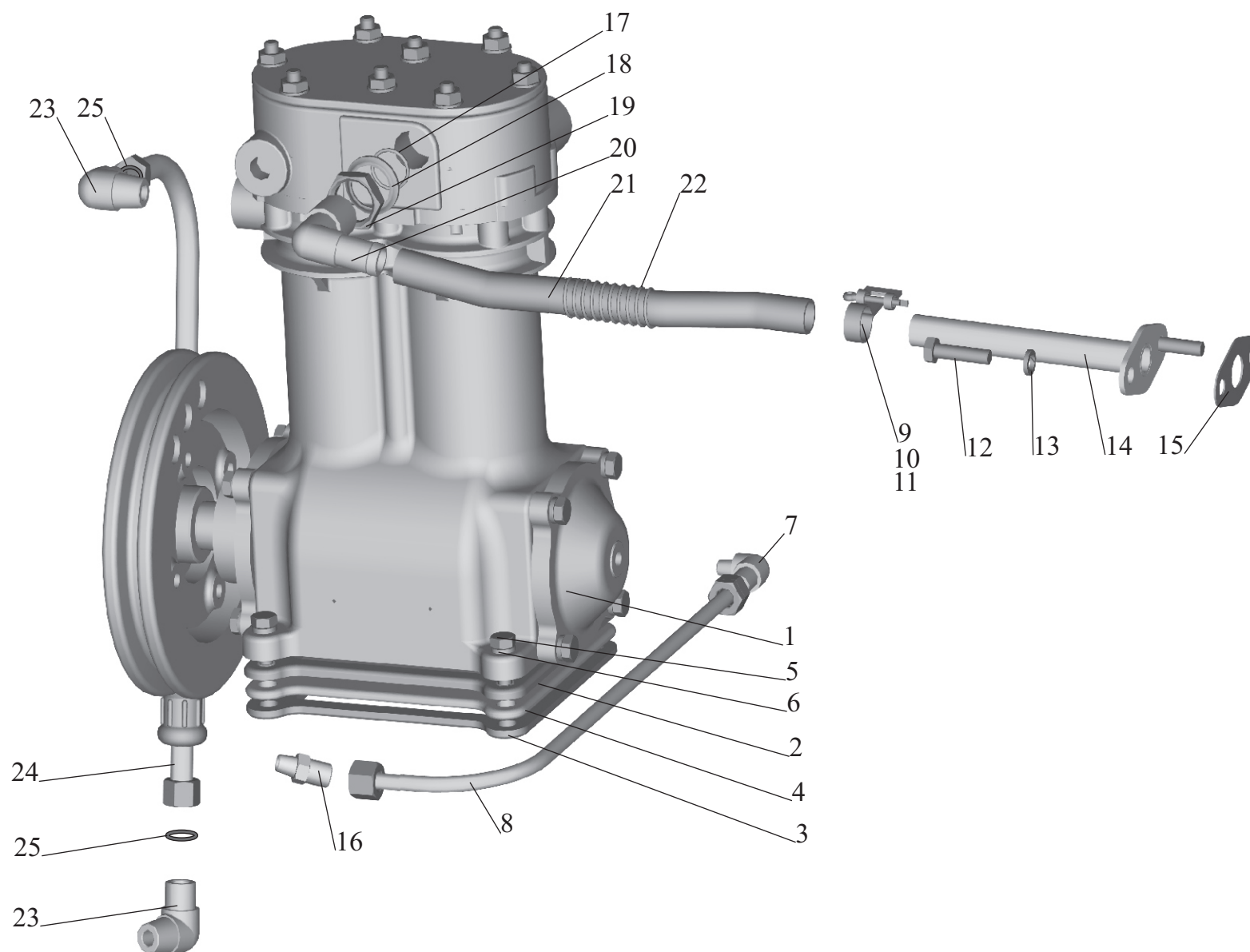
Рис. 102 Установка пневмокомпрессора 642208-3500014 (-700) Fig. 102 Installation of pneumatic compressor 642208-3500014 (-700)
