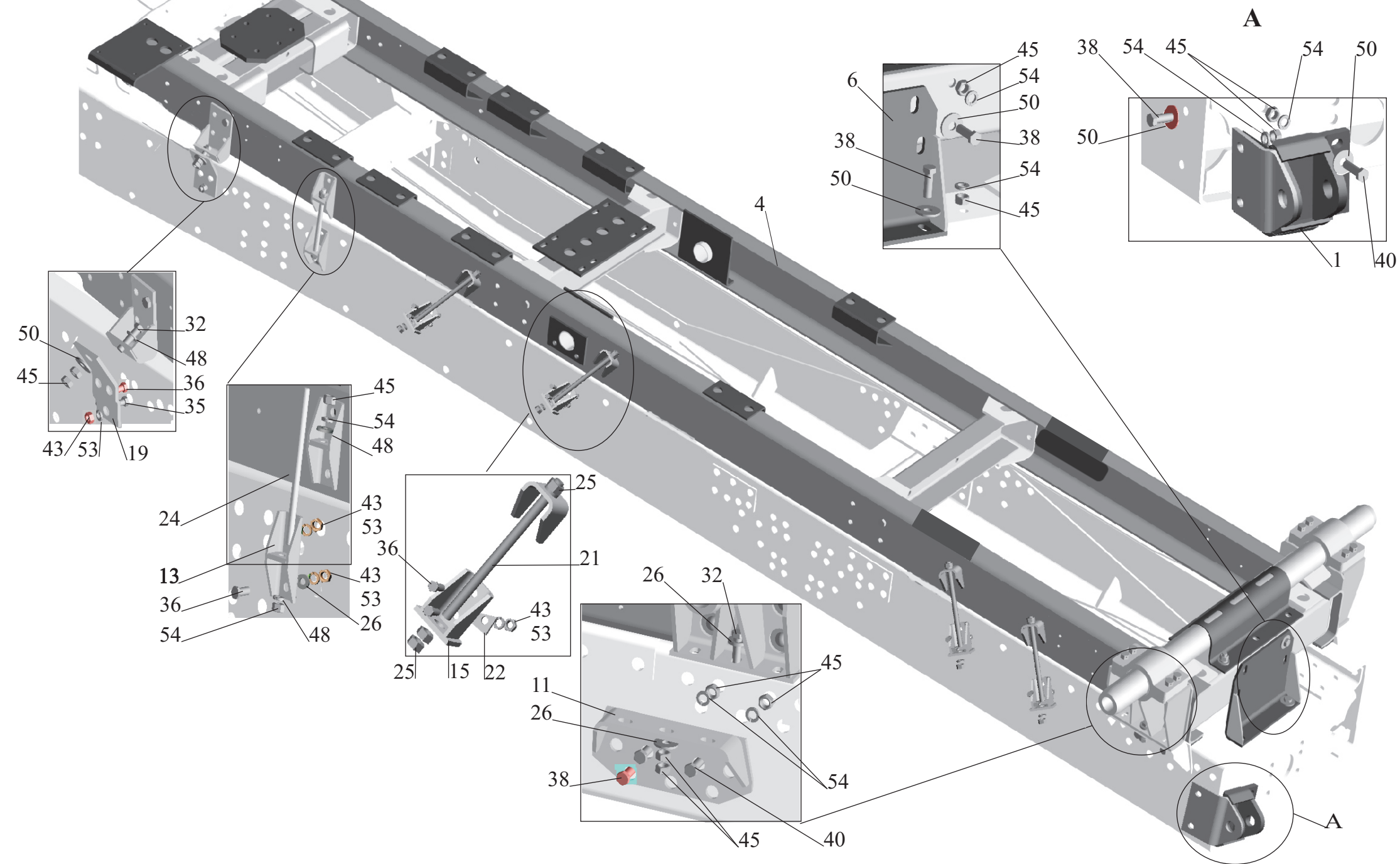
Рис. 231 Установка надрамника 5516-8600002-030 Fig. 231 Installation above frame 5516-8600002-030
