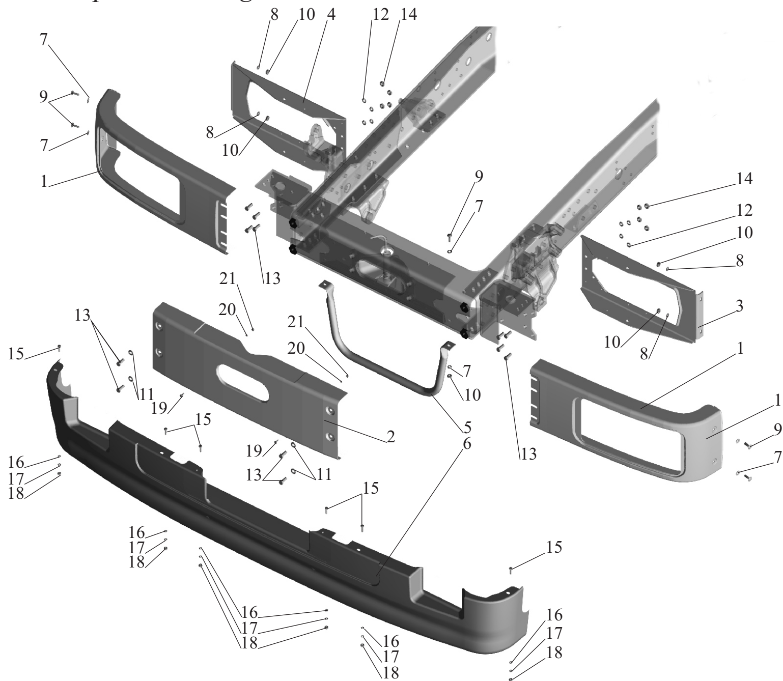
Рис. 67 Крепление бампера Fig. 67 Bumper mounthing on trucks
