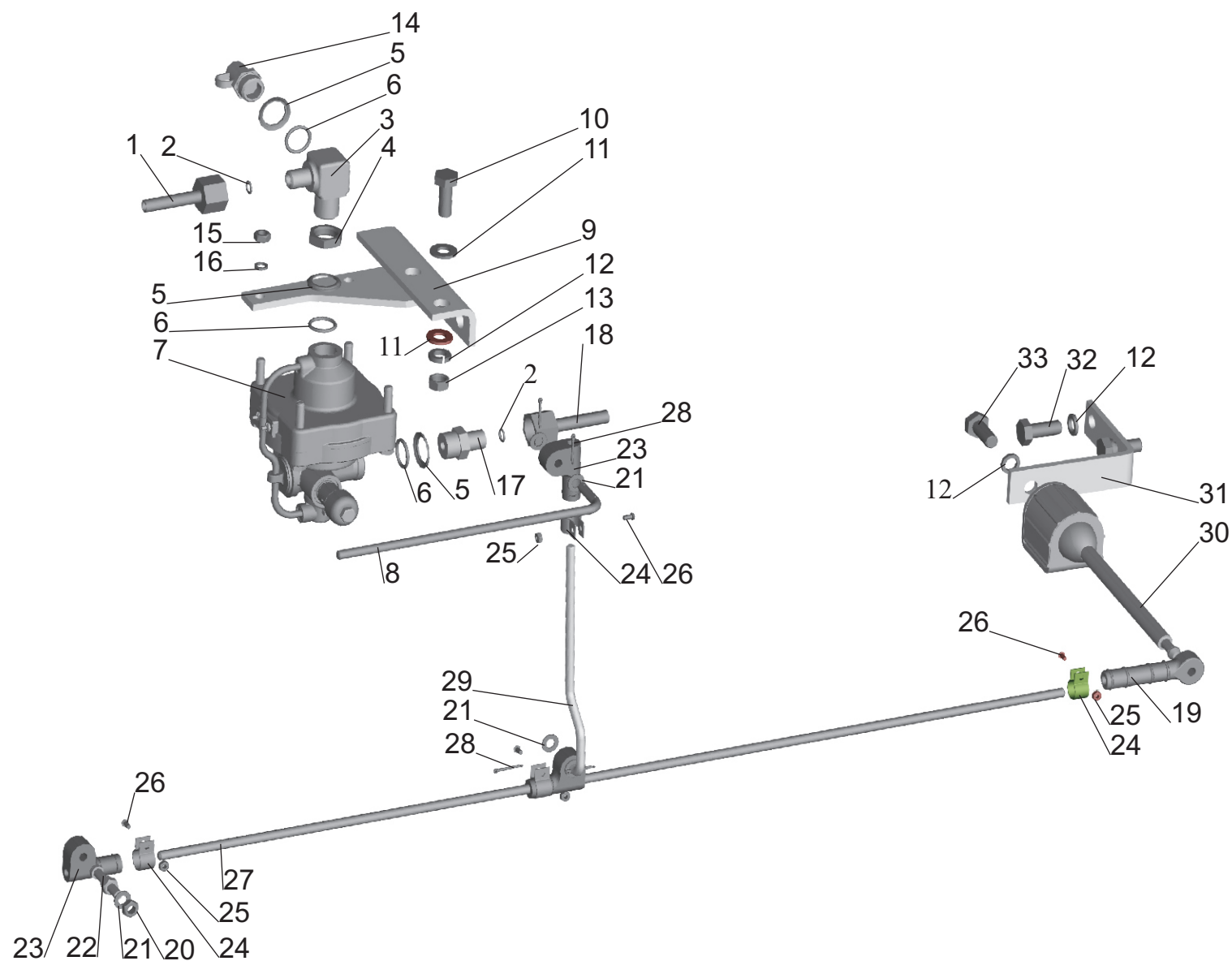
Рис. 118 Крепление регулятора тормозных сил 64221-3533002-02 Fig. 118 Mounting of brake force regulator 64221-3533002-02
