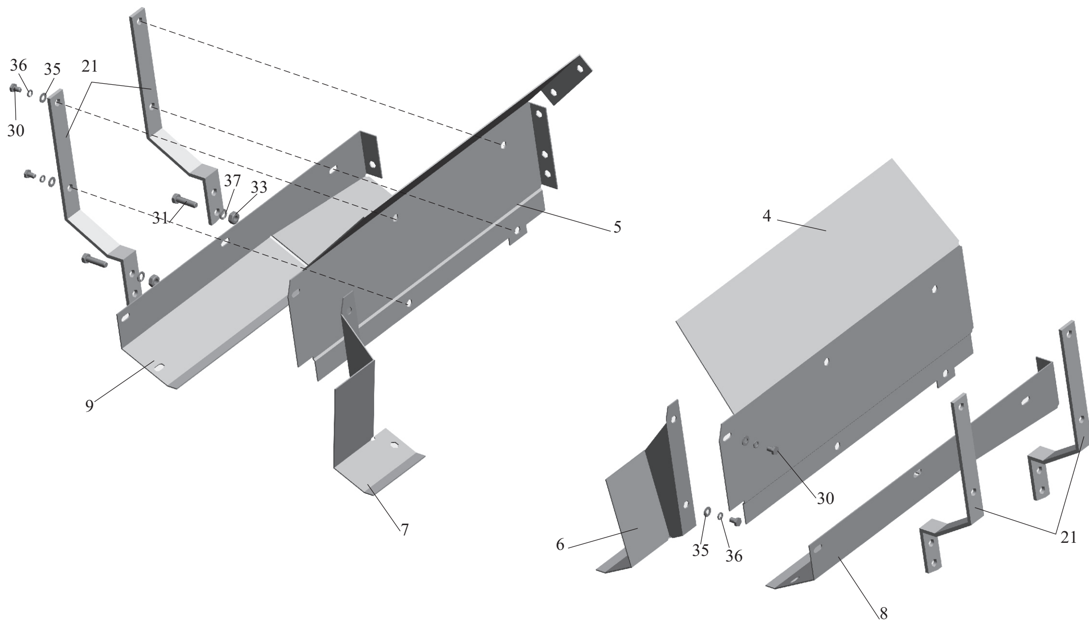
Рис. 8 Установки шумоизоляционных экранов 555102-1061003-040 (551605-1061002-040) Fig. 8 Mounting noise isolation screens 555102-1061003-040 (551605-1061002-040)
