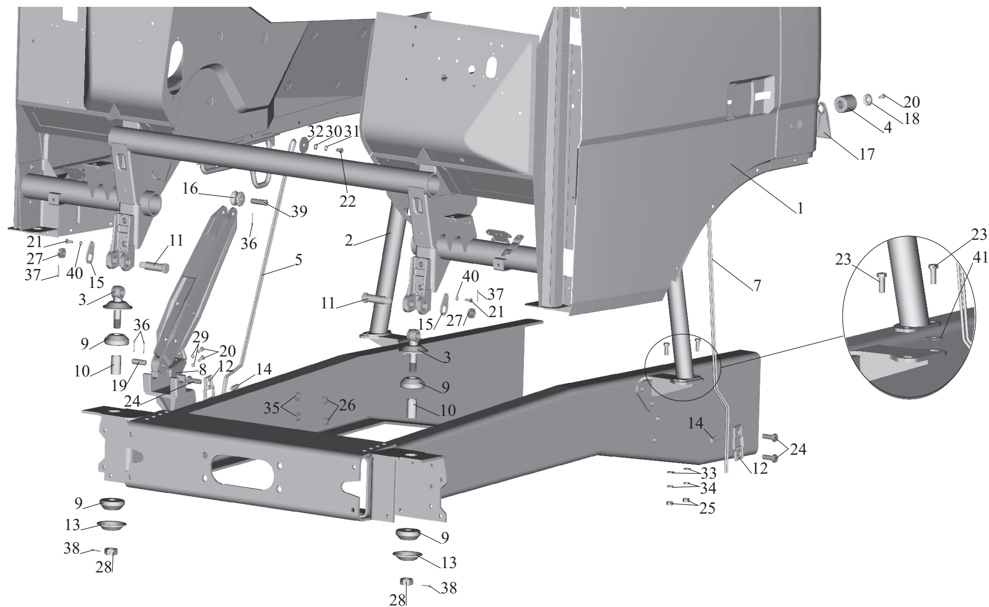
Рис. 173 Установка малой кабины Fig. 173 Installation of small cab
