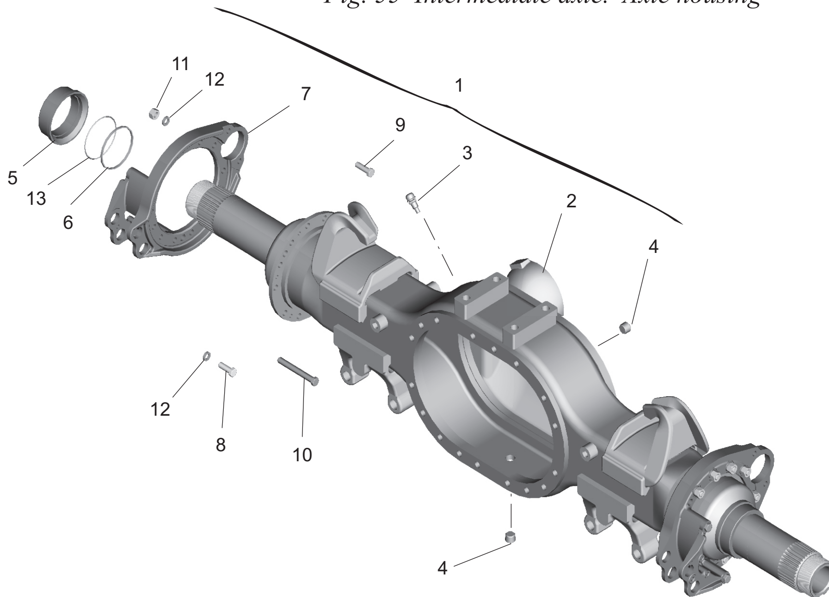
Рис. 55 Мост средний. Картер моста Fig. 55 Intermediate axle. Axle housing
