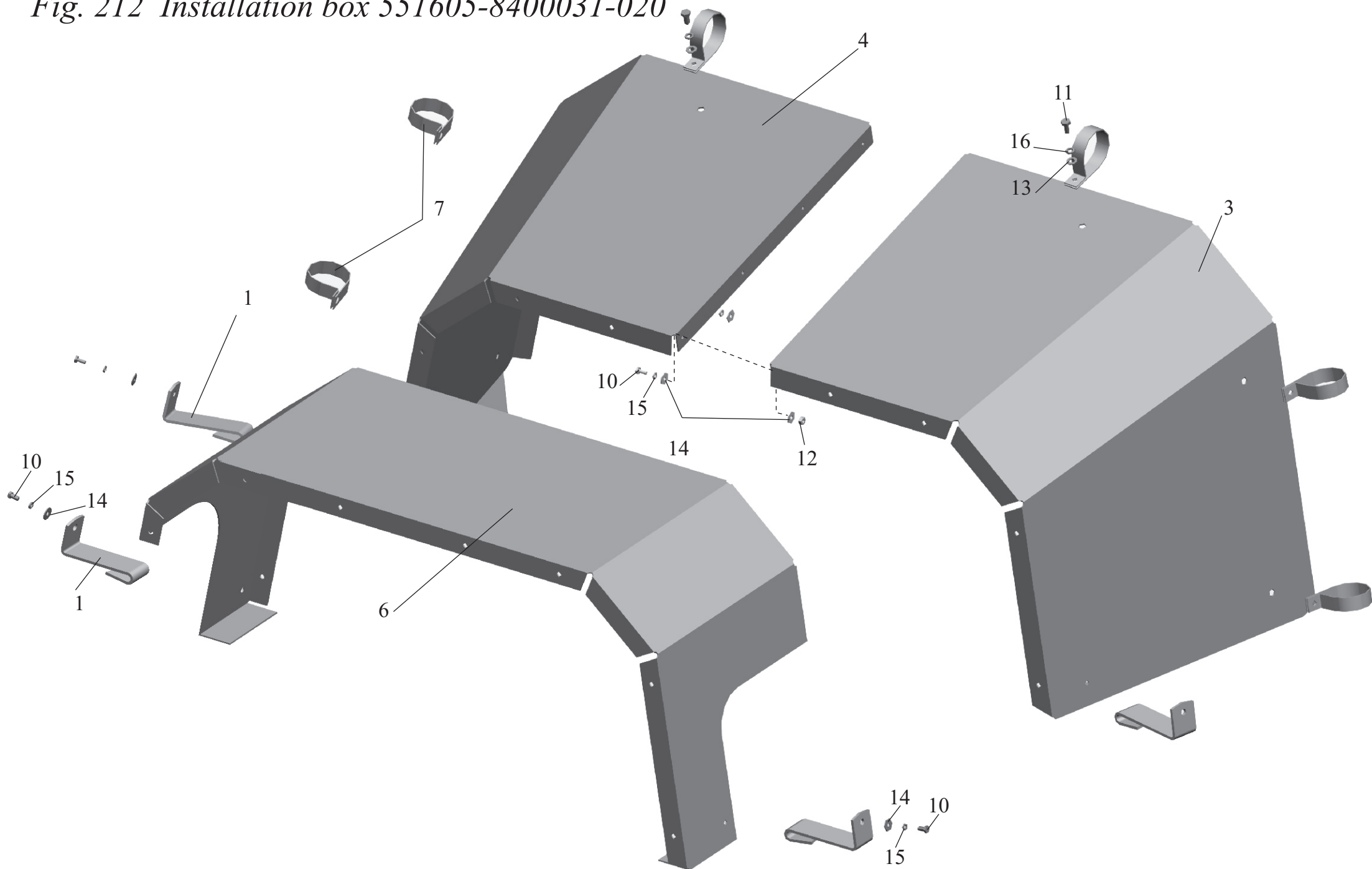
Рис. 212 Установка короба 551605-8400031-020
