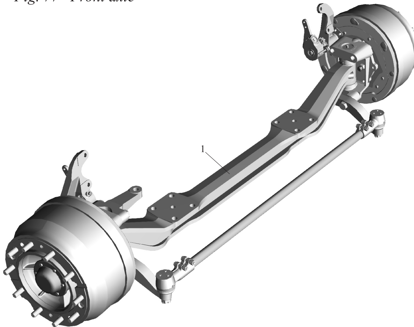
Рис. 77 Передняя ось Fig. 77 Front axle
