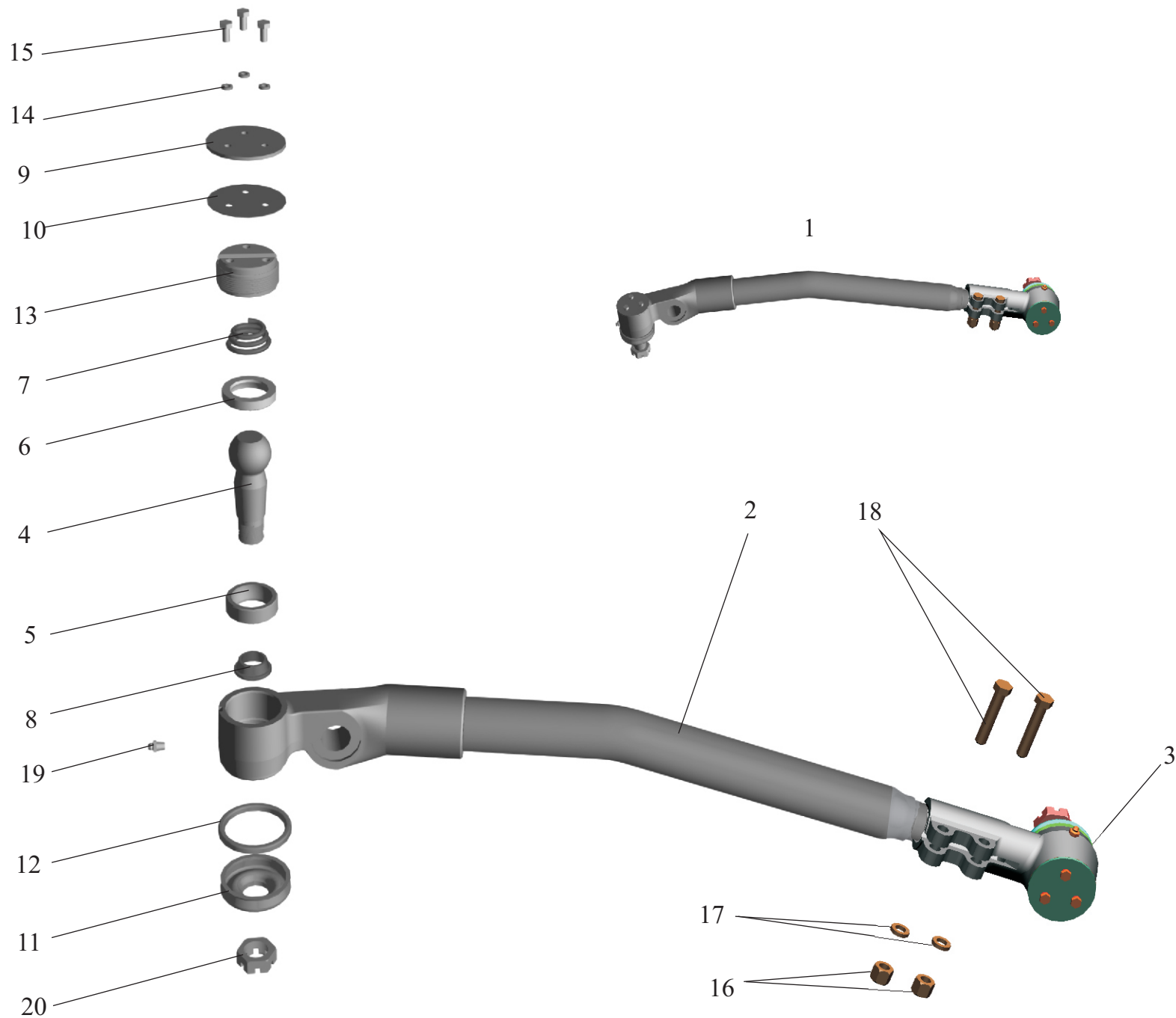
Рис. 82 Тяга продольная 5551-3003010-30 Fig. 82 Drag rod 5551-3003010-30
