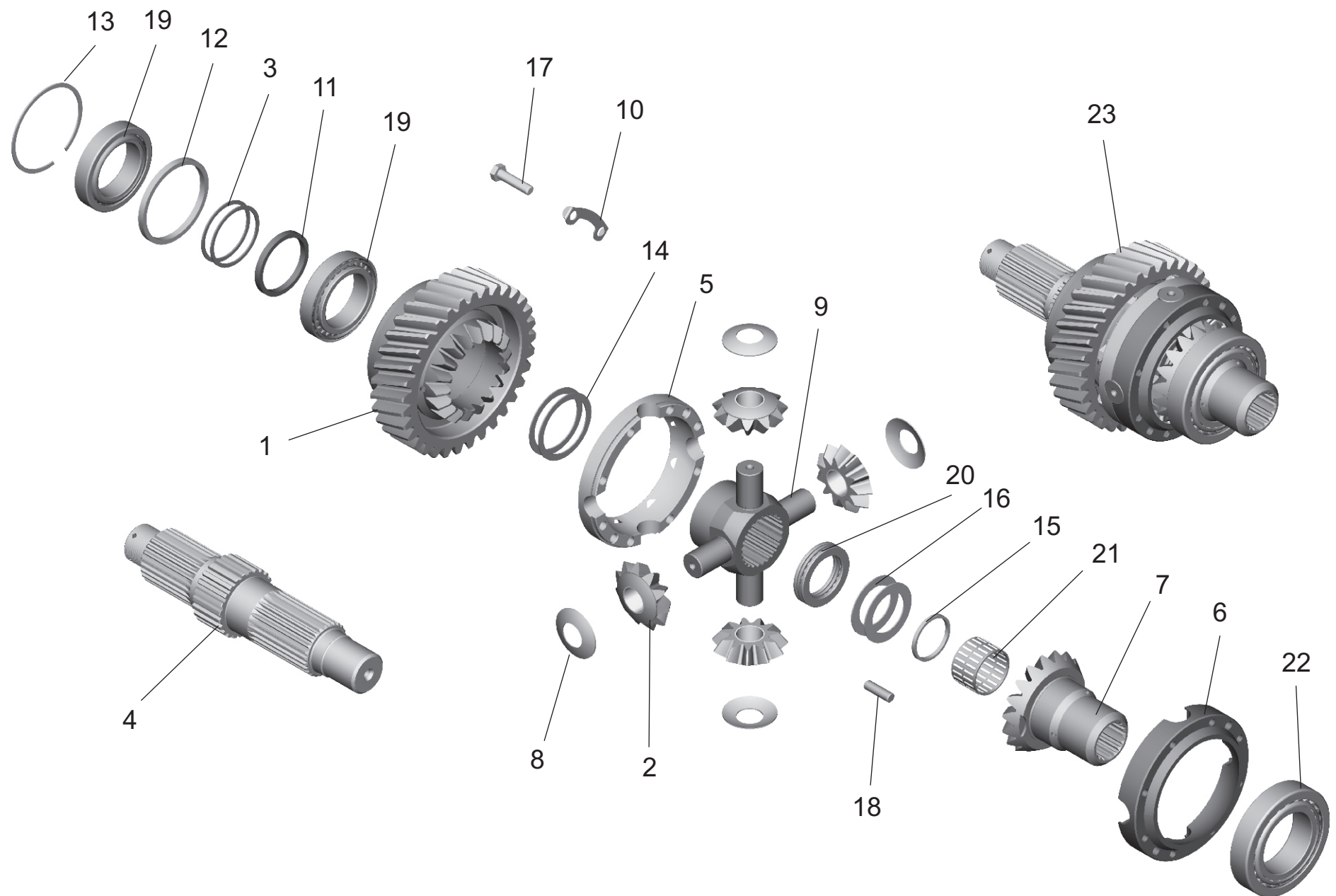
Рис. 59 Редуктор среднего моста. Дифференциал межосевой Fig. 59 Intermediate axle reduction gear. Interaxle differential
