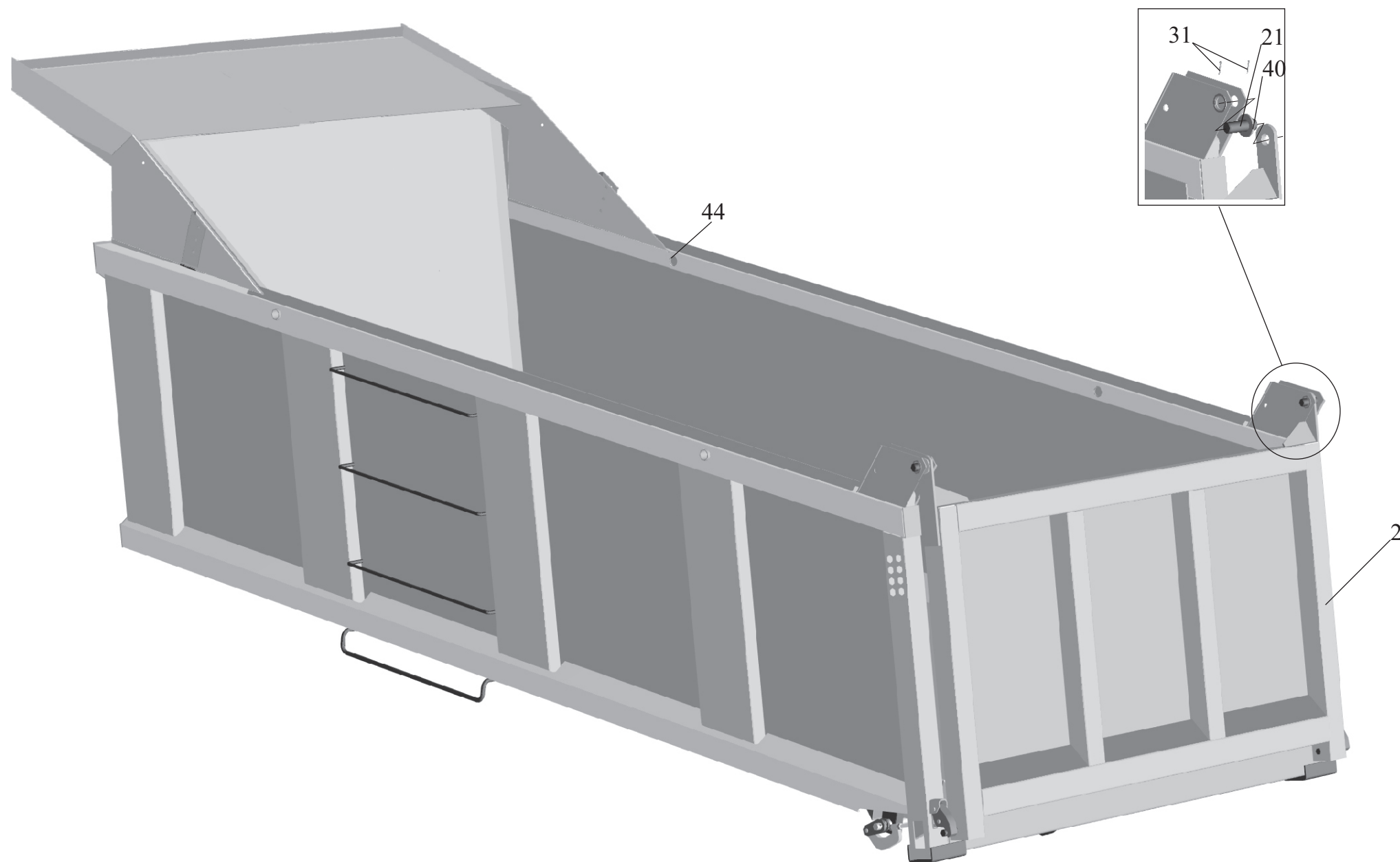
Рис. 215 Платформа V=10,3\text{м}^3 (лист 1) Fig. 215 Platform V=10,3\text{м}^3 (page 1)
