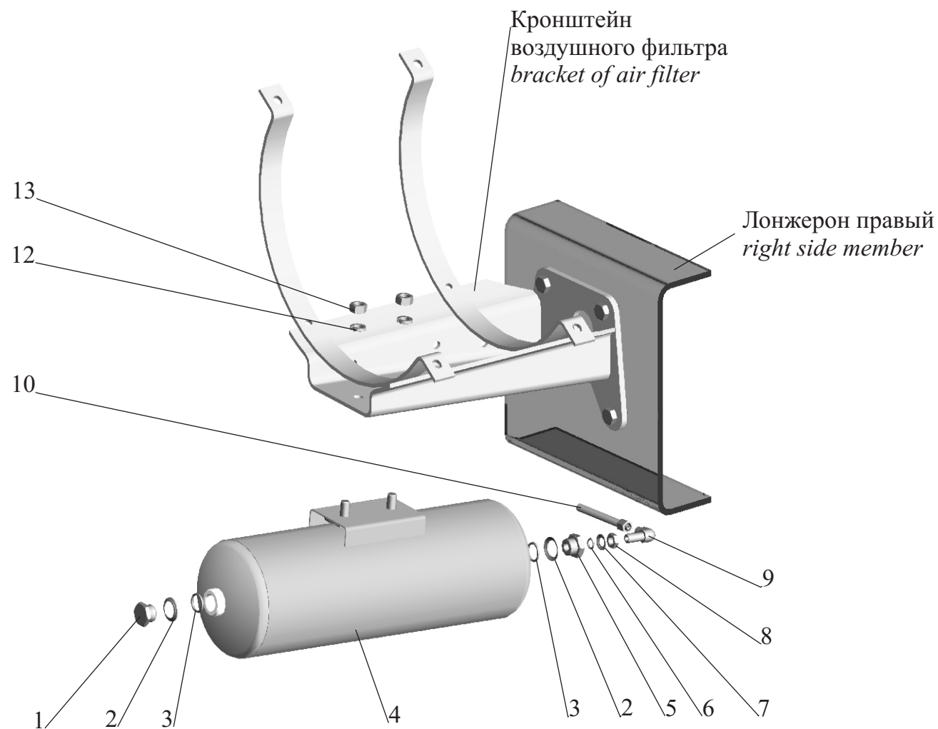
Рис. 103 Ресивер регенерации 64226-3513015 Fig. 103 Receiver of regeneration 64226-3513015
