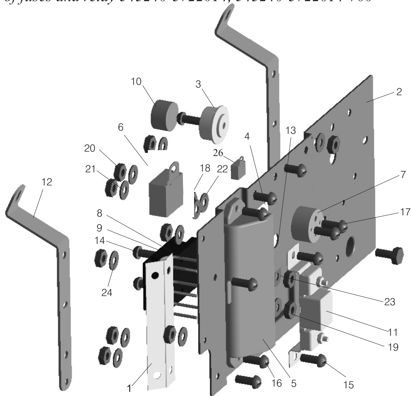
Рис. 140 Панель блоков предохранителей и реле 543240-3722014, 543240-3722014-700 Fig. 140 Panel of fuses and relay 543240-3722014, 543240-3722014-700
