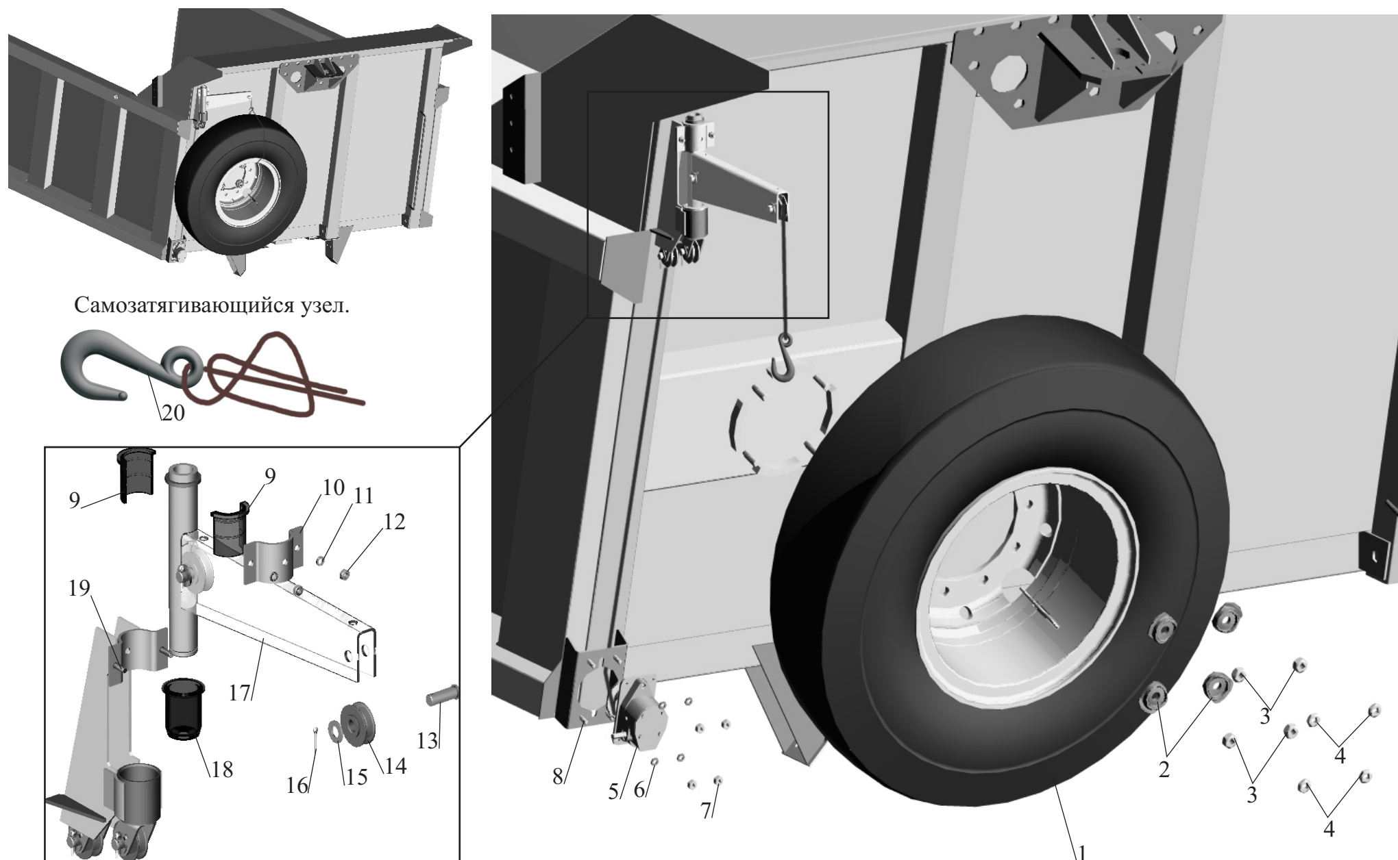
Рис. 84 Установка запасного колеса 551607-3100001-40, 5516-3100001-40 Fig. 84 Installation spare wheel 551607-3100001-40, 5516-3100001-40
