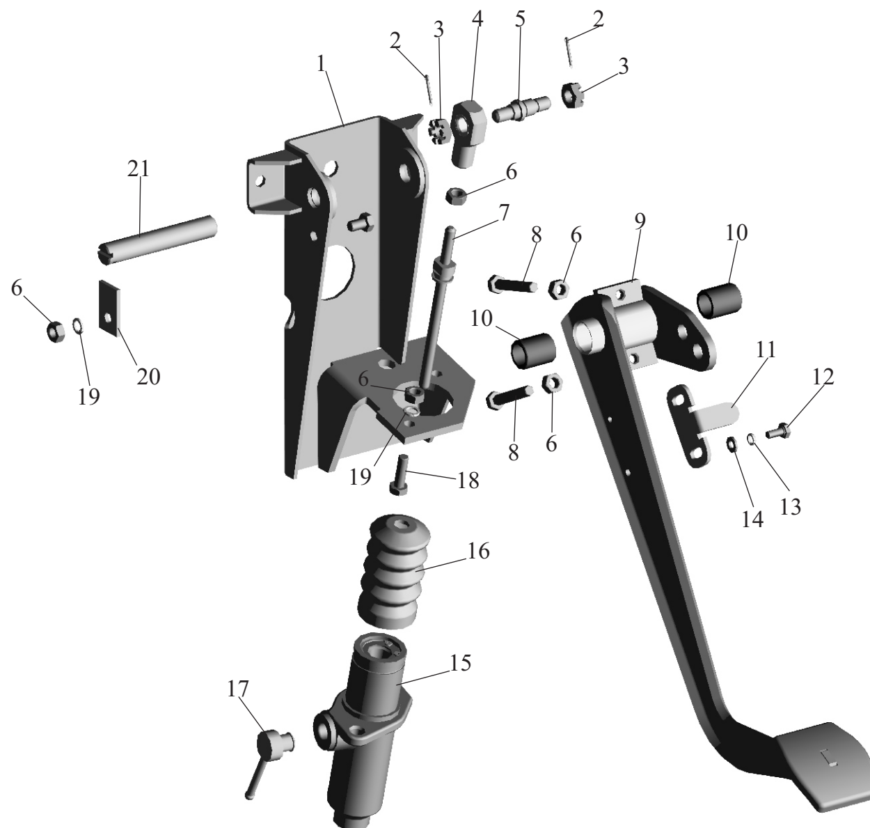
Рис. 29 Основание педали 64226-1602004, 64221-1602004-10 Fig. 29 Pedal base 64226-1602004, 64221-1602004-10
