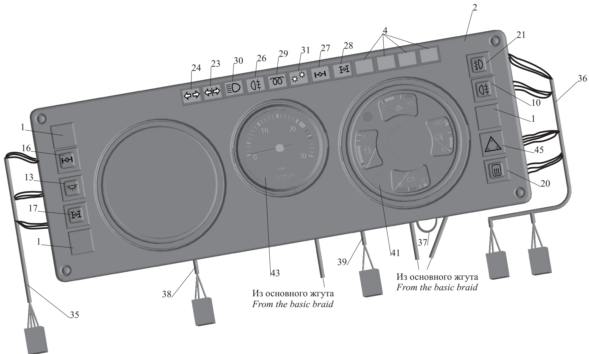
Рис. 138 Щиток приборов 6303-3805010 (на автомобилях с трехсторонней разгрузкой) Fig. 138 Board of devices 6303-3805010 (on automobiles with tripartite unloading)
