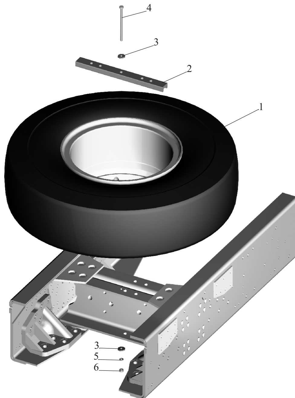
Рис. 83 Установка запасного колеса 551605-3100001, 551605-3100001-700 Fig. 83 Installation spare wheel 551605-3100001, 551605-3100001-700
