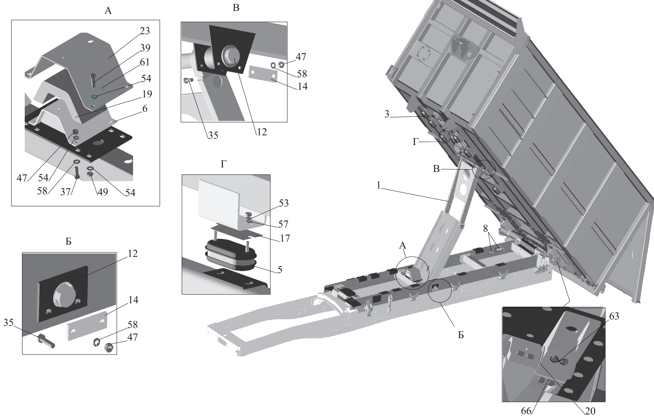
Рис. 218 Установка платформы V=15.4\text{m}^3 (лист 2) Fig. 218 Installation of platform V=15.4\text{m}^3 (page 2)
