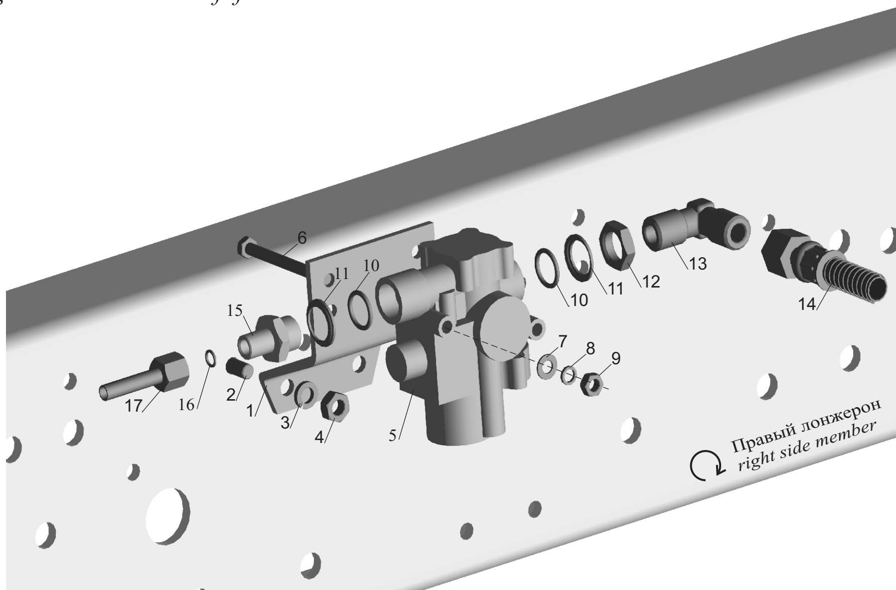
Рис. 125 Установка передних модуляторов и соединительной арматуры Fig. 125 Installation of front modulators and attach accessories
