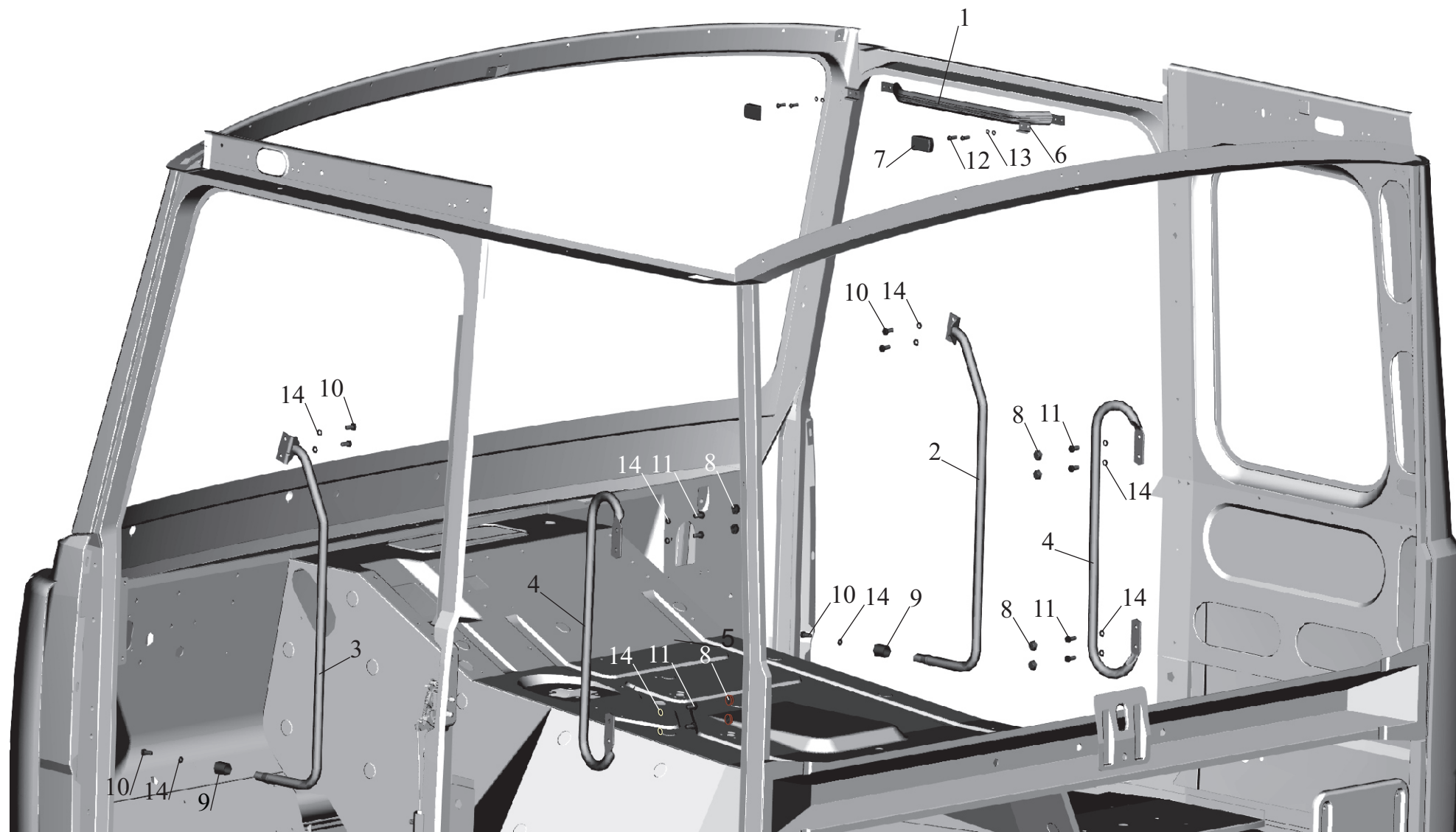
Рис. 199 Установка поручней в кабине 64221-8200030-10 Fig. 199 Installation of grab handles in cab 64221-8200030-10
