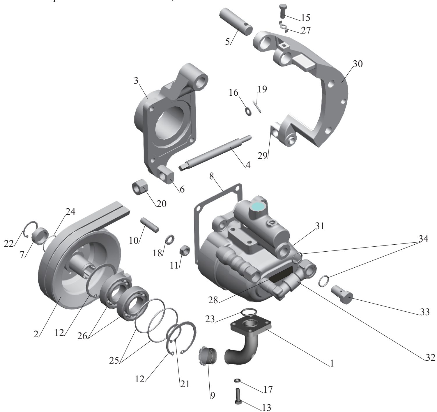
Fig. 91 Pump 630300-3407010, 630300-3407010-700
