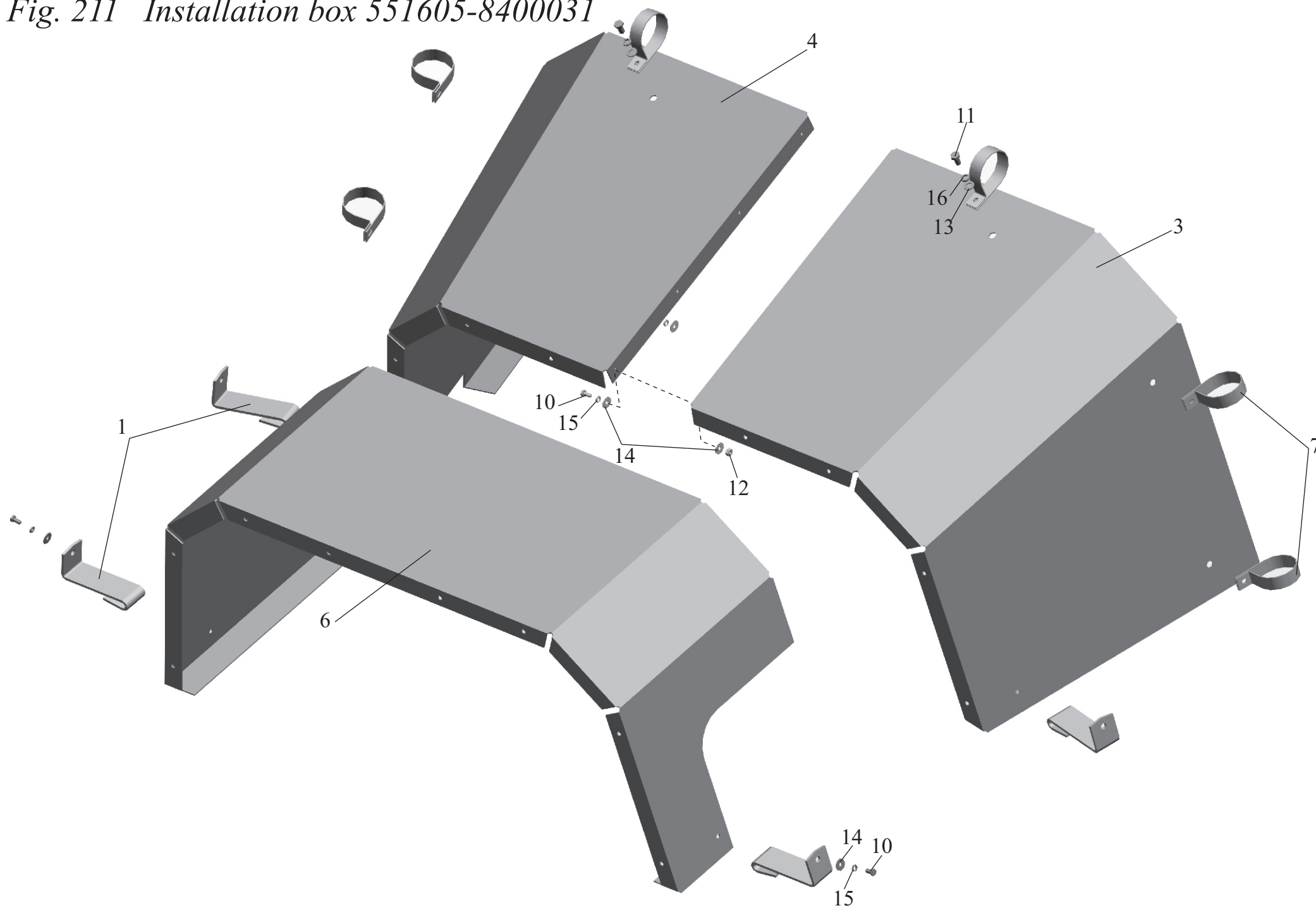
Рис. 211 Установка короба 551605-8400031
