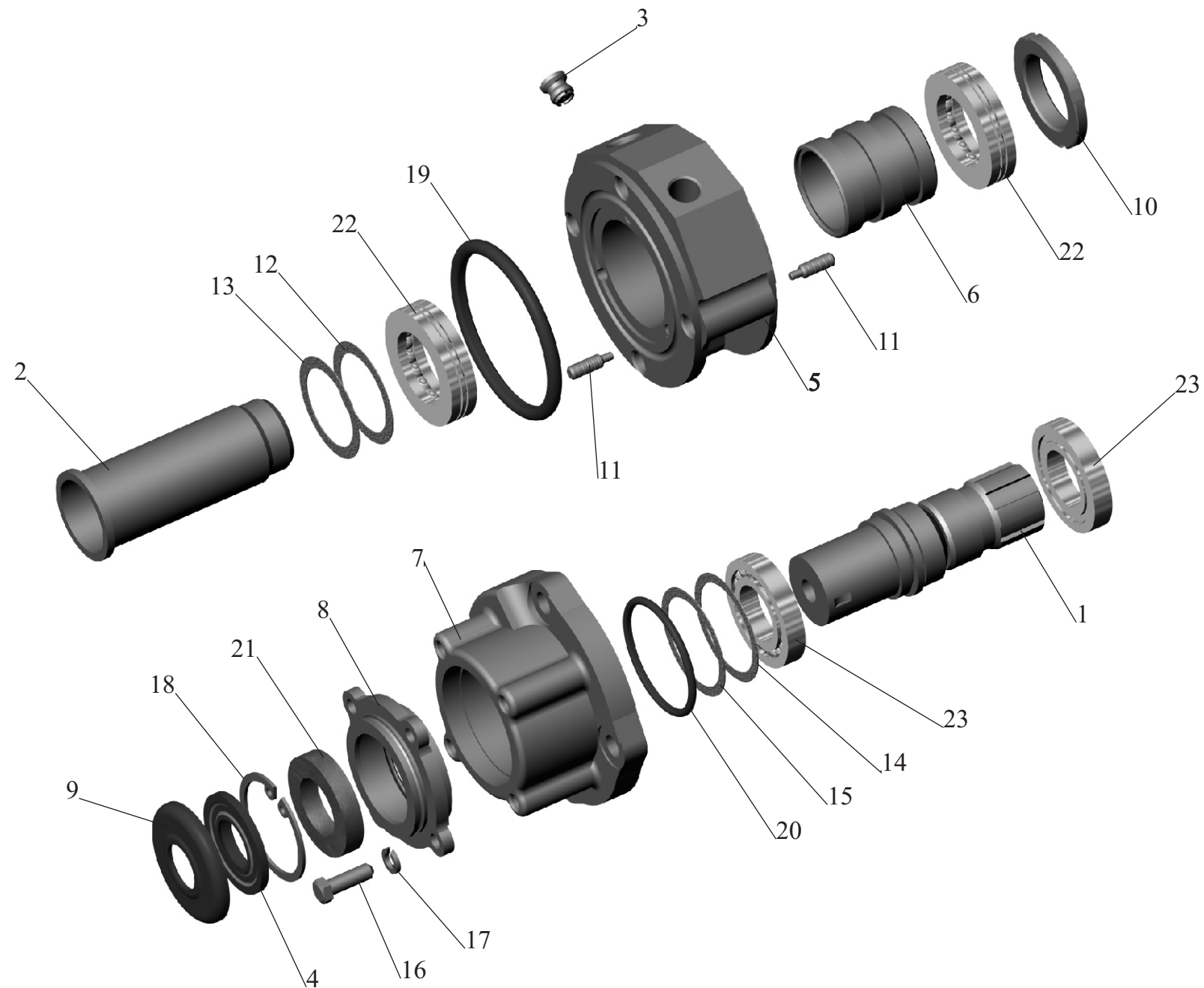
Рис. 96 Распределитель 5336-3416010-01 Fig. 96 Control valve 5336-3416010-01
