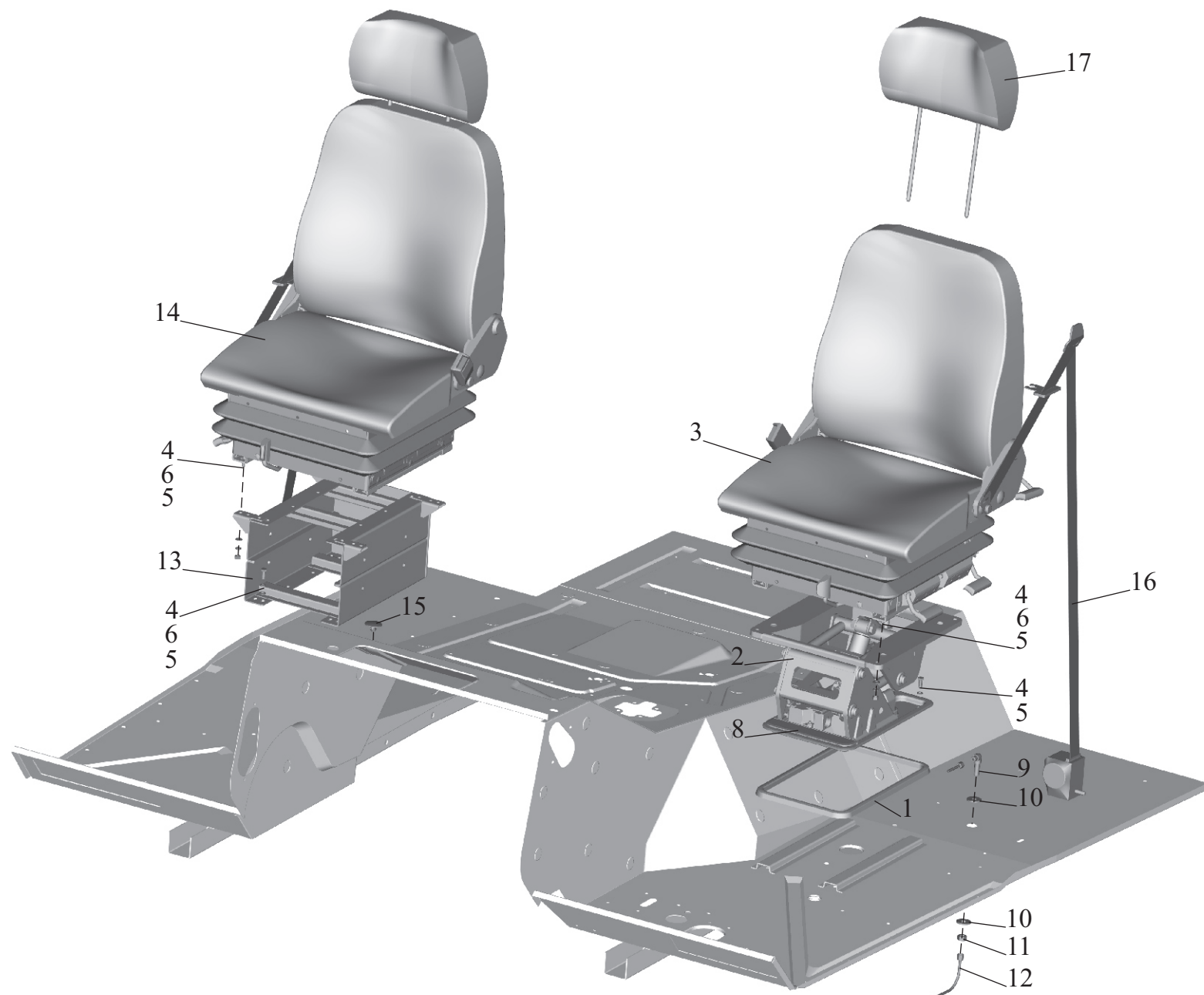
Рис. 190 Установка и пневмопитание сидений 5433-6800006 Fig. 190 Installation and pneumatic supply of seat 5433-6800006
