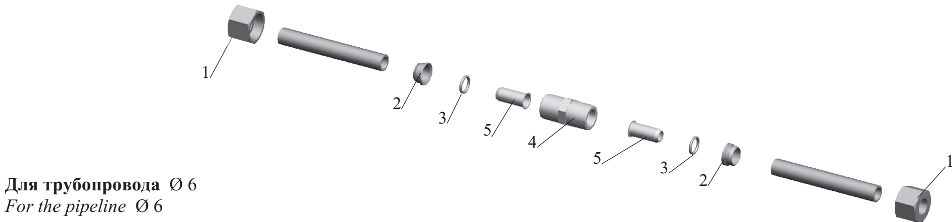
Рис. 127 Соединение для ремонта поврежденных трубопроводов Fig. 127 Connection for repair of the damaged pipelines
