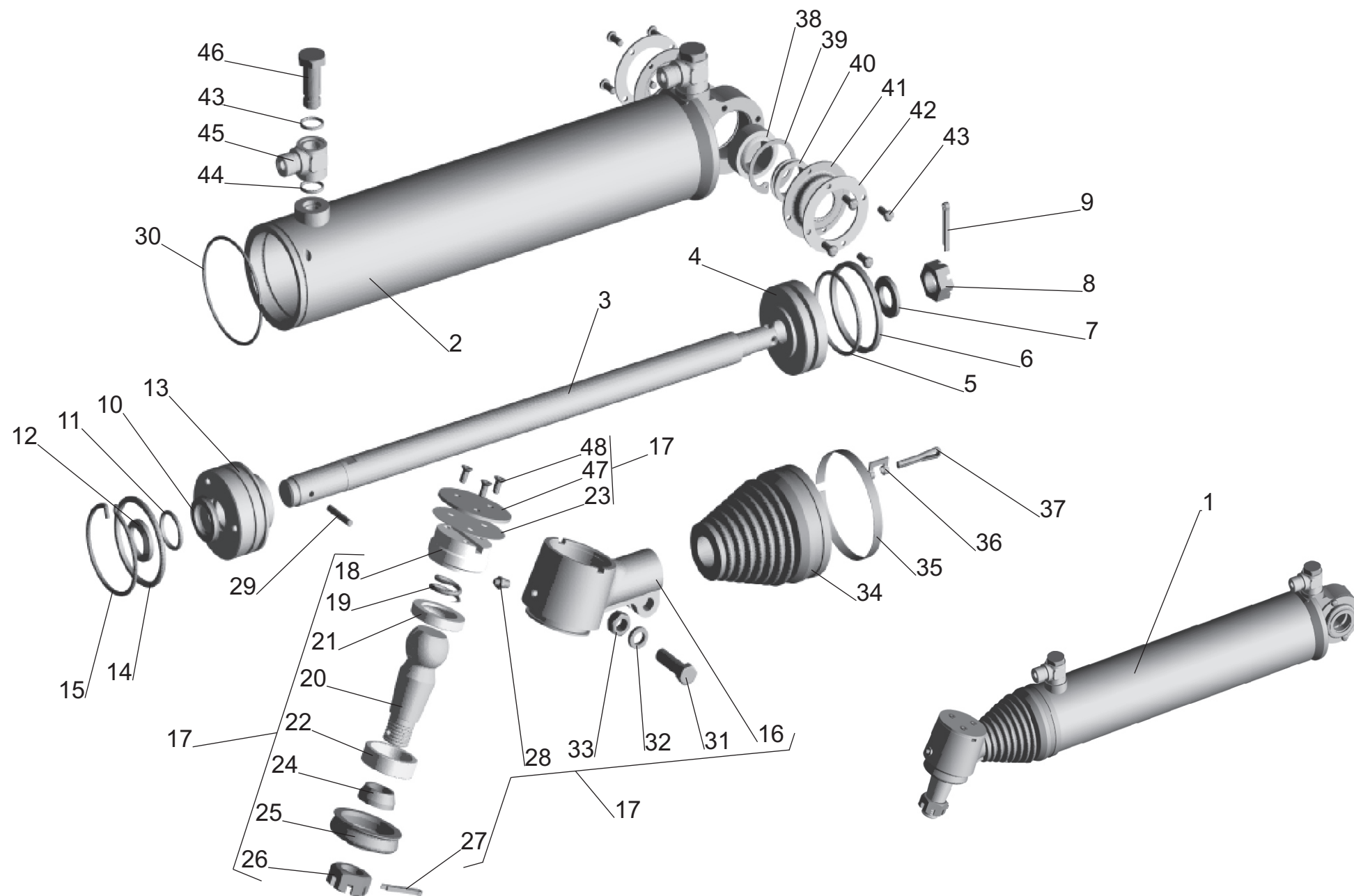
Рис. 93 Силовой цилиндр гидроусилителя рулевого управления 6422-3405004 Fig. 93 Steering hydraulic booster power cylinder 6422-3405004
