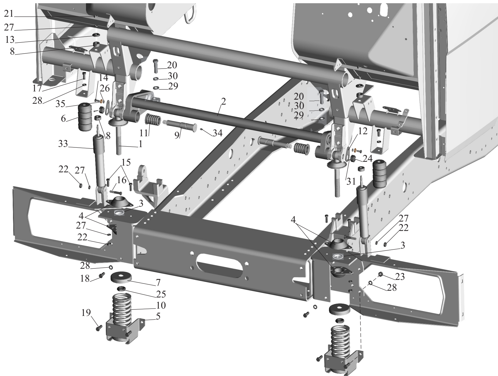
Рис. 179 Переднее подрессоривание большой кабины 64226-5001700 Fig. 179 Front springing the large cab 64226-5001700
