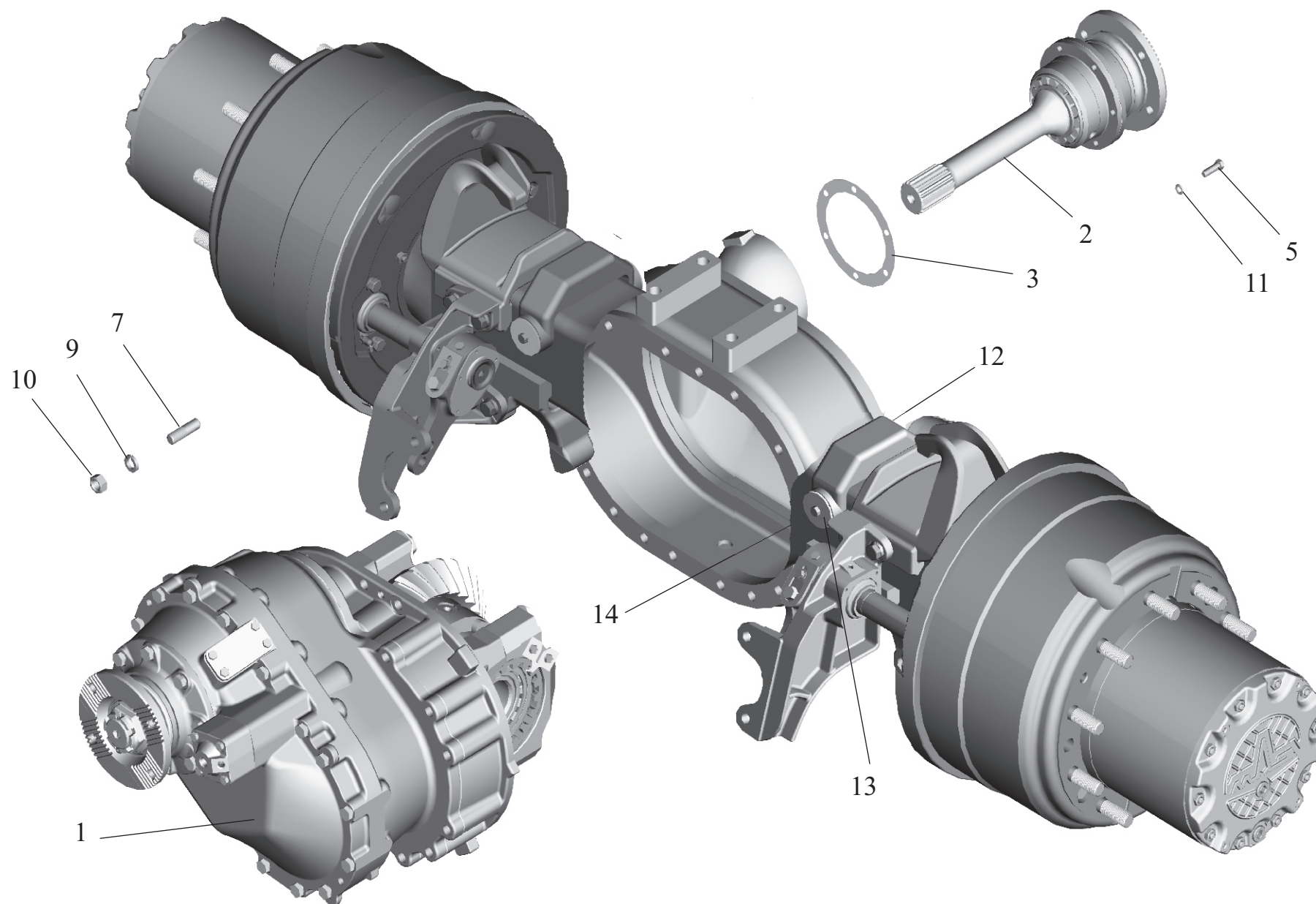
Рис. 54 Мост средний. Установка редуктора и вала заднего. Fig. 54 Intermediate axle. Installation of reduction gear and rear shaft.
