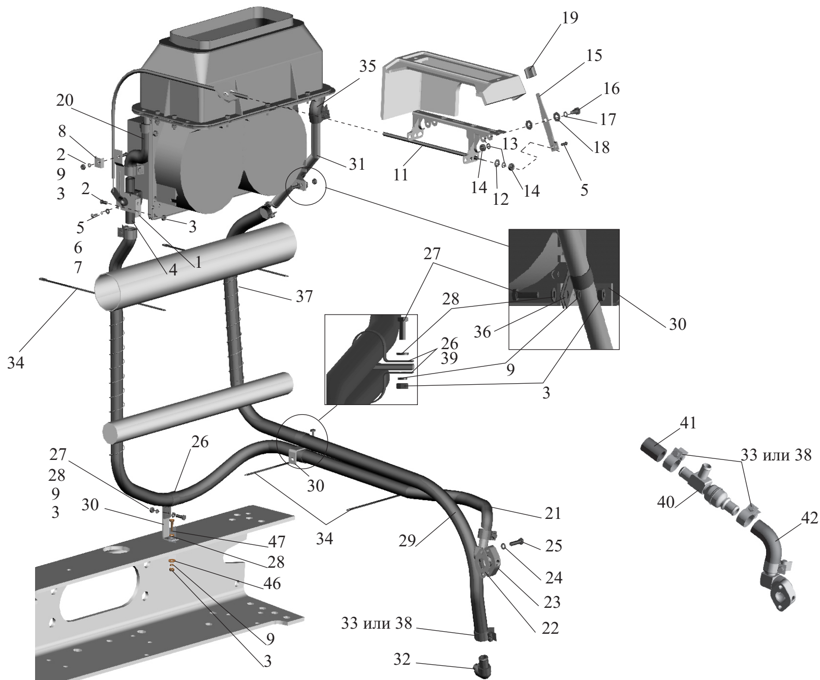
Рис. 205 Установка шлангов и крана управления отопителем Fig. 205 Installation of hoses and control cock of heater
