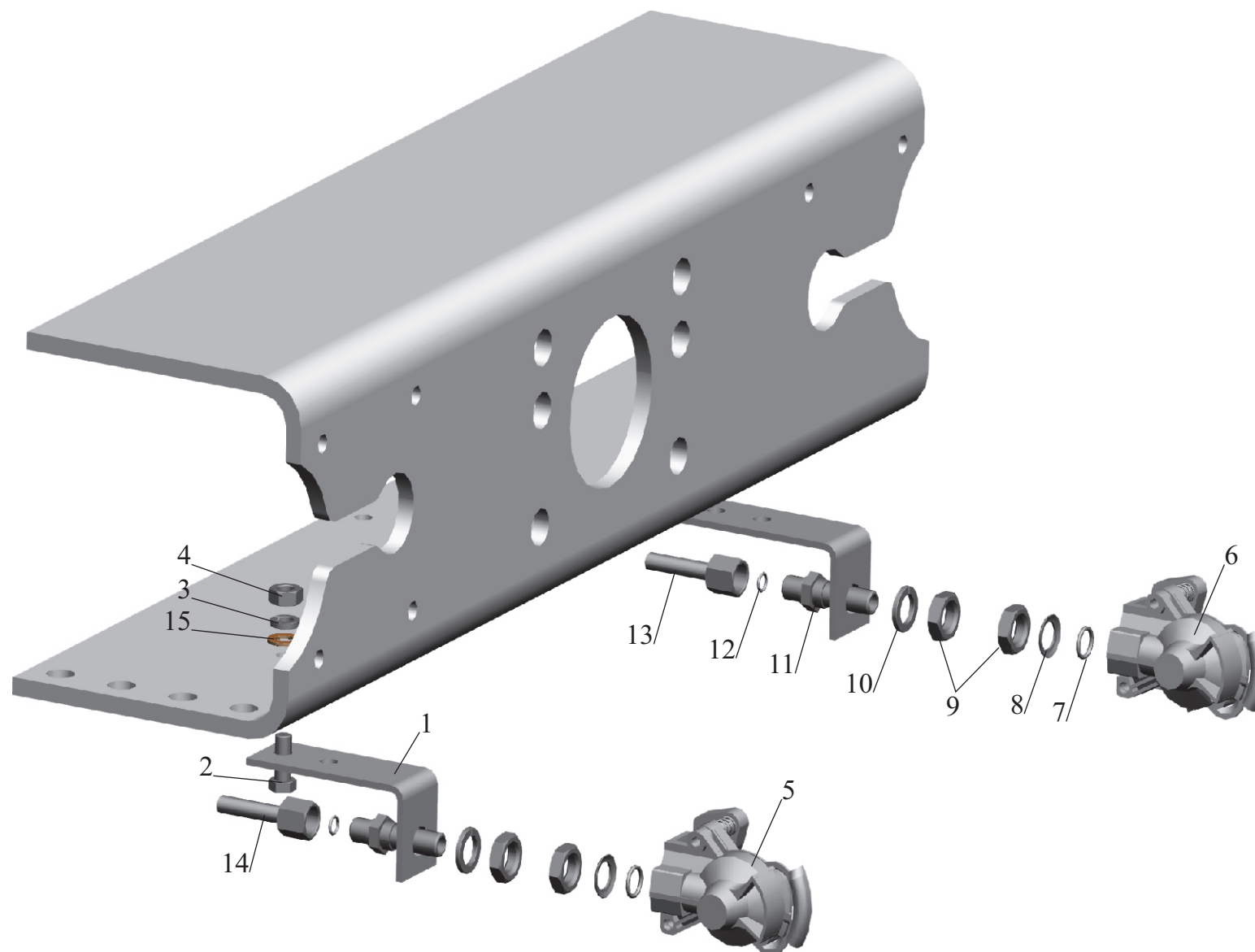
Рис. 116 Пневмовыводы к прицепу 63031-3521004 Fig. 116 Pneumatic leads to the trailer 63031-3521004
