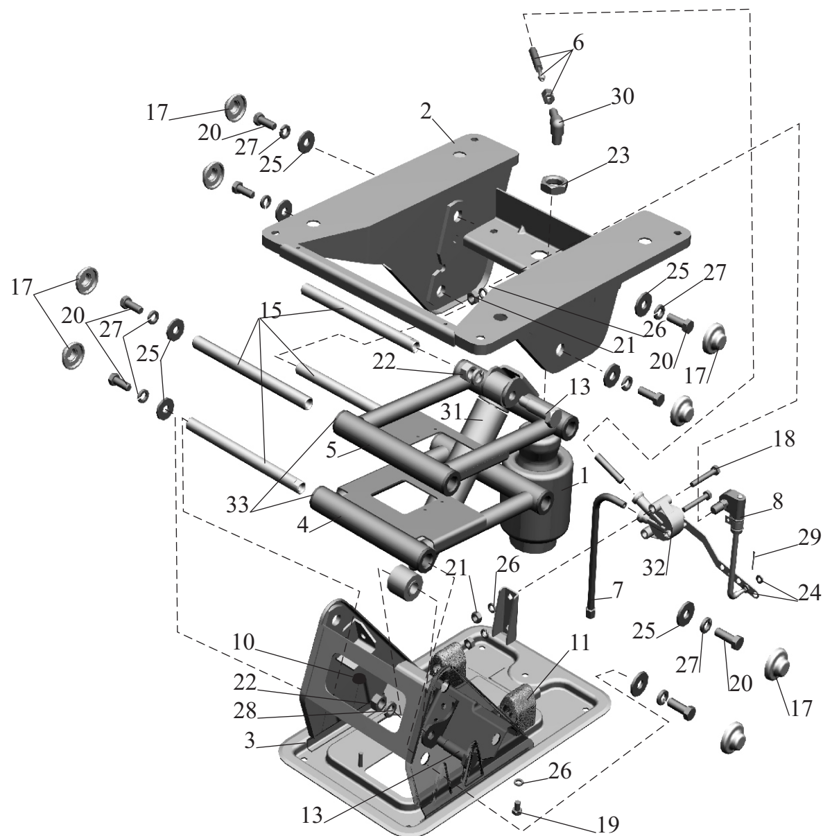
Рис. 195 Подставка сидения с пневмооборудованием 6430-6807006-010 Fig. 195 Seat support with pneumatic equipment 6430-6807006-010
