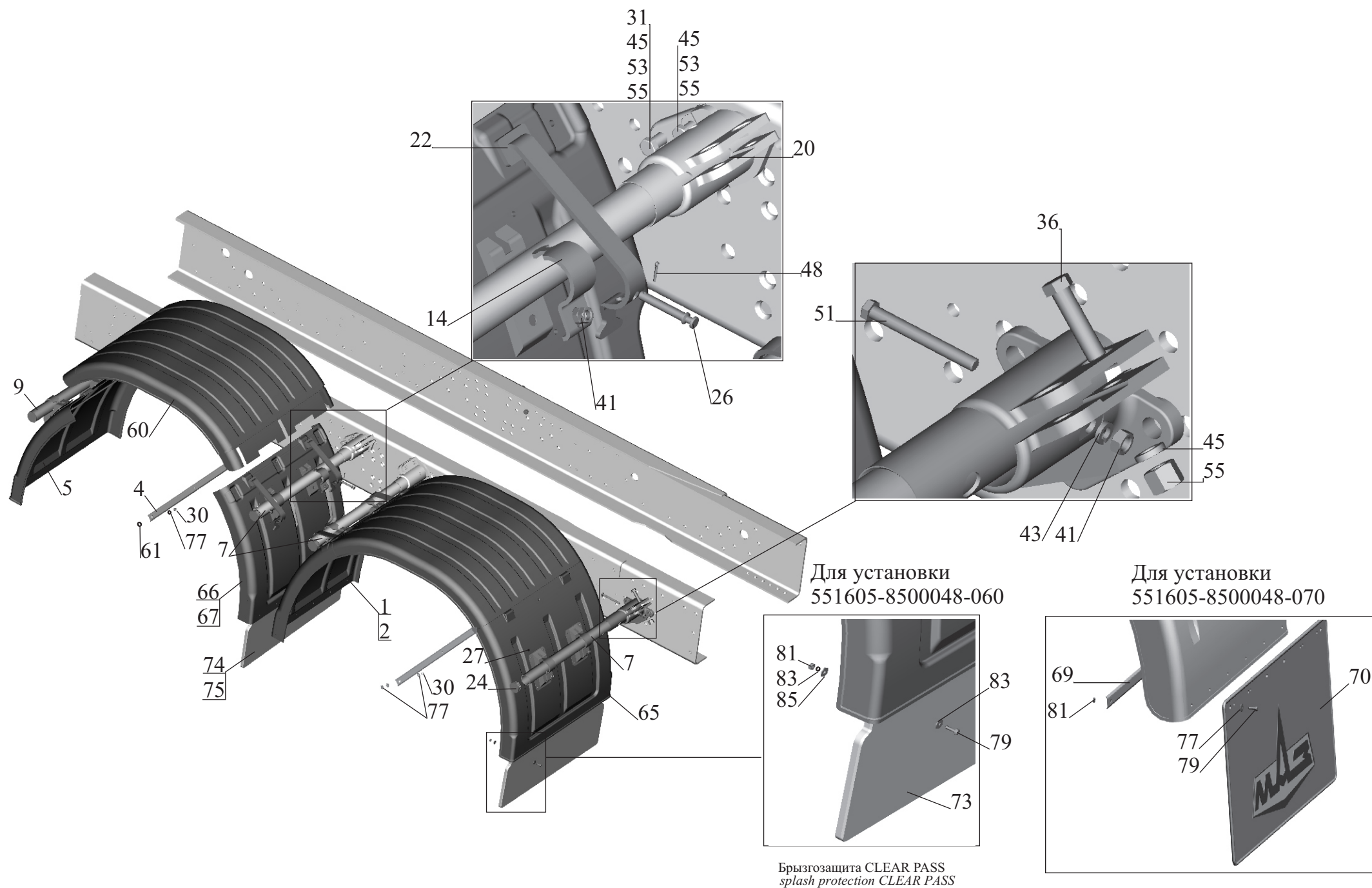
Рис. 229 Установка крыльев 551605-8500048-060, 551605-8500048-070 Fig. 229 The fenders installation 551605-8500048-060, 551605-8500048-070
