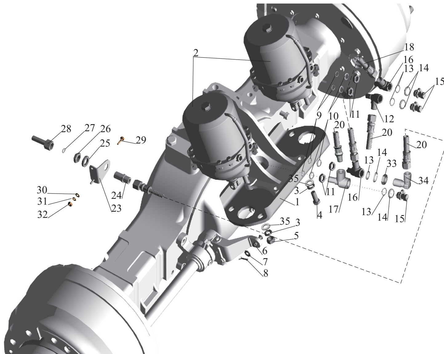
Рис. 114 Крепление тормозных камер 5440-3519002-10 (на задний мост) Fig. 114 Mounting of brake chambers 5440-3519002-10 (on rear axle)
