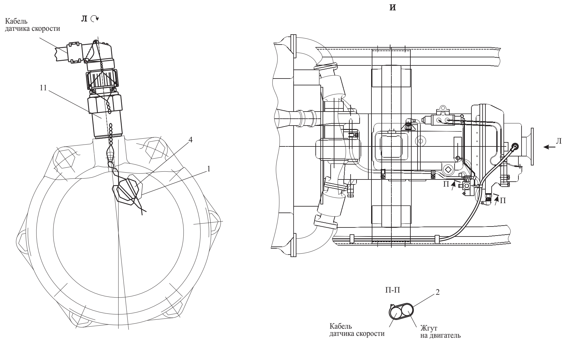
Рис. 142 Установка и пломбировка спидометра 551605-3800004, 551605-3800004-700 (лист 2) Fig. 142 Installation and identification seal of a speedometer 551605-3800004, 551605-3800004-700 (page 2)
