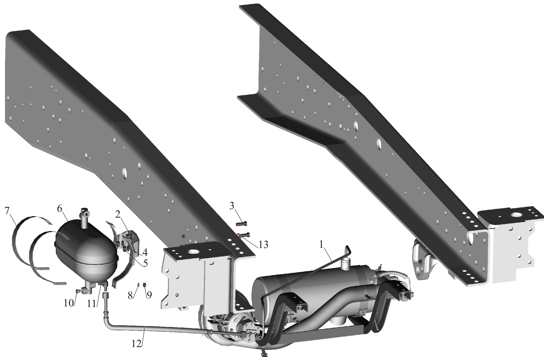
Рис. 7 Топливопроводы питания подогревателя 6422-1015004 Fig. 7 Fuel lines of heater 6422-1015004
