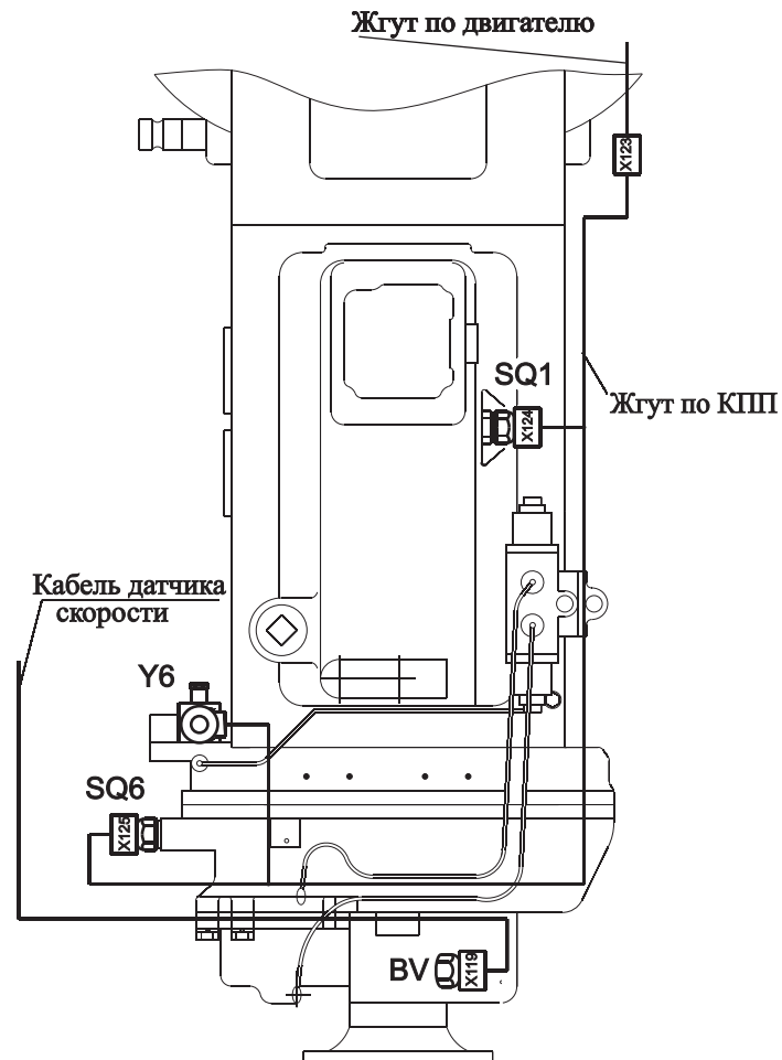
КПП ЯМЗ-238М gearbox ЯМЗ-238М
