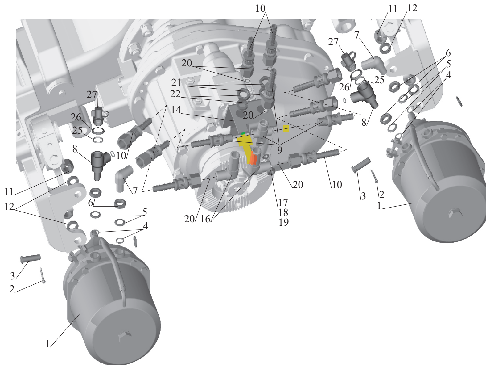
Рис. 115 Крепление тормозных камер 551605-3519003 (на средний мост) Fig. 115 Mounting of brake chambers 551605-3519003 (on intermediate axle)
