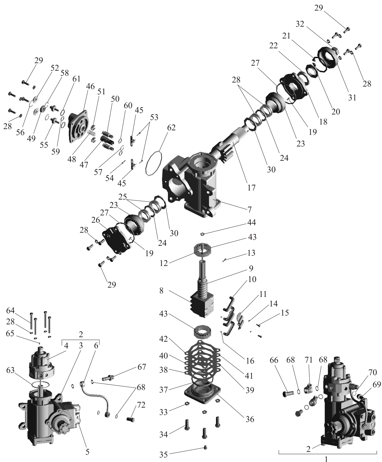
Рис. 94 Механизм рулевой 64221-3400008-02 Fig. 94 Steering mechanism 64221-3400008-02
