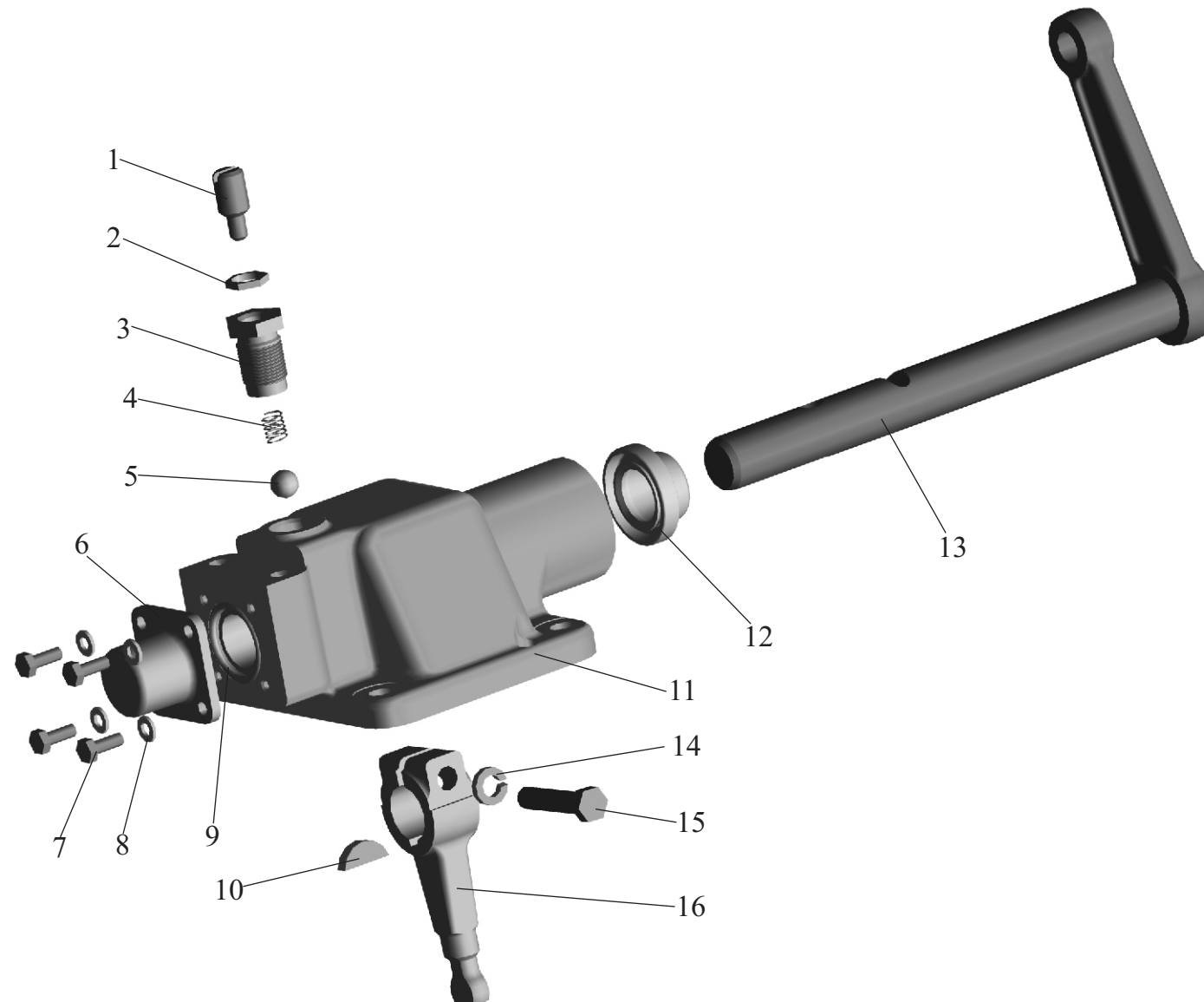
Рис. 33 Механизм переключения передач 5336-1702200-10 Fig. 33 Mechanism of gearshift 5336-1702200-10
