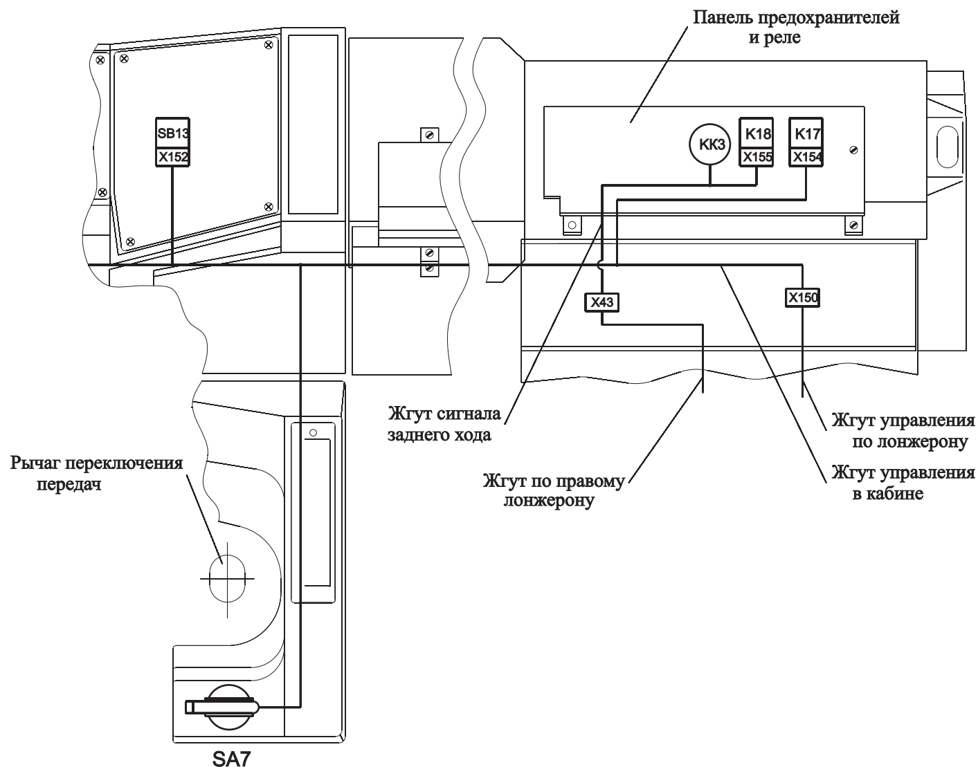
Рис. 152 Расположение разъемов и элементов электрооборудования управления подъемом и опусканием платформы, звукового сигнала заднего хода Fig. 152 An arrangement of sockets and elements of an electric equipment of management of rise and lowering of a platform, a sound signal of a backing
