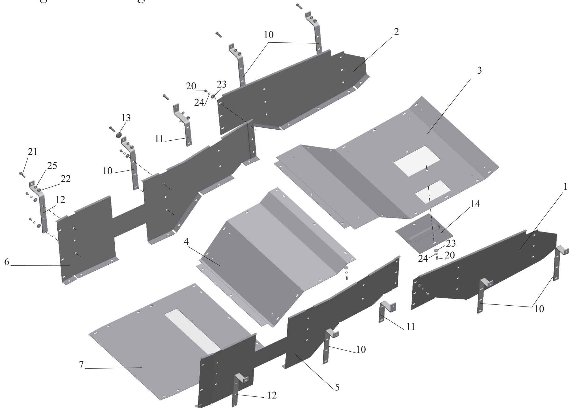
Рис. 10 Установки шумоизоляционных экранов 551605-1061004-040 Fig. 10 Mounting noise isolation screens 551605-1061004-040
