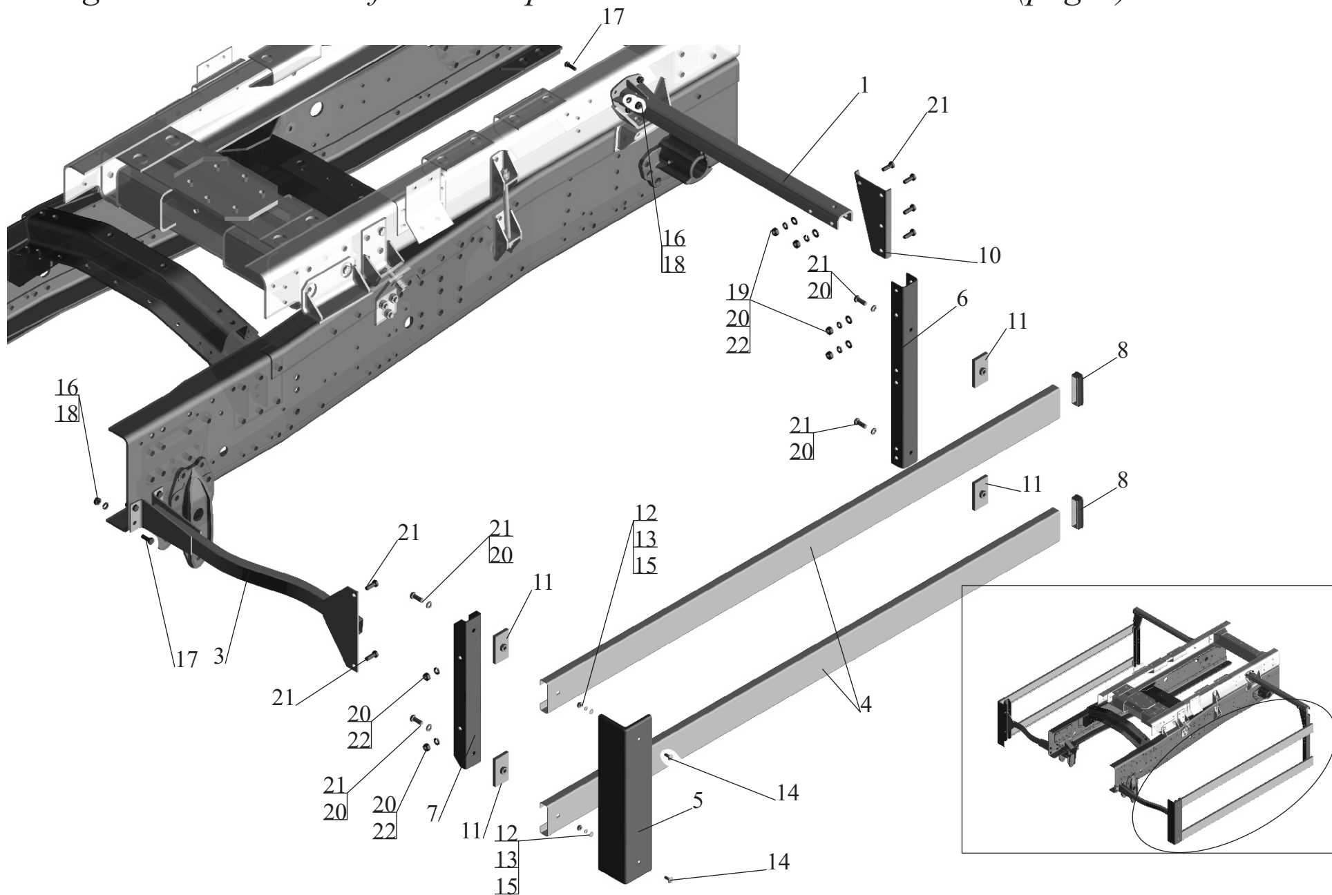
Рис. 72 Установка бокового ограждения 551605-2800040-010 (лист 2) Fig. 72 Installation of a lateral protection 551605-2800040-010 (page 2)
