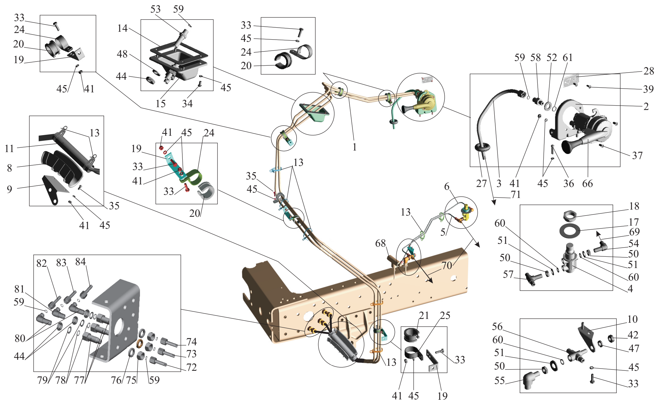
Рис. 121 Привод стояночного и моторного тормозов 64255-3537004 Fig. 121 The parking and motor brakes drive 64255-3537004
