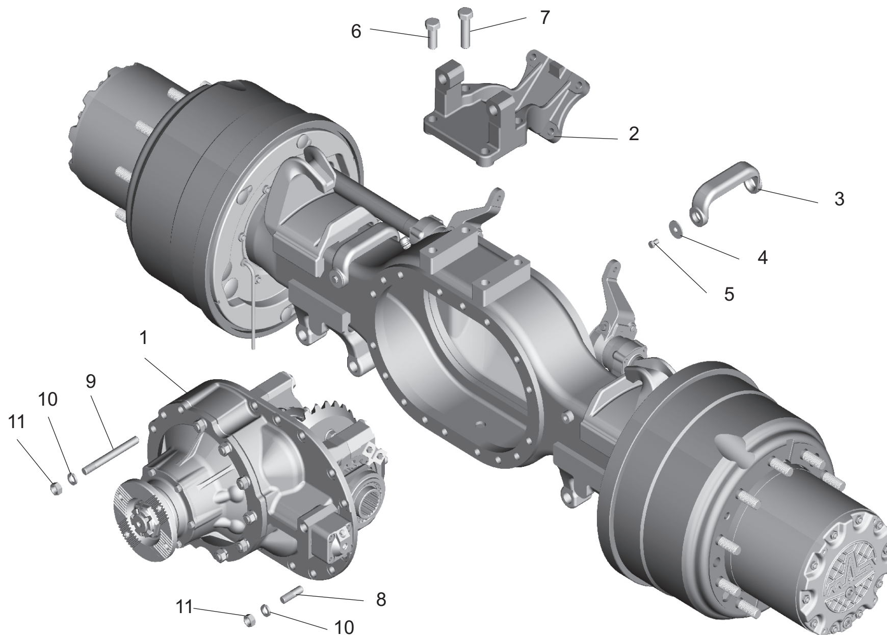
Рис. 43 Мост задний. Установка редуктора и элементов подвески. Fig. 43 Rear axle. Installation of reduction gear and elements of suspension
