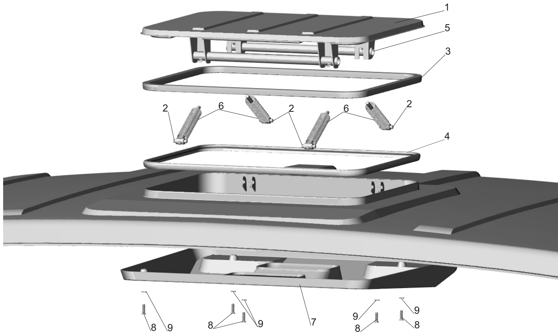
Рис. 183 Установка вентиляционного люка 64221-5700010 Fig. 183 Installation vent hatch 64221-5700010
