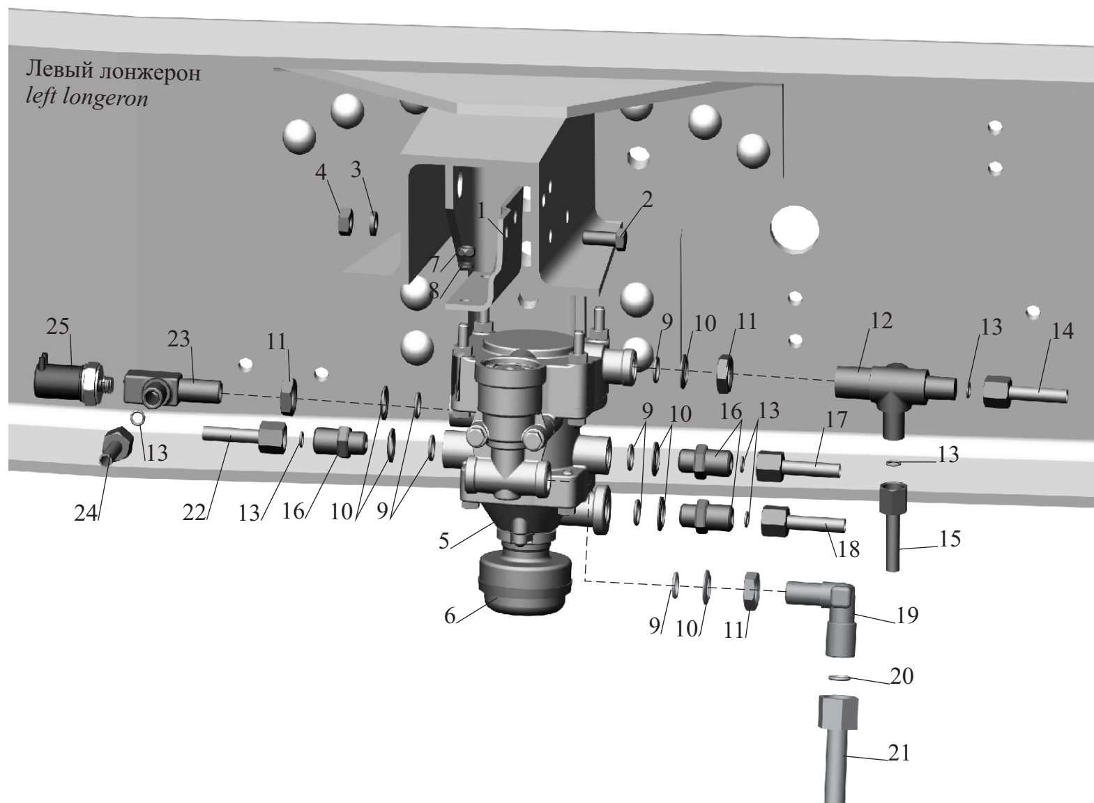
Рис. 117 Установка клапана прицепа 642208-3522005 Fig. 117 Installation of trailer valve 642208-3522005
