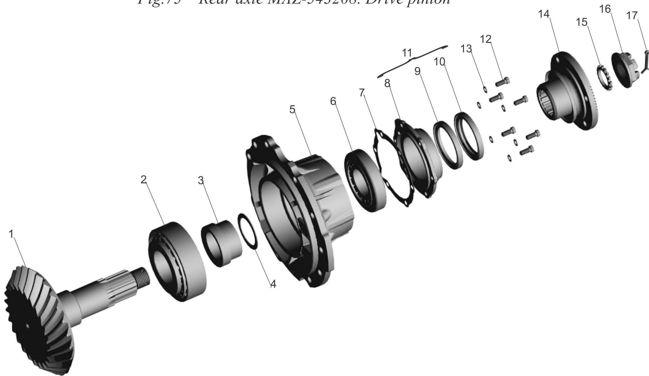
Рис.75 Мост задний МАЗ-543208. Шестерня ведущая Fig.75 Rear axle MAZ-543208. Drive pinion
