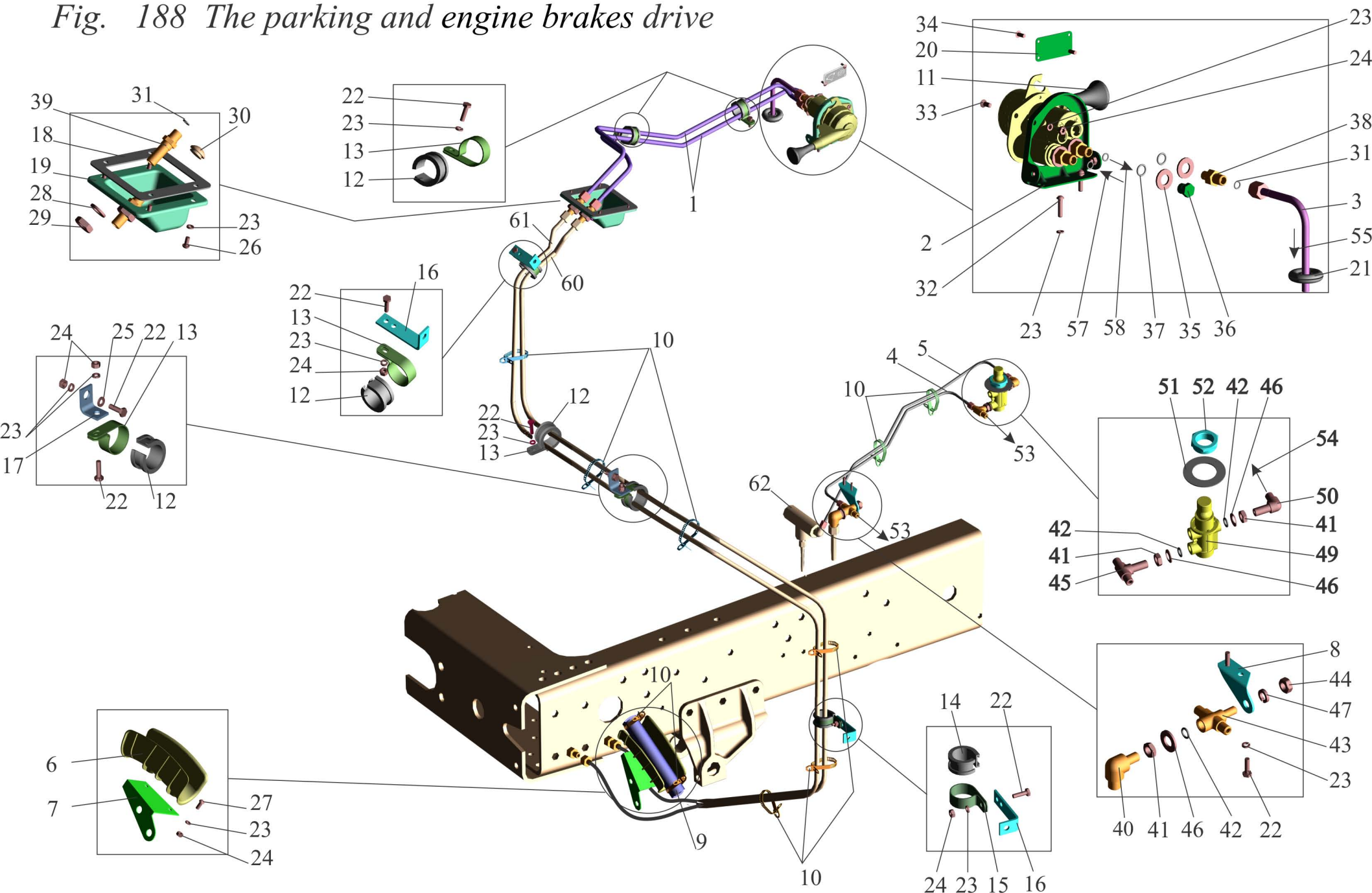
Рис. 188 Привод стояночного и моторного тормоза
