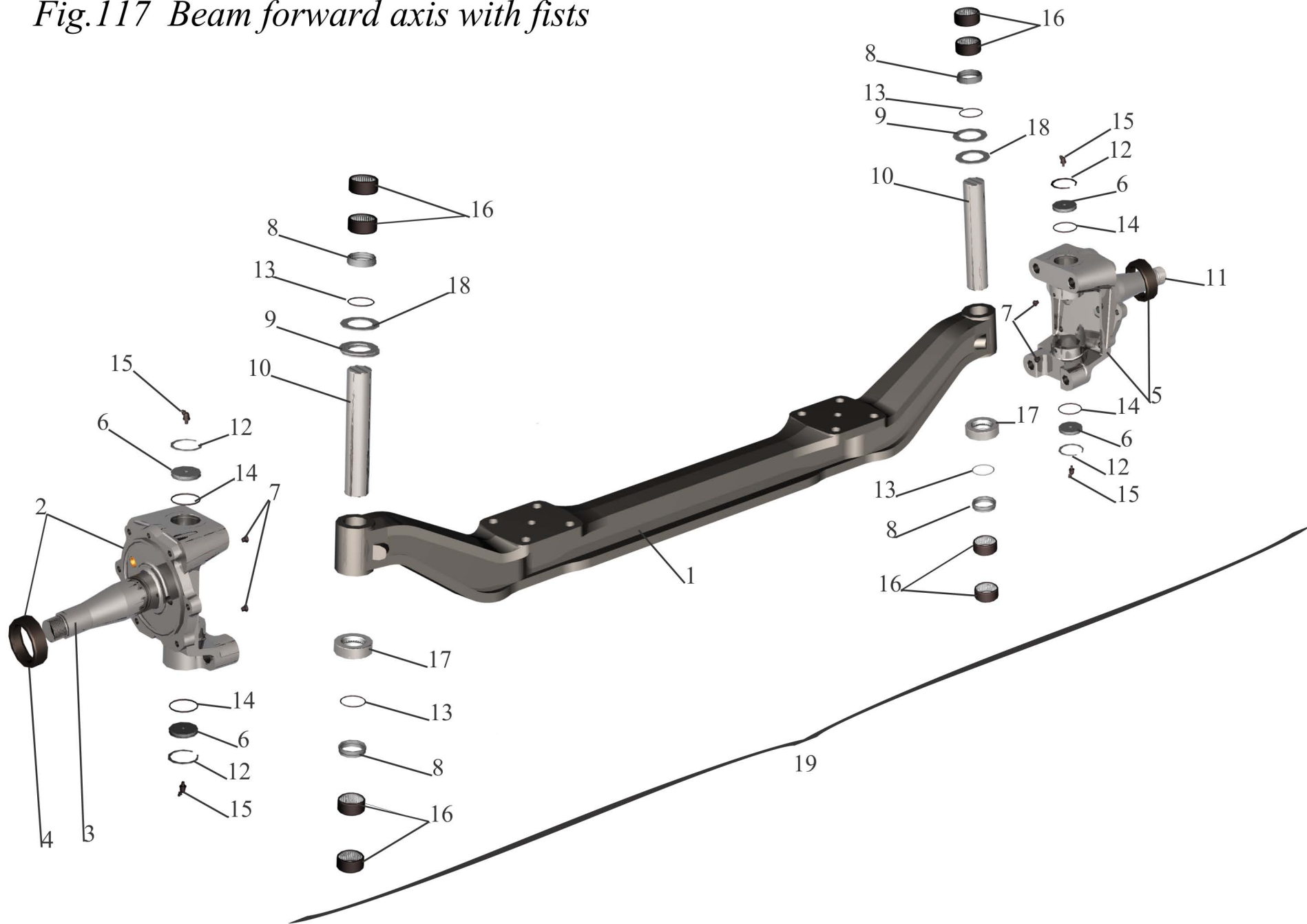
рис. 117 Балка передней оси с кулаками
