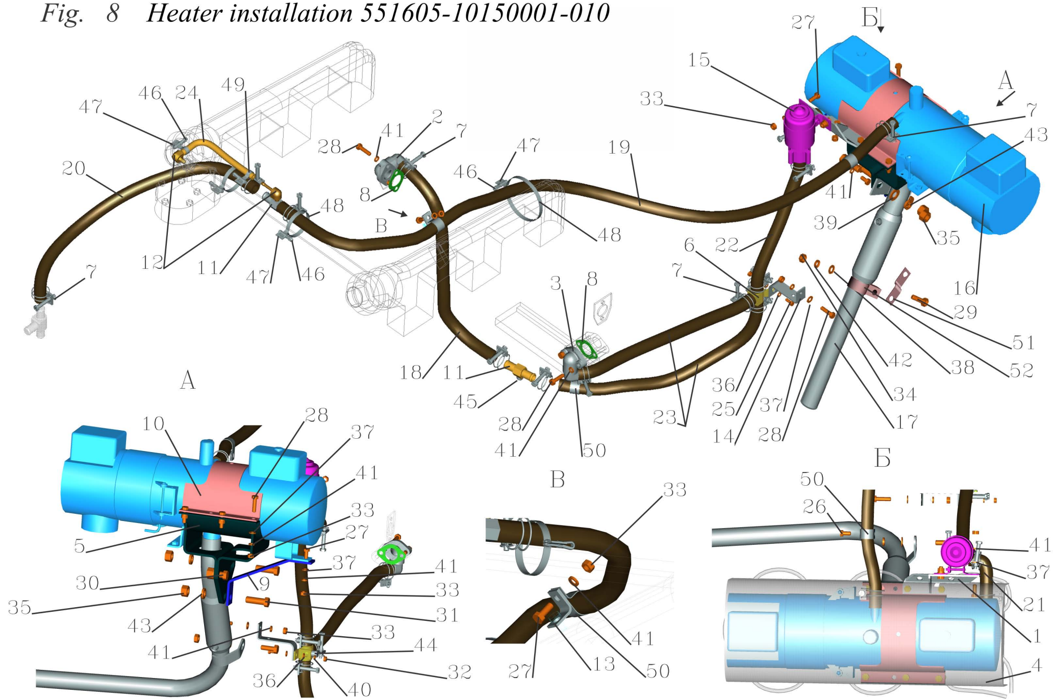
Рис. 8 Установка подогревателя 551605-10150001-010
