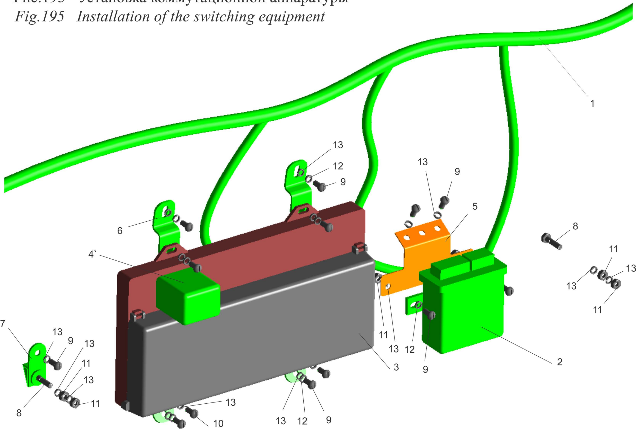
Рис.195 Установка коммутационной аппаратуры
