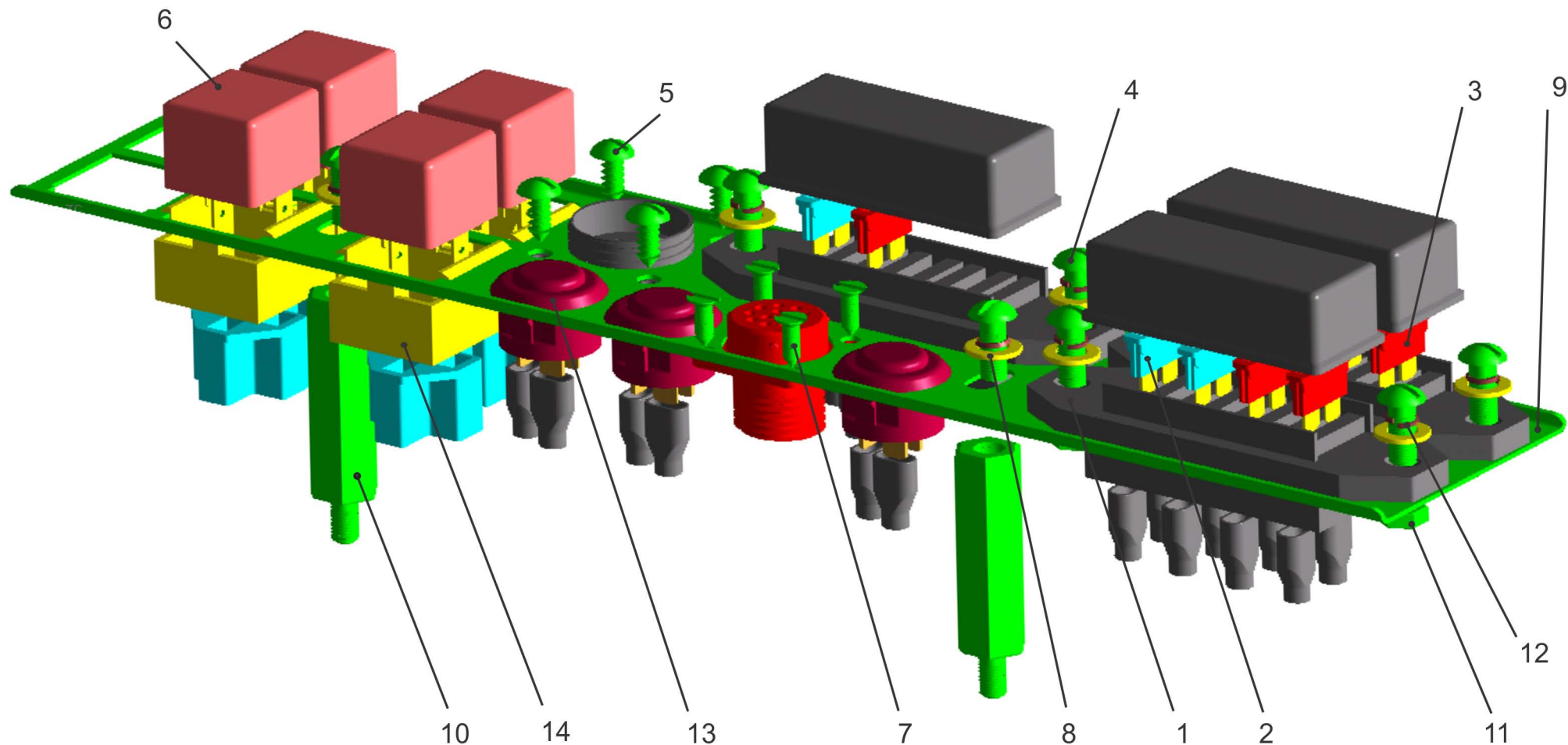
Рис.213 Панель реле и предохранителей автомобиля МАЗ-533602, 533603, 533605, 533608, 533702, 641708, 641705, 543403, 642208, 642205, 543208, 543205, 543202, 543203, 555102, 551605, 642505, 642508, 631705, 631708 vehicles
