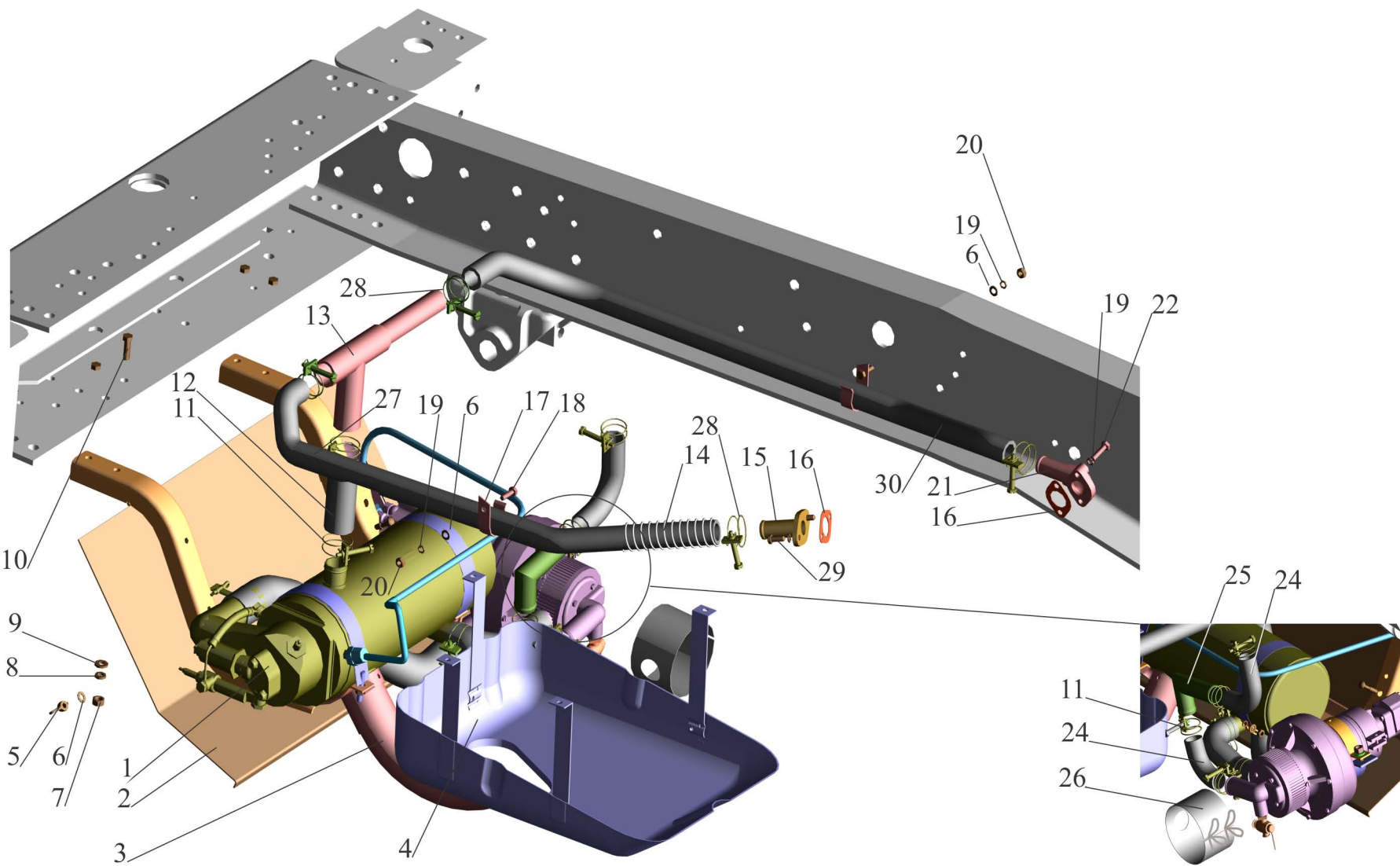
Рис. 12 Крепление предпускового подогревателя 543403-1015001. Fig. 12 Mounting of a prestarting heater 543403-1015001.
