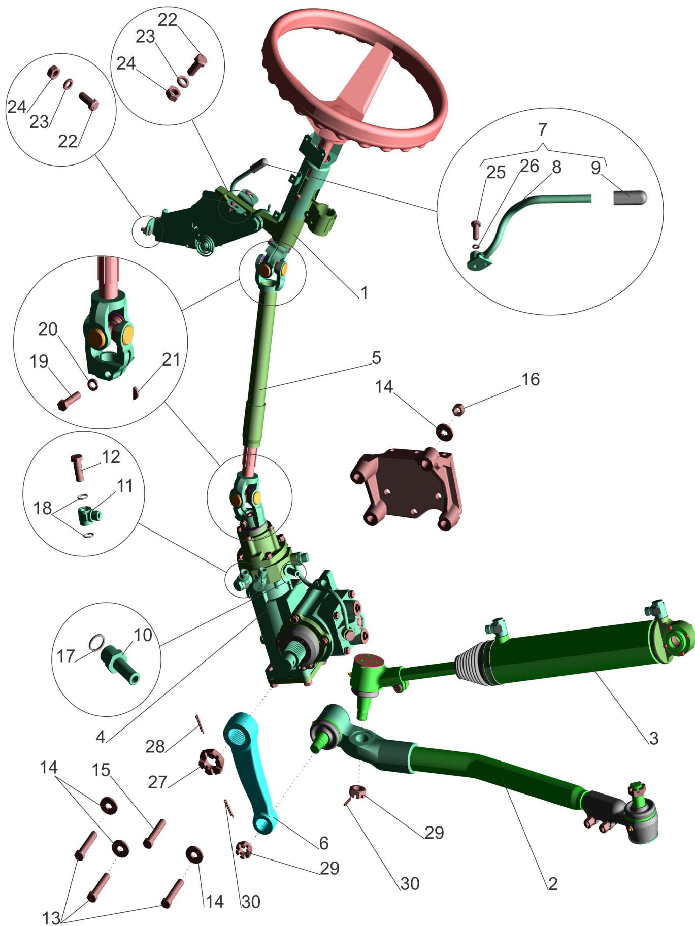
Рис.120 Установка рулевой колонки и рулевого механизма Fig.120 Steering column and steering mechanism mounting.
