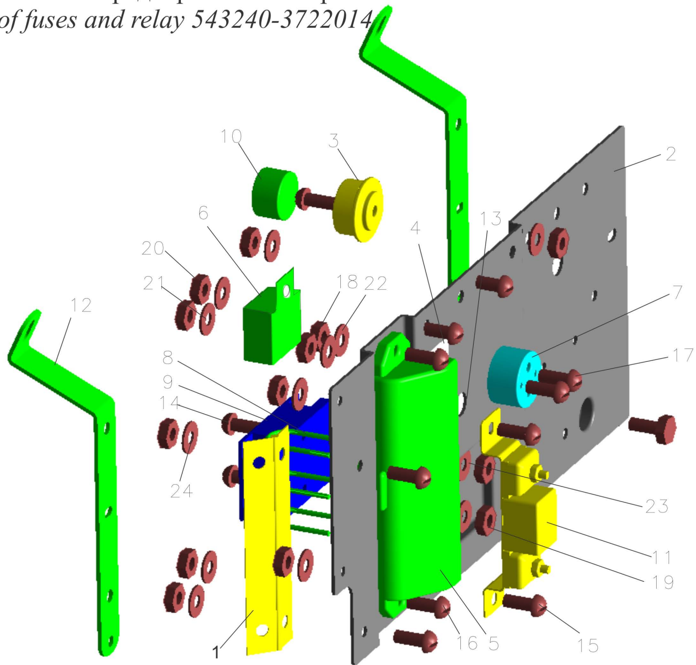
Рис.193 Панель блоков предохранителей и реле 543240-3722014
