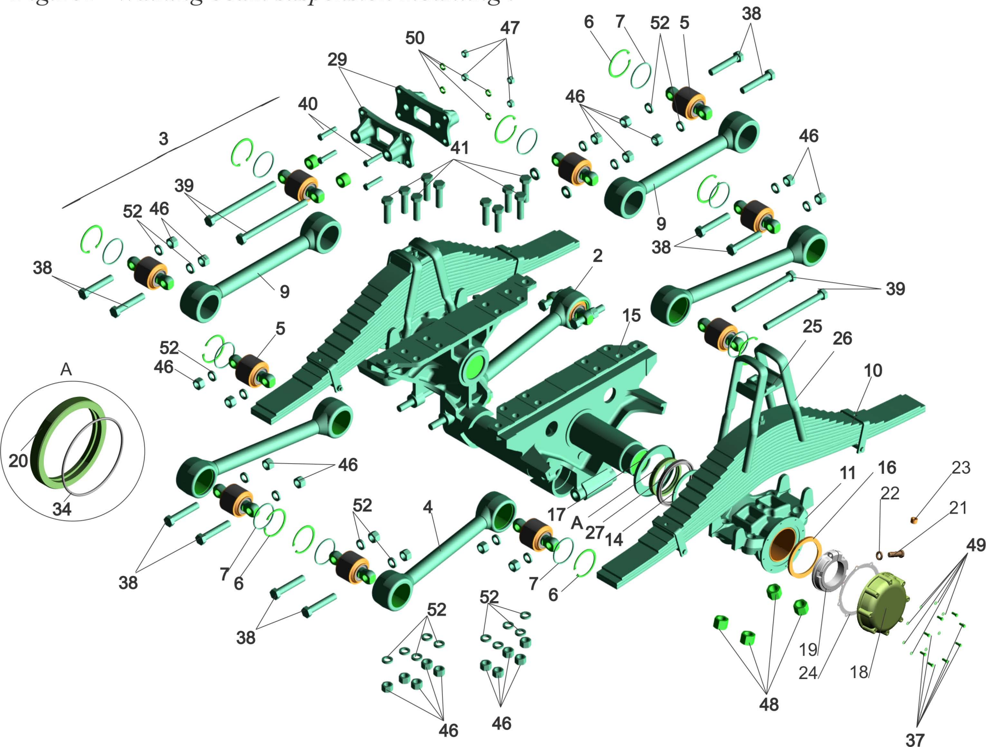
Рис.101 Подвеска балансирующая. Fig.101 Walking beam suspension mounting.
