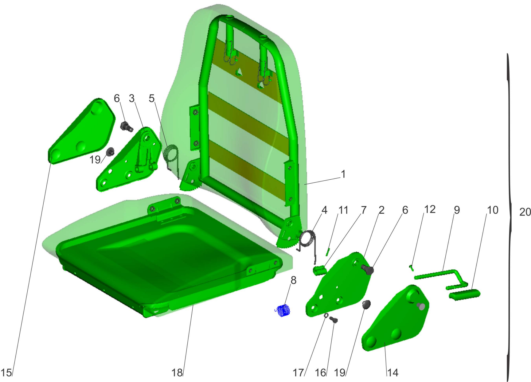
Рис.242 Подушка и спинка сиденья 6430-6800012, 6430-6810012*. Fig.242 Pad and back seat 6430-6800012, 6430-6810012*.
