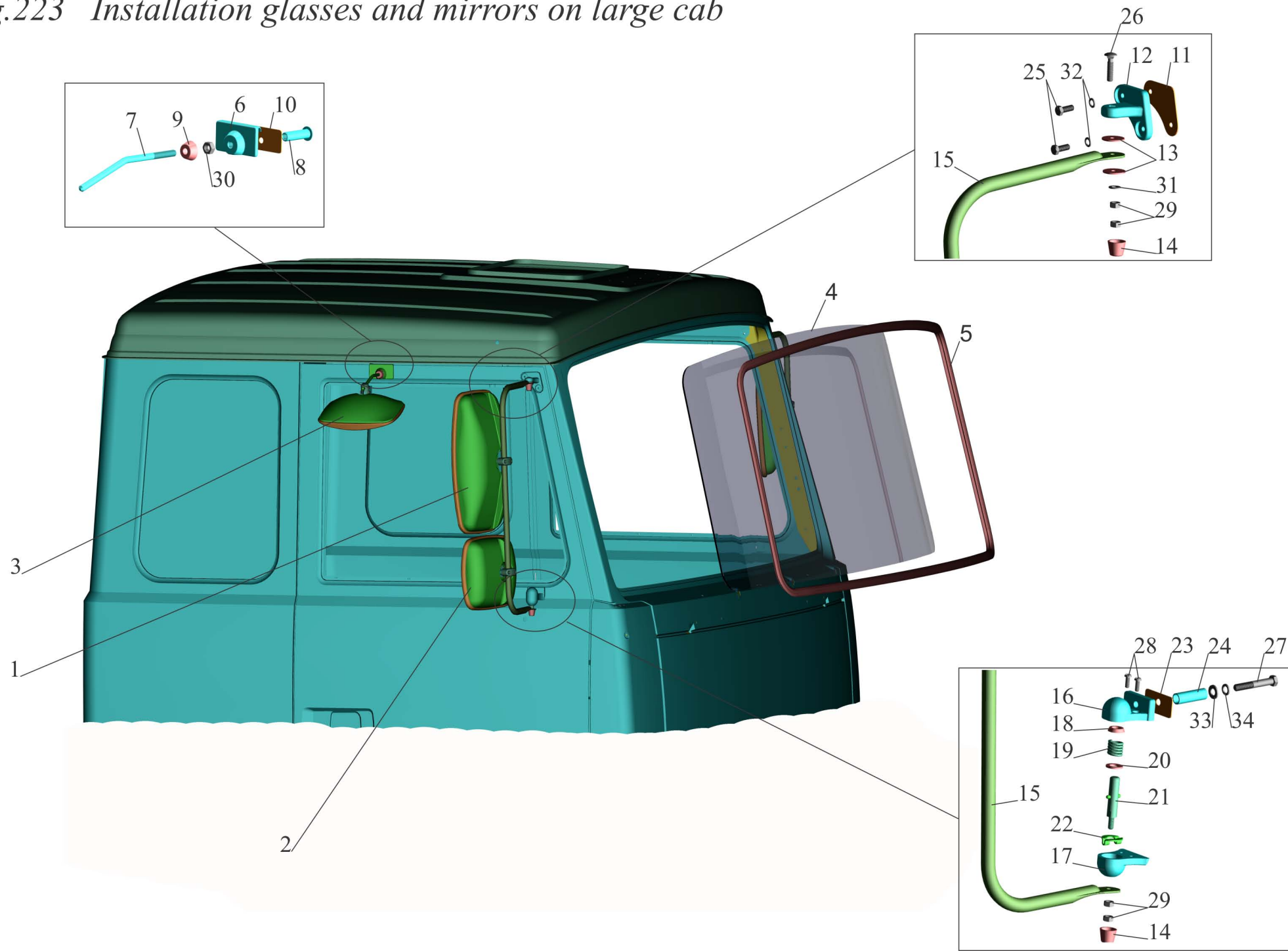
Рис.223 Установка стекол и зеркал на большую кабину
