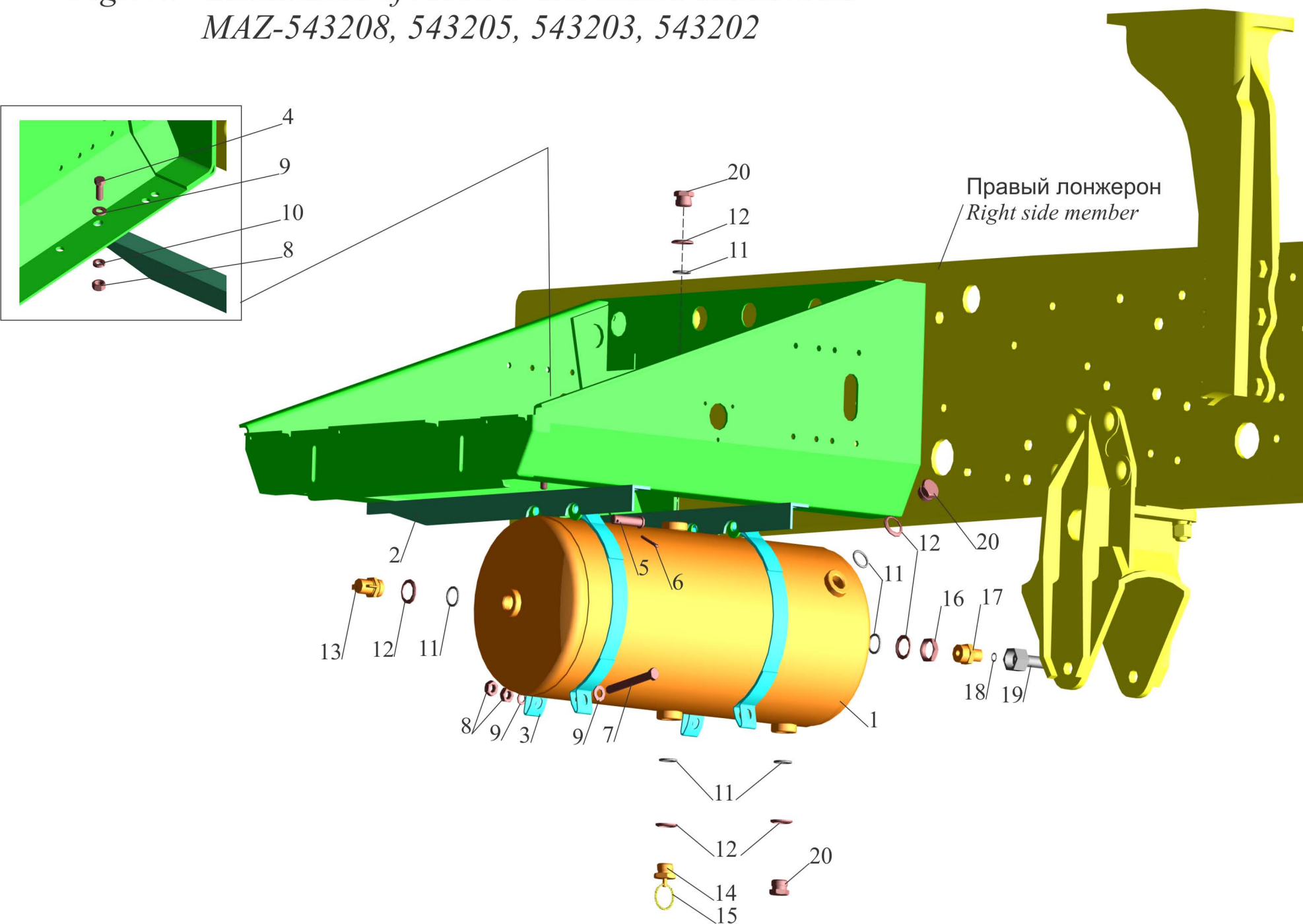
Рис.172 Установка ресивера и присоединительной арматуры МАЗ-543208, 543205, 543203, 543202
