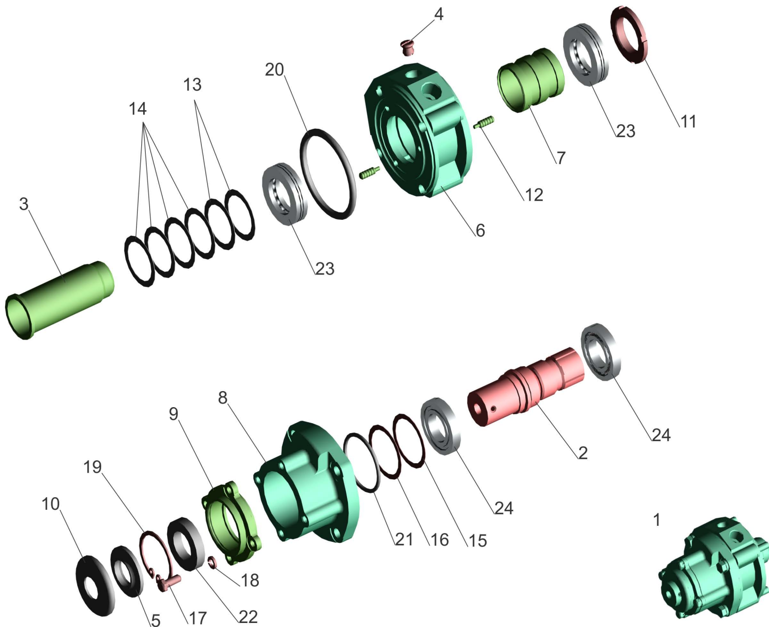
Fig.125 Divider
