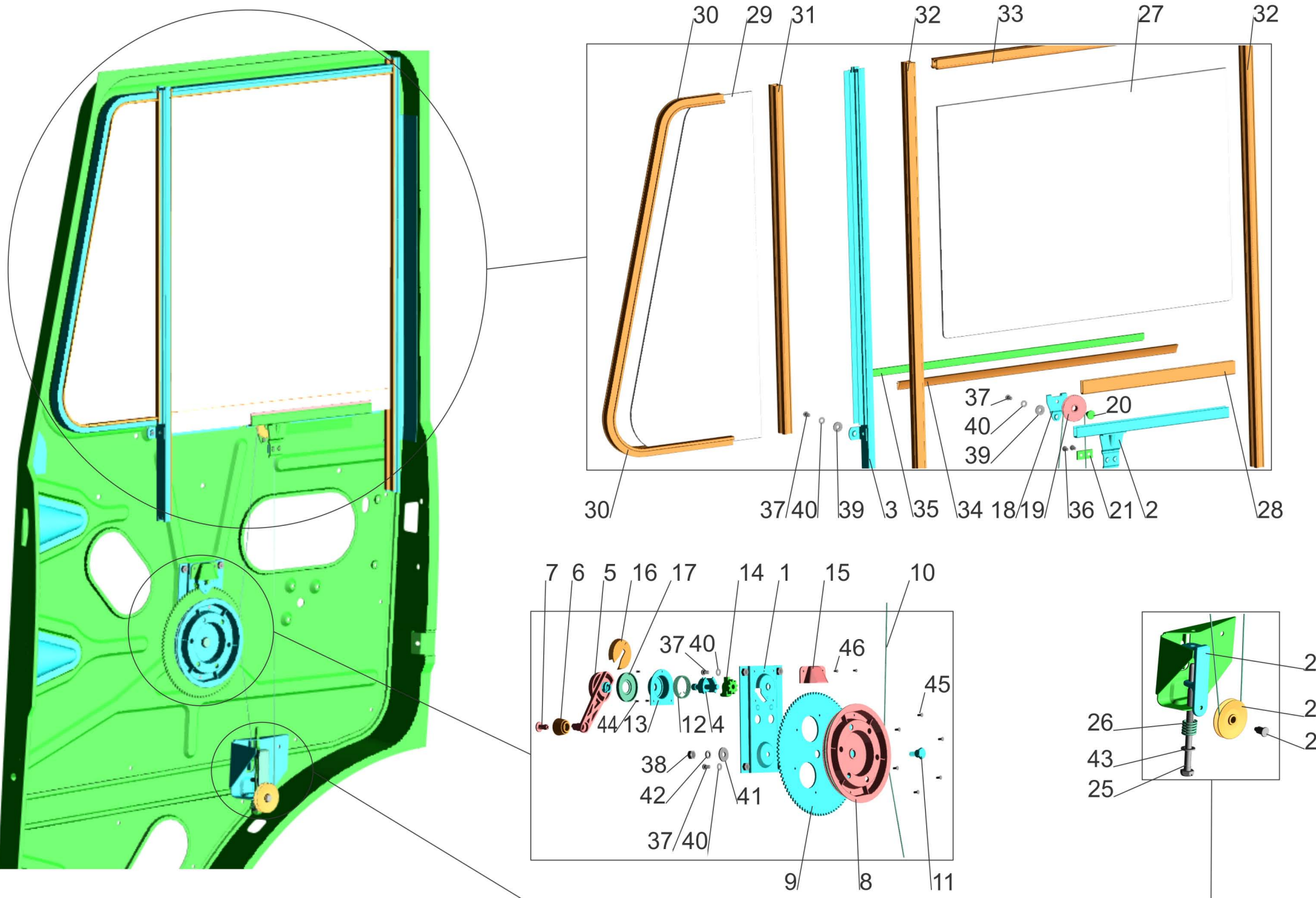
Рис.230 Установка стеклоподъемника и ручки стеклоподъемника Fig.230 Installation window regulator and window regulator handle
