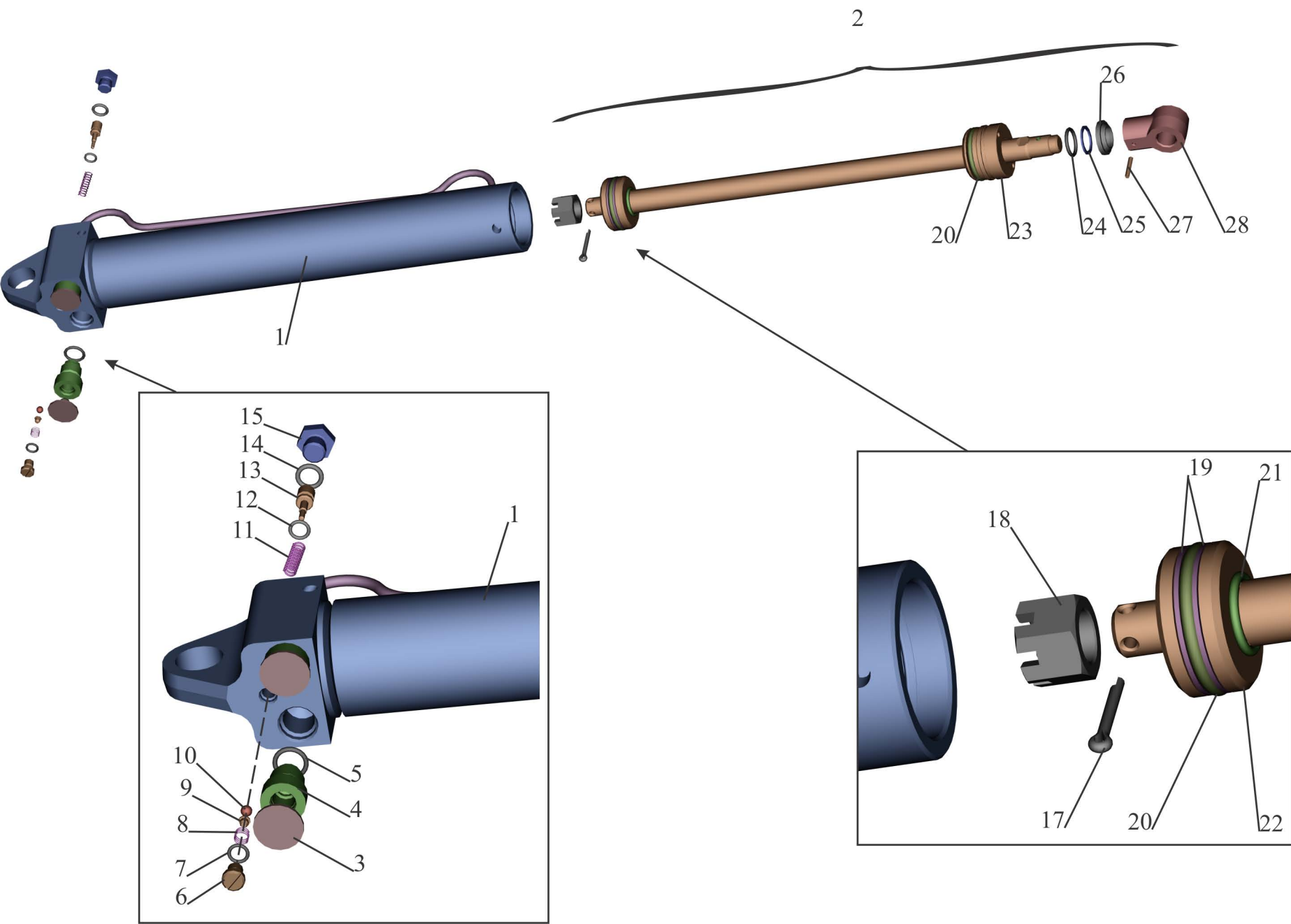
Рис. 221 Гидроцилиндр 64221-5003010 Fig. 221 Hydrocylinder 64221-5003010
