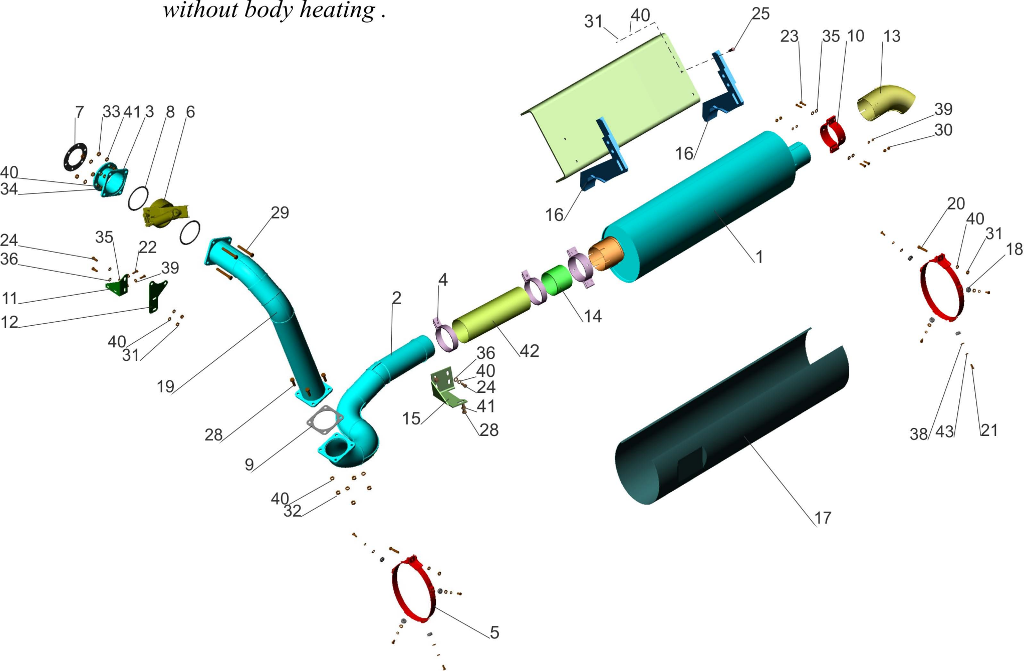
Рис.40 Установка системы выпуска отработавших газов МАЗ-551605 с КП МАЗ-543205 без обогрева кузова
