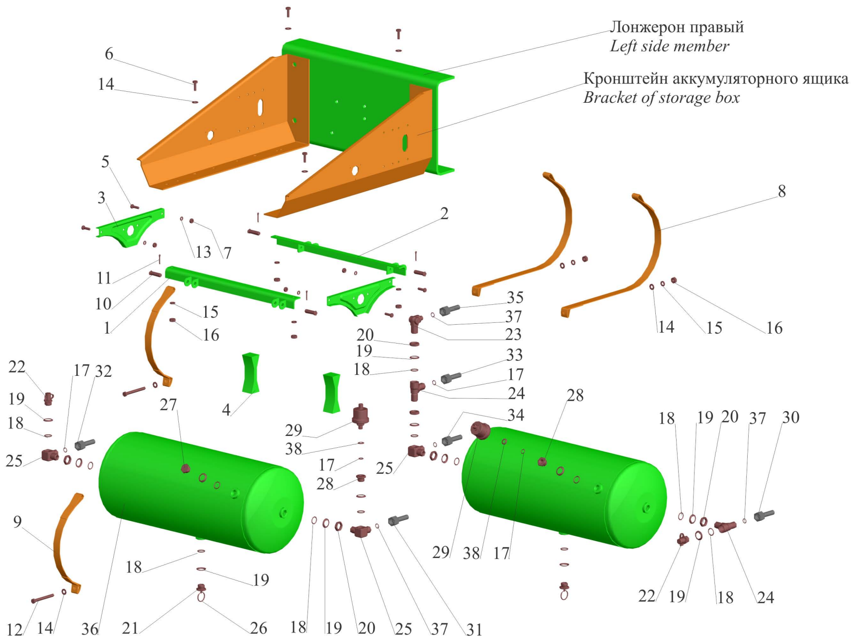
Рис.166 Установка ресивера и присоединительной арматуры МАЗ-642208, 642205. Fig.166 Installation of receiver and attach accessories MAZ-642208, 642205.
