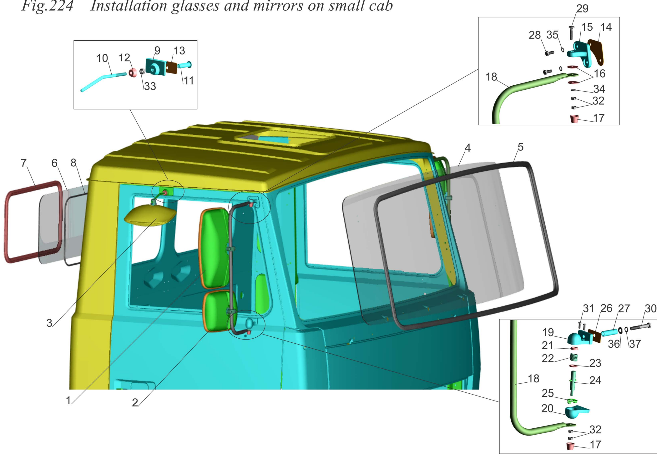
Рис.224 Установка стекол и зеркал на малую кабину
