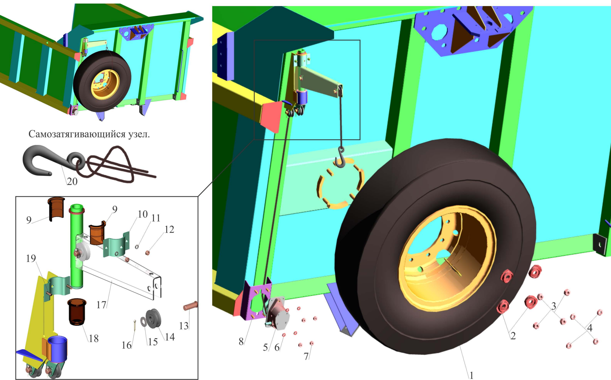
Рис.109 Установка запасного колеса МАЗ-551603, 551605 (5516-3100001-10). Fig.109 Installation spare wheel MAZ-551603, 551605 (5516-3100001-10).
