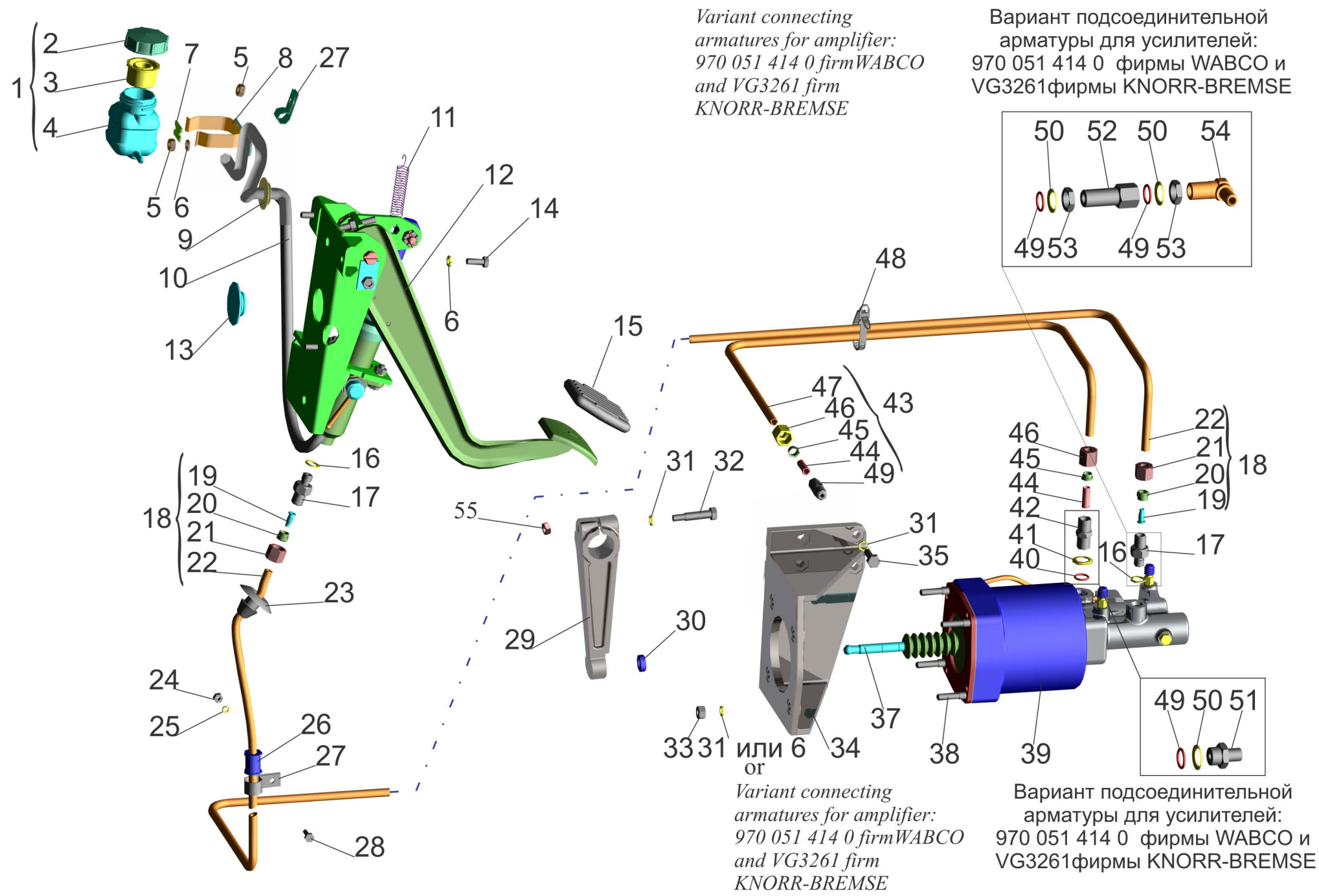
Рис.48 Механизм управления сцеплением 64229-1600005-012, 64229-1600005-013, 64229-014 Fig.48 Clutch control mechanism 64229-1600005-012, 64229-1600005-013, 64229-014
