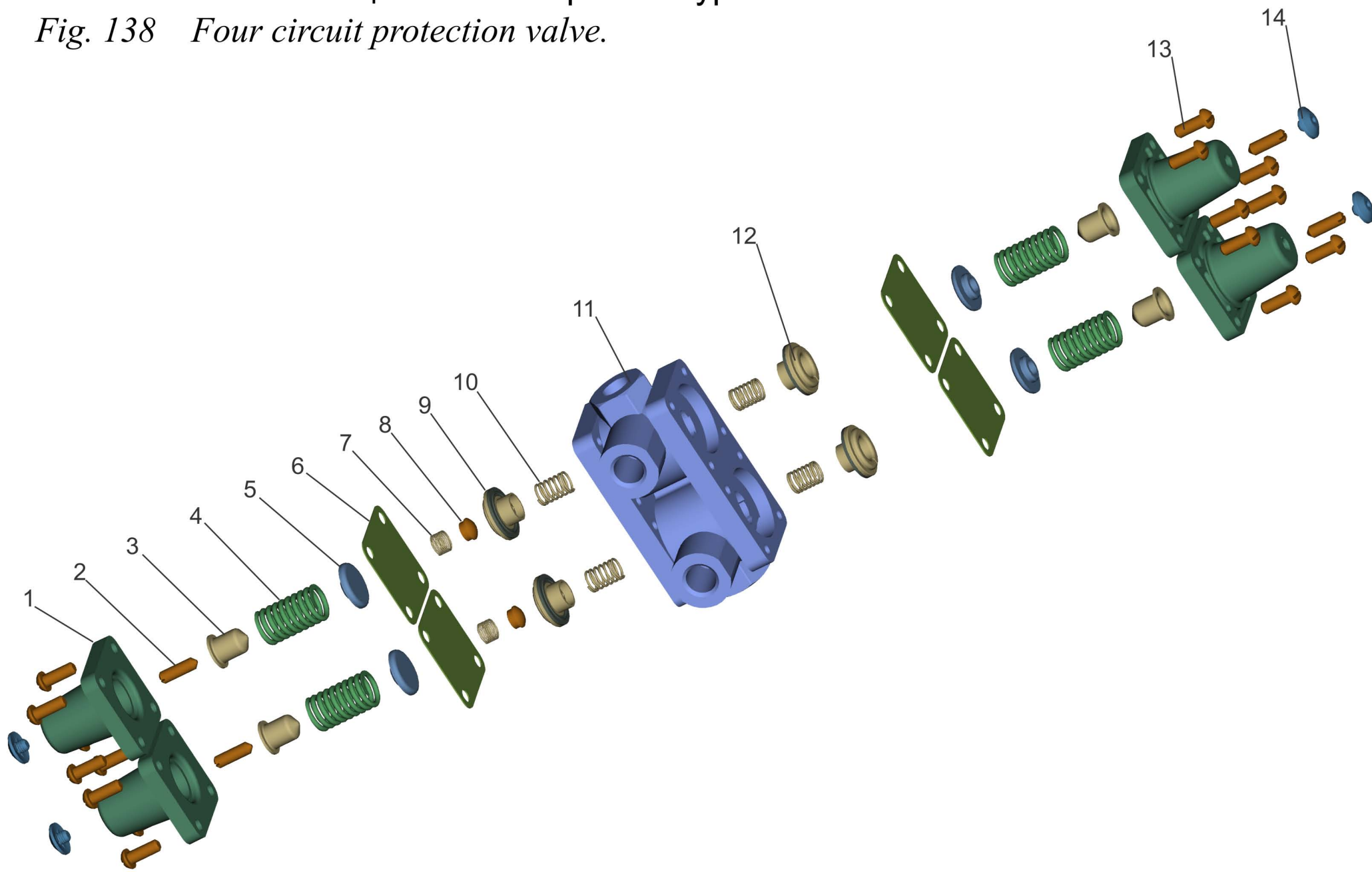
Рис. 138 Клапан защитный четырехконтурный.
