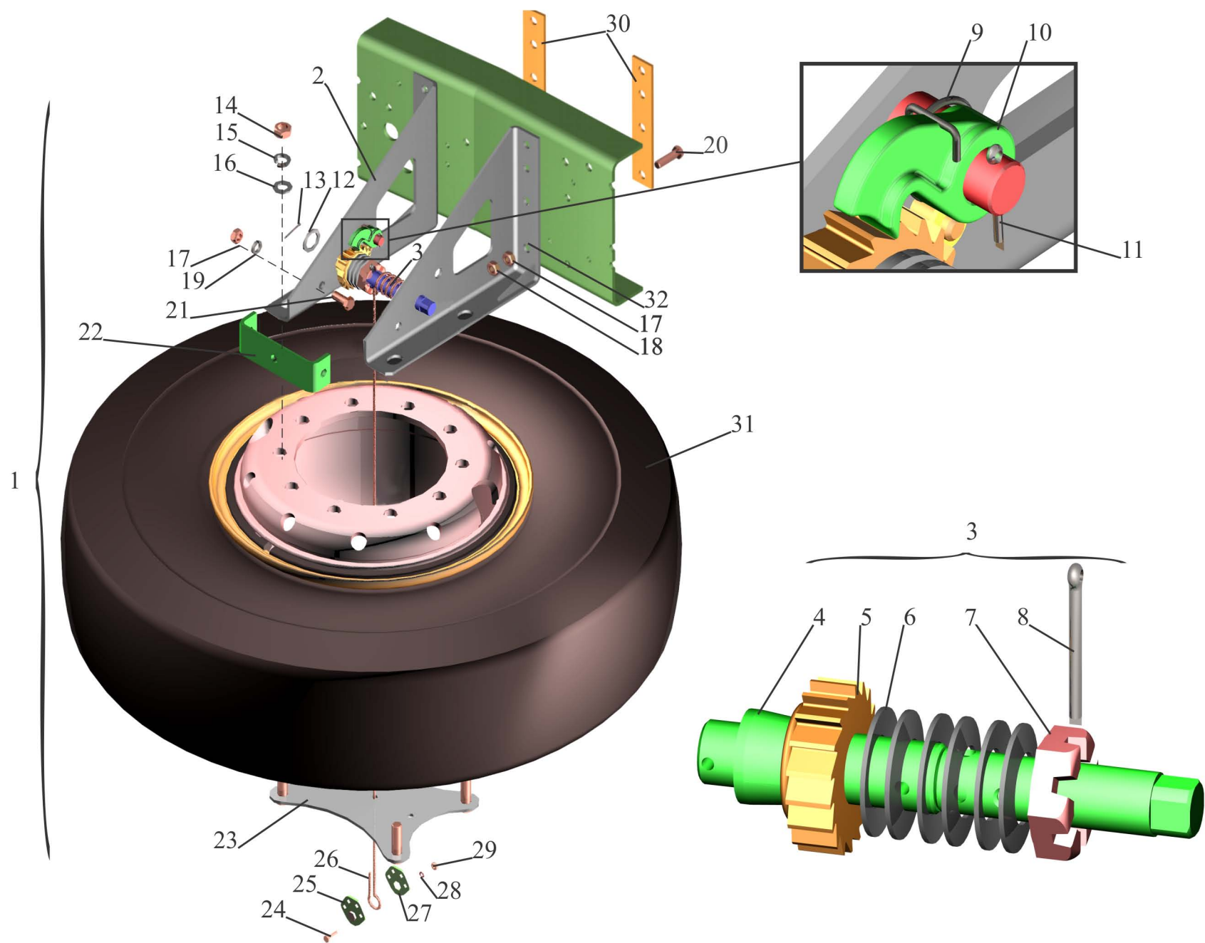
Рис. 107 Установка запасного колеса МАЗ-543208, 543205, 543203, 543202, 555102. Fig. 107 Installation spare wheel MAZ-543208, 543205, 543203, 543202, 555102.
