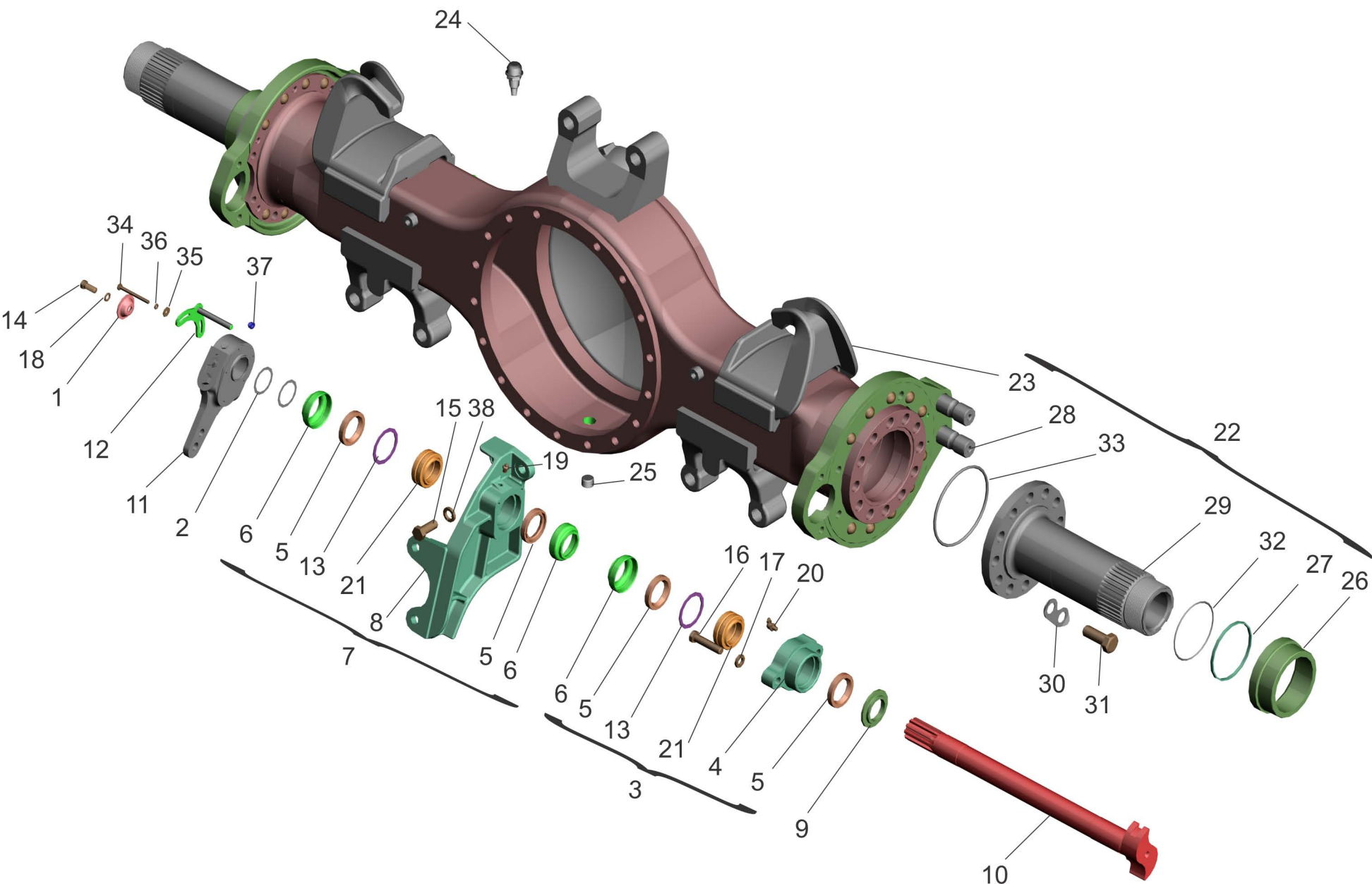
Рис.78 Мост средний. Картер моста с приводом тормозного механизма. Fig.78 Intermediate axle. Axle housing with brake gear drive.
