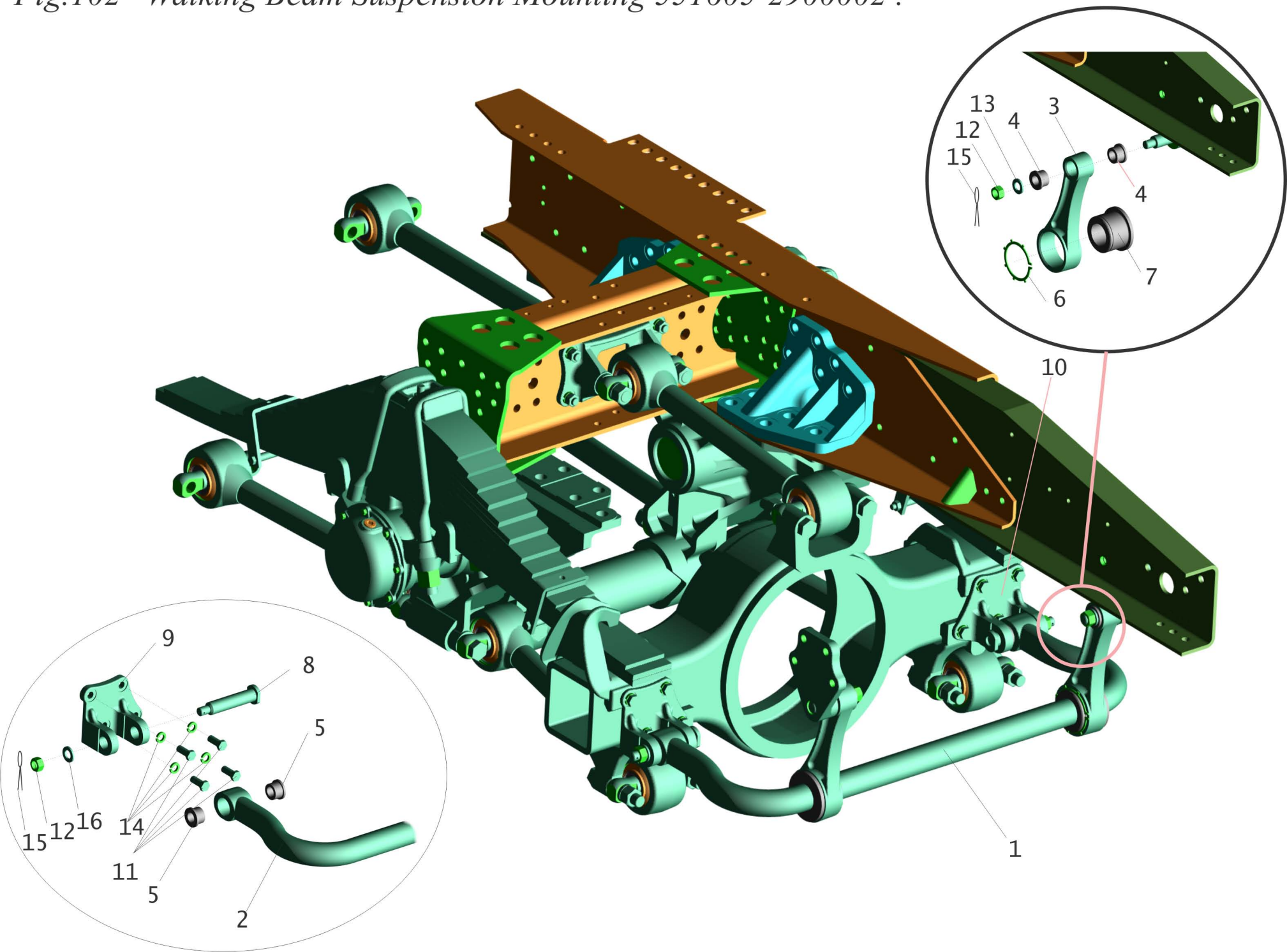
Рис.102 Подвеска балансирная 551605-2900002 Fig.102 Walking Beam Suspension Mounting 551605-2900002 .
