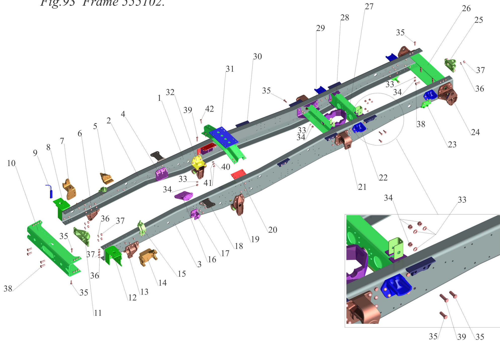
Рис.93 Рама 555102.
