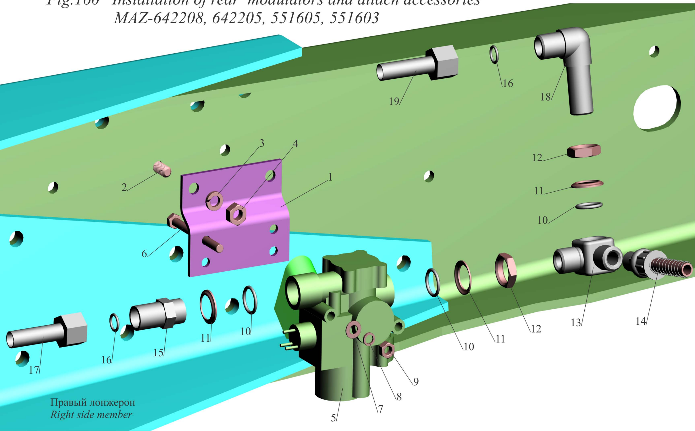
Рис.160 Установка задних модуляторов и присоединительной арматуры МАЗ-642208, 642205, 551605, 551603
