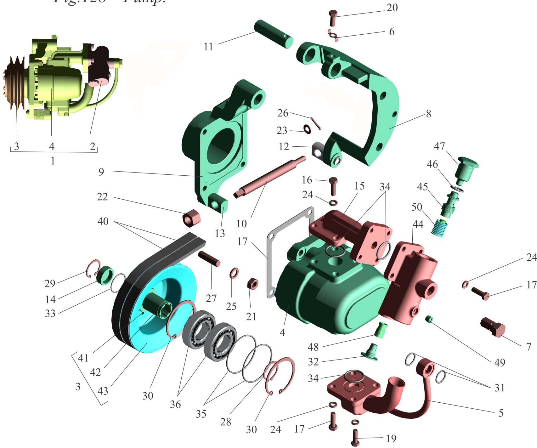
Рис.128 Насос. Fig.128 Pump.
