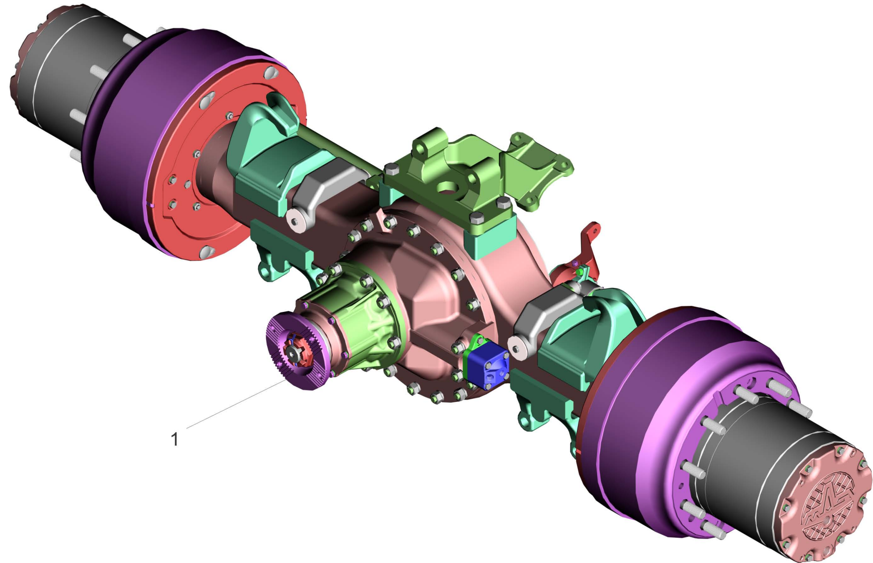
Рис. 61 Мост задний Fig. 61 Rear Axle
