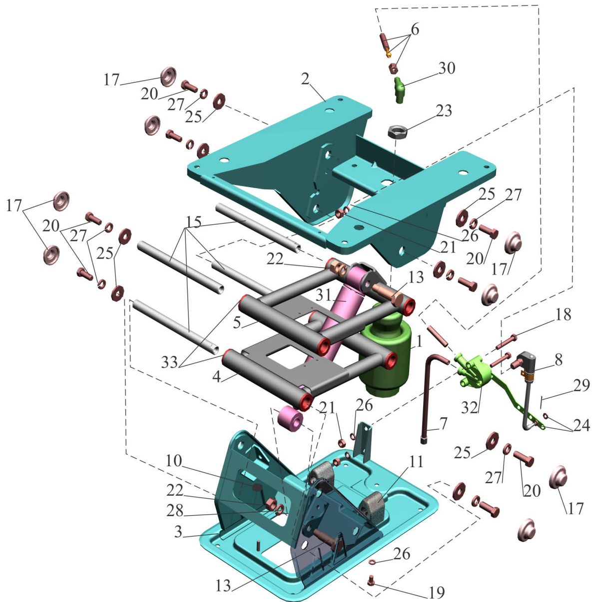
Рис. 239 Подставка сидения с пневмооборудованием 6430-6807006-010. Fig. 239 Seat support with pneumatic equipment 6430-680706-010.
