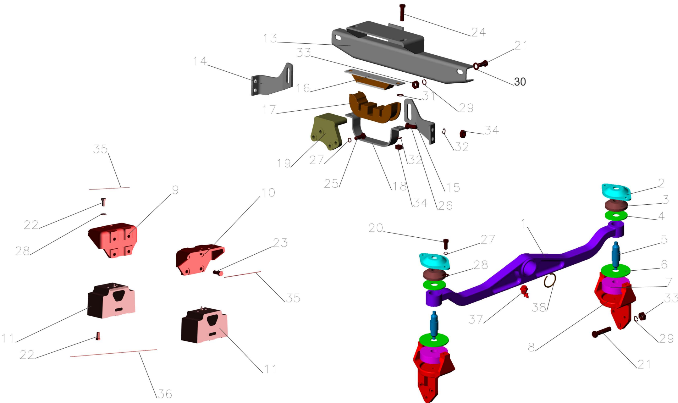
Рис.2 Крепление двигателя на автомобилях МАЗ-642205, МАЗ-543205 с КП ЯМЗ-238М. Fig.2 Mounting of engine on vehicles MAZ-642205, MAZ-543205 with gear box YaMZ-238M.
