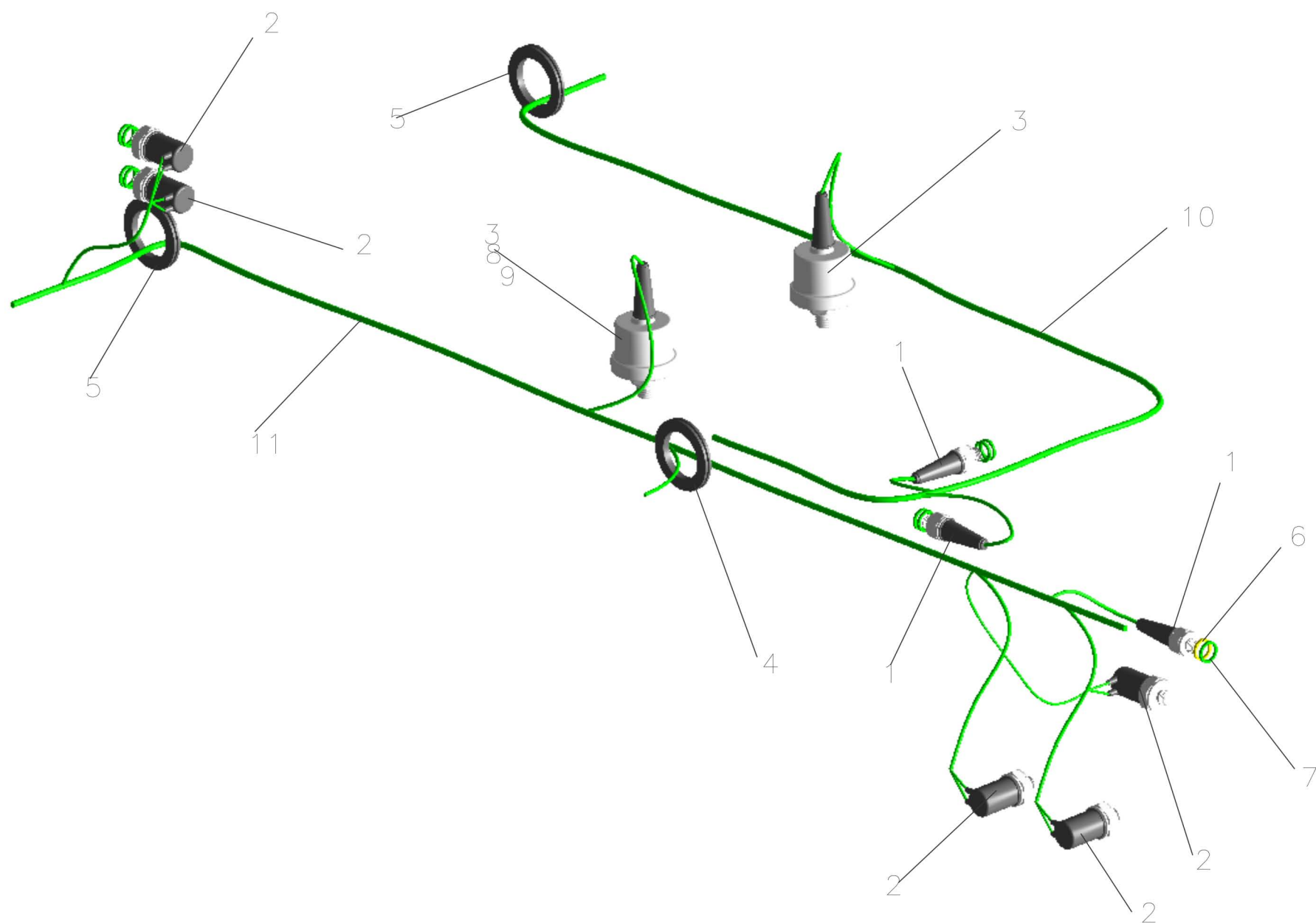
Рис.189 Установка датчиков на шасси Fig.189 Installation of sensors on chassis
