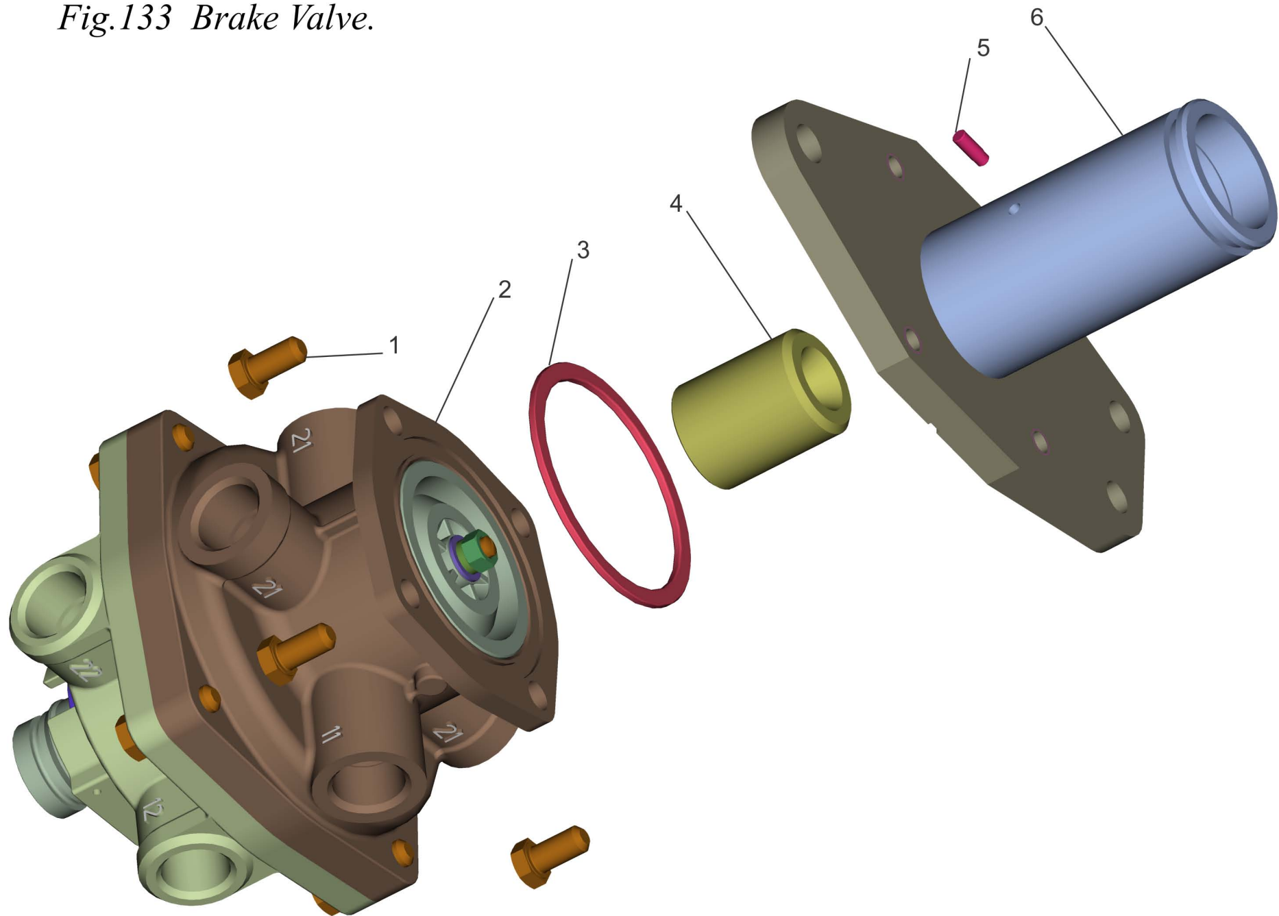
Рис.133 Тормозной кран.
