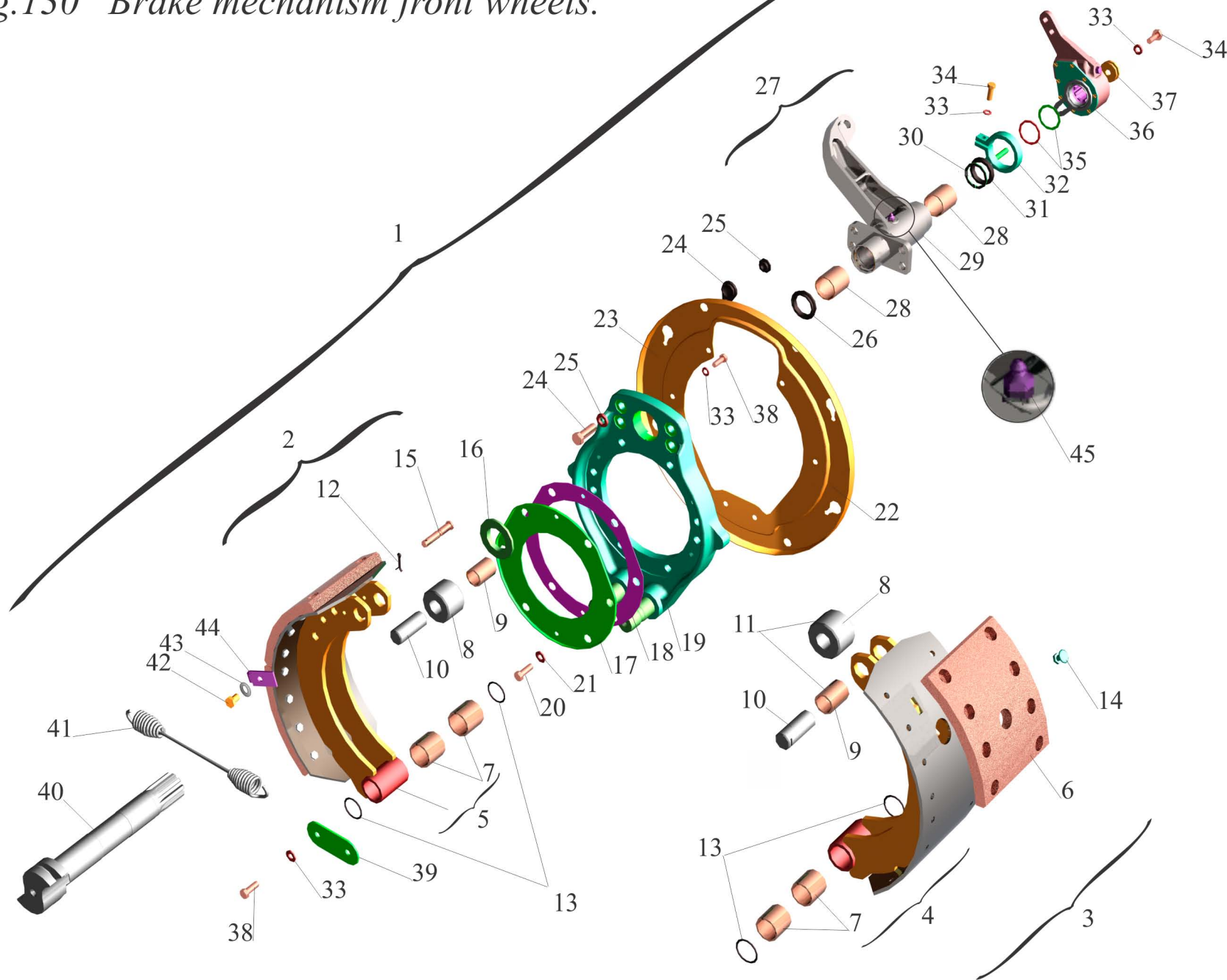
Рис.130 Тормозной механизм передних колес
