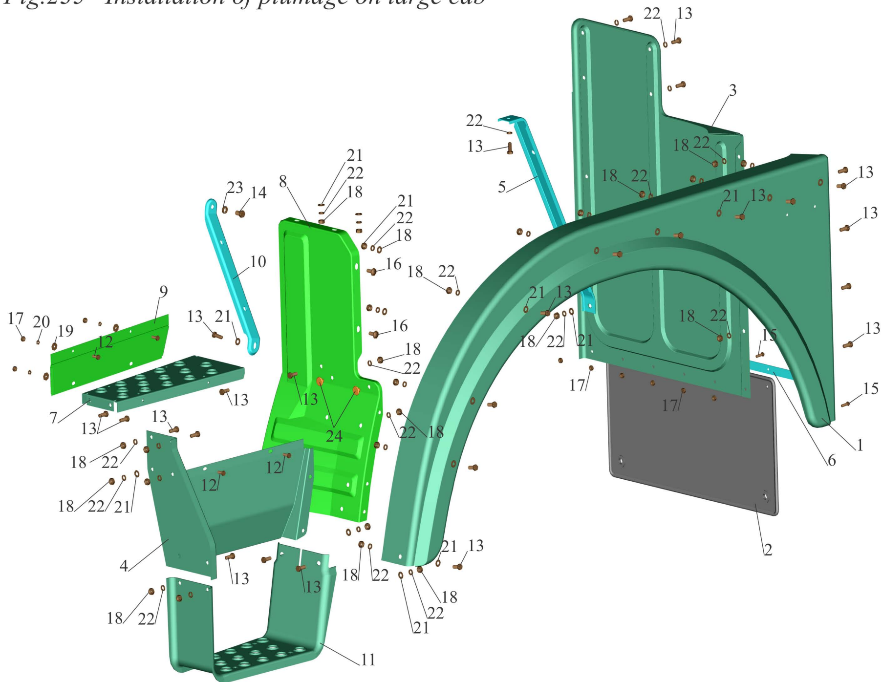
Рис.235 Установка оперения на большую кабину Fig.235 Installation of plumage on large cab
