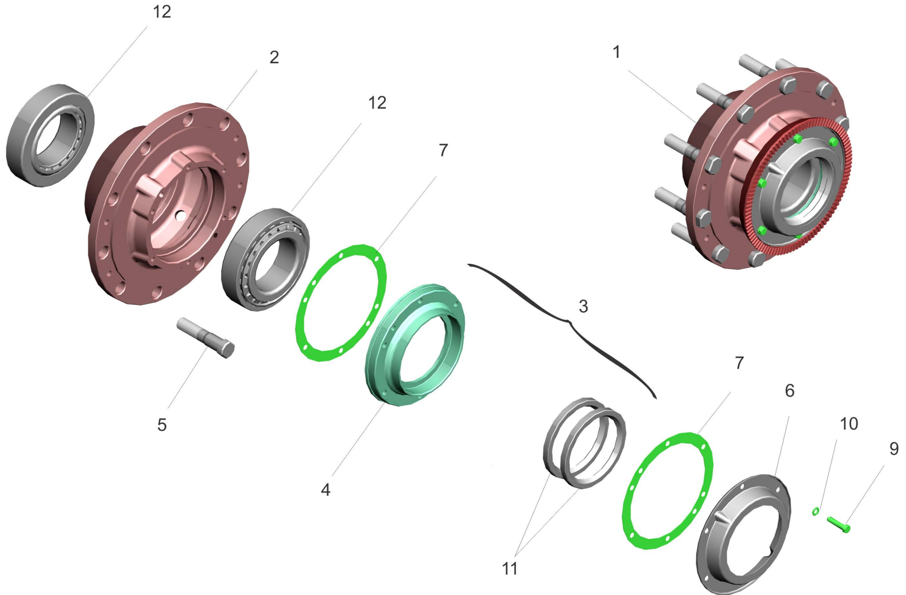
Рис.86 Ступица среднего моста. Fig.86 Intermediate Axle Hub.
