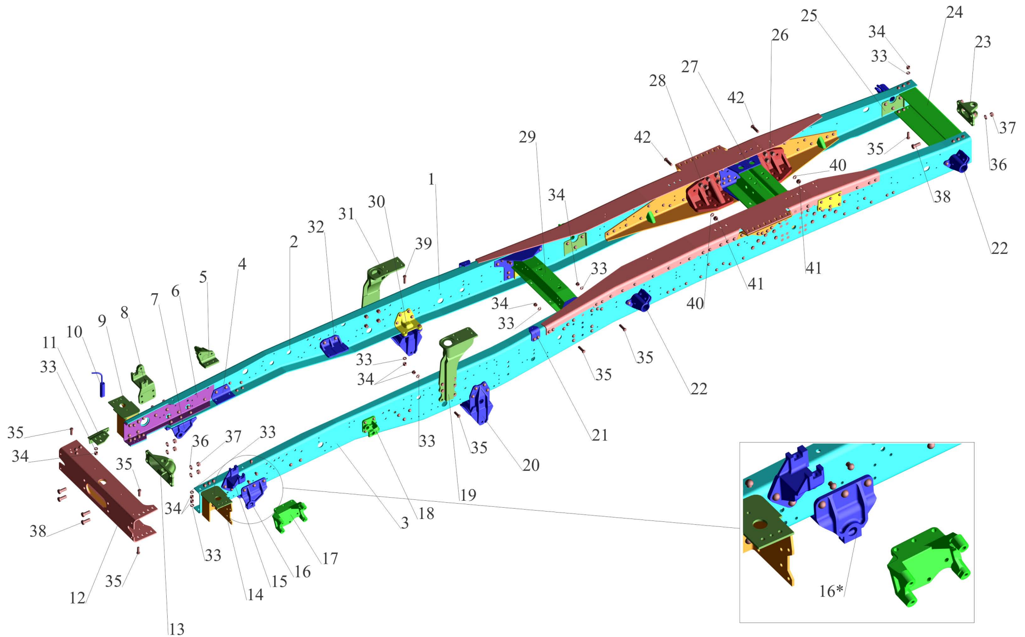
Рис.89 Рама 642208, 642205-рессорная подвеска Fig.89 Frame 642208, 642205-spring suspension
