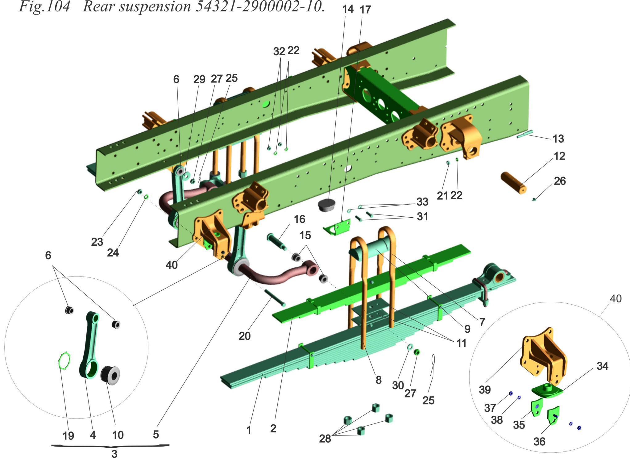
Рис.104 Подвеска задняя 54321-2900002-10.
