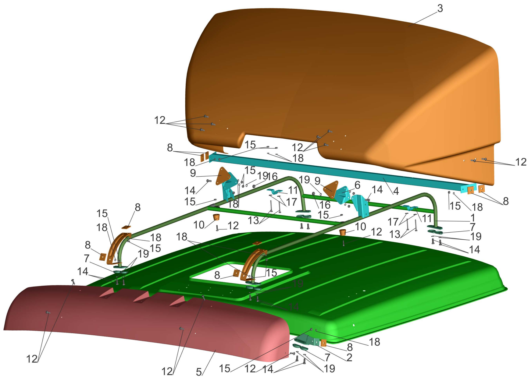
Рис.234 Установка обтекателей Fig.234 Installation of fairing
