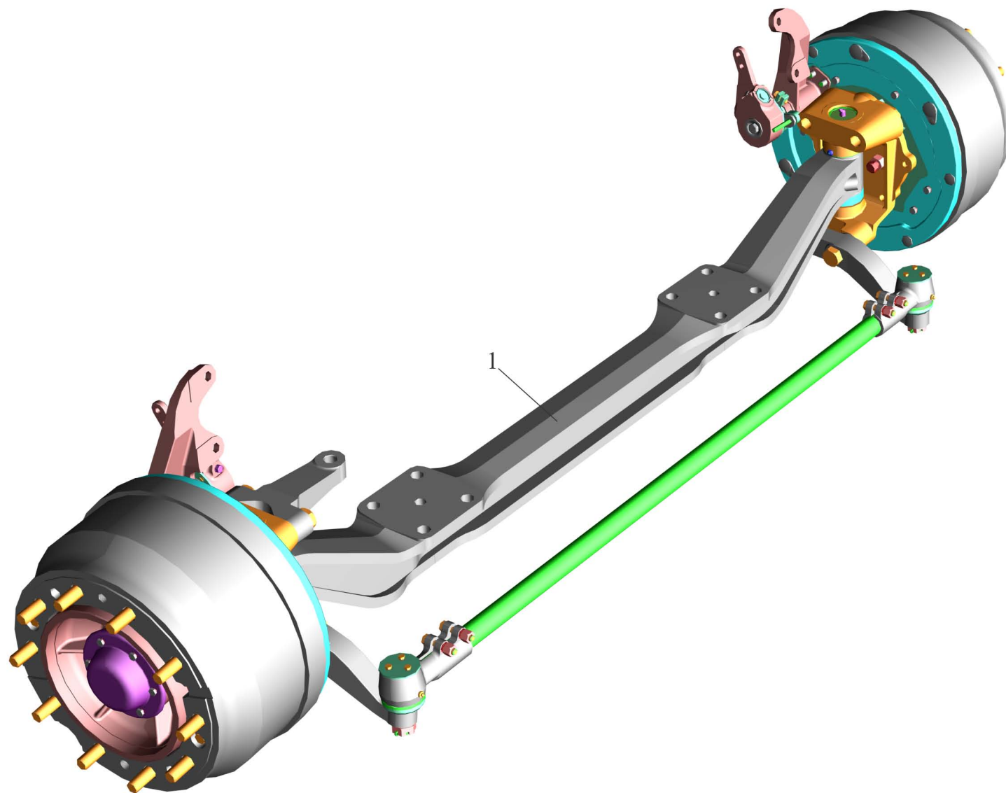
Рис.114 Передняя ось . Fig.114 Front axle.
