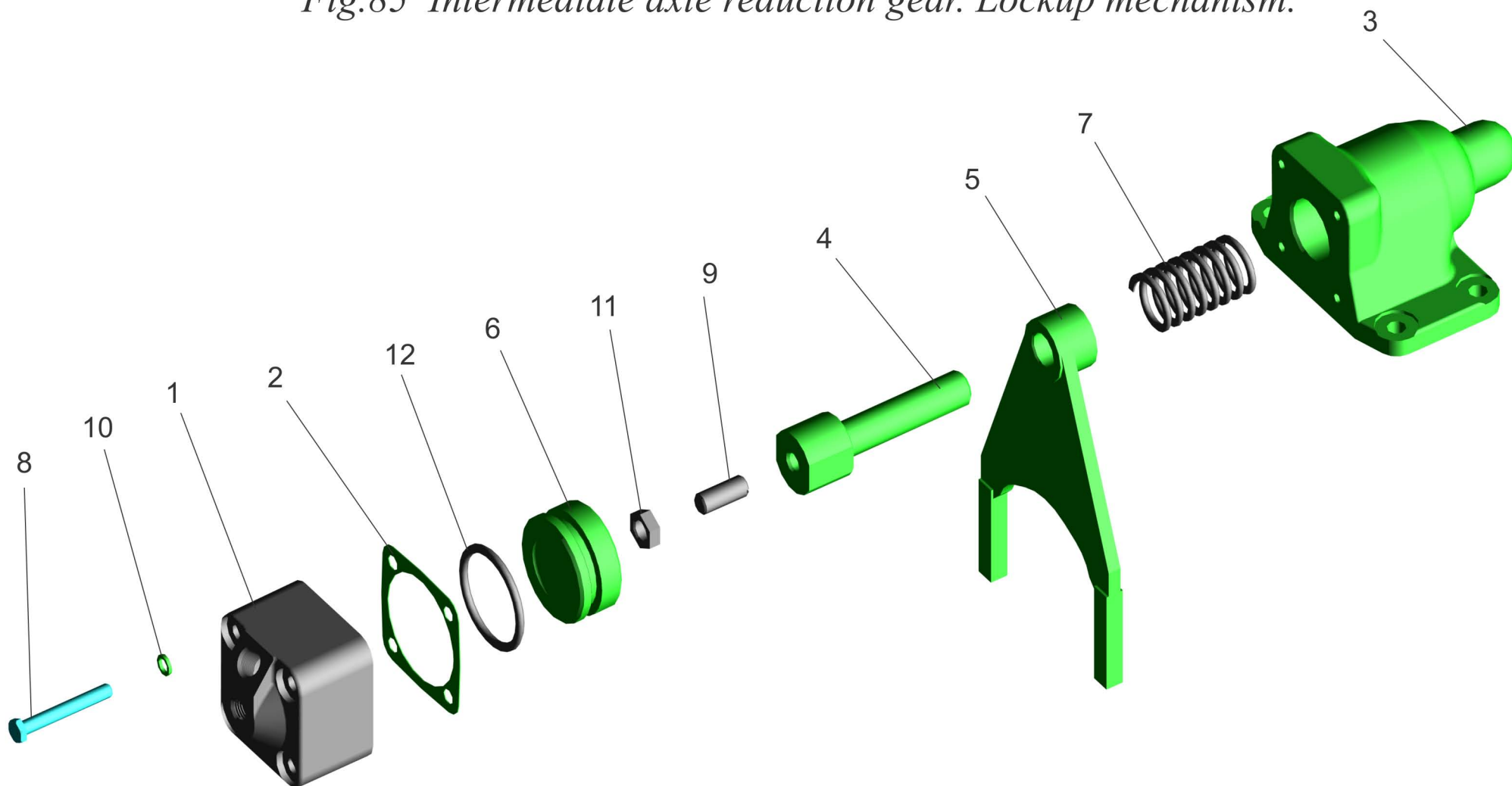
Рис.85 Редуктор среднего моста. Механизм блокировки. Fig.85 Intermediate axle reduction gear. Lockup mechanism.
