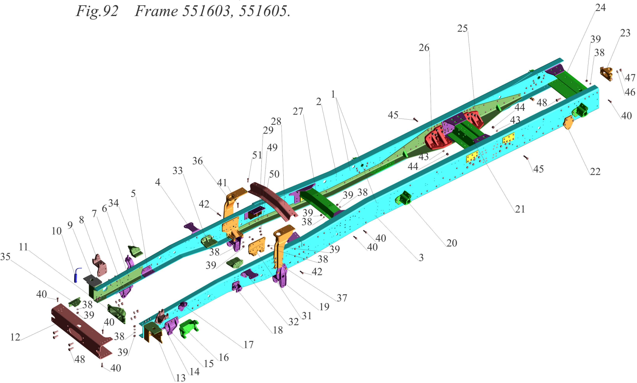
Рис.92 Рама 551603, 551605.
