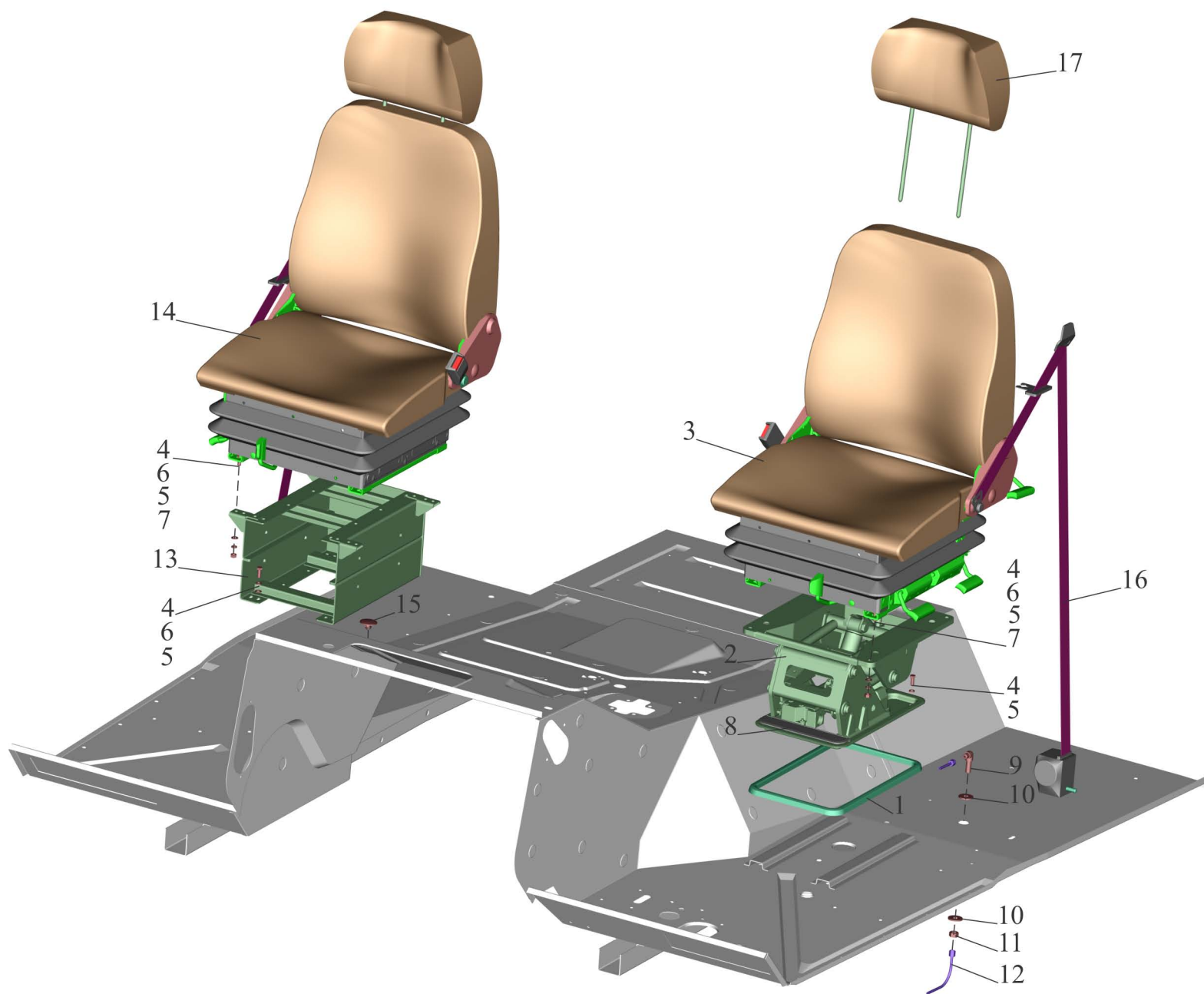
Рис.237 Установка и пневмопитание сидений 5433-6800006 Fig.237 Installation and pneumatic supply of seat 5433-6800006
