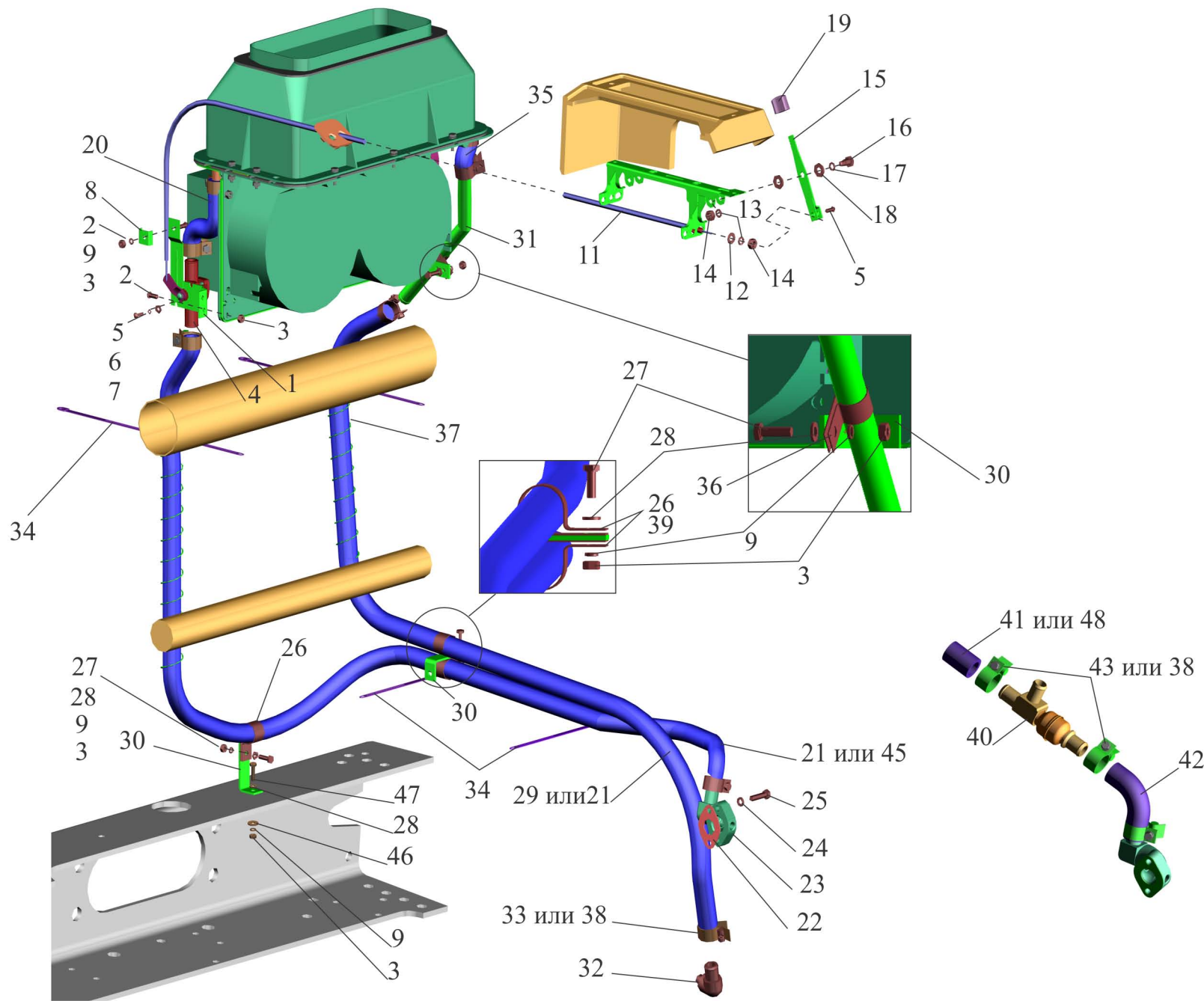
Рис. 245 Установка шлангов и крана управления отопителем Fig. 245 Installation of hoses and control cock of heater
