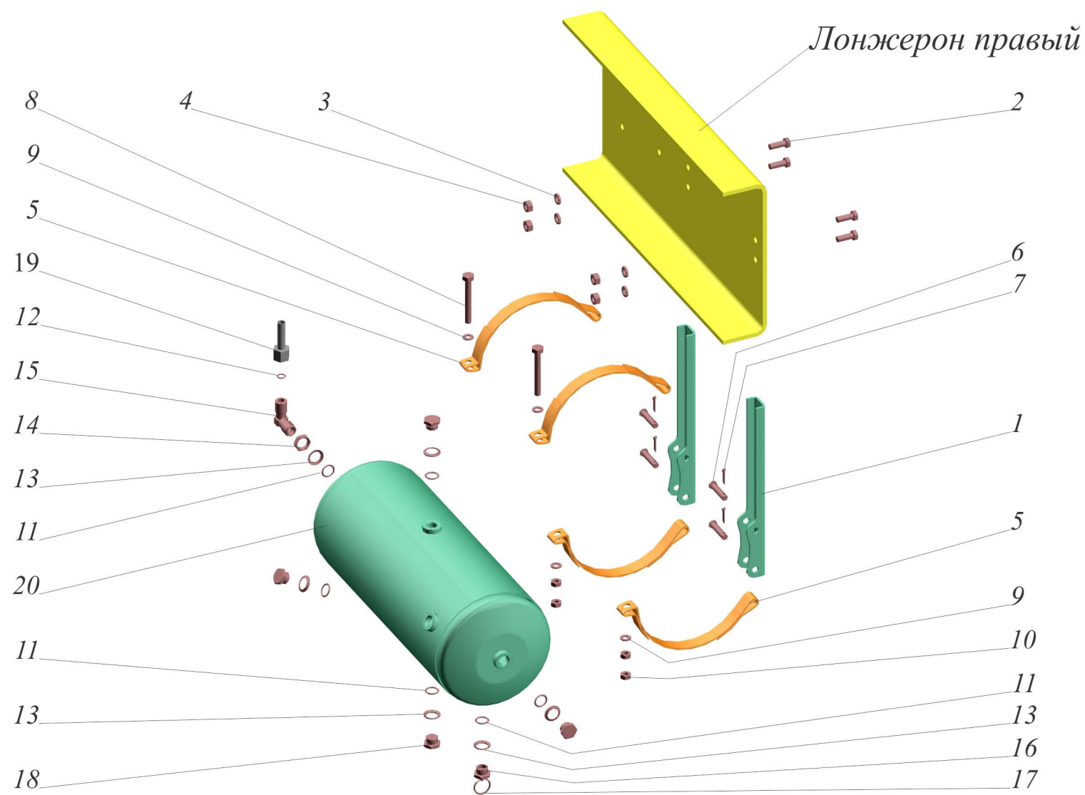
Рис.168 Установка ресивера и соединительной арматуры на МАЗ-642208, 642205. Fig.168 Installation of receiver and accessories on MAZ-642208, 642205.
