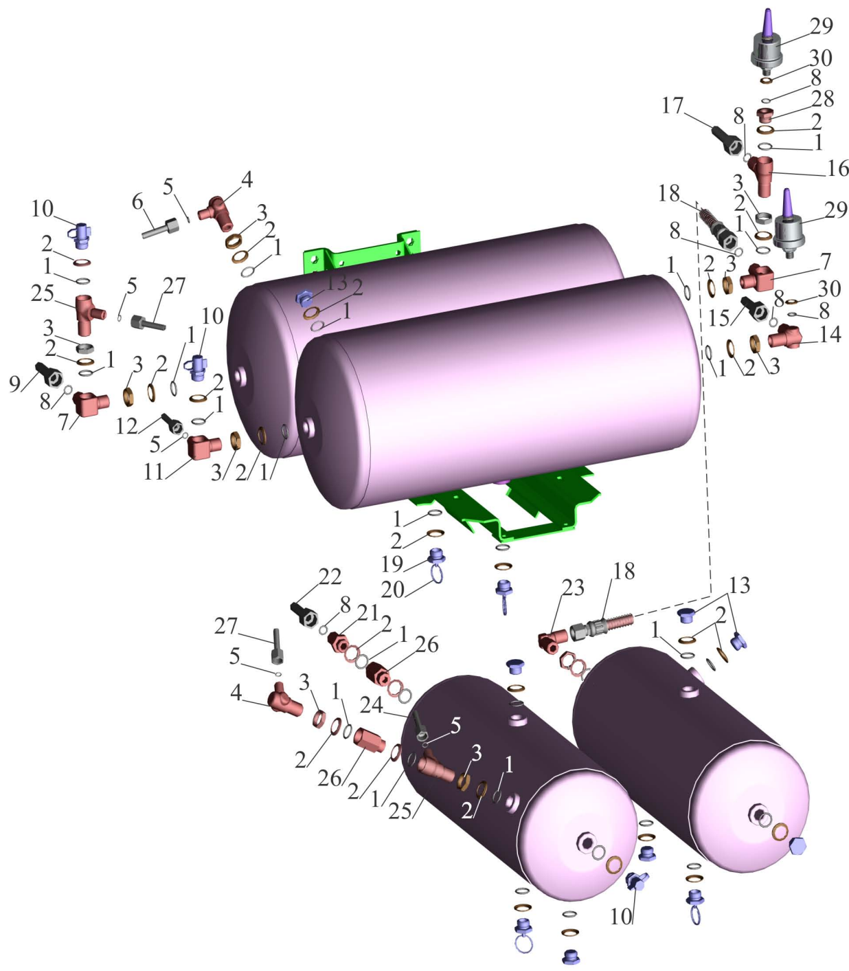
Рис.175 Установка присоединительной арматуры на ресиверах МАЗ-551605, 551603 Fig.175 Installation attach accessories on receivers MAZ-551605, 551603
