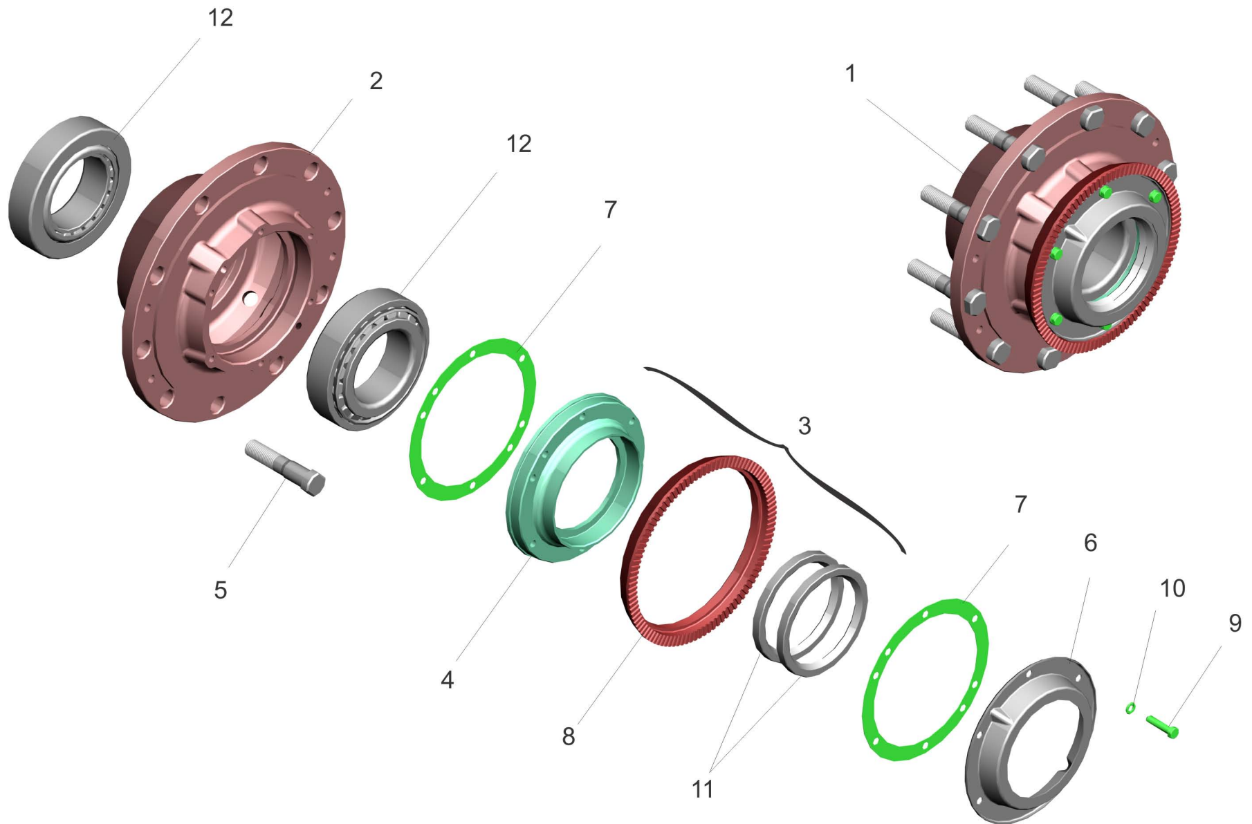
Рис.69 Ступица заднего моста. Fig.69 Rear axle hub.
