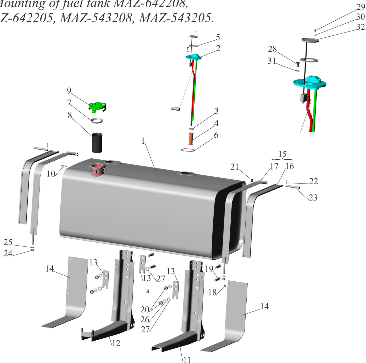
Рис.16 Крепление топливного бака МАЗ-642208, МАЗ-642205, МАЗ-543208, МАЗ-543205.
