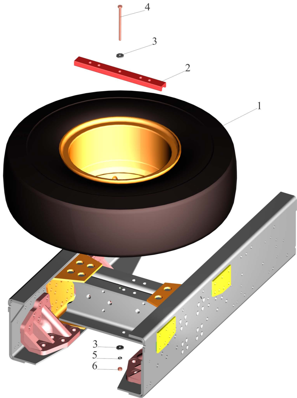
Рис.108 Установка запасного колеса МАЗ-551605 (5516-3100001-30). Fig.108 Installation spare wheel MAZ-551605 (5516-3100001-30).
