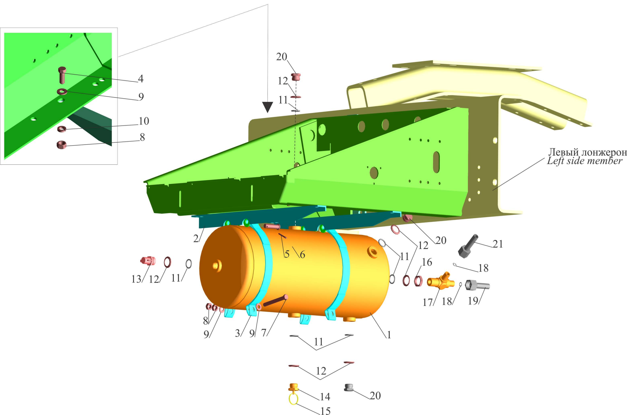
Рис.177 Установка ресивера и присоединительной арматуры МАЗ-555102 Fig.177 Installation of receiver and attach accessories MAZ-555102
