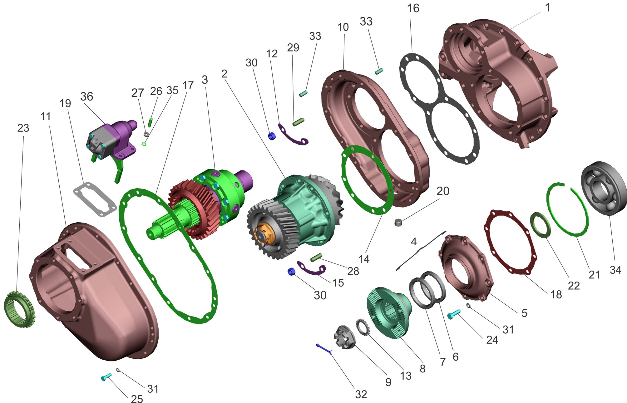
Рис.79 Редуктор среднего моста. Fig.79 Intermediate axle reduction gear
