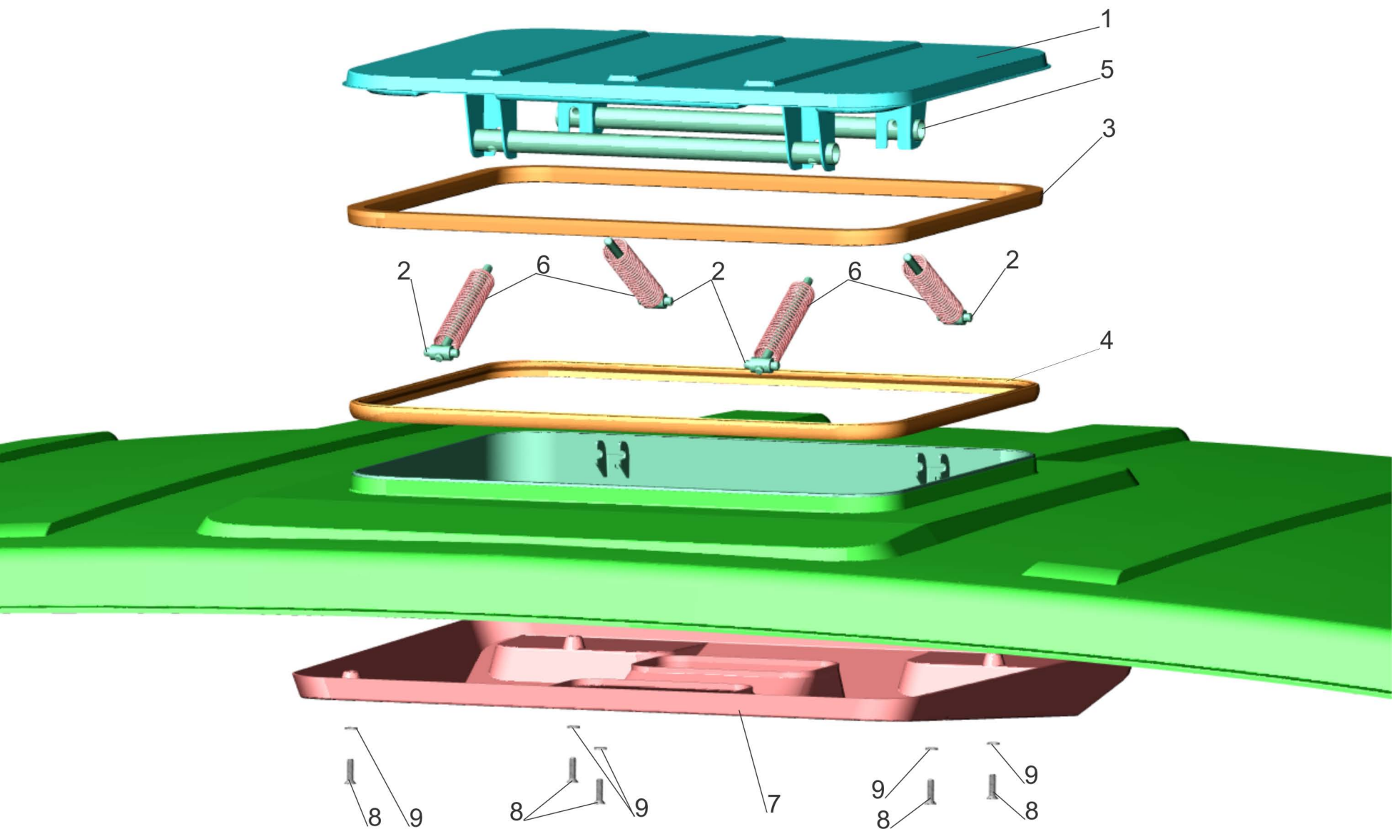
Рис.233 Установка крышки вентиляционного люка Fig.233 Installation vent hatch cover
