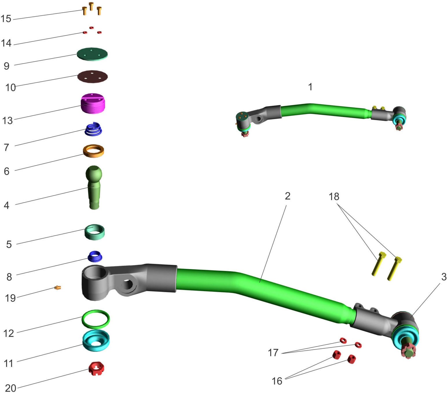
Рис.127 Тяга продольная Fig.127 Drag Rod.
