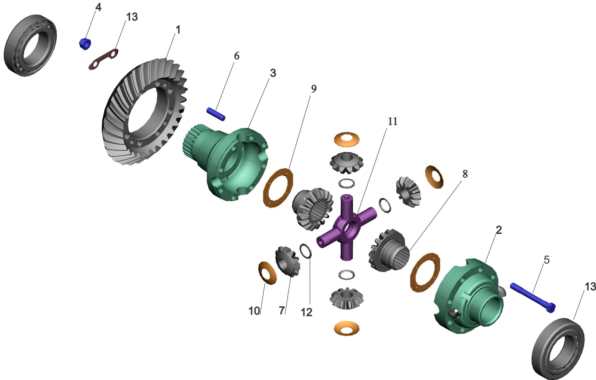
Рис.81 Редуктор среднего моста. Дифференциал Fig.81 Intermediate axle reduction gear.Differential
