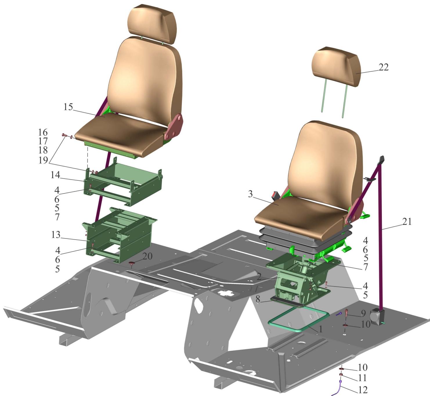
Рис.238 Установка и пневмопитание сидений 5551-6800006-040 Fig.238 Installation and pneumatic supply of seat 5551-6800006-040
