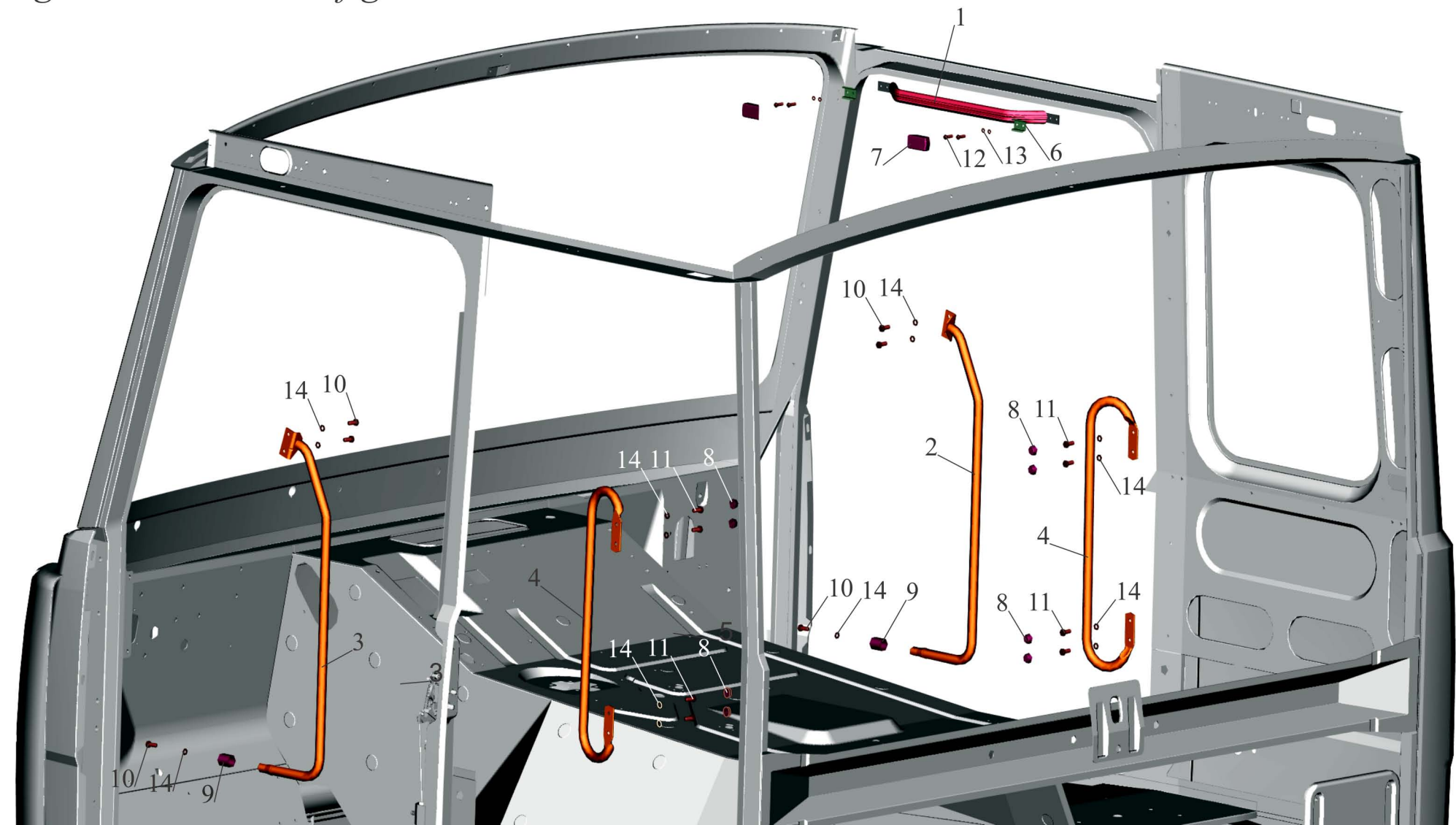
Рис.231 Установка поручней в кабине Fig 231 Installation of grab handles in cab
