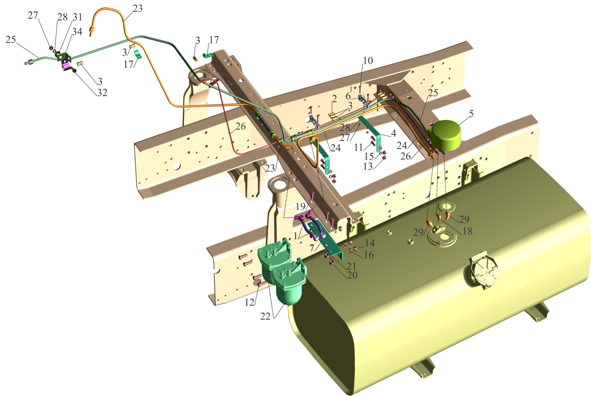
Рис. 19 Установка топливопроводов МАЗ-543208 (без подогревателя) Fig. 19 Installation of fuel lines MAZ-543208 (without heater)
