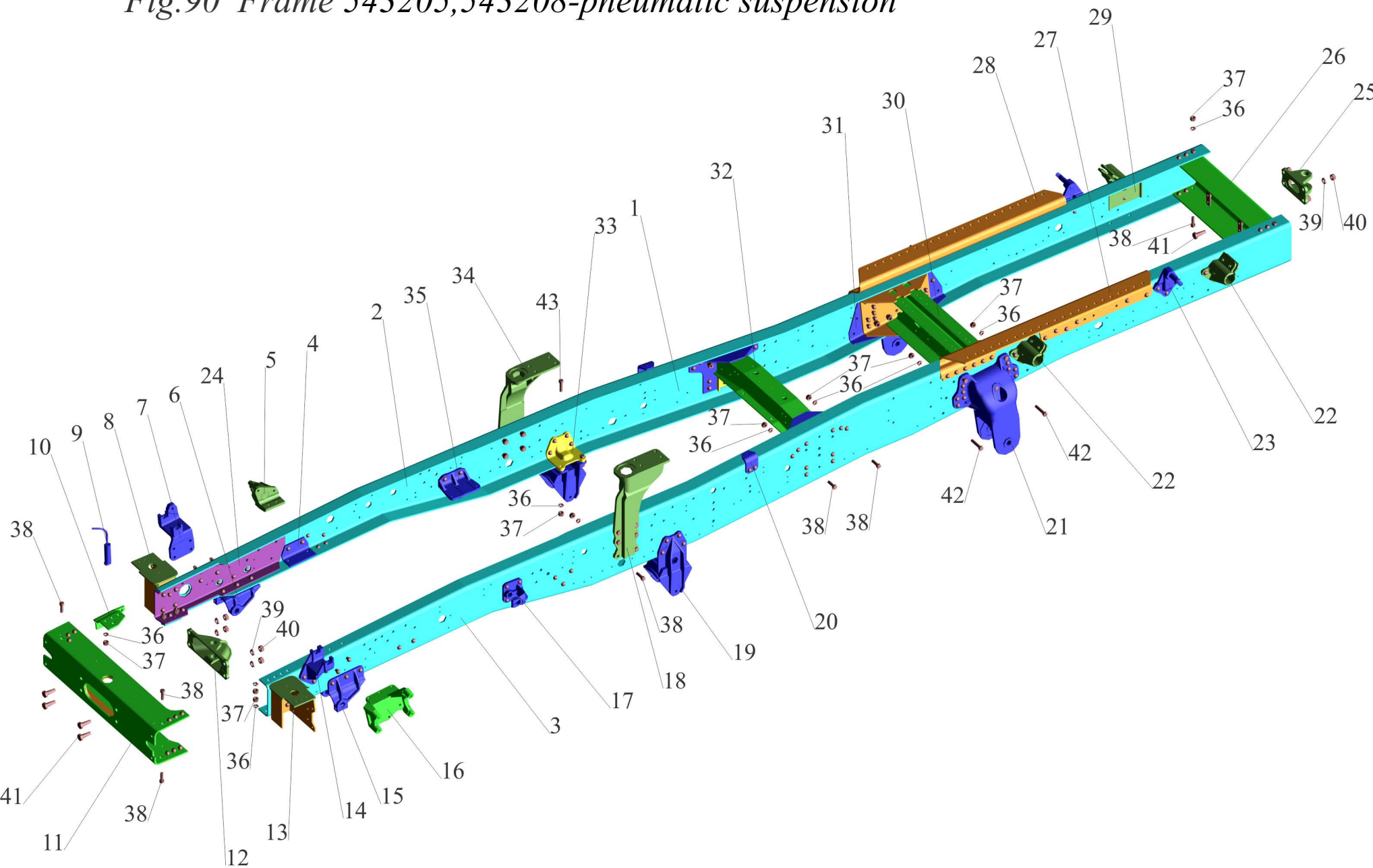
Рис.90 Рама 543205, 543208-пневмоподвеска
