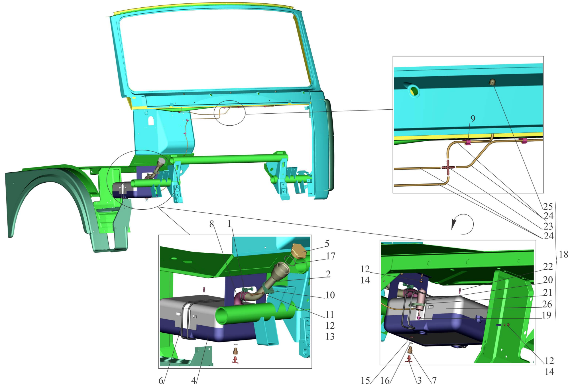
Рис. 227 Установка омывателя. Fig. 227 Installation of washer
