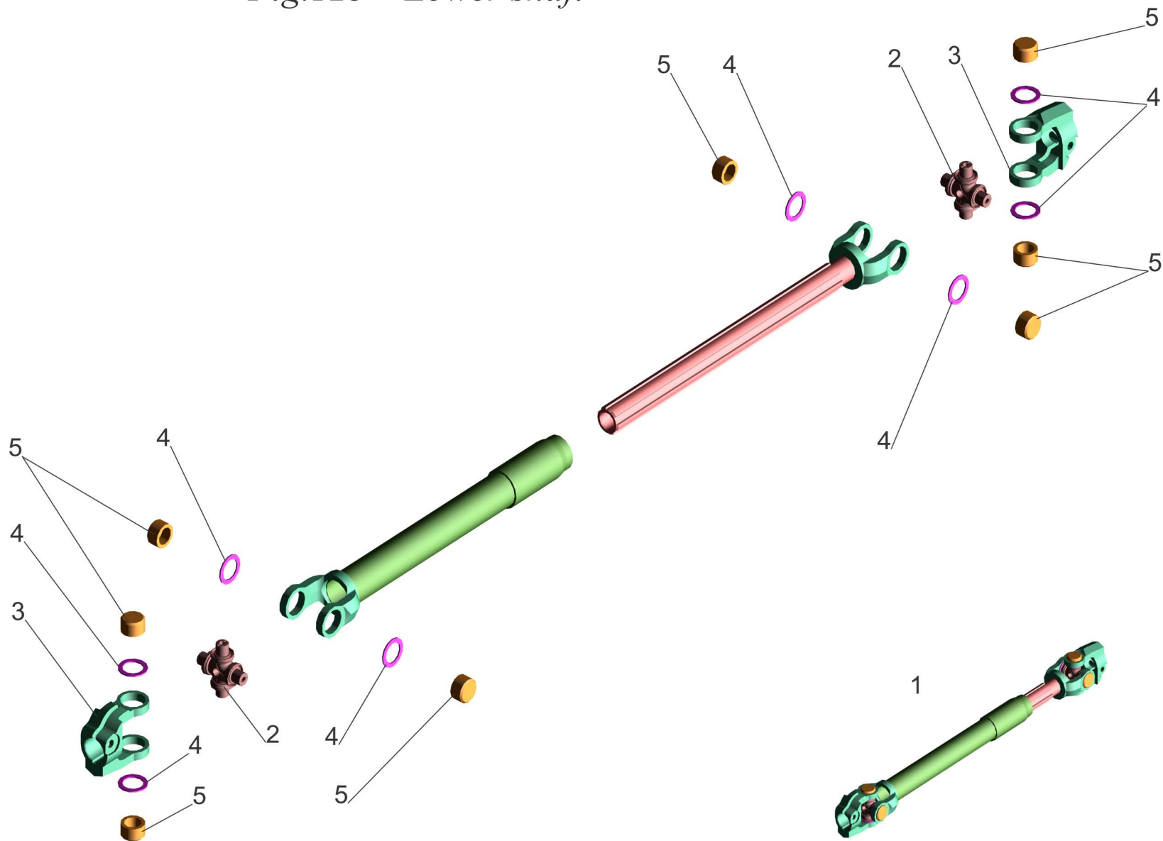
Рис.123 Вал нижний Fig.123 Lower shaft
